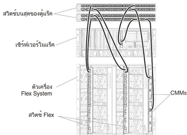
รูปภาพ 19. ตัวอย่างการเดินสายสำหรับเครือข่ายข้อมูลและเครือข่ายการจัดการที่แยกจากกันแบบเสมือนจริง
