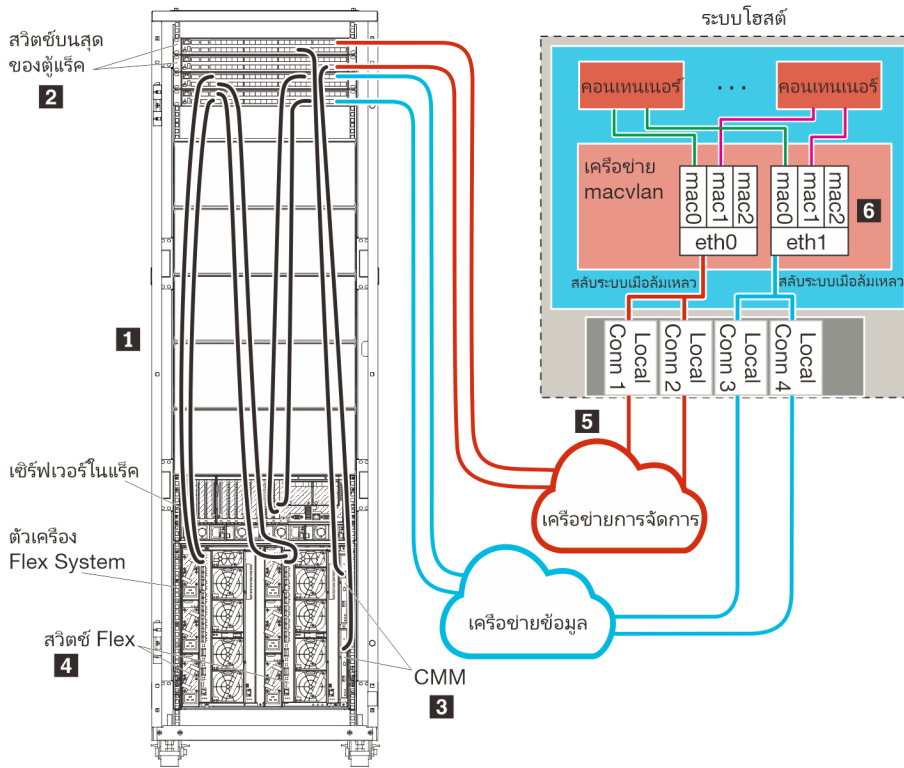
รูปภาพ 14. ตัวอย่างโทโพโลยีเครือข่ายข้อมูลและการจัดการที่แยกจากกันทางกายภาพสำหรับคอนเทนเนอร์
