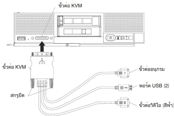
รูปภาพ 22. สายเคเบิลคอนโซลเบรกเอาท์และฝาครอบด้านหน้าของเซิร์ฟเวอร์
