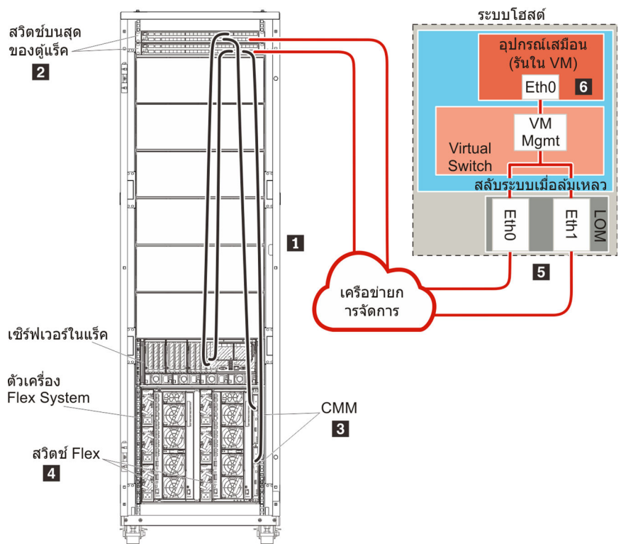
รูปภาพ 25. ตัวอย่างโทโพโลยีเครือข่ายการจัดการอย่างเดียวดำเนินการสำหรับอุปกรณ์เสมือน
