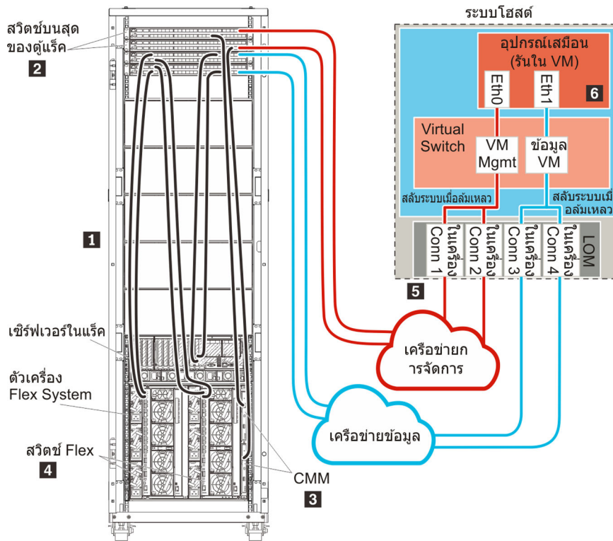
รูปภาพ 13. ตัวอย่างโทโพโลยีเครือข่ายข้อมูลและการจัดการที่แยกจากกันทางกายภาพสำหรับอุปกรณ์เสมือน
