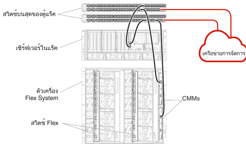
รูปภาพ 27. ตัวอย่างการเดินสายสำหรับเครือข่ายการจัดการอย่างเดียว
