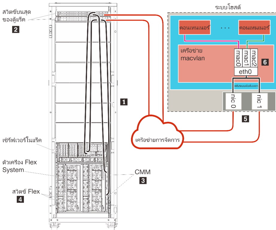
รูปภาพ 26. ตัวอย่างโทโพโลยีเครือข่ายการจัดการอย่างเดียวนำสำหรับคอนเทนเนอร์
