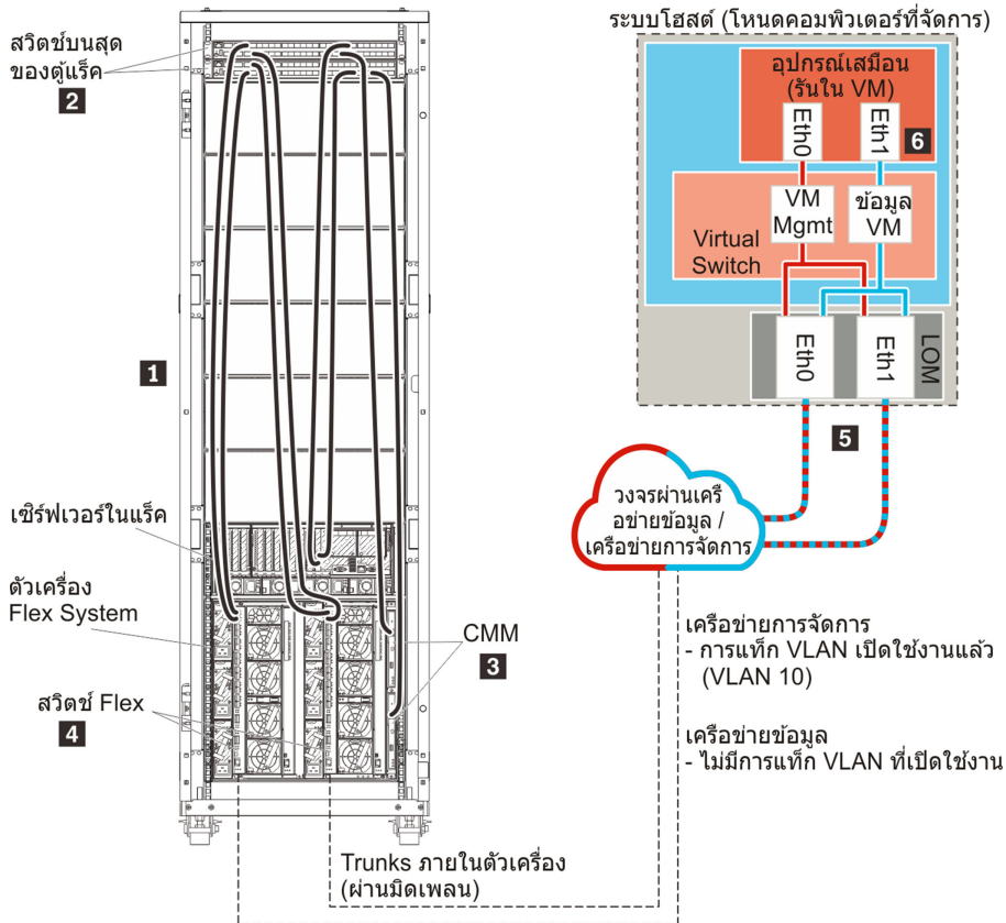
รูปภาพ 17. ตัวอย่างโทโพโลยีเครือข่ายข้อมูลและการจัดการที่แยกจากกันแบบเสมือนสำหรับอุปกรณ์เสมือน
