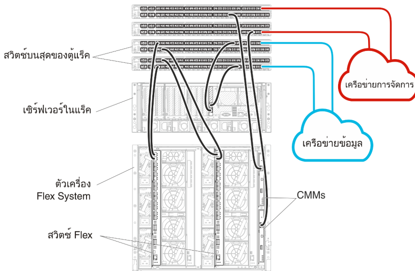
รูปภาพ 15. ตัวอย่างการเดินสายสำหรับเครือข่ายข้อมูลและเครือข่ายการจัดการที่แยกจากกันทางกายภาพ
