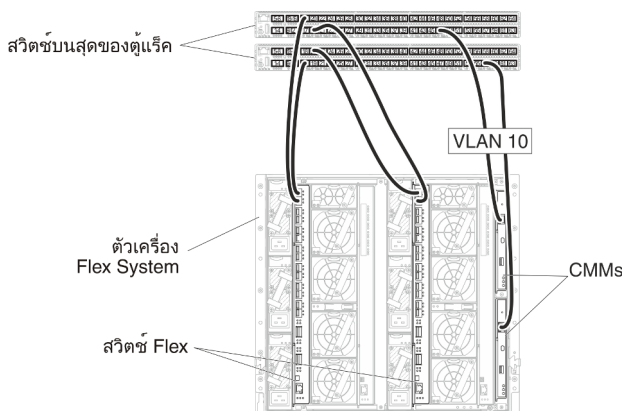
รูปภาพ 21. ตัวอย่างการกำหนดค่าสำหรับ สวิตช์ Flex ในเครือข่ายข้อมูลและเครือข่ายการจัดการที่แยกจากกันแบบเสมือนจริง (VMware ESXi) ที่เปิดใช้งานการแท็ก VLAN ในเครือข่ายการจัดการ
