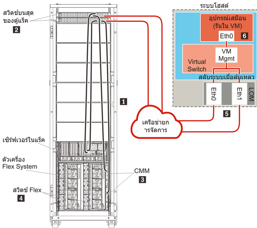
รูปภาพ 23. ตัวอย่างโทโพโลยีเครือข่ายการจัดการอย่างเดียวนำสำหรับอุปกรณ์เสมือน
