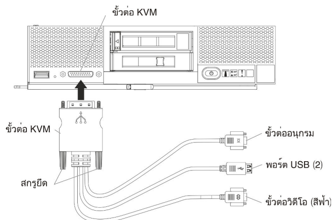
รูปภาพ 21. สายเคเบิลคอนโซลเบรกเอาท์และฝาครอบด้านหน้าของเซิร์ฟเวอร์
