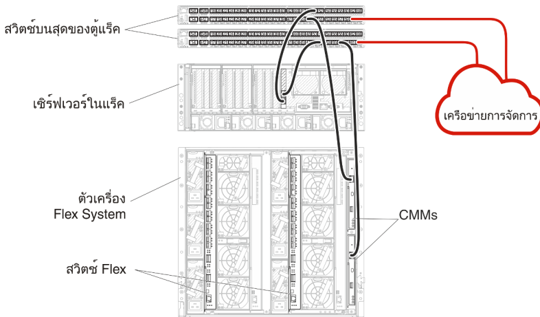
รูปภาพ 25. ตัวอย่างการเดินสายสำหรับเครือข่ายการจัดการอย่างเดียว
