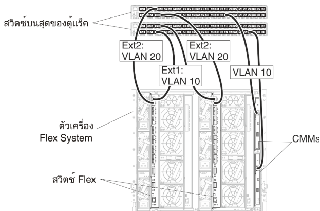
รูปภาพ 20. ตัวอย่างการกำหนดค่าสำหรับ สวิตช์ Flex ในเครือข่ายข้อมูลและเครือข่ายการจัดการที่แยกจากกันแบบเสมือนจริง (VMware ESXi) ที่เปิดใช้งานการแท็ก VLAN ในทั้งสองเครือข่าย
