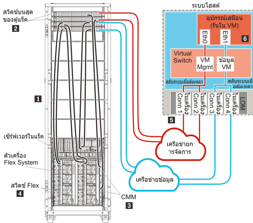
รูปภาพ 12. ตัวอย่างโทโพโลยีเครือข่ายข้อมูลและการจัดการที่แยกจากกันทางกายภาพสำหรับอุปกรณ์เสมือน
