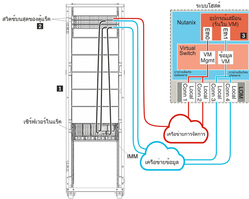
รูปภาพ 10. ตัวอย่างโทโพโลยีเครือข่าย - เครือข่ายข้อมูลและเครือข่ายการจัดการที่แยกจากกันทางกายภาพ (Nutanix AHV)
