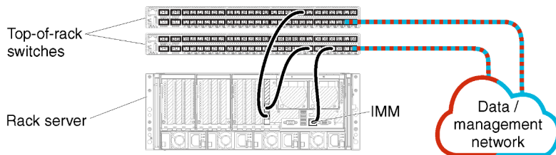
รูปภาพ 9. ตัวอย่างการเดินสายสำหรับเครือข่ายข้อมูลและเครือข่ายการจัดการเดี่ยว
