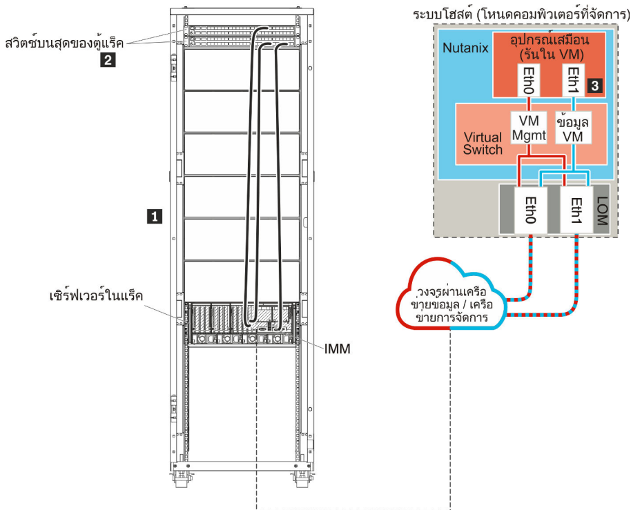
รูปภาพ 12. ตัวอย่างโทโพโลยีเครือข่าย - เครือข่ายข้อมูลและเครือข่ายการจัดการที่แยกจากกันแบบเสมือนจริง (Nutanix AHV)
