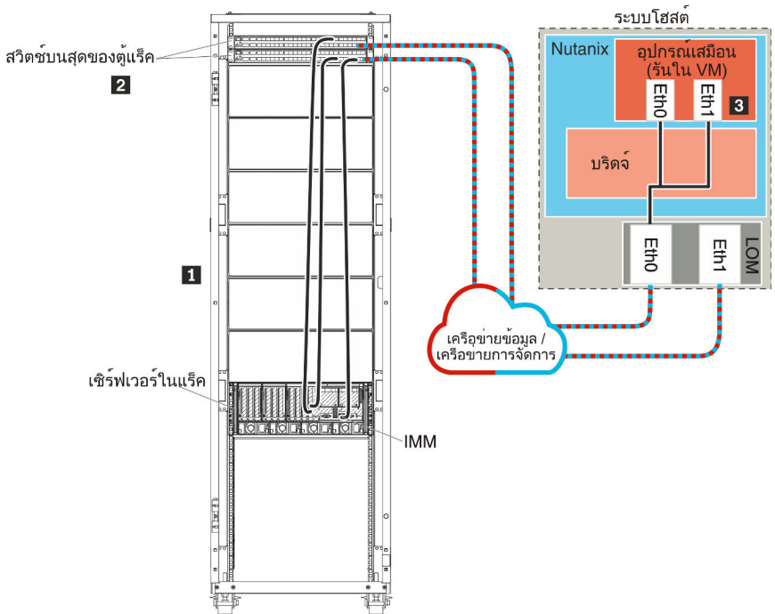
รูปภาพ 8. ตัวอย่างโทโพโลยีเครือข่ายข้อมูลและเครือข่ายการจัดการเดียว (Nutanix AHV)
