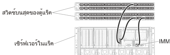
รูปภาพ 13. ตัวอย่างการเดินสายสำหรับเครือข่ายข้อมูลและเครือข่ายการจัดการที่แยกจากกันแบบเสมือนจริง
