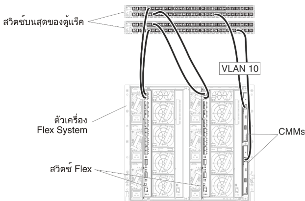
รูปภาพ 14. ตัวอย่างการกำหนดค่าสำหรับ สวิตช์ Flex ในเครือข่ายข้อมูลและเครือข่ายการจัดการที่แยกจากกันแบบเสมือนจริง (KVM) ที่เปิดใช้งานการแท็ก VLAN ในเครือข่ายการจัดการ
