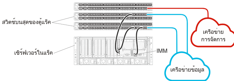
รูปภาพ 11. ตัวอย่างการเดินสายสำหรับเครือข่ายข้อมูลและเครือข่ายการจัดการที่แยกจากกันทางกายภาพ (VMware ESXi)
