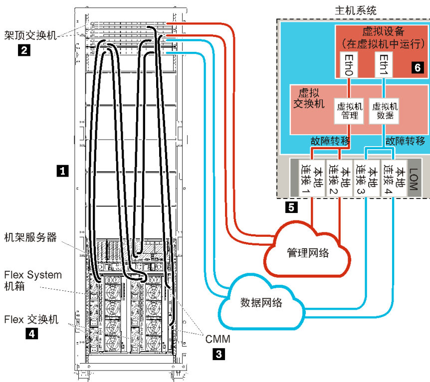
图 12. 虚拟设备物理隔离的数据和管理网络拓扑示例
