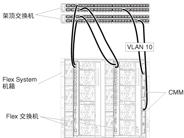
图 20. 在管理网络上启用 VLAN 标记的虚拟隔离的数据和管理网络上 Flex 交换机的示例配置
