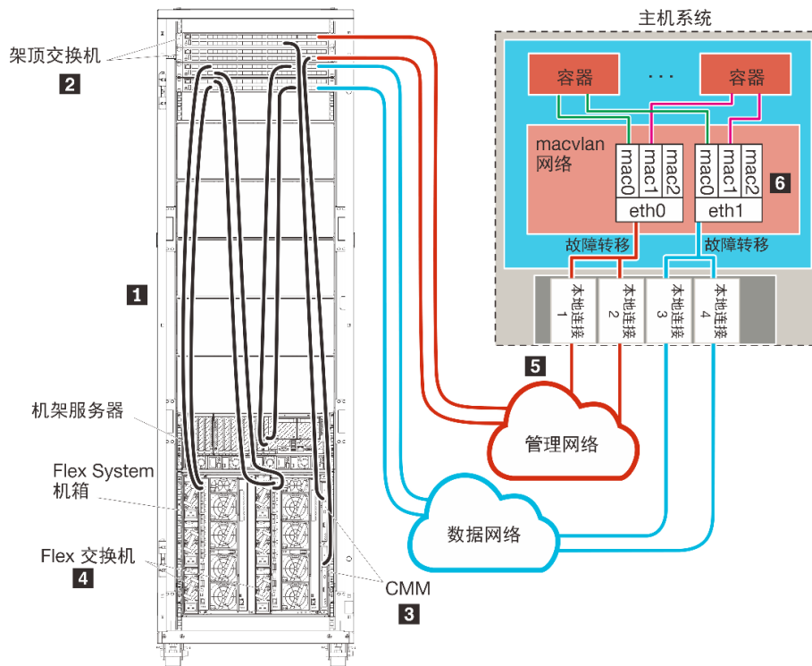
图 14. 容器物理隔离的数据和管理网络拓扑示例
