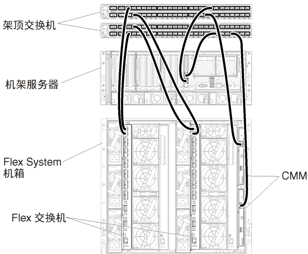
图 19. 虚拟隔离的数据和管理网络的示例线缆连接
