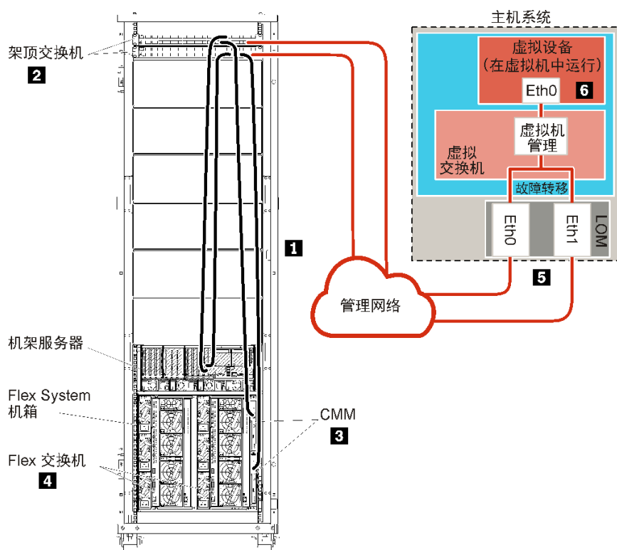
图 25. 虚拟设备仅限于管理的网络拓扑示例
