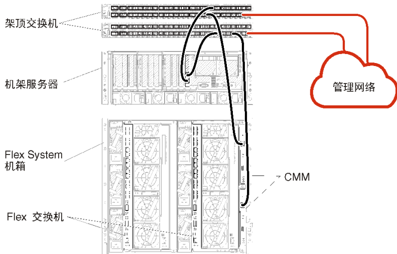
图 27. 仅限于管理的网络的示例线缆连接
