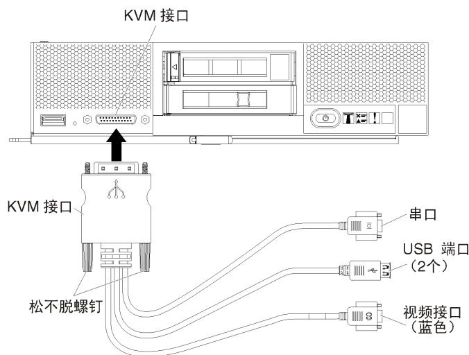
图 22. 控制台分支线缆和服务器的前挡板
