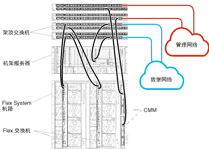
图 15. 物理隔离的数据和管理网络的示例线缆连接
