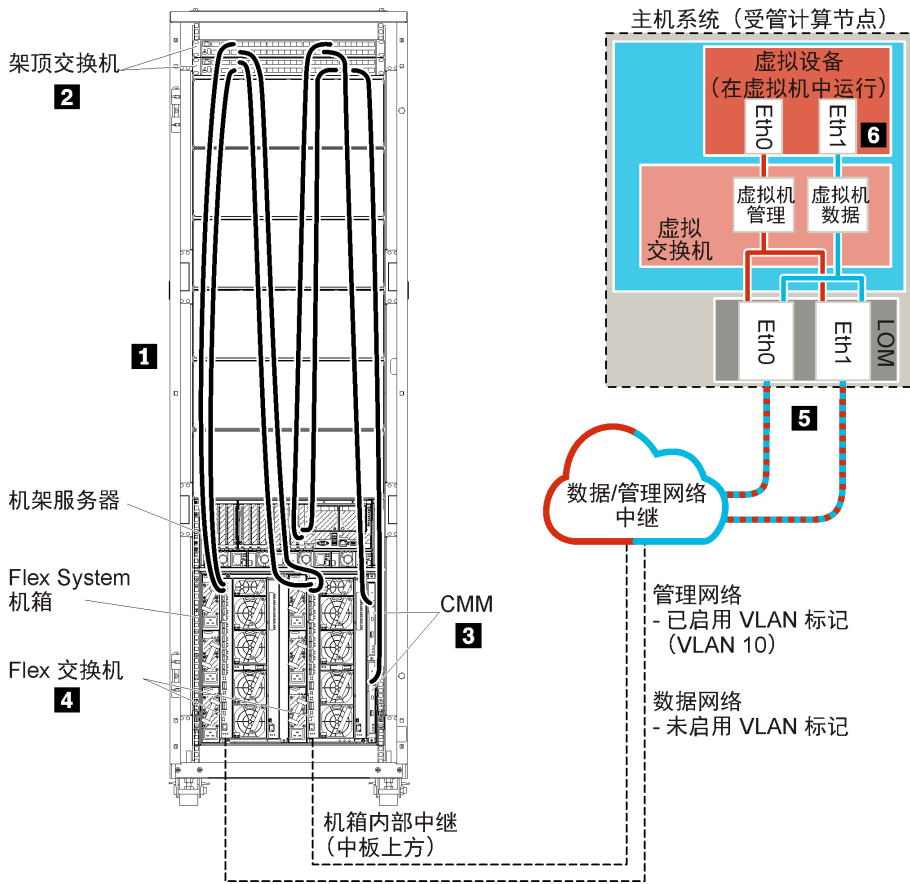
图 17. 虚拟设备的虚拟隔离的数据和管理网络拓扑示例
