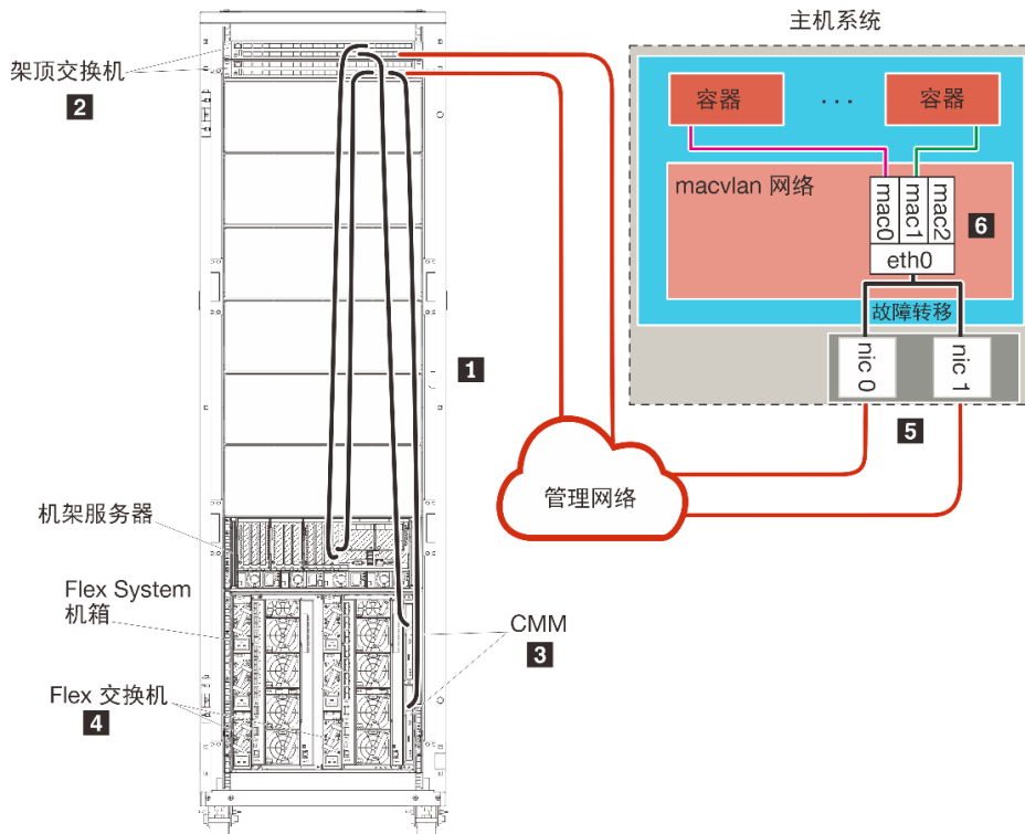
图 26. 容器仅限于管理的网络拓扑示例
