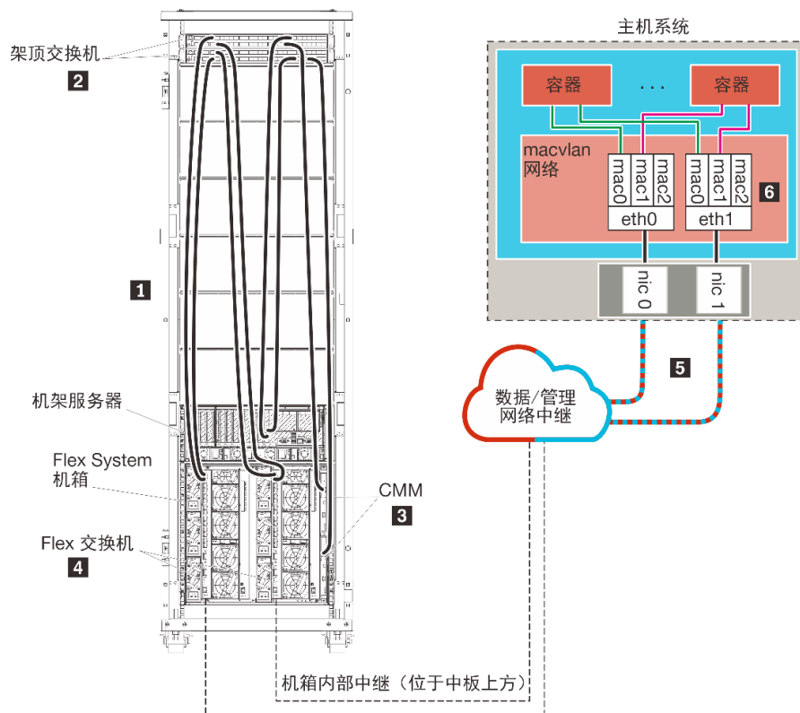
图 18. 容器的虚拟隔离的数据和管理网络拓扑示例
