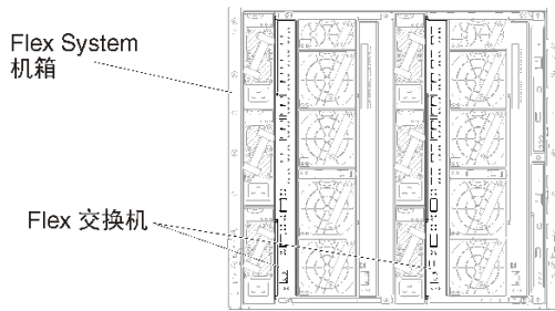
图 16. 机箱中的 Flex 交换机位置
