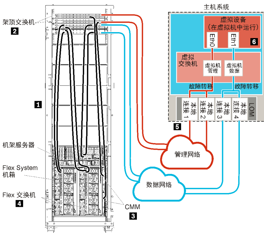
图 13. 虚拟设备物理隔离的数据和管理网络拓扑示例
