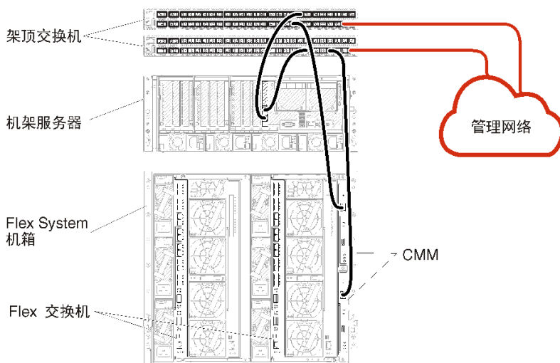
图 25. 仅限于管理的网络的示例线缆连接
