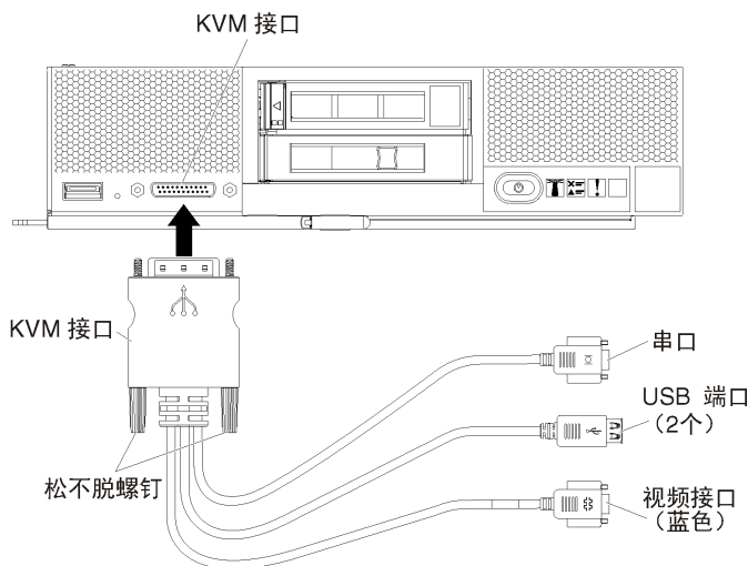
图 21. 控制台分支线缆和服务器的前挡板
