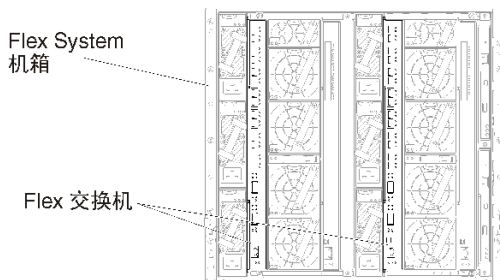
图 26. 机箱中的 Flex 交换机位置
