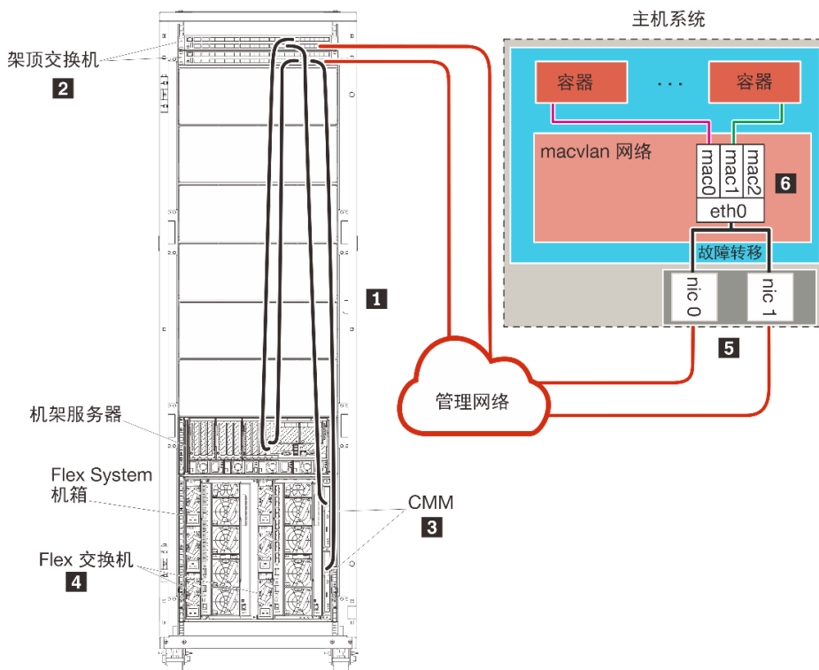
图 24. 容器仅限于管理的网络拓扑示例
