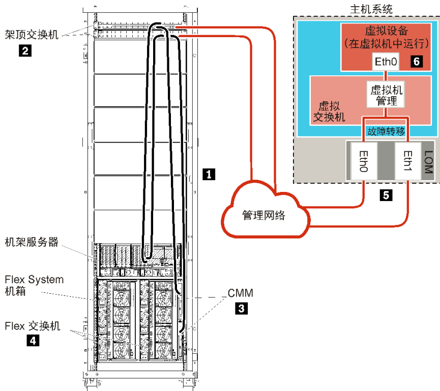
图 23. 虚拟设备仅限于管理的网络拓扑示例
