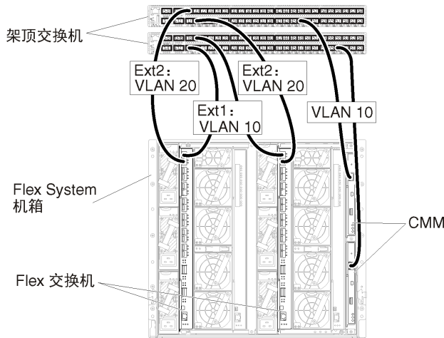
图 20. 在两个网络上均启用了 VLAN 标记的虚拟隔离的数据和管理网络 (VMware ESXi) 上 Flex 交换机的示例配置
