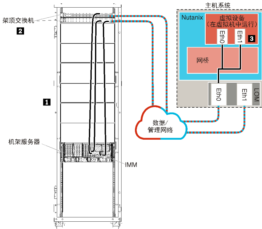
图 8. 示例单一数据和管理网络拓扑 (Nutanix AHV)
