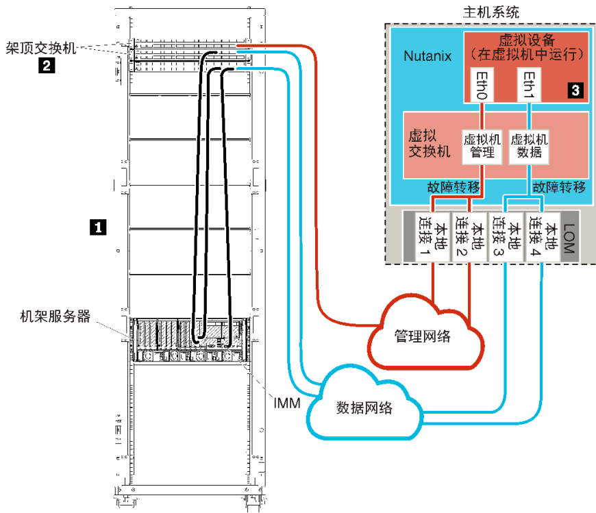
图 10. 示例网络拓扑 - 物理隔离的数据和管理网络 (Nutanix AHV)
