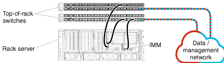
图 9. 单一数据和管理网络的示例线缆连接
