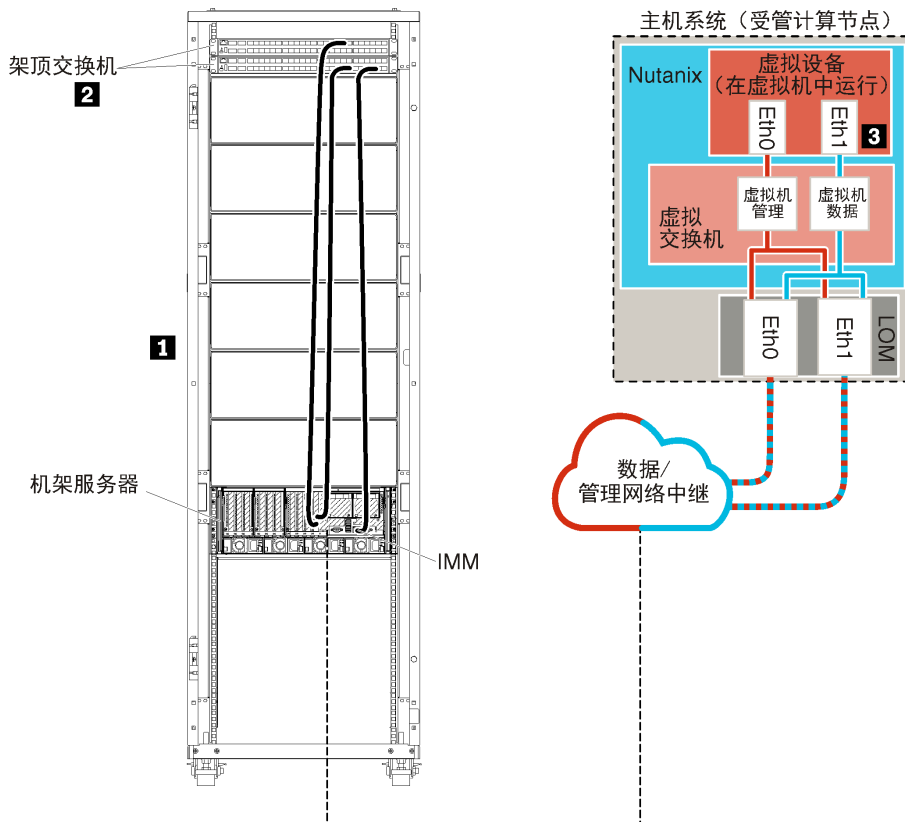
图 12. 示例网络拓扑 - 虚拟隔离的数据和管理网络 (Nutanix AHV)
