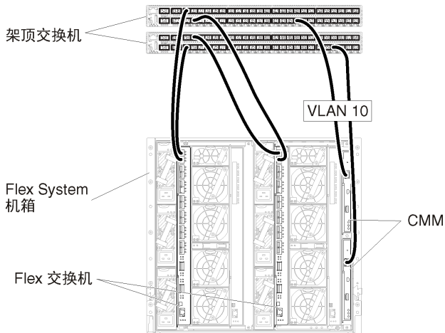
图 14. 在管理网络上启用 VLAN 标记的虚拟隔离数据和管理网络 (KVM) 上 Flex 交换机的示例配置
