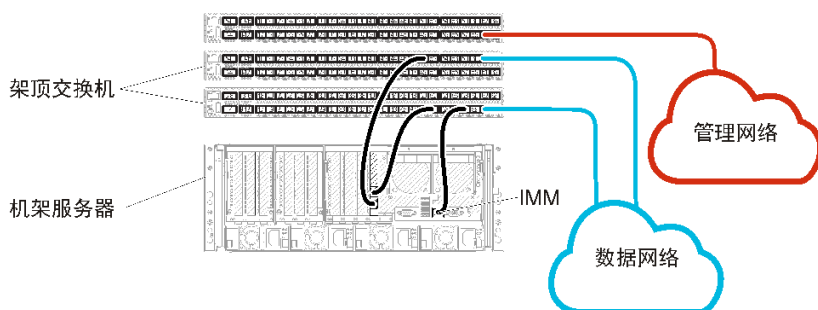
图 11. 物理隔离的数据和管理网络的示例线缆连接 (VMware ESXi)
