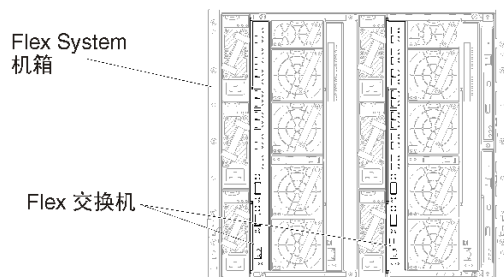
图 15. 机箱中的 Flex 交换机位置
