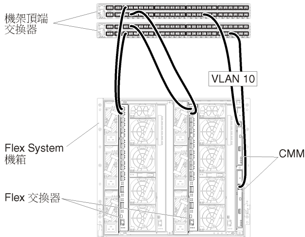
圖例 20. 虛擬分離資料和管理網路上的 Flex 交換器 範例配置，其中 VLAN 標記是在管理網路上啟用
