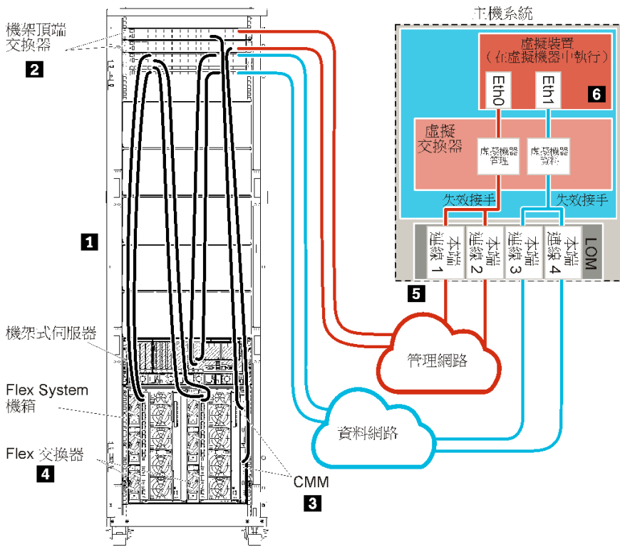
圖例 12. 虛擬裝置的實體分離資料和管理網路拓撲範例
