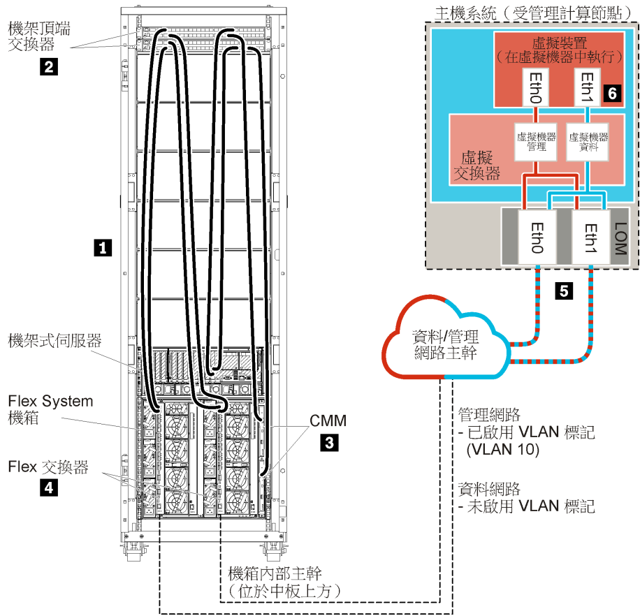
圖例 17. 虛擬裝置的虛擬分離資料和管理網路拓撲範例
