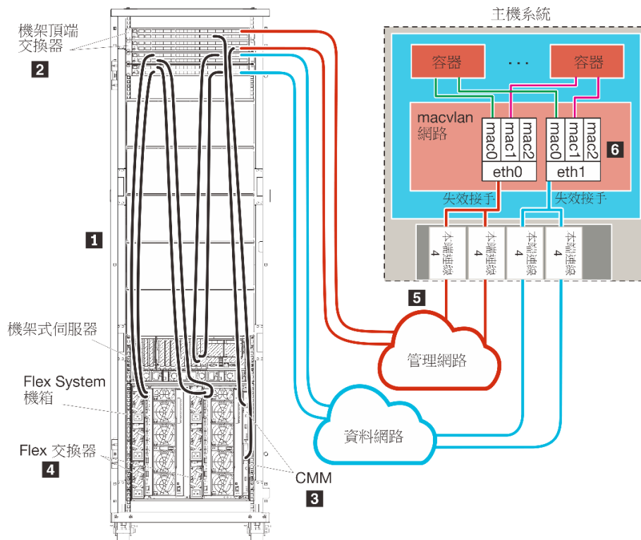
圖例 14. 容器的實體分離資料和管理網路拓撲範例
