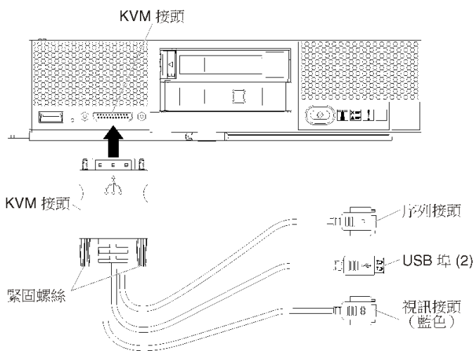
圖例 22. 伺服器的主控台分支纜線和前方擋板
