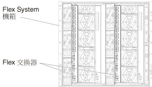
圖例 28. Flex 交換器 在機箱中的位置
