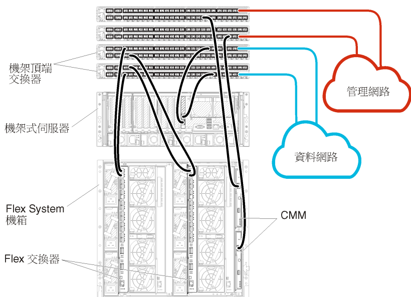
圖例 15. 實體分離資料和管理網路的纜線佈線範例
