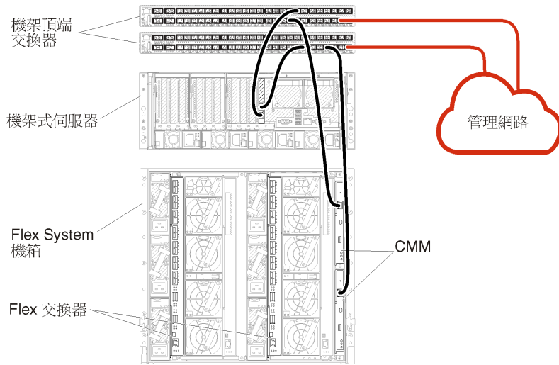
圖例 27. 管理專用網路的纜線連接範例
