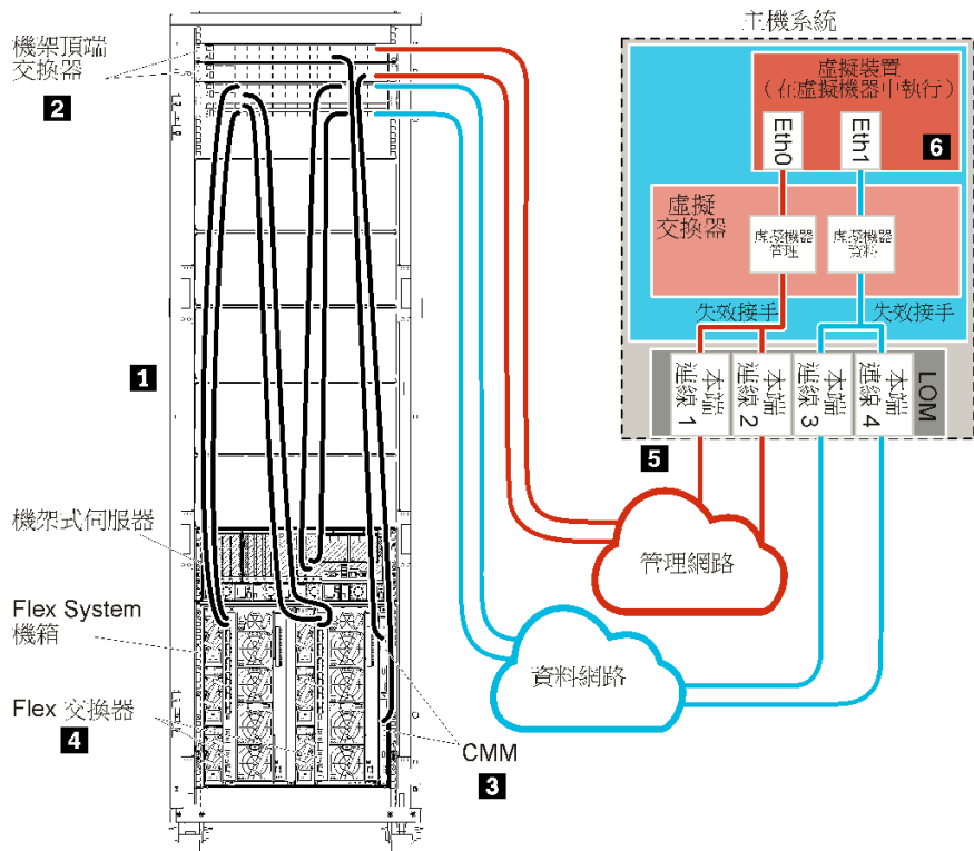
圖例 13. 虛擬裝置的實體分離資料和管理網路拓撲範例
