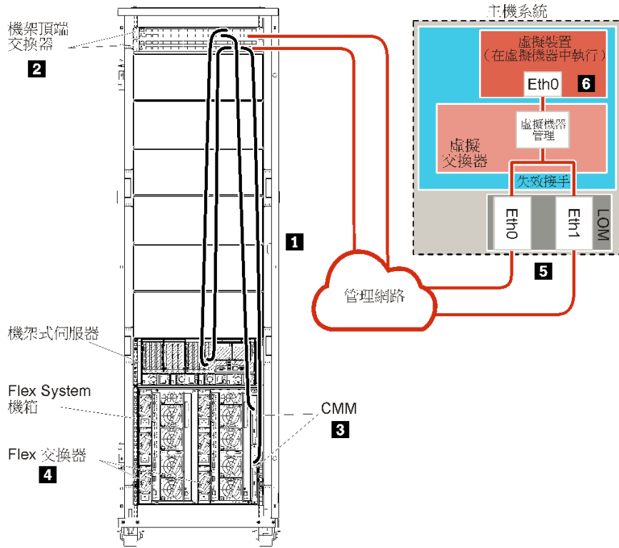
圖例 25. 虛擬裝置的管理專用網路拓撲範例
