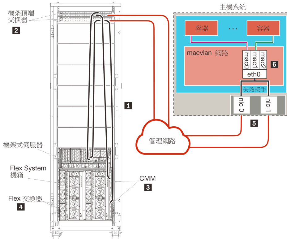
圖例 26. 容器的管理專用網路拓撲範例
