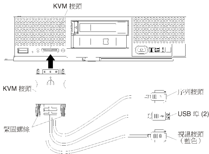
圖例 21. 伺服器的主控台分支纜線和前方擋板
