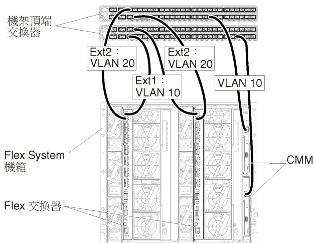
圖例 20. 虛擬分離資料和管理網路 (VMware ESXi) 上的 Flex 交換器 範例配置，其中 VLAN 標記會在這兩種網路上啟用
