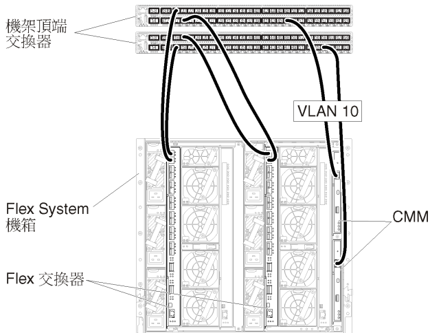
圖例 14. 虛擬分離資料和管理網路 (KVM) 上的 Flex 交換器 範例配置，其中 VLAN 標記是在管理網路上啟用
