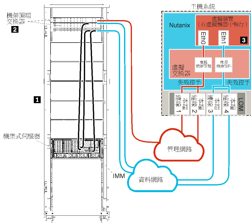
圖例 10. 範例網路拓撲 - 實體分離資料和管理網路 (Nutanix AHV)
