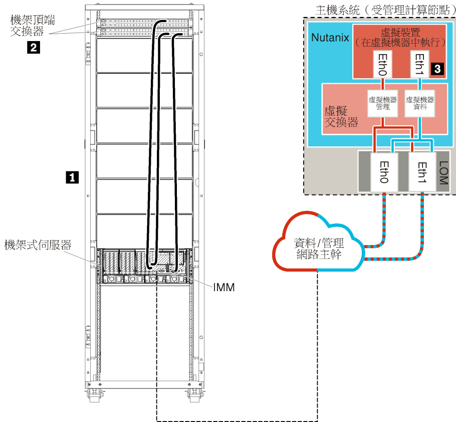
圖例 12. 範例網路拓撲 - 虛擬分離資料和管理網路 (Nutanix AHV)
