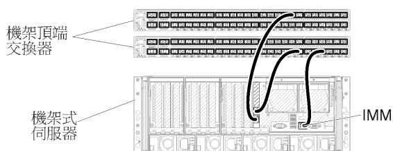
圖例 13. 虛擬分離資料和管理網路的纜線佈線範例
