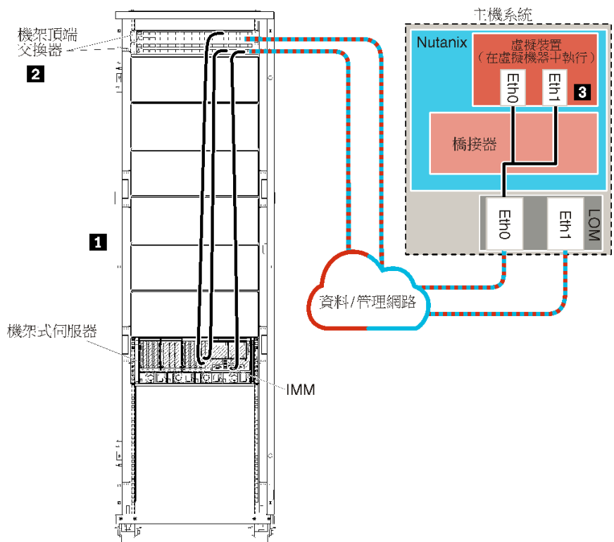
圖例 8. 單一資料和管理網路拓撲範例 (Nutanix AHV)
