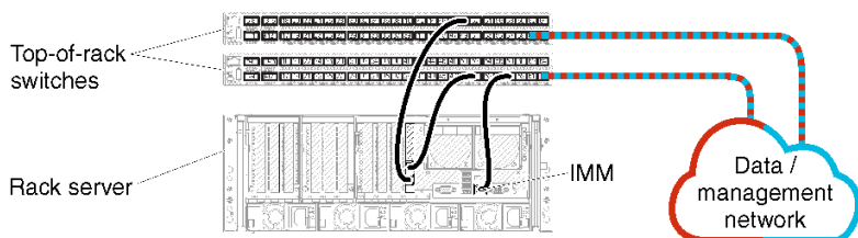
圖例 9. 單一資料和管理網路的纜線佈線範例
