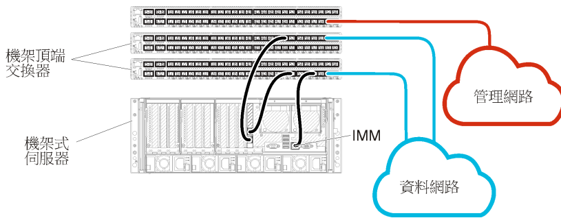
圖例 11. 實體分離資料和管理網路的纜線佈線範例 (VMware ESXi)
