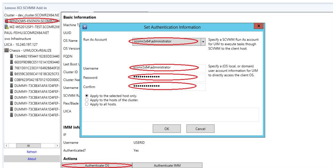
Abbildung 4. Hostauthentifizierung einrichten
