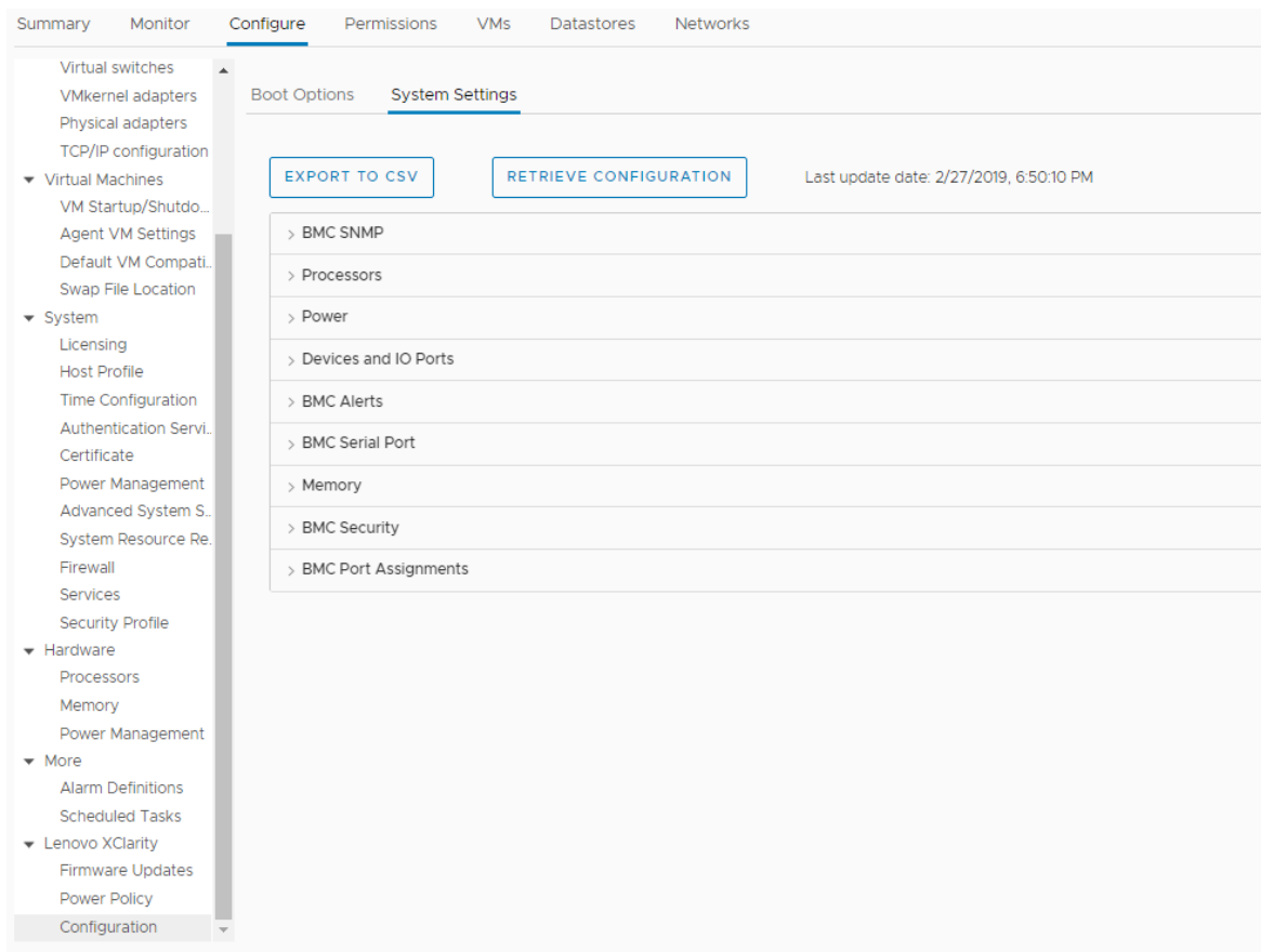
Abbildung 11. Bereich Systemeinstellungen
