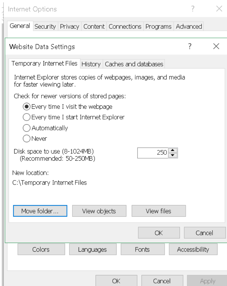
Abbildung 12. Internet Explorer-Einstellungen
