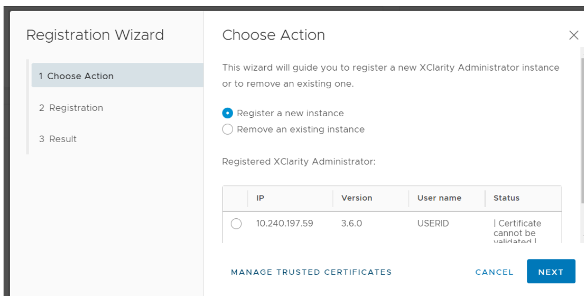
Abbildung 2. Seite „Registrierungsassistent“
