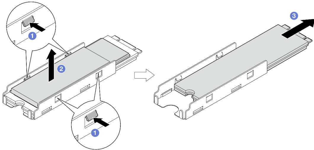
Abbildung 49. Entfernen des M.2-Kühlkörpers
