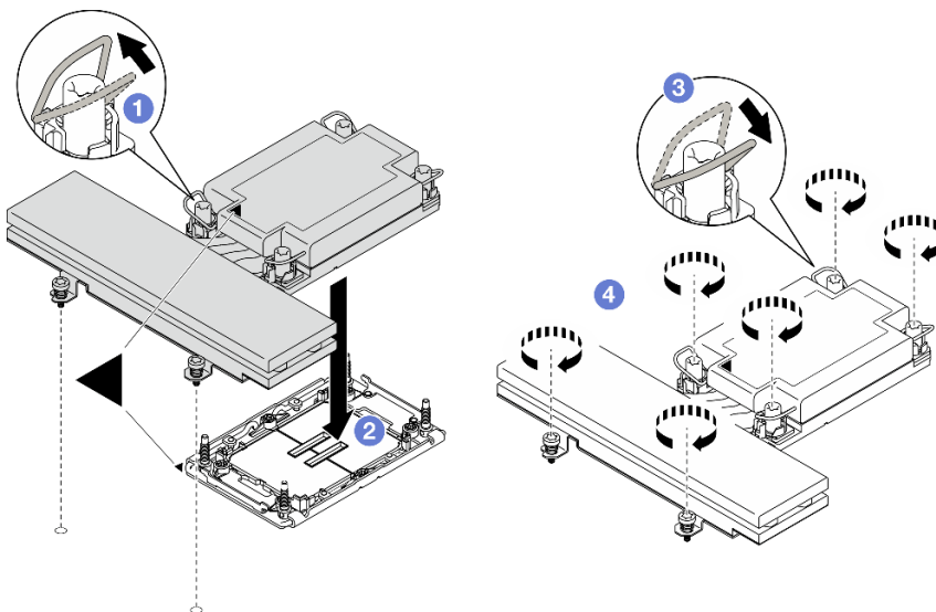
Abbildung 99. Installation des Hochleistungs-PHM
