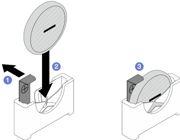
Abbildung 30. Installieren einer CMOS-Batterie
