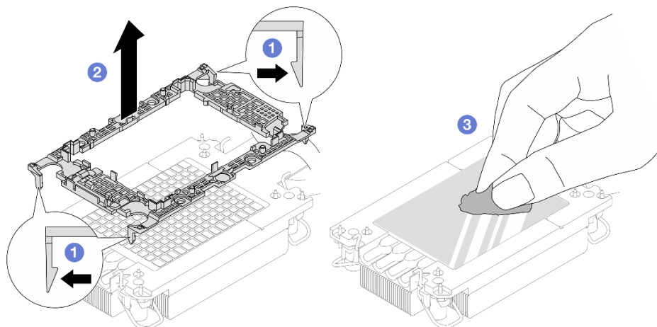
Abbildung 92. Trennen eines Prozessorträgers vom Kühlkörper
