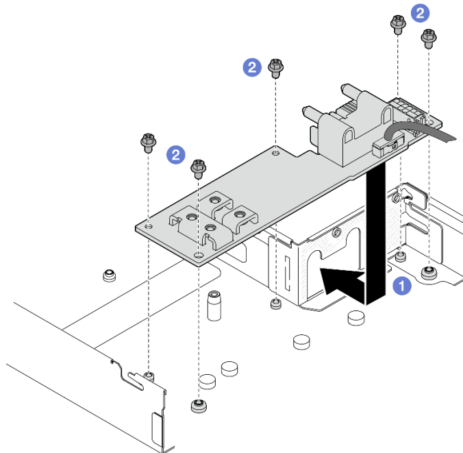
Abbildung 87. Installation einer Stromversorgungsplatine
