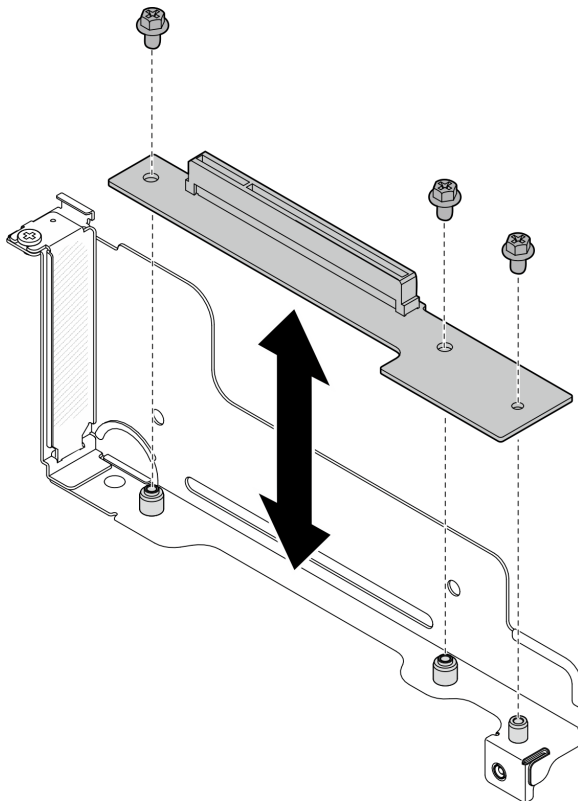
Abbildung 78. Austausch der PCIe-Adapterkarte
