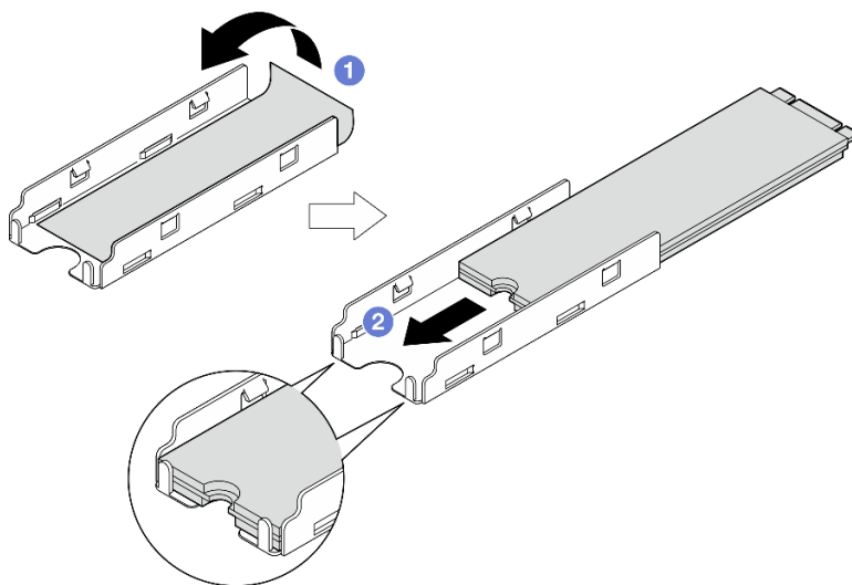
Abbildung 60. Installieren des Wärmepads und des M.2-Laufwerks im Einbaurahmen
