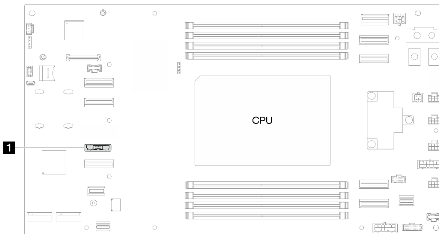
Abbildung 29. Position des CMOS-Batteriesockels
