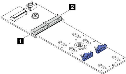
Abbildung 63. M.2-Laufwerksteckplätze
