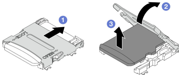
Abbildung 70. Entfernen der microSD-Karte
