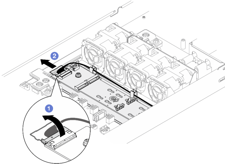
Abbildung 51. Abziehen des Kabels vom M.2-Bootadapter
