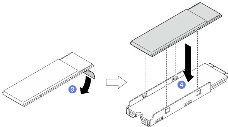
Abbildung 61. Installieren eines M.2-Kühlkörpers im M.2-Einbaurahmen
