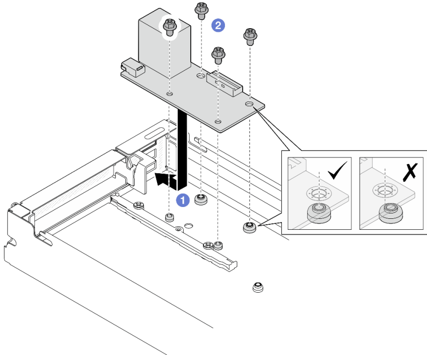
Abbildung 101. Installation des E/A-Moduls an der Rückseite
