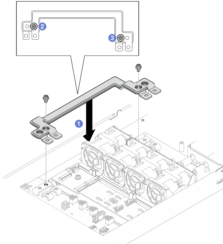
Abbildung 84. Installation der Sammelschiene
