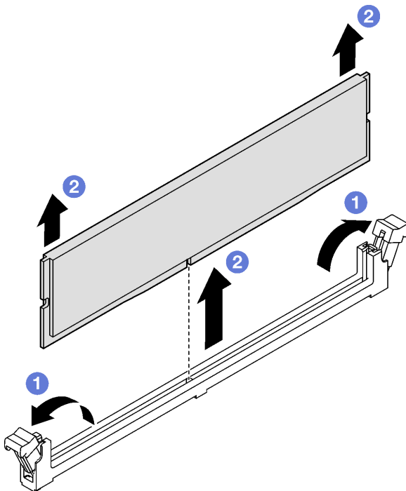
Abbildung 66. Entfernen eines Speichermoduls
