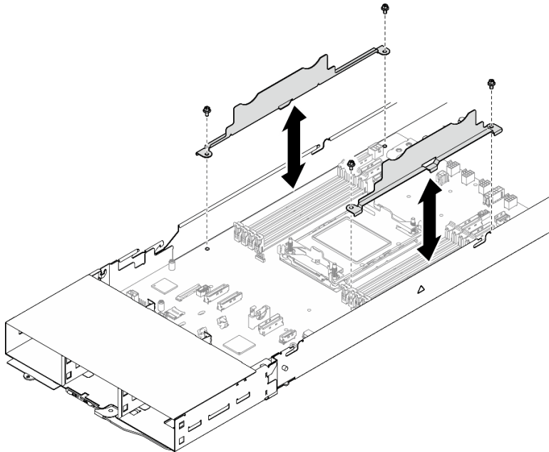
Abbildung 106. Entfernen der Kabelwand
