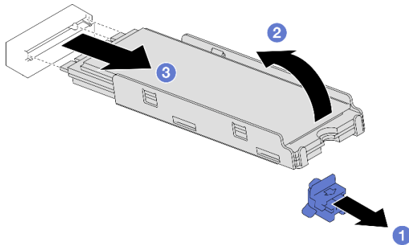
Abbildung 48. Entfernen eines M.2-Laufwerks
