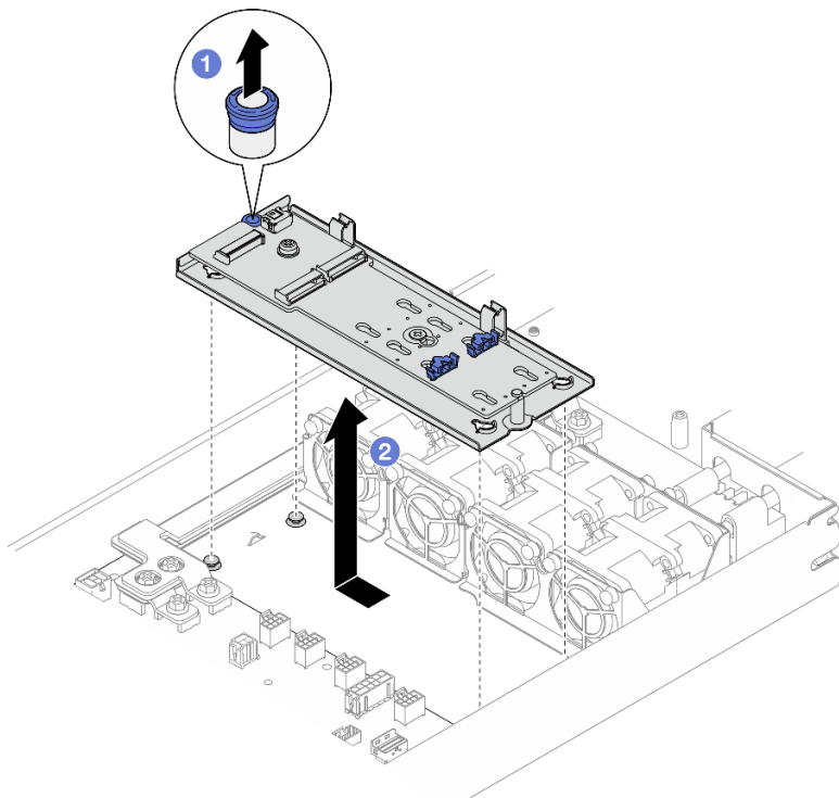
Abbildung 52. Entfernen des M.2-Bootadapterrahmens
