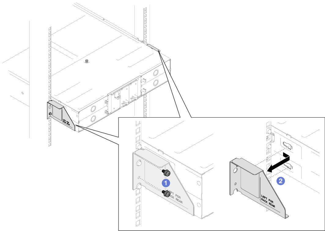
Abbildung 2. Entfernen von Transporthalterungen für 29 Zoll oder 28,31 Zoll tiefe Racks
