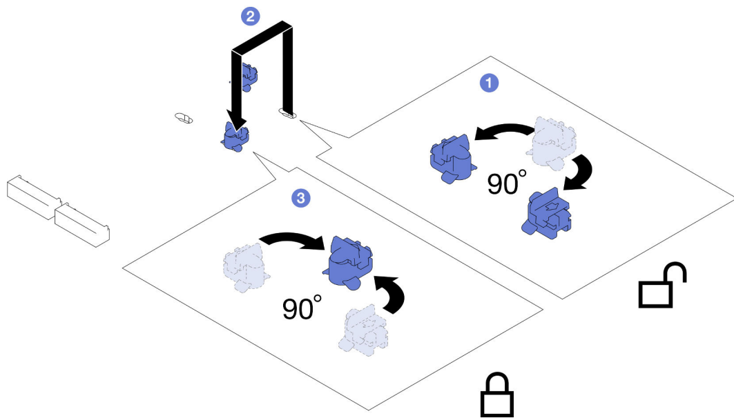
Abbildung 57. Anpassung einer M.2-Laufwerkhalterung
