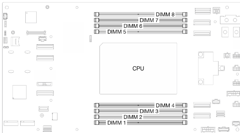
Abbildung 67. Layout für Speichermodule und Prozessoren
