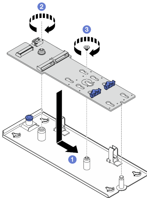
Abbildung 54. Installieren des M.2-Bootadapters
