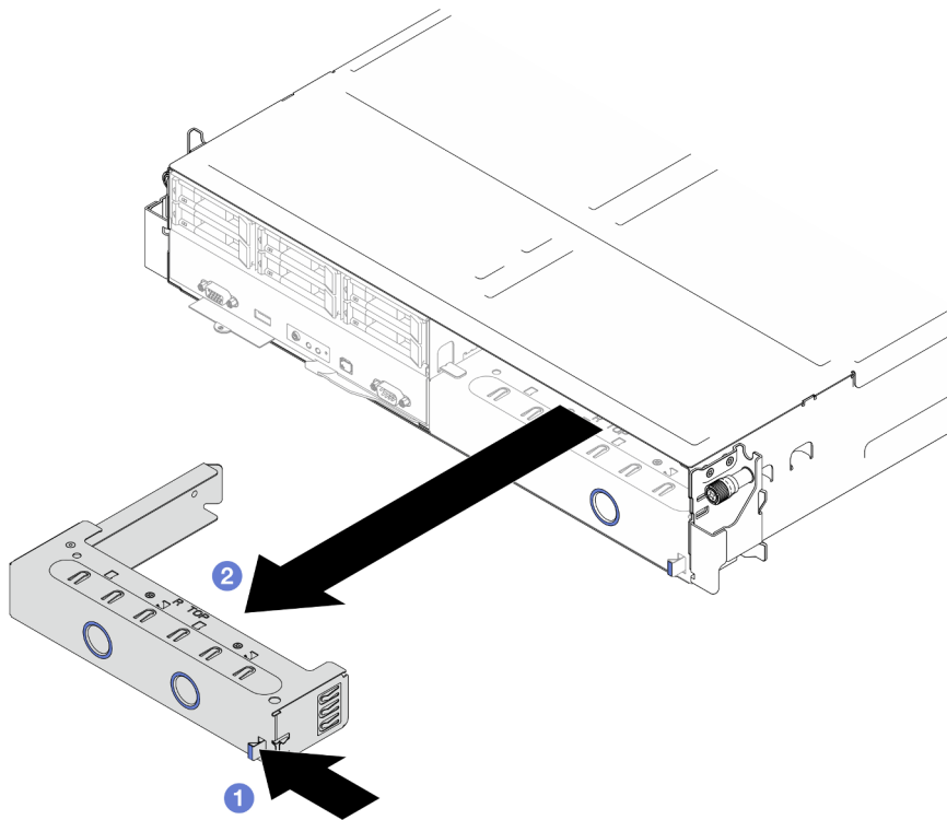
Abbildung 23. Entfernen der Abdeckblende für einen Knotenrahmen an der Vorderseite
