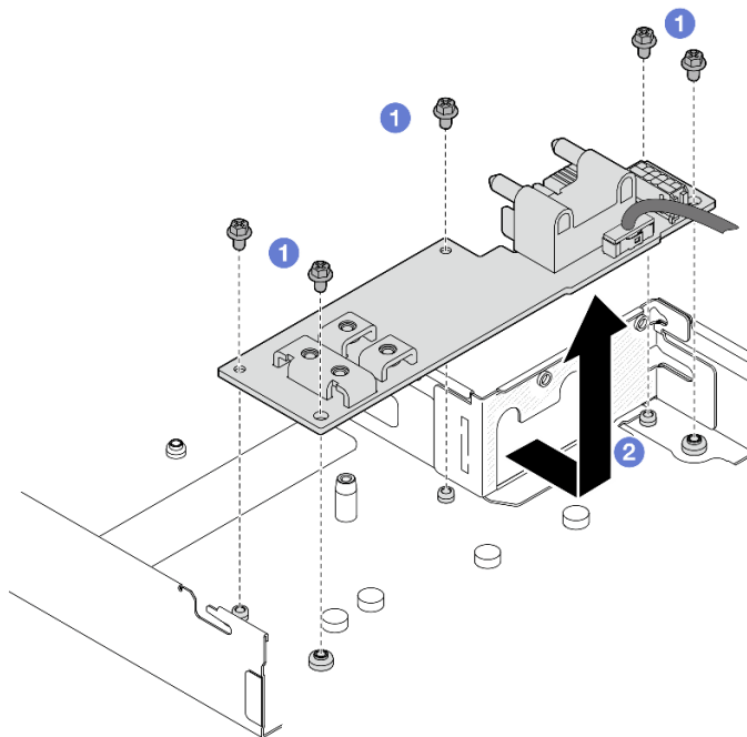
Abbildung 86. Entfernen der Stromversorgungsplatine
