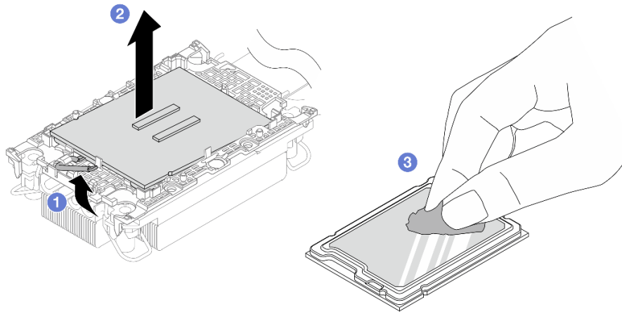
Abbildung 91. Trennen eines Prozessors von Kühlkörper und Träger
