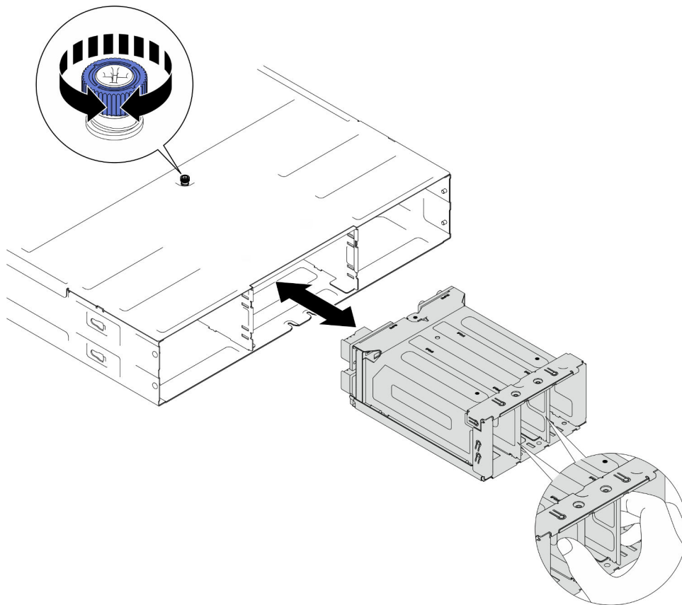
Abbildung 15. Entfernen des PSU-Rahmens
