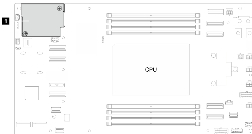
Abbildung 102. Position des Firmware- und RoT-Sicherheitsmodul
