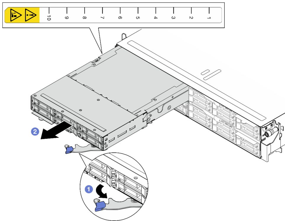
Abbildung 19. Knotenentfernung aus einem linken Rahmen
