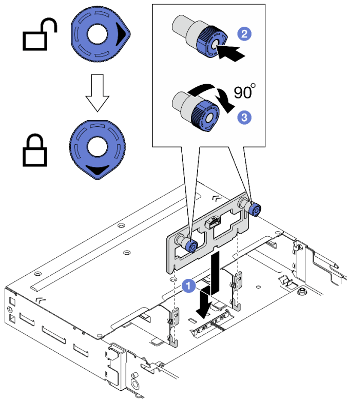
Abbildung 42. Installation der E/A-Platine an der Vorderseite
