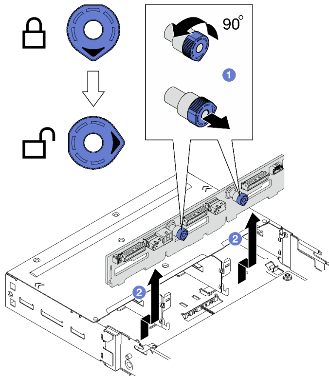
Abbildung 31. Entfernen der Rückwandplatine für Laufwerke
