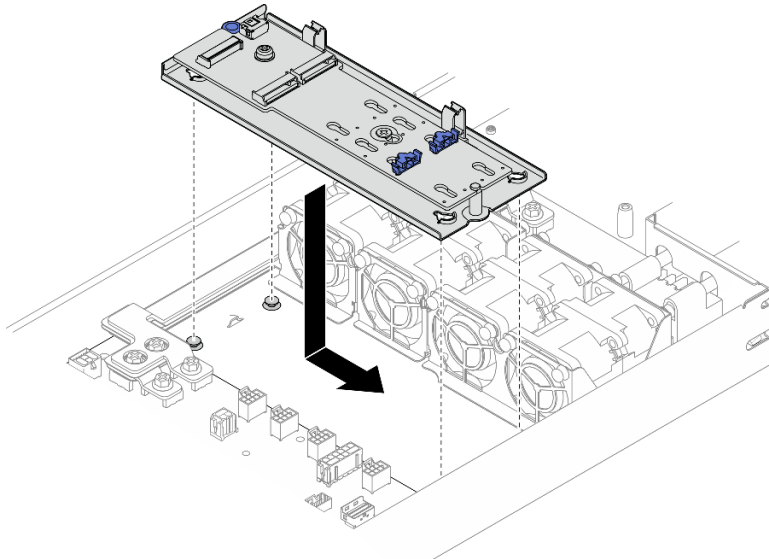
Abbildung 55. Installation eines M.2-Bootadapters
