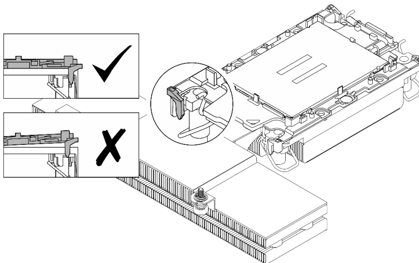
Abbildung 97. Visuelle Inspektion der Trägerklammern
