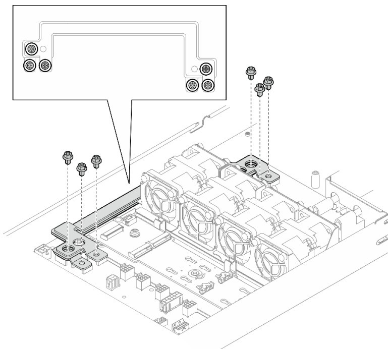
Abbildung 85. Anbringen der äußeren Schrauben der Sammelschiene
