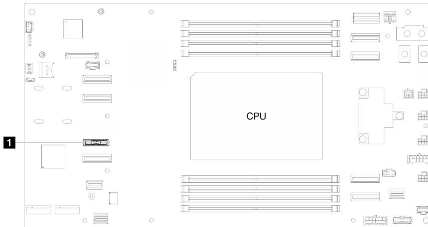
Abbildung 27. Position des CMOS-Batteriesockels
