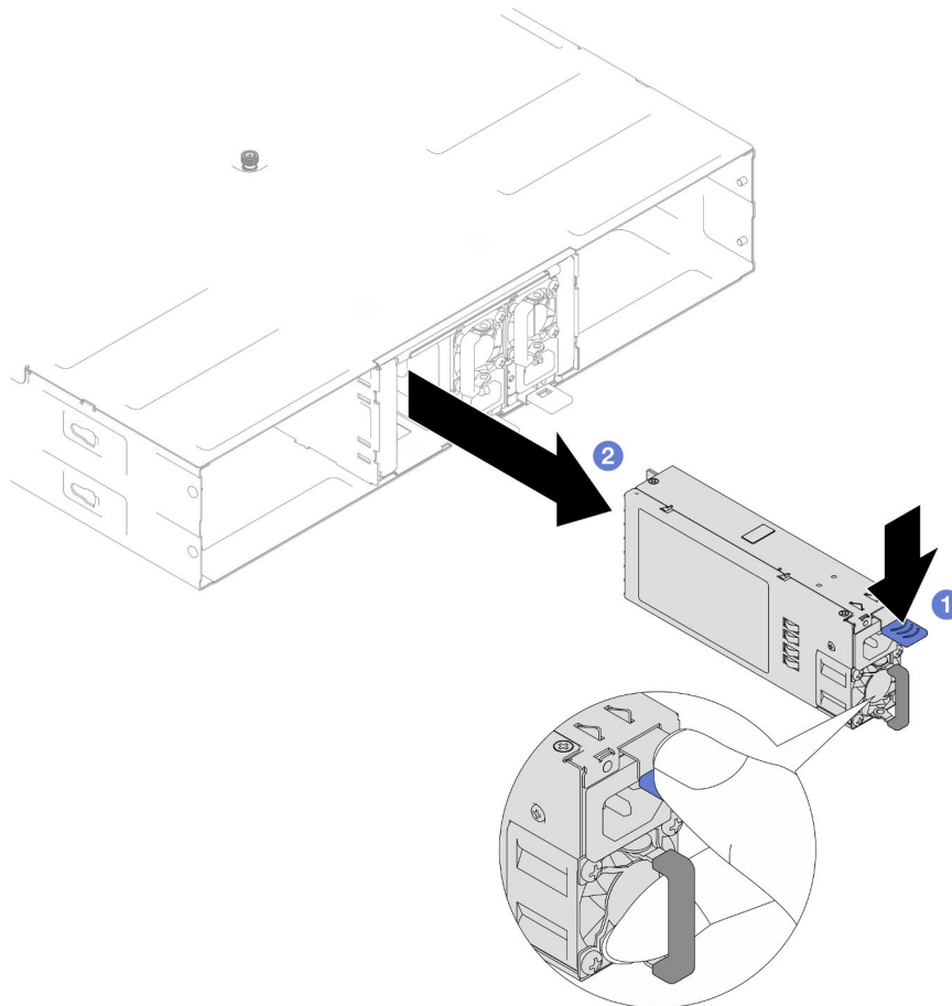
Abbildung 10. Entfernen eines Hot-Swap-PSUs
