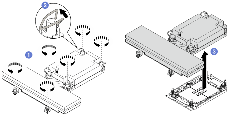
Abbildung 90. Entfernen des Hochleistungs-PHM
