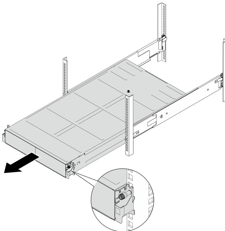
Abbildung 4. Entfernen des Gehäuses
