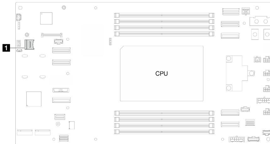
Abbildung 71. Position des microSD-Steckplatzes
