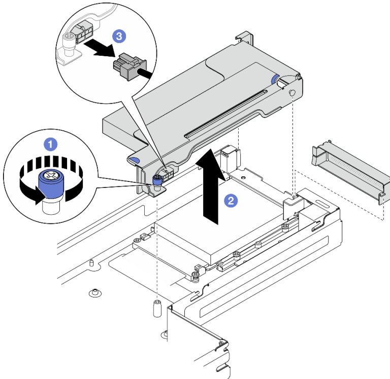
Abbildung 75. Entfernen der PCIe-Adapterkartenbaugruppe
