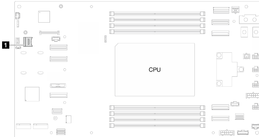
Abbildung 69. Position des microSD-Steckplatzes
