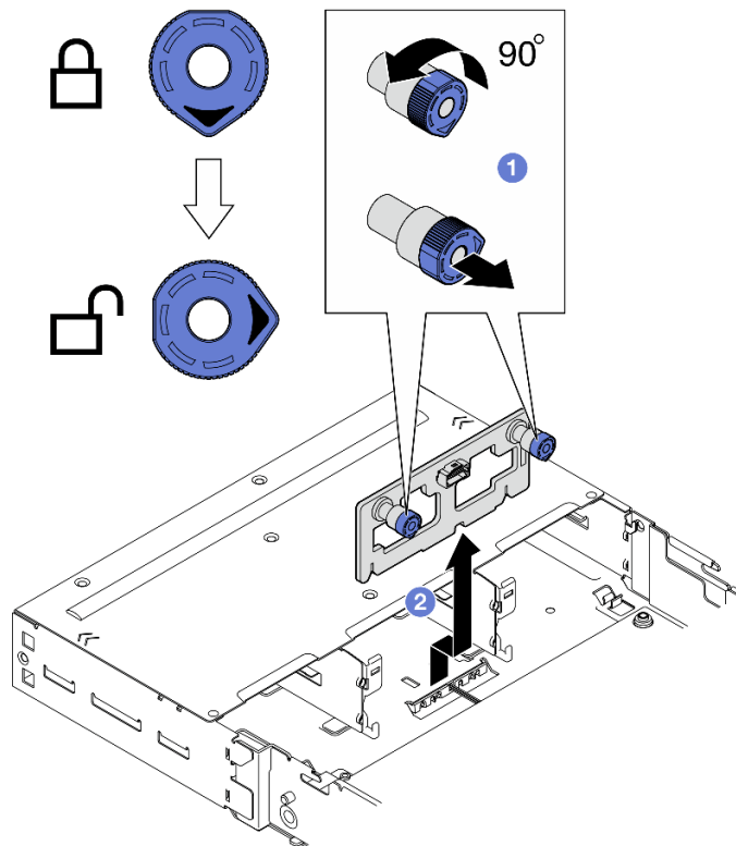
Abbildung 41. Entfernen der E/A-Platine an der Vorderseite
