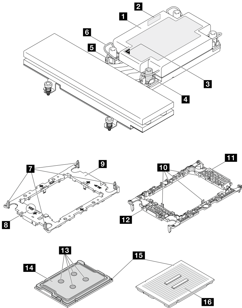
Abbildung 88. PHM-Komponenten
