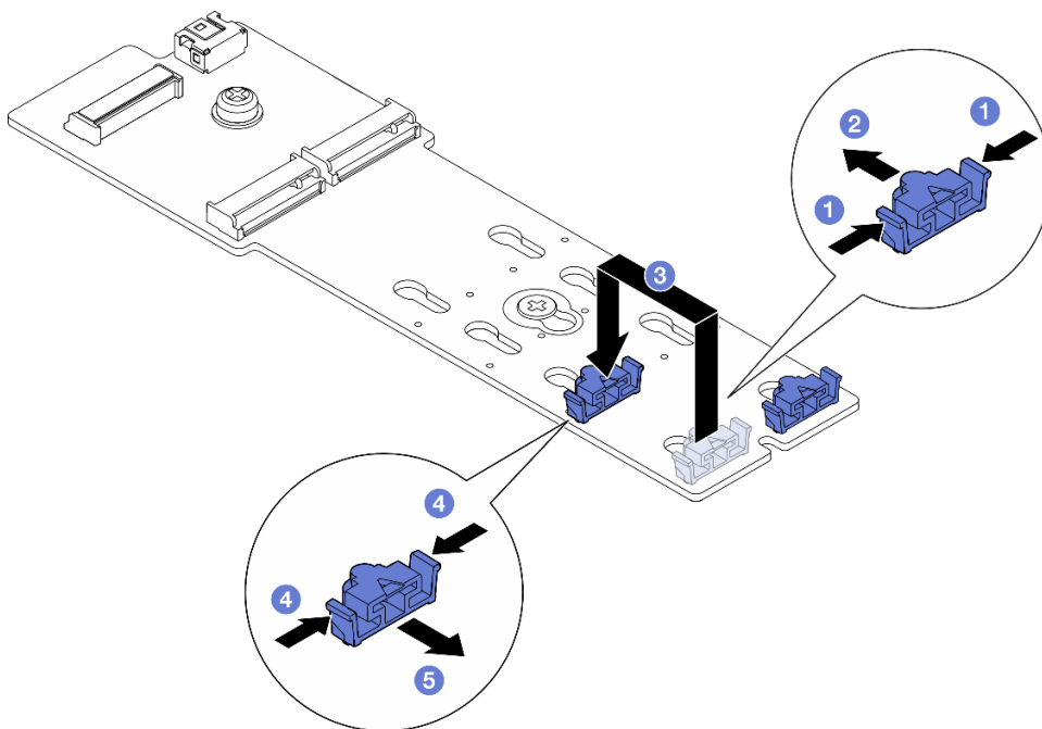
Abbildung 58. Positionsanpassung der M.2-Halterung
