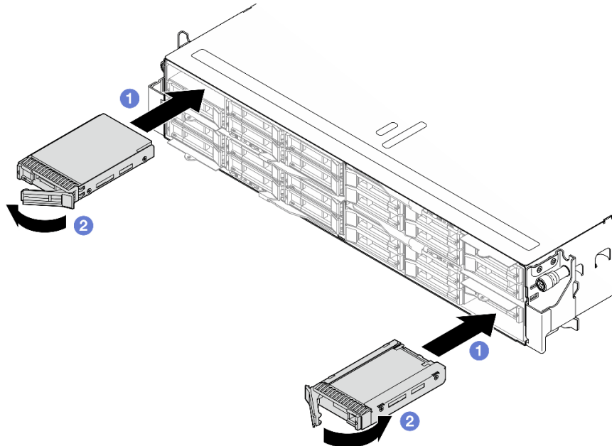
Abbildung 46. Installation eines Solid-State-Laufwerks
