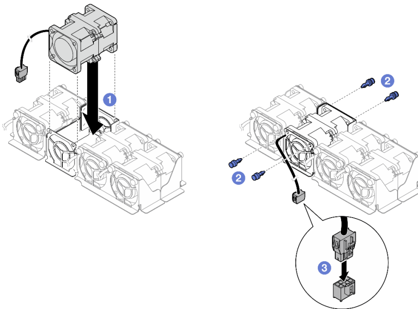
Abbildung 34. Lüftereinbau
