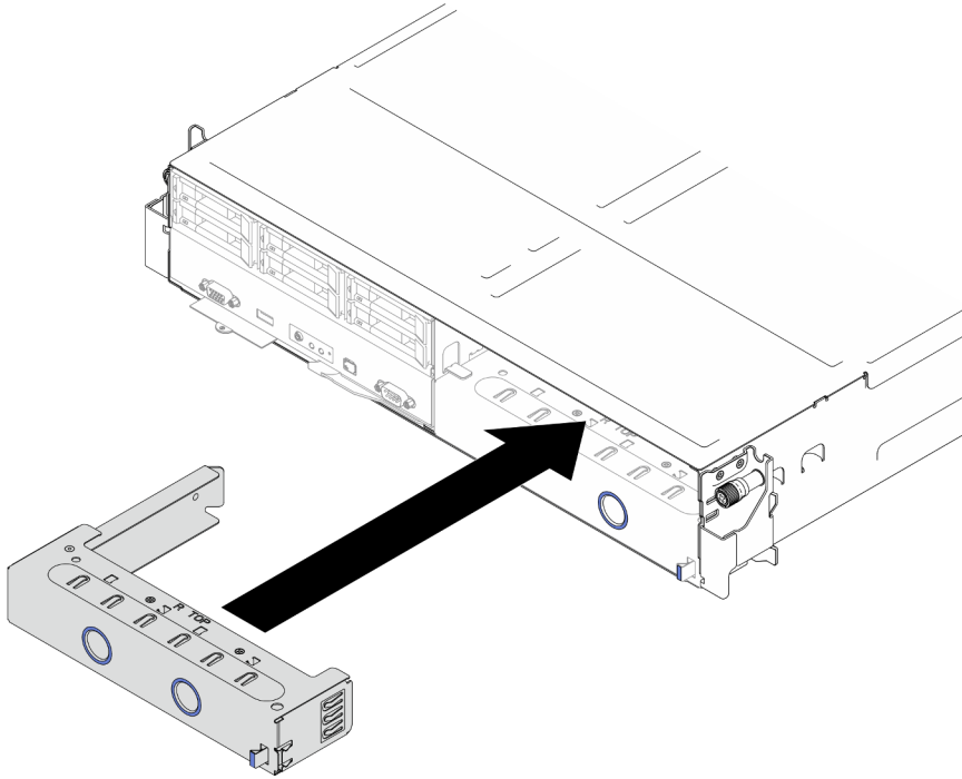
Abbildung 21. Installation einer Abdeckblenden für einen Knotenrahmen an der Vorderseite
