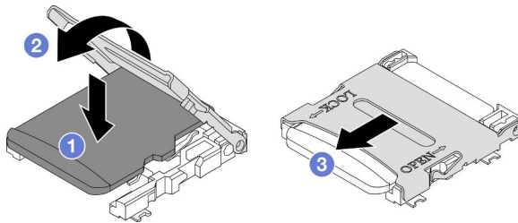
Abbildung 72. Installation einer MicroSD-Karte
