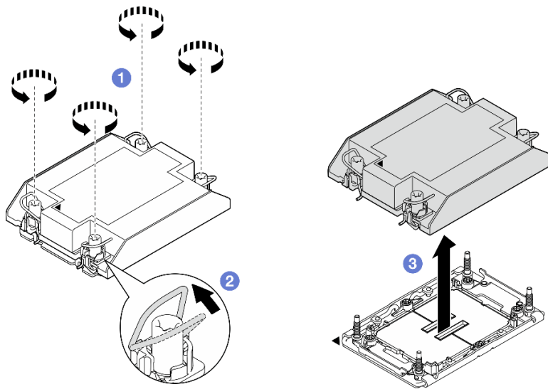
Abbildung 89. Entfernen des Standard-PHM
