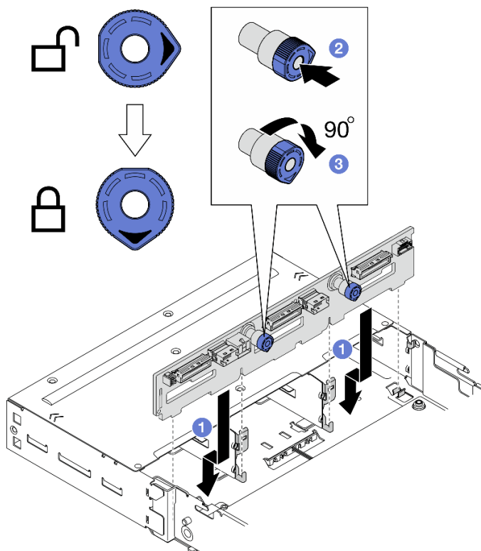
Abbildung 32. Installation der Rückwandplatine für Laufwerke
