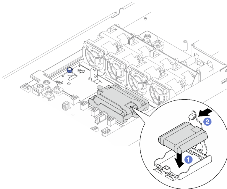
Abbildung 39. Installation des Flash-Stromversorgungsmoduls
