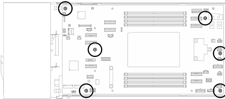
Abbildung 110. Position der Schrauben auf der Systemplatine
