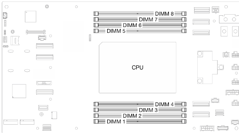
Abbildung 65. Layout für Speichermodule und Prozessoren
