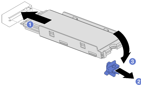
Abbildung 62. Installation eines M.2-Laufwerks
