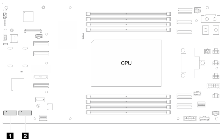
Abbildung 59. Positionen der M.2-Steckplätze auf der Systemplatine
