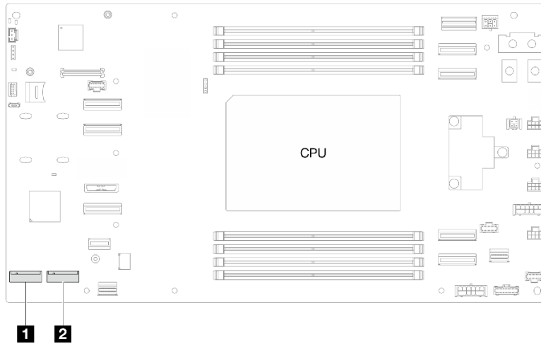
Abbildung 47. Position der M.2-Steckplätze auf der Systemplatine
