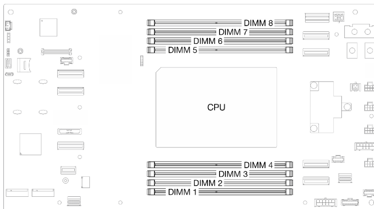
Abbildung 1. Layout für Speichermodule und Prozessoren
