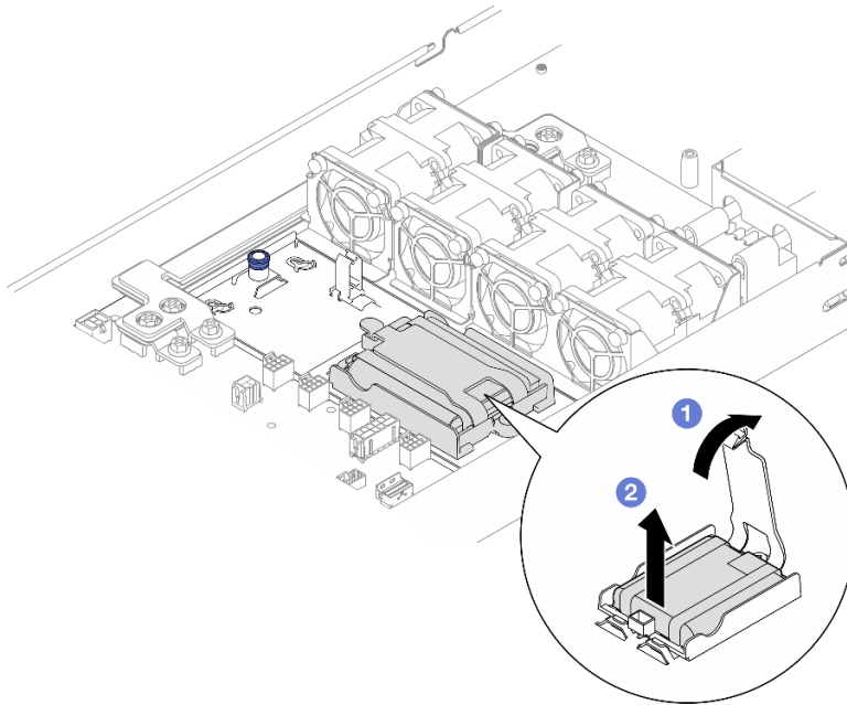
Abbildung 36. Entfernen des Flash-Stromversorgungsmoduls
