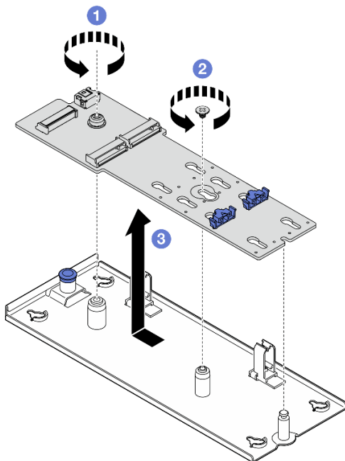
Abbildung 53. Entfernen des M.2-Bootadapters
