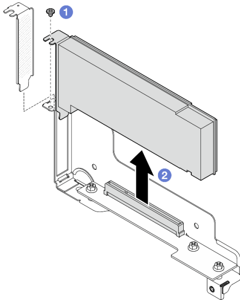
Abbildung 77. Entfernen eines PCIe-Adapters
