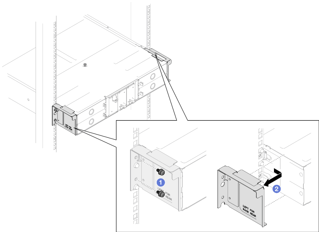
Abbildung 3. Entfernen von Transporthalterungen für 29,5 Zoll tiefe Racks
