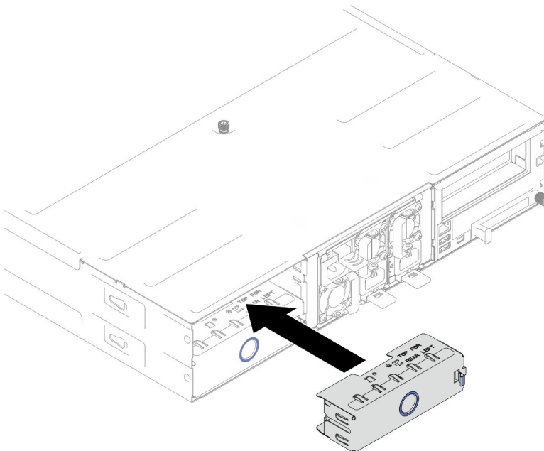
Abbildung 22. Installation einer Abdeckblenden für einen Knotenrahmen an der Rückseite
