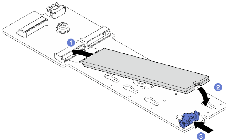
Abbildung 64. Installation eines M.2-Laufwerks
