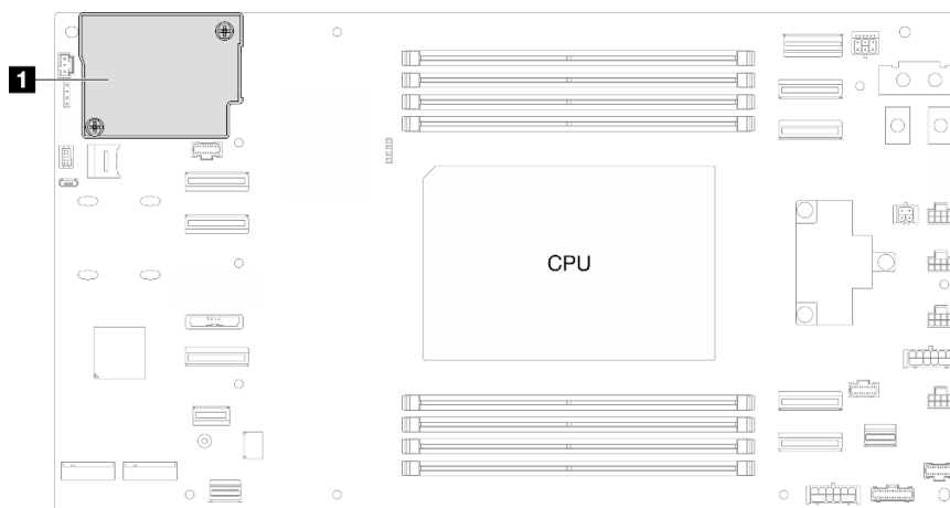
Abbildung 104. Position des Firmware- und RoT-Sicherheitsmodul
