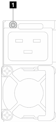
Abbildung 117. Netzteilanzeige
