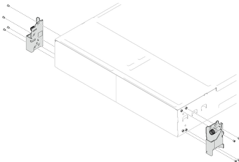
Abbildung 8. Entfernen der EIA-Halterungen
