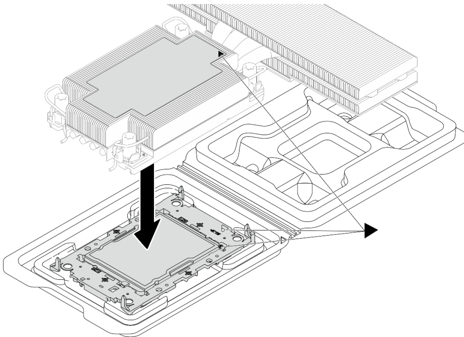
Abbildung 96. Zusammenbauen der PHM mit Prozessor im Versandeinbaurahmen
