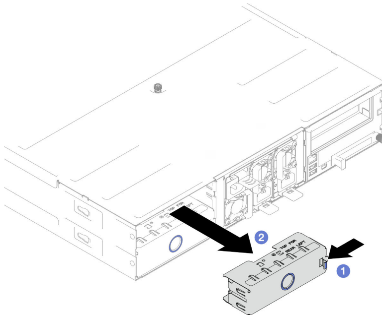
Abbildung 24. Entfernen der Abdeckblende für einen Knotenrahmen an der Rückseite
