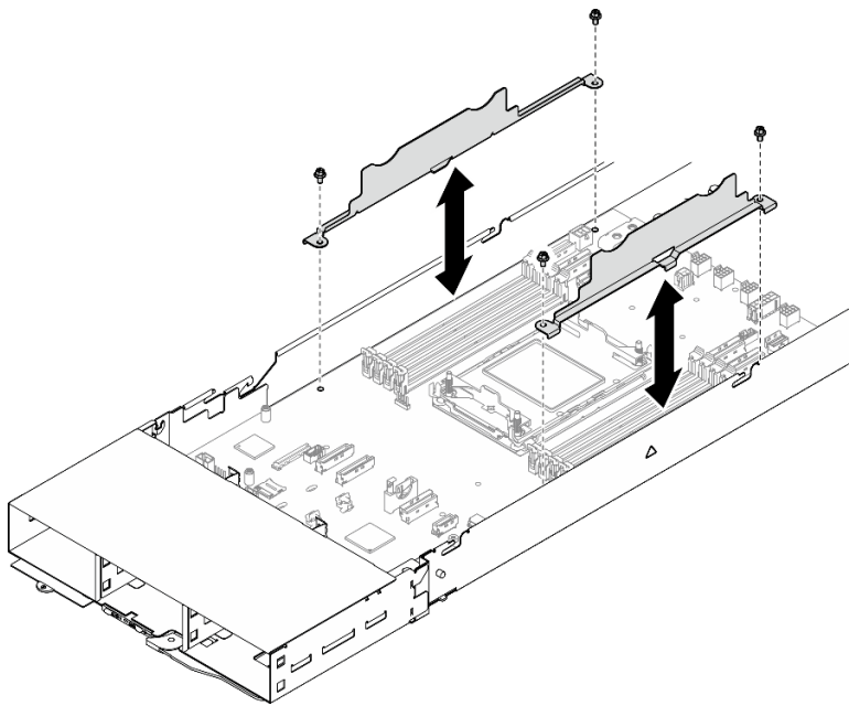
Abbildung 111. Installation der Kabelwand
