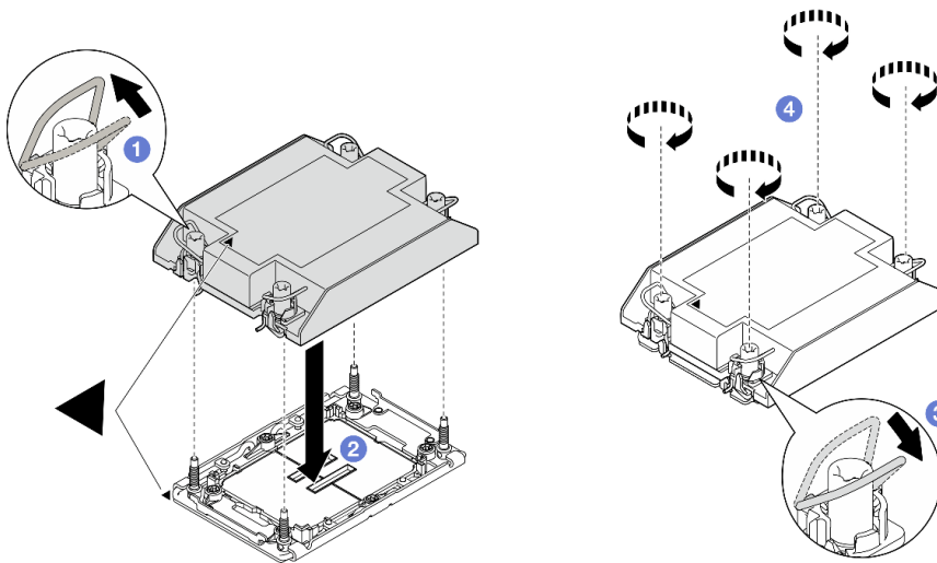
Abbildung 98. Installation des Standard-PHM
