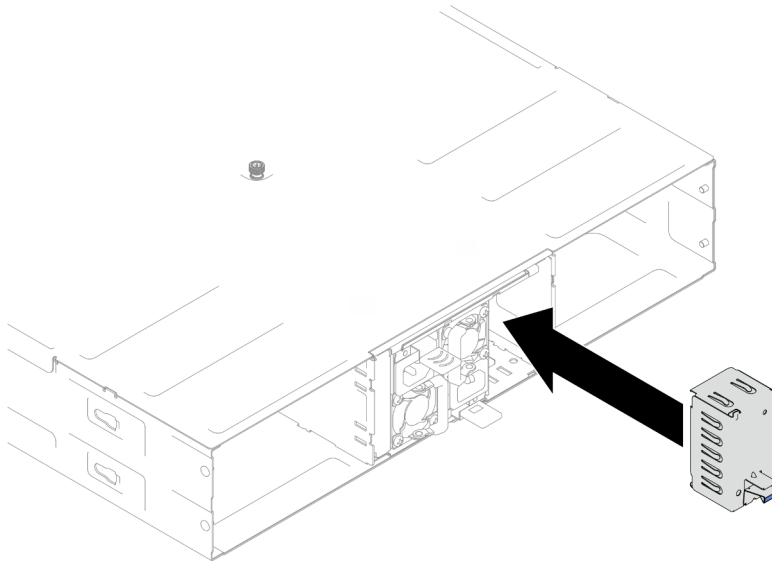
Abbildung 11. Installation einer PSU-Abdeckblende
