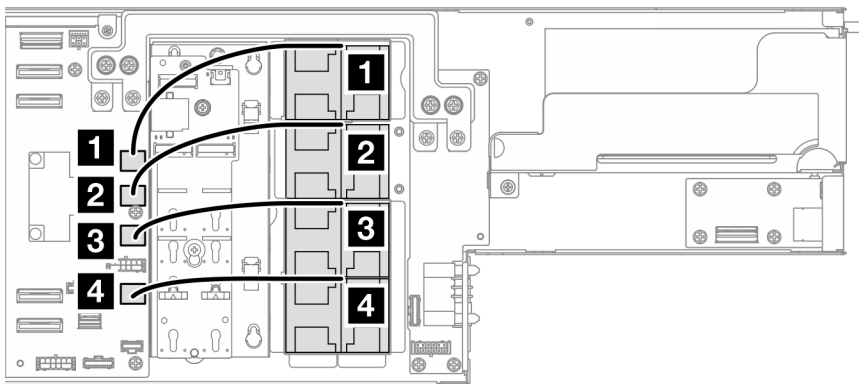
Abbildung 35. Lüfterkabelführung
