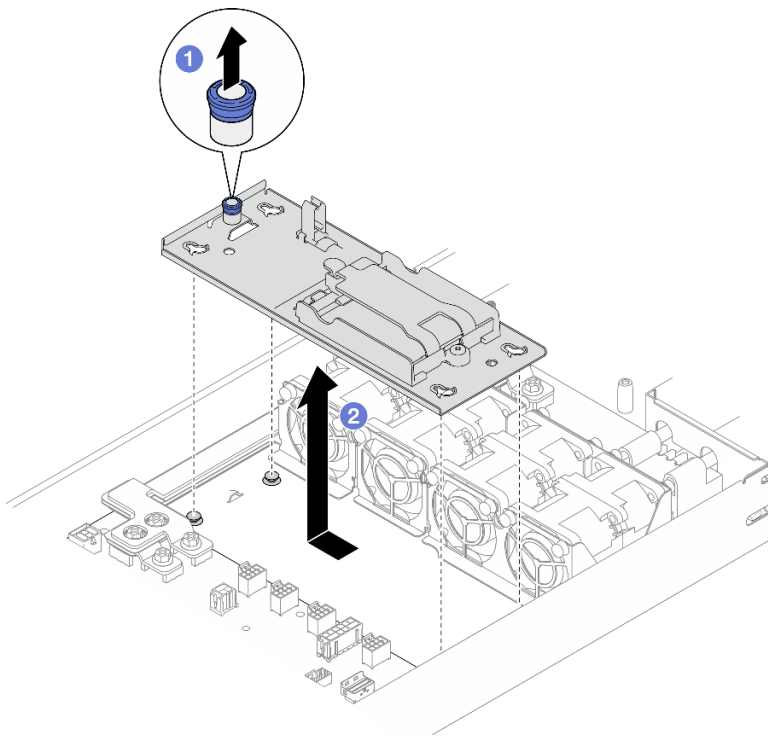
Abbildung 37. Entfernen der Halterung des Flash-Stromversorgungsmoduls
