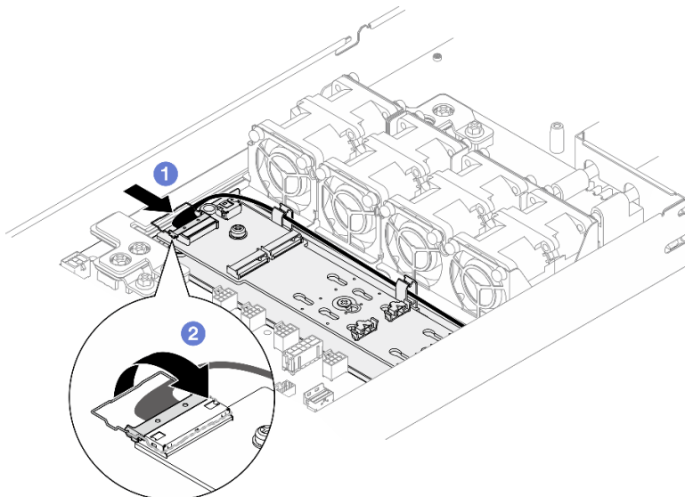
Abbildung 56. Anschließen des Kabels am SATA/NVMe M.2-Bootadapter
