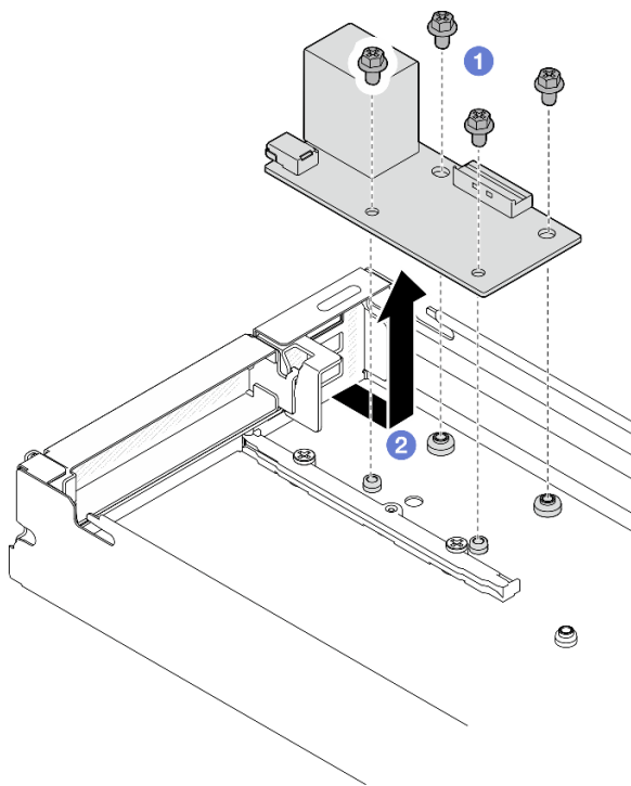
Abbildung 100. Entfernen des E/A-Modul an der Rückseite
