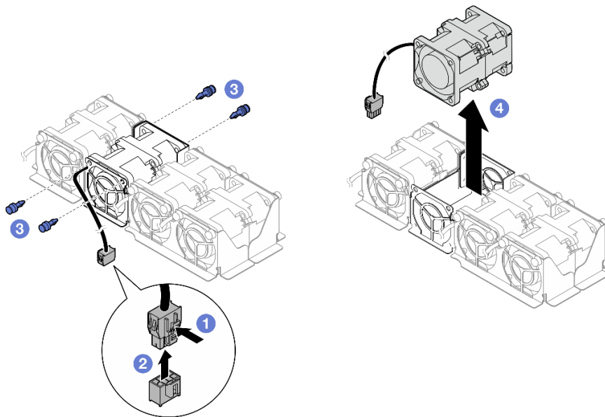
Abbildung 33. Entfernen des Lüfters
