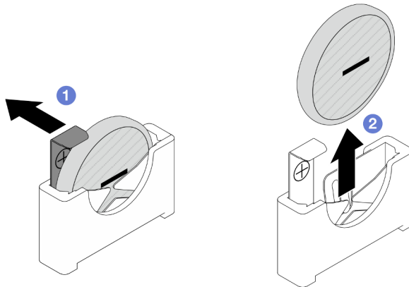
Abbildung 28. Entfernen der CMOS-Batterie
