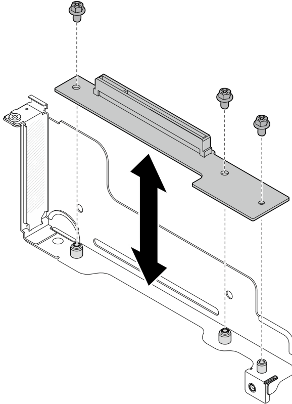
Abbildung 80. Austausch der PCIe-Adapterkarte
