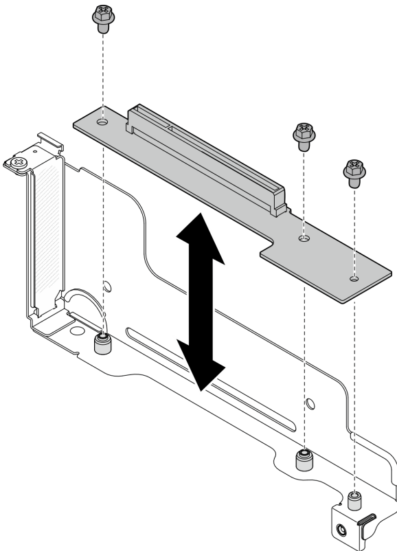
Abbildung 76. Austausch der PCIe-Adapterkarte
