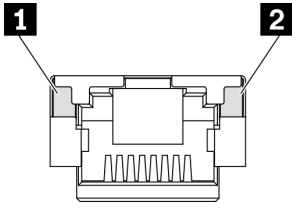
Abbildung 119. Anzeigen am XCC-Systemmanagement-Anschluss (10/100/1.000 Mbit/s RJ-45)
