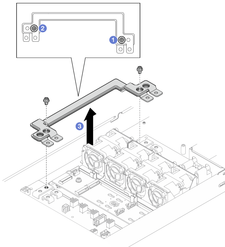
Abbildung 83. Entfernen der Sammelschiene
