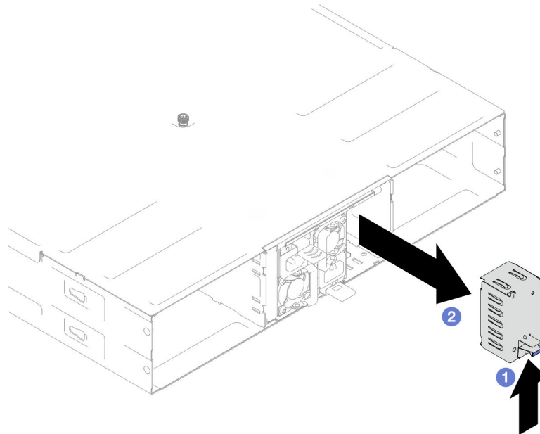
Abbildung 12. Entfernen einer PSU-Abdeckblende
