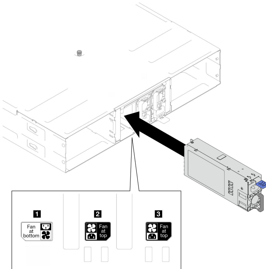
Abbildung 13. Installation eines Hot-Swap-Netzteils
