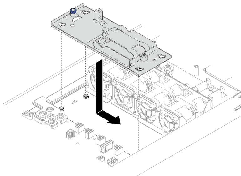
Abbildung 38. Installation der Halterung für das Flash-Stromversorgungsmodul
