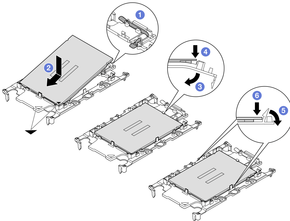
Abbildung 94. Installation des Prozessorträgers
