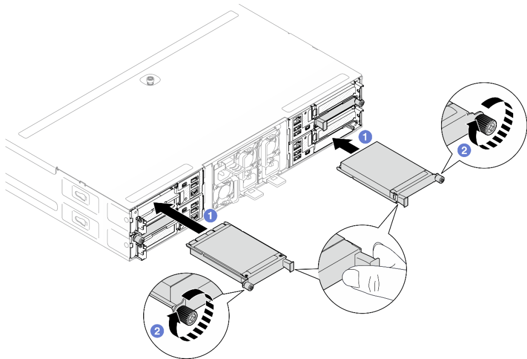
Abbildung 73. Entfernen des hinteren OCP-Moduls
