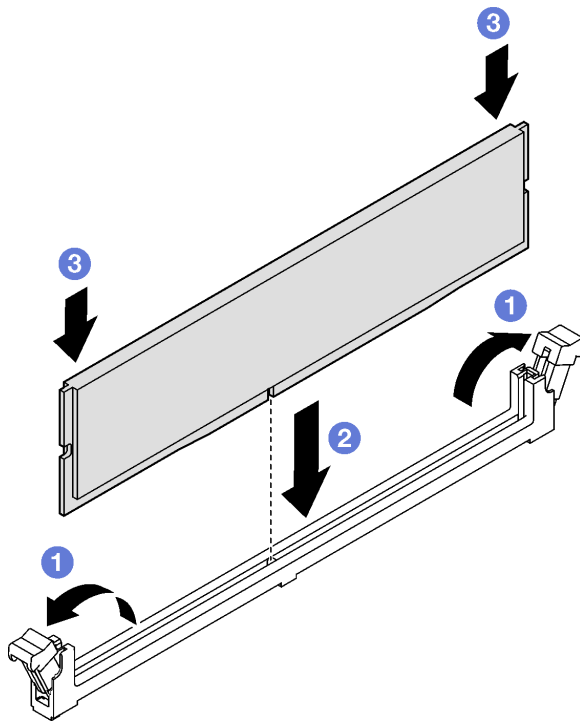
Abbildung 68. Installieren eines Speichermoduls
