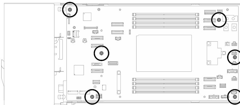
Abbildung 107. Position der Schrauben auf der Systemplatine
