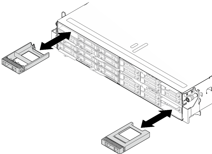
Abbildung 45. Austausch einer Abdeckblende für Laufwerke
