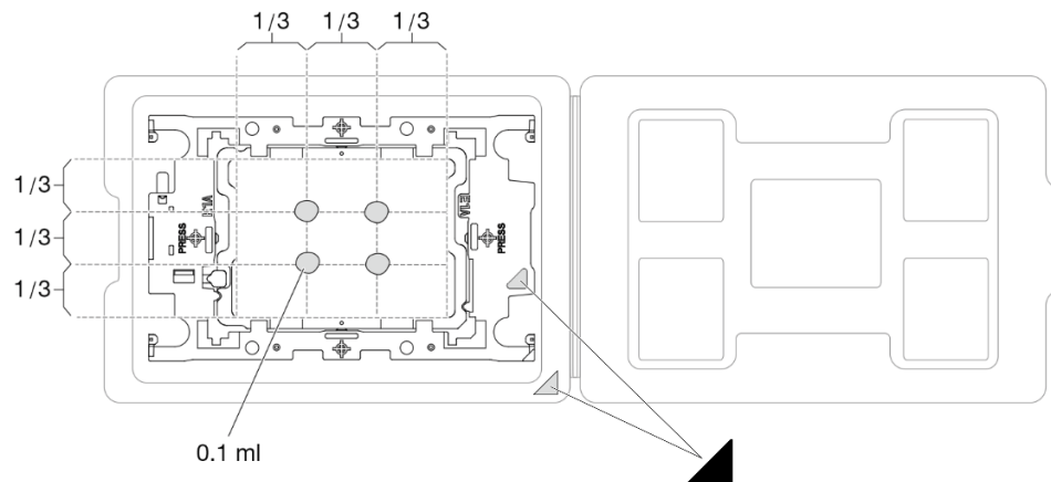
Abbildung 95. Auftragen von Wärmeleitpaste mit Prozessor im Versandeinbaurahmen
