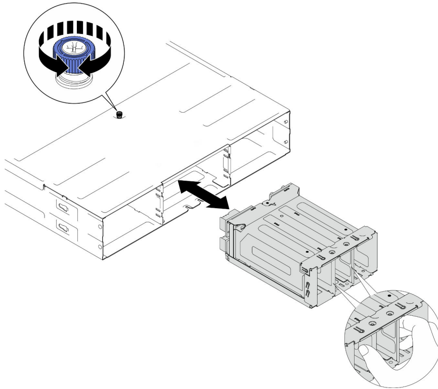
Abbildung 18. Installation des PSU-Rahmens
