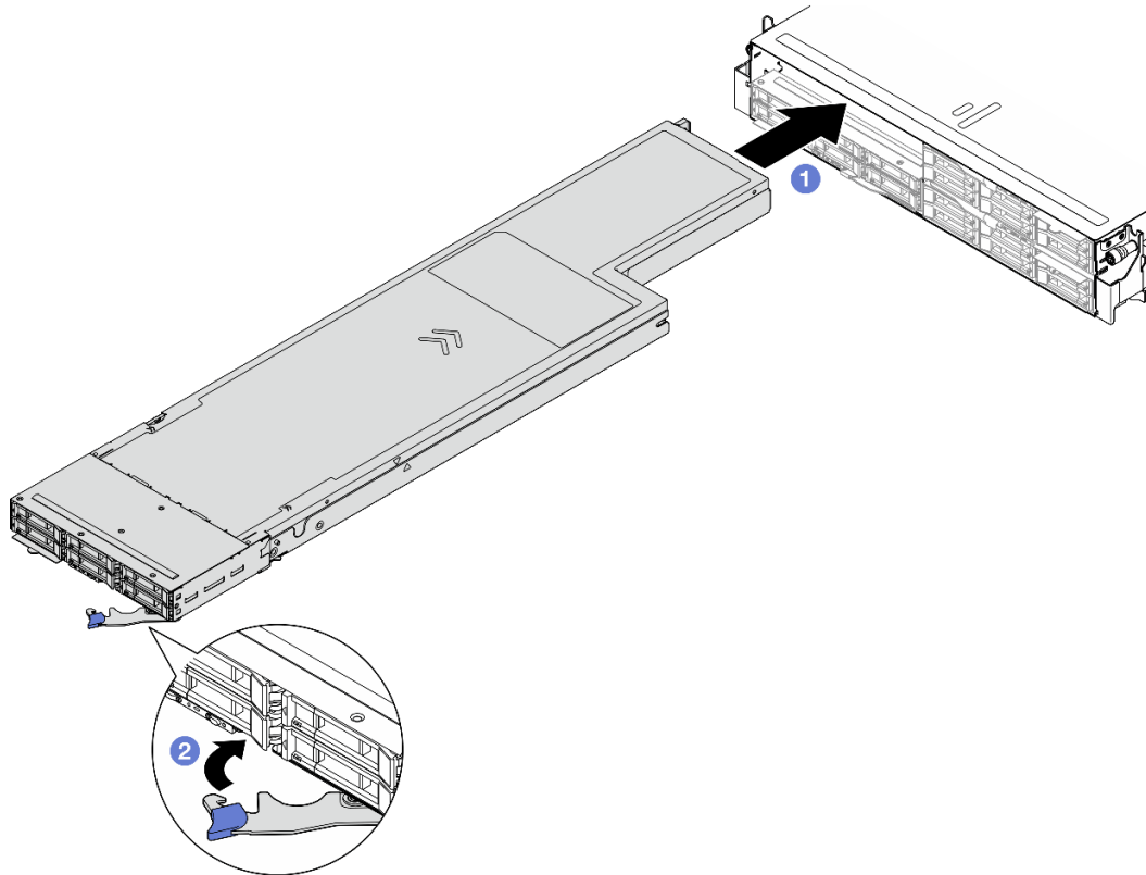
Abbildung 25. Knoteninstallation in einem linken Rahmen
