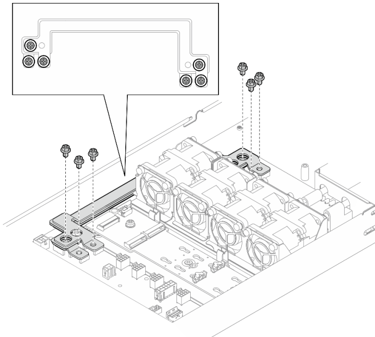
Abbildung 82. Entfernen der äußeren Schrauben der Sammelschiene
