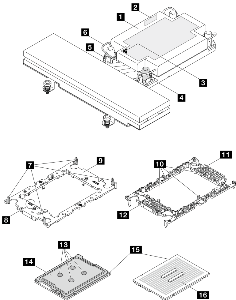
Abbildung 93. PHM-Komponenten
