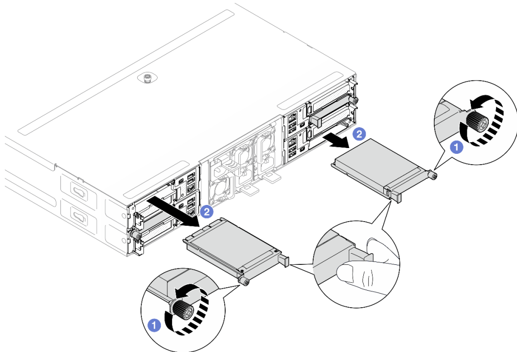
Abbildung 74. Installation des hinteren OCP-Moduls
