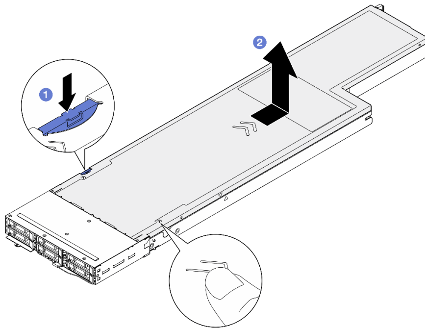
Abbildung 112. Entfernen der oberen Abdeckung
