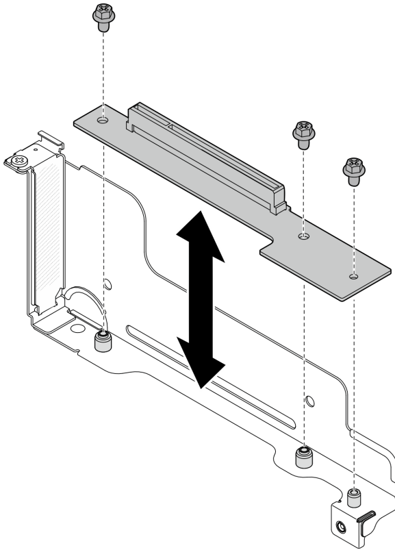
Figura 80. Sostituzione della scheda verticale PCIe
