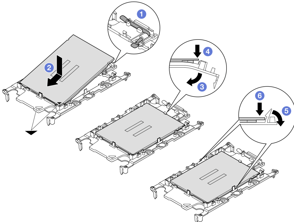
Figura 94. Installazione della piastra del processore
