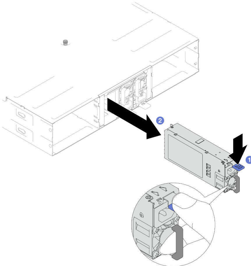
Figura 10. Rimozione di una PSU hot-swap
