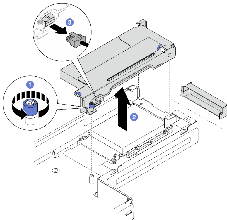
Figura 75. Rimozione dell'assieme verticale PCIe
