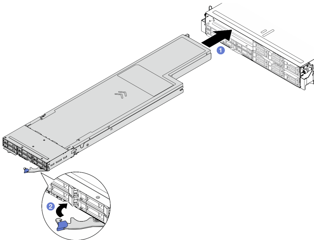
Figura 25. Installazione del nodo in un vassoio sinistro
