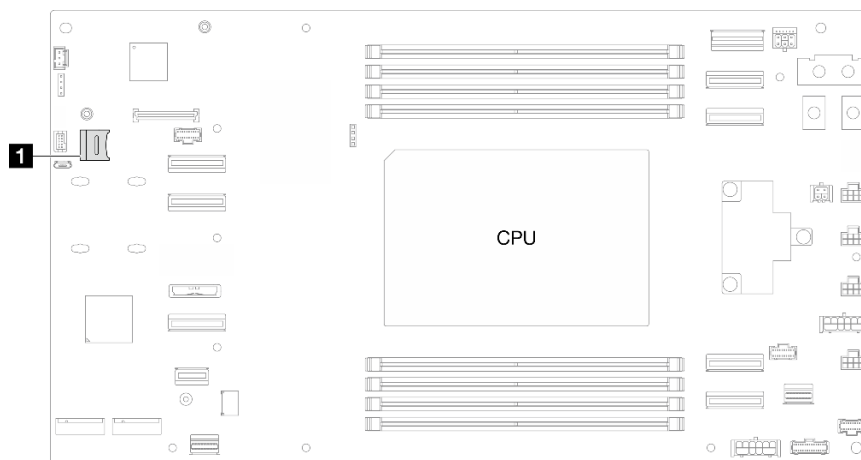
Figura 71. Posizione del socket MicroSD
