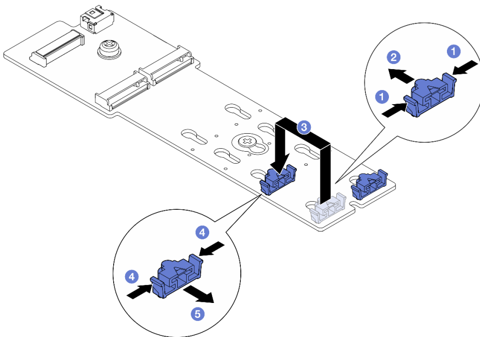
Figura 58. Regolazione del blocco M.2
