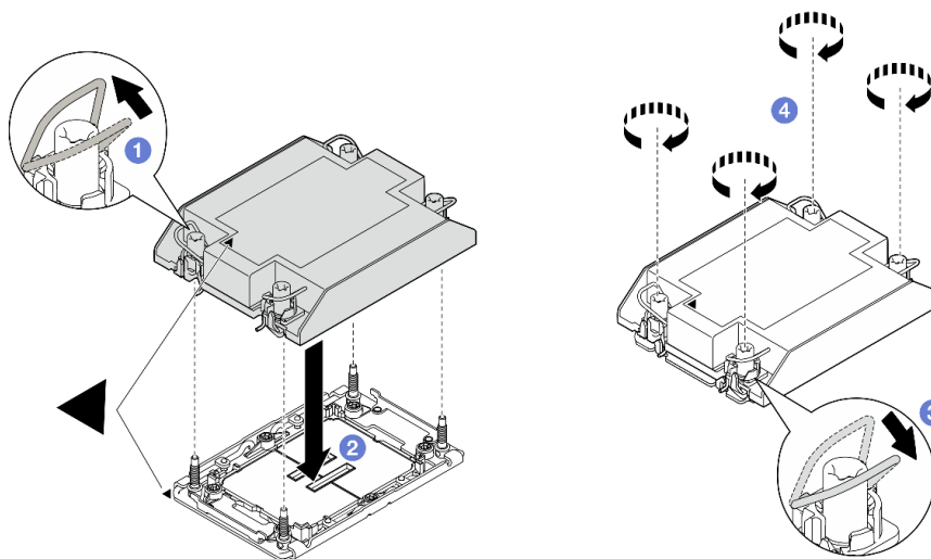
Figura 98. Installazione del PHM standard
