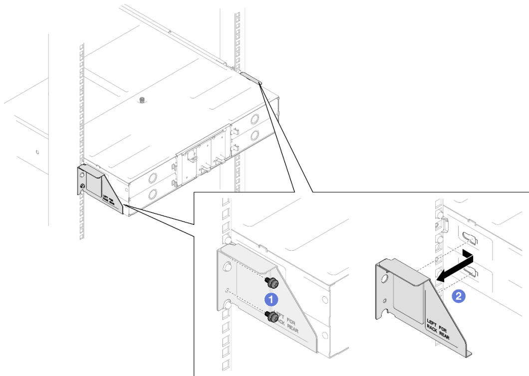
Figura 2. Rimozione delle staffe di spedizione per rack profondi 29 pollici o 28,31 pollici
