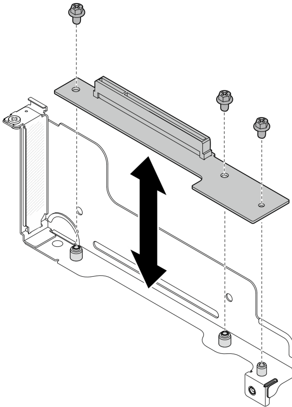
Figura 78. Sostituzione della scheda verticale PCIe
