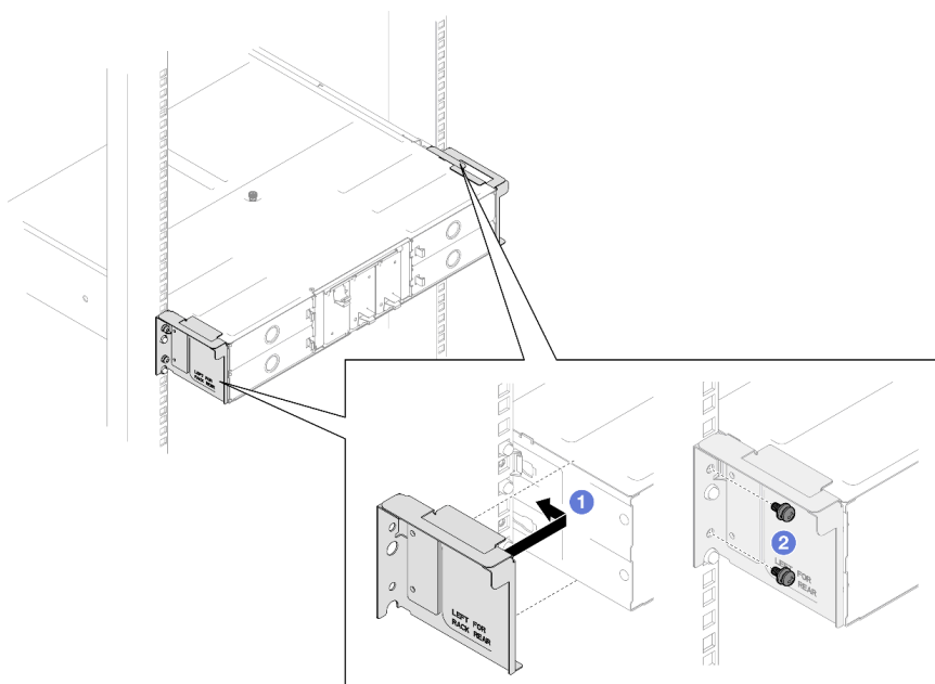
Figura 7. Installazione delle staffe di spedizione per rack profondi 29,5 pollici
