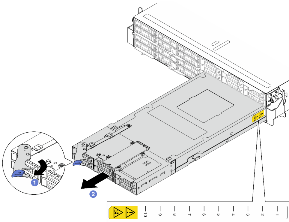
Figura 20. Rimozione del nodo da un vassoio destro
