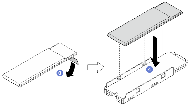
Figura 61. Installazione di un dissipatore di calore M.2 nel vassoio M.2
