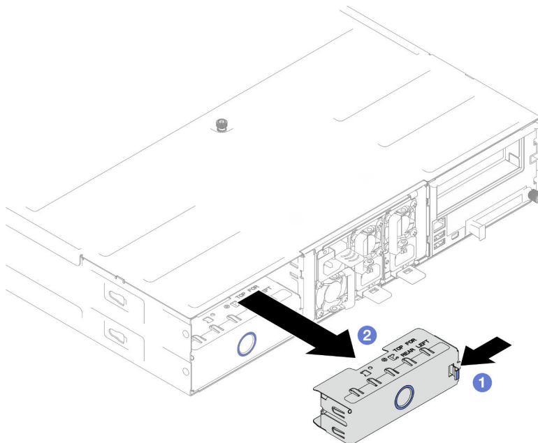
Figura 24. Rimozione di un elemento di riempimento del vassoio del nodo posteriore
