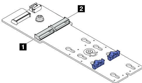
Figura 63. Slot dell'unità M.2
