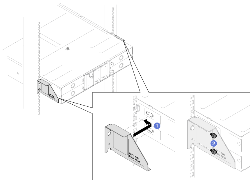
Figura 6. Installazione delle staffe di spedizione per rack profondi 29 pollici o 28,31 pollici
