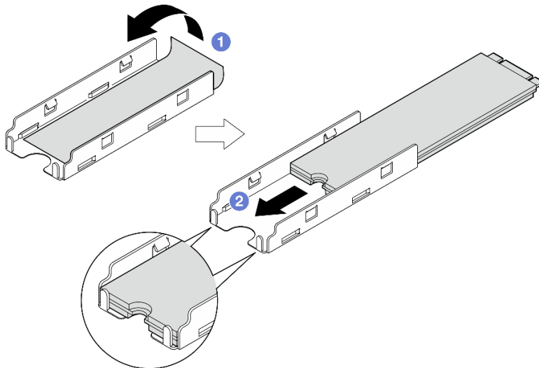
Figura 60. Installazione di un pad termico e di un'unità M.2 nel vassoio
