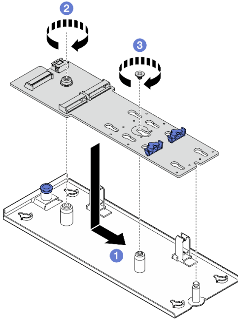
Figura 54. Installazione dell'adattatore di avvio M.2
