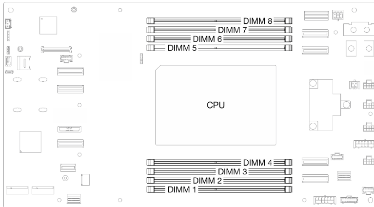
Figura 1. Layout dei moduli di memoria e dei processori
