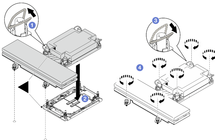
Figura 99. Installazione del PHM ad alte prestazioni
