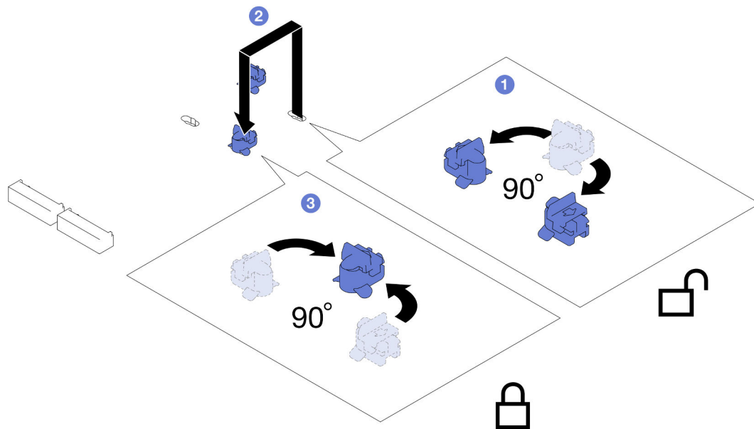
Figura 57. Regolazione del fermo di un'unità M.2
