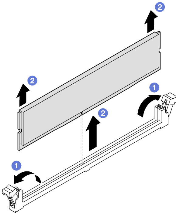
Figura 66. Rimozione di un modulo di memoria
