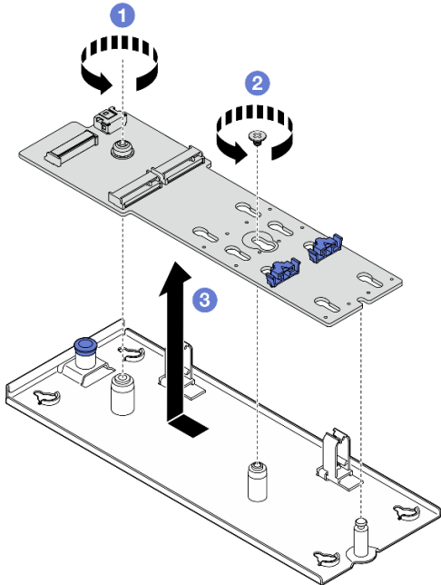
Figura 53. Rimozione dell'adattatore di avvio M.2
