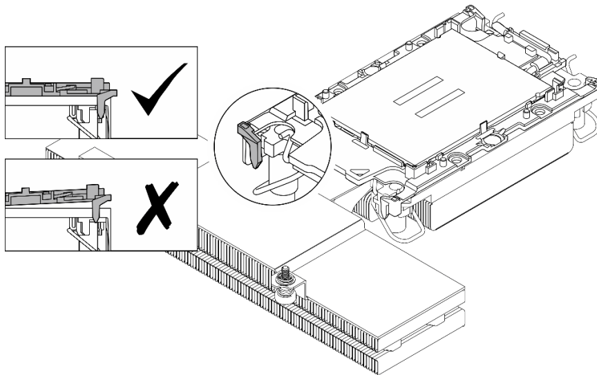
Figura 97. Controllo visivo dei fermi della piastra
