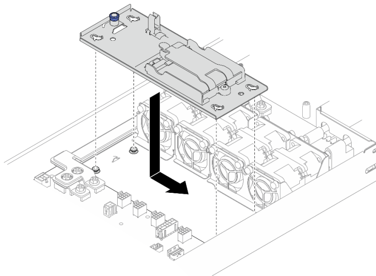
Figura 38. Installazione del supporto del modulo di alimentazione flash
