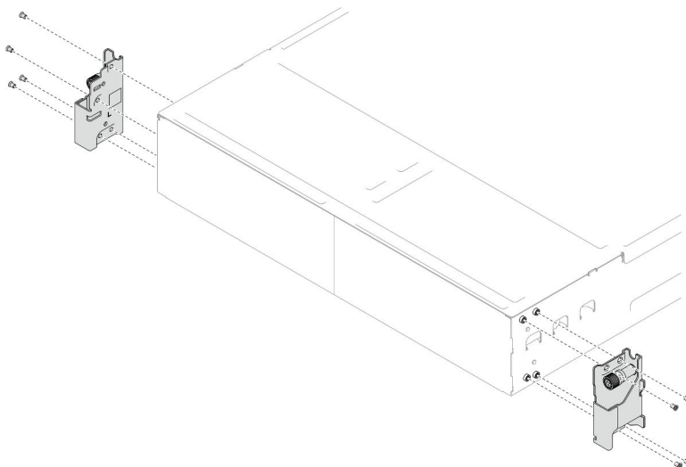
Figura 8. Rimozione delle staffe EIA
