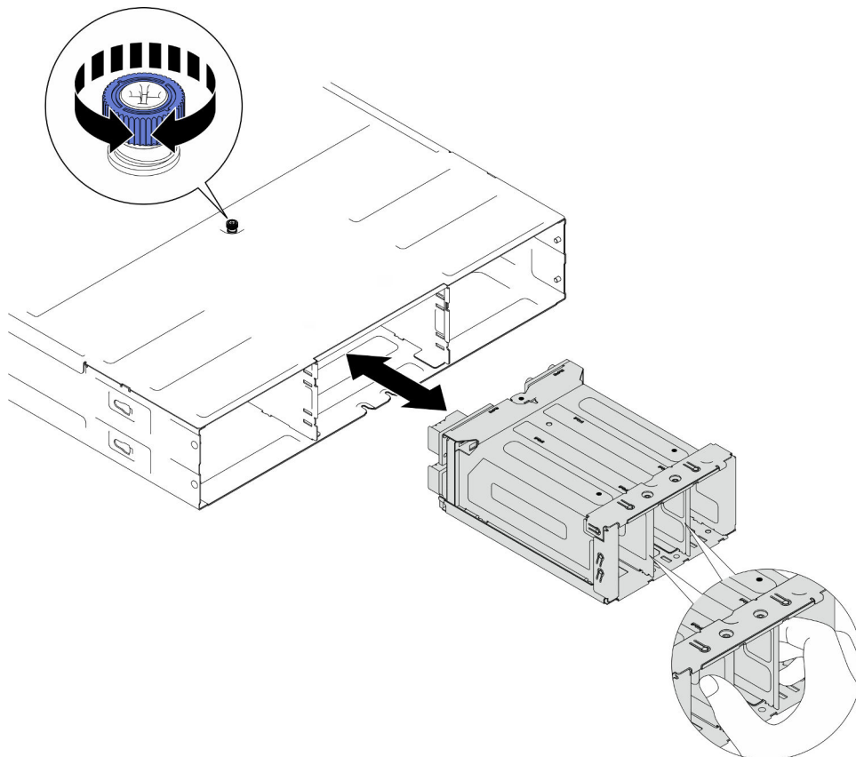
Figura 15. Rimozione del telaio PSU
