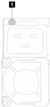
Figura 117. LED alimentatore
