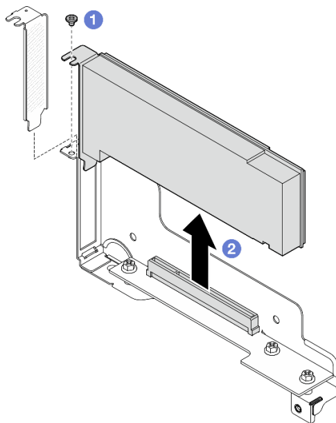
Figura 77. Rimozione di un adattatore PCIe
