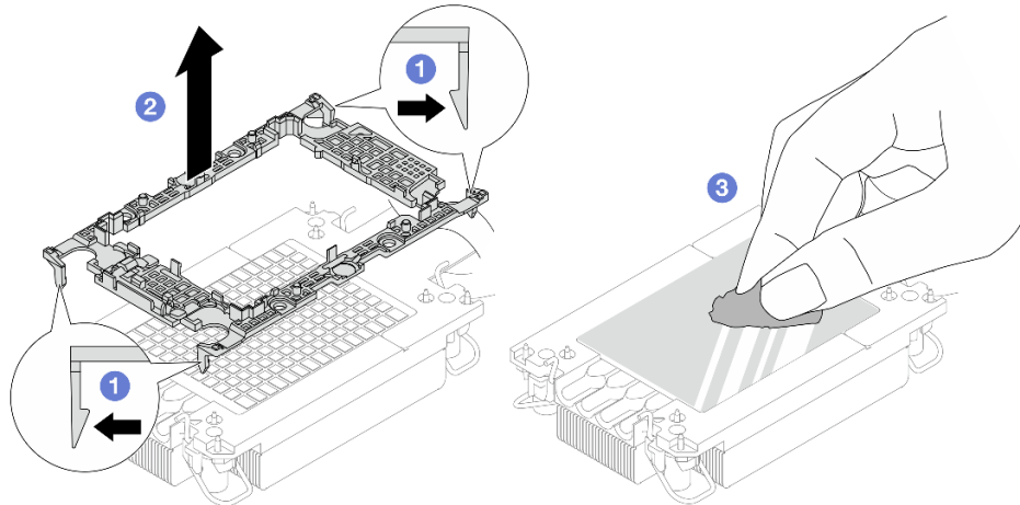
Figura 92. Separazione di una piastra del processore dal dissipatore di calore
