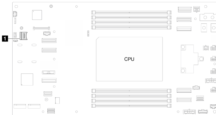
Figura 69. Posizione del socket MicroSD
