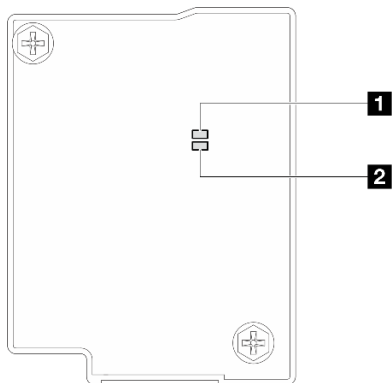
Figura 118. LED sul modulo firmware e sicurezza RoT
