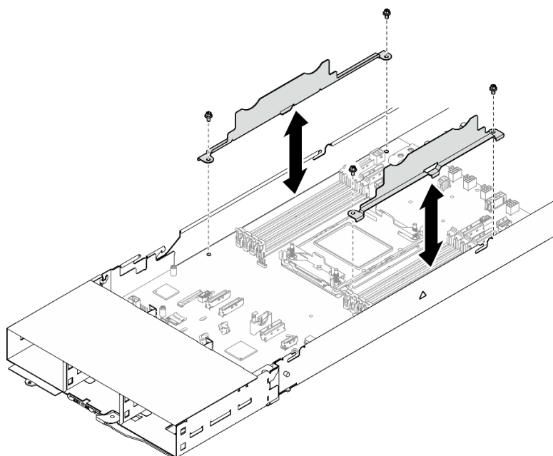
Figura 111. Installazione delle pareti del cavo
