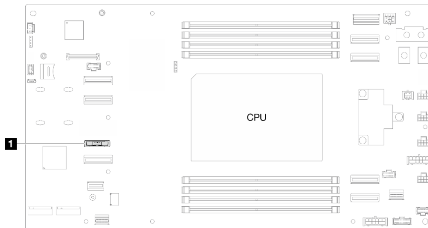
Figura 29. Posizione del socket della batteria CMOS
