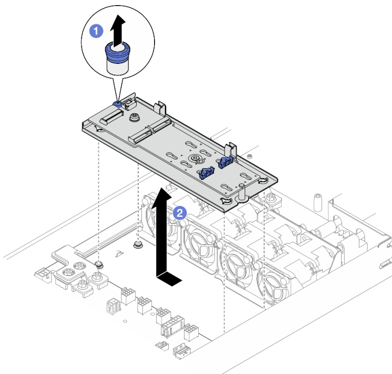
Figura 52. Rimozione del vassoio dell'adattatore di avvio M.2
