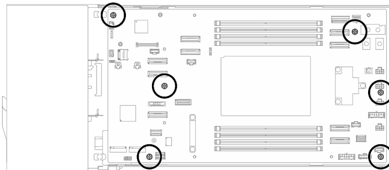
Figura 107. Posizione delle viti della scheda di sistema
