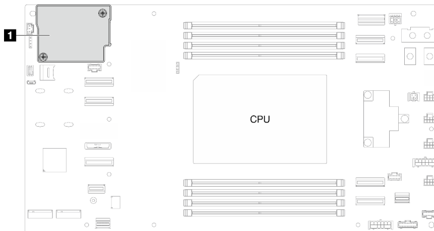
Figura 102. Posizione del Modulo firmware e sicurezza RoT
