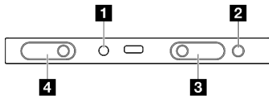
Figura 116. Pulsanti e LED sul pannello anteriore dell'operatore
