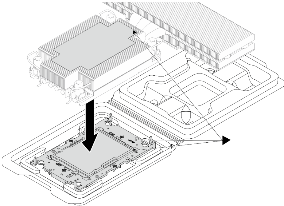
Figura 96. Assemblaggio del PHM con il processore nella confezione di spedizione
