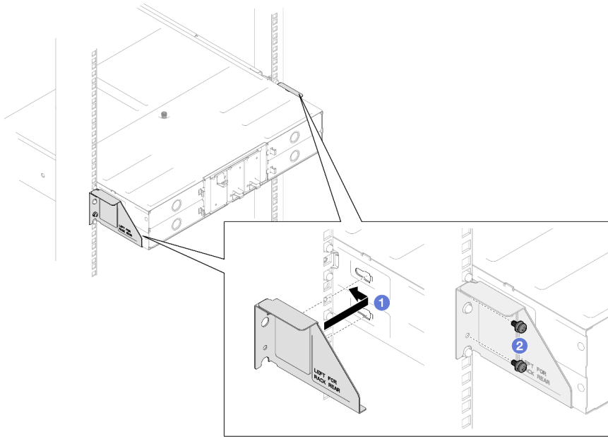
圖例 6. 安裝 29 吋或 28.31 吋深機架的出貨托架
