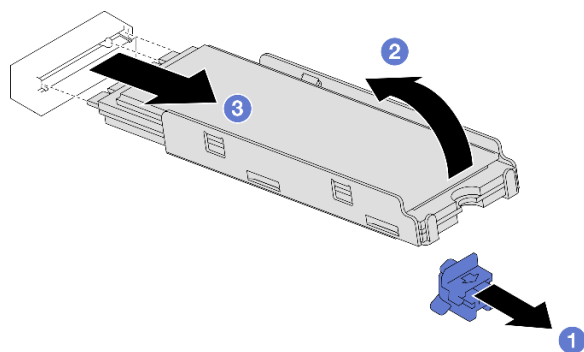
圖例 48. 卸下 M.2 硬碟
