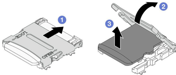
圖例 70. 卸下 MicroSD 卡
