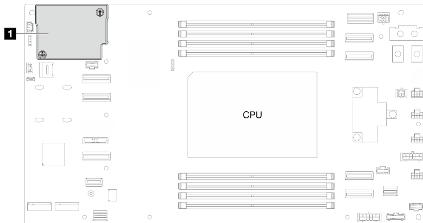
圖例 104. 韌體和 RoT 安全模組的位置
