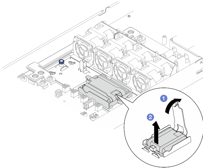
圖例 36. 卸下快閃記憶體電源模組
