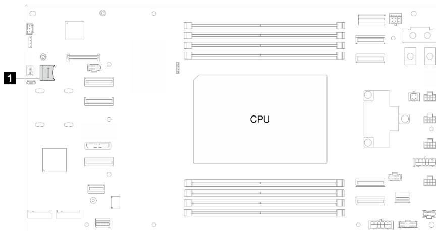
圖例 71. MicroSD 插座的位置
