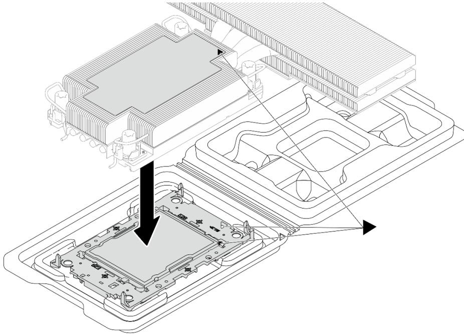
圖例 96. 將 PHM 和處理器裝到運送匣中
