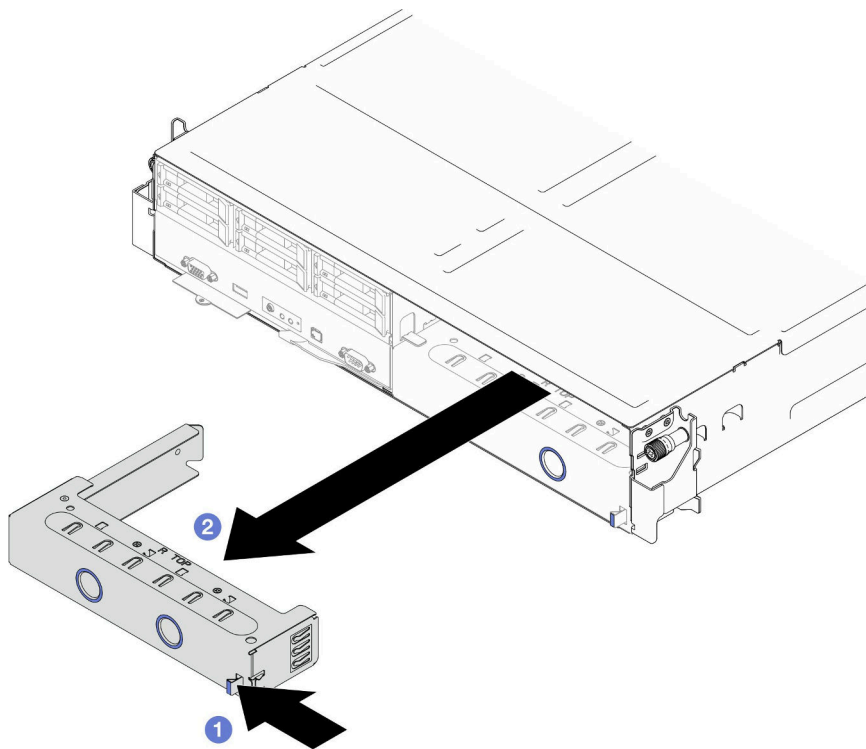
圖例 23. 卸下正面節點匣填充板
