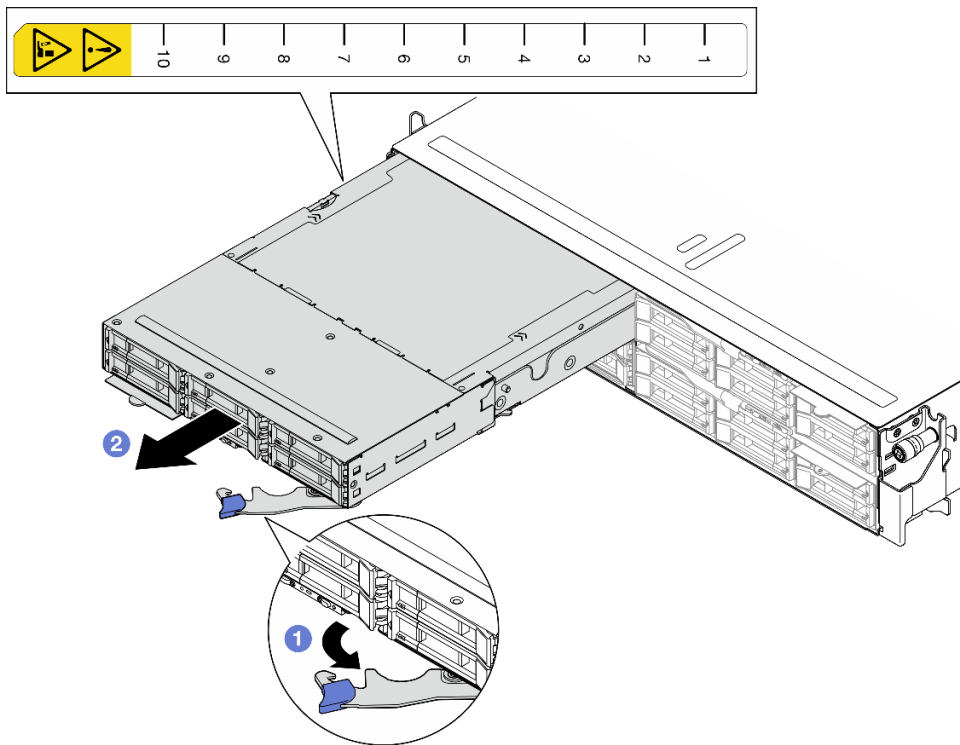
圖例 19. 節點從左匣卸下
