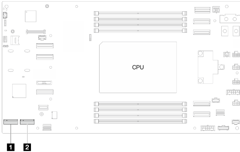
圖例 59. 主機板上 M.2 機槽的位置
