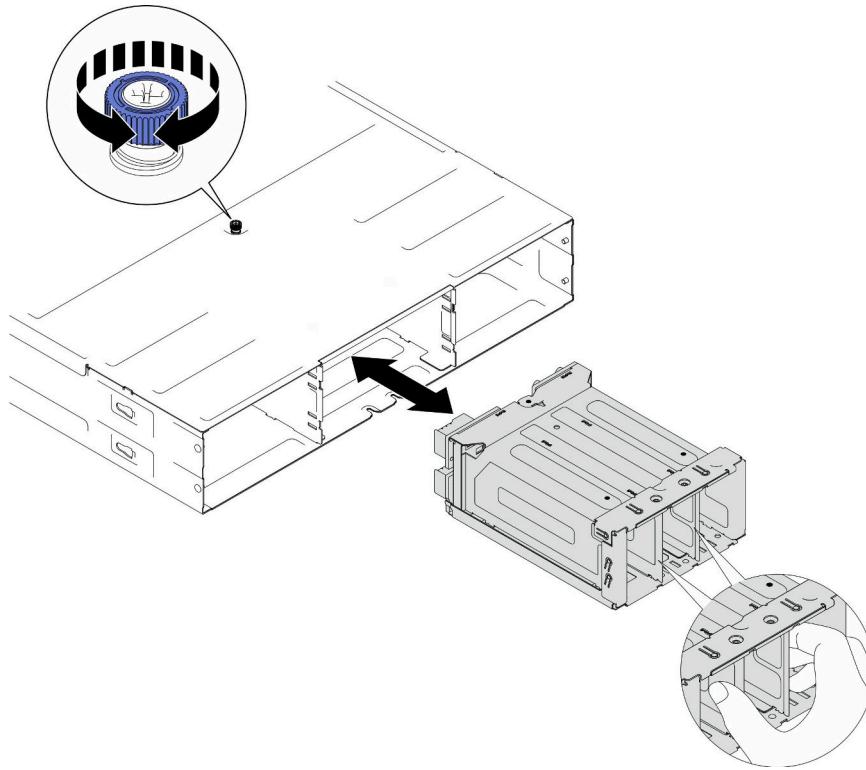
圖例 18. 安裝 PSU 機盒
