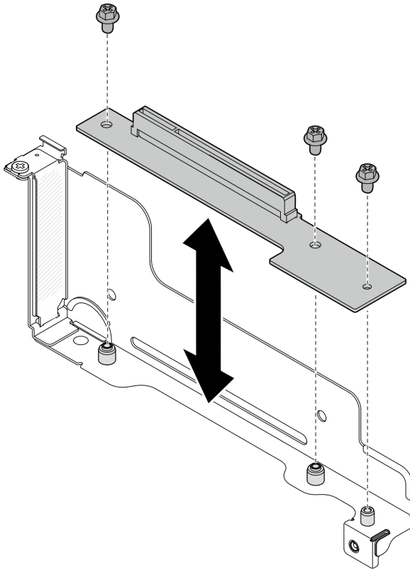
圖例 80. 更換 PCIe 擴充卡
