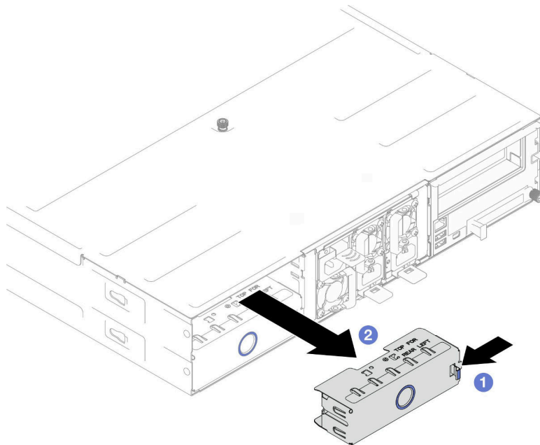
圖例 24. 卸下背面節點匣填充板
