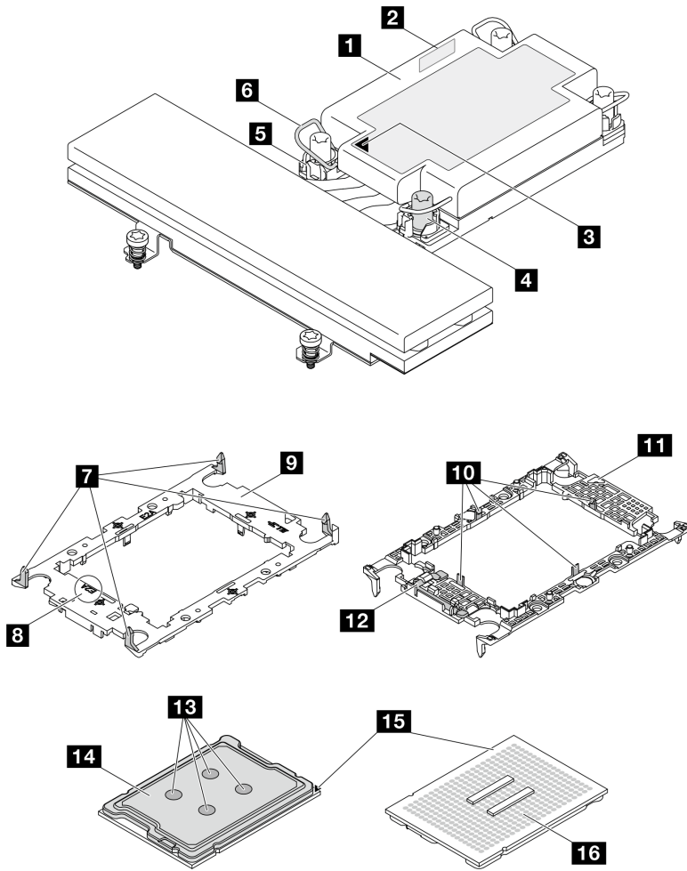
圖例 88. PHM 元件
