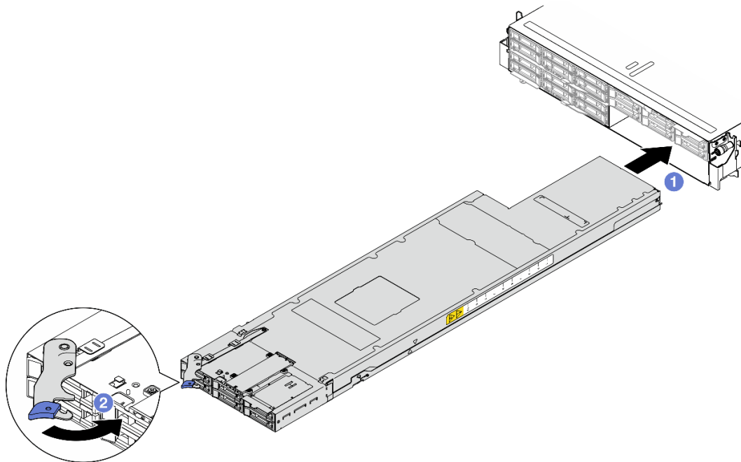
圖例 26. 節點安裝到右匣
