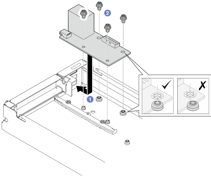
圖例 101. 安裝背面 I/O 模組
