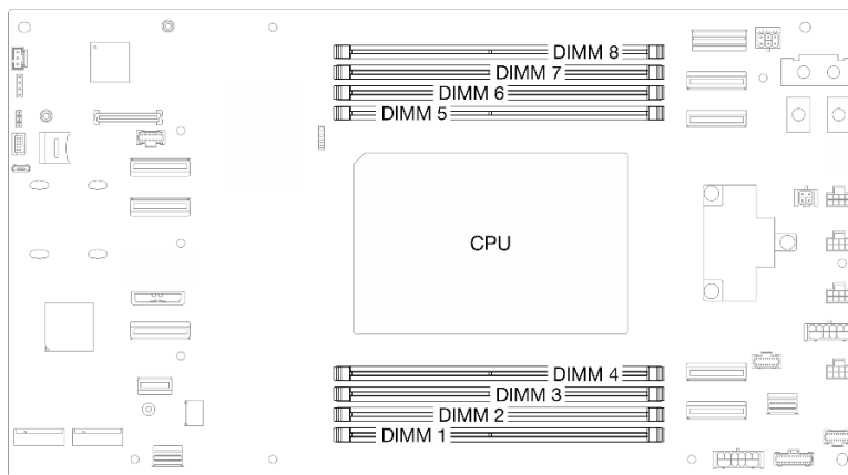
圖例 67. 記憶體模組和處理器佈置
