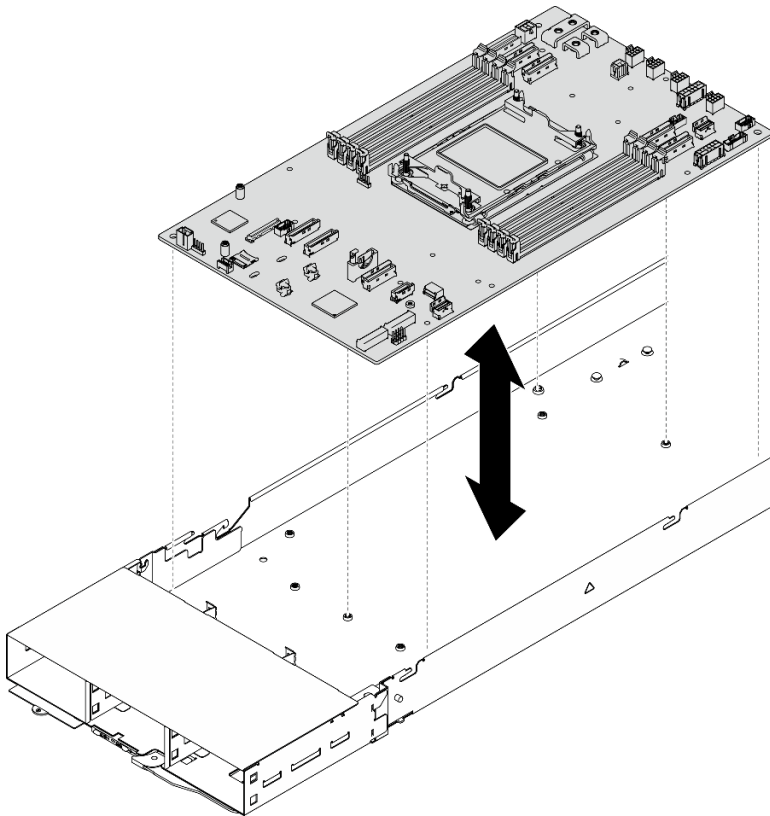
圖例 108. 卸下主機板
