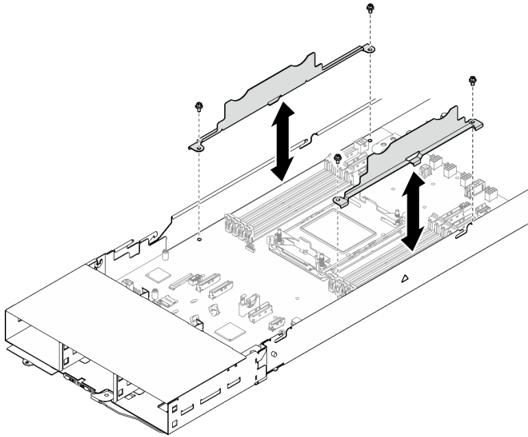
圖例 111. 安裝纜線壁
