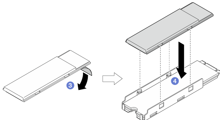
圖例 61. 將 M.2 散熱槽安裝到 M.2 匣
