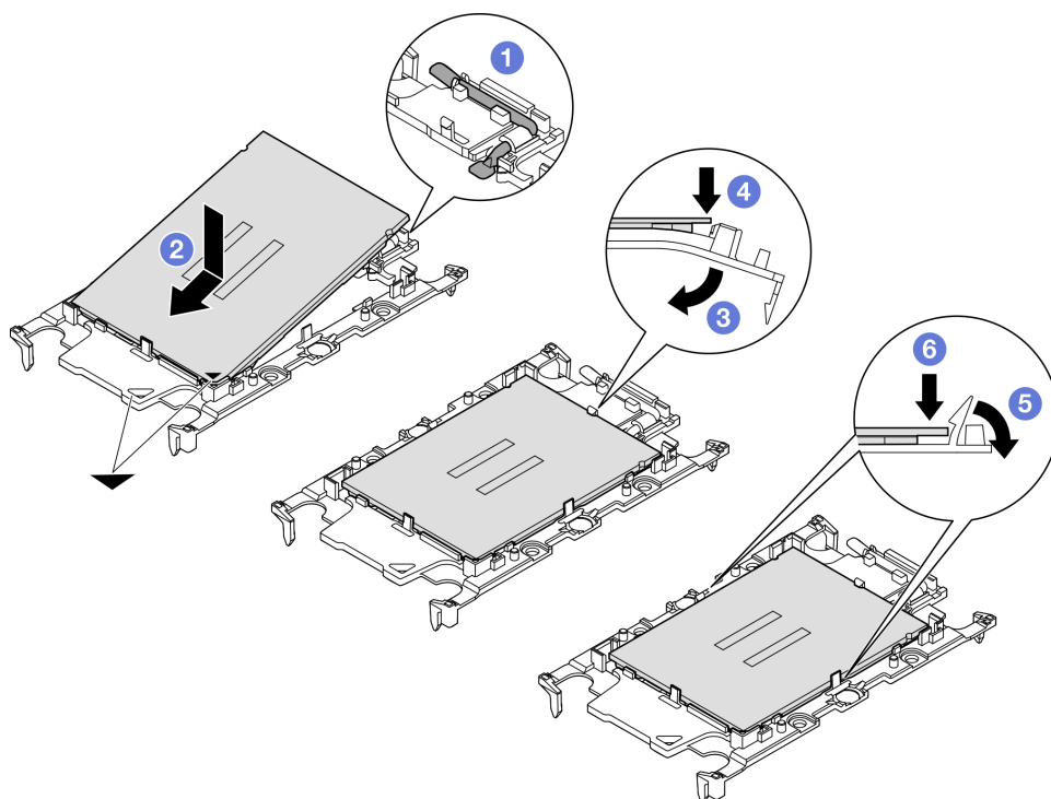
圖例 94. 安裝處理器支架
