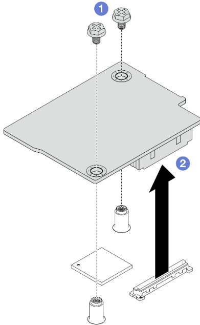
圖例 103. 卸下韌體和 RoT 安全模組
