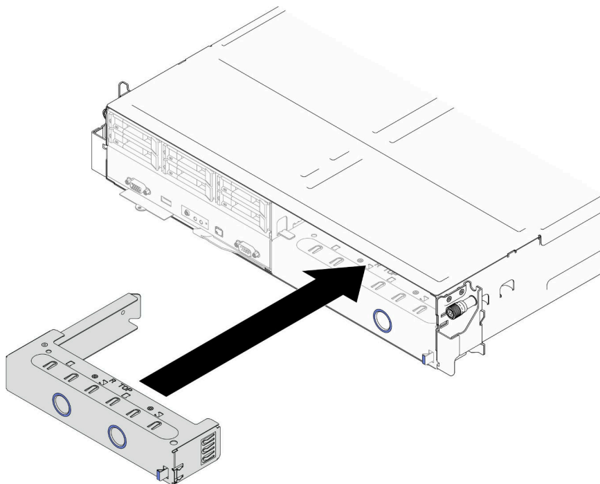
圖例 21. 安裝正面節點匣填充板
