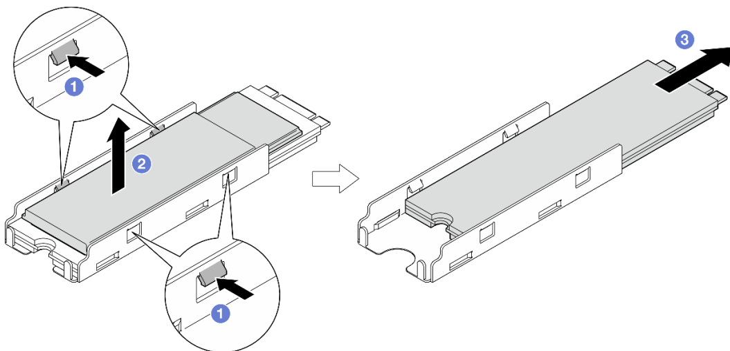
圖例 49. 卸下 M.2 散熱槽
