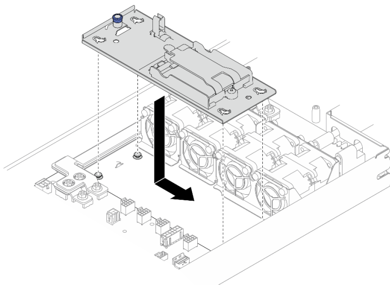
圖例 38. 安裝快閃記憶體電源模組匣
