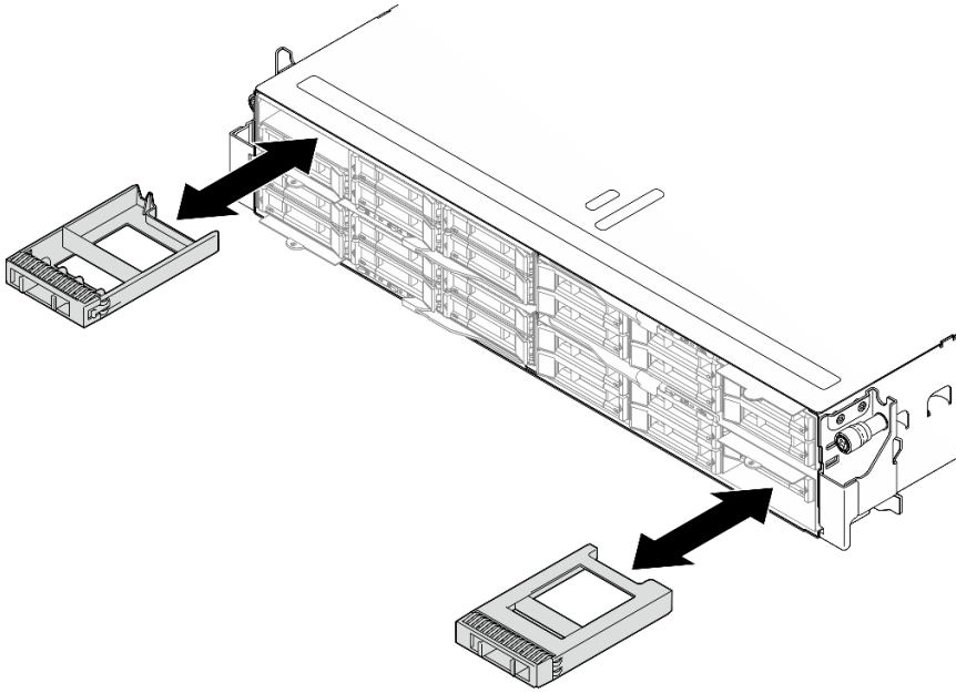
圖例 45. 更換硬碟填充板
