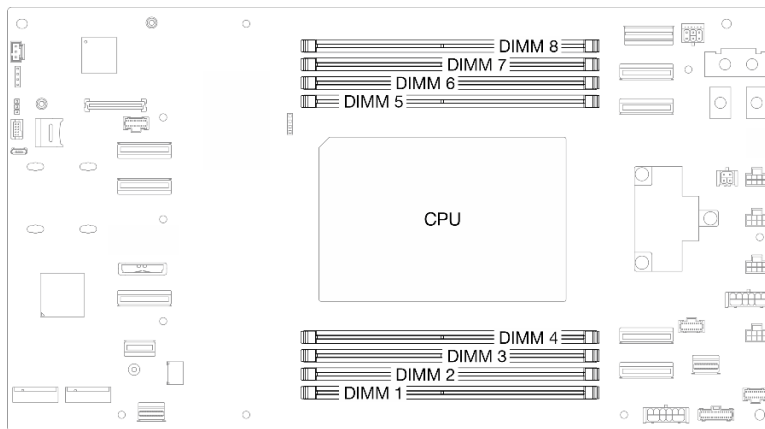
圖例 65. 記憶體模組和處理器佈置
