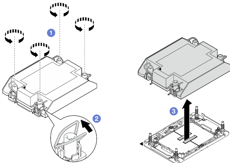
圖例 89. 卸下標準 PHM
