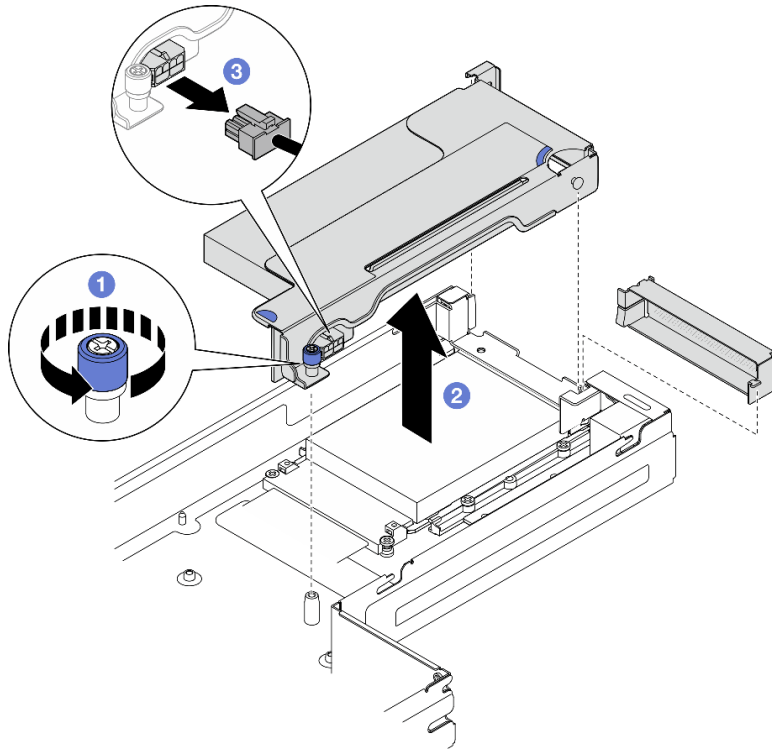
圖例 75. 卸下 PCIe 擴充卡組件
