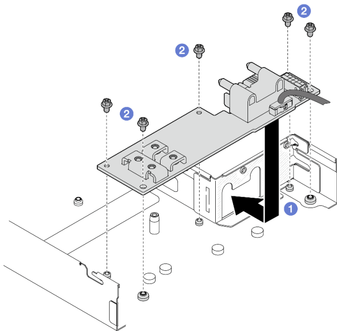
圖例 87. 安裝電源配送板
