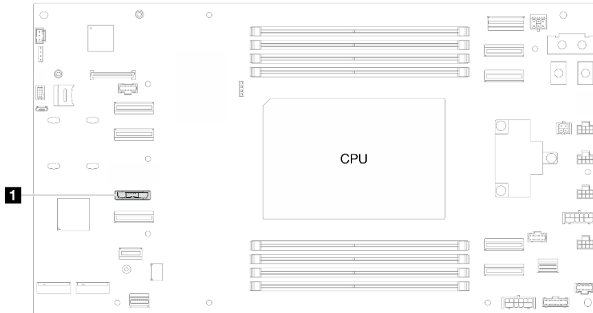
圖例 27. CMOS 電池插座的位置
