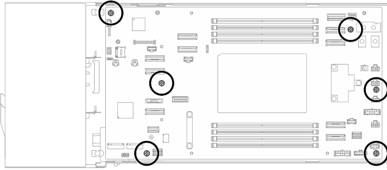
圖例 107. 主機板螺絲位置
