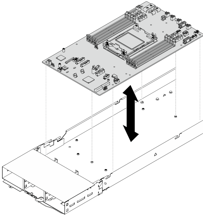
圖例 109. 安裝主機板
