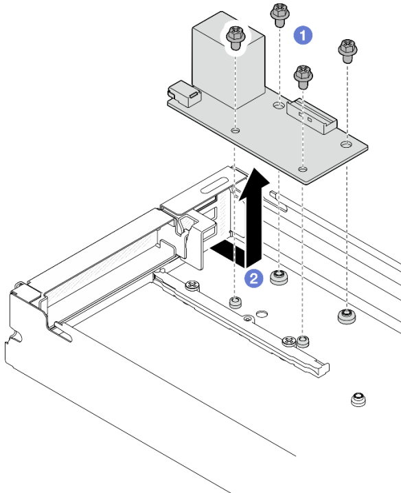
圖例 100. 卸下背面 I/O 模組
