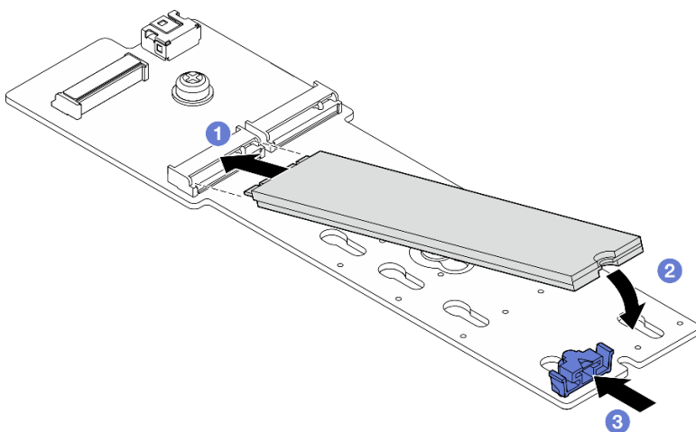
圖例 64. 安裝 M.2 硬碟
