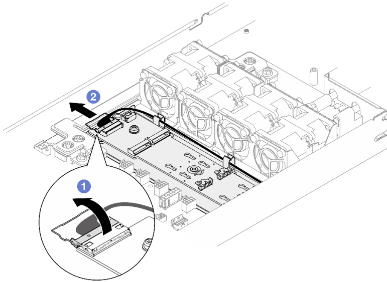
圖例 51. 從 M.2 開機配接卡拔掉纜線
