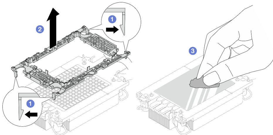
圖例 92. 將處理器支架與散熱槽分開
