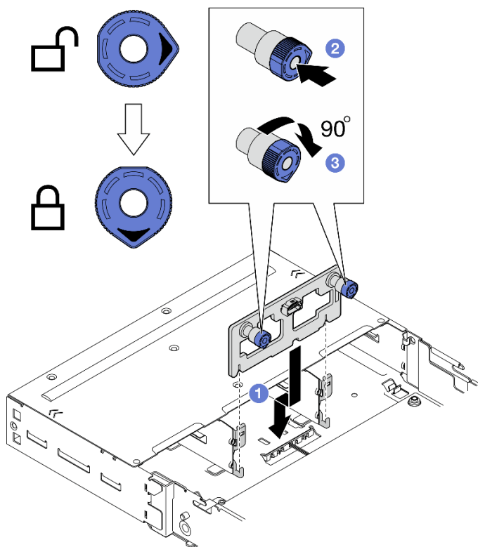
圖例 42. 安裝正面 I/O 板
