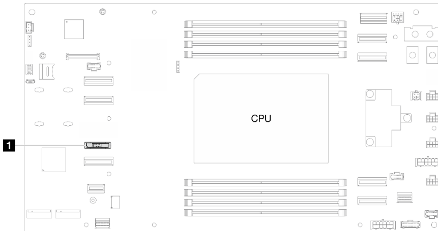
圖例 29. CMOS 電池插座的位置
