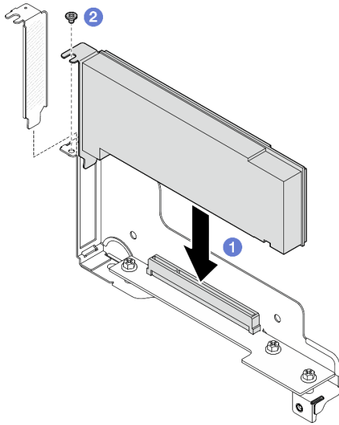
圖例 79. 安裝 PCIe 配接卡
