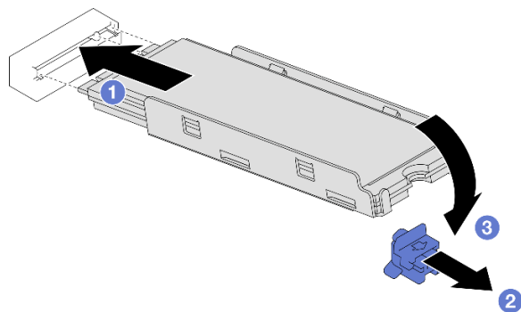
圖例 62. 安裝 M.2 硬碟
