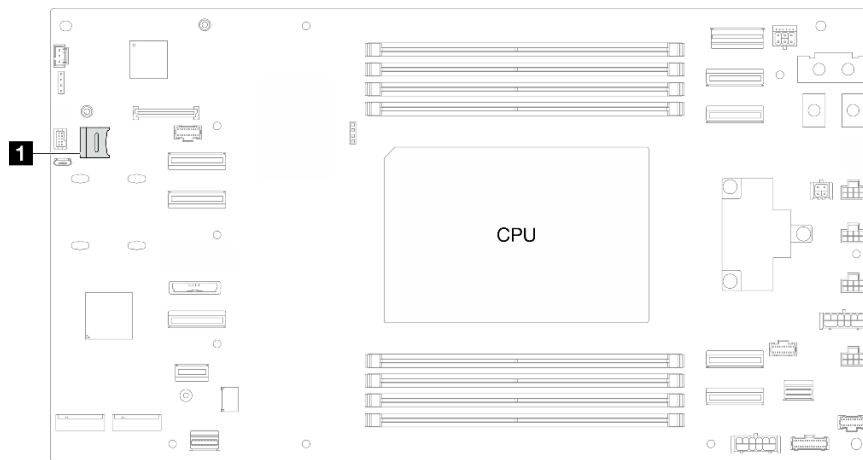
圖例 69. MicroSD 插座的位置
