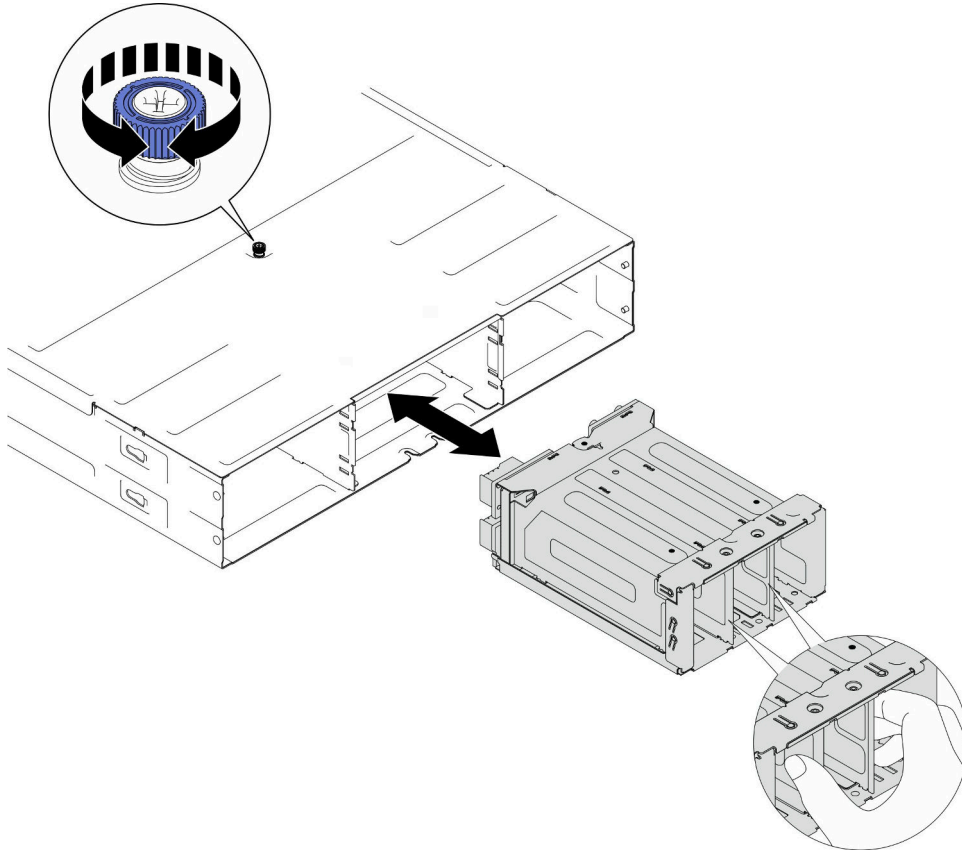
圖例 15. 卸下 PSU 機盒
