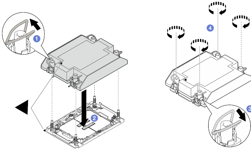
圖例 98. 安裝標準 PHM
