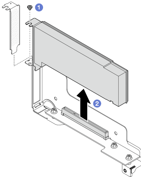
圖例 77. 卸下 PCIe 配接卡
