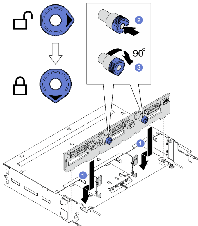
圖例 32. 安裝硬碟背板
