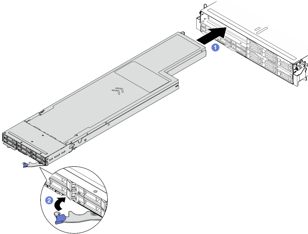
圖例 25. 節點安裝到左匣
