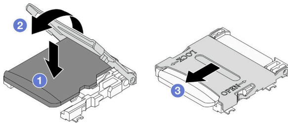
圖例 72. 安裝 MicroSD 卡
