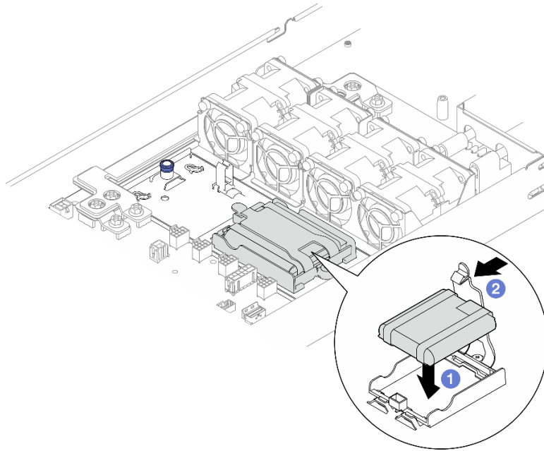
圖例 39. 安裝快閃記憶體電源模組
