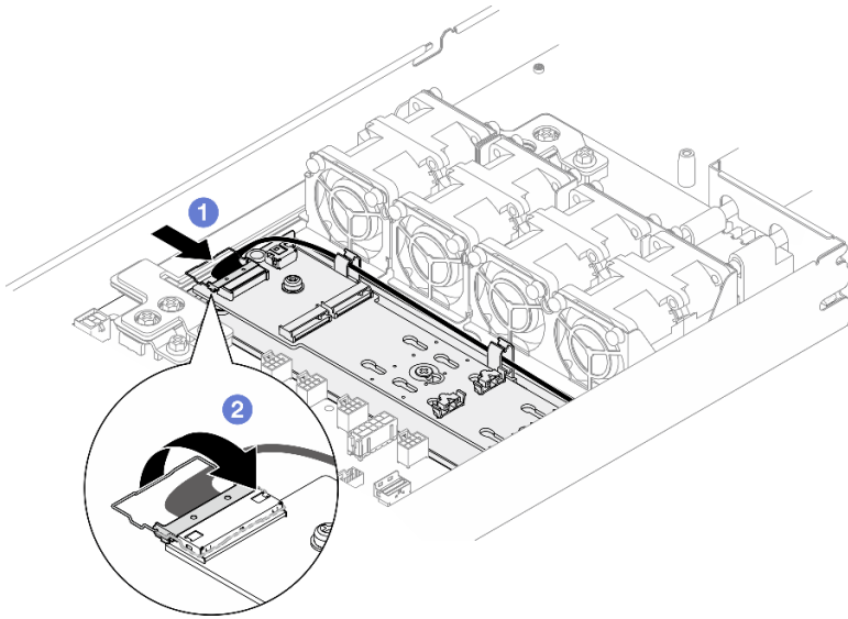
圖例 56. 將纜線連接到 SATA/NVMe M.2 開機配接卡
