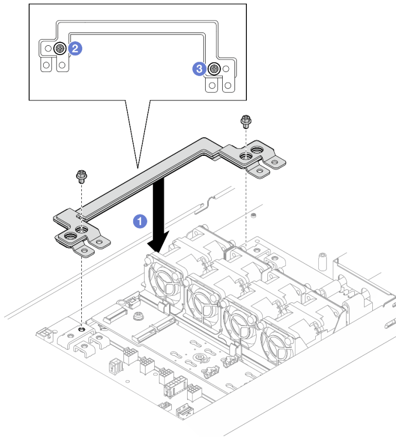
圖例 84. 安裝電源匯流排桿
