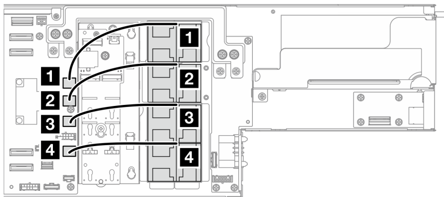
圖例 35. 風扇纜線佈線
