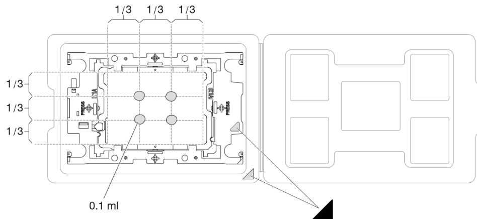
圖例 95. 運送匣中的處理器塗上散熱膏
