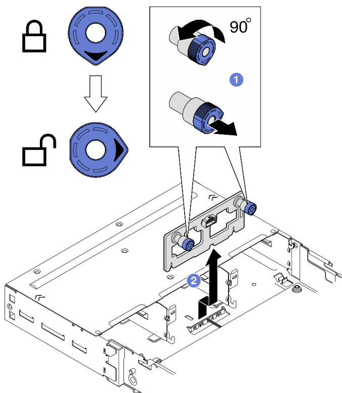
圖例 41. 卸下正面 I/O 板
