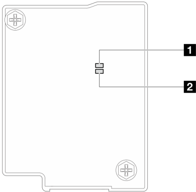
圖例 118. 韌體和 RoT 安全模組上的 LED
