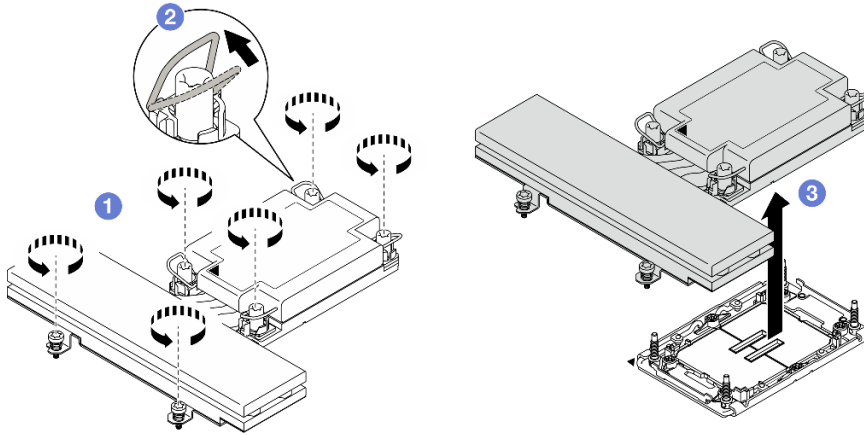
圖例 90. 卸下效能 PHM
