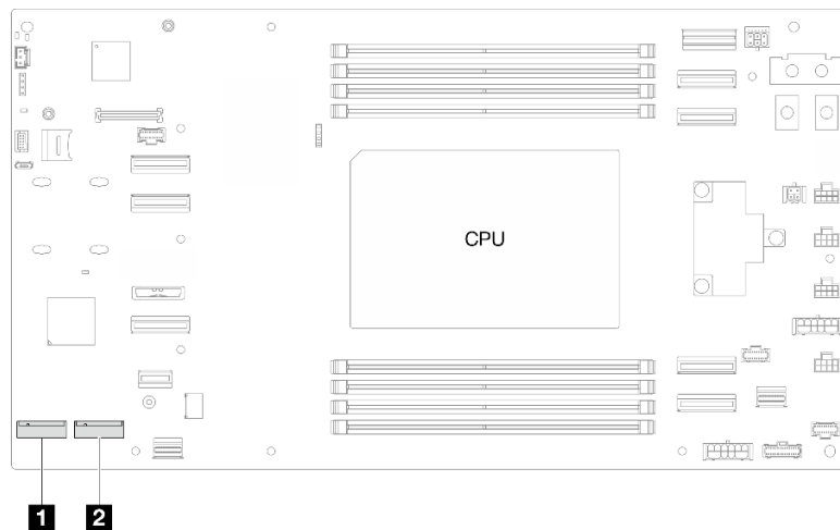
圖例 47. 主機板上 M.2 機槽的位置
