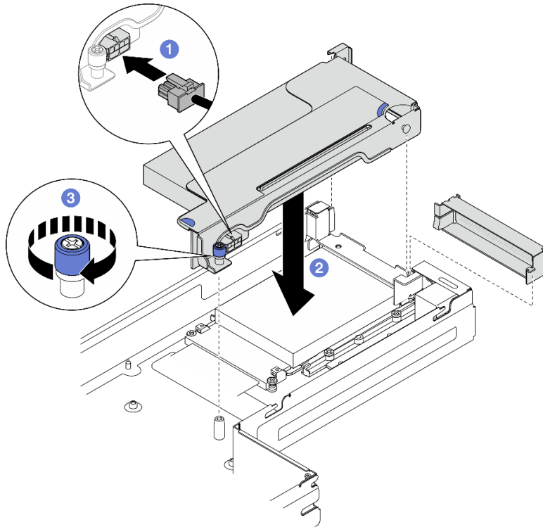
圖例 81. 安裝 PCIe 擴充卡組件
