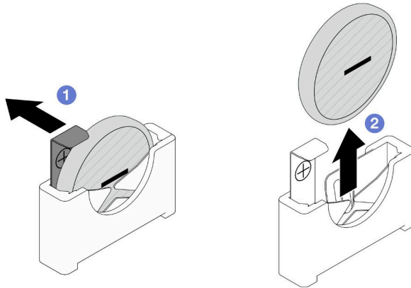
圖例 28. 卸下 CMOS 電池
