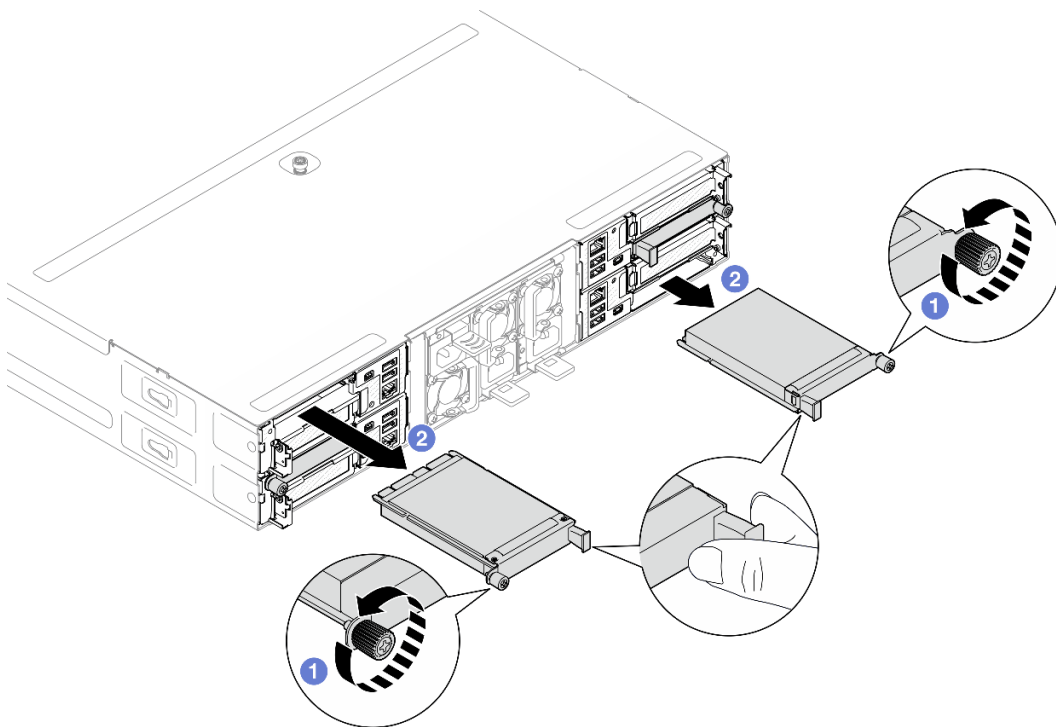
圖例 74. 安裝背面 OCP 模組
