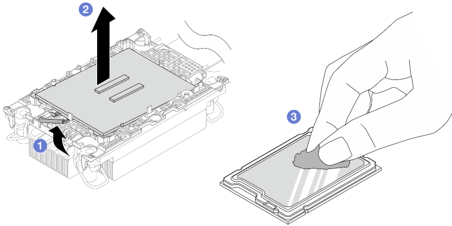
圖例 91. 將處理器與散熱槽和支架分開
