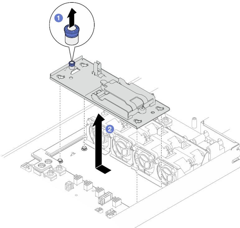
圖例 37. 卸下快閃記憶體電源模組匣
