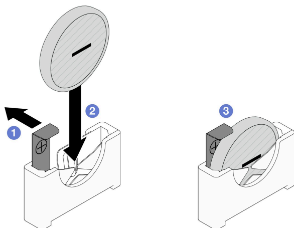
圖例 30. 安裝 CMOS 電池
