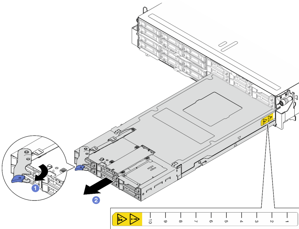
圖例 20. 節點從右匣卸下
