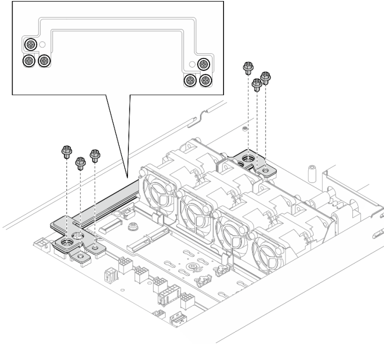
圖例 82. 卸下電源匯流排桿的外側螺絲
