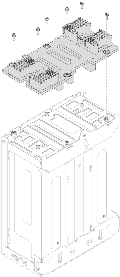
圖例 16. 卸下機箱中板
