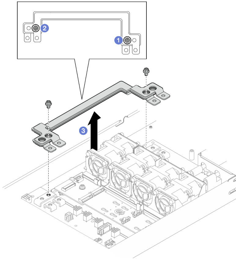
圖例 83. 卸下電源匯流排桿
