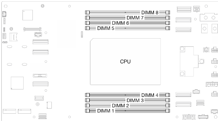
圖例 1. 記憶體模組和處理器佈置
