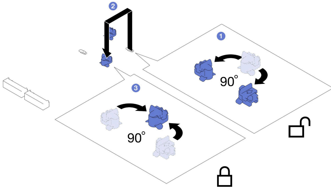
圖例 57. 調整 M.2 磁碟機固定器
