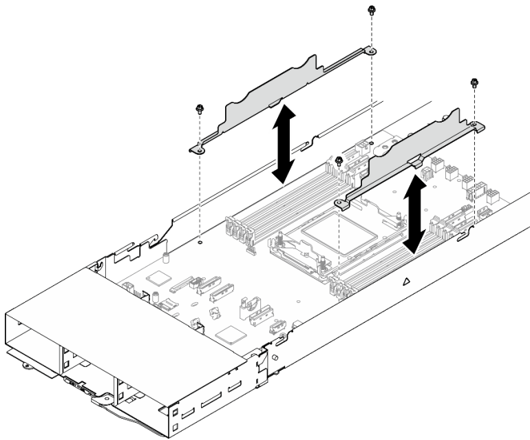
圖例 106. 卸下纜線壁
