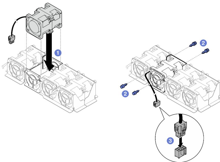
圖例 34. 安裝風扇
