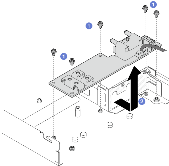
圖例 86. 卸下電源配送板
