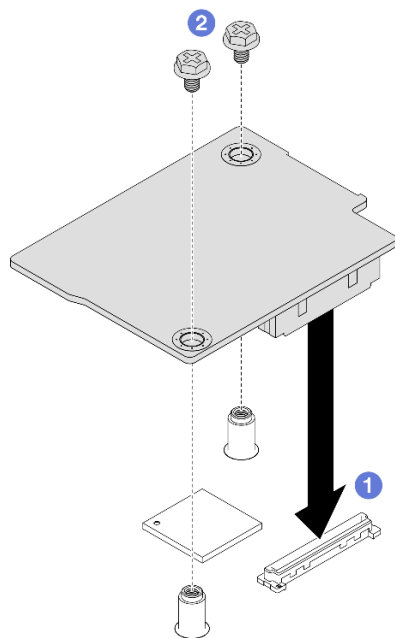
圖例 105. 安裝韌體和 RoT 安全模組
