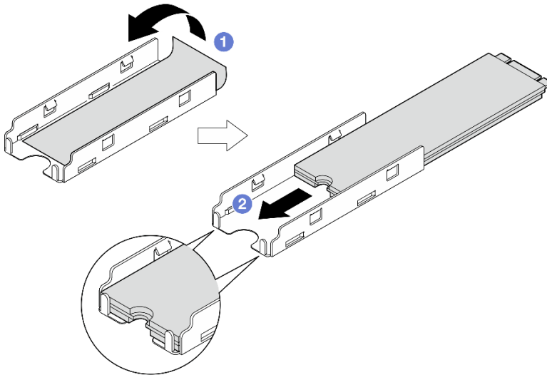
圖例 60. 將散熱墊和 M.2 硬碟安裝到匣中
