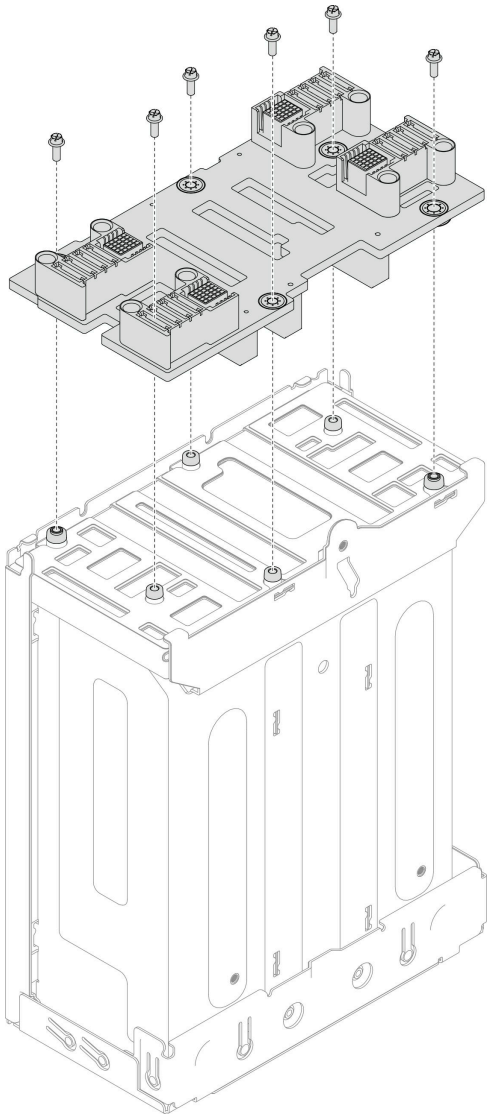
圖例 17. 安裝機箱中板
