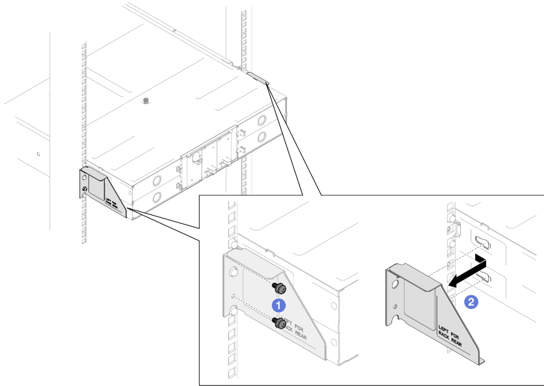
圖例 2. 卸下 29 吋或 28.31 吋深機架的出貨托架
