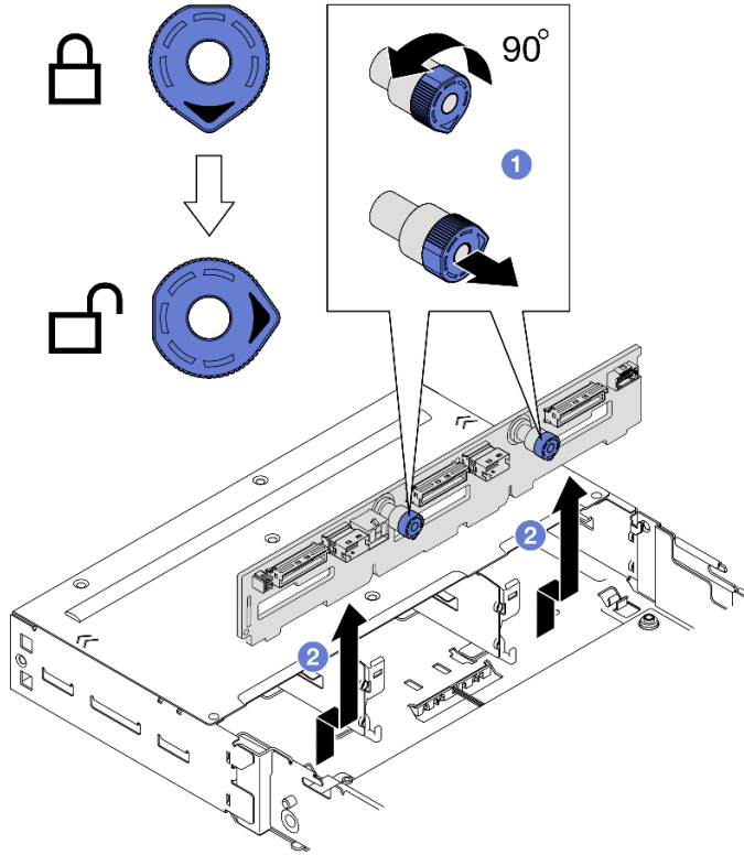
圖例 31. 卸下硬碟背板
