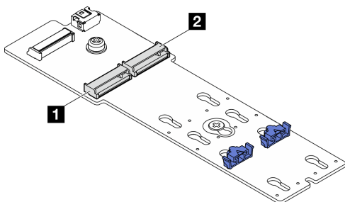
圖例 63. M.2 硬碟插槽
