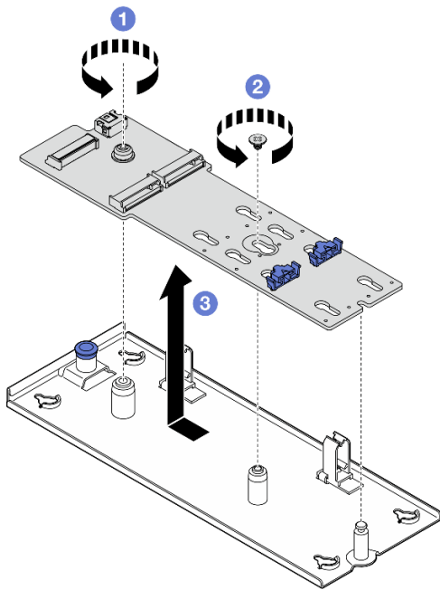
圖例 53. 卸下 M.2 開機配接卡
