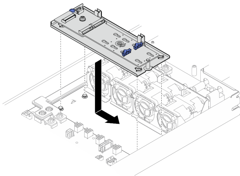
圖例 55. 安裝 M.2 開機配接卡匣
