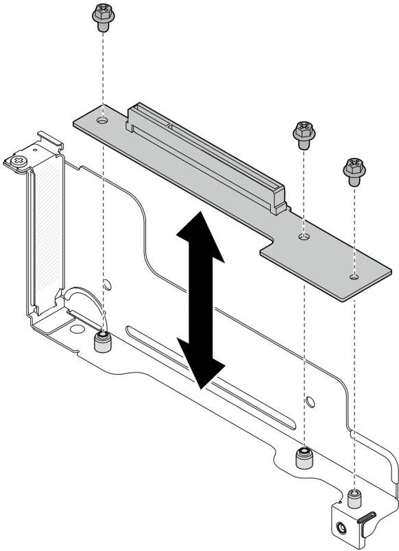
圖例 76. 更換 PCIe 擴充卡
