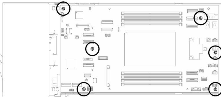
圖例 110. 主機板螺絲位置
