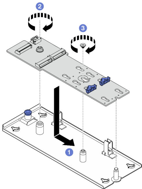
圖例 54. 安裝 M.2 開機配接卡
