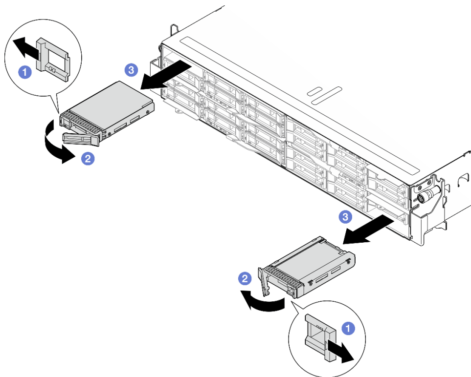
圖例 43. 卸下固態硬碟
