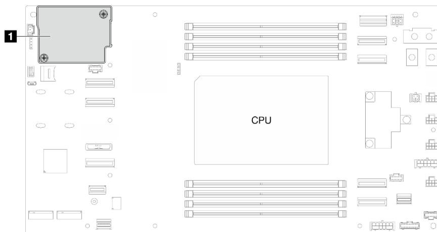
圖例 102. 韌體和 RoT 安全模組的位置
