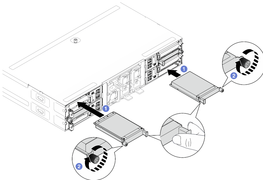
圖例 73. 卸下背面 OCP 模組
