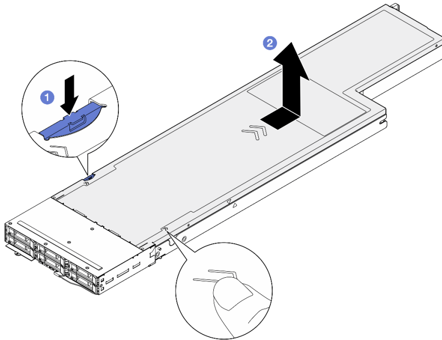
圖例 112. 卸下上蓋
