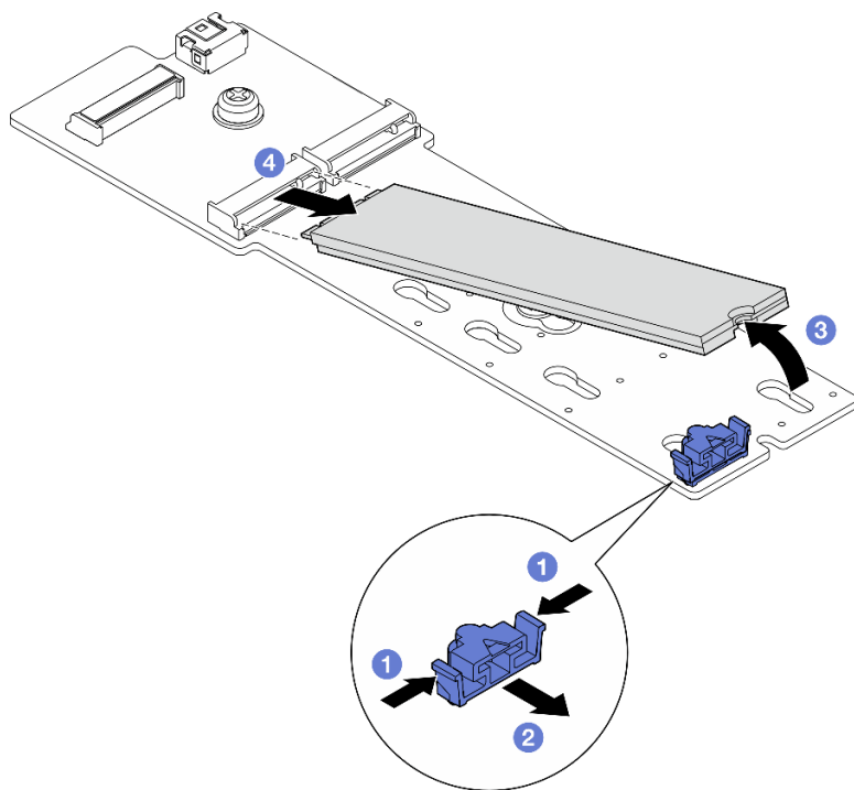
圖例 50. 卸下 M.2 硬碟
