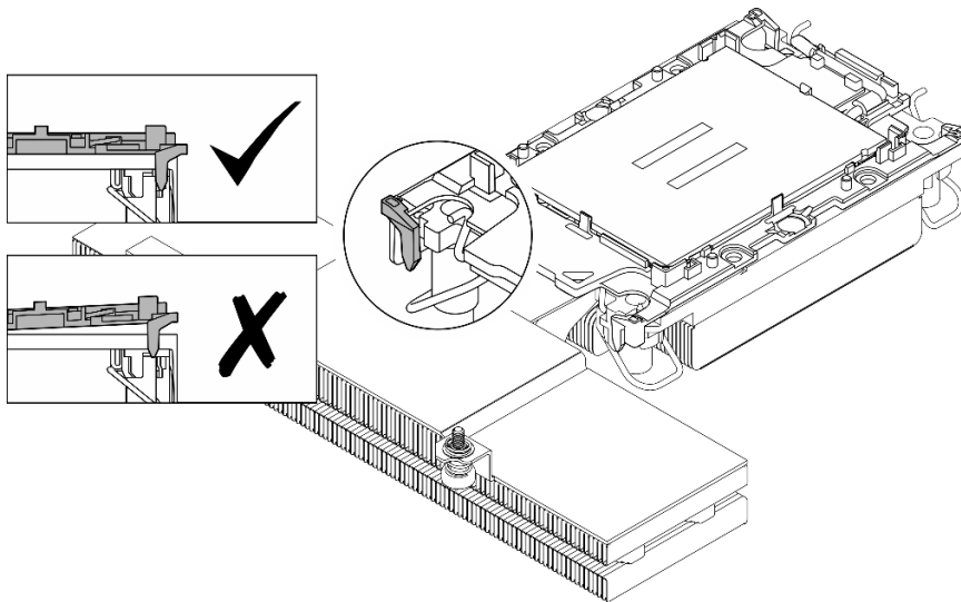
圖例 97. 目視檢查支架夾
