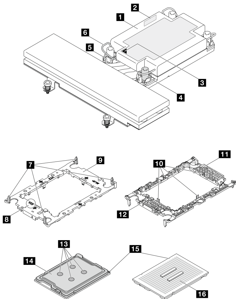
圖例 93. PHM 元件
