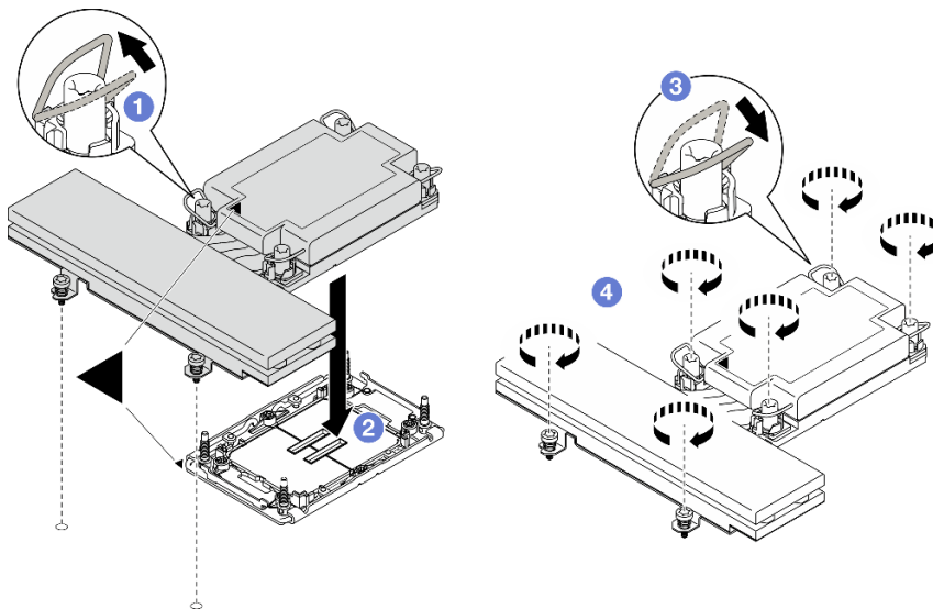
圖例 99. 安裝效能 PHM
