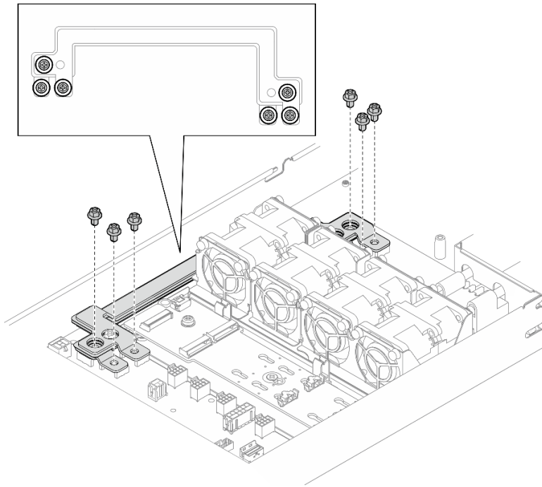
圖例 85. 安裝電源匯流排桿外側螺絲
