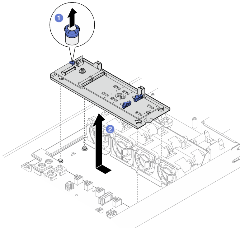
圖例 52. 卸下 M.2 開機配接卡匣
