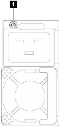
圖例 117. 電源供應器 LED
