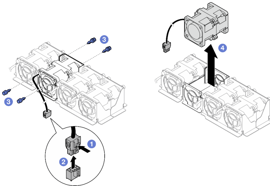
圖例 33. 卸下風扇
