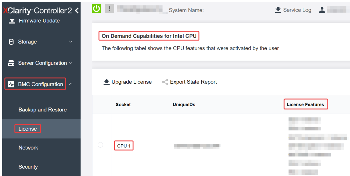
Abbildung 25. In einem Prozessor installierte Intel On Demand-Funktionen in der XCC-Webschnittstelle überprüfen
