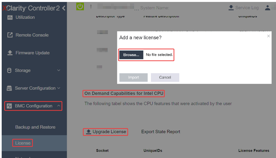
Abbildung 23. Aktivierungsschlüssel über XCC-Webschnittstelle hochladen
