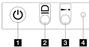
Abbildung 12. Tasten und Anzeigen der vorderen Bedienerkonsole
