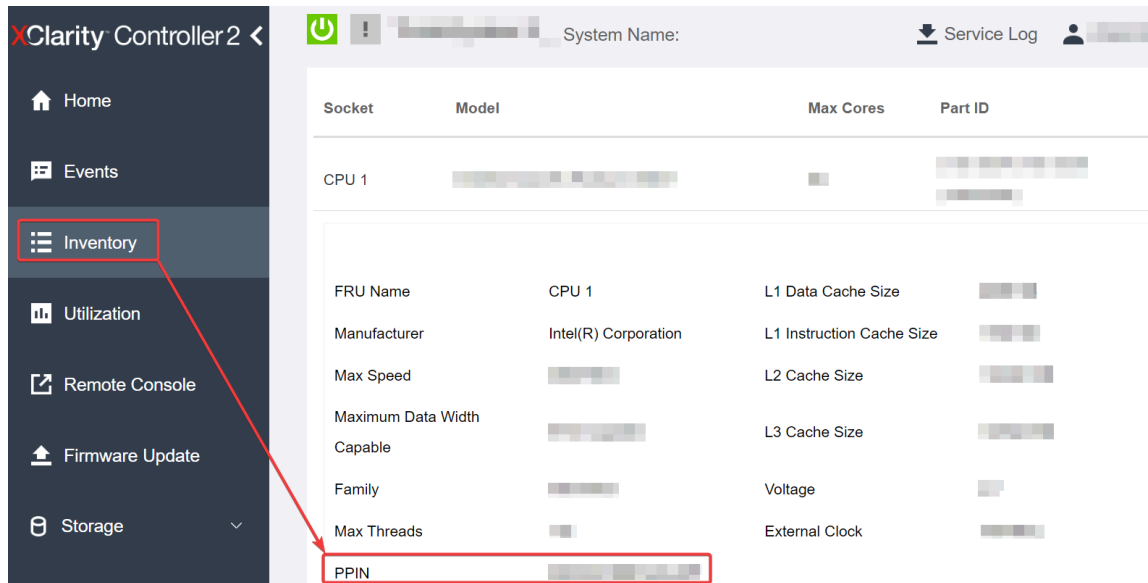
Abbildung 22. PPIN über XCC-Webschnittstelle lesen
