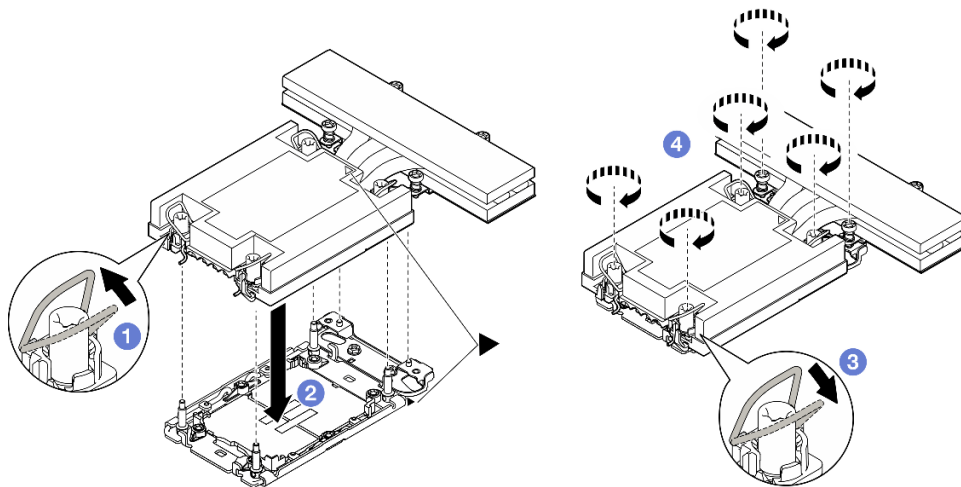
Figura 93. Instalación de un PHM de rendimiento 1U para la configuración de un procesador
