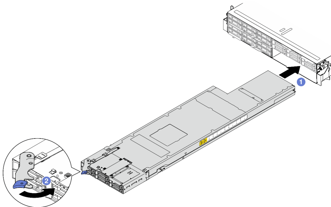
Figura 31. Instalación de un nodo en una bandeja derecha
