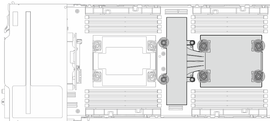
Figura 80. Ubicación de PHM para la configuración de dos procesadores
