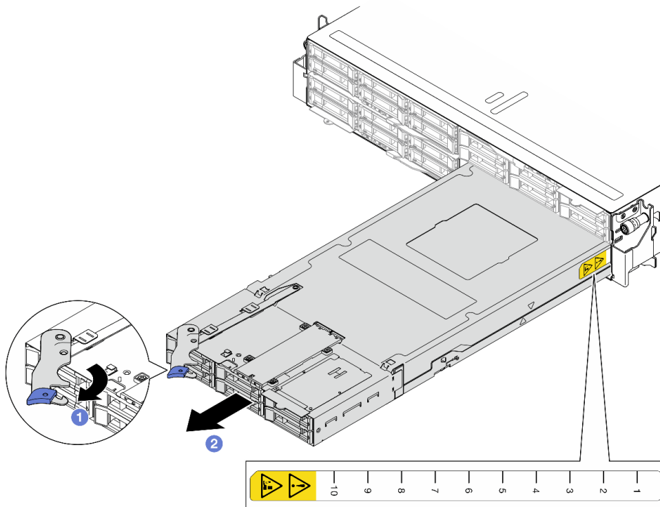
Figura 21. Extracción del nodo de una bandeja derecha
