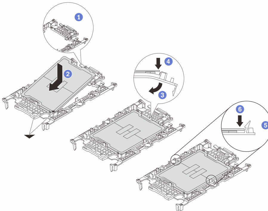
Figura 88. Instalación del transportador del procesador
