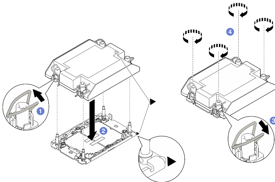
Figura 95. Instalación de un PHM estándar 1U para la configuración de dos procesadores
