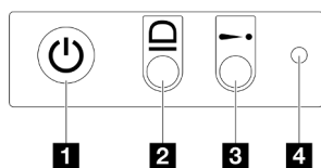
Figura 133. Botones y LED del panel frontal del operador
