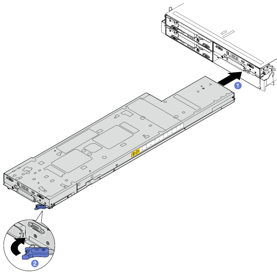
Figura 30. Instalación de un nodo en una bandeja derecha
