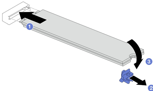
Figura 54. Instalación de una unidad M.2
