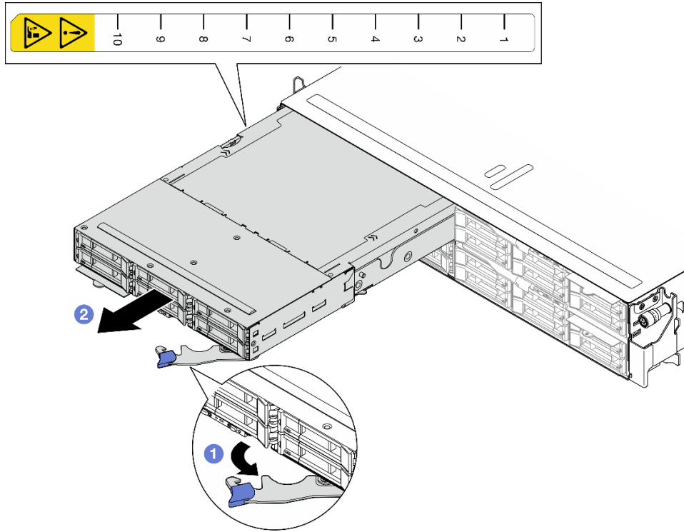
Figura 18. Extracción del nodo de una bandeja izquierda
