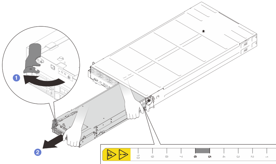
Figura 19. Extracción del nodo de la bandeja derecha
