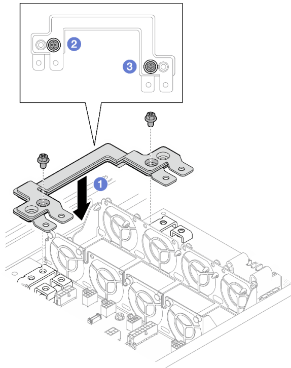
Figura 74. Instalación de la barra de bus de alimentación
