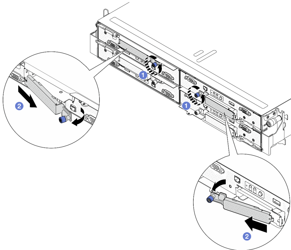
Figura 44. Extracción de la cubierta del compartimiento de la unidad E3.S
