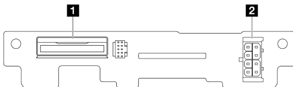
Figura 120. Conectores de la placa posterior de la unidad E3.S
