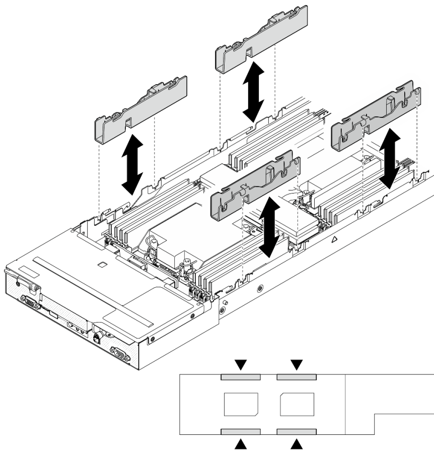
Figura 115. Sustitución del conducto del cable (configuración de dos procesadores)
