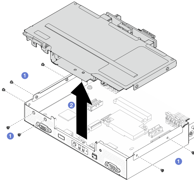
Figura 36. Extracción del conjunto del compartimiento de la unidad
