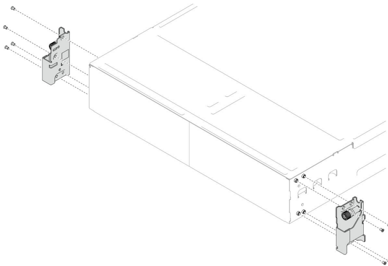
Figura 7. Instalación de los soportes EIA
