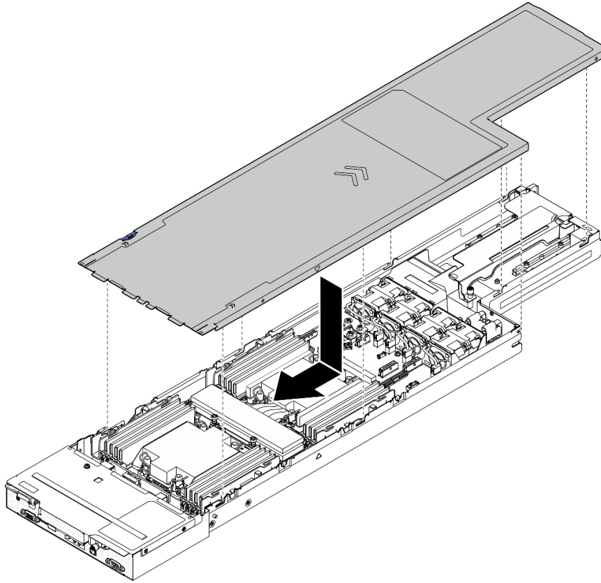
Figura 118. Instalación de la cubierta superior
