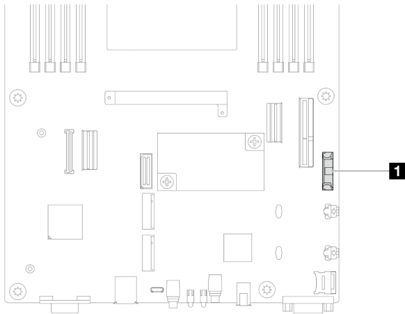
Figura 32. Ubicación del zócalo de la batería CMOS
