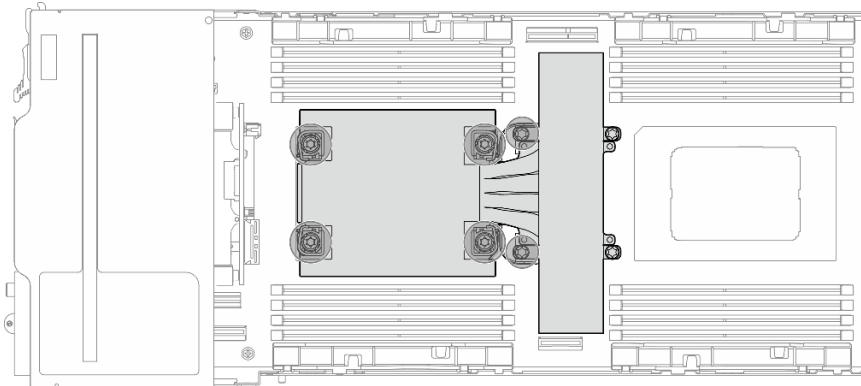
Figura 79. Ubicación de PHM para la configuración de un solo procesador
