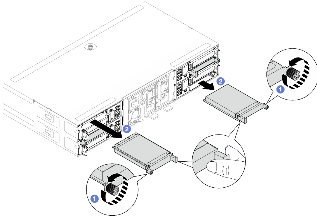
Figura 63. Extracción del módulo de OCP posterior
