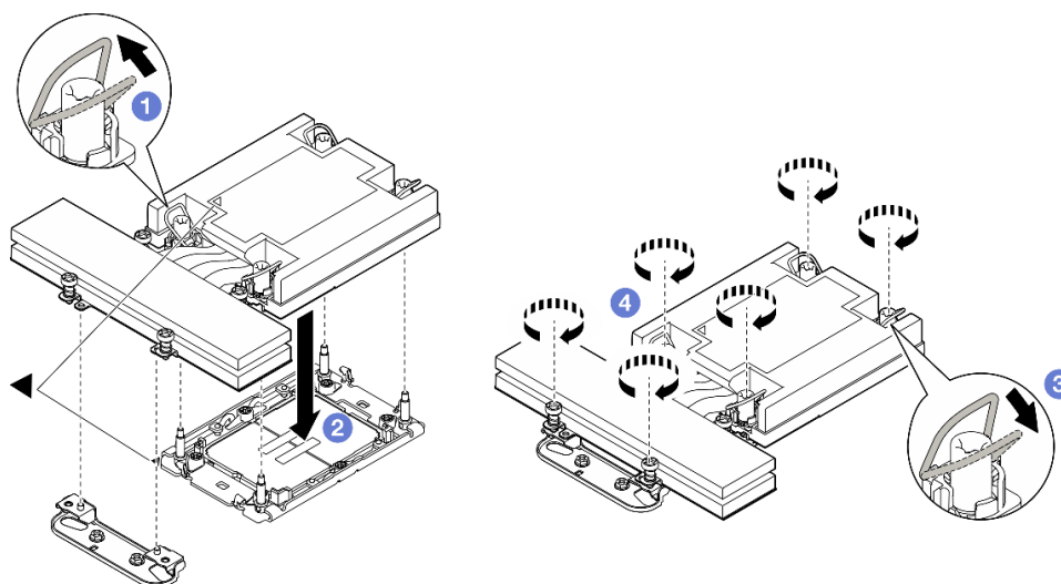
Figura 96. Instalación de un PHM de rendimiento 1U para la configuración de dos procesadores
