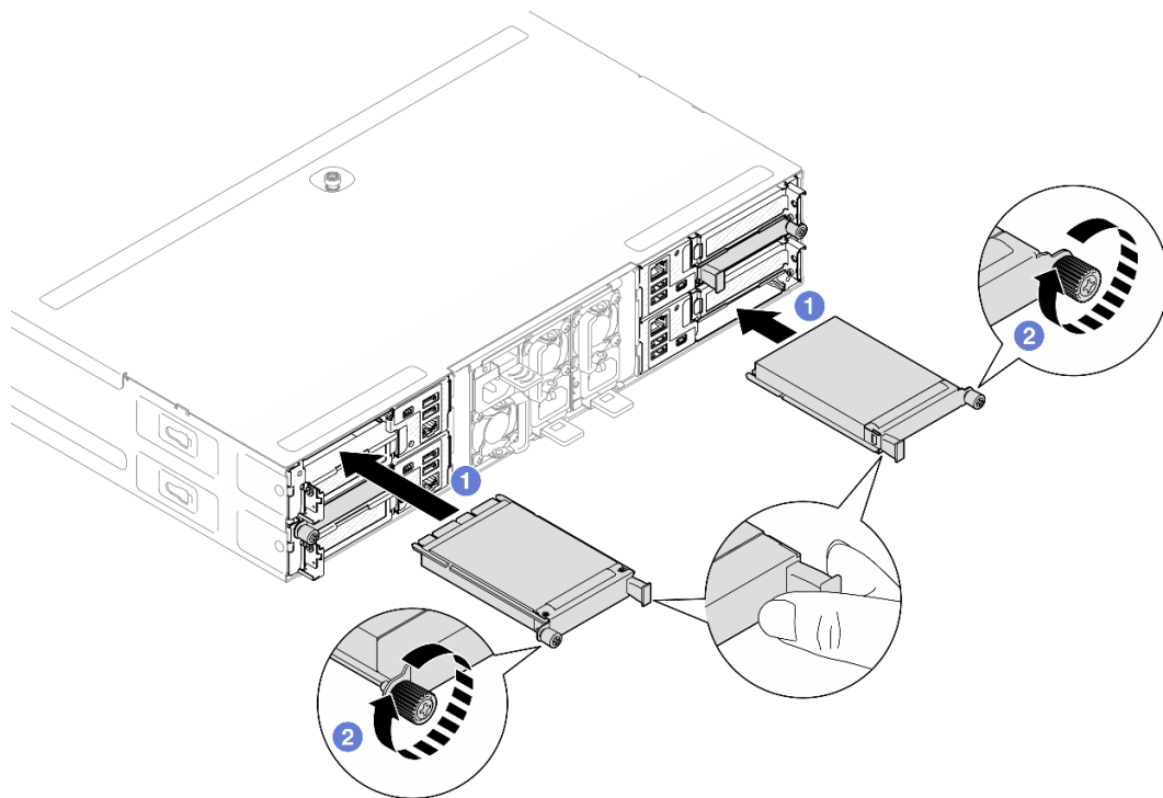
Figura 64. Instalación del módulo de OCP posterior
