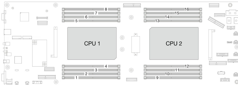
Figura 57. Diseño de los módulos de memoria y el procesador
