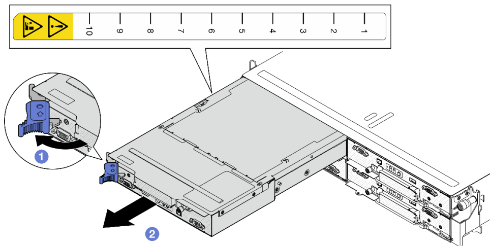
Figura 17. Extracción del nodo de una bandeja izquierda
