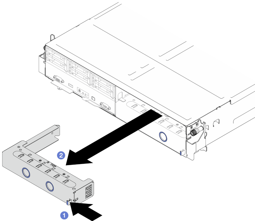
Figura 24. Extracción de un relleno de la bandeja del nodo frontal
