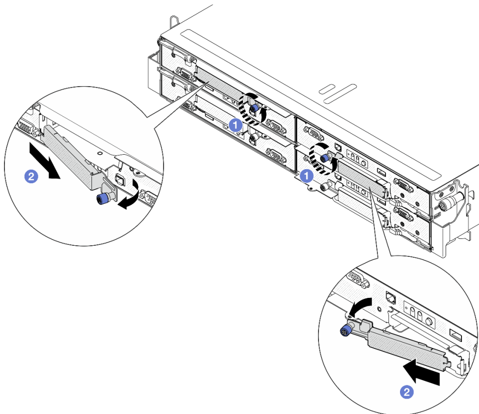
Figura 47. Extracción de la cubierta del compartimiento de la unidad E3.S
