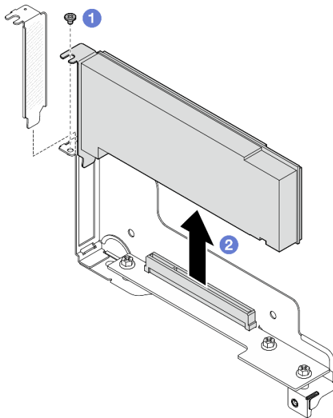
Figura 67. Extracción de un adaptador PCIe
