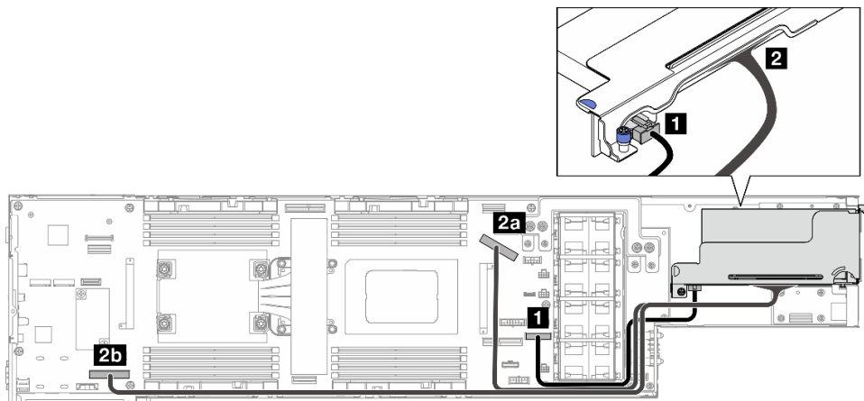
Figura 125. Disposición de cables de la expansión PCIe – un procesador
