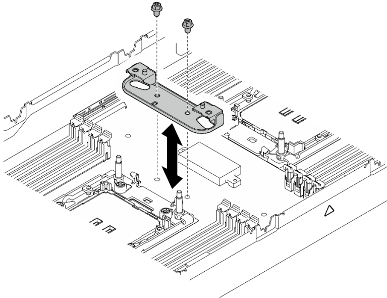
Figura 105. Sustitución de la abrazadera de soporte del disipador de calor
