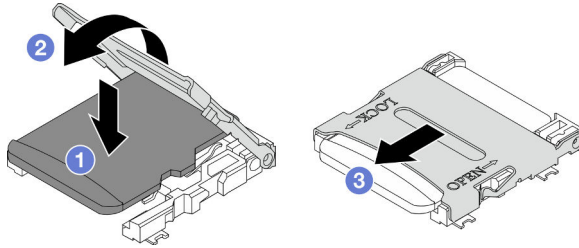
Figura 62. Instalación de una tarjeta MicroSD
