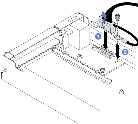
Figura 100. Instalación del cable de E/S posterior y del cable de conexión a tierra
