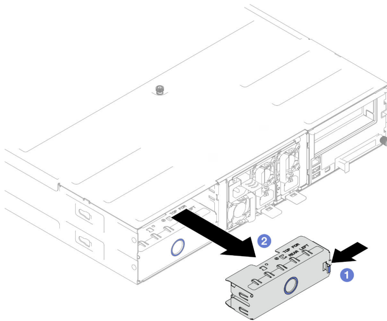
Figura 25. Extracción de un relleno de la bandeja del nodo posterior
