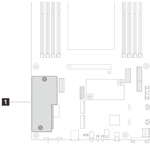
Figura 103. Ubicación del Firmware y módulo de seguridad de RoT
