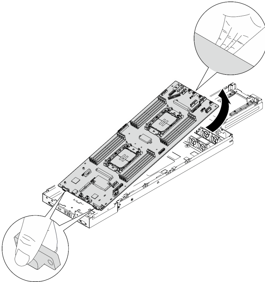
Figura 110. Extracción de la placa de sistema
