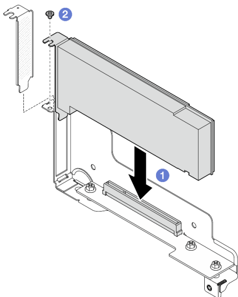
Figura 69. Instalación de un adaptador PCIe
