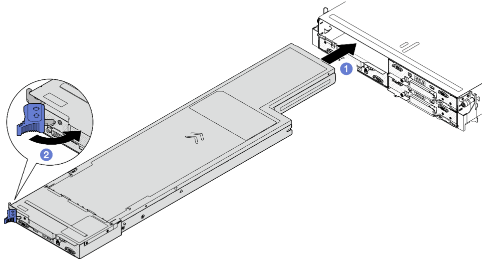
Figura 27. Instalación de un nodo en una bandeja izquierda
