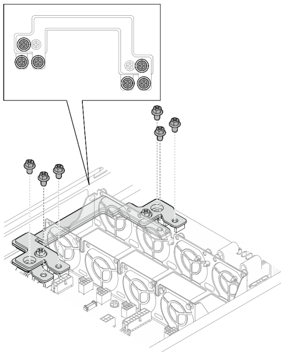
Figura 72. Extracción de los tornillos externos de la barra de bus de alimentación
