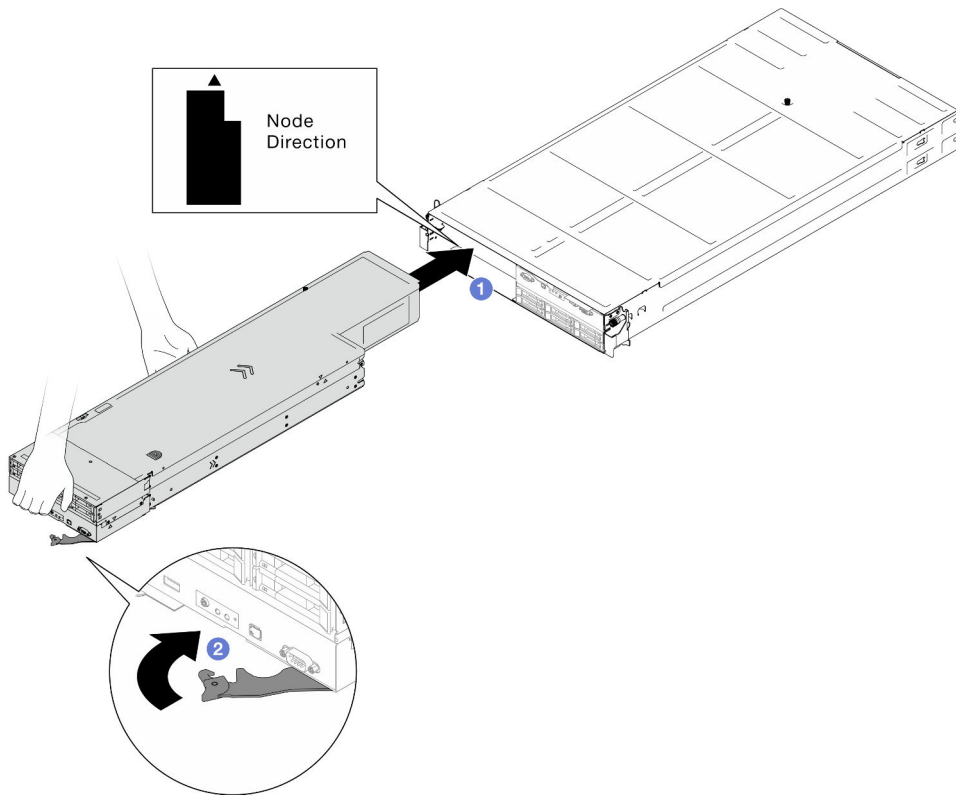
Figura 26. Instalación de un nodo en la bandeja izquierda
