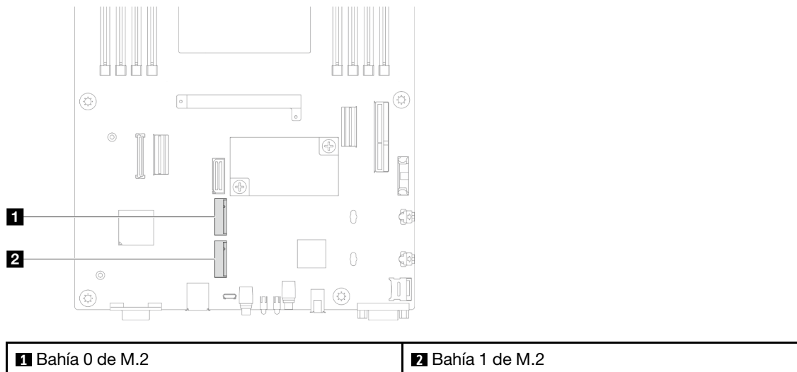
Figura 50. Ubicación de las bahías M.2 en la placa del sistema
