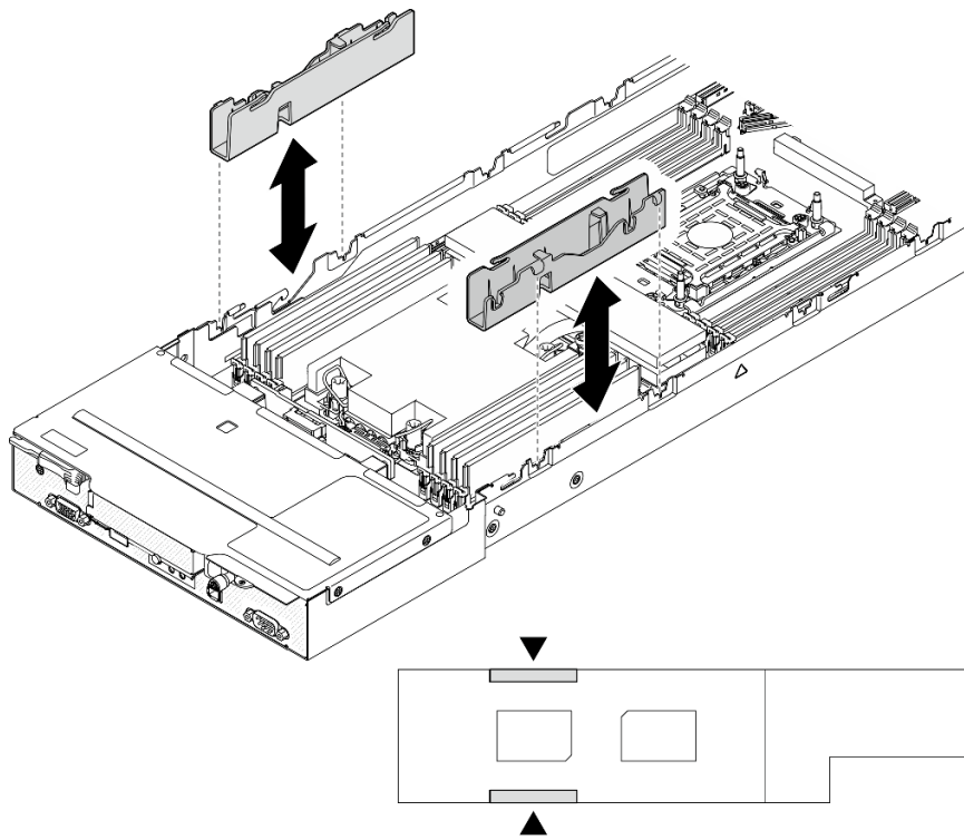
Figura 114. Sustitución del conducto del cable (configuración de un procesador)
