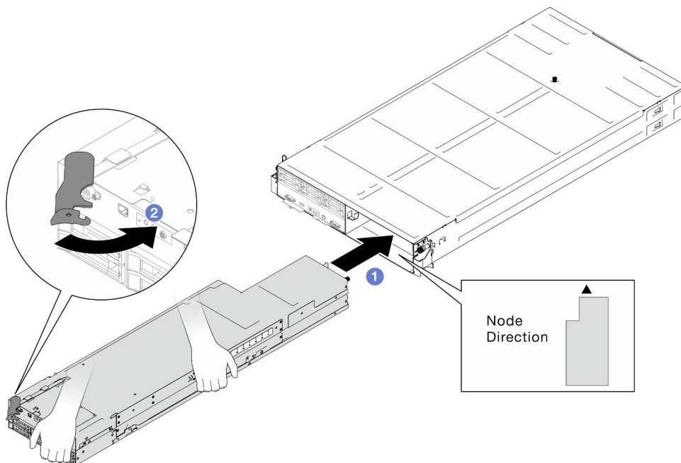
Figura 29. Instalación de un nodo en la bandeja derecha
