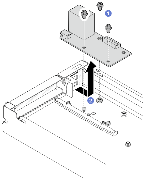
Figura 98. Extracción del módulo de E/S posterior
