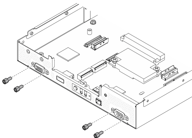
Figura 108. Extracción de los tornillos
