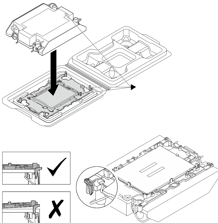
Figura 90. Ensamblaje del PHM con el procesador en la bandeja de envío
