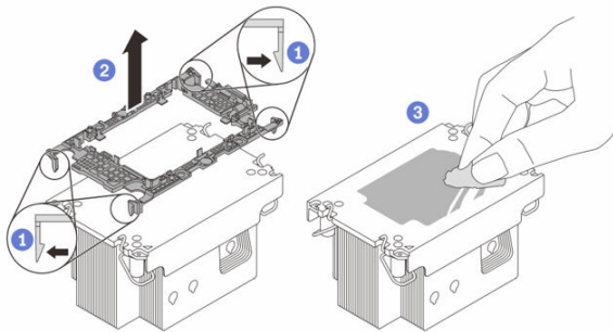
Figura 86. Separación de un transportador de procesador del disipador de calor
