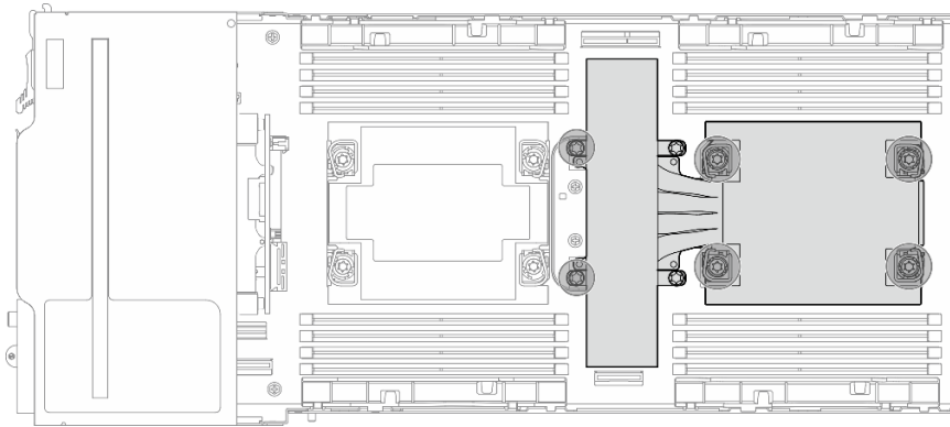
Figura 94. Ubicación de PHM para la configuración de dos procesadores
