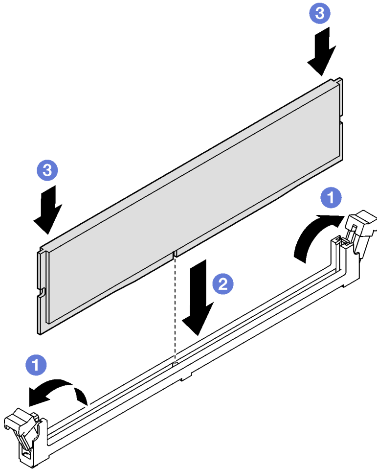
Figura 58. Instalación de un módulo de memoria
