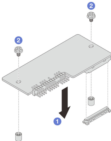
Figura 104. Instalación de la firmware y módulo de seguridad de RoT
