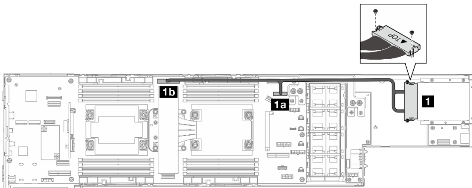
Figura 128. Cables para el módulo de E/S posterior y el módulo OCP
