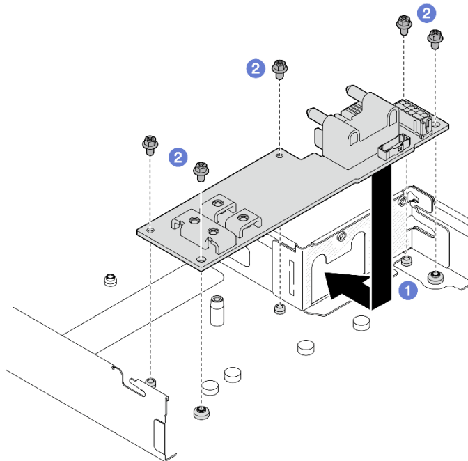
Figura 77. Instalación de una placa de distribución de alimentación
