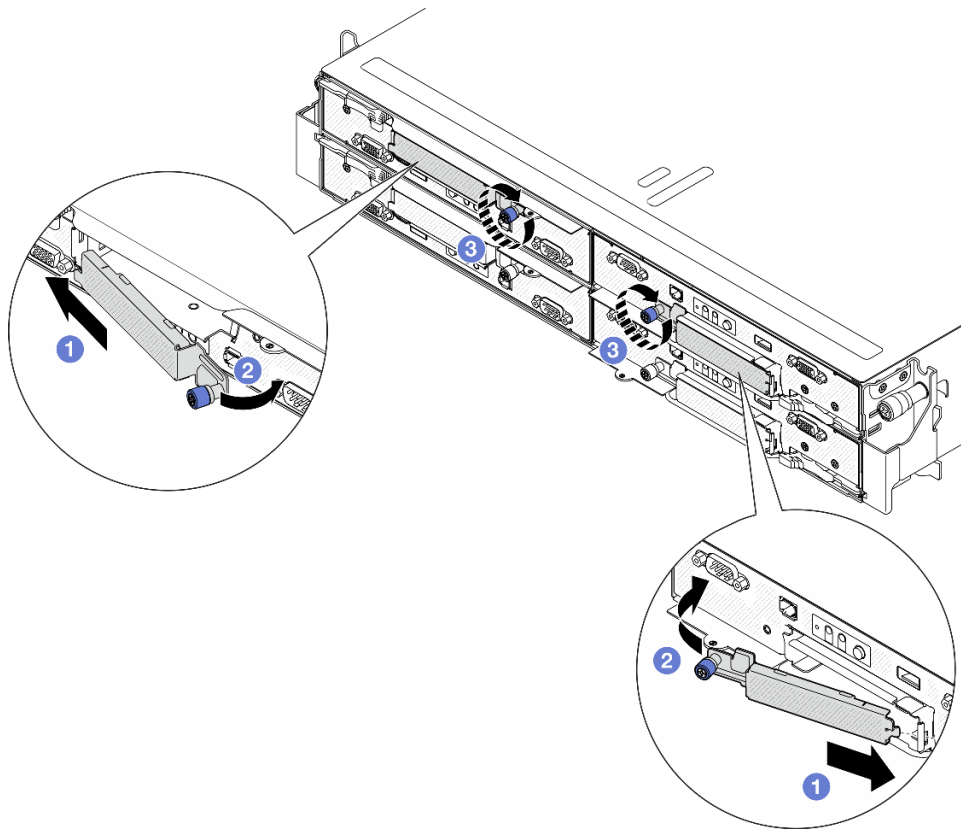
Figura 46. Instalación de la cubierta del compartimiento de la unidad E3.S
