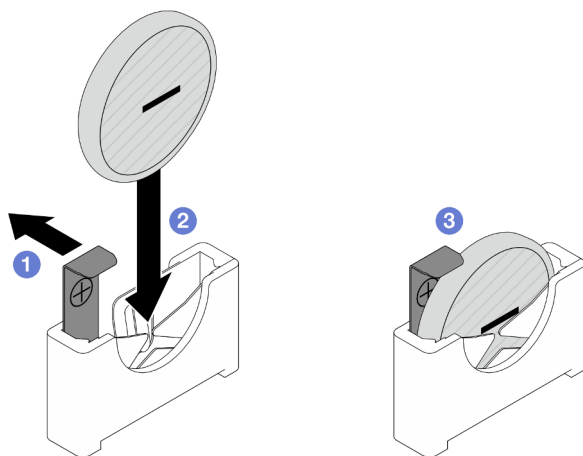
Figura 35. Instalación de una batería CMOS
