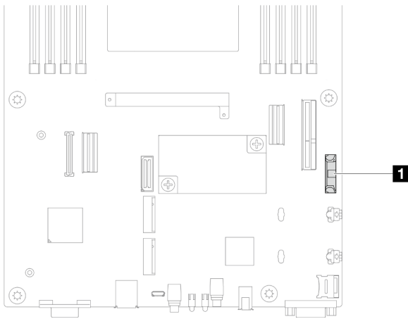
Figura 34. Ubicación del zócalo de la batería CMOS
