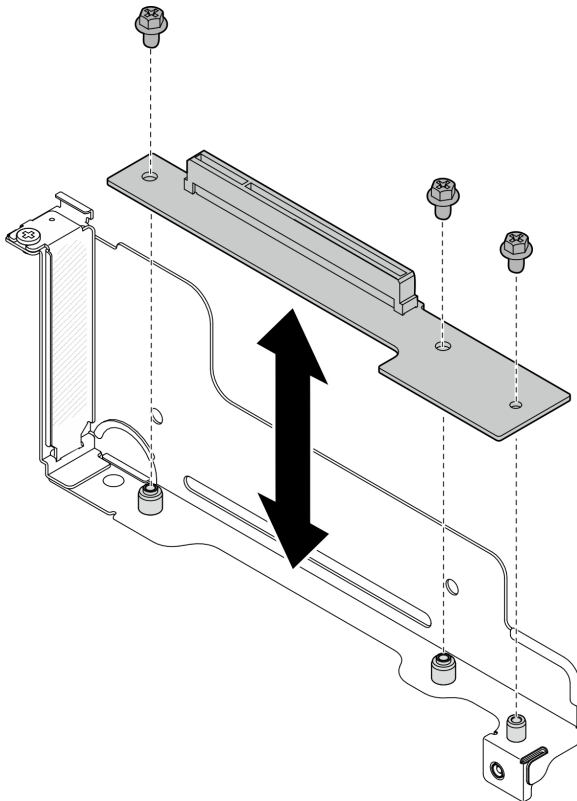
Figura 68. Sustitución de la tarjeta de expansión PCIe
