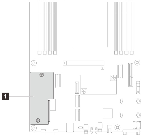
Figura 101. Ubicación del Firmware y módulo de seguridad de RoT
