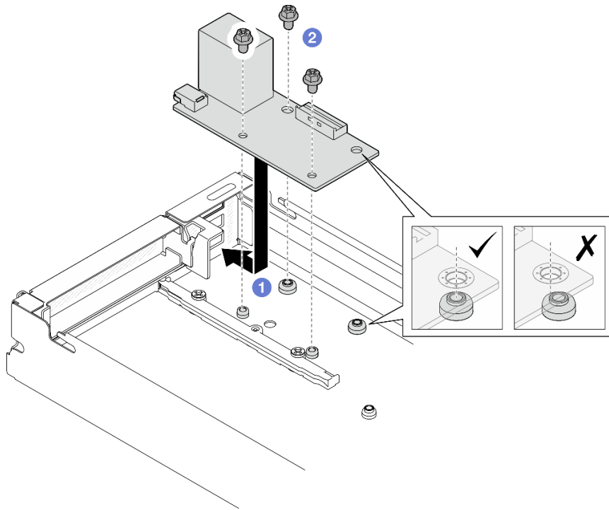
Figura 99. Instalación del módulo de E/S posterior
