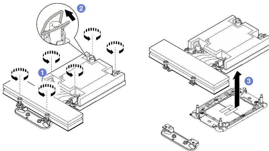
Figura 83. Extracción del PHM de rendimiento 1U del procesador 2
