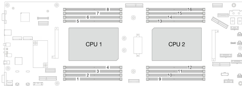
Figura 55. Diseño de los módulos de memoria y el procesador
