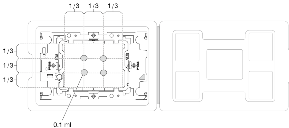
Figura 89. Aplicación de grasa térmica con el procesador en la bandeja de envío
