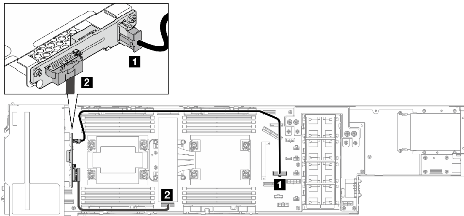
Figura 123. Disposición de los cables para la placa posterior de la unidad E3.S
