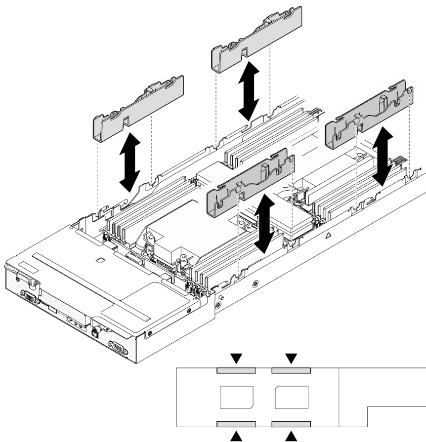
Figura 107. Sustitución del conducto del cable (configuración de dos procesadores)
