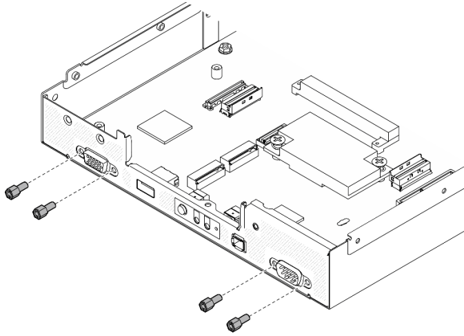
Figura 112. Instalación de los tornillos de la placa del sistema en la parte frontal
