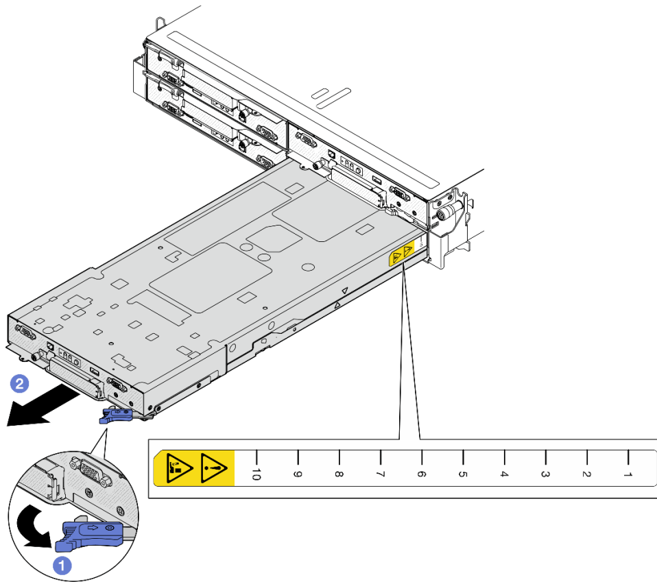
Figura 20. Extracción del nodo de una bandeja derecha
