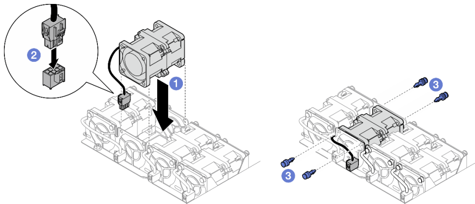
Figura 41. Instalación de ventilador
