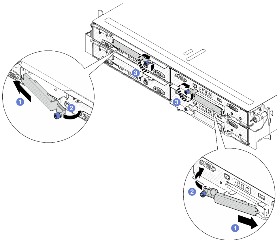
Figura 49. Instalación de la cubierta del compartimiento de la unidad E3.S
