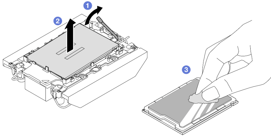
Figura 85. Separación de un procesador del disipador de calor y del transportador
