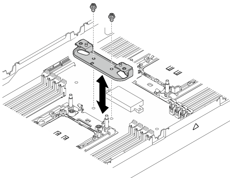
Figura 116. Sustitución de la abrazadera de soporte del dissipador de calor
