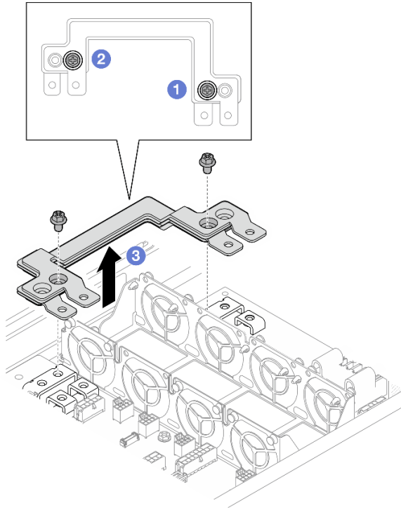
Figura 73. Extracción de la barra de bus de alimentación
