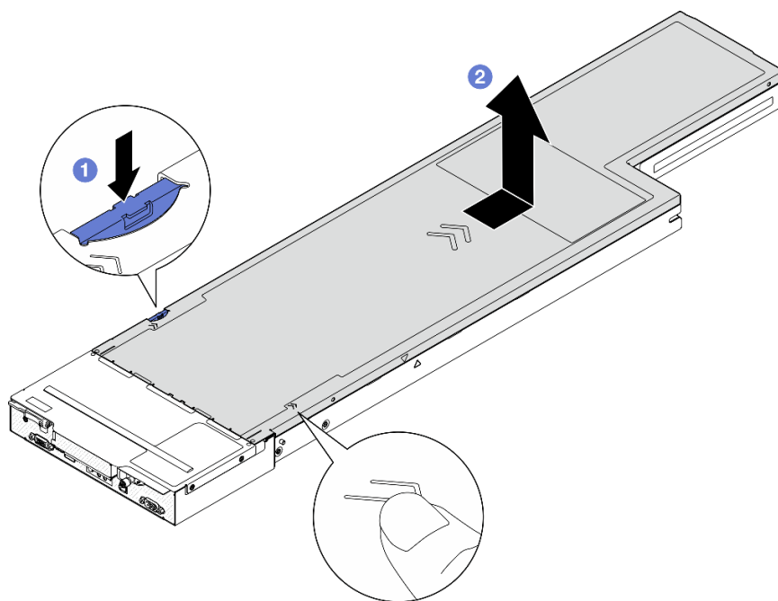
Figura 117. Extracción de la cubierta superior
