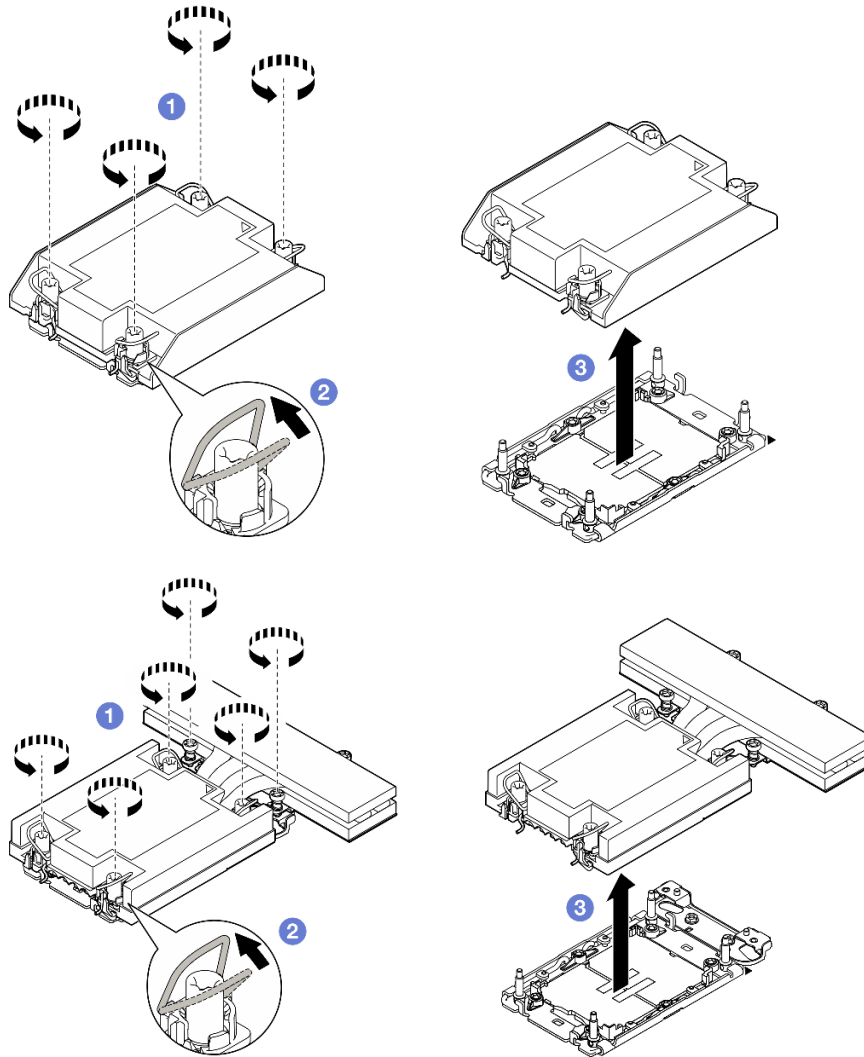
Figura 82. Extracción del PHM de rendimiento 1U del procesador 1
