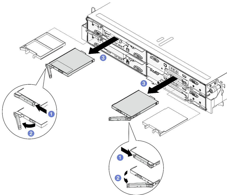
Figura 45. Extracción de una unidad de intercambio en caliente E3.S
