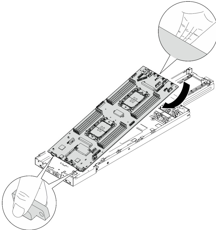
Figura 111. Instalación de la placa del sistema
