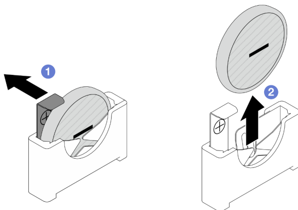
Figura 33. Extracción de la batería CMOS
