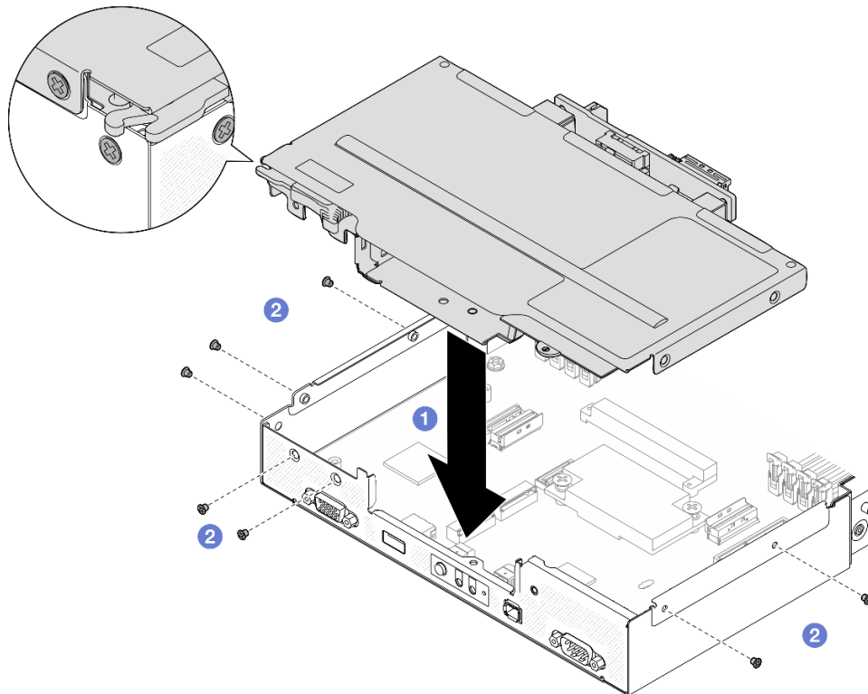
Figura 39. Instalación del conjunto del compartimiento de la unidad
