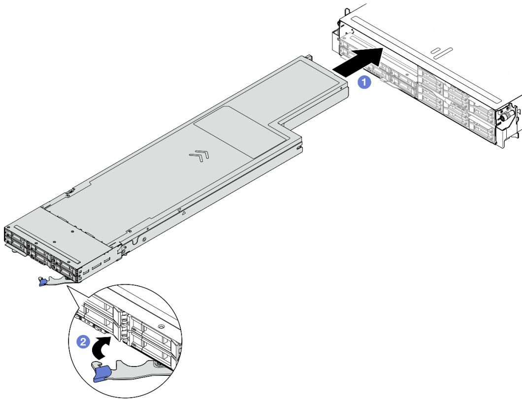
Figura 28. Instalación de un nodo en una bandeja izquierda
