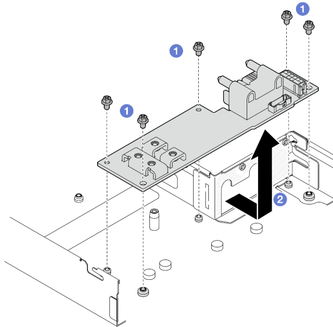
Figura 76. Extracción de la placa de distribución de alimentación
