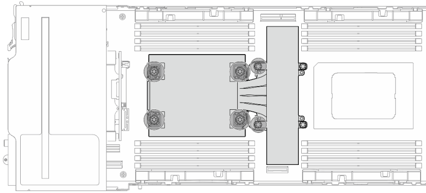
Figura 92. Ubicación de PHM para la configuración de un solo procesador
