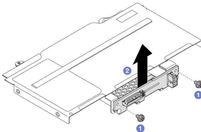
Figura 37. Extracción de la placa posterior de la unidad
