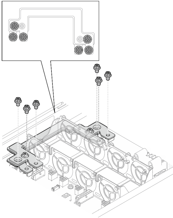
Figura 75. Instalación de los tornillos externos de la barra de bus de alimentación
