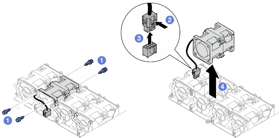
Figura 40. Extracción del ventilador
