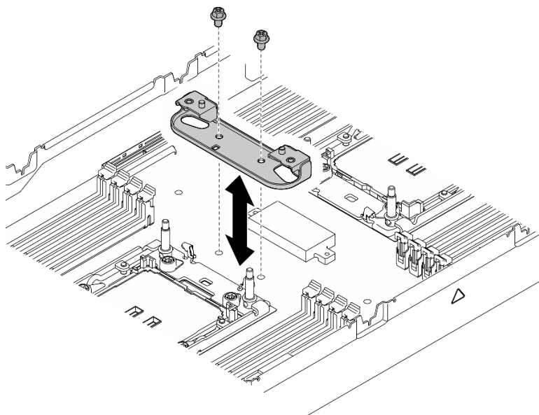
Figura 91. Sustitución de la abrazadera de soporte del disipador de calor
