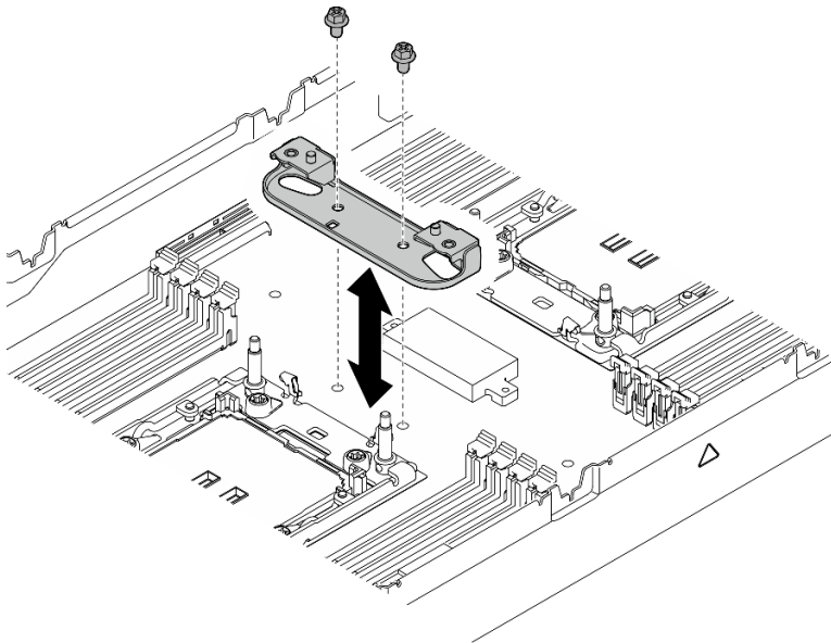
Figura 84. Sustitución de la abrazadera de soporte del disipador de calor
