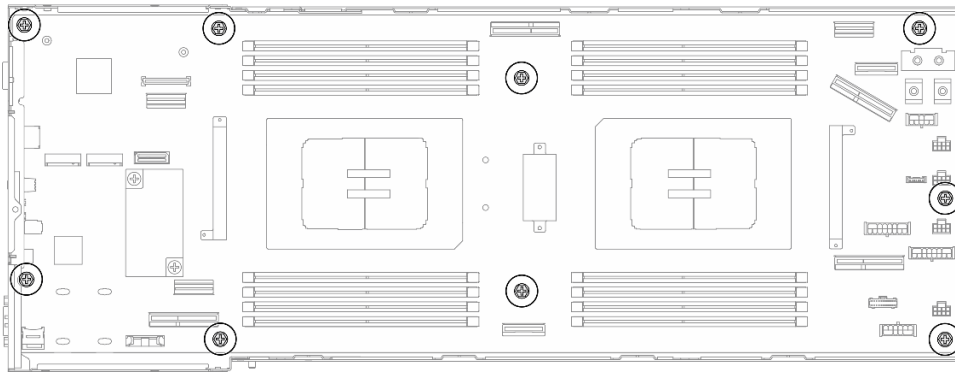
Figura 113. Instalación de los tornillos en la placa del sistema
