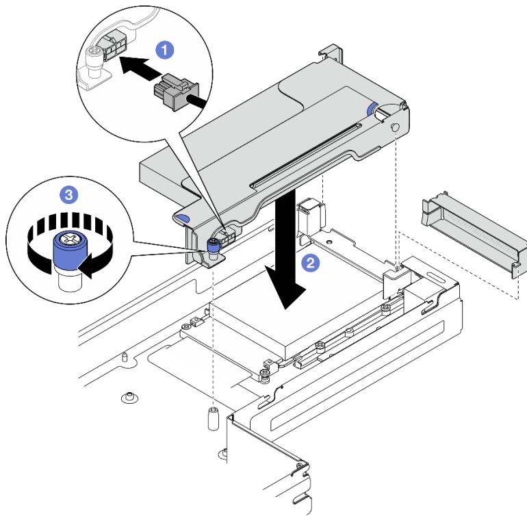
Figura 71. Instalación del conjunto de expansión PCIe
