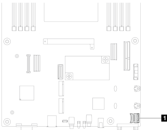
Figura 61. Ubicación del zócalo de MicroSD
