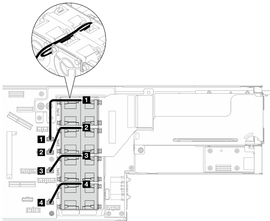
Figura 124. Disposición de los cables del ventilador
