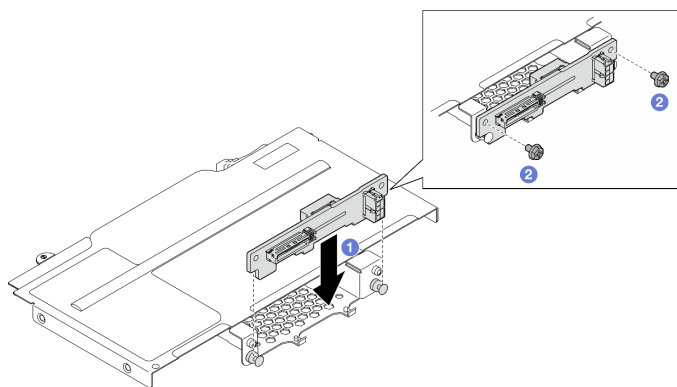
Figura 38. Instalación de la placa posterior de la unidad
