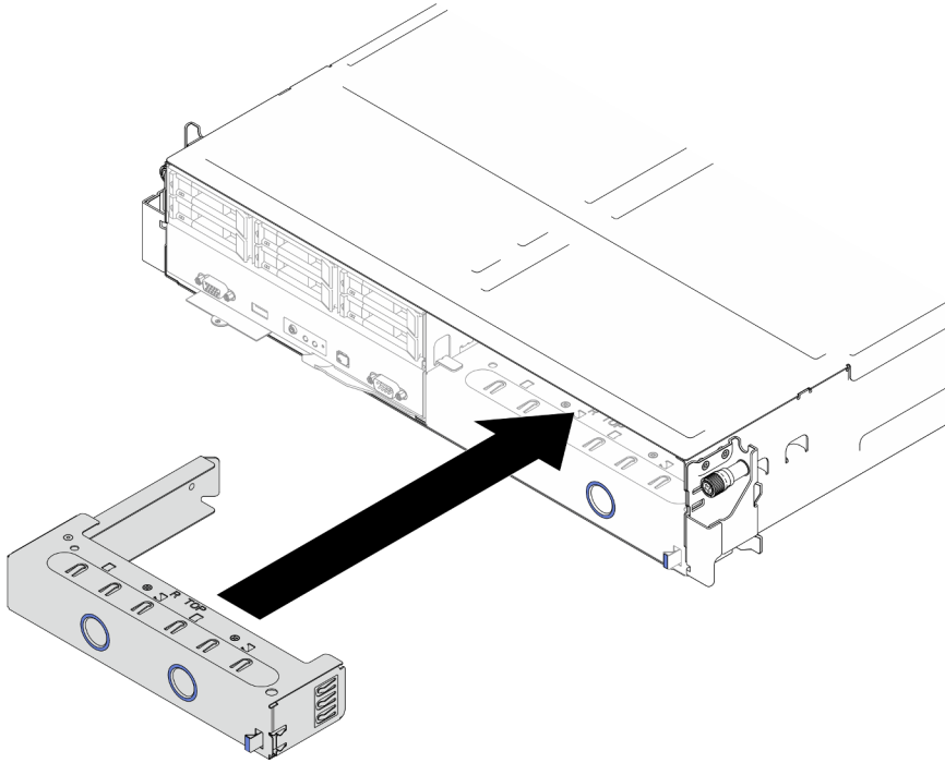
Figura 22. Instalación de un relleno de la bandeja del nodo frontal
