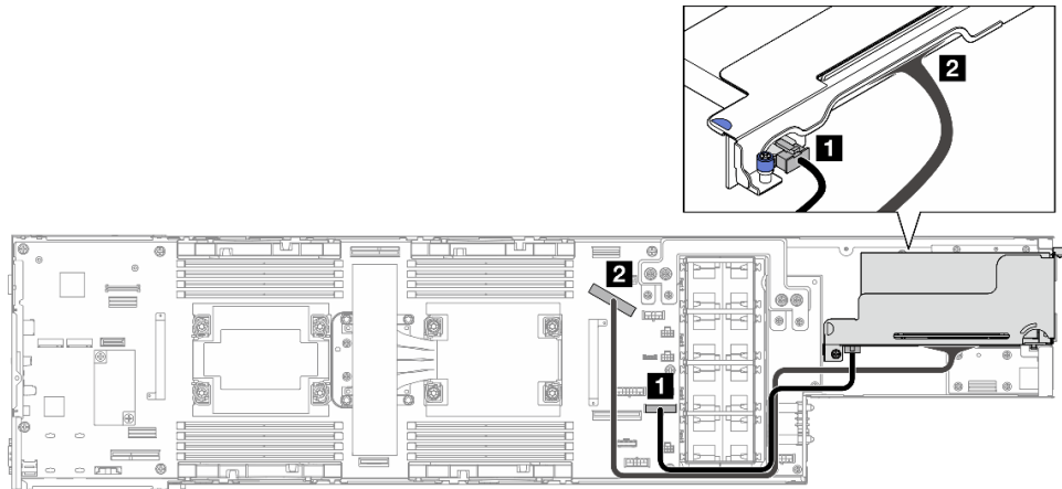
Figura 126. Disposición de cables de la expansión PCIe – dos procesadores
