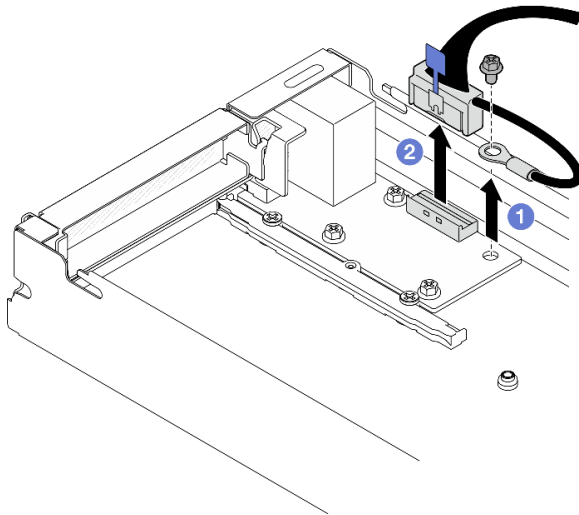
Figura 97. Extracción del cable de E/S posterior y del cable de conexión a tierra
