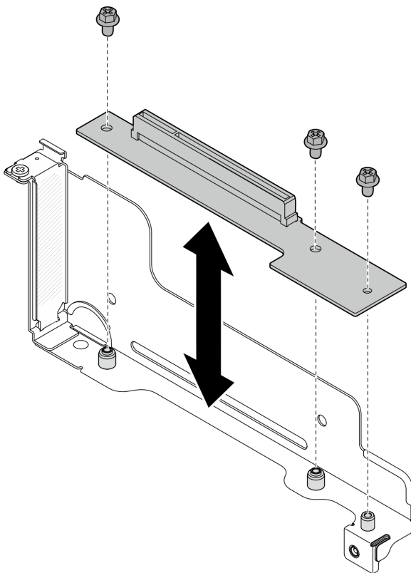
Figura 70. Sustitución de la tarjeta de expansión PCIe
