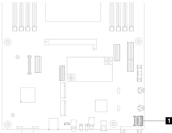
Figura 59. Ubicación del zócalo de MicroSD
