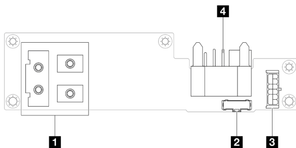
Figura 122. Conectores de placa de distribución de alimentación
