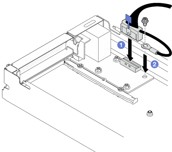
Figura 129. Instalación del cable de E/S posterior y del cable de conexión a tierra
