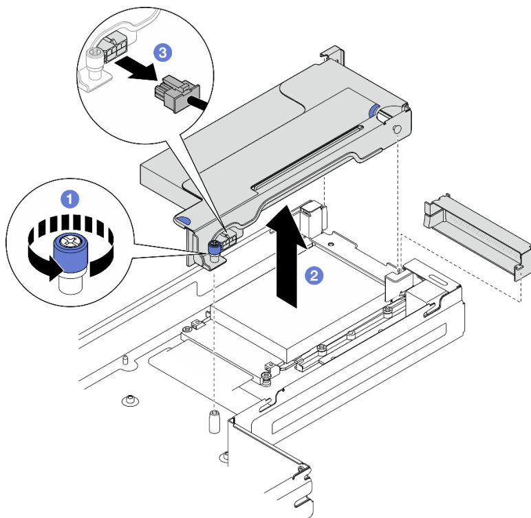
Figura 65. Extracción del conjunto de expansión PCIe
