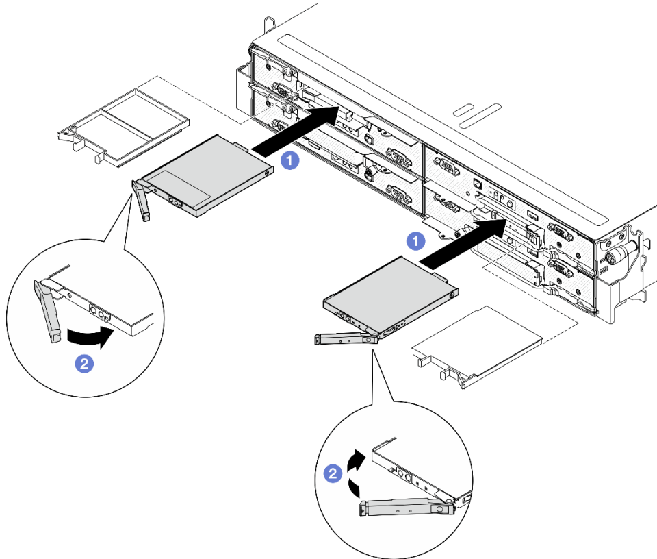
Figura 48. Instalación de una unidad de intercambio en caliente E3.S
