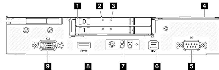
Figura 3. Vista frontal del nodo de ThinkSystem SD530 V3
