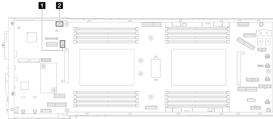
Figura 10. Conmutadores de la placa del sistema
