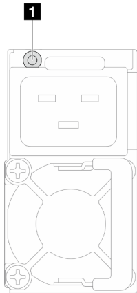
Figura 13. LED de fuente de alimentación
