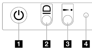
Figura 12. Botones y LED del panel frontal del operador
