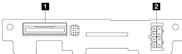
Figure 120. Connecteurs de fond de panier d'unité E3.S
