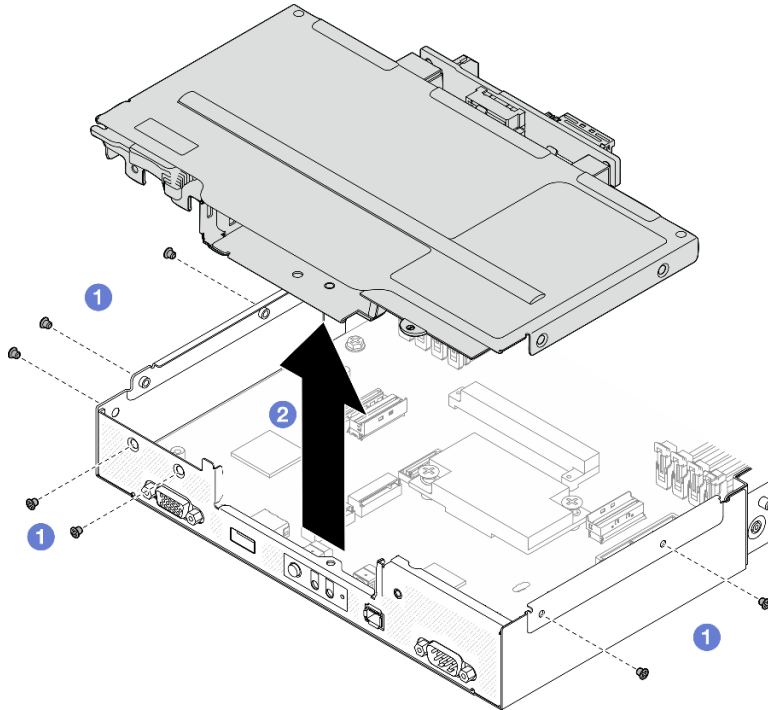
Figure 36. Retrait du bloc boîtier d'unités de disque dur
