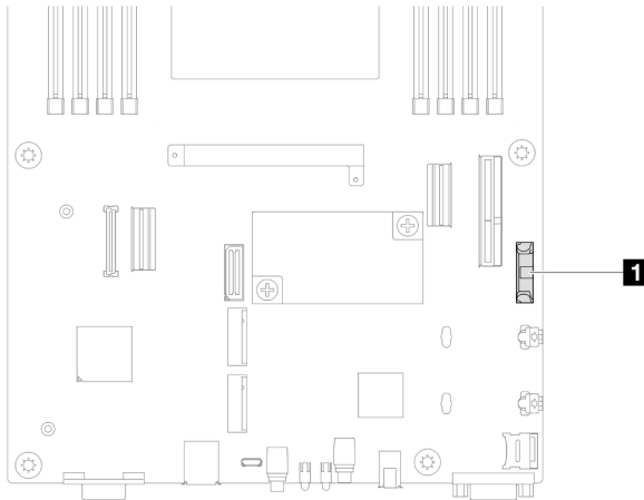
Figure 34. Emplacement du socket de la pile CMOS
