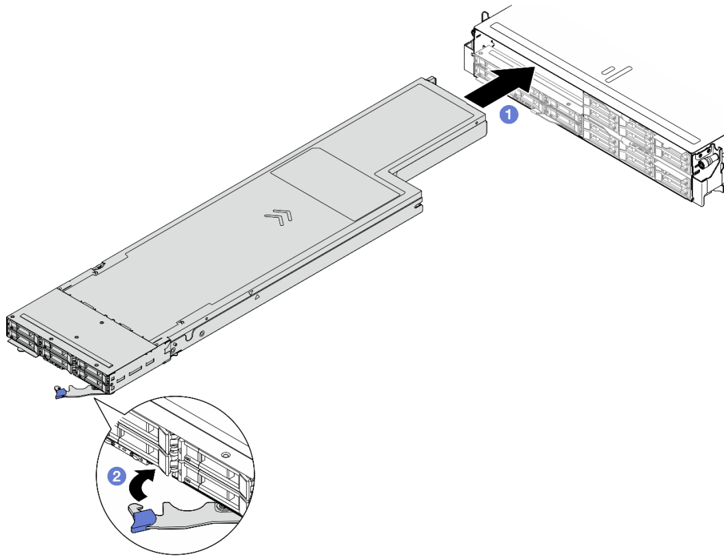
Figure 28. Installation du nœud dans un plateau de gauche
