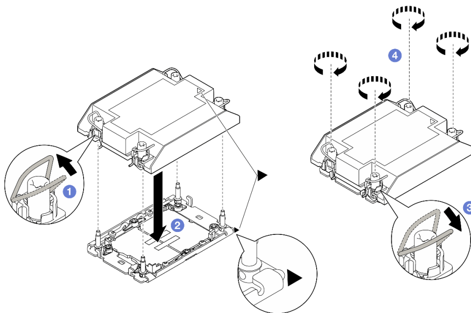
Figure 95. Installation d'un PHM standard 1U pour une configuration à deux processeurs
