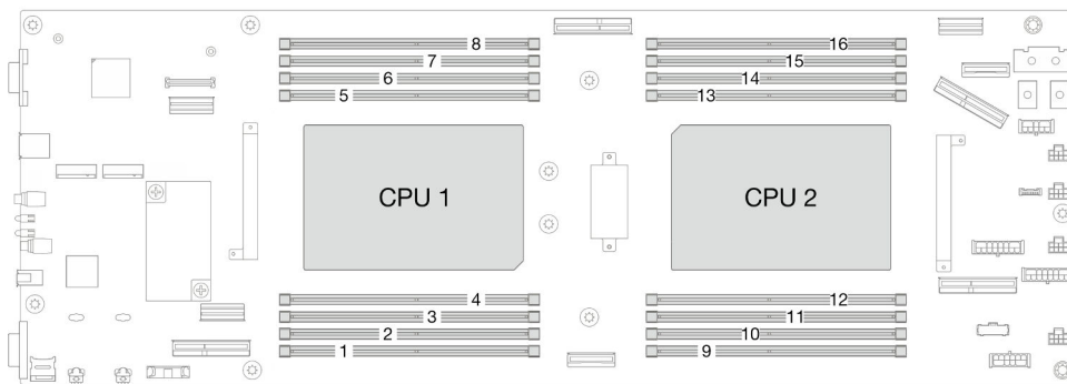
Figure 55. Disposition des modules de mémoire et des processeurs
