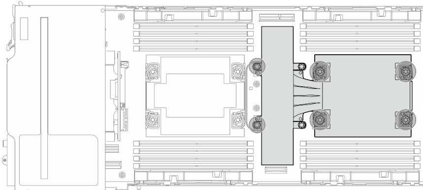
Figure 80. Emplacement du PHM sur la configuration à deux processeurs
