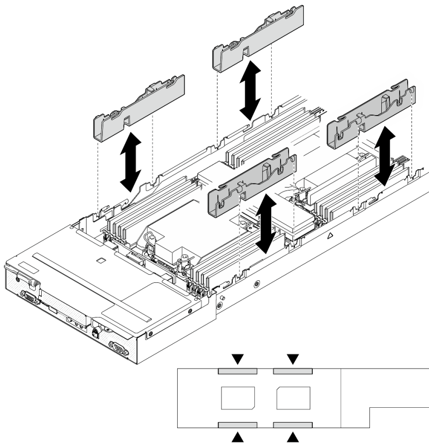
Figure 115. Remplacement d'un conduit de câbles (configuration à deux processeurs)
