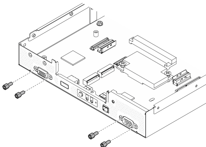
Figure 112. Installation des vis de la carte mère sur le devant
