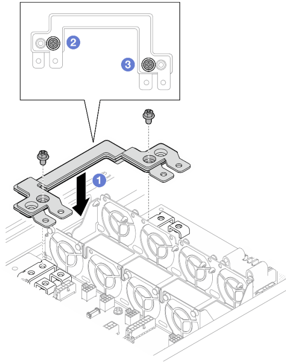
Figure 74. Installation de la barre-bus d'alimentation
