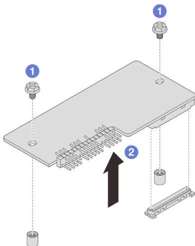
Figure 102. Retrait du Module de microprogramme et de sécurité RoT
