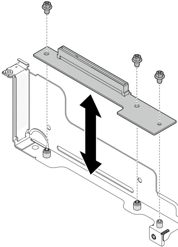
Figure 70. Remplacement de la carte mezzanine PCIe
