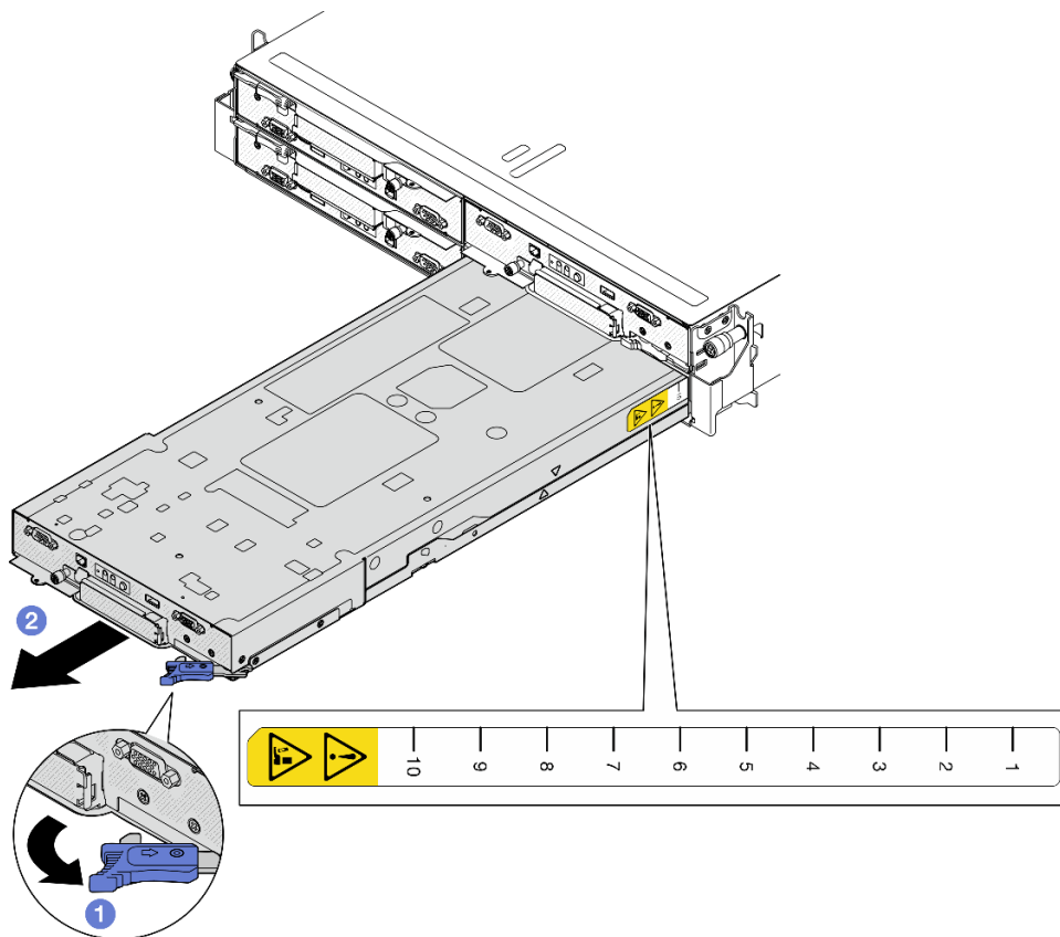
Figure 20. Retrait du nœud d'un plateau de droite
