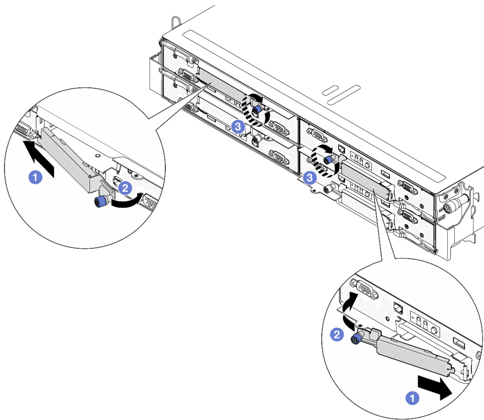
Figure 46. Installation du carter du boîtier d'unités de disque dur E3.S
