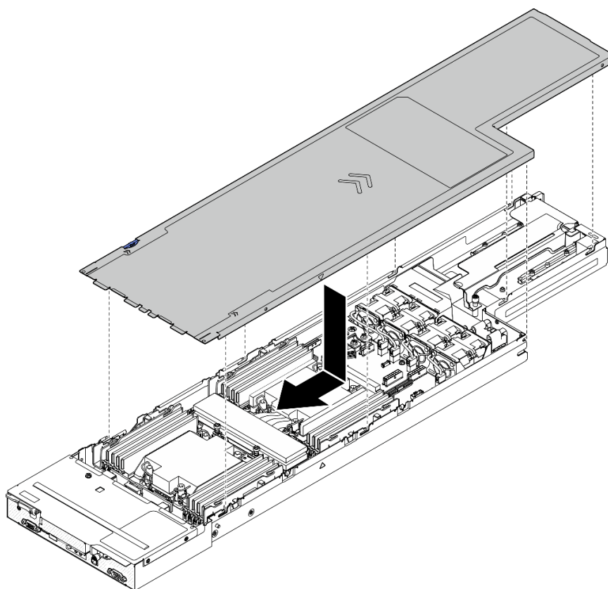
Figure 118. Installation du carter supérieur
