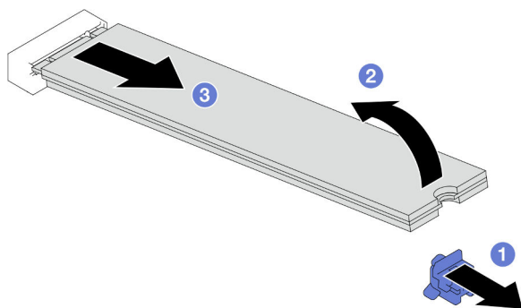
Figure 51. Retrait d'une unité M.2
