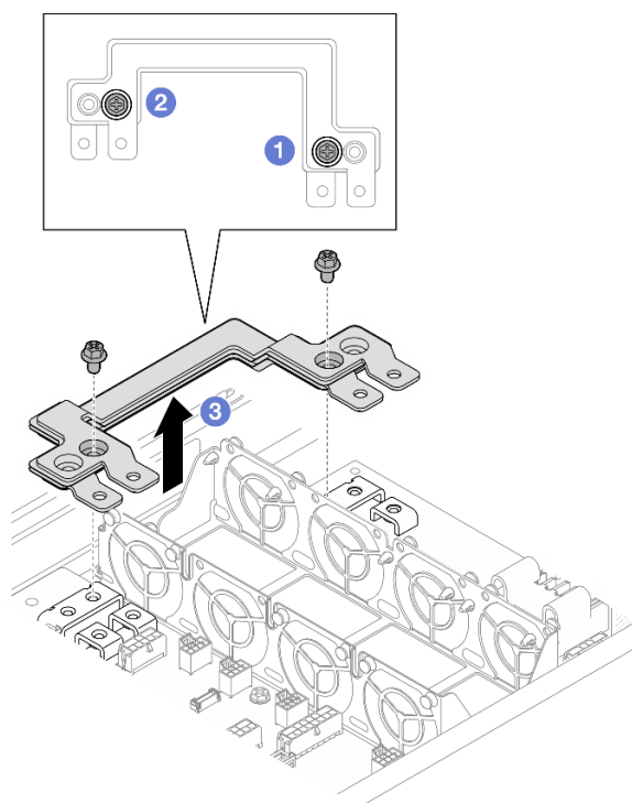
Figure 73. Retrait de la barre-bus d'alimentation
