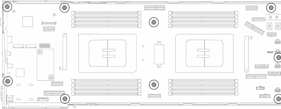
Figure 113. Installation des vis de la carte mère
