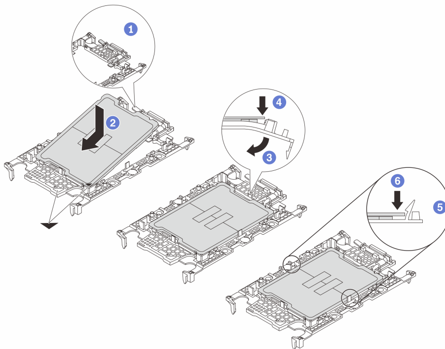
Figure 88. Installation du support de processeur
