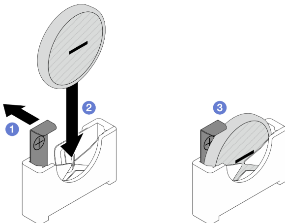
Figure 35. Installation d'une pile CMOS
