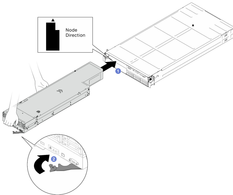
Figure 26. Installation du nœud dans le plateau de gauche
