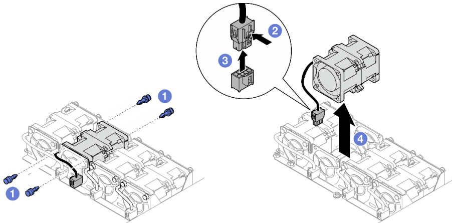
Figure 40. Retrait du ventilateur
