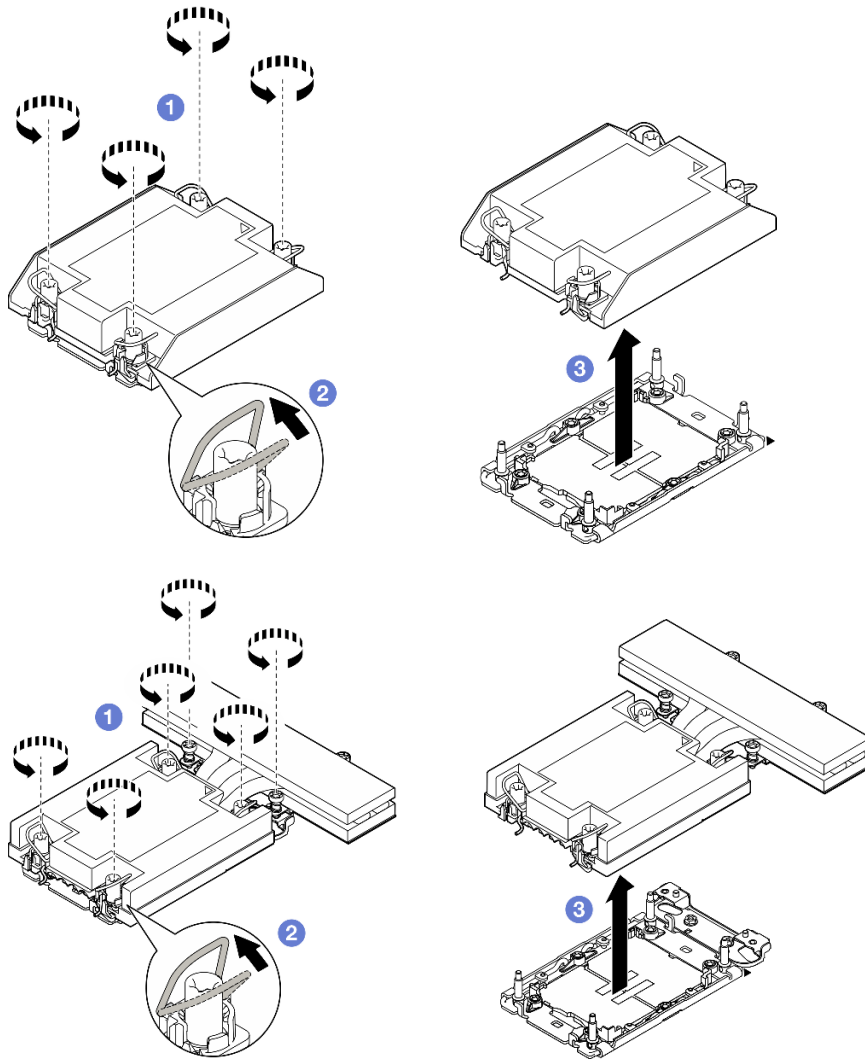
Figure 82. Retrait du PHM de performances 1U du processeur 1
