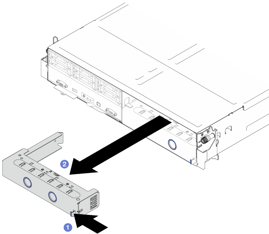
Figure 24. Retrait d'un obturateur de plateau de nœud avant
