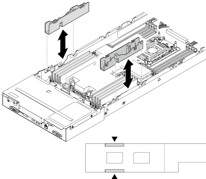
Figure 106. Remplacement d'un conduit de câbles (configuration à un processeur)
