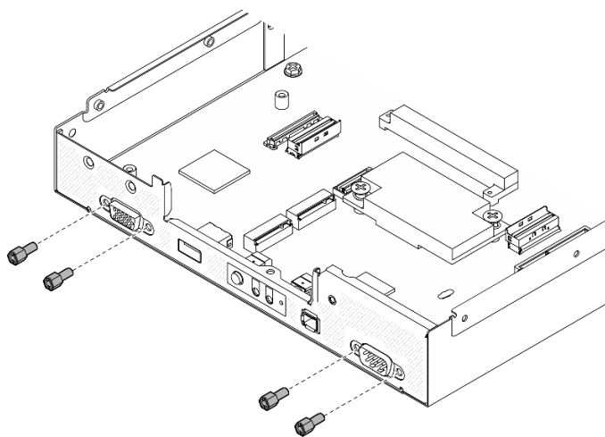
Figure 108. Retrait des vis
