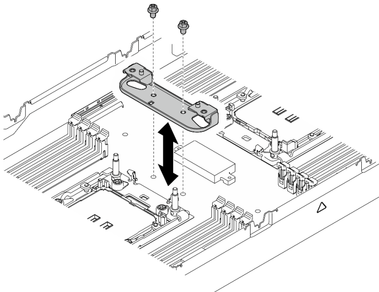
Figure 105. Remplacement du support du dissipateur thermique
