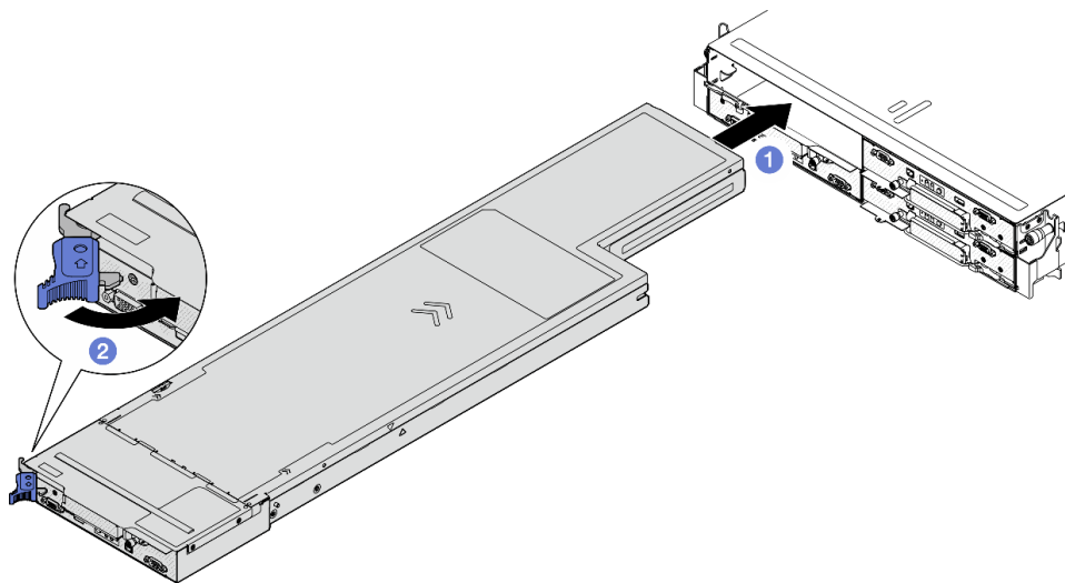
Figure 27. Installation du nœud dans un plateau de gauche
