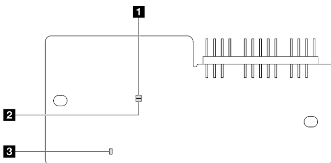
Figure 135. Voyants du module de microprogramme et de sécurité RoT
