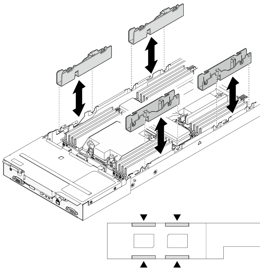
Figure 107. Remplacement d'un conduit de câbles (configuration à deux processeurs)
