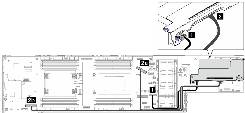
Figure 125. Cheminement des câbles de la carte mezzanine PCIe – un processeur
