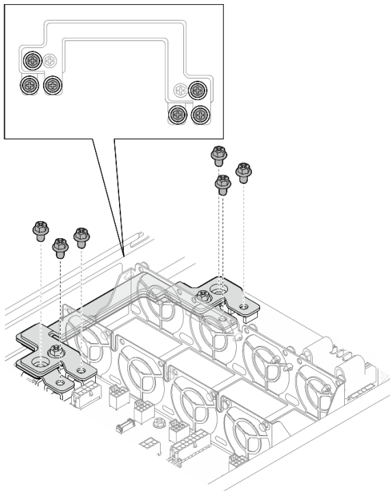
Figure 72. Retrait des vis externes de la barre-bus d'alimentation
