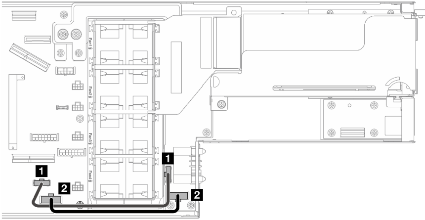
Figure 127. Cheminement des câbles pour le tableau de distribution
