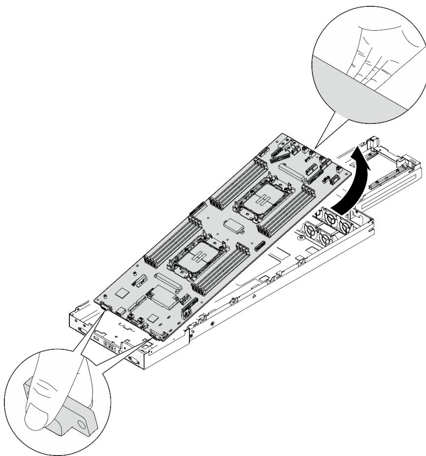
Figure 110. Retrait de la carte mère
