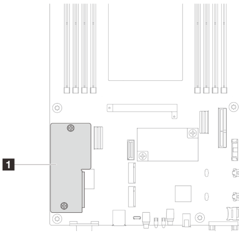
Figure 101. Emplacement du Module de microprogramme et de sécurité RoT
