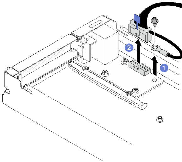
Figure 97. Retrait du câble d'E-S arrière et du câble de mise à la terre
