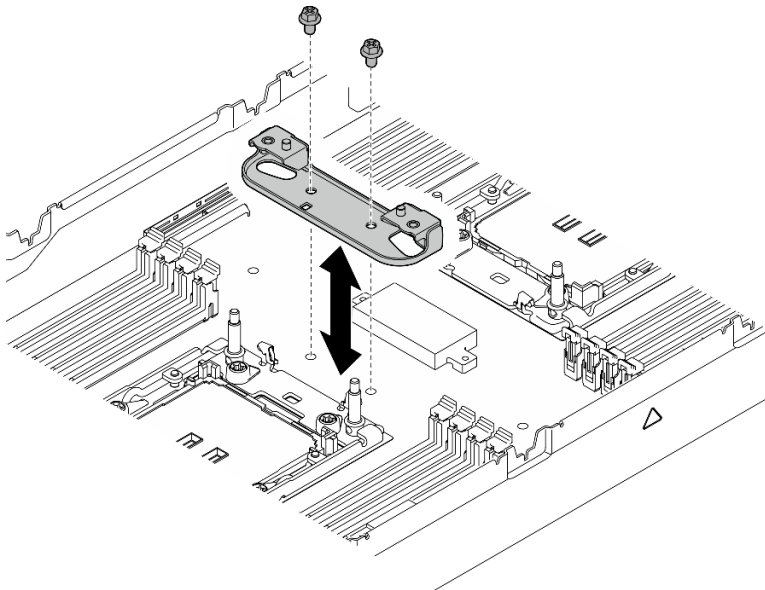
Figure 84. Remplacement du support du dissipateur thermique
