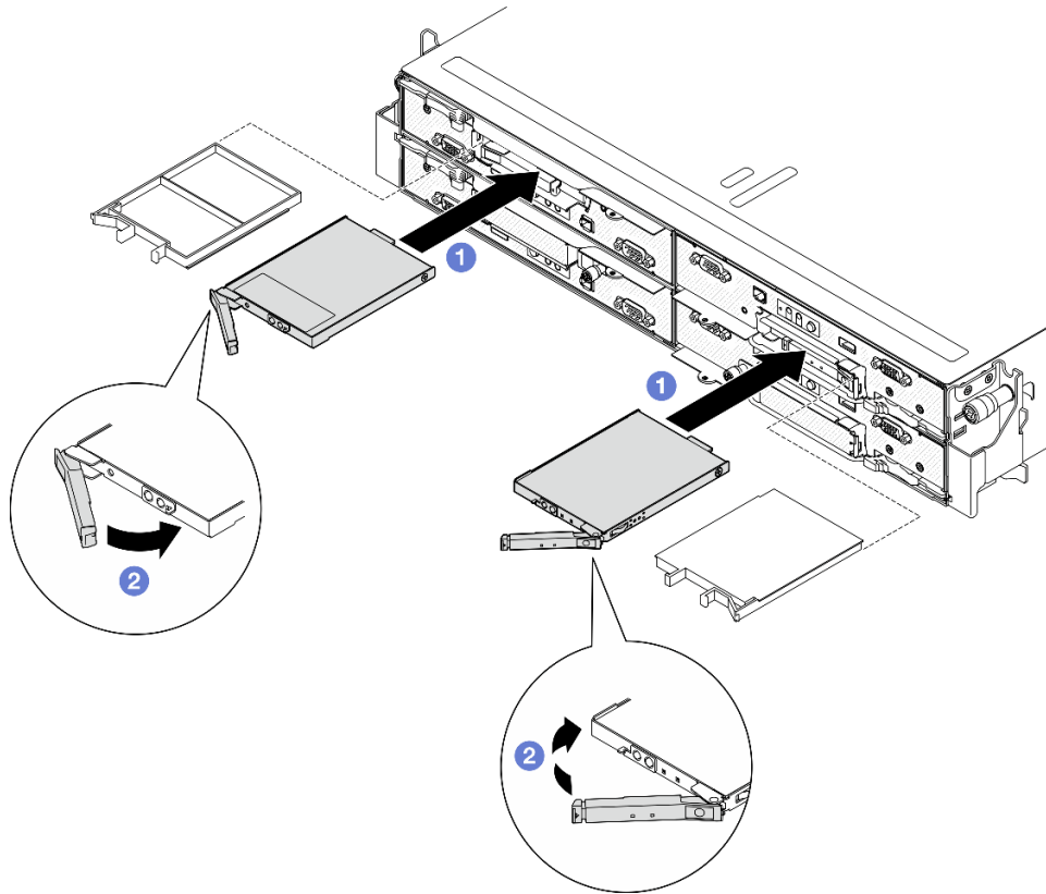
Figure 48. Installation d'une unité remplaçable à chaud E3.S
