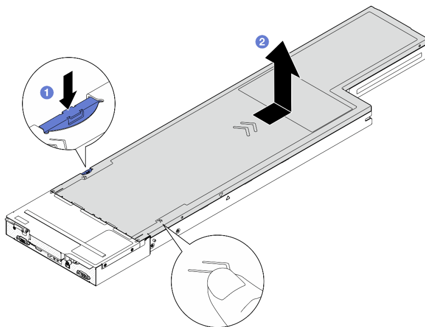
Figure 117. Retrait du carter supérieur
