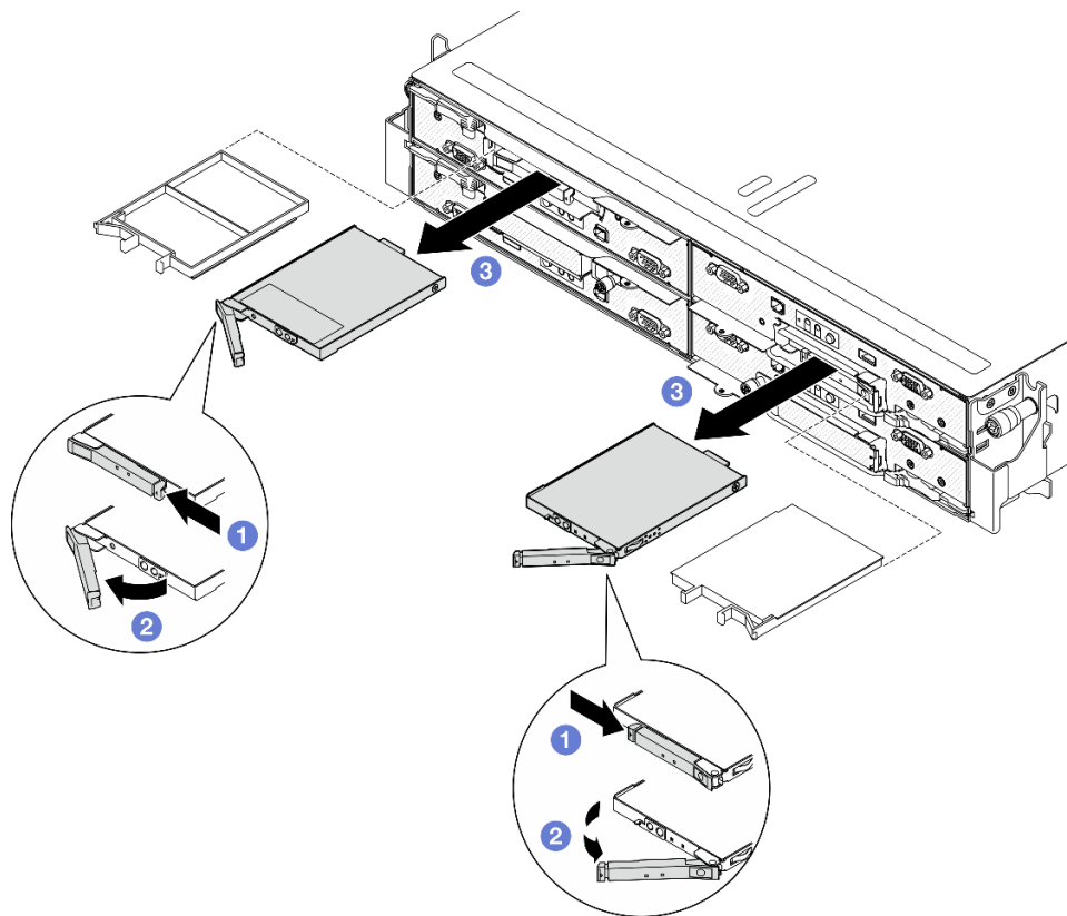
Figure 45. Retrait de l'unité remplaçable à chaud E3.S
