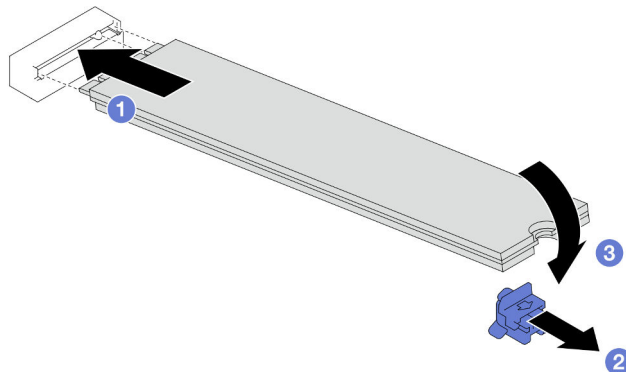
Figure 54. Installation d'une unité M.2
