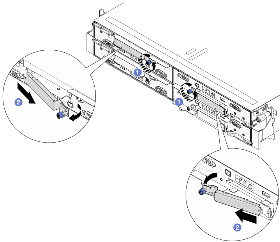
Figure 44. Retrait du carter du boîtier d'unités de disque dur E3.S
