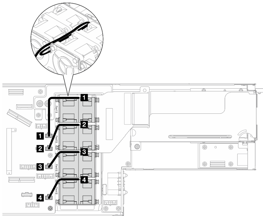
Figure 124. Cheminement des câbles de ventilateur
