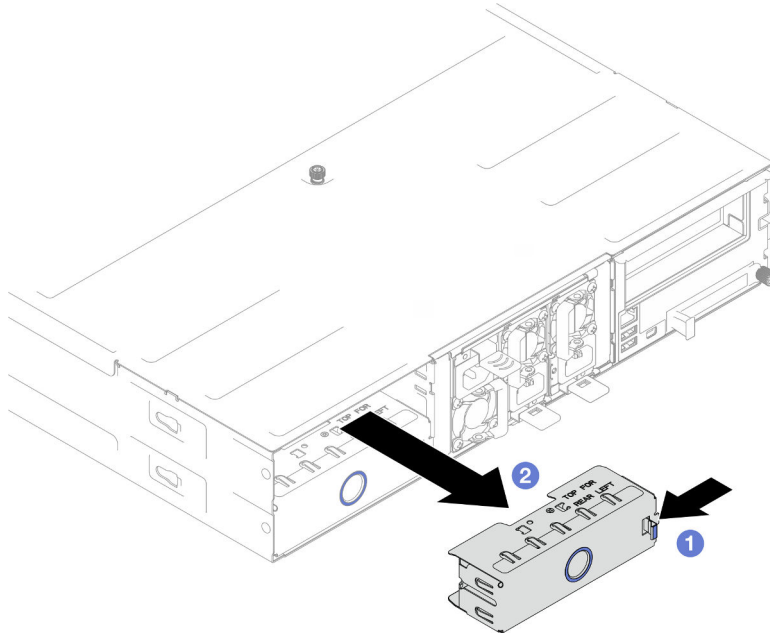
Figure 25. Retrait d'un obturateur de plateau de nœud arrière
