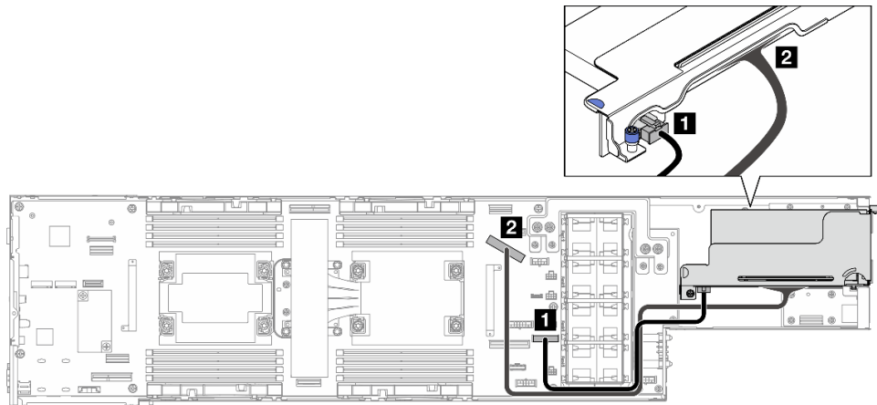
Figure 126. Cheminement des câbles de la carte mezzanine PCIe – deux processeurs
