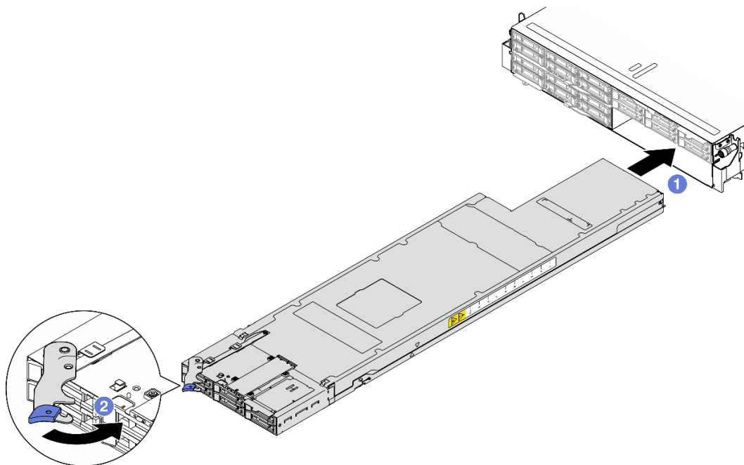
Figure 31. Installation du nœud dans un plateau de droite
