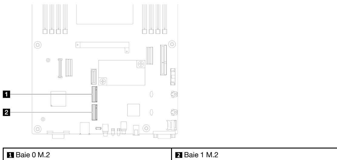
Figure 50. Emplacement des baies M.2 sur la carte mère
