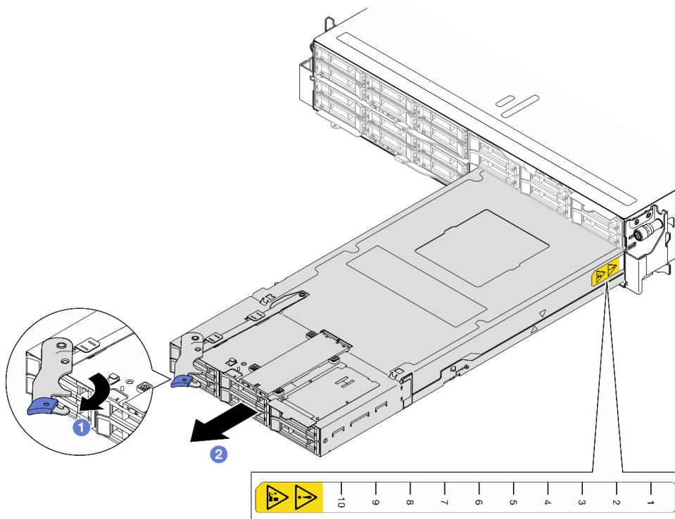
Figure 21. Retrait du nœud d'un plateau de droite
