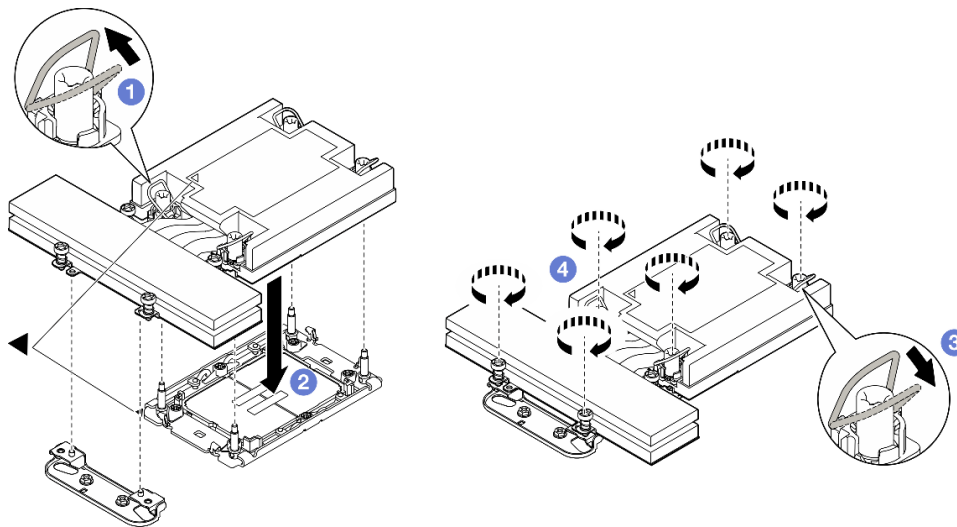
Figure 96. Installation d'un PHM de performances 1U pour une configuration à deux processeurs
