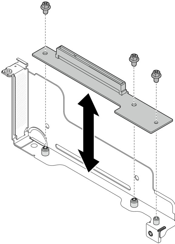
Figure 66. Remplacement de la carte mezzanine PCIe
