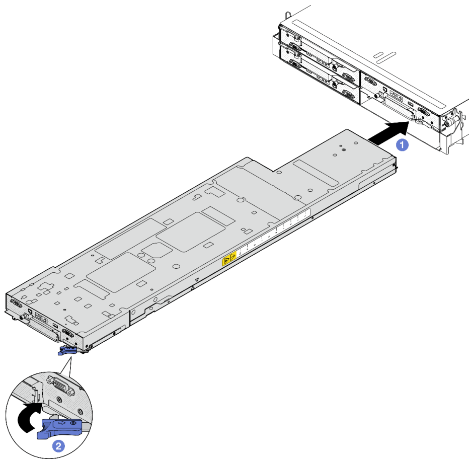
Figure 30. Installation du nœud dans un plateau de droite
