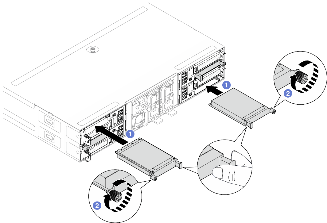
Figure 64. Installation du module OCP arrière
