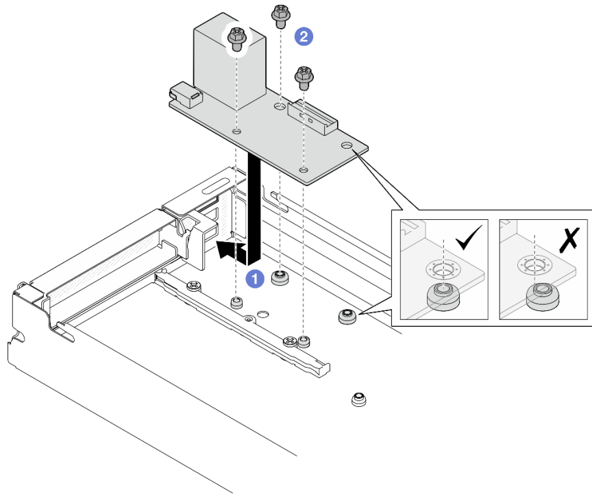
Figure 99. Installation du module d'E-S arrière
