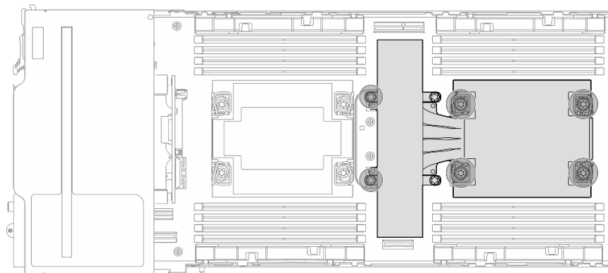
Figure 94. Emplacement du PHM sur la configuration à deux processeurs
