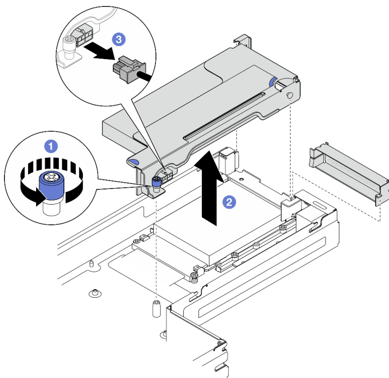
Figure 65. Retrait de l'assemblage de cartes mezzanines PCIe
