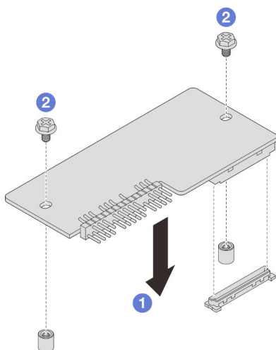
Figure 104. Installation du module de microprogramme et de sécurité RoT
