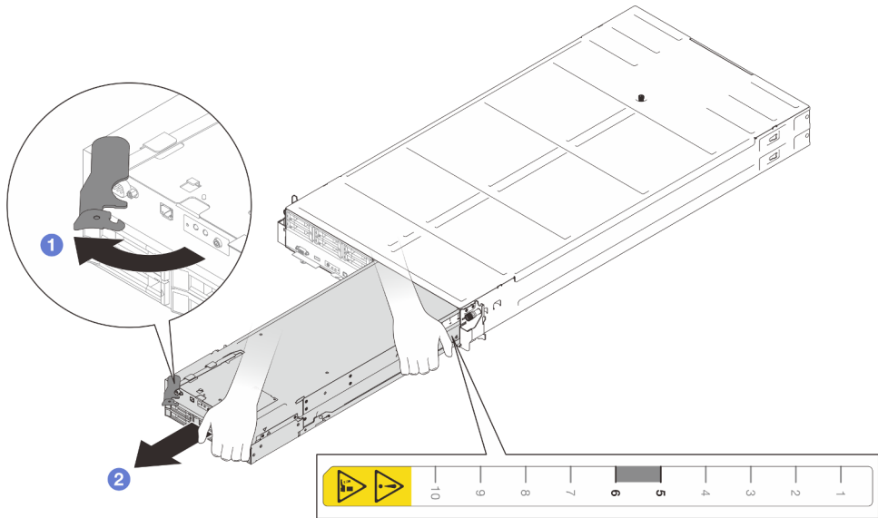
Figure 19. Retrait du nœud du plateau de droite
