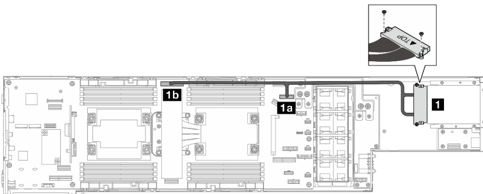
Figure 128. Câbles pour le module OCP et d'E-S arrière
