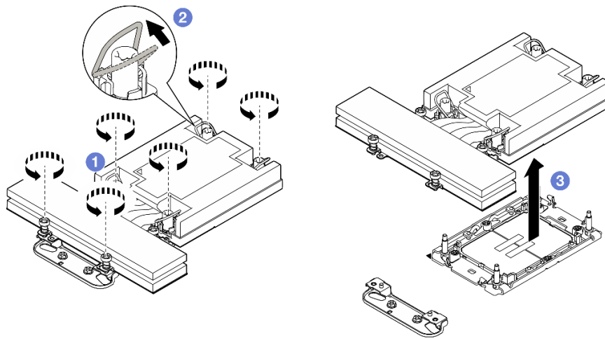
Figure 83. Retrait du PHM de performances 1U du processeur 2
