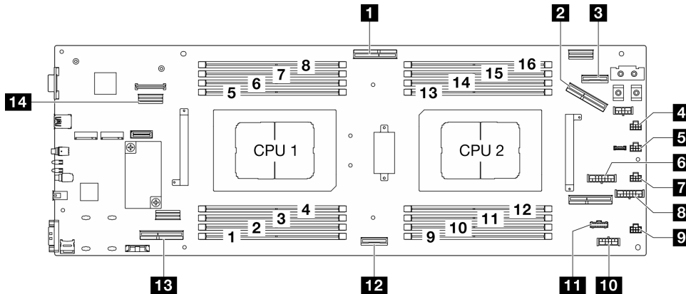
Figure 119. Connecteurs de la carte mère pour le cheminement des câbles
