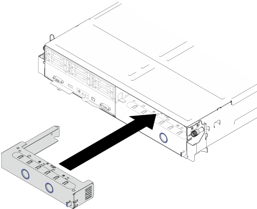
Figure 22. Installation d'un obturateur de plateau de nœud avant
