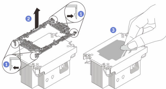
Figure 86. Dissociation d'un support de processeur du dissipateur thermique
