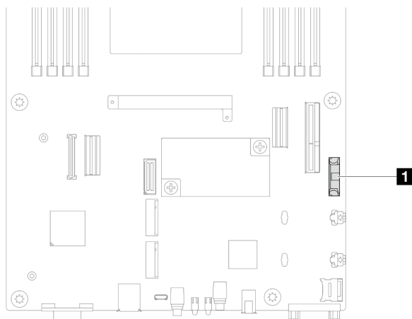
Figure 32. Emplacement du socket de la pile CMOS
