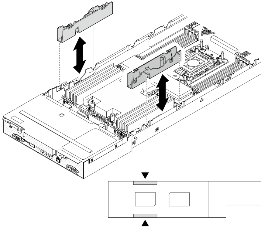
Figure 114. Remplacement d'un conduit de câbles (configuration à un processeur)
