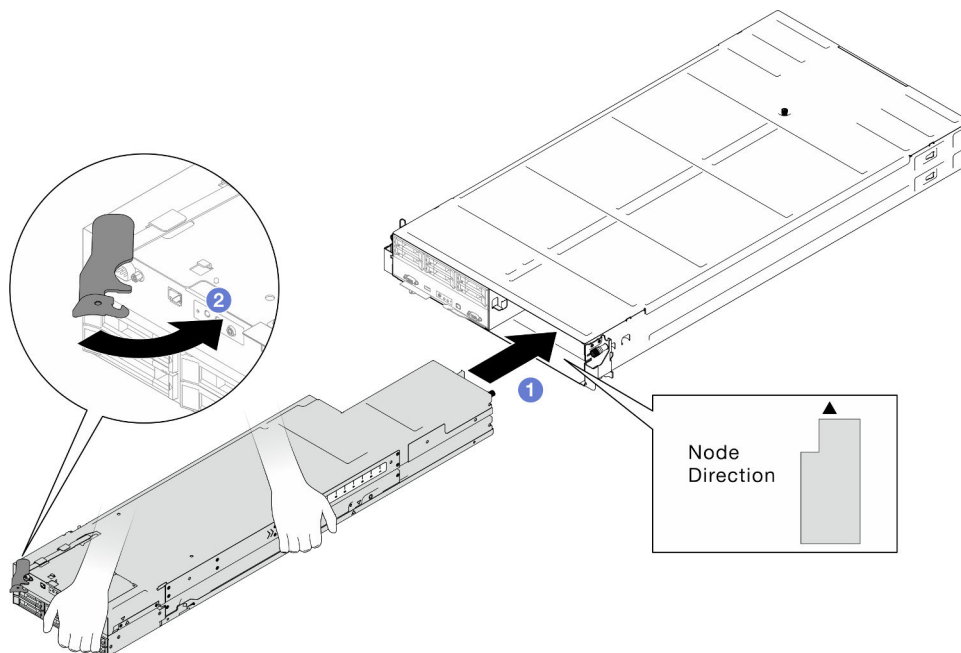
Figure 29. Installation du nœud dans le plateau de droite
