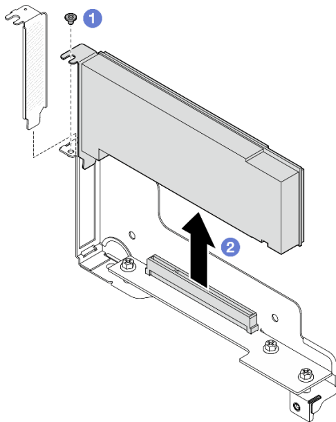
Figure 67. Retrait d'un adaptateur PCIe
