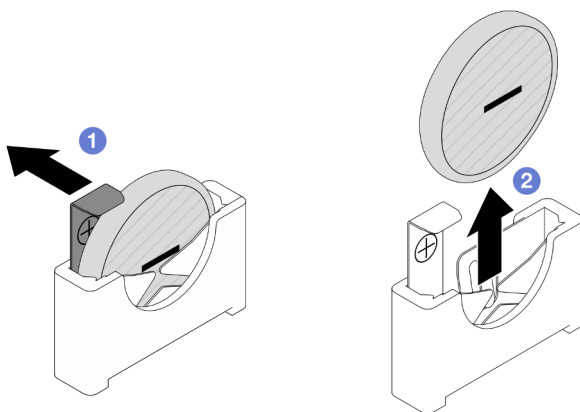
Figure 33. Retrait de la pile CMOS
