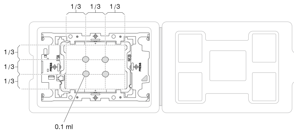
Figure 89. Application de pâte thermoconductrice avec processeur dans le plateau d'expédition
