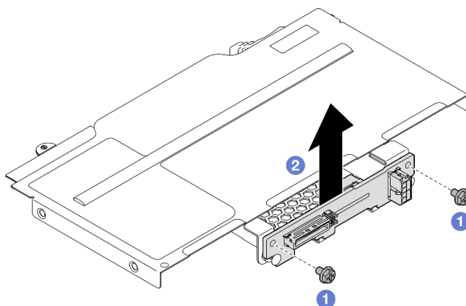
Figure 37. Retrait du fond de panier d'unité
