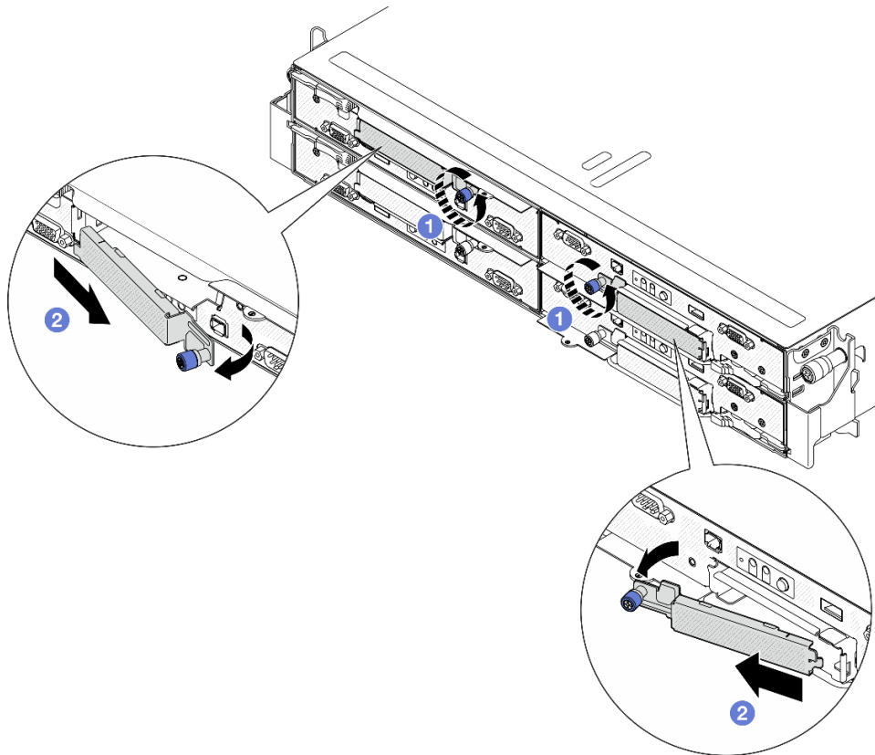
Figure 47. Retrait du carter du boîtier d'unités de disque dur E3.S
