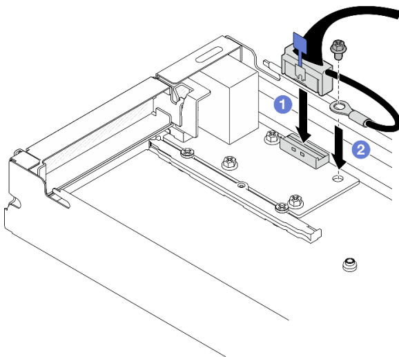
Figure 100. Installation du câble d'E-S arrière et du câble de mise à la terre
