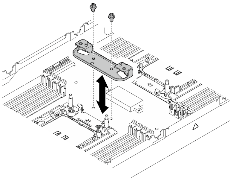
Figure 116. Remplacement du support du dissipateur thermique
