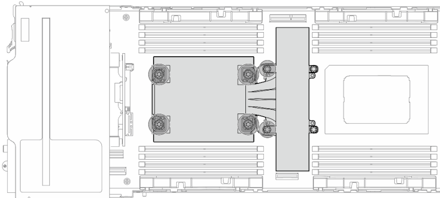
Figure 79. Emplacement du PHM sur la configuration à un processeur
