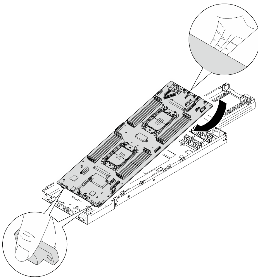
Figure 111. Installation de la carte mère
