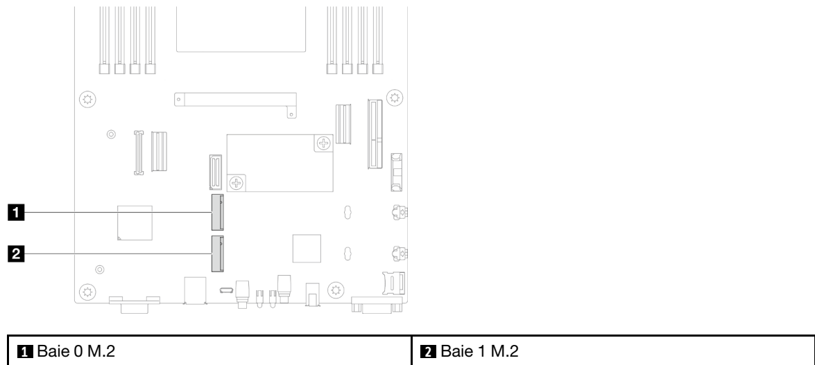
Figure 53. Emplacement des baies M.2 sur la carte mère
