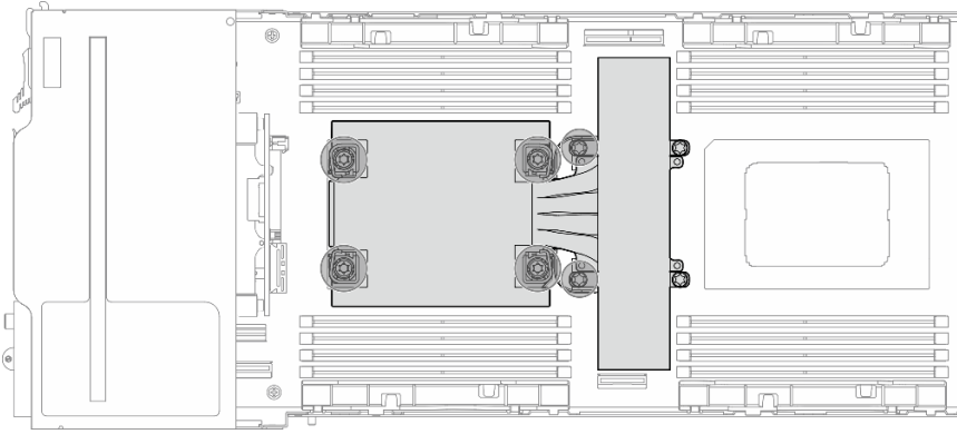
Figure 92. Emplacement du PHM sur la configuration à un processeur
