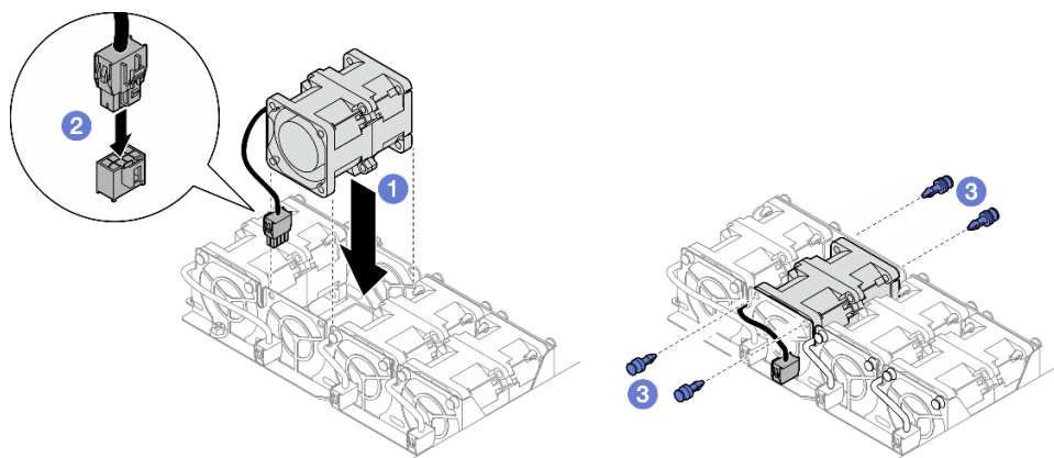
Figure 41. Installation du ventilateur
