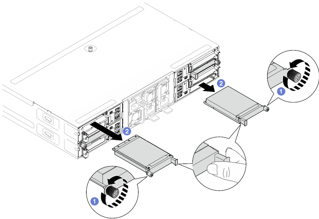
Figure 63. Retrait du module OCP arrière
