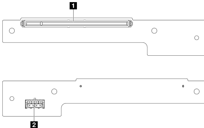
Figure 121. Connecteurs de carte mezzanine PCIe
