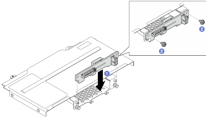
Figura 38. Installazione del backplane dell'unità
