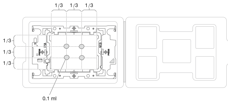
Figura 89. Applicazione del lubrificante termico con il processore nella confezione di spedizione
