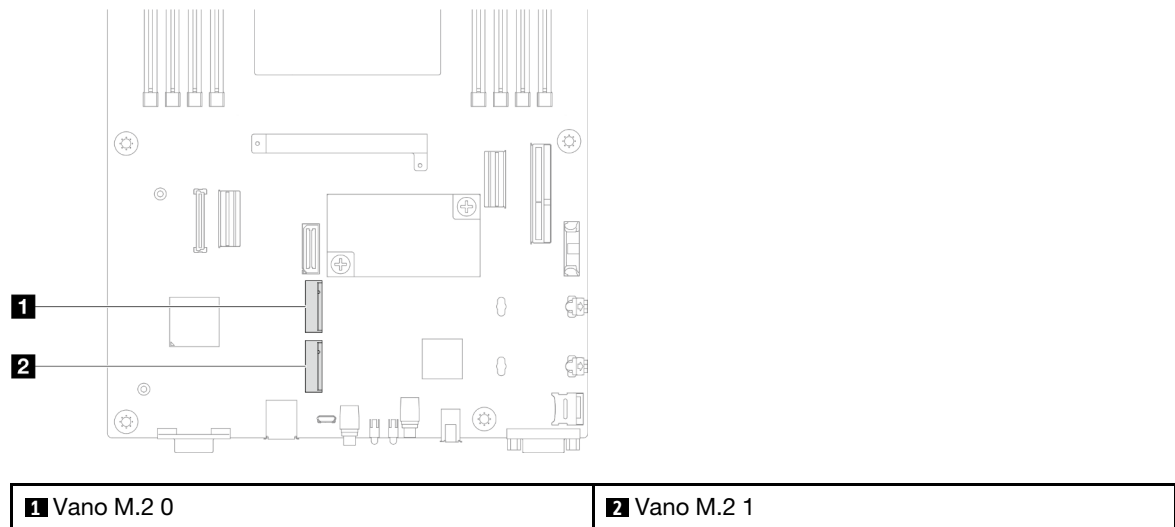
Figura 53. Posizione dei vani M.2 sulla scheda di sistema
