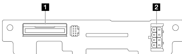
Figura 120. Connettori backplane dell'unità E3.S
