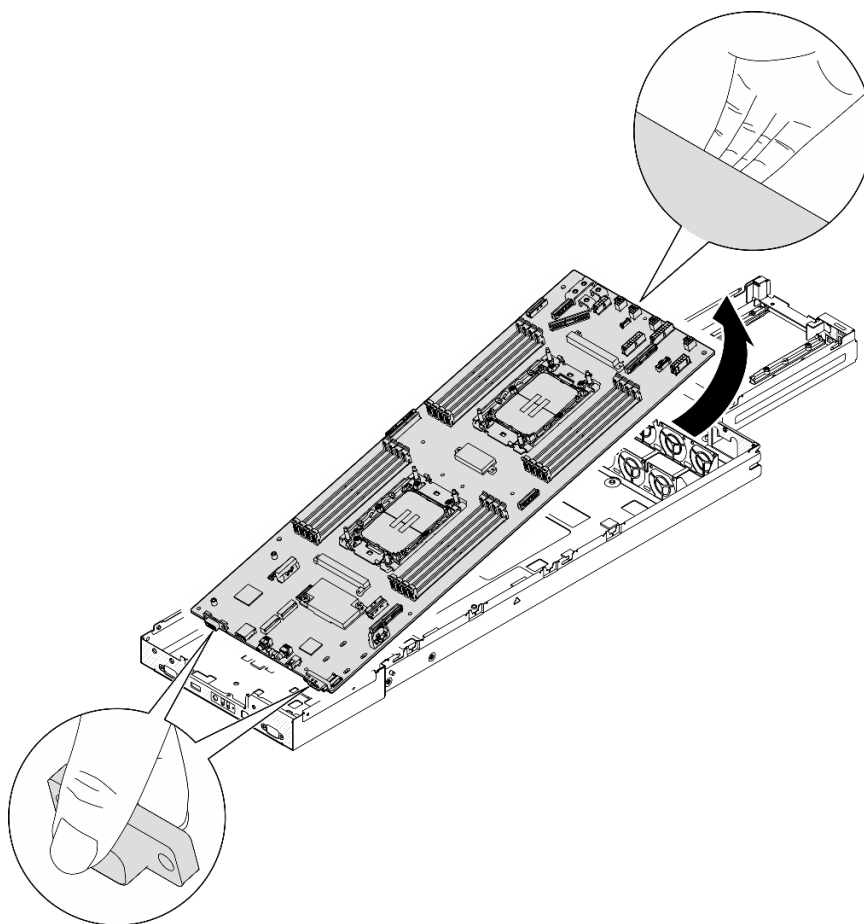
Figura 110. Rimozione della scheda di sistema
