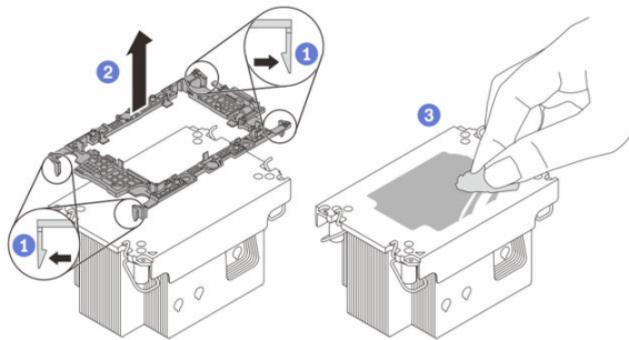
Figura 86. Separazione di una piastra del processore dal dissipatore di calore
