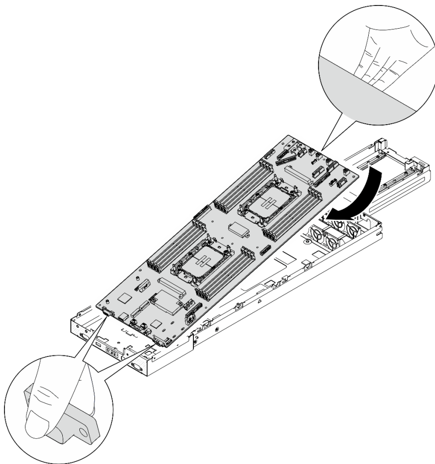
Figura 111. Installazione della scheda di sistema
