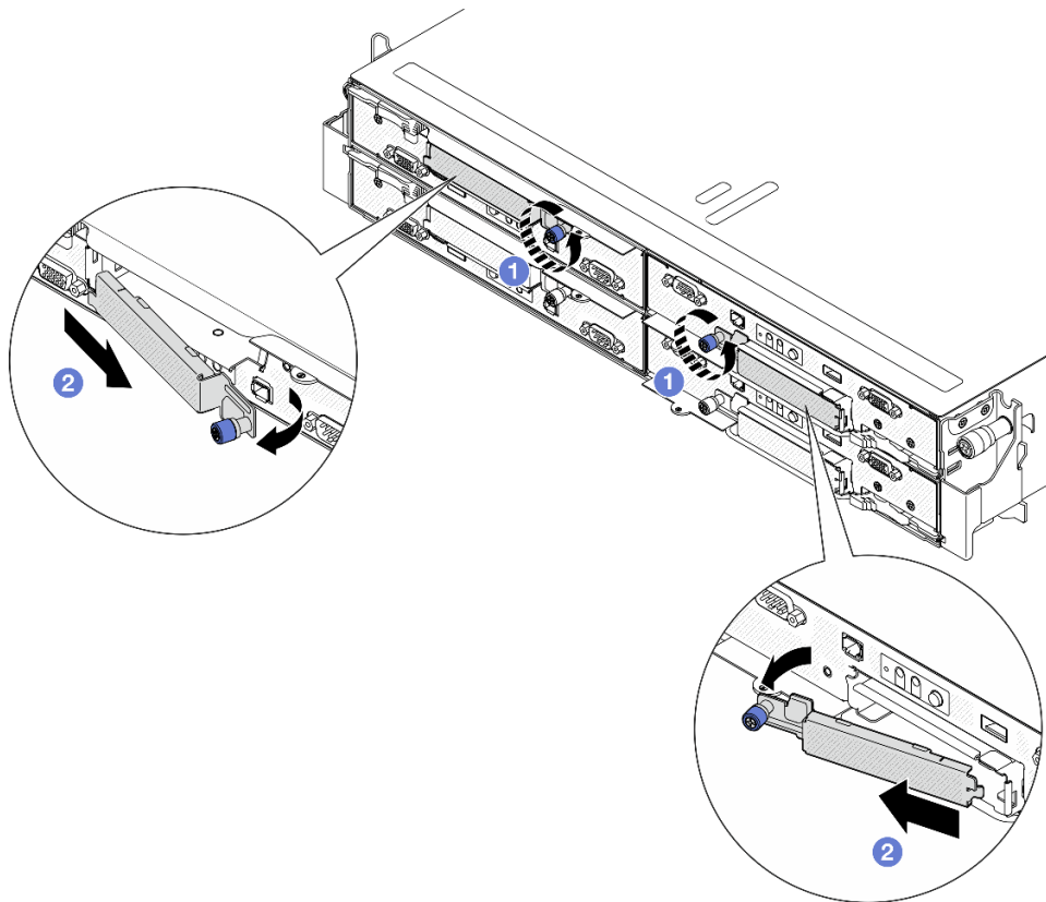
Figura 47. Rimozione del coperchio del telaio unità E3.S
