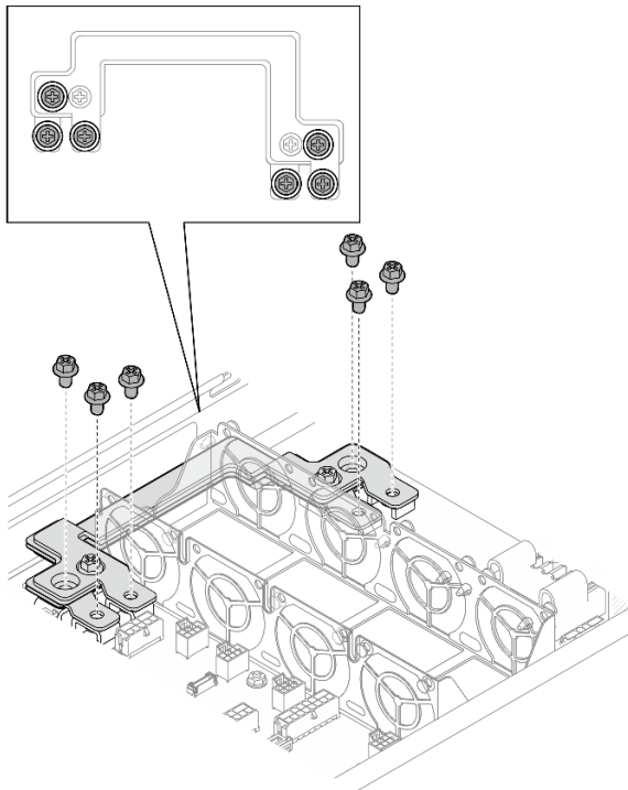
Figura 72. Rimozione delle viti esterne della barra del bus di alimentazione
