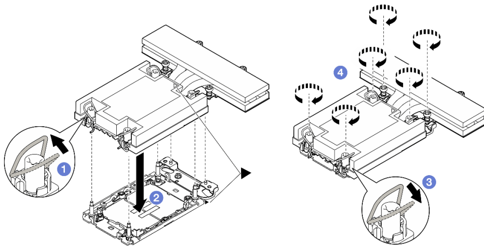
Figura 93. Installazione di un PHM 1U ad alte prestazioni per una configurazione con un processore
