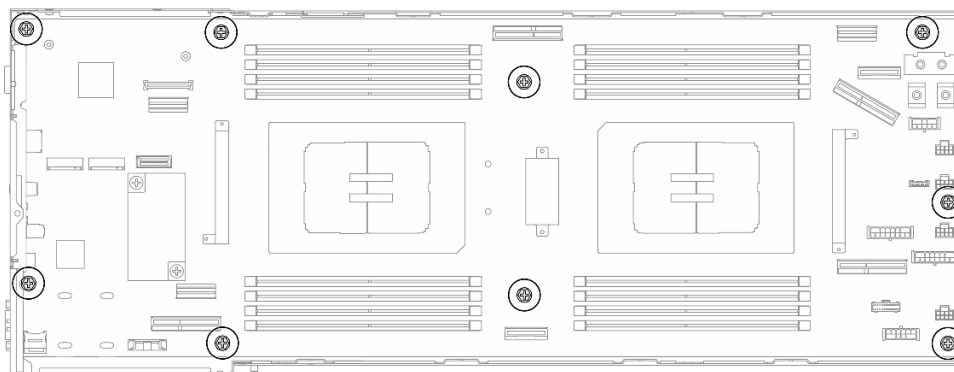
Figura 113. Installazione delle viti sulla scheda di sistema
