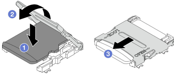
Figura 62. Installazione di una scheda MicroSD
