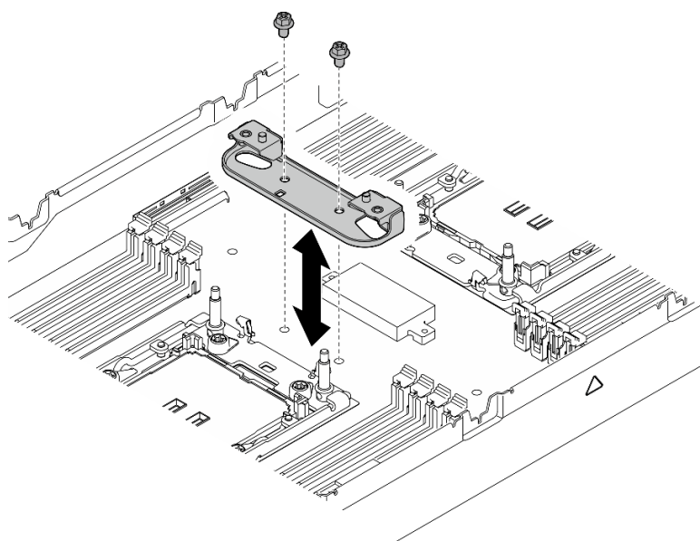
Figura 116. Sostituzione della staffa di supporto del dissipatore di calore
