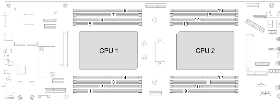
Figura 55. Layout dei moduli di memoria e dei processori
