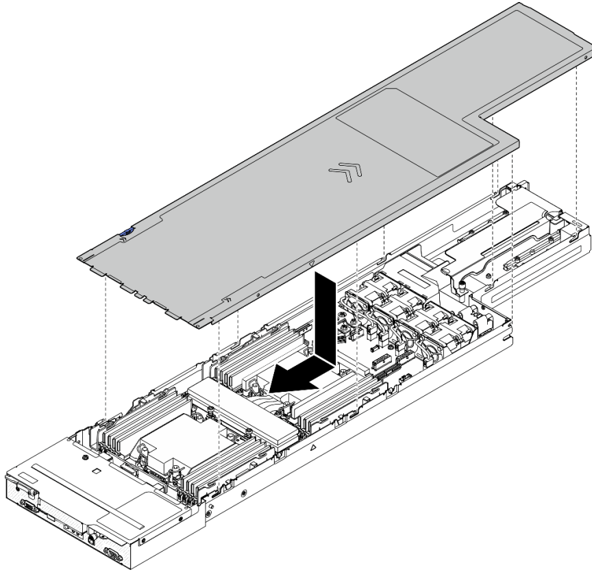
Figura 118. Installazione del coperchio superiore
