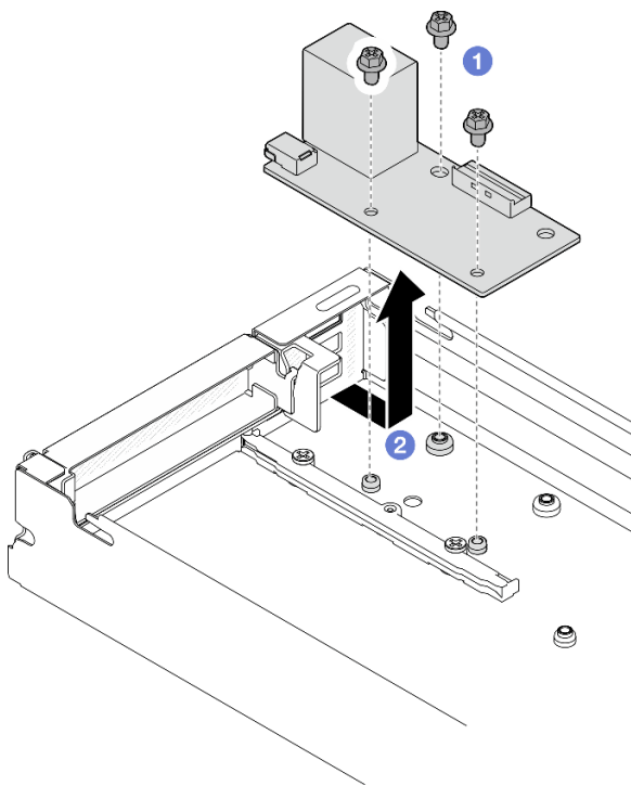
Figura 98. Rimozione del modulo I/O posteriore
