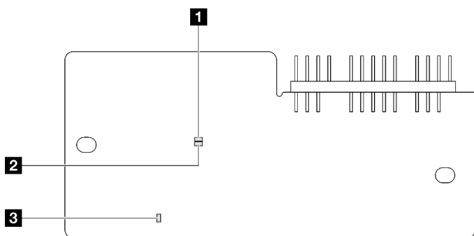
Figura 135. LED sul modulo firmware e sicurezza RoT
