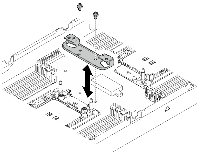
Figura 84. Sostituzione della staffa di supporto del dissipatore di calore
