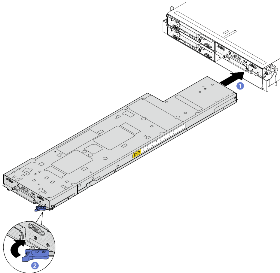
Figura 30. Installazione del nodo in un vassoio destro
