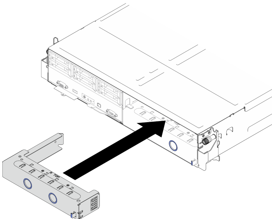
Figura 22. Installazione di un elemento di riempimento del vassoio del nodo anteriore
