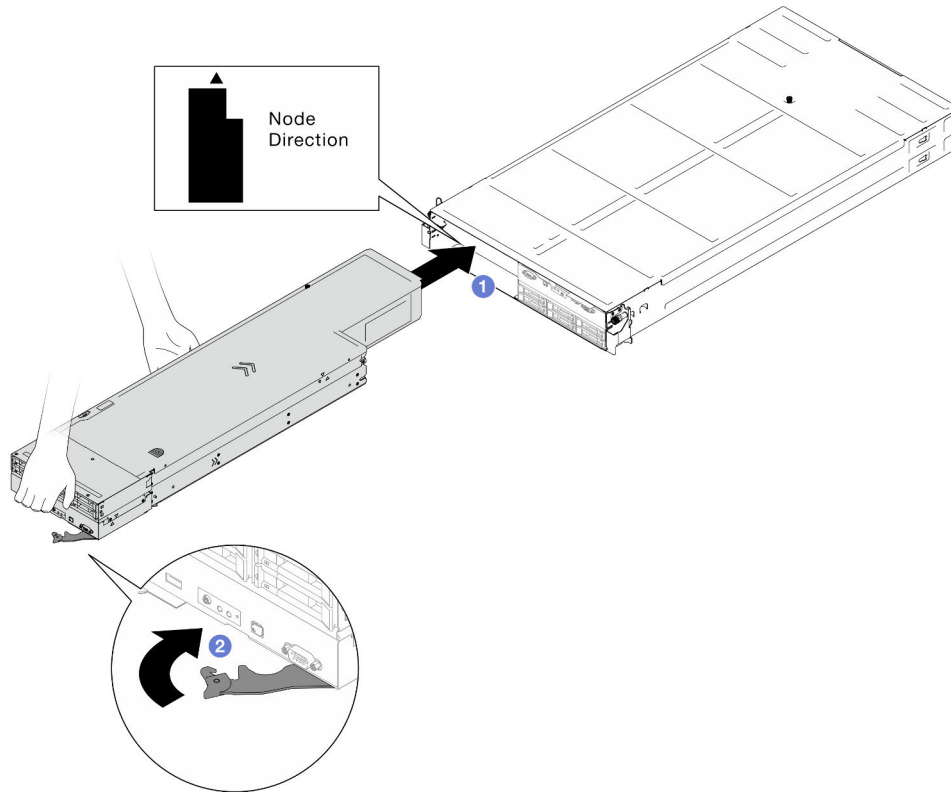
Figura 26. Installazione del nodo nel vassoio sinistro
