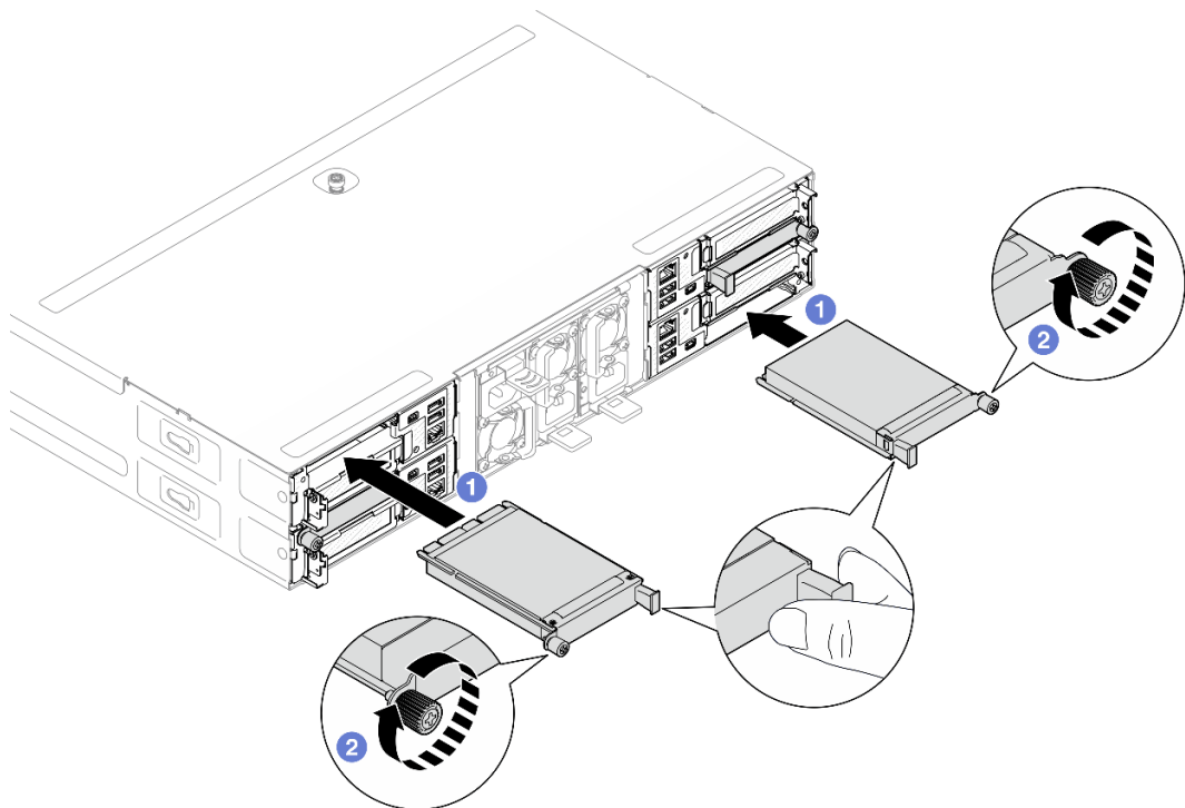
Figura 64. Installazione del modulo OCP posteriore
