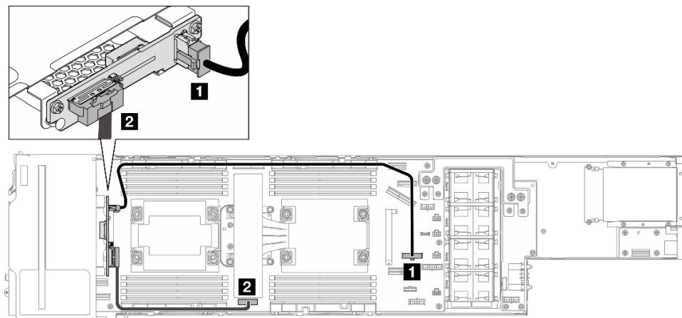
Figura 123. Instradamento dei cavi per il backplane dell'unità E3.S
