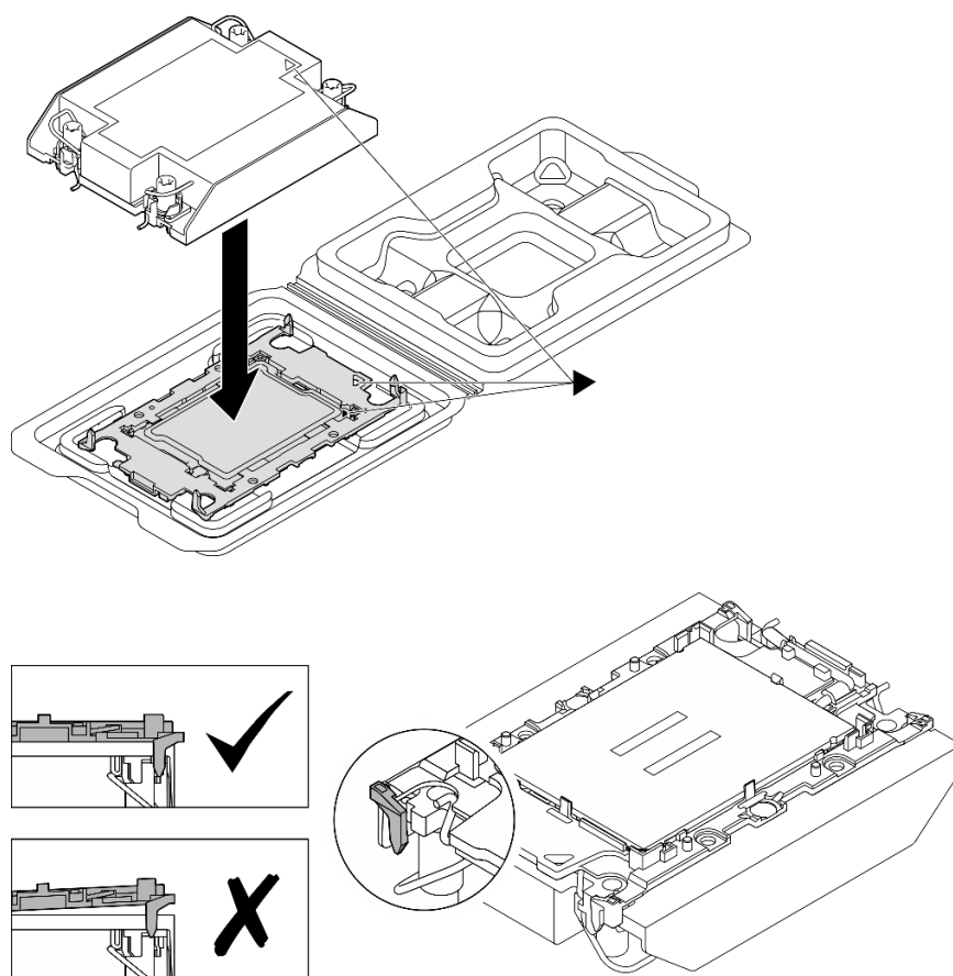
Figura 90. Assemblaggio del PHM con il processore nella confezione di spedizione
