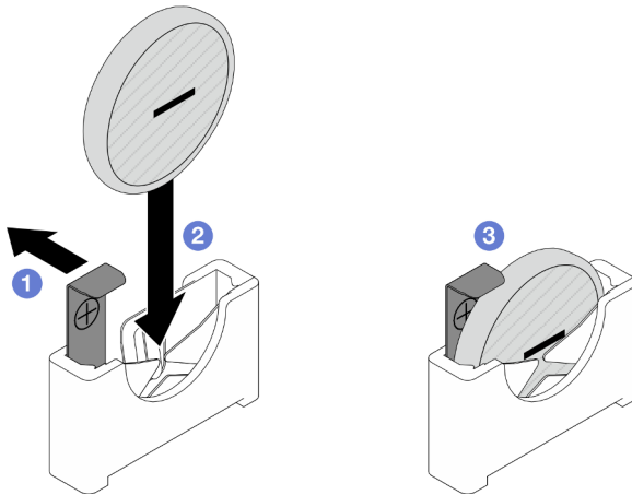
Figura 35. Installazione di una batteria CMOS
