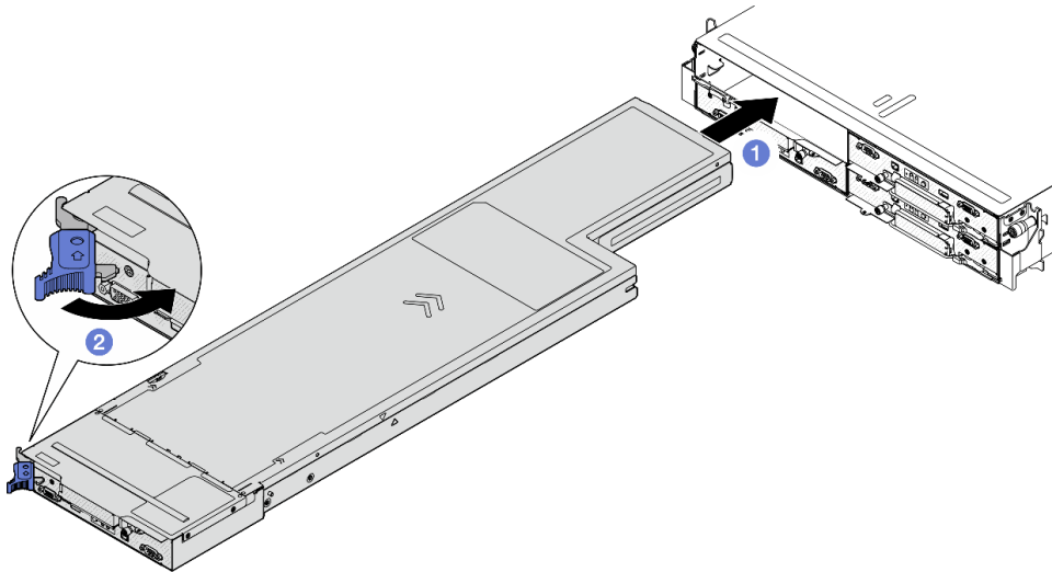
Figura 27. Installazione del nodo in un vassoio sinistro
