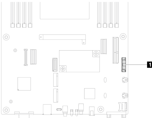
Figura 34. Posizione del socket della batteria CMOS
