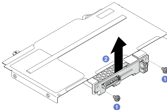
Figura 37. Rimozione del backplane dell'unità
