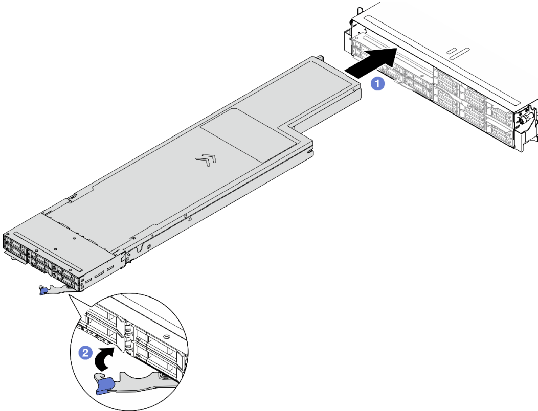
Figura 28. Installazione del nodo in un vassoio sinistro
