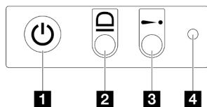
Figura 133. Pulsanti e LED sul pannello anteriore dell'operatore
