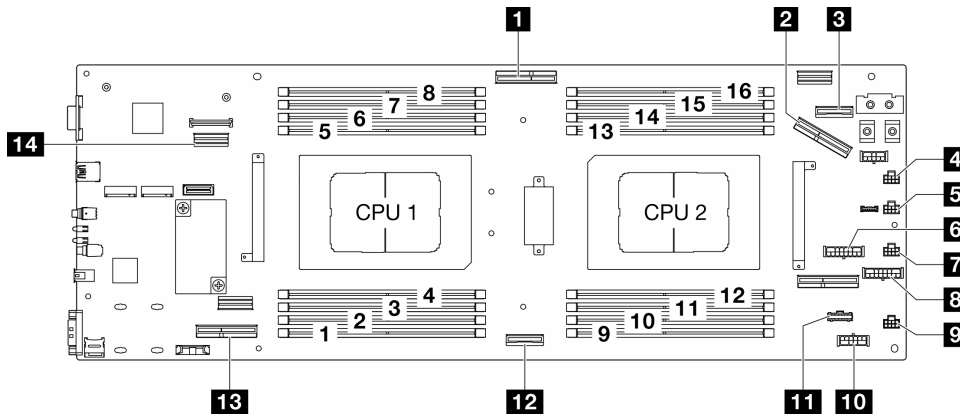
Figura 119. Connettori della scheda di sistema per l'instradamento dei cavi
