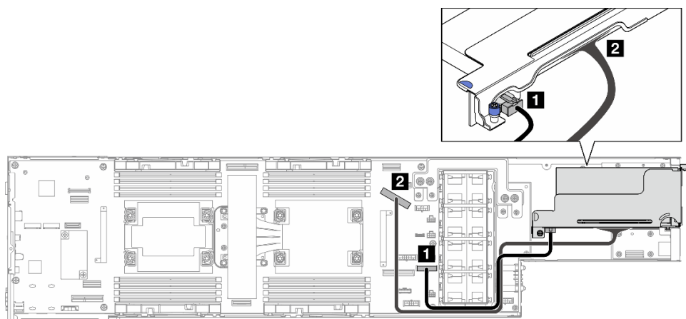
Figura 126. Instradamento dei cavi delle schede verticali PCIe – due processori
