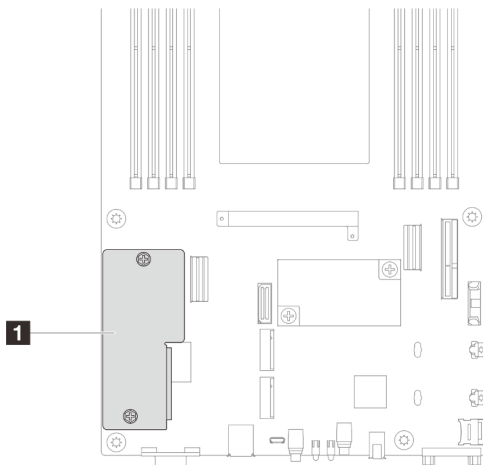
Figura 101. Posizione del Modulo firmware e sicurezza RoT
