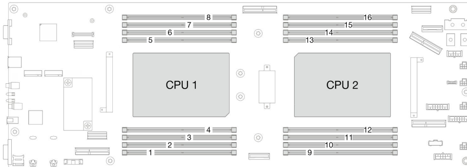
Figura 57. Layout dei moduli di memoria e dei processori
