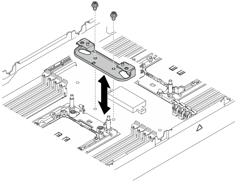
Figura 105. Sostituzione della staffa di supporto del dissipatore di calore
