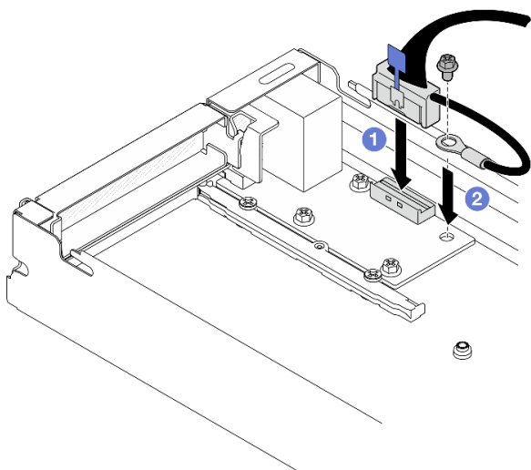
Figura 129. Installazione del cavo I/O posteriore e del cavo di messa a terra
