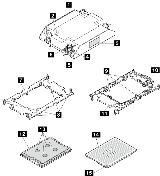
Figura 78. Componenti del PHM
