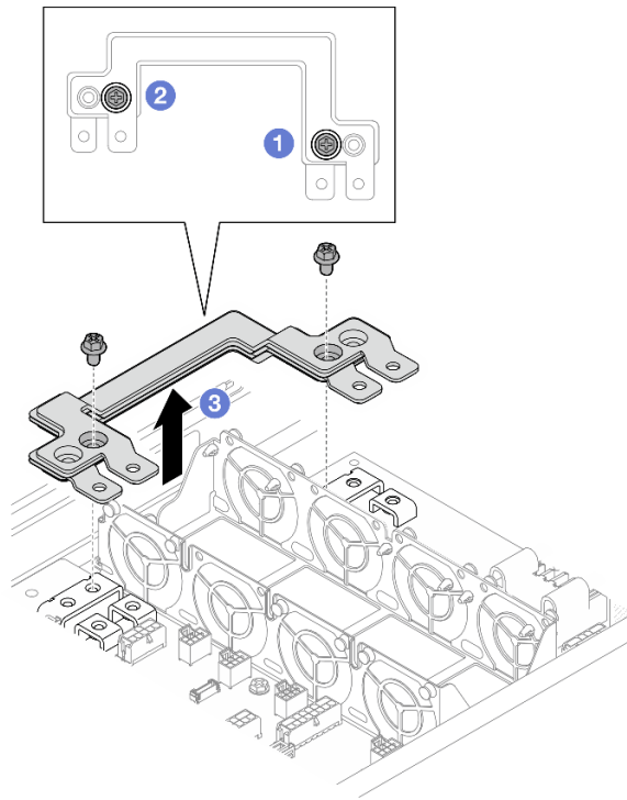
Figura 73. Rimozione della barra del bus di alimentazione
