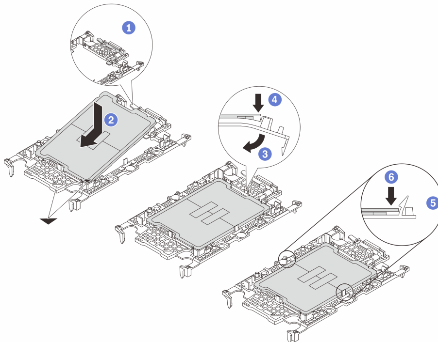
Figura 88. Installazione della piastra del processore
