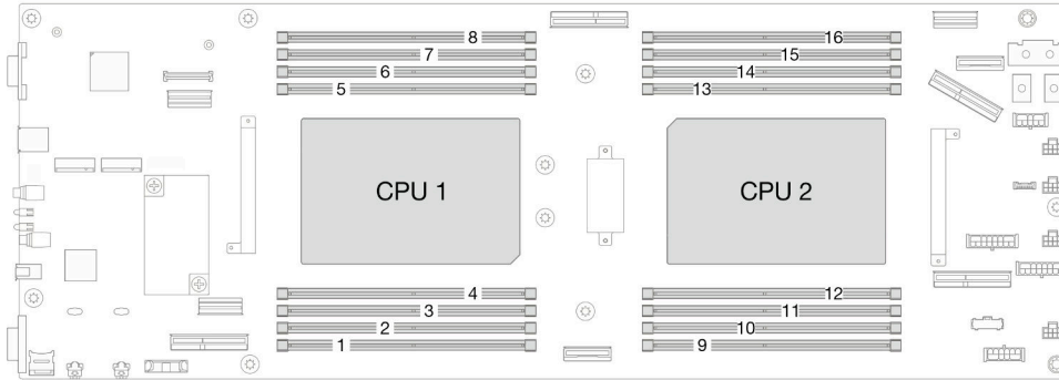
図 55. メモリー・モジュールおよびプロセッサのレイアウト
