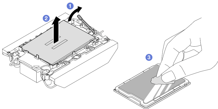
図85. プロセッサをキャリアとヒートシンクから取り外す
