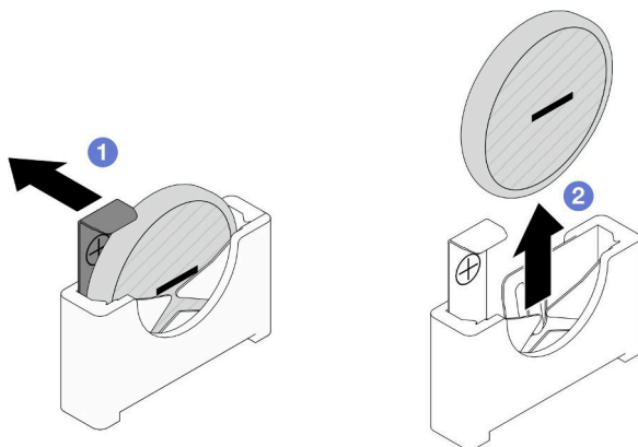
図 33. CMOS バッテリーの取り外し
