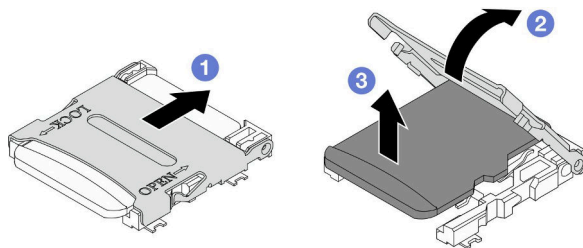
図 60. MicroSD カードの取り外し
