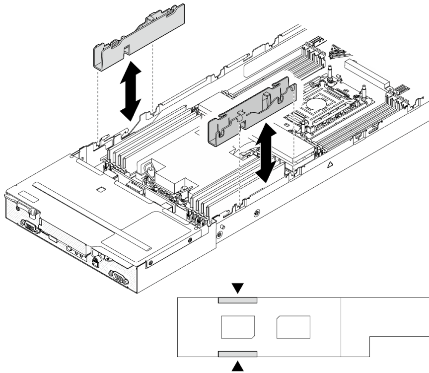
図 106. ケーブル・ダクトの交換 (プロセッサ構成 1 つ)
