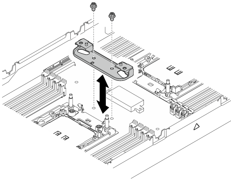
図 105. ヒートシンク・サポート・ブラケットの交換
