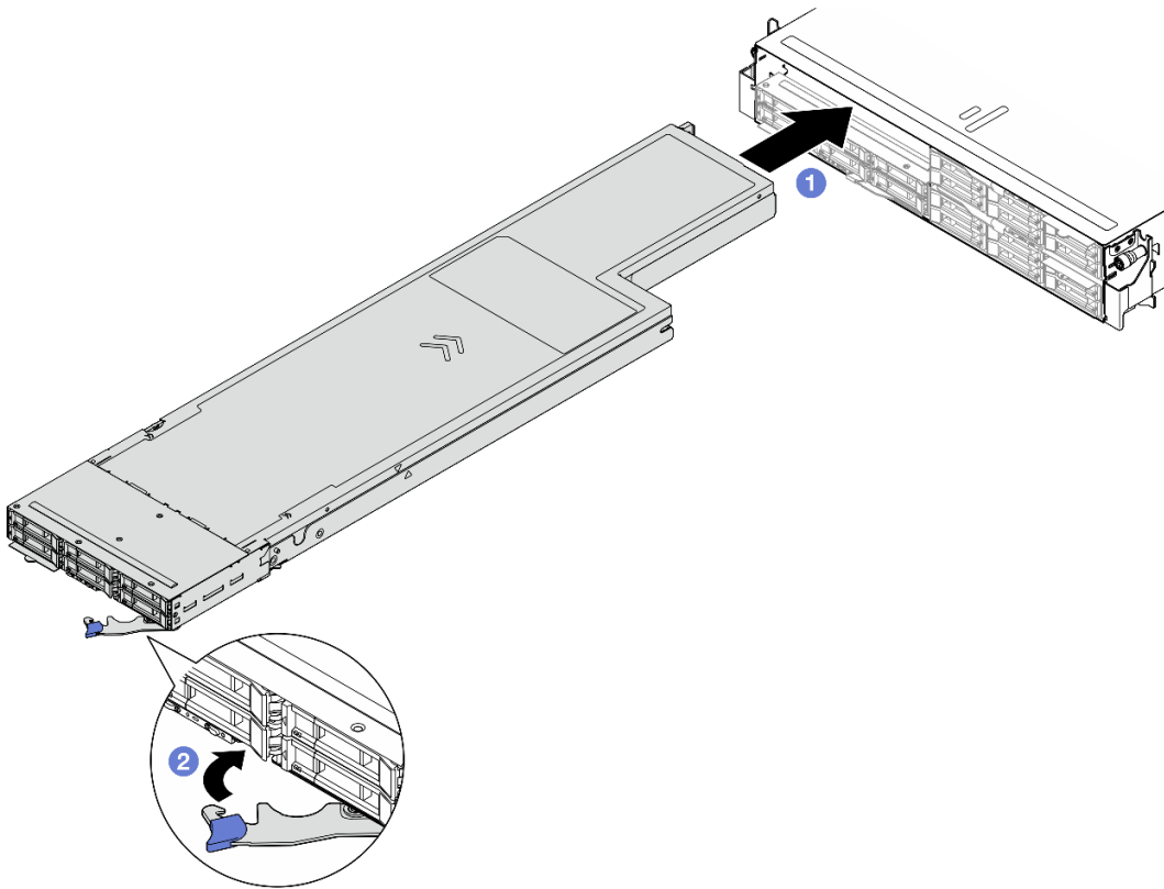
図 28. 左トレイへのノードの取り付け
