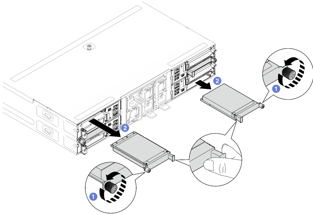
図63. 背面 OCP モジュールの取り外し
