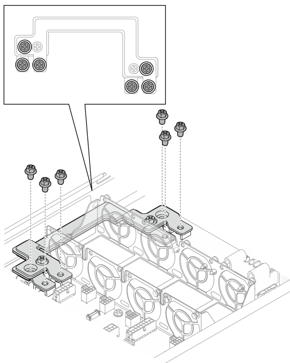
図 72. 電源バス・バーの外側ねじの取り外し
