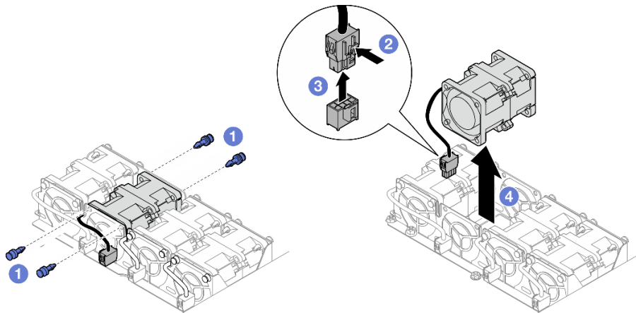
図40. ファンの取り外し
