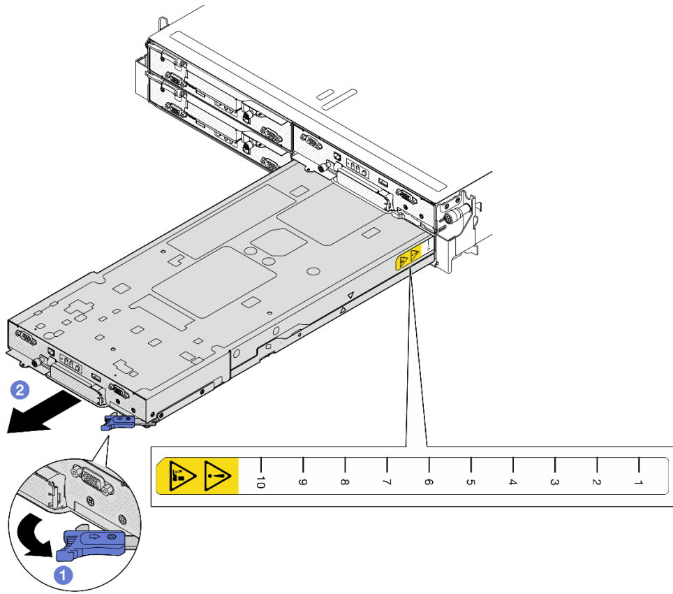
図20. 右トレイからのノードの取り外し
