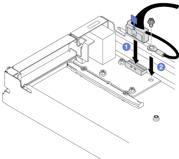
図 129. 背面 I/O ケーブルと接地用ケーブルの取り付け
