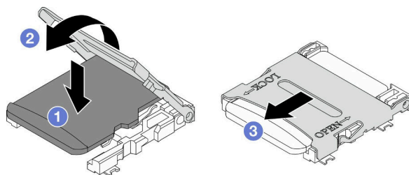
図 62. MicroSD カードの取り付け
