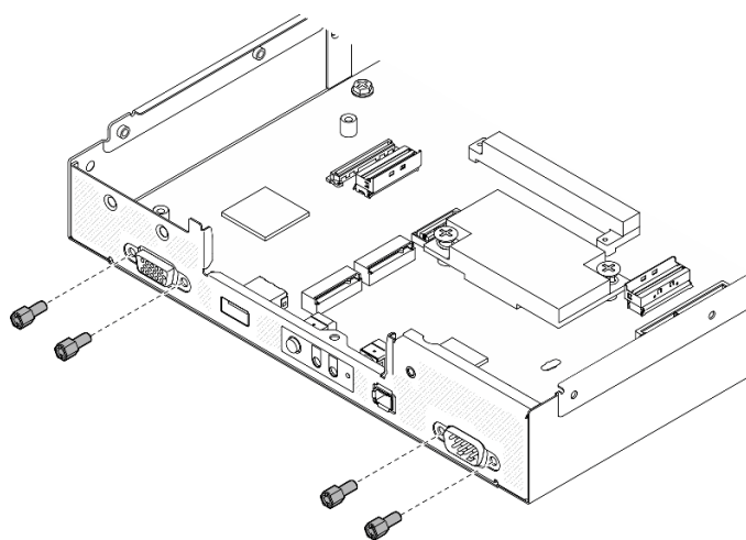
図108. ねじの取り外し
