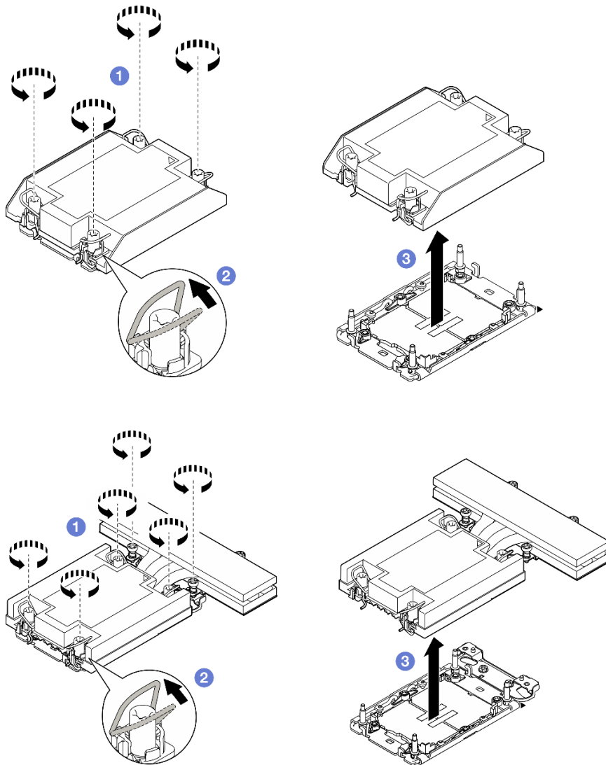
図 82. プロセッサ 1 から 1U パフォーマンス PHM を取り外す
