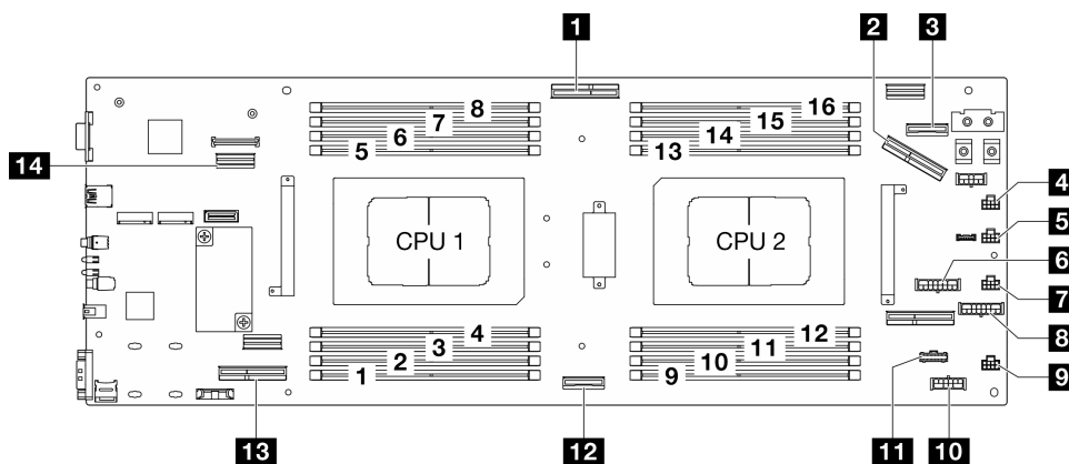
図 119. ケーブル配線用のシステム・ボード・コネクタ
