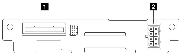
図 120. E3.S ドライブ・バックプレーン・コネクタ
