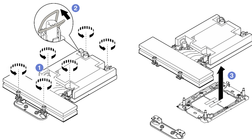
図83. プロセッサ-2から1UパフォーマンスPHMを取り外す
