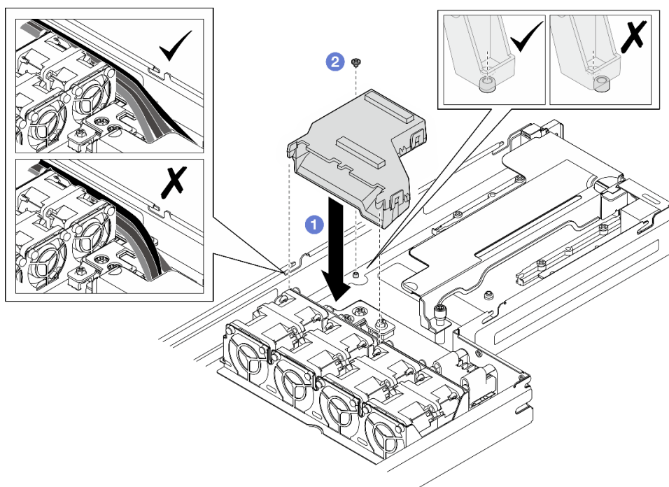
図 43. GPU エアークラウドの取り付け
