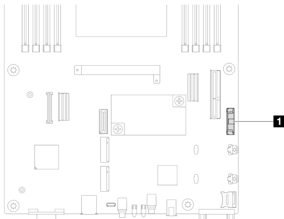
図 32. CMOS バッテリー・ソケットの位置
