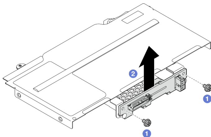
図 37. ドライブ・バックプレーンの取り外し
