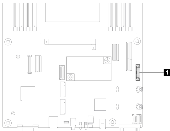
図 34. CMOS バッテリー・ソケットの位置
