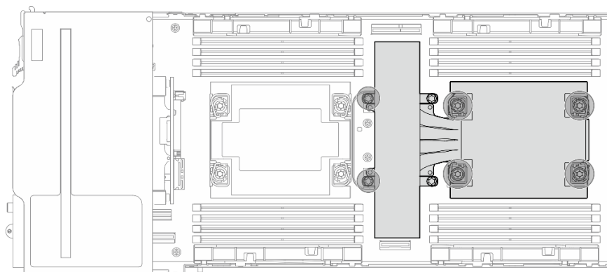
図80. 2 プロセッサ構成のPHMの位置
