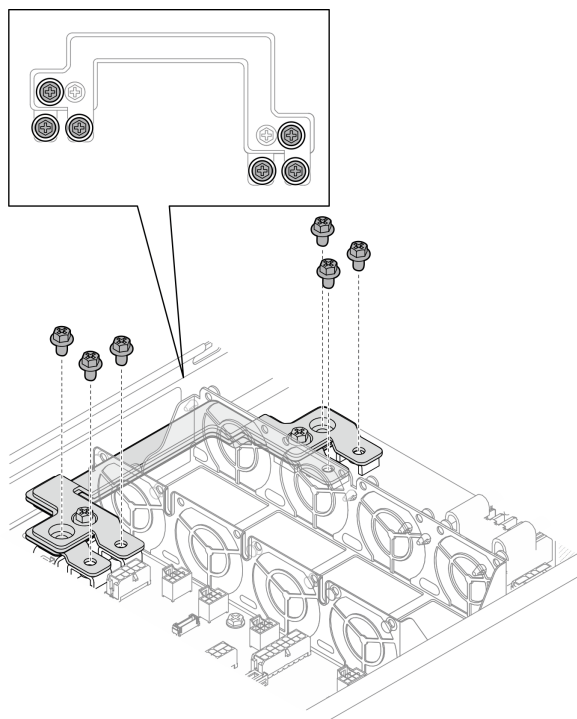
図75. 電源バス・バーねじの取り付け
