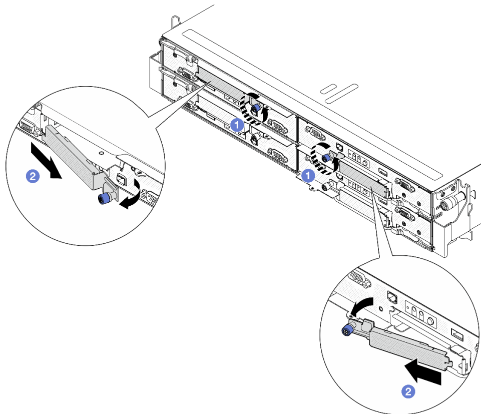
図 44. E3.S ドライブ・ケージ・カバーの取り外し
