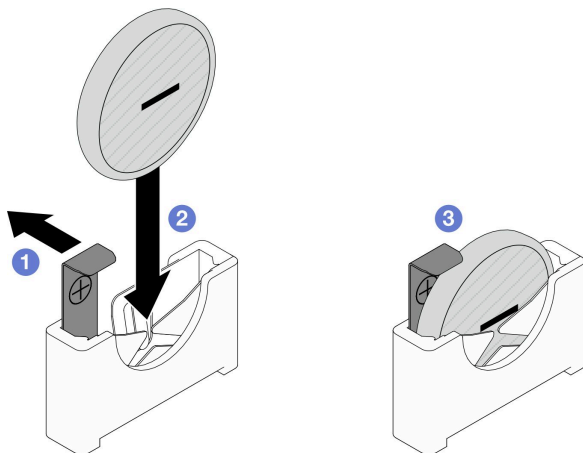
図 35. CMOS バッテリーの取り付け
