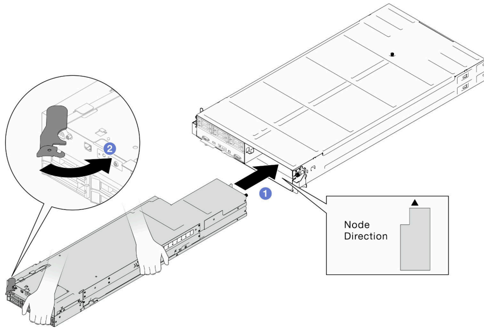
図 29. 右トレイへのノードの取り付け
