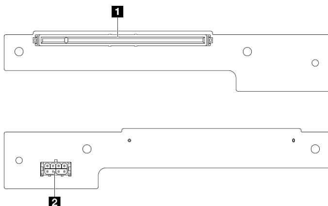
図 121. PCIe ライザー・カード・コネクタ
