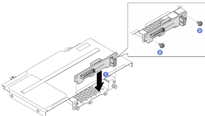
図38. ドライブ・バックプレーンの取り付け
