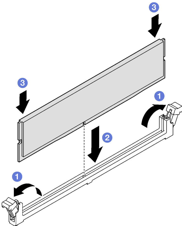
図 58. メモリー・モジュールの取り付け
