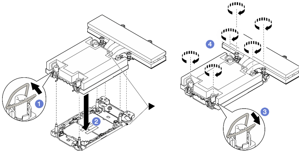
図93. 1 プロセッサ構成の 1U パフォーマンス PHM の取り付け
