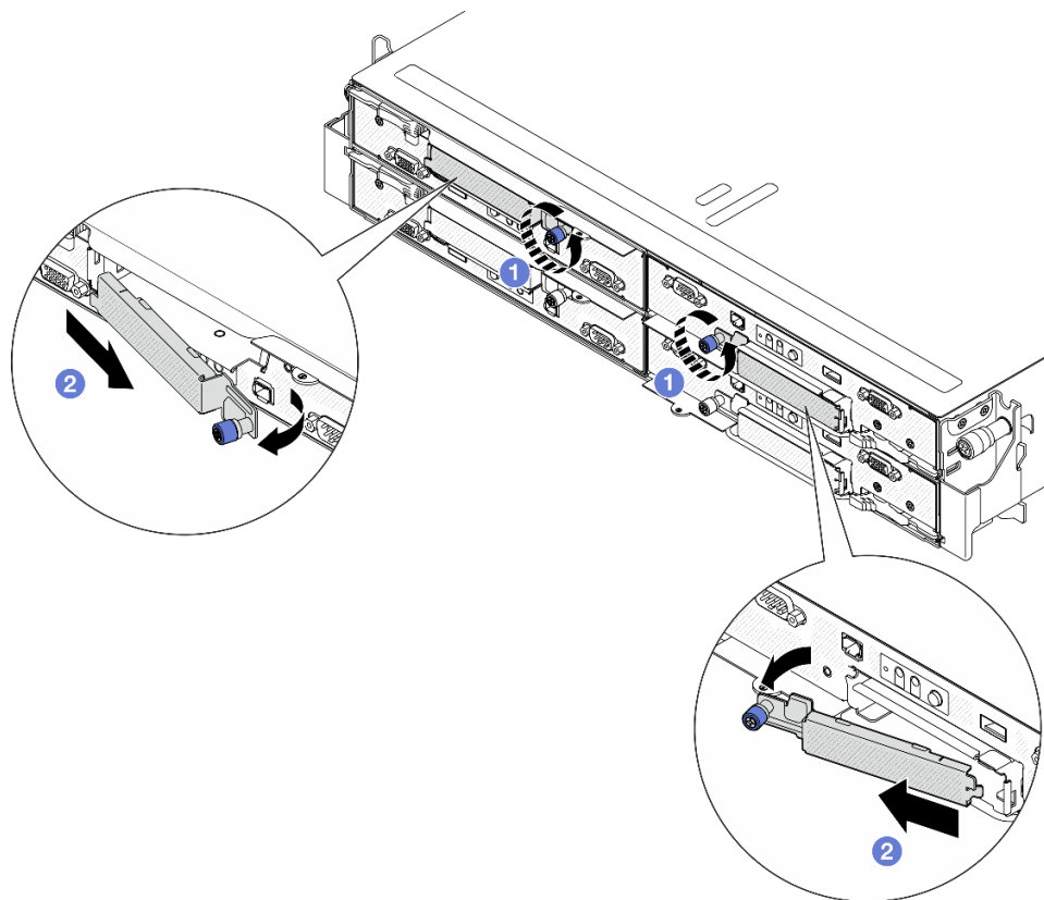
図 47. E3.S ドライブ・ケージ・カバーの取り外し
