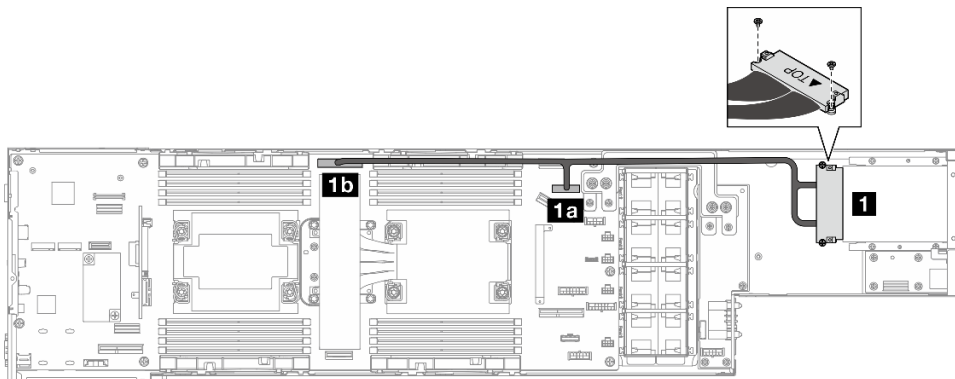
図 128. 背面 I/O モジュールと OCP モジュールのケーブル
