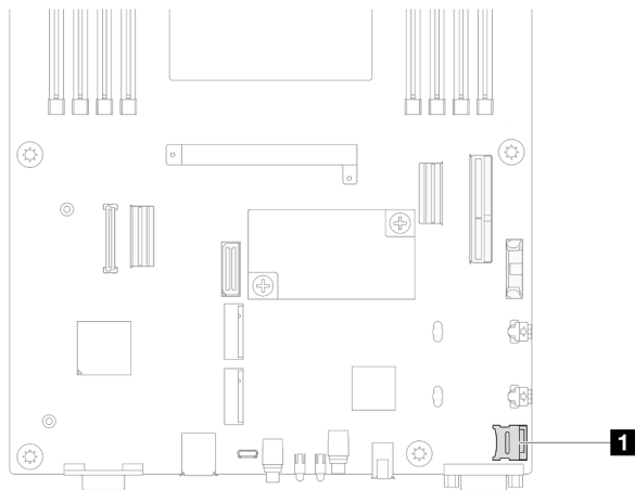
図 59. MicroSD ソケットの位置
