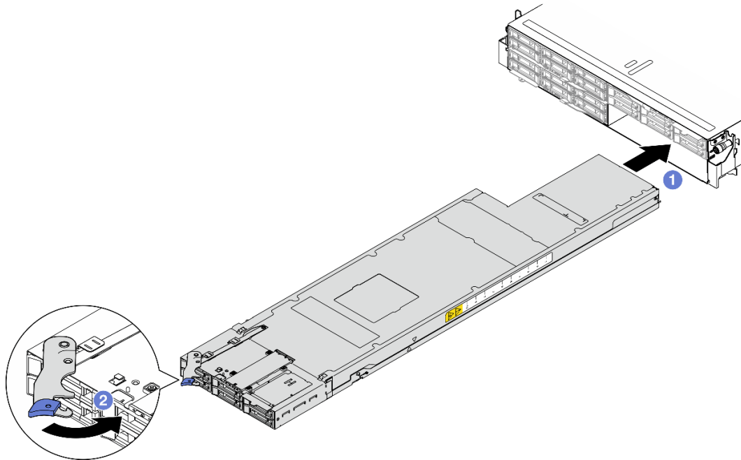
図31. 右トレイへのノードの取り付け
