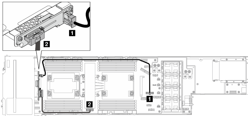
図 123. E3.S ドライブ・バックプレーンのケーブル配線
