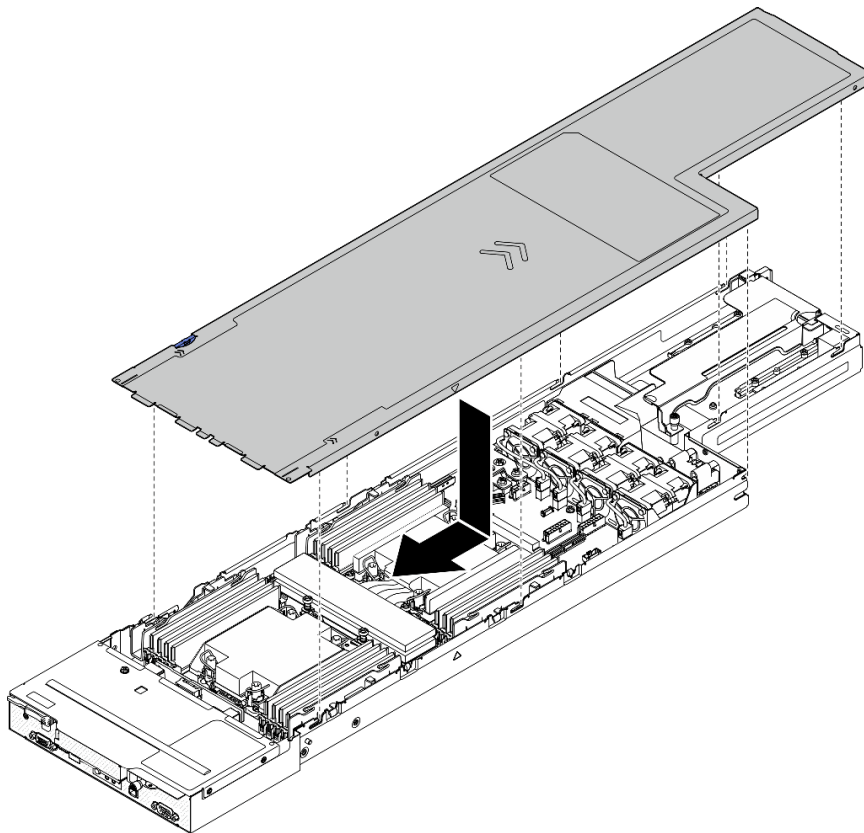
図118. トップ・カバーの取り付け
