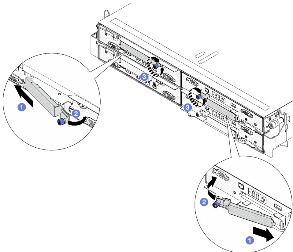
図 49. E3.S ドライブ・ケージ・カバーの取り付け
