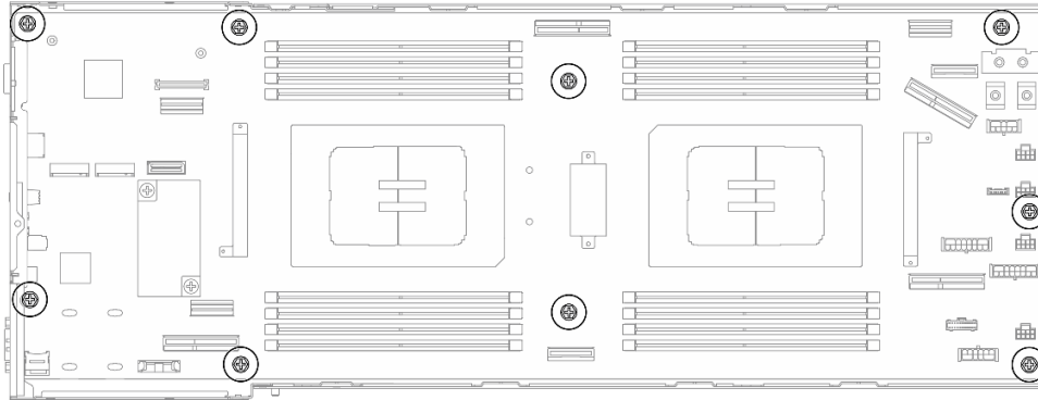
図109. ねじの取り外し
