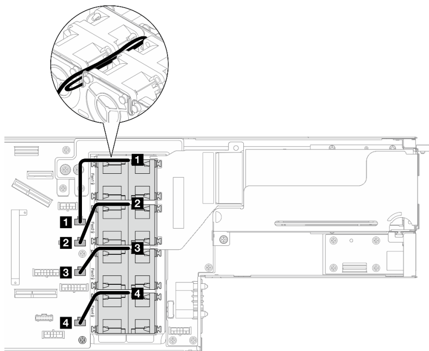
図 124. ファンのケーブル配線
