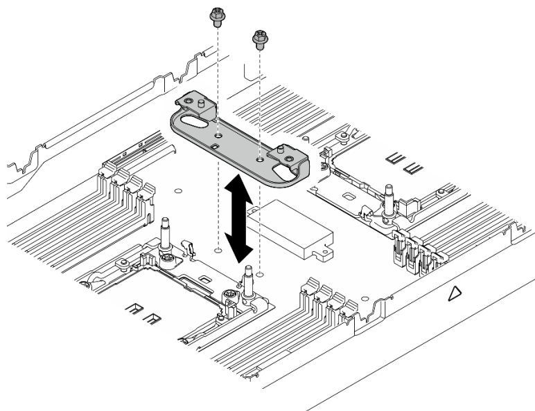
図84. ヒートシンク・サポート・ブラケットの交換
