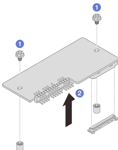
図 102. ファームウェアおよび RoT セキュリティー・モジュールの取り外し
