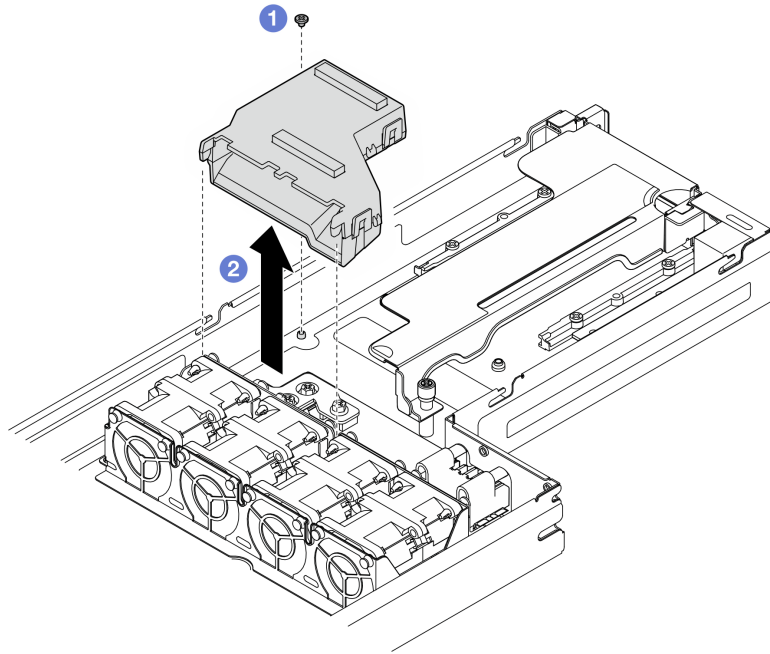
図 42. GPU エアー・ダクトの取り外し
