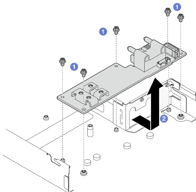
図 76. 分電盤の取り外し
