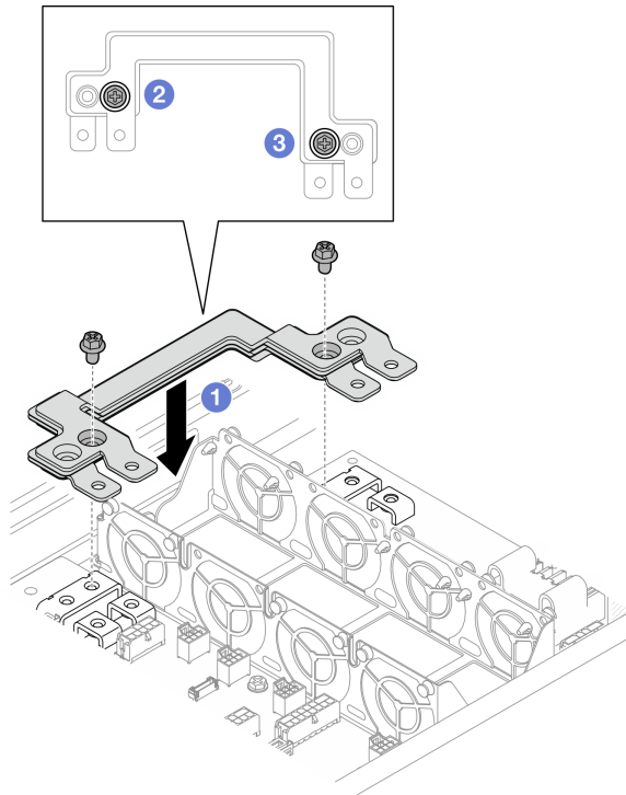
図 74. 電源バス・バーの取り付け
