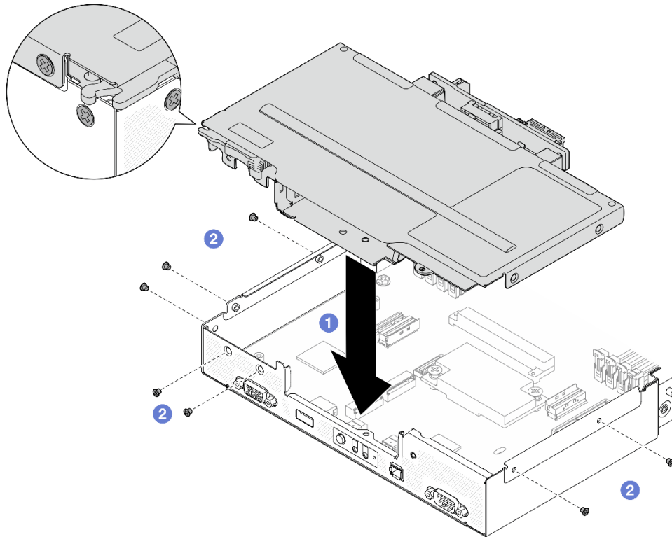
図 39. ドライブ・ケージ・アセンブリの取り付け
