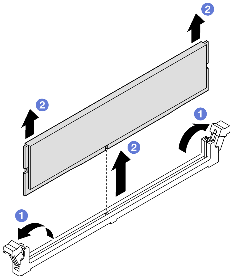
図 56. メモリー・モジュールの取り外し
