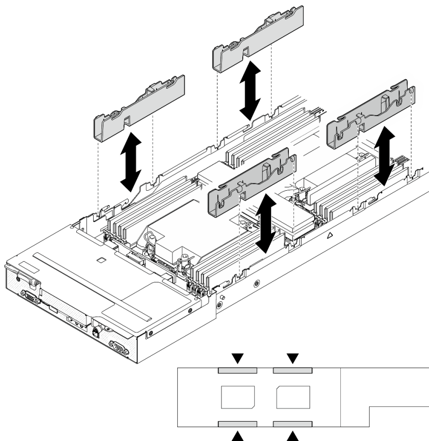
図 115. ケーブル・ダクトの交換 (プロセッサ構成 2 つ)
