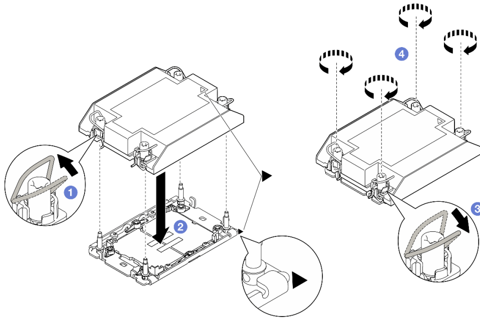
図95. 2 プロセッサ構成の 1U スタANDARD PHM の取り付け
