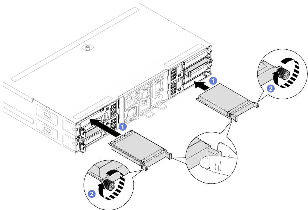
図 64. 背面 OCP モジュールの取り付け
