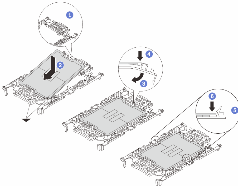
図88. プロセッサ・キャリアの取り付け
