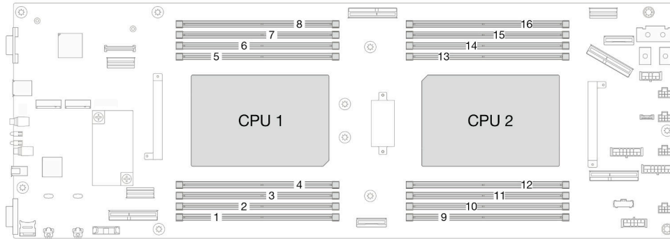
図57. メモリー・モジュールおよびプロセッサのレイアウト
