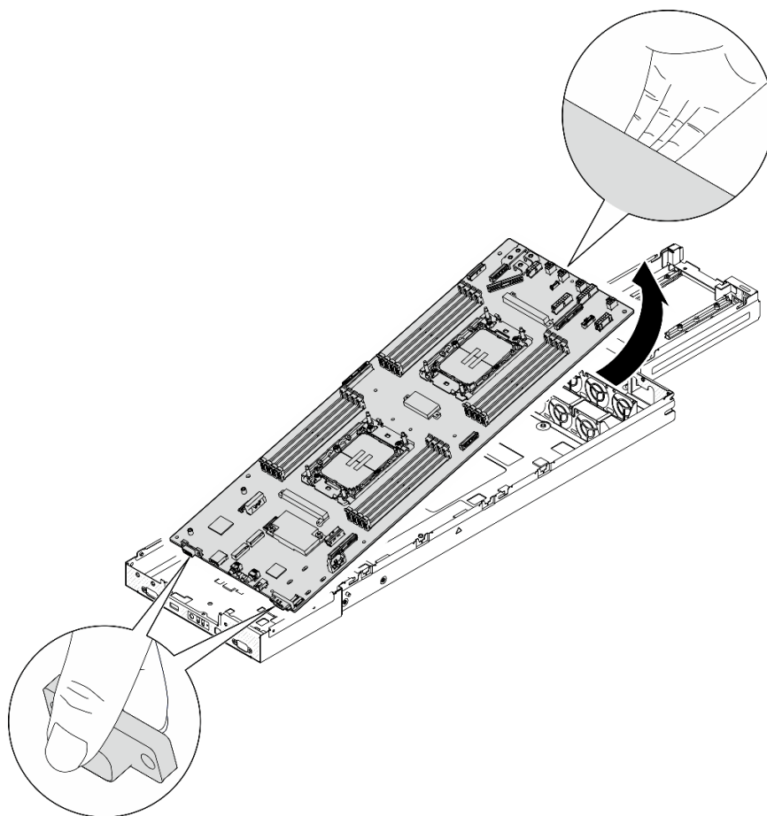
図110. システム・ボードの取り外し
