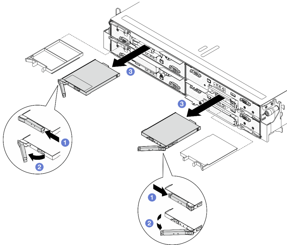
図45. E3.S ホット・スワップ・ドライブの取り外し
