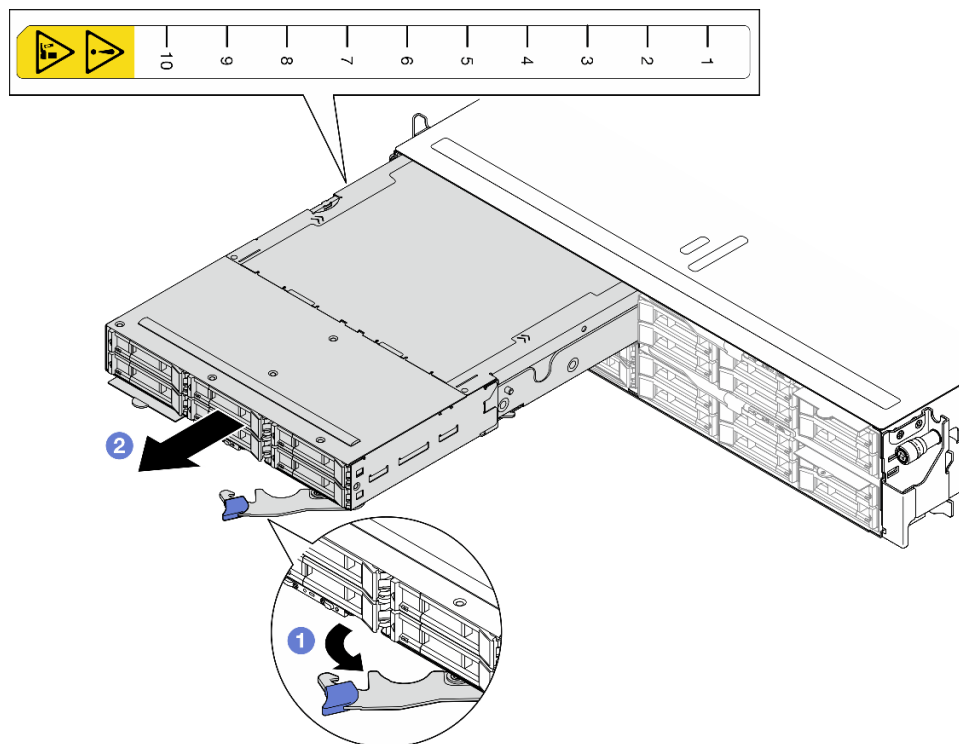
図 18. 左トレイからの ノードの取り外し
