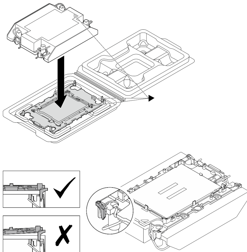
図90. 配送用トレイのプロセッサでPHMを取り付けます。
