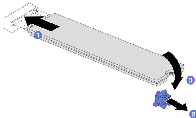
図54. M.2 ドライブの取り付け
