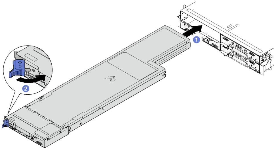
図 27. 左トレイへのノードの取り付け
