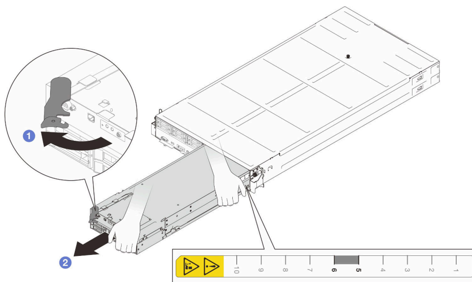
図 19. 右トレイからの ノードの取り外し
