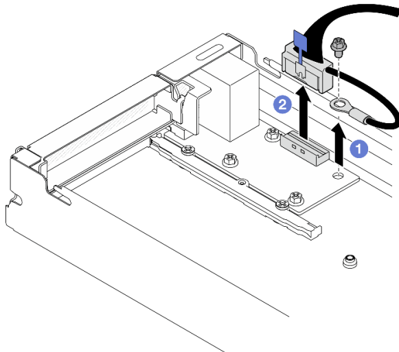
図 97. 背面 I/O ケーブルと接地用ケーブルの取り外し
