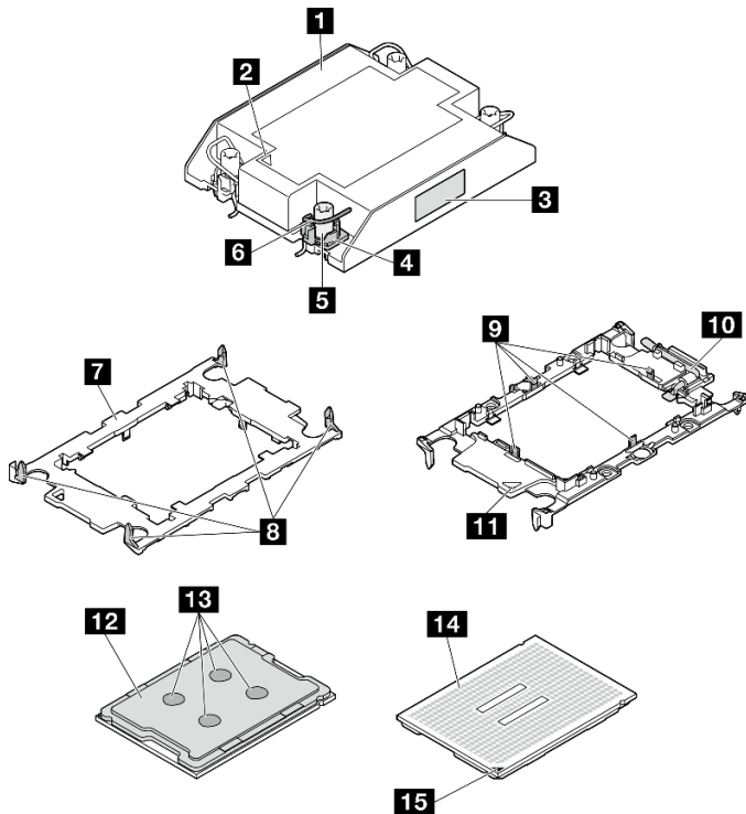
図 78. PHM コンポーネント
