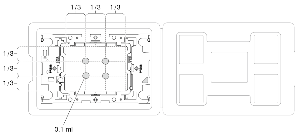
図 89. 配送トレイのプロセッサで熱伝導グリースを塗布する
