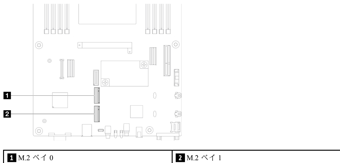
図 50. システム・ボードの M.2 ベイの位置
