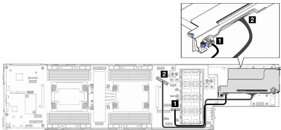
図 126. PCIe ライザーのケーブル配線 - プロセッサ 2 個
