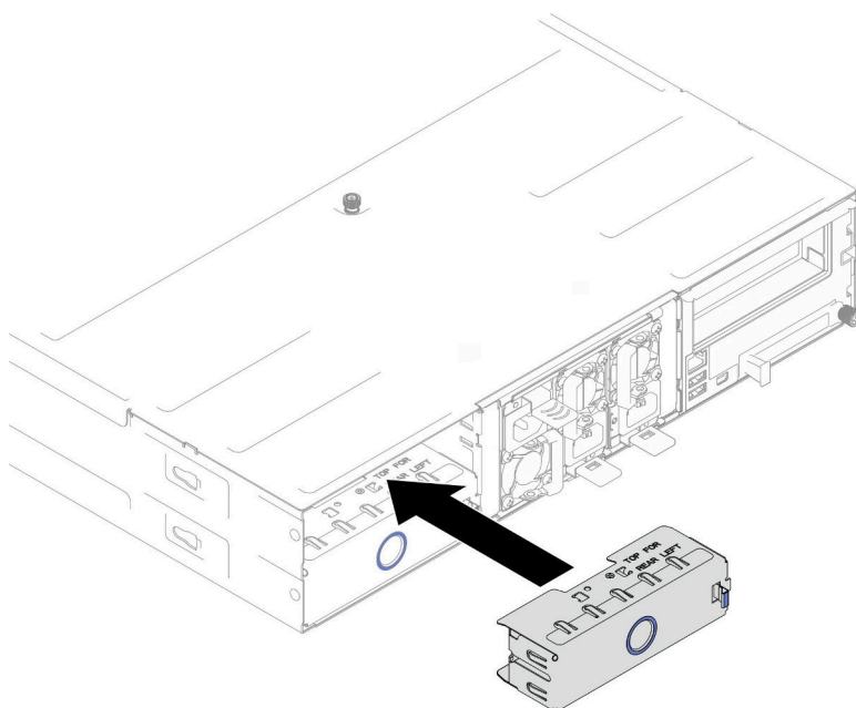
図23. 背面ノード・トレイ・フィルターの取り付け
