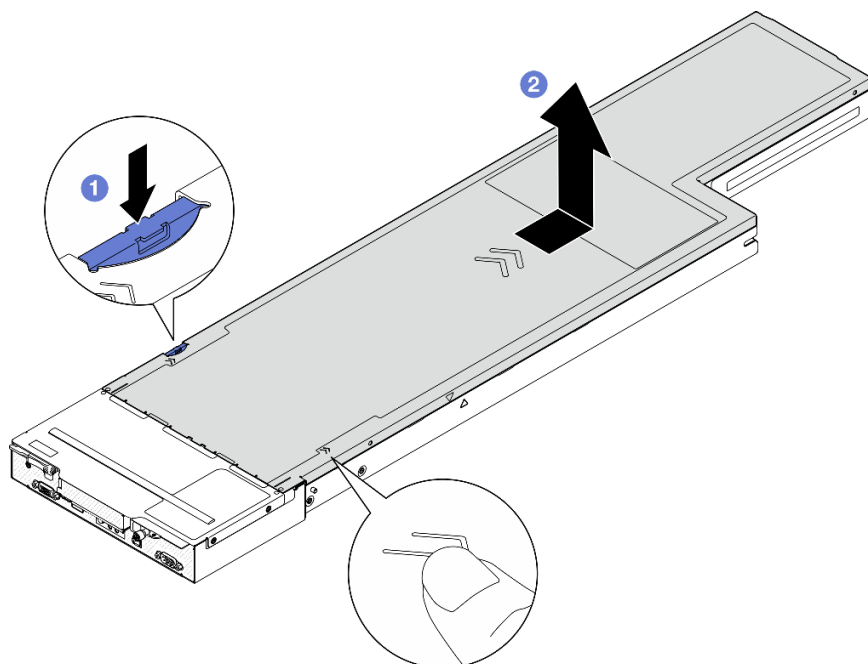
図 117. トップ・カバーの取り外し
