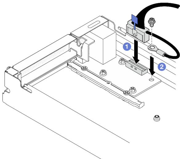
図 100. 背面 I/O ケーブルと接地用ケーブルの取り付け
