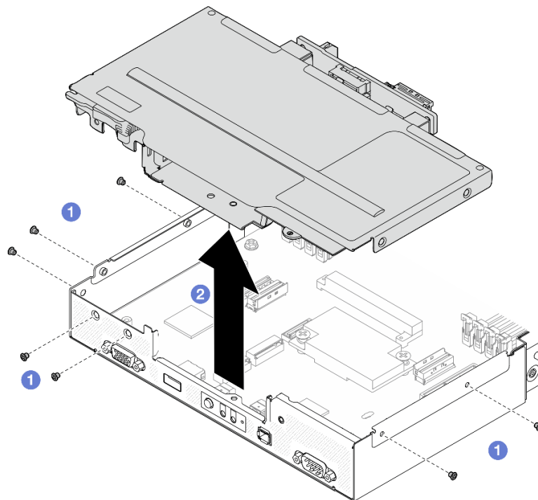
図 36. ドライブ・ケージ・アセンブリーの取り外し
