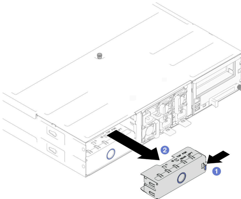
図 25. 背面ノード・トレイ・フィルターの取り外し
