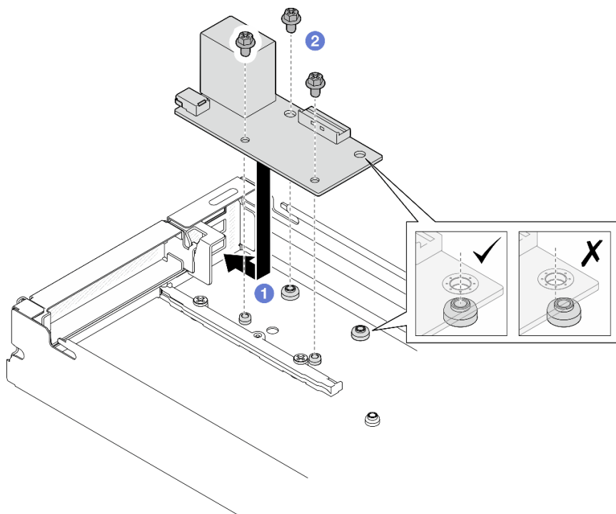
図 99. 背面 I/O モジュールの取り付け
