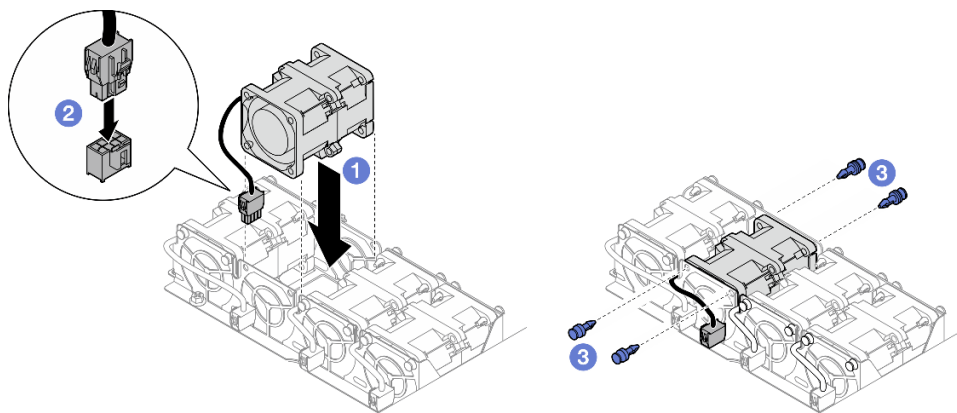
図 41. ファンの取り付け
