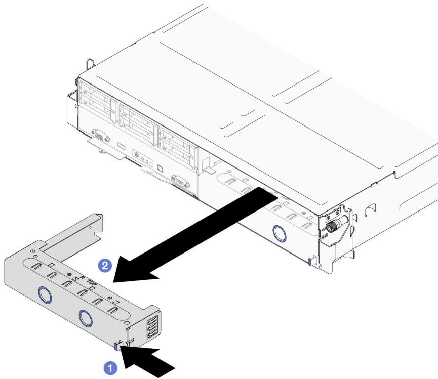
図 24. 前面ノード・トレイ・フィルターの取り外し
