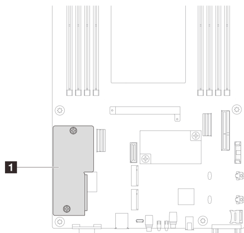
図 103. ファームウェアおよび RoT セキュリティ・モジュール の位置
