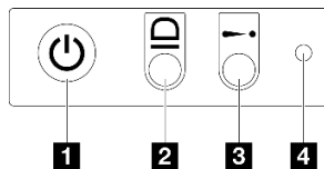
図 133. 前面オペレーター・パネル・ボタンと LED
