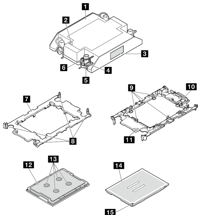
図 87. PHM コンポーネント
