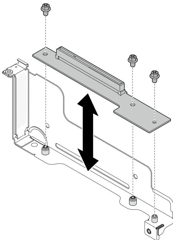
図 68. PCIe ライザー・カードの交換
