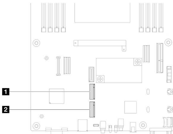
図53. システム・ボードの M.2 ベイの位置
