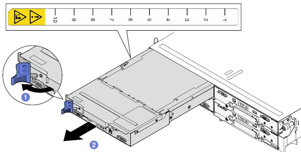
図 17. 左トレイからのノードの取り外し
