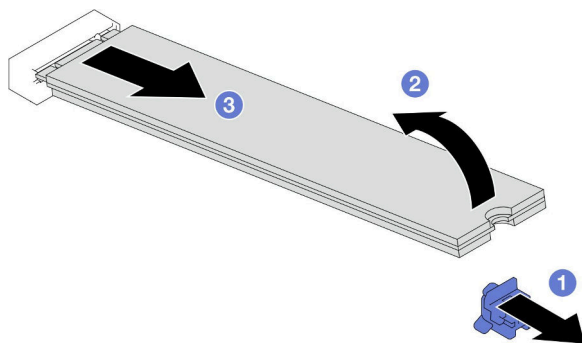
図 51. M.2 ドライブの取り外し
