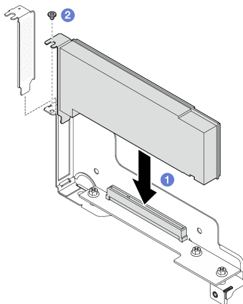
図 69. PCIe アダプターの取り付け
