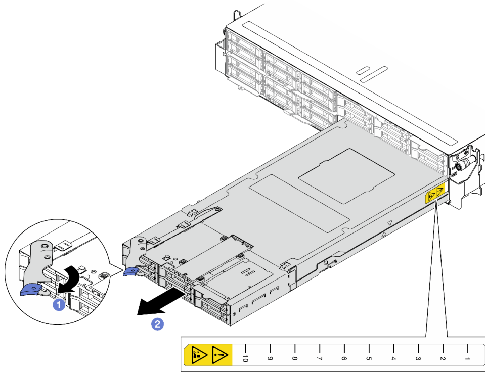
図21. 右トレイからのノードの取り外し
