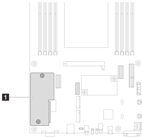
図 101. ファームウェアおよび RoT セキュリティー・モジュールの位置
