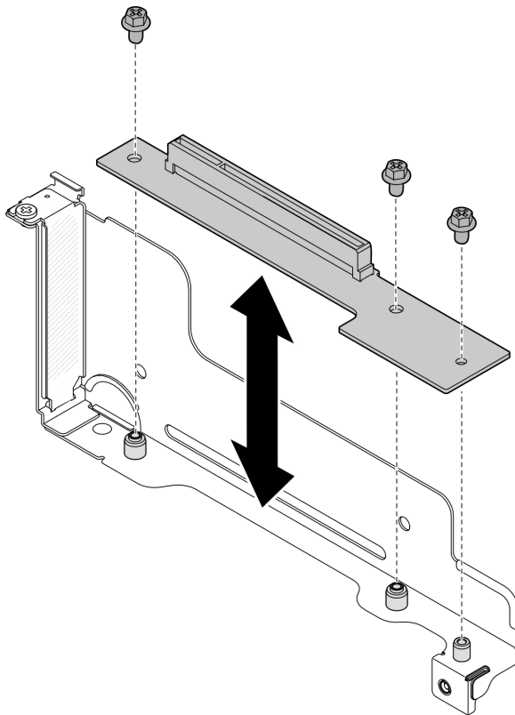
図70. PCIe ライザー・カードの交換
