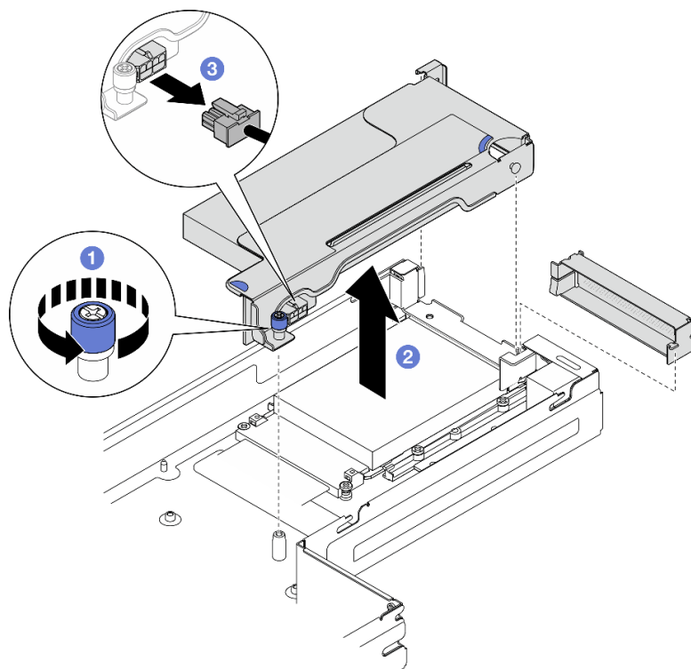
図 65. PCIe ライザー・アセンブリーの取り外し
