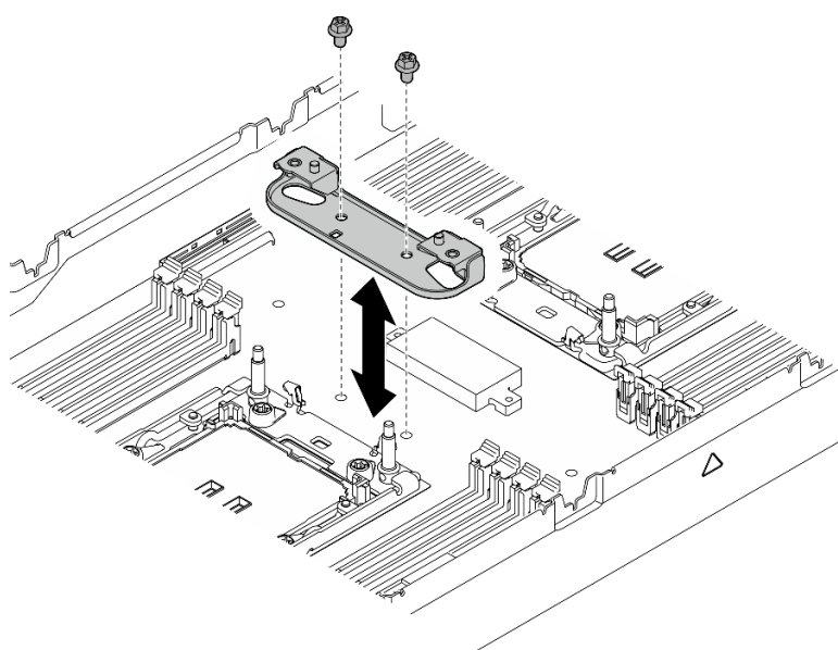
図 116. ヒートシンク・サポート・ブラケットの交換
