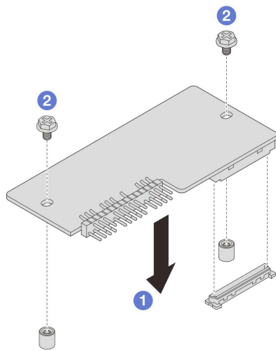
図 104. ファームウェアおよび RoT セキュリティ・モジュール の取り付け
