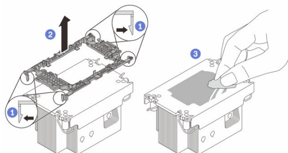
図86. ヒートシンクからプロセッサ・キャリアを取り外す
