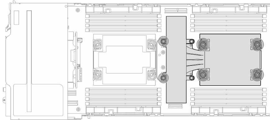
図94. 2 プロセッサ構成の PHM の位置
