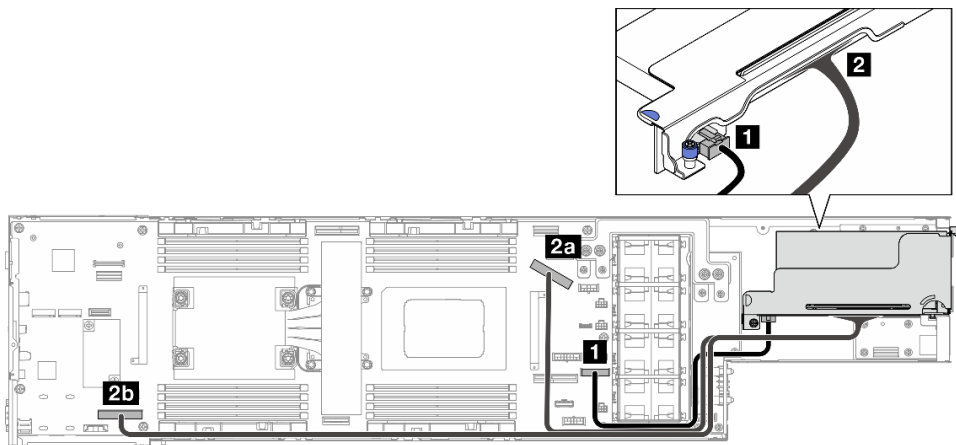
図 125. PCIe ライザーのケーブル配線 - プロセッサ x 1
