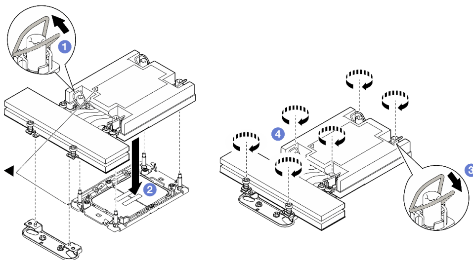
図 96. 2 プロセッサ構成の 1U パフォーマンス PHM の取り付け
