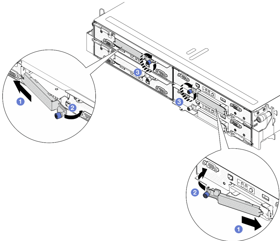
図46. E3.S ドライブ・ケージ・カバーの取り付け
