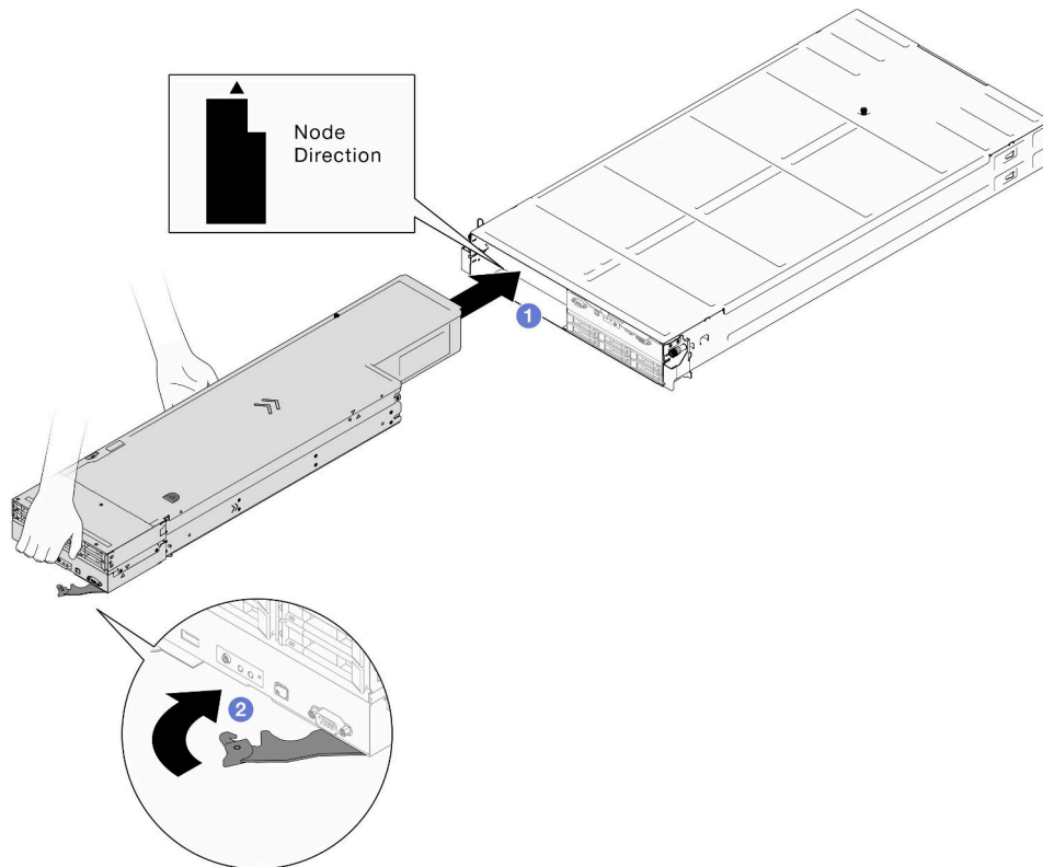
図 26. 左トレイへのノードの取り付け
