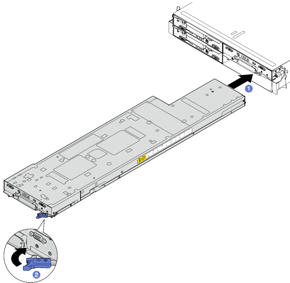
図 30. 右トレイへのノードの取り付け
