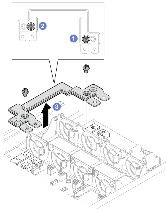
図 73. 電源バス・バーの取り外し
