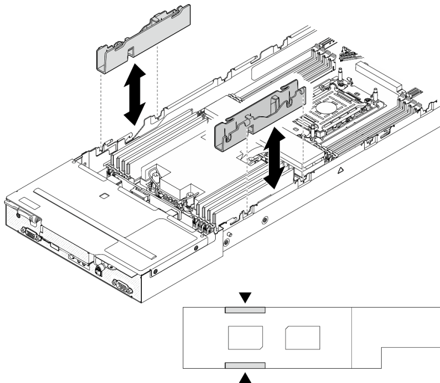
図114. ケーブル・ダクトの交換 (プロセッサ構成1つ)
