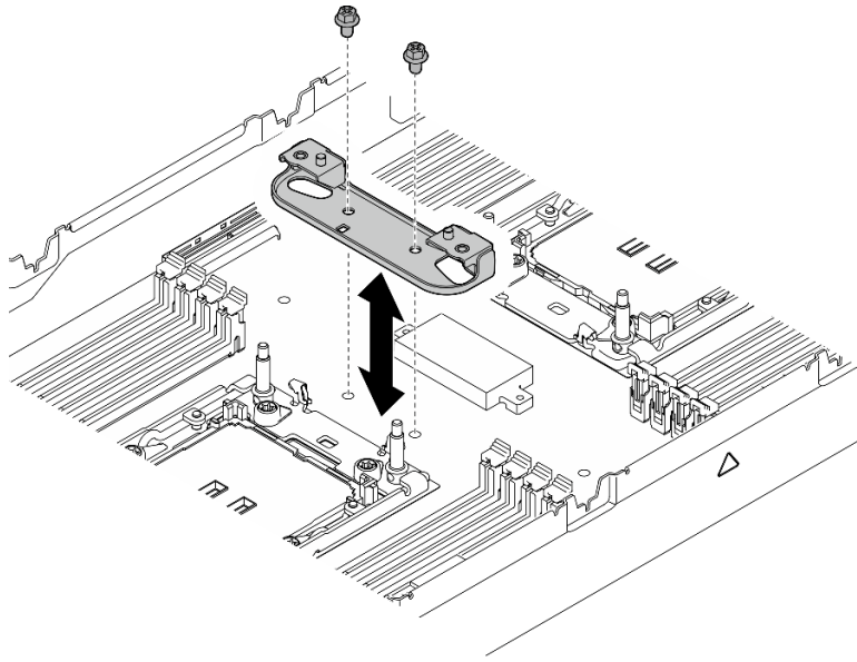
図91. ヒートシンク・サポート・ブラケットの交換
