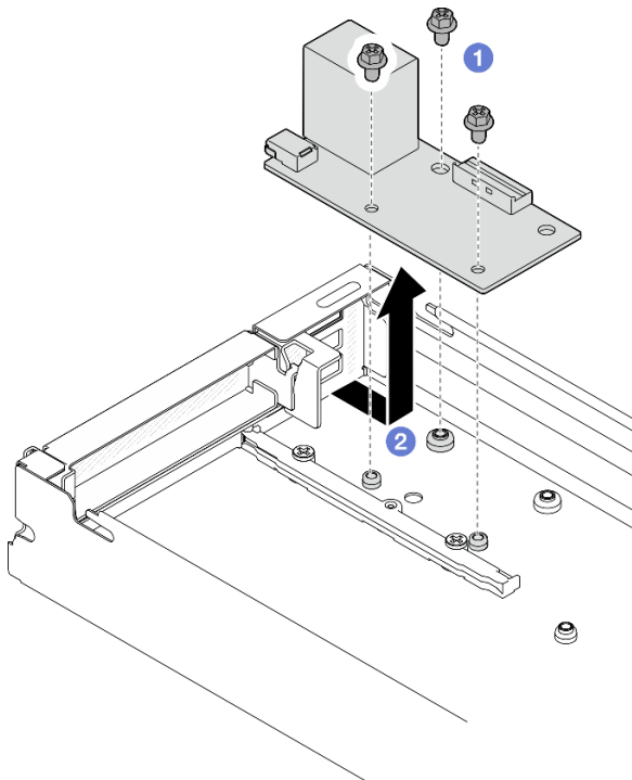
図98. 背面 I/O モジュールの取り外し
