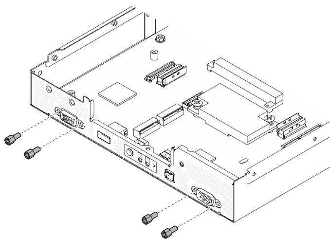
図112. 前面のシステム・ボード上のねじの取り付け
