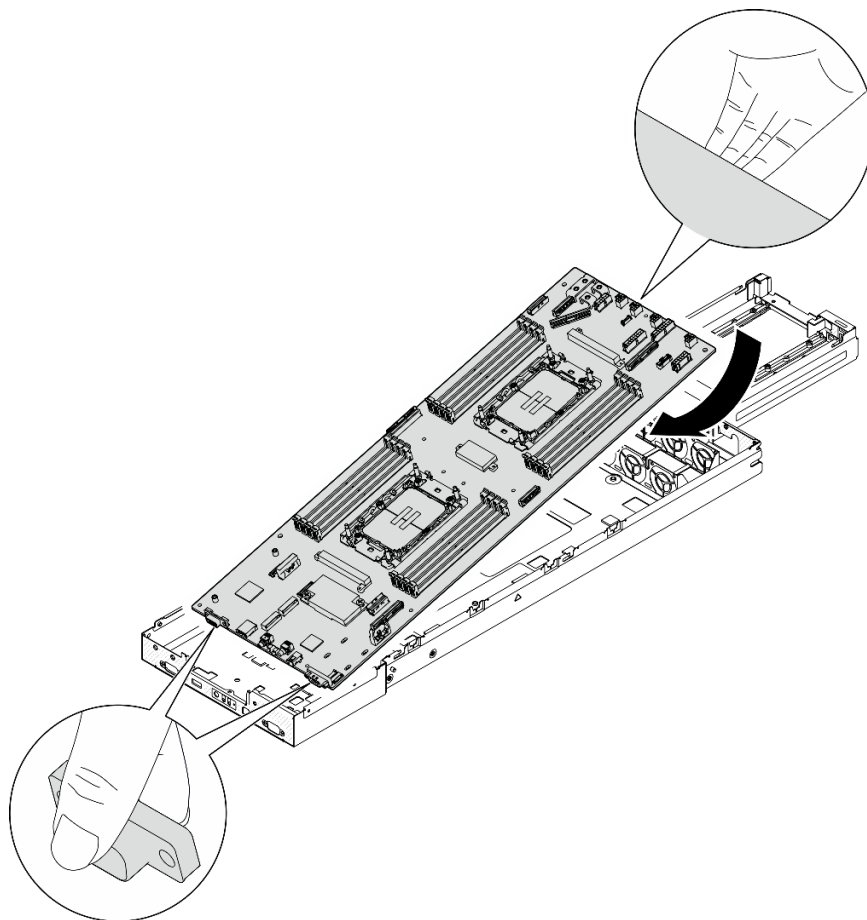
図111. システム・ボードの取り付け
