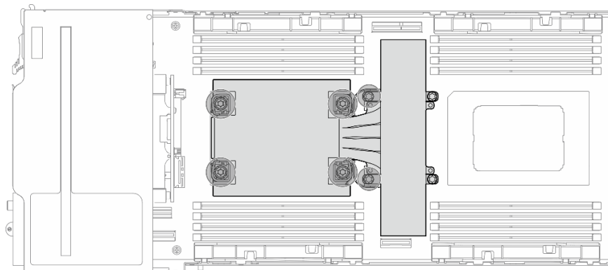
図79. 1 プロセッサ構成のPHMの位置
