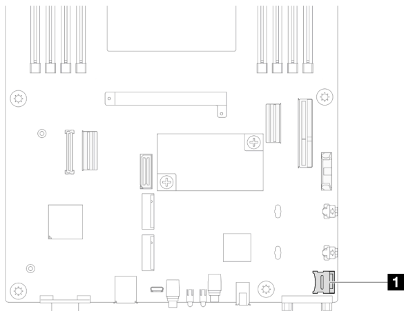
図 61. MicroSD ソケットの位置
