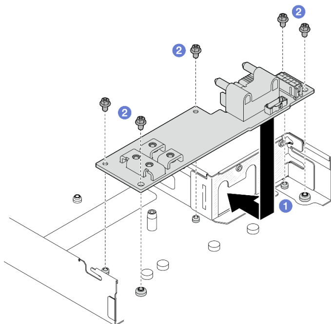
図 77. 分電盤の取り付け
