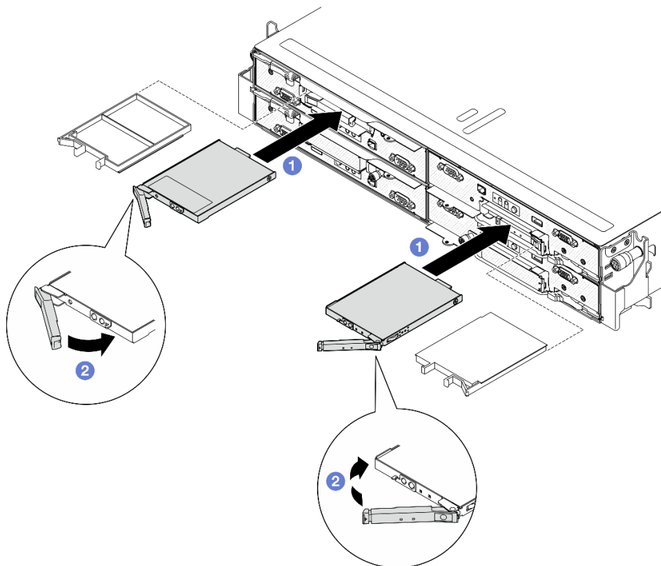
図48. E3.S ホット・スワップ・ドライブの取り付け
