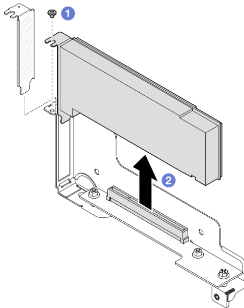
図 67. PCIe アダプターの取り外し
