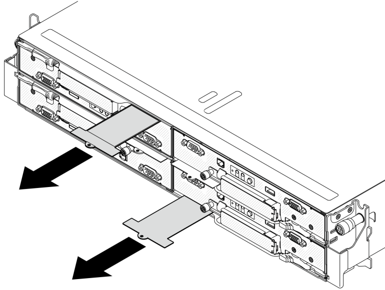
그림 19. 탈착식 정보 탭에 있는 Lenovo XClarity Controller 네트워크 액세스 레이블
