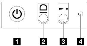
그림 12. 앞면 오퍼레이터 패널 버튼 및 LED
