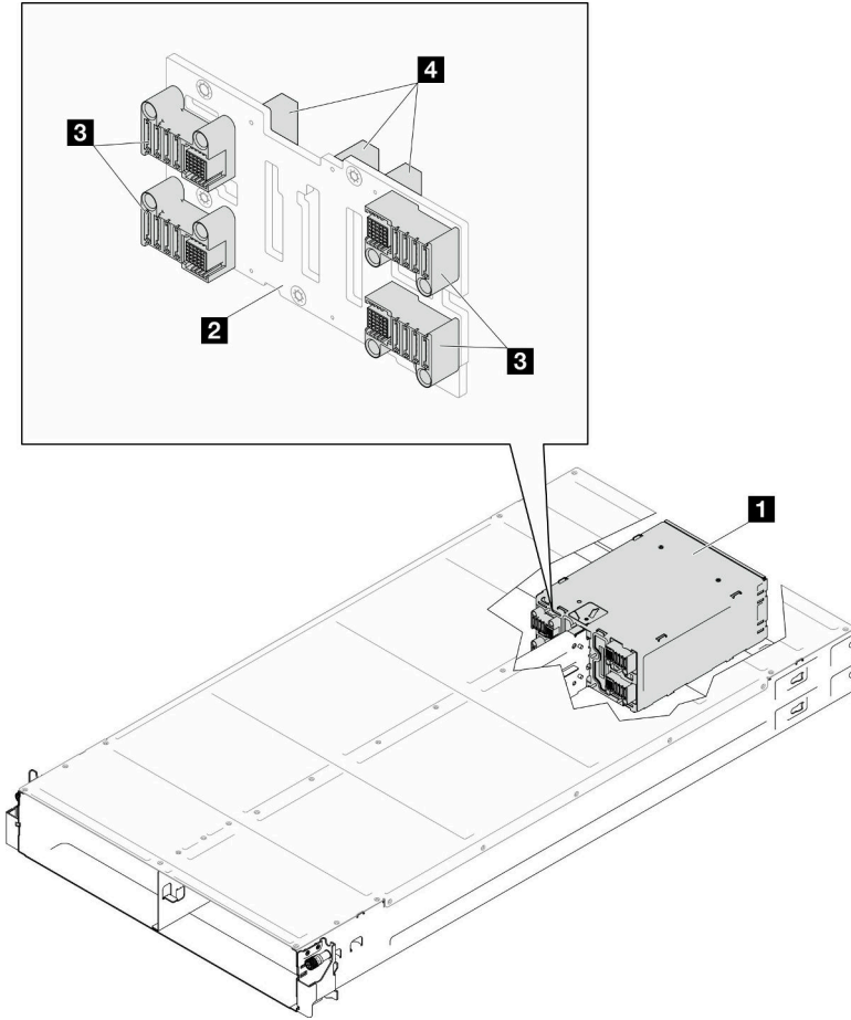
그림 9. D3 새시 미드플레인 위치 및 커넥터
