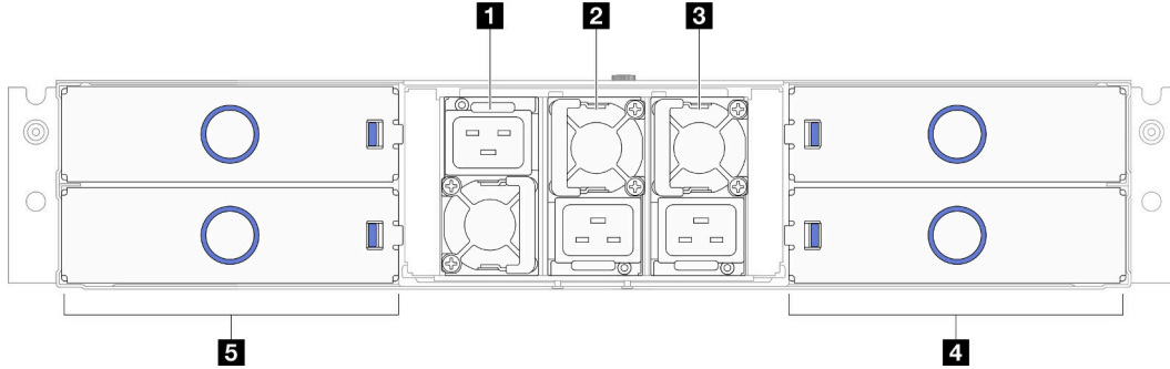
그림 4. 새시 뒷면 보기
