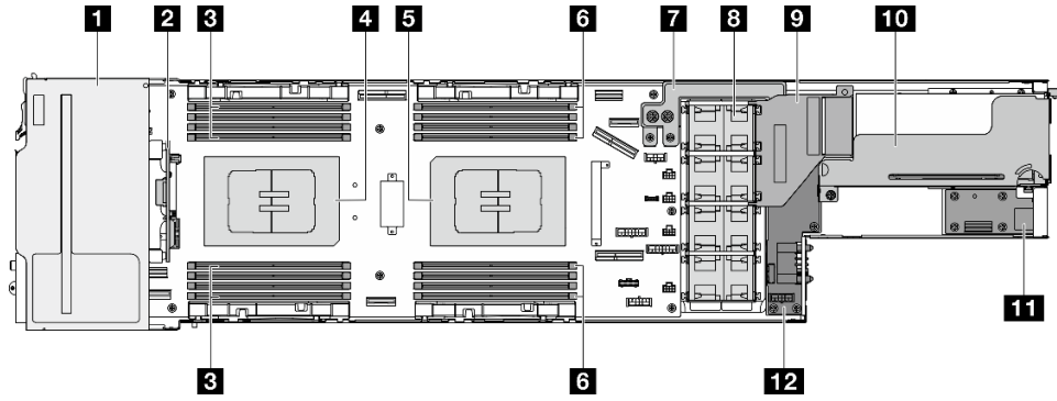
그림 8. SD530 V3의 평면도
