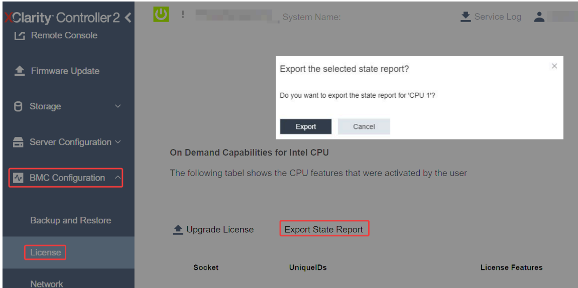
그림 24. XCC 웹 GUI를 통해 상태 보고서 내보내기
