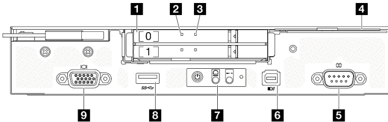
그림 3. ThinkSystem SD530 V3 노드의 앞면 보기
