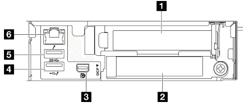
그림 5. 뒷면 보기
