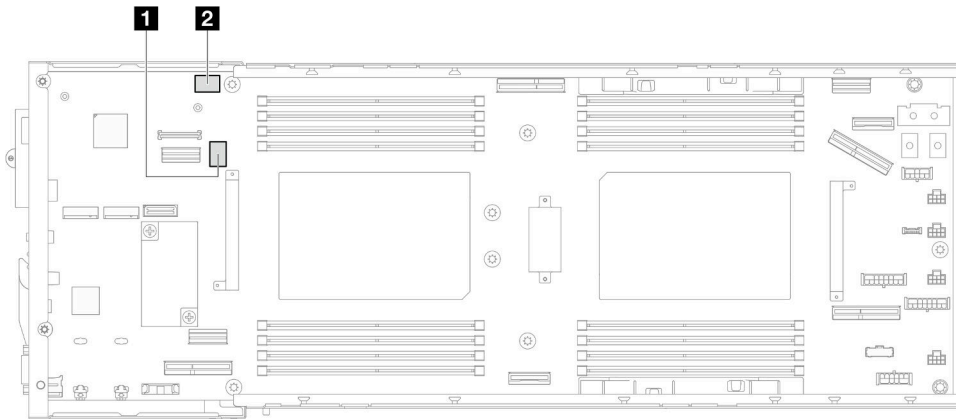
그림 10. 시스템 보드 스위치
