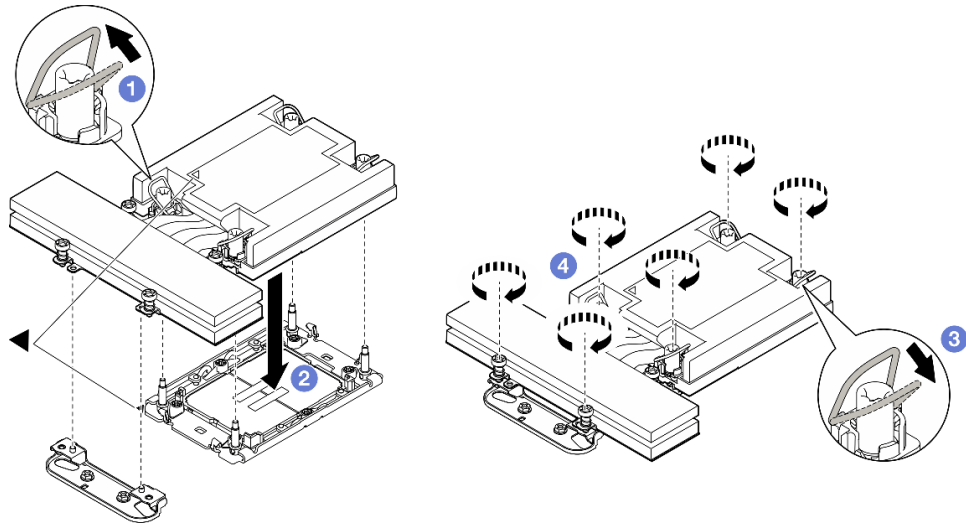
그림 111. 프로세서가 2개인 구성의 1U 성능 PHM 설치
