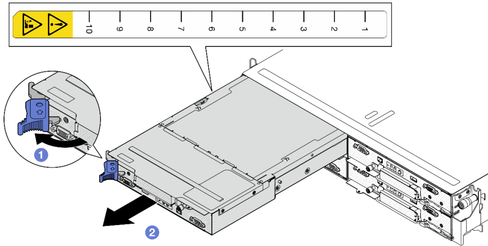
그림 32. 왼쪽 트레이에서 노드 제거
