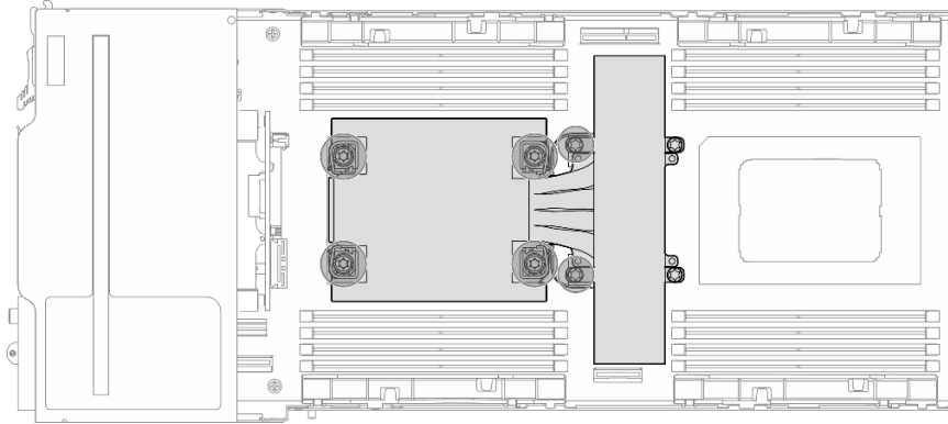
그림 94. 프로세서 1개 구성의 PHM 위치
