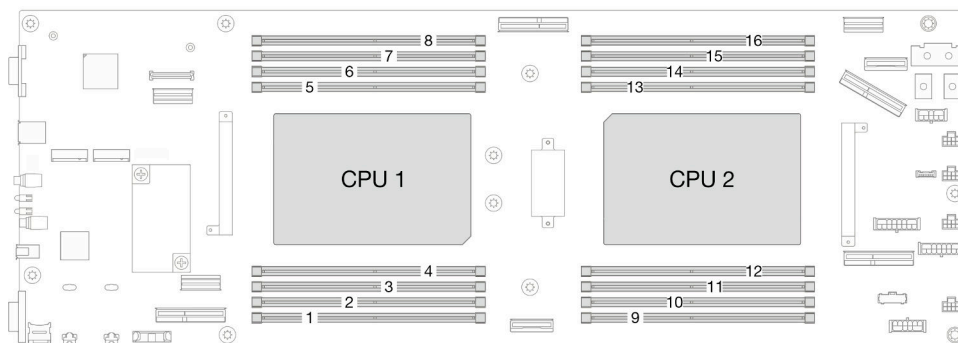
그림 70. 메모리 모듈 및 프로세서 레이아웃
