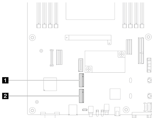
그림 68. 시스템 보드에서 M.2 베이의 위치
