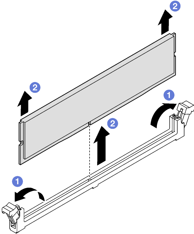
그림 71. 메모리 모듈 제거
