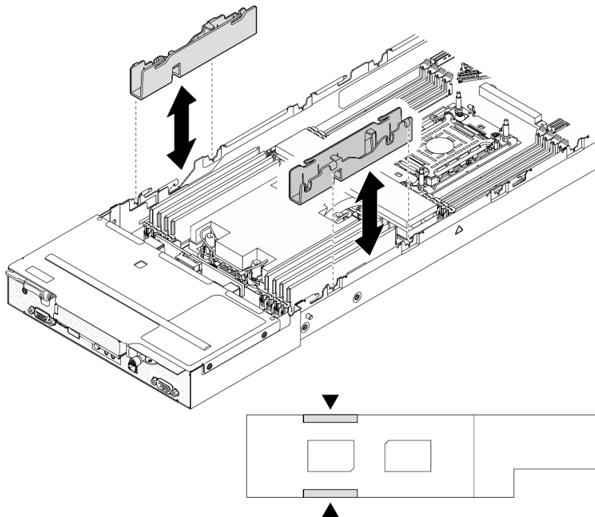
그림 129. 케이블 덕트 교체(프로세서 1개 구성)
