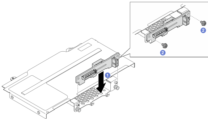
그림 53. 드라이브 백플레인 설치
