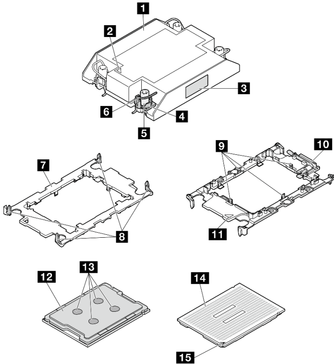
그림 102. PHM 구성 요소
