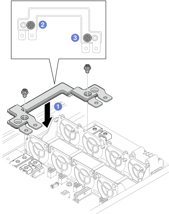
그림 89. 전원 버스 바 설치
