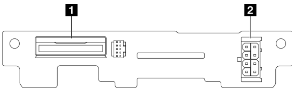
그림 135. E3.S 드라이브 백플레인 커넥터
