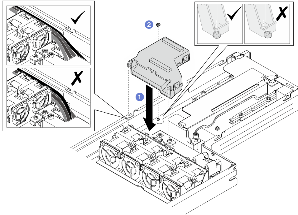
그림 58. GPU 통풍관 설치
