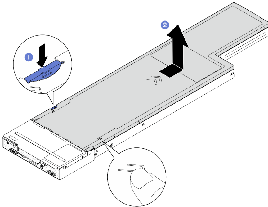
그림 132. 윗면 덮개 제거
