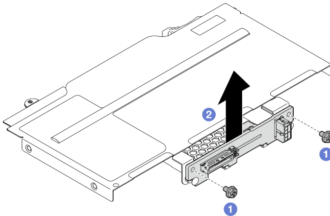
그림 52. 드라이브 백플레인 제거
