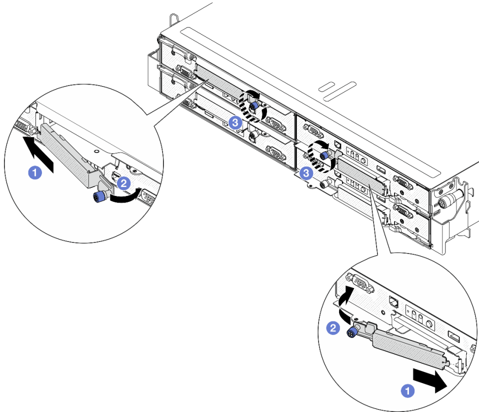
그림 61. E3.S 드라이브 케이지 덮개 설치
