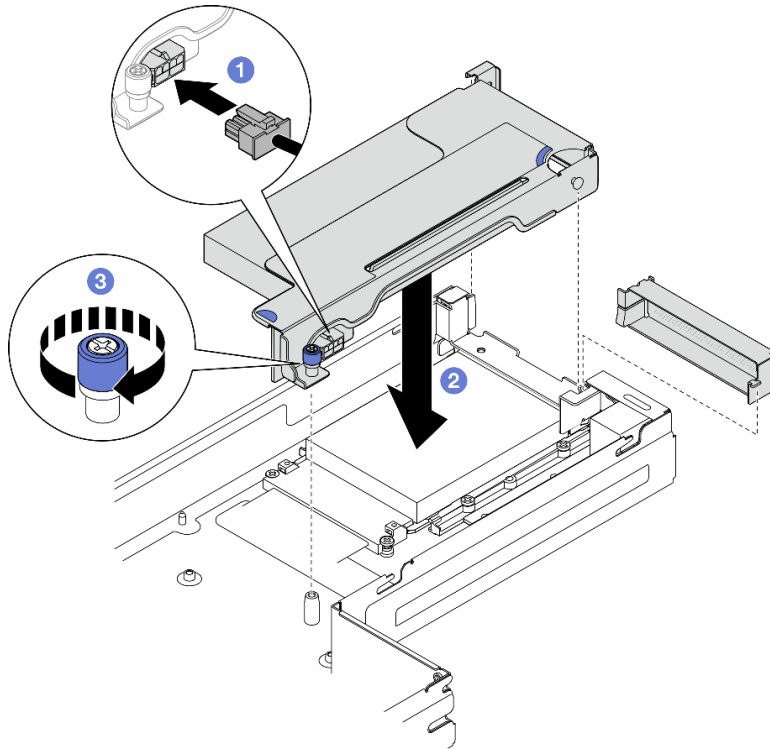
그림 86. PCIe 라이저 어셈블리 설치
