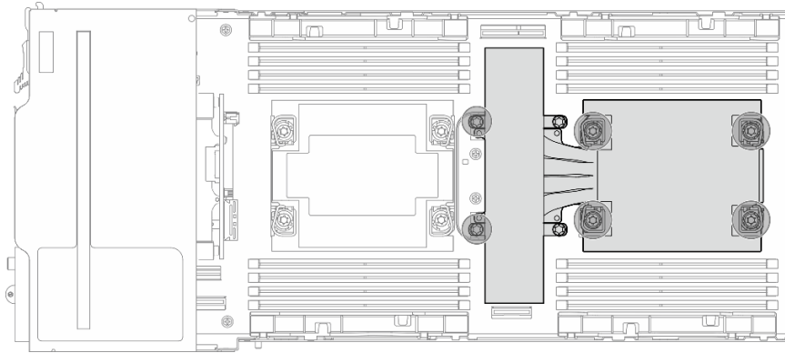
그림 95. 프로세서 2개 구성의 PHM 위치
