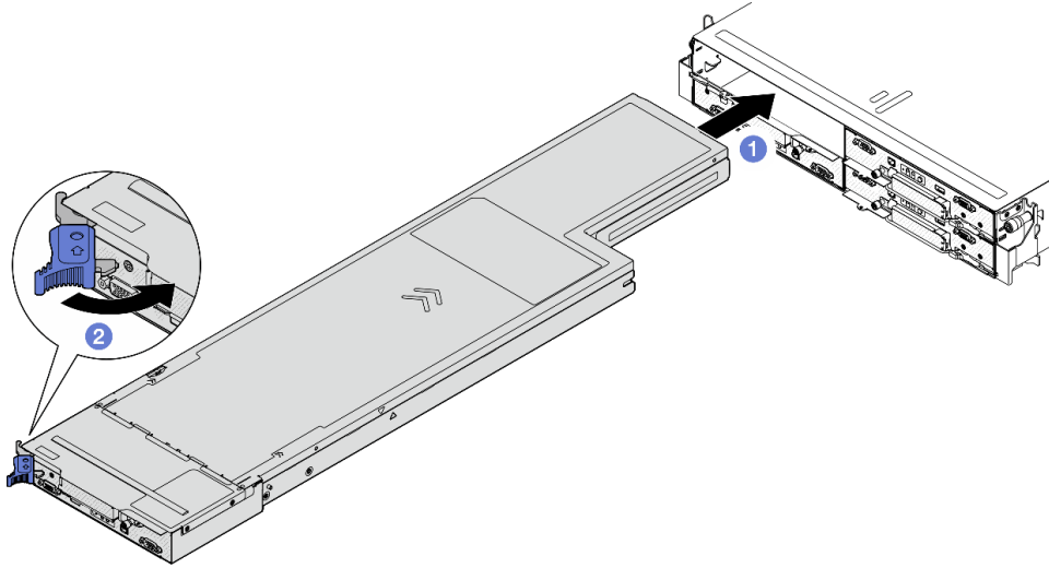
그림 42. 왼쪽 트레이에 노드 설치
