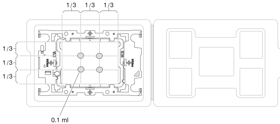
그림 104. 운송 트레이에 프로세서가 있는 열전도 그리스 도포
