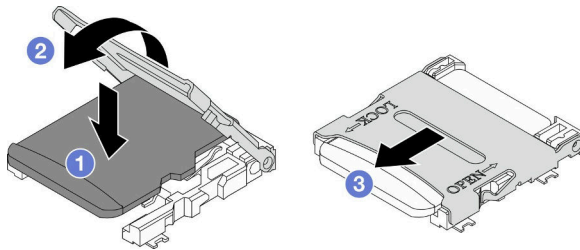
그림 77. MicroSD 카드 설치
