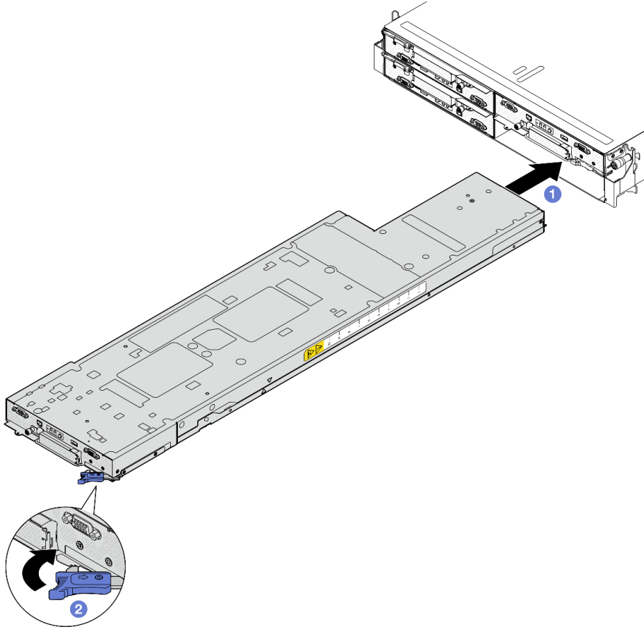
그림 45. 오른쪽 트레이에 노드 설치
