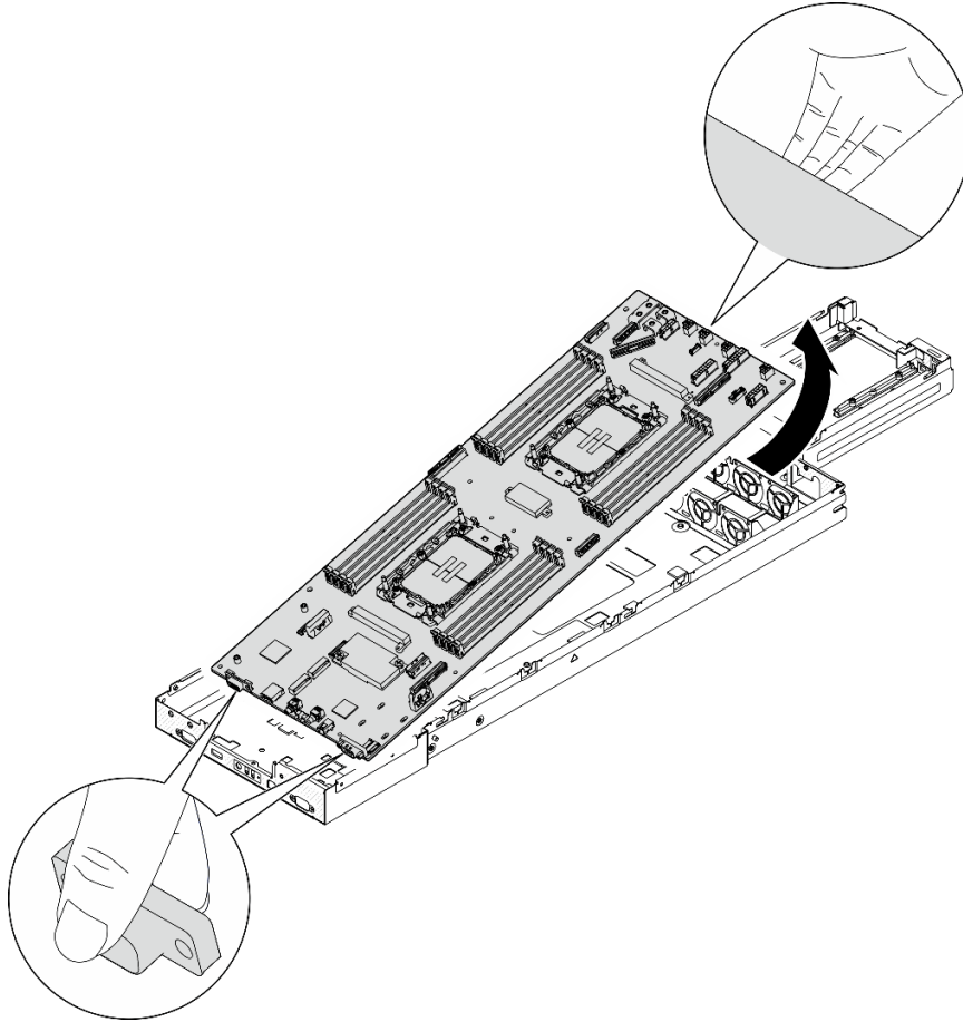
그림 125. 시스템 보드 제거
