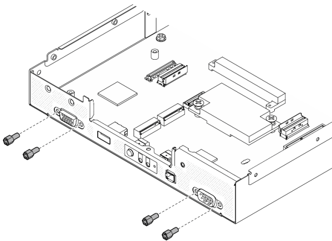
그림 123. 나사 제거
