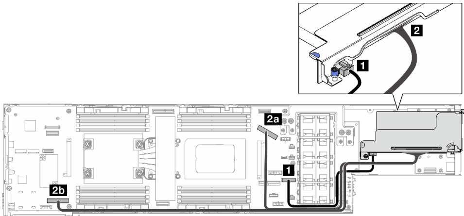
그림 140. PCIe 라이저 케이블 배선 - 프로세서 1개
