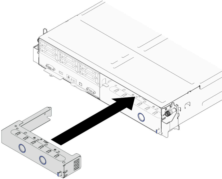
그림 37. 앞면 노드 트레이 필터 설치
