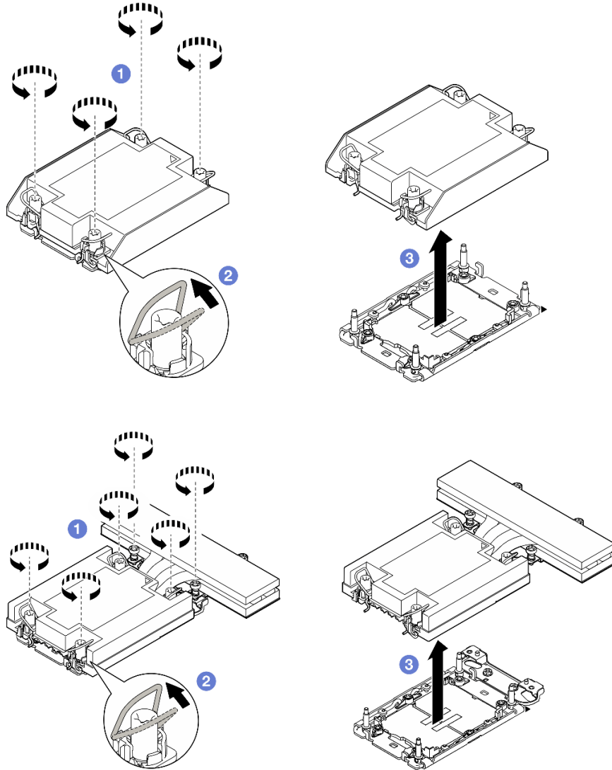
그림 97. 프로세서 1에서 1U 성능 PHM 제거
