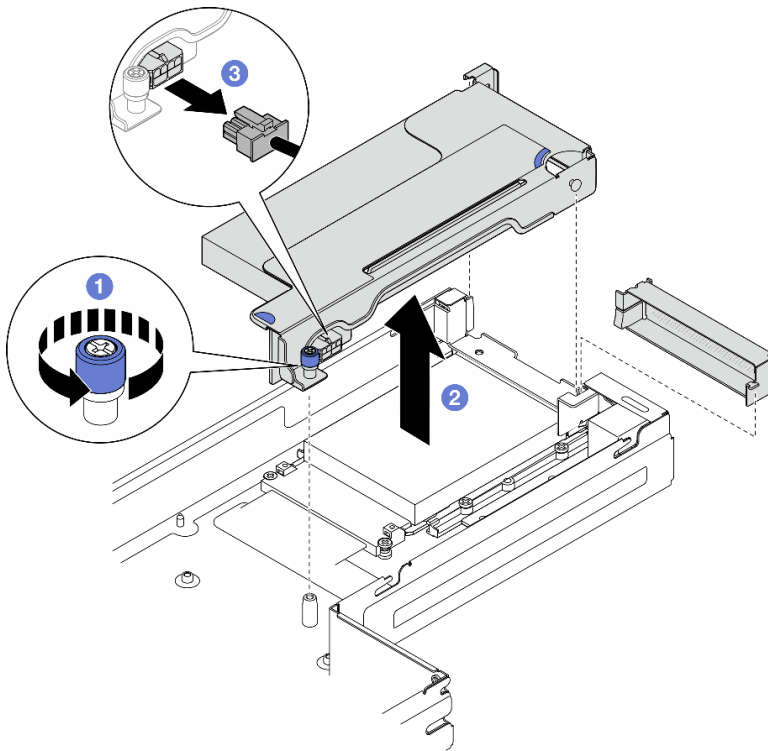
그림 80. PCIe 라이저 어셈블리 제거
