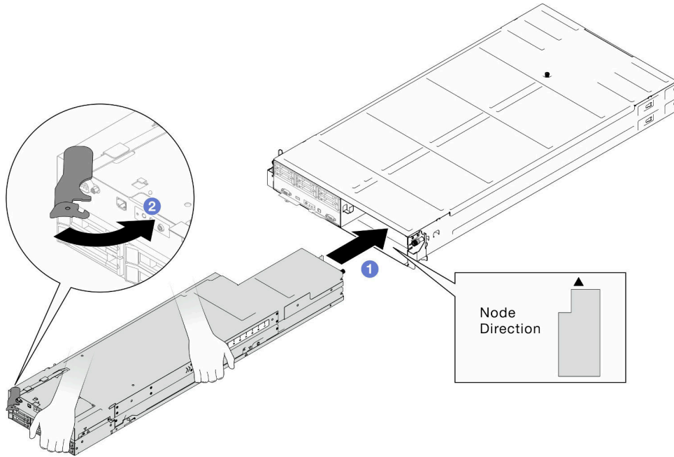
그림 44. 오른쪽 트레이에 노드 설치
