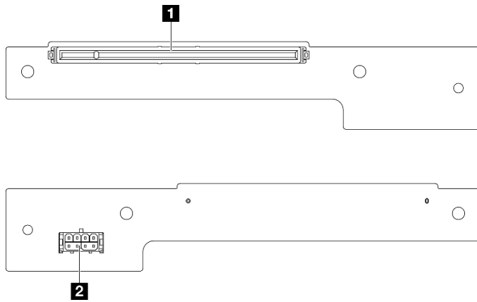
그림 136. PCIe 라이저 카드 커넥터
