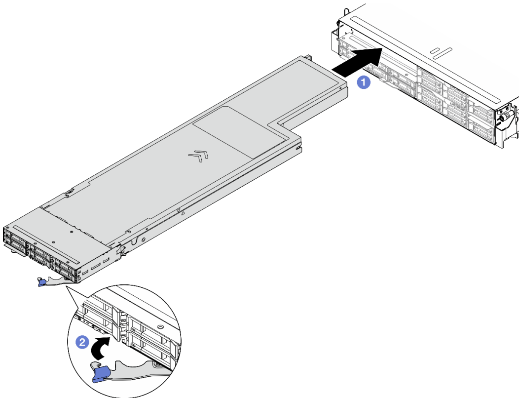
그림 43. 왼쪽 트레이에 노드 설치
