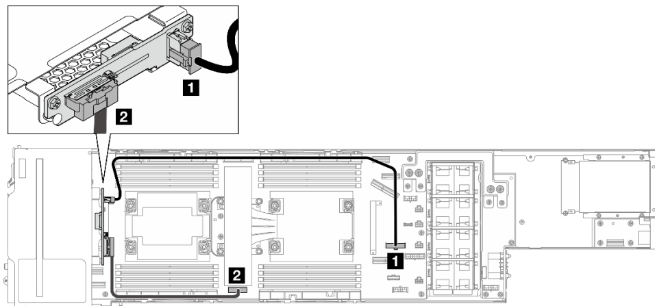
그림 138. E3.S 드라이브 백플레인의 케이블 배선
