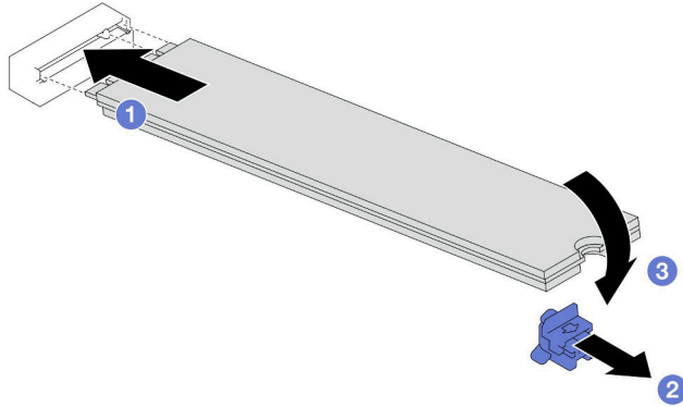
그림 69. M.2 드라이브 설치
