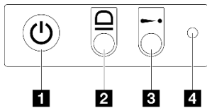
그림 153. 앞면 오퍼레이터 패널 버튼 및 LED
