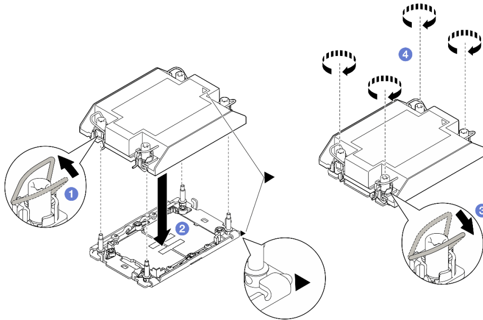
그림 110. 프로세서가 2개인 구성의 1U 표준 PHM 설치
