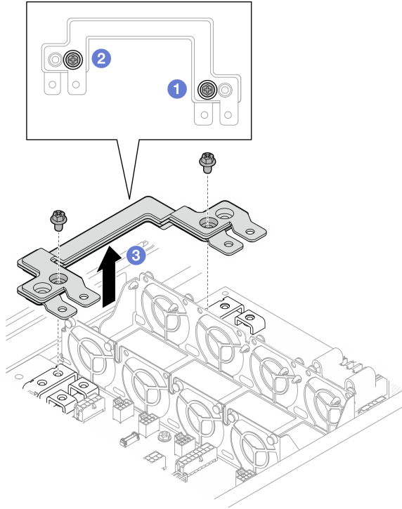
그림 88. 전원 버스 바 제거
