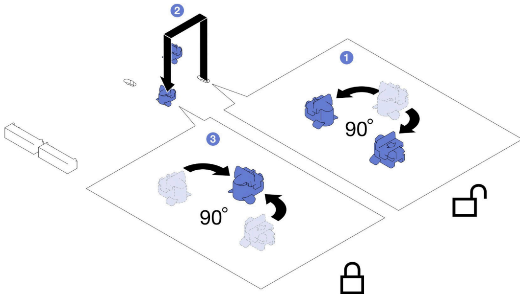
그림 67. M.2 드라이브 고정장치 조정
