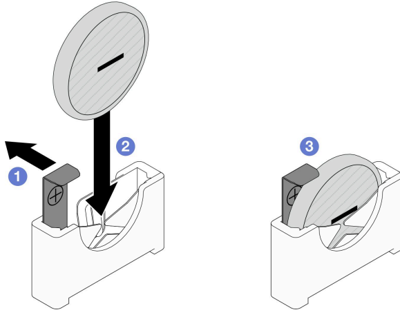
그림 50. CMOS 배터리 설치
