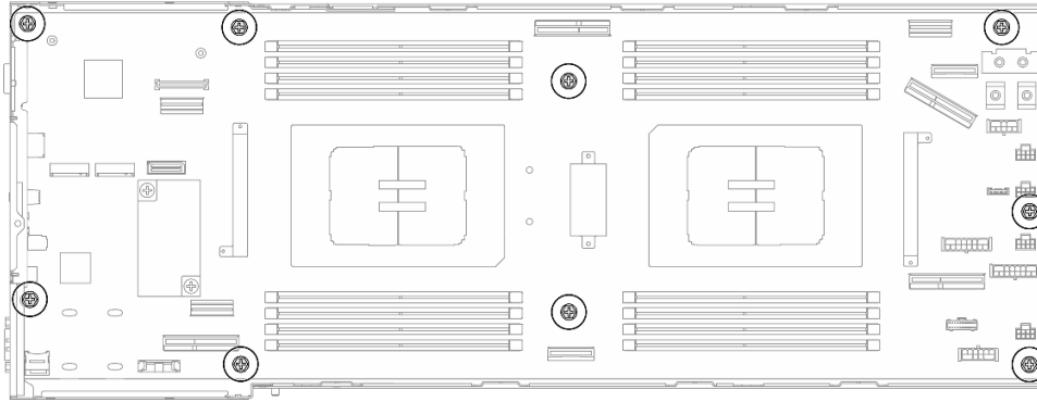
그림 124. 나사 제거
