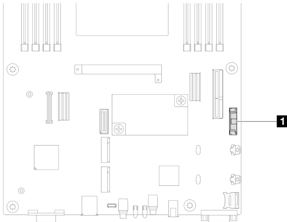
그림 49. CMOS 배터리 소켓의 위치
