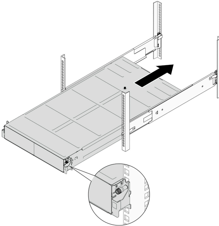
그림 19. 새시 설치
