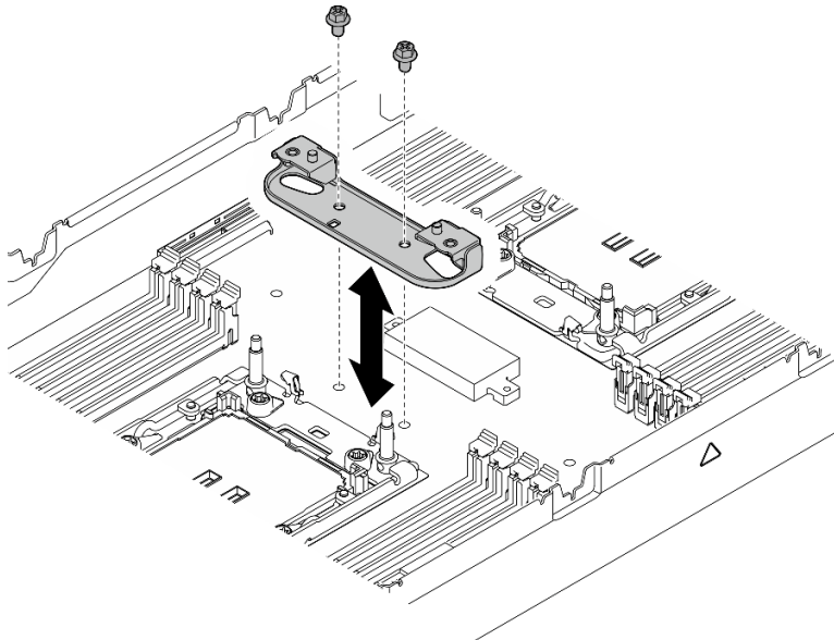
그림 120. 방열판 지지 브래킷 교체
