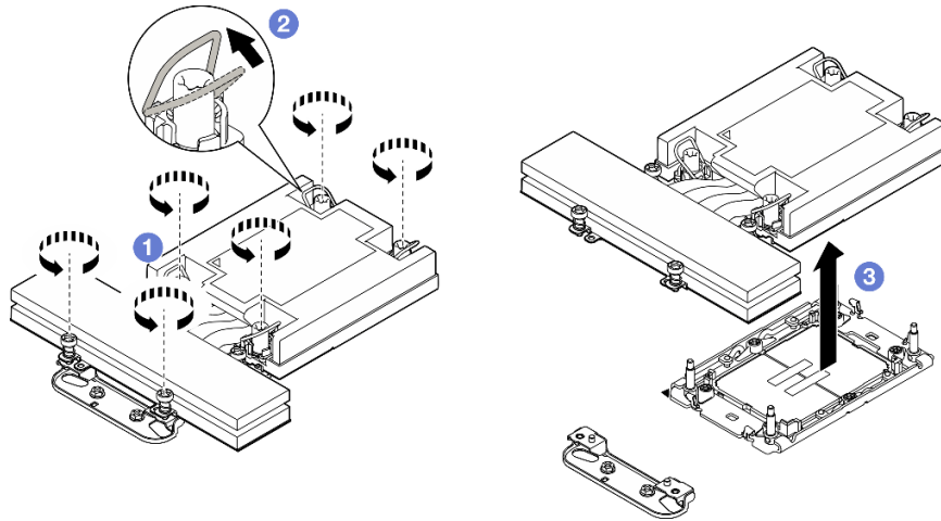
그림 98. 프로세서 2에서 1U 성능 PHM 제거
