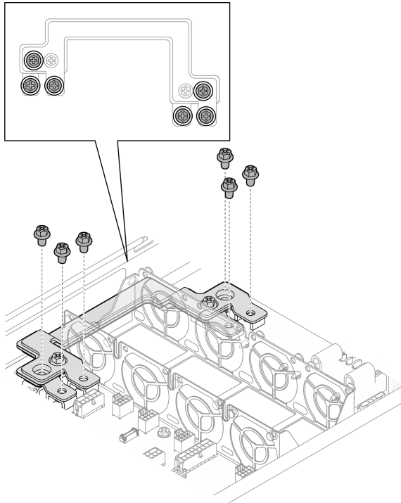
그림 87. 전원 버스 바의 외부 나사 제거
