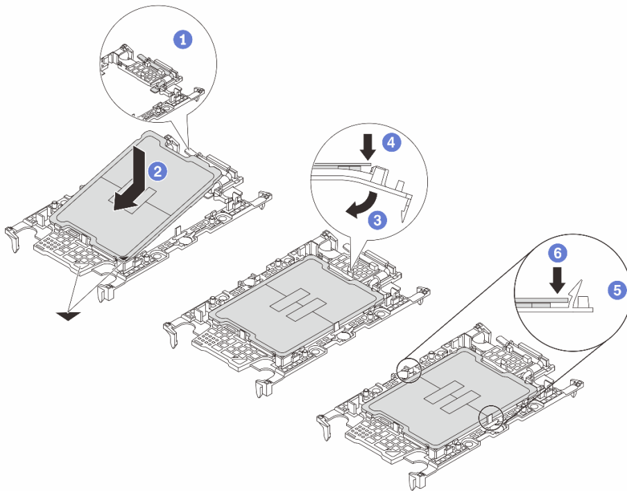
그림 103. 프로세서 캐리어 설치
