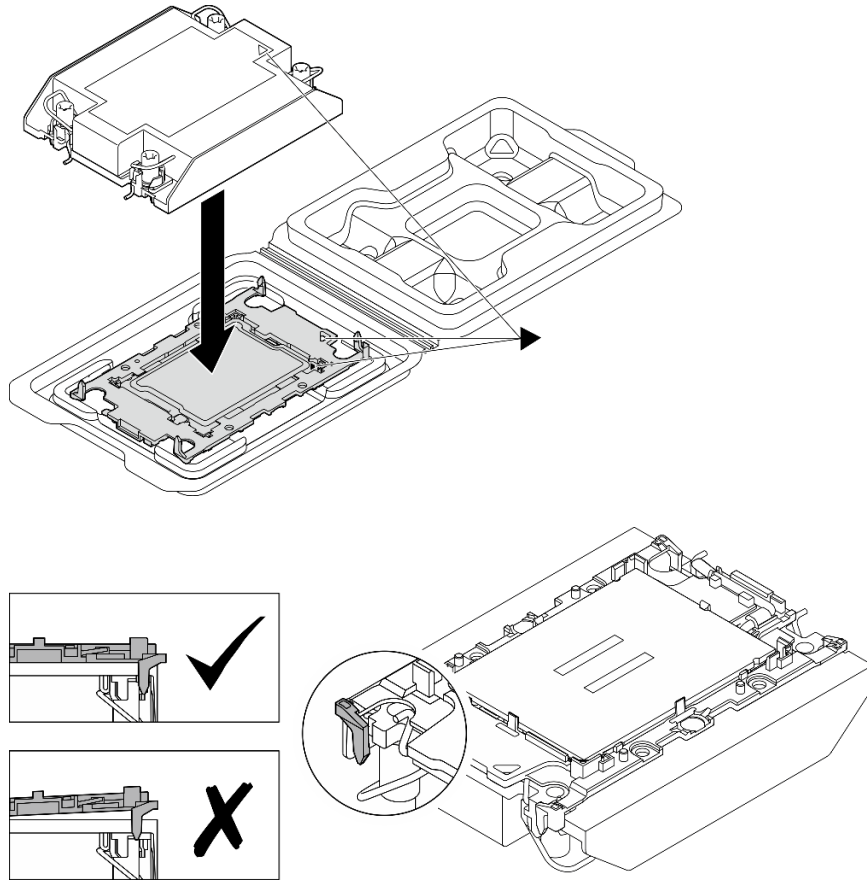
그림 105. 운송 트레이 내 프로세서로 PHM 조립
