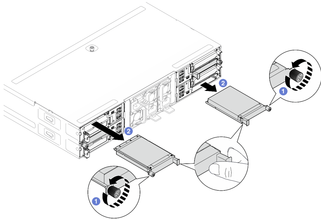
그림 78. 뒷면 OCP 모듈 제거
