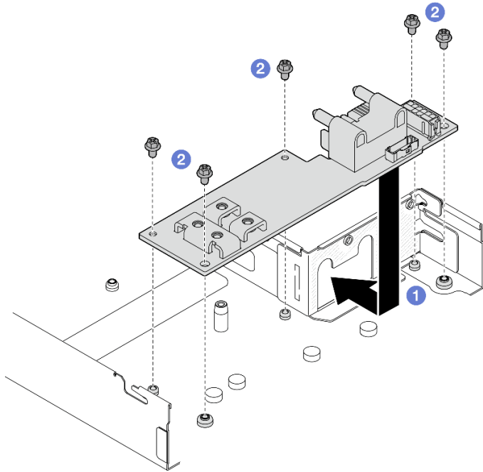
그림 92. 전원 분배 보드 설치
