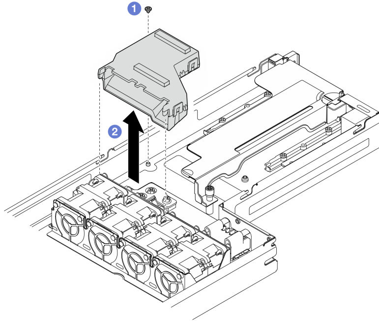
그림 57. GPU 통풍관 제거
