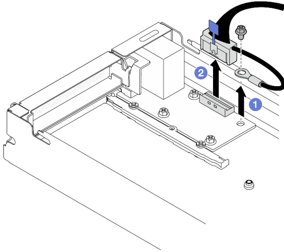
그림 112. 뒷면 I/O 케이블 및 접지 케이블 제거
