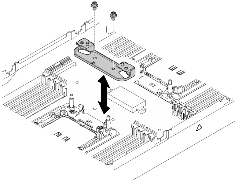
그림 106. 방열판 지지 브래킷 교체
