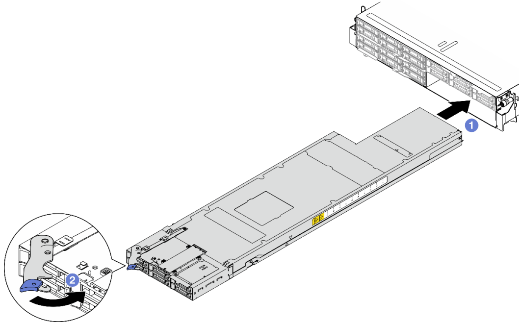
그림 46. 오른쪽 트레이에 노드 설치
