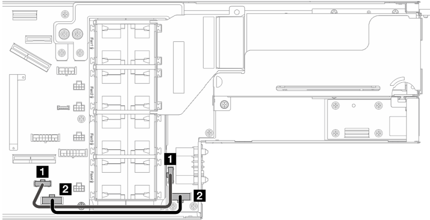
그림 142. 전원 분배 보드의 케이블 배선
