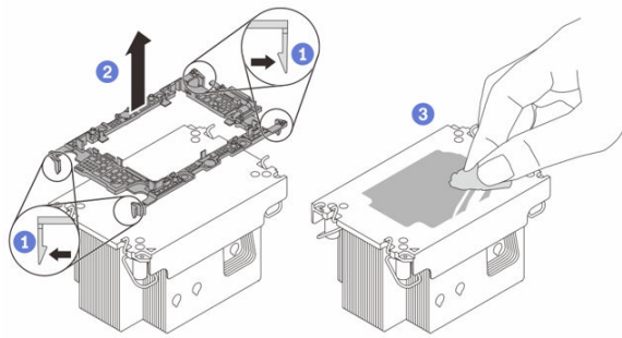
그림 101. 방열판에서 프로세서 캐리어 분리 중
