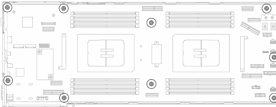
그림 128. 시스템 보드에 나사 설치
