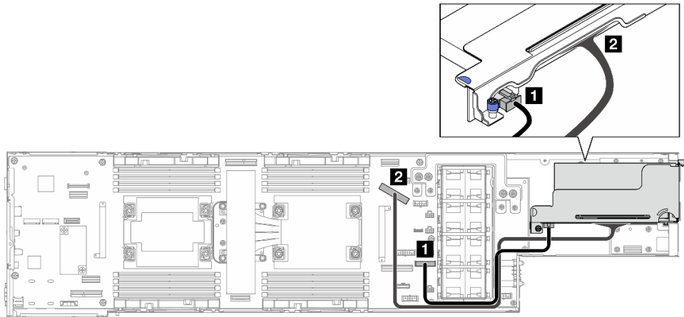
그림 141. PCIe 라이저 케이블 배선 - 프로세서 2개
