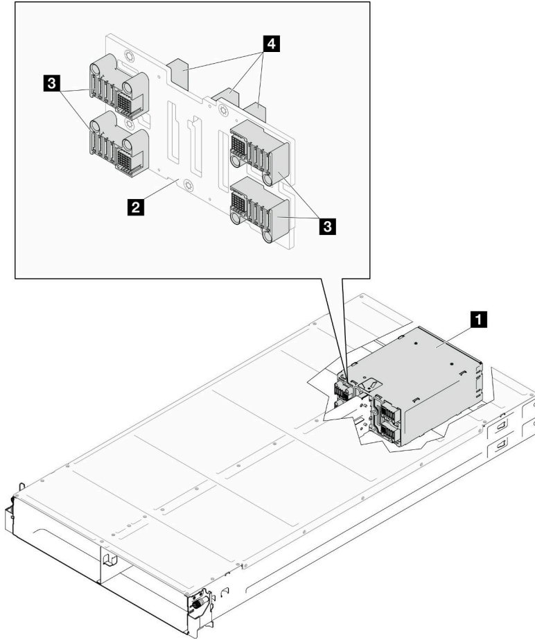
그림 9. D3 새시 미드플레인 위치 및 커넥터
