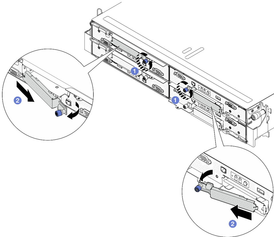
그림 62. E3.S 드라이브 케이지 덮개 제거
