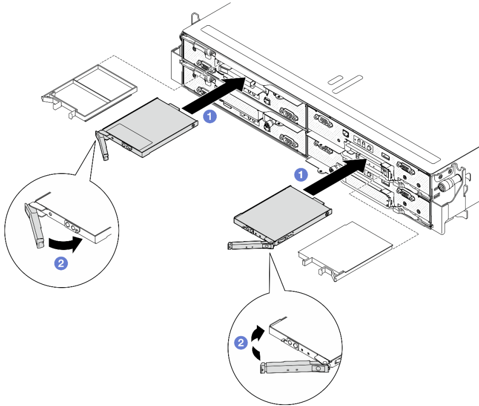
그림 63. E3.S 핫 스왑 드라이브 설치
