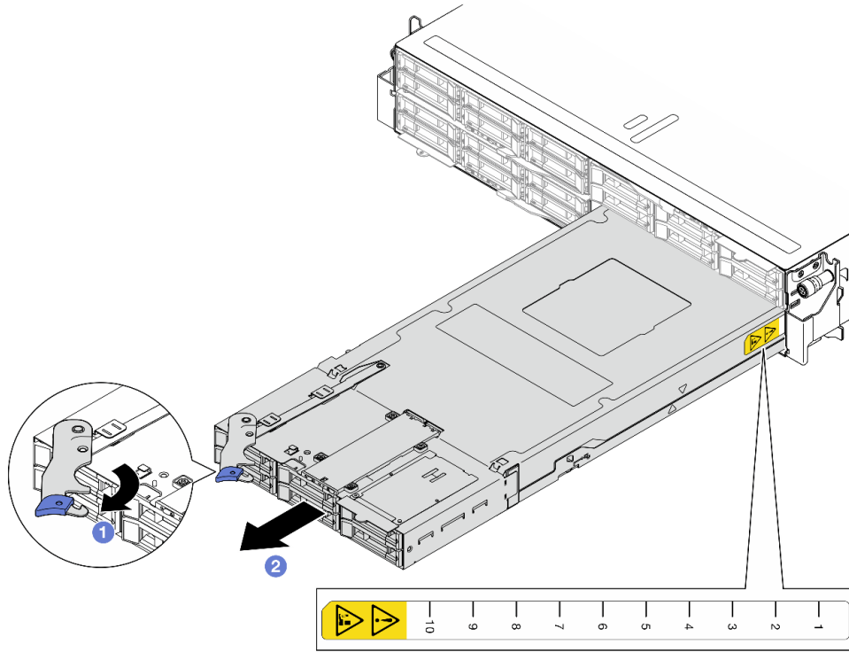
그림 36. 오른쪽 트레이에서 노드 제거
