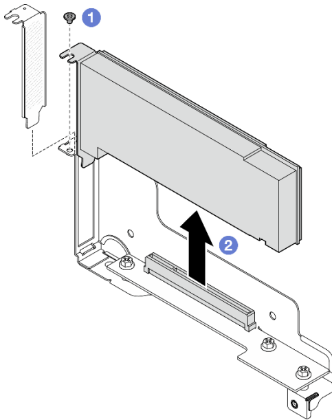
그림 82. PCIe 어댑터 제거
