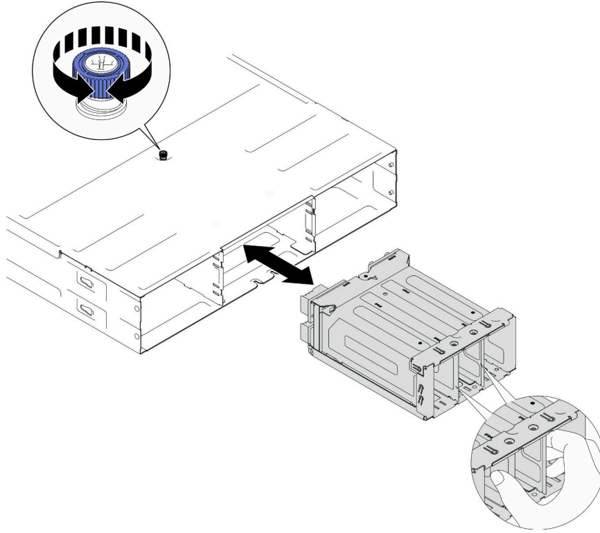
그림 30. PSU 케이스 설치
