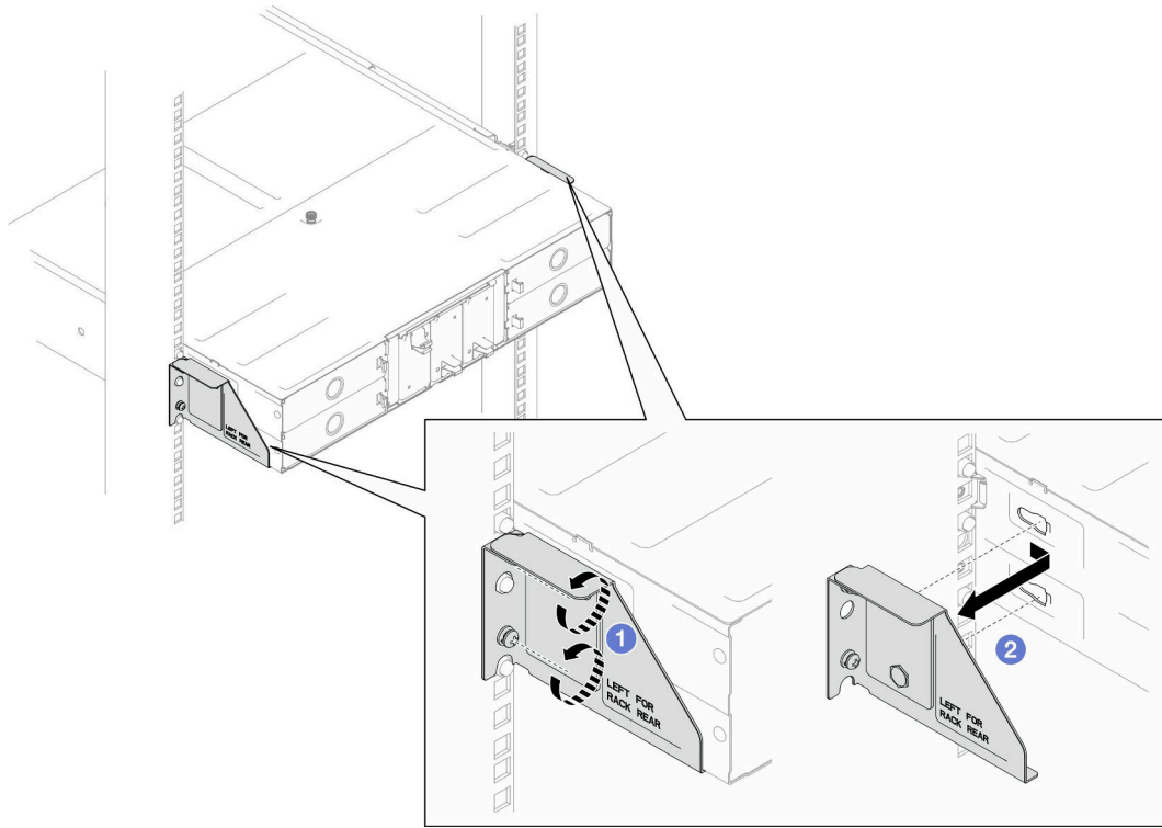
그림 17. 운반 브래킷 제거
