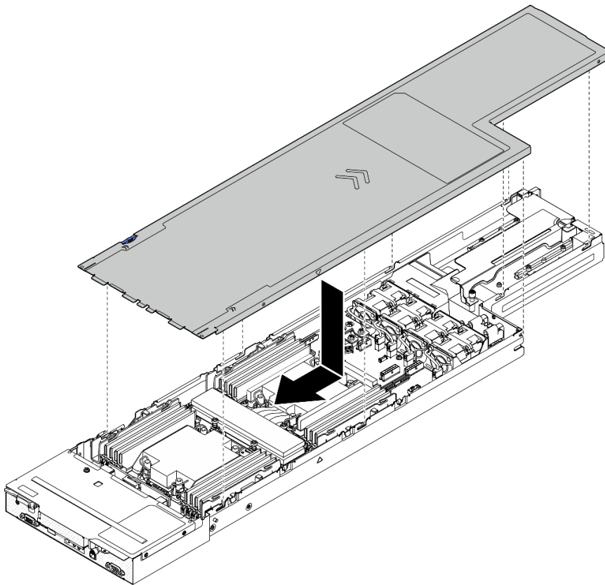
그림 133. 윗면 덮개 설치
