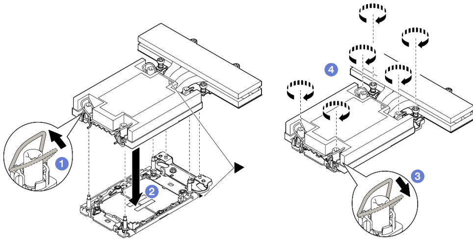
그림 108. 프로세서가 1개인 구성의 1U 성능 PHM 설치
