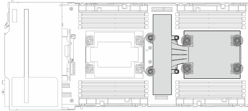
그림 109. 프로세서 2개 구성의 PHM 위치
