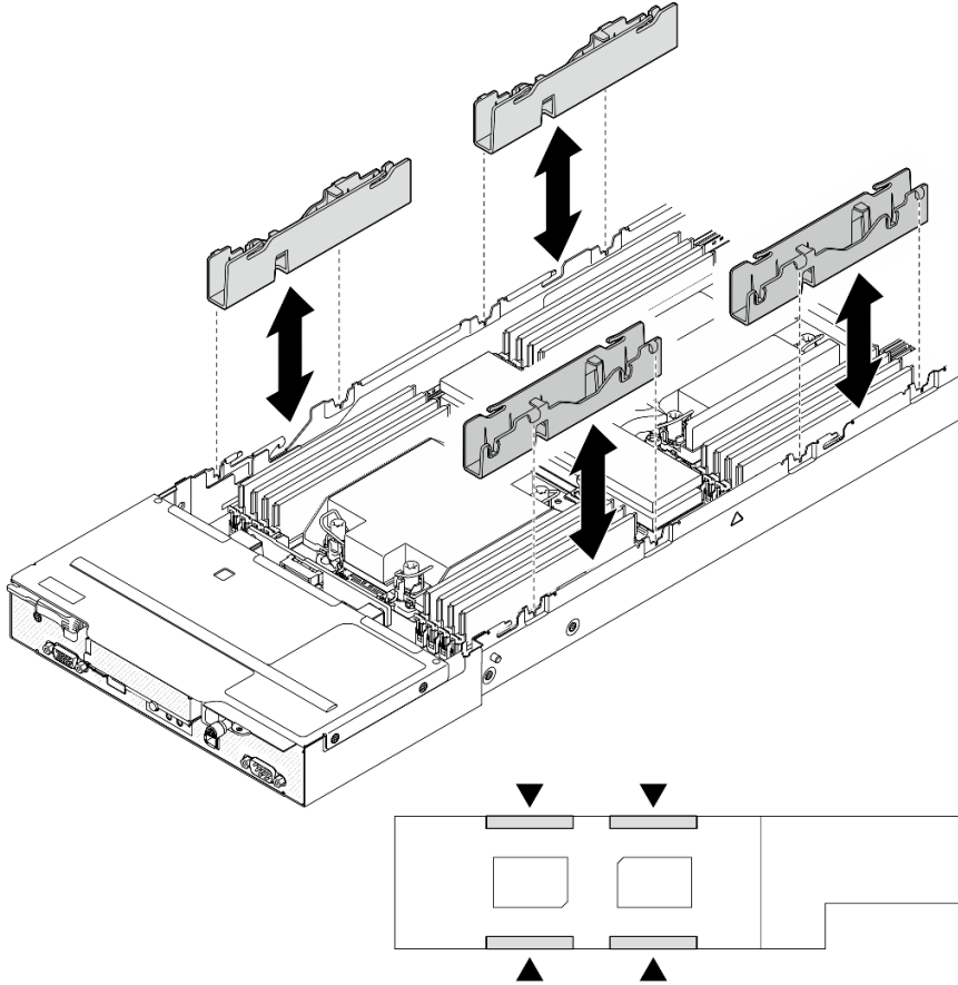
그림 122. 케이블 덕트 교체(프로세서 2개 구성)
