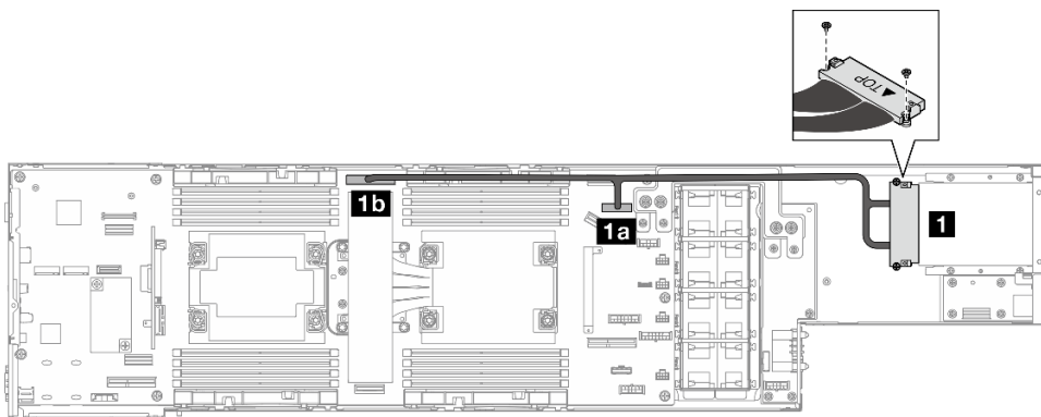
그림 143. 뒷면 I/O 모듈 및 OCP 모듈의 케이블
