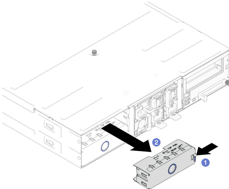
그림 40. 뒷면 노드 트레이 필터 제거
