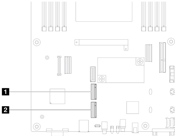
그림 65. 시스템 보드에서 M.2 베이의 위치
