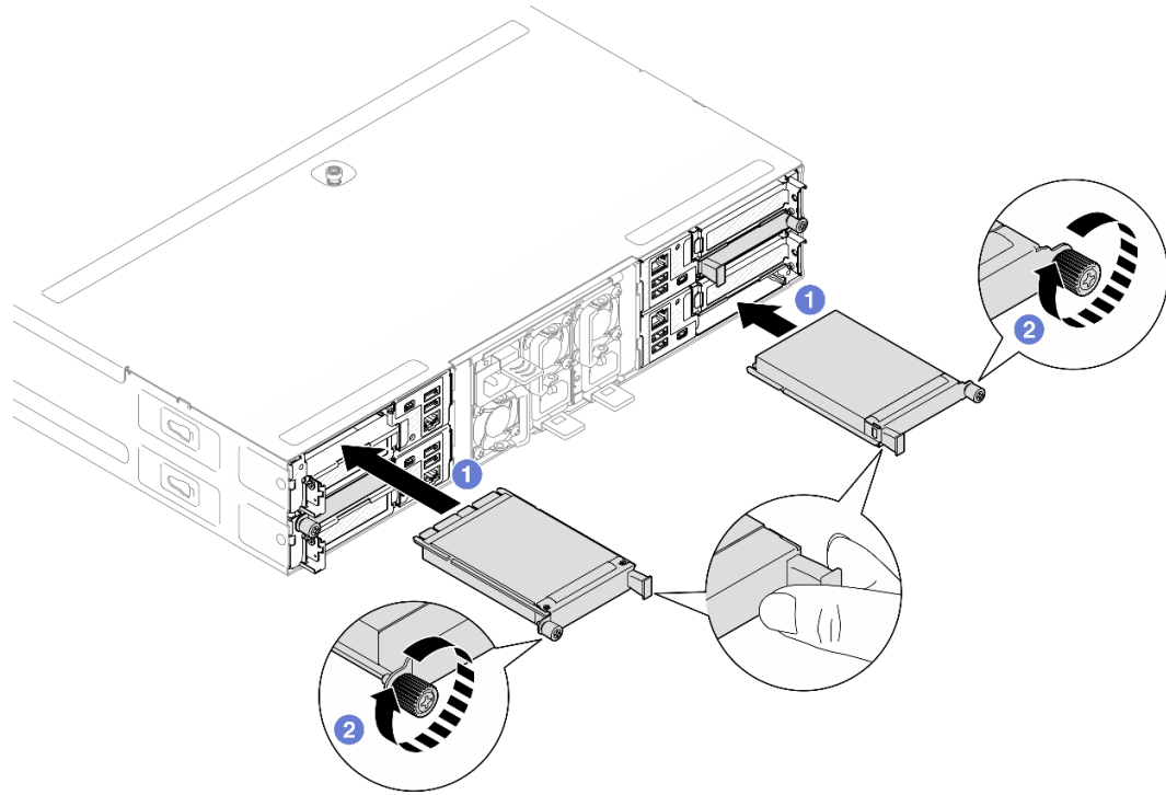
그림 79. 뒷면 OCP 모듈 설치
