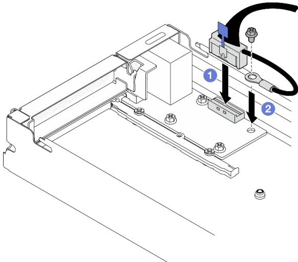
그림 144. 뒷면 I/O 케이블 및 접지 케이블 설치
