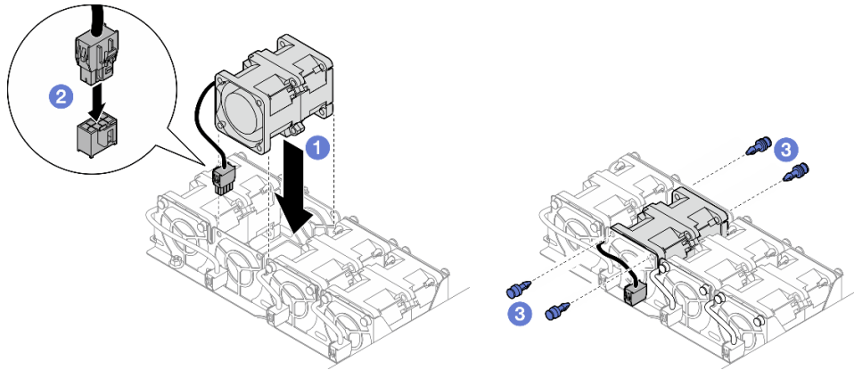
그림 56. 팬 설치
