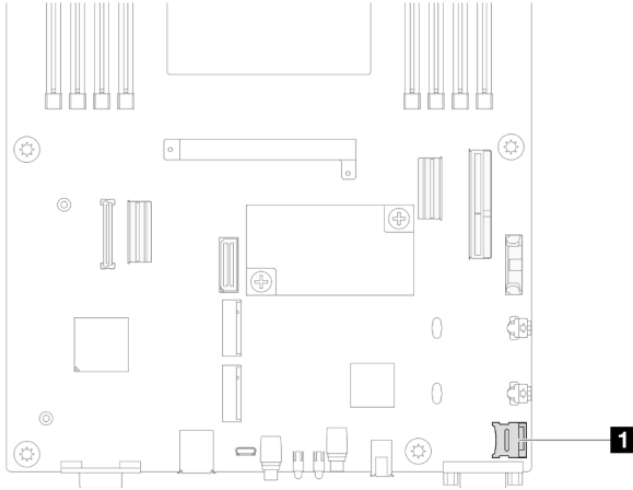
그림 76. MicroSD 소켓의 위치
