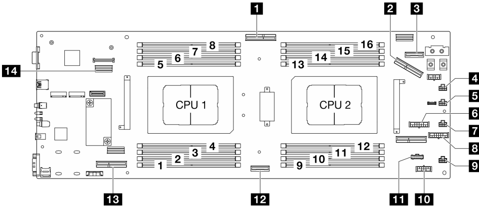
그림 134. 케이블 배선용 시스템 보드 커넥터
