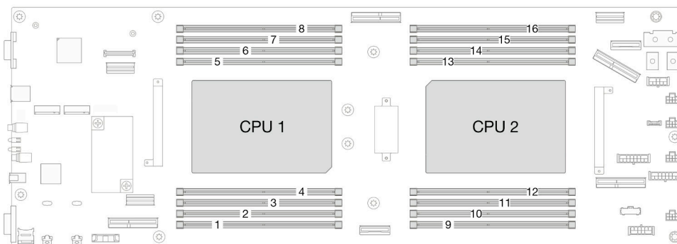
그림 72. 메모리 모듈 및 프로세서 레이아웃
