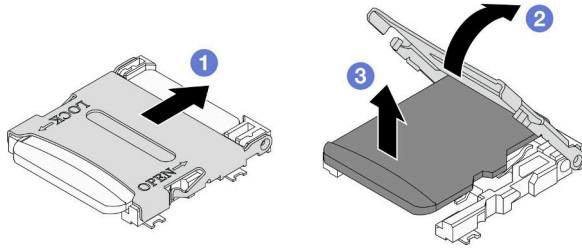
그림 75. MicroSD 카드 제거
