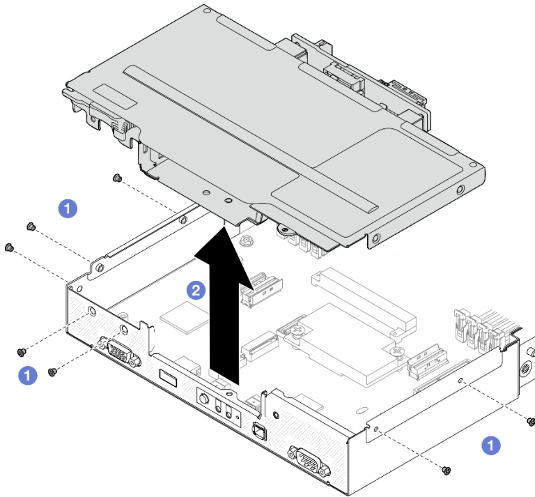
그림 51. 드라이브 케이징 어셈블리 제거
