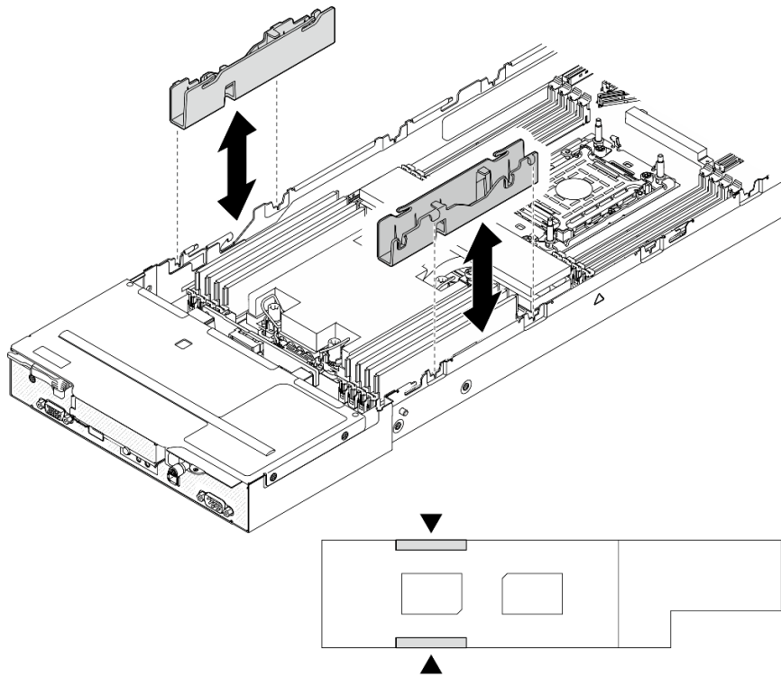
그림 121. 케이블 덕트 교체(프로세서 1개 구성)
