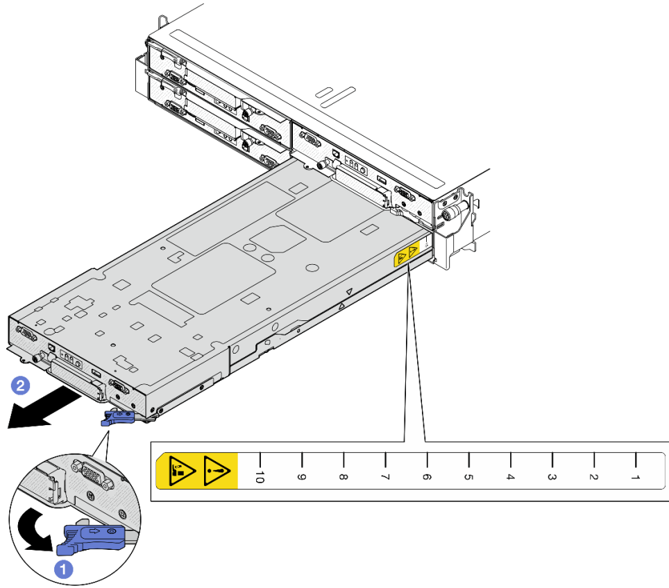
그림 35. 오른쪽 트레이에서 노드 제거
