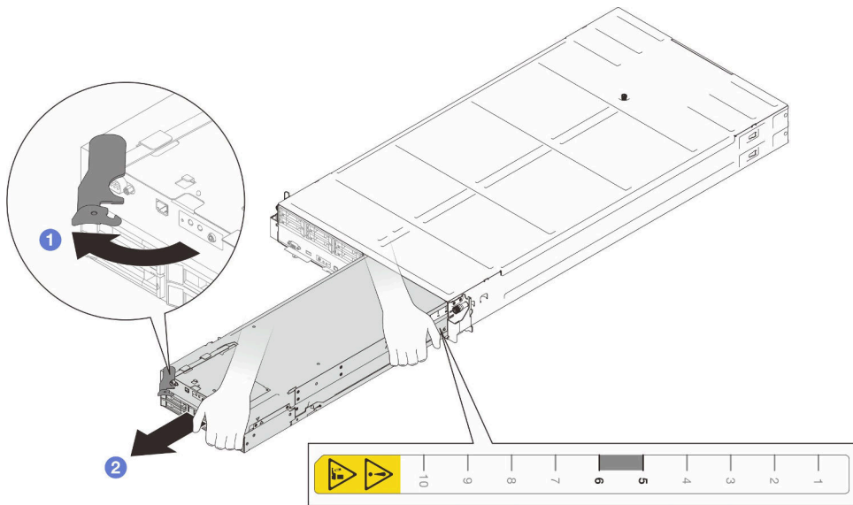
그림 34. 오른쪽 트레이에서 노드 제거
