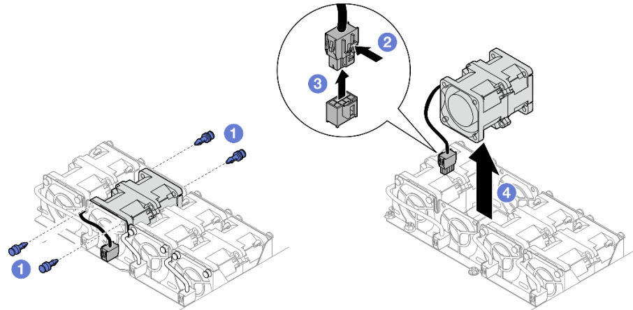
그림 55. 팬 제거
