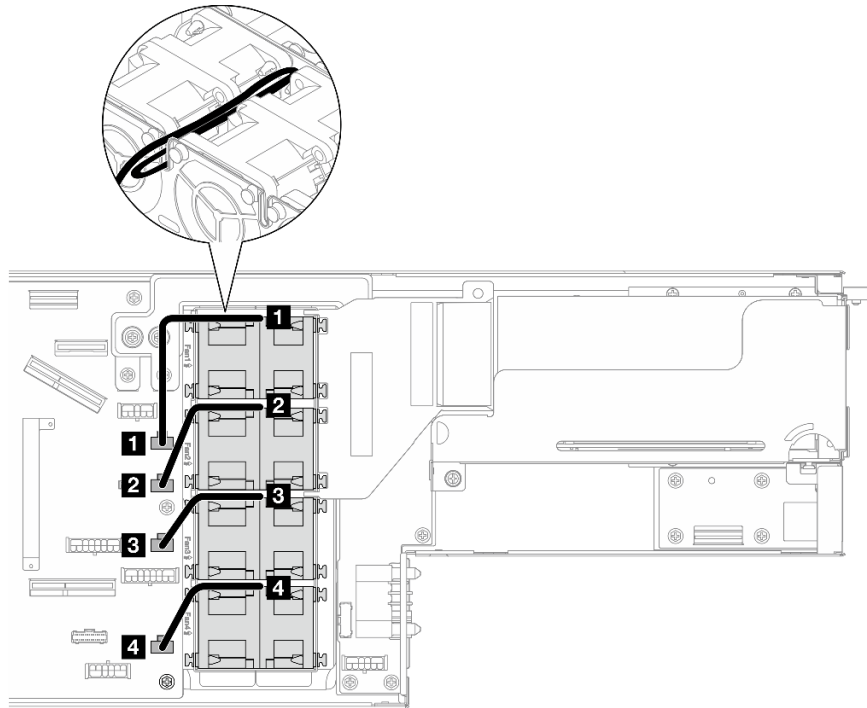
그림 139. 팬 케이블 배선
