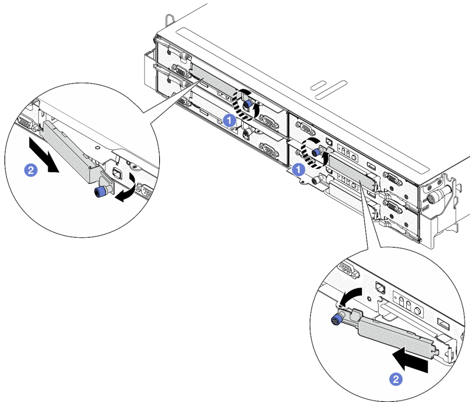
그림 59. E3.S 드라이브 케이징 덮개 제거
