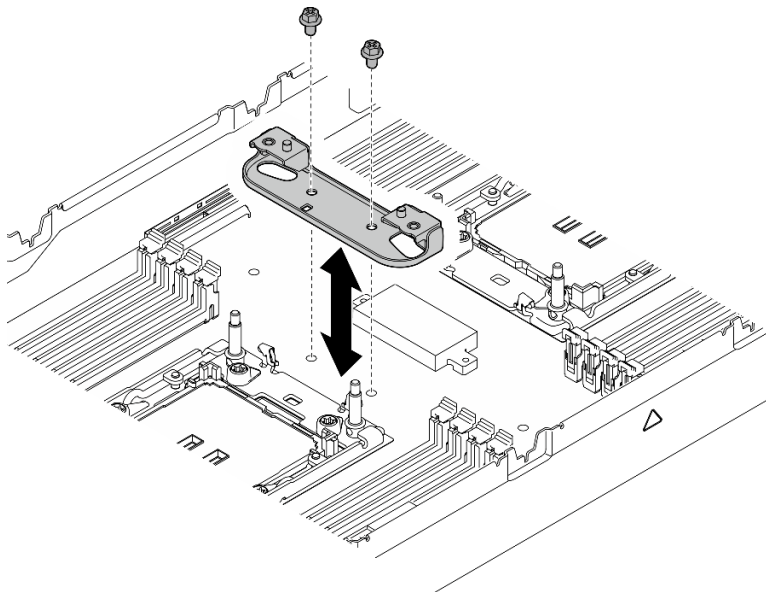
그림 99. 방열판 지지 브래킷 교체
