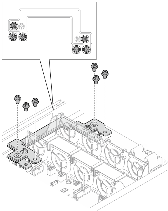
그림 90. 전원 버스 바 외부 나사 설치
