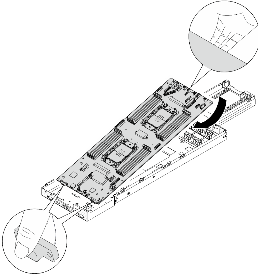
그림 126. 시스템 보드 설치
