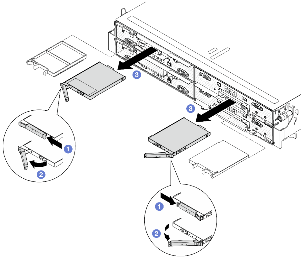
그림 60. E3.S 핫 스왑 드라이브 제거
