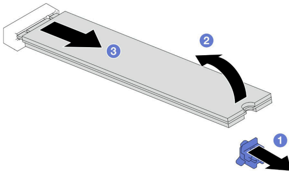
그림 66. M.2 드라이브 제거
