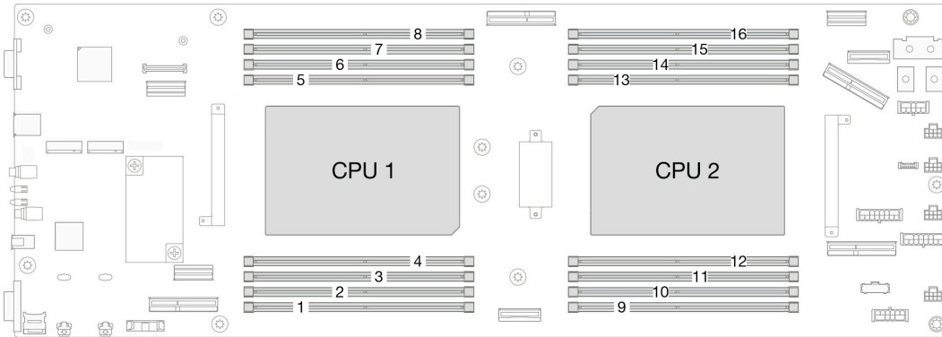
그림 16. 메모리 모듈 및 프로세서 레이아웃
