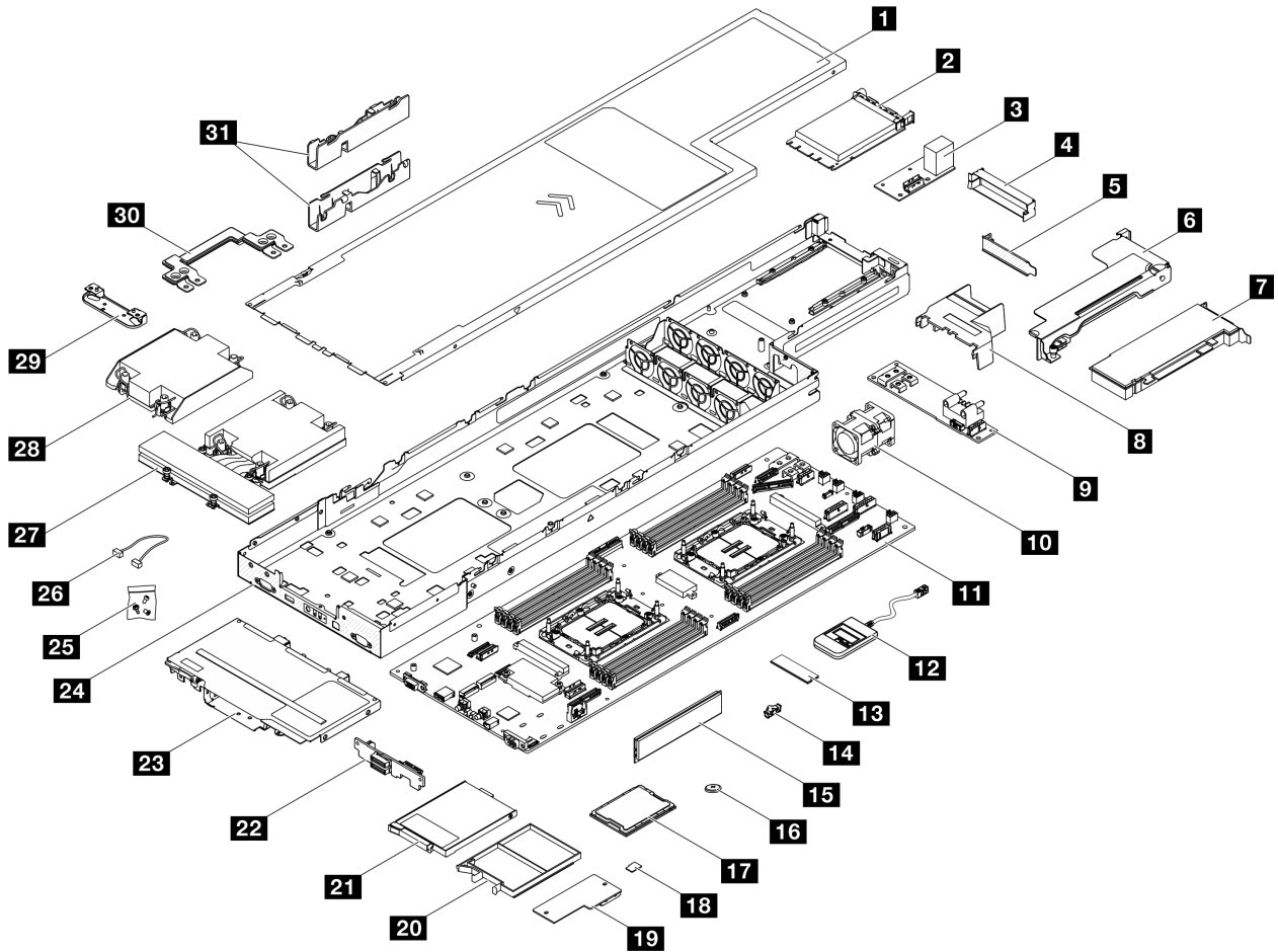
그림 12. 노드 구성 요소
