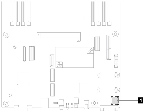
그림 74. MicroSD 소켓의 위치
