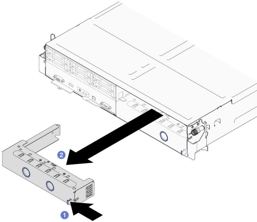
그림 39. 앞면 노드 트레이 필터 제거
