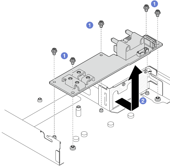
그림 91. 전원 분배 보드 제거
