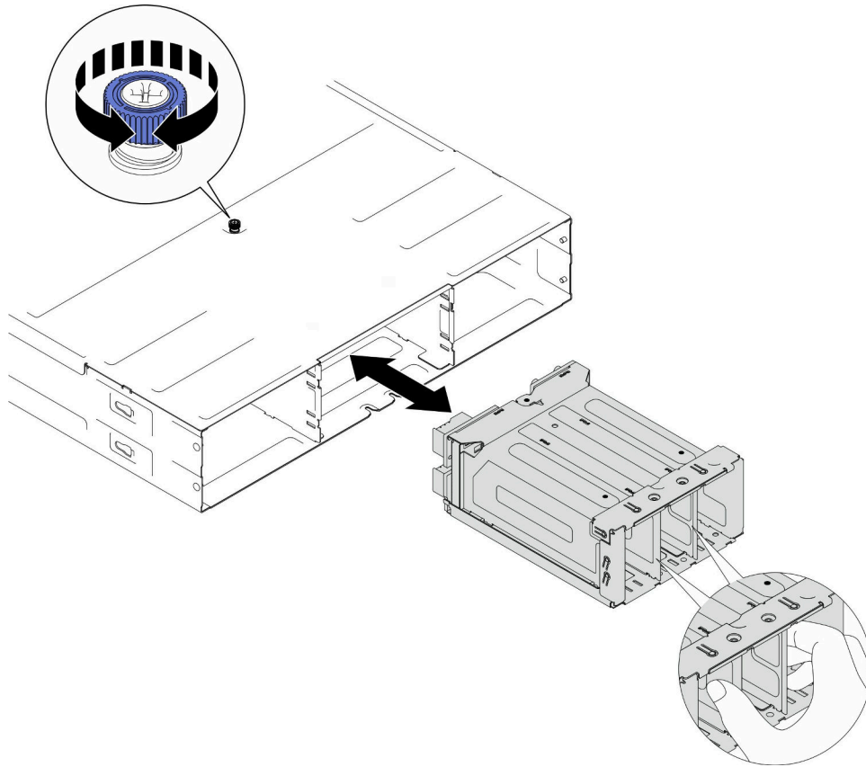
그림 27. PSU 케이스 제거
