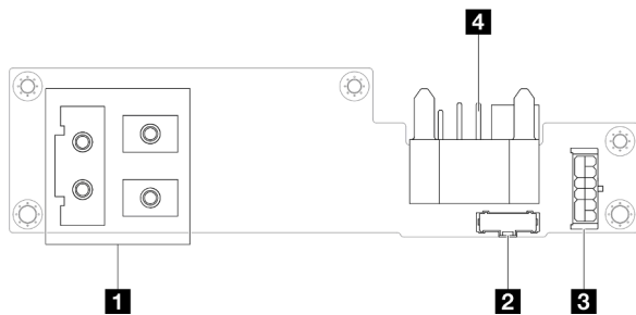
그림 137. 전원 분배 보드 커넥터
