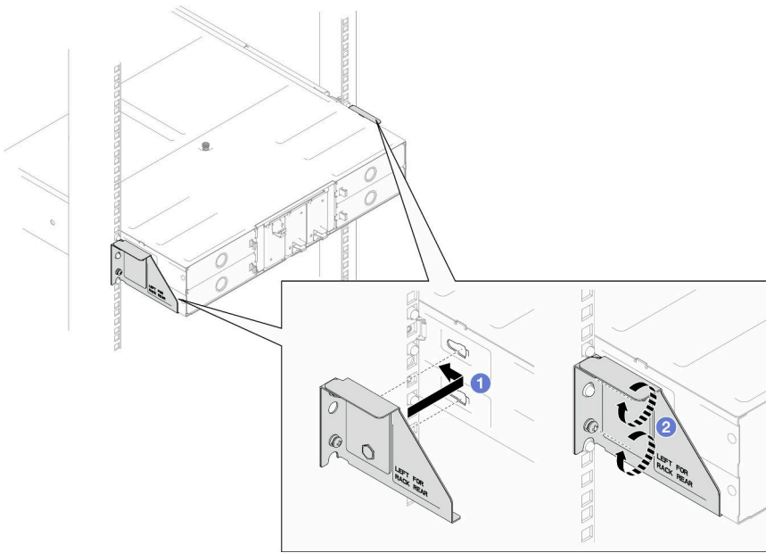
그림 20. 운반 브래킷 설치
