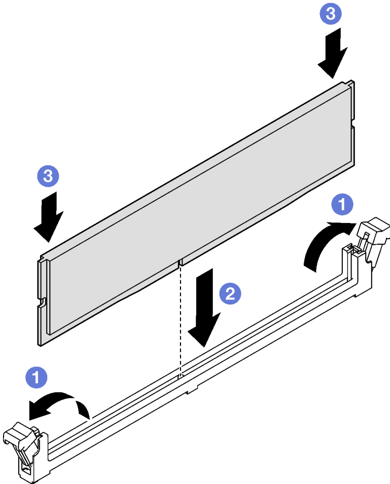
그림 73. 메모리 모듈 설치
