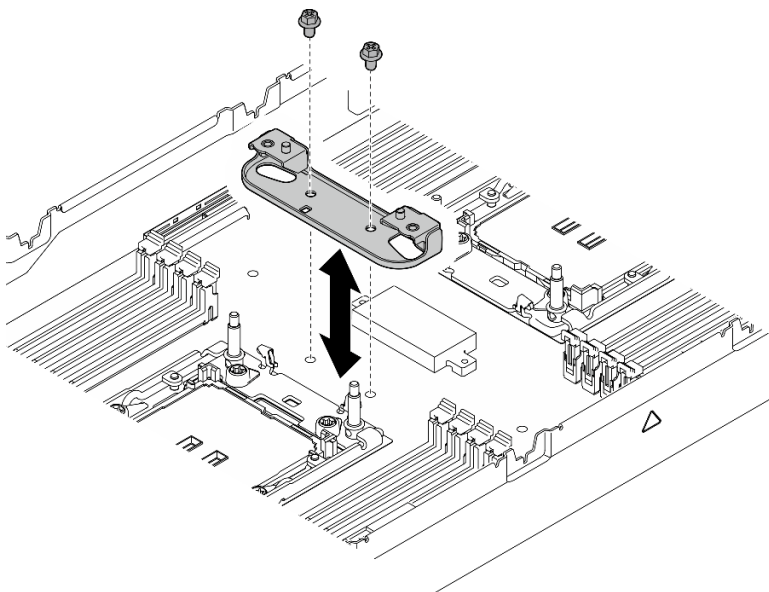
그림 131. 방열판 지지 브래킷 교체
