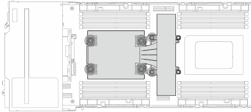
그림 107. 프로세서 1개 구성의 PHM 위치
