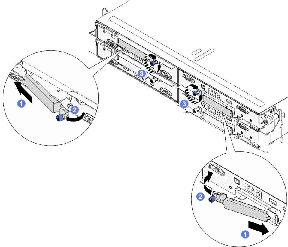
그림 64. E3.S 드라이브 케이지 덮개 설치
