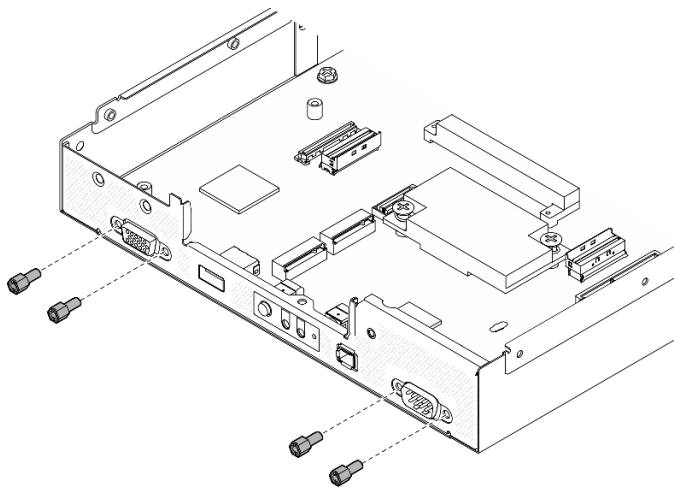
그림 127. 앞면에 시스템 보드 나사 설치
