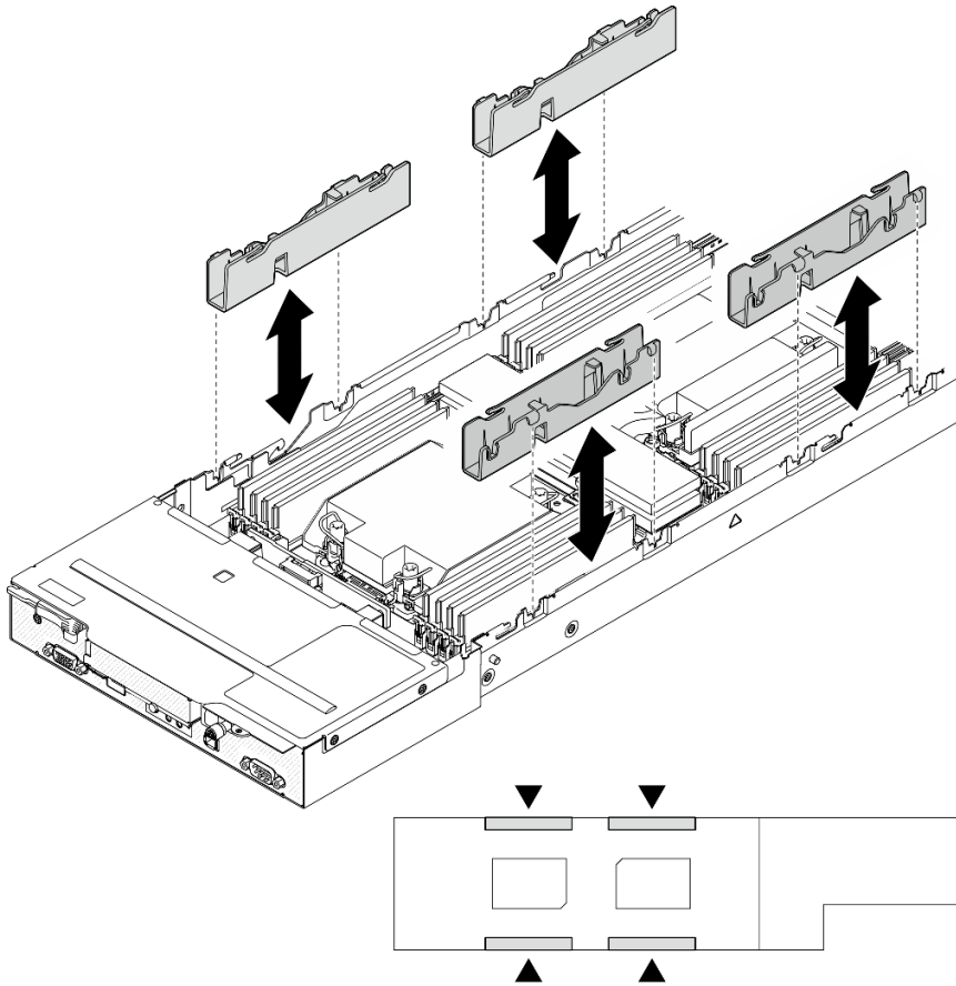
그림 130. 케이블 덕트 교체(프로세서 2개 구성)
