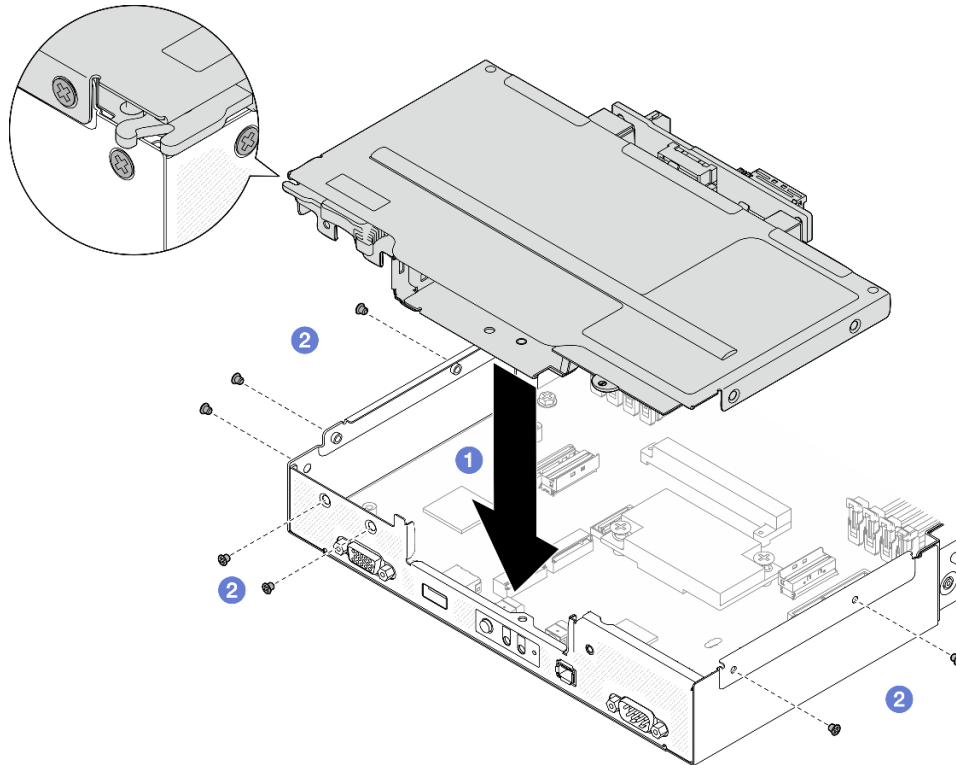
그림 54. 드라이브 케이징 어셈블리 설치
