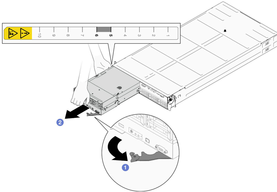
그림 31. 왼쪽 트레이에서 노드 제거
