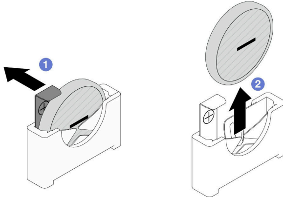
그림 48. CMOS 배터리 제거
