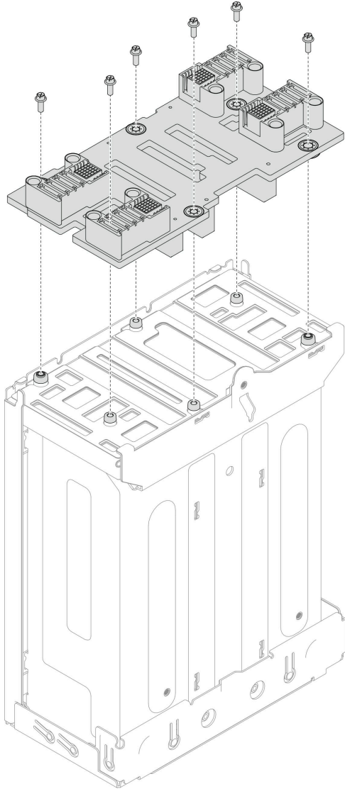
그림 28. 새시 미드플레인 제거
