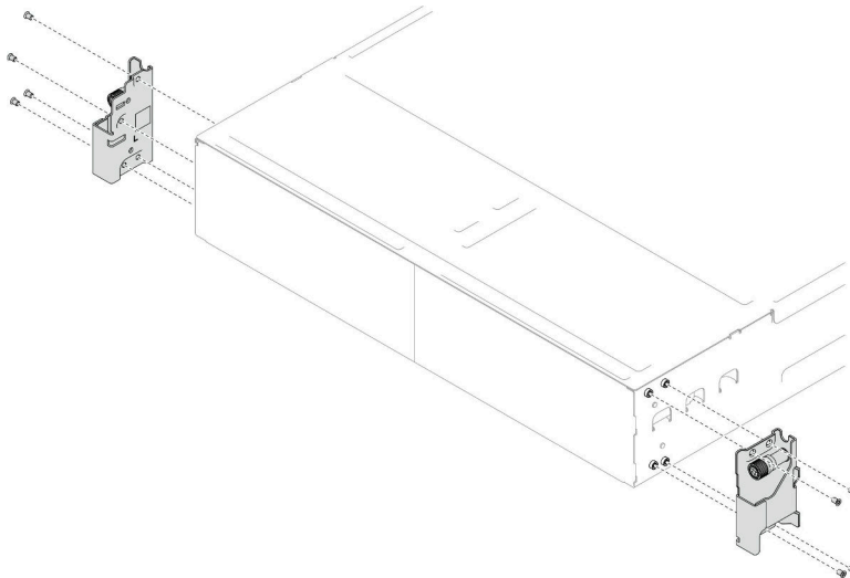
그림 22. EIA 브래킷 설치
