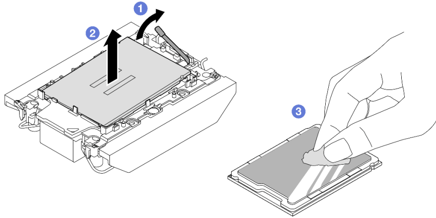
그림 100. 방열판 및 캐리어에서 프로세서 분리 중
