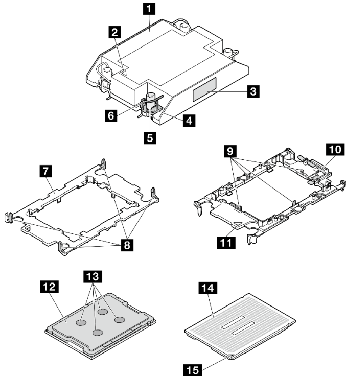
그림 93. PHM 구성 요소
