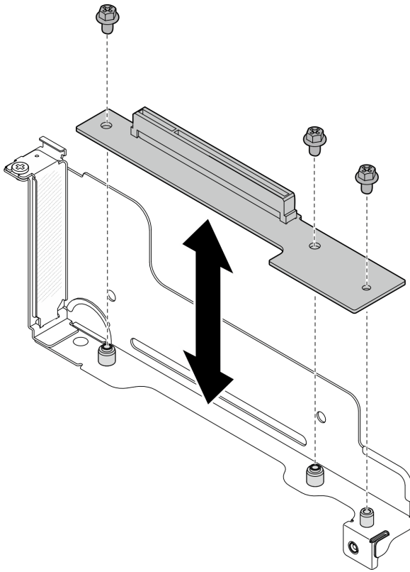
그림 81. PCIe 라이저 카드 교체
