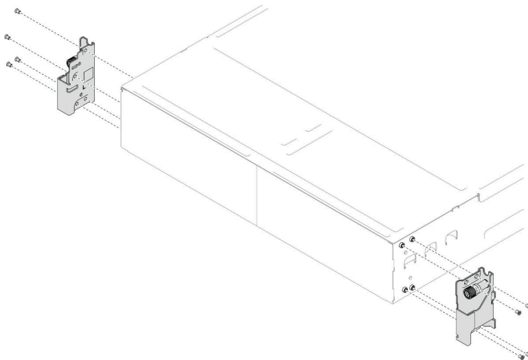
그림 21. EIA 브래킷 제거
