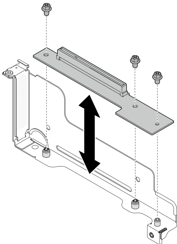
图 66. 更换 PCIe 转接卡
