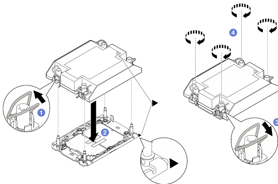
图 95. 为双处理器配置安装 1U 标准 PHM
