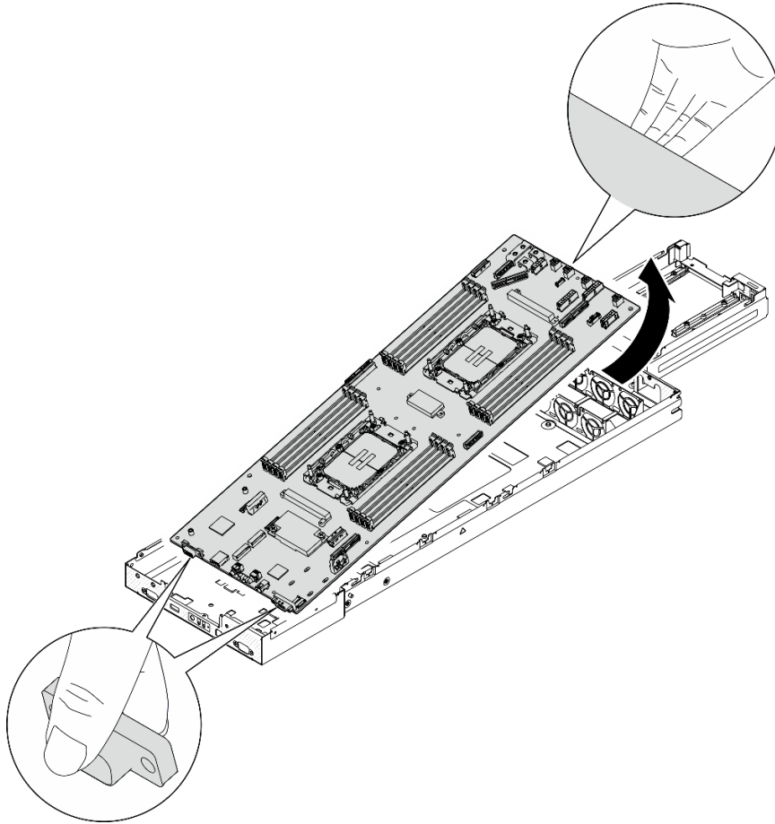
图 110. 卸下主板
