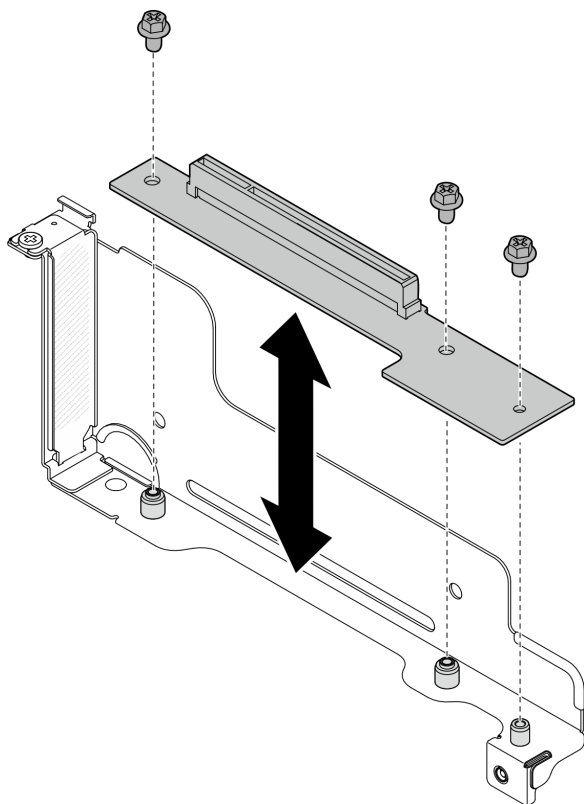
图 70. 更换 PCIe 转接卡
