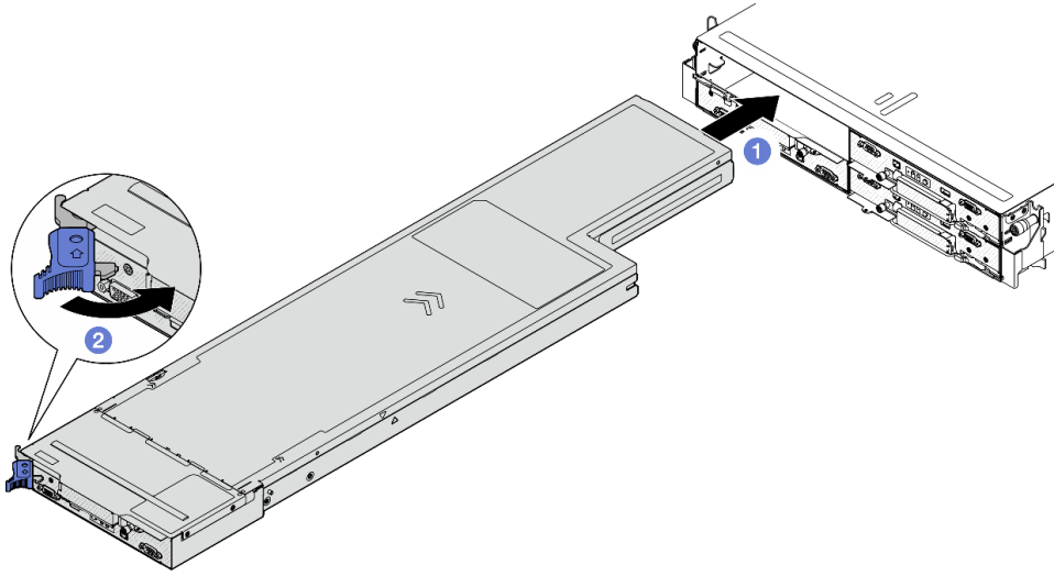
图 27. 将节点安装到左侧托盘
