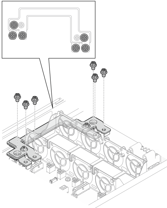
图 75. 安装电源汇流条外侧螺钉
