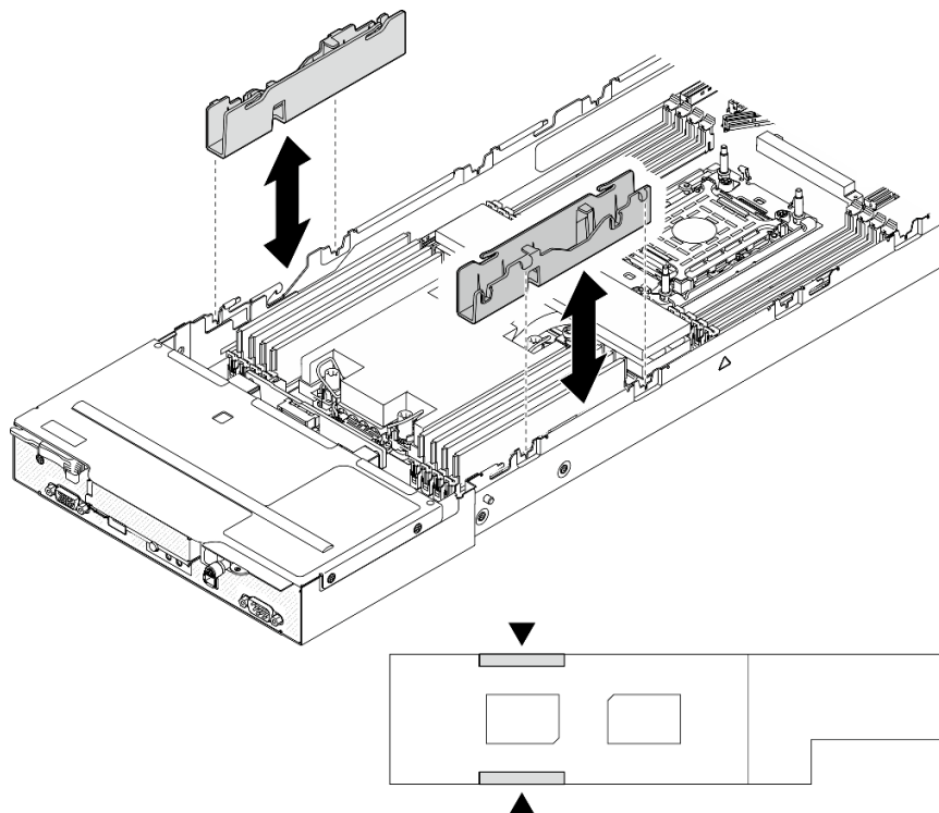
图 106. 更换线缆槽（单处理器配置）
