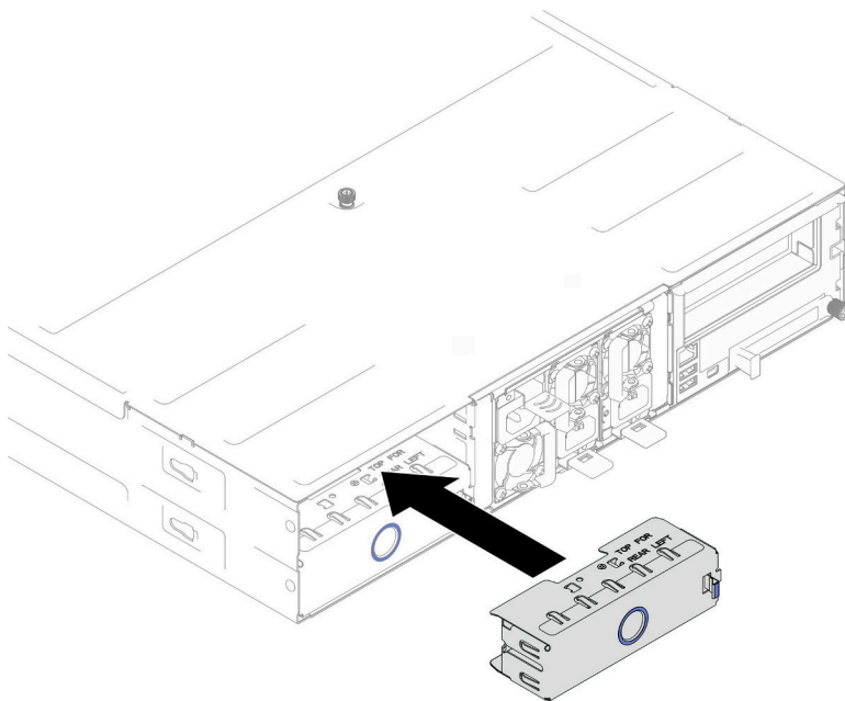
图 23. 安装背面节点托盘填充件
