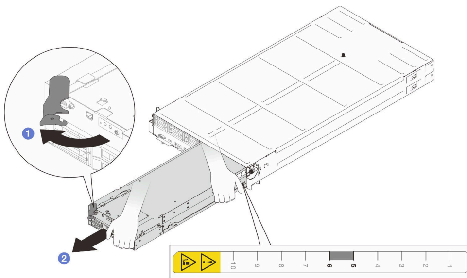
图 19. 将节点从右侧托盘卸下
