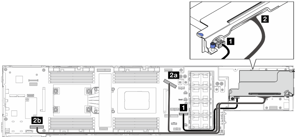
图 125. PCIe 转接卡线缆布放 - 一个处理器
