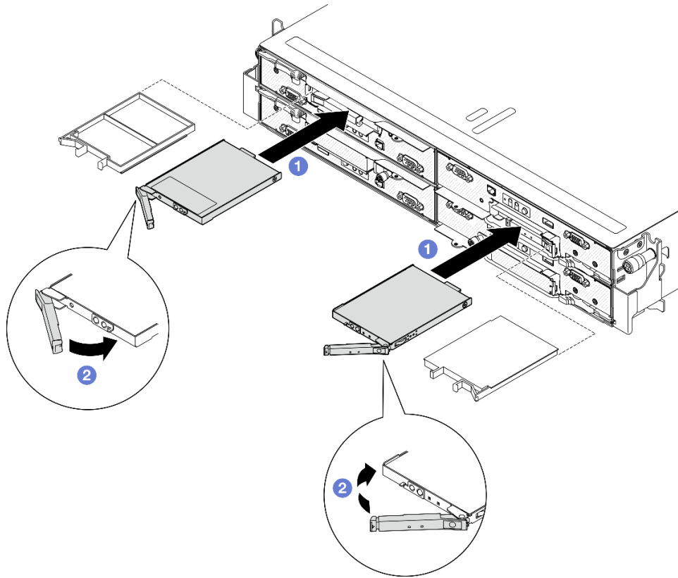
图 48. 安装 E3.S 热插拔硬盘
