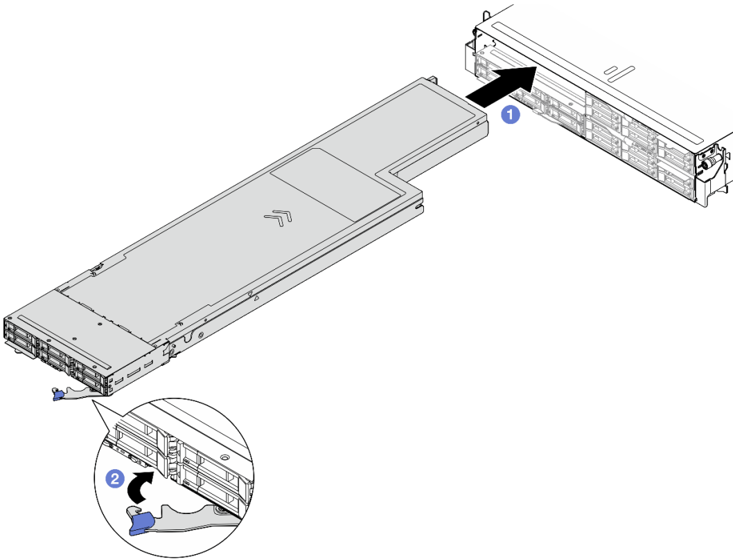
图 28. 将节点安装到左侧托盘
