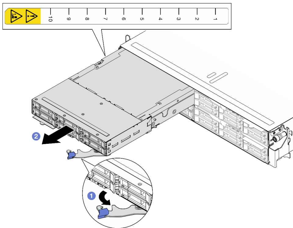
图 18. 将节点从左侧托盘卸下
