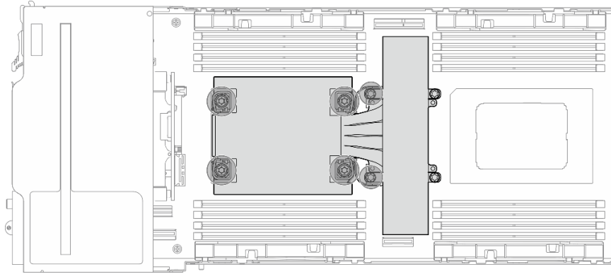
图 79. 单处理器配置的 PHM 位置
