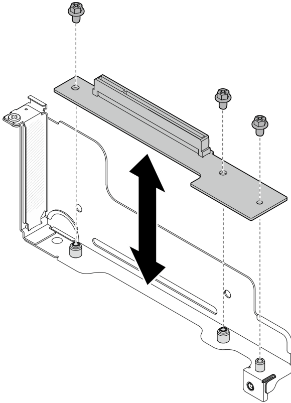
图 68. 更换 PCIe 转接卡
