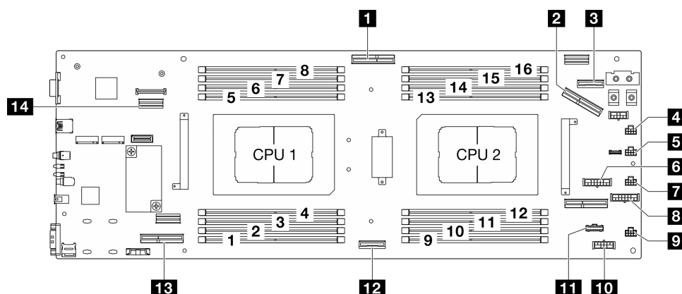
图 119. 用于线缆布放的主板接口
