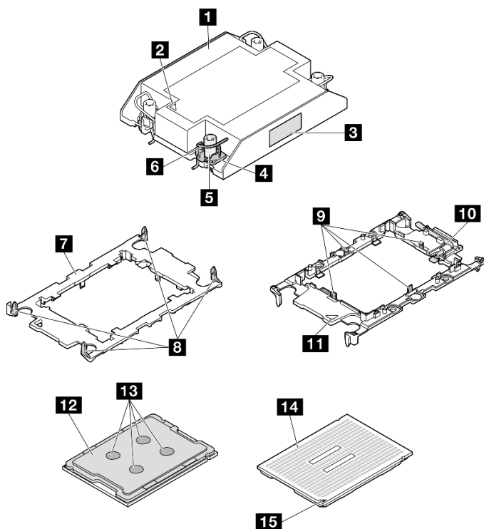
图 87. PHM 组件
