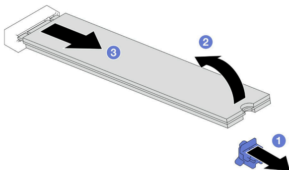
图 51. 卸下 M.2 硬盘
