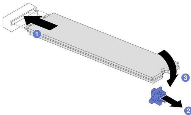
图 54. 安装 M.2 硬盘
