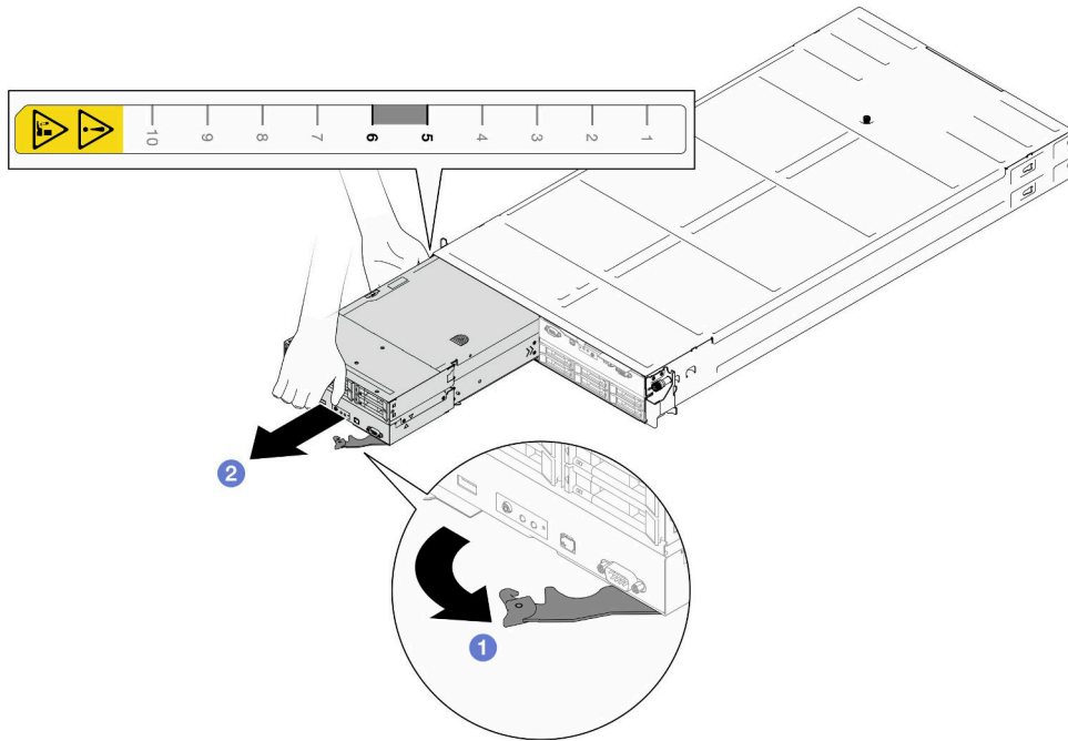
图 16. 将节点从左侧托盘卸下
