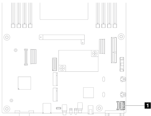
图 61. MicroSD 插槽位置
