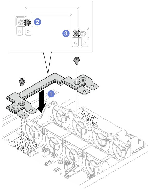
图 74. 安装电源汇流条
