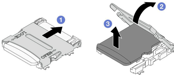
图 60. 卸下 MicroSD 卡
