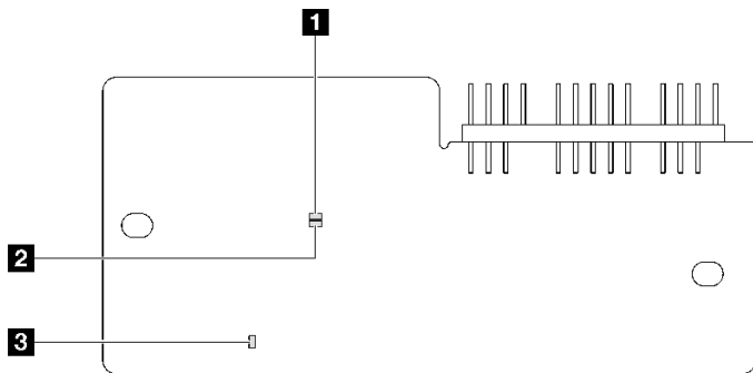
图 135. 固件和 RoT 安全模块上的 LED
