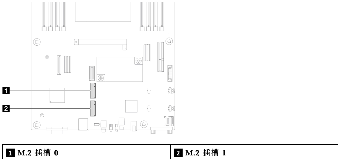
图 50. 主板上 M.2 插槽的位置
