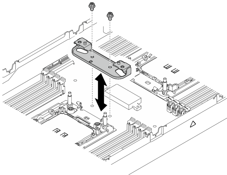
图 116. 更换散热器支撑架
