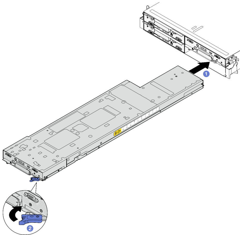
图 30. 将节点安装到右侧托盘
