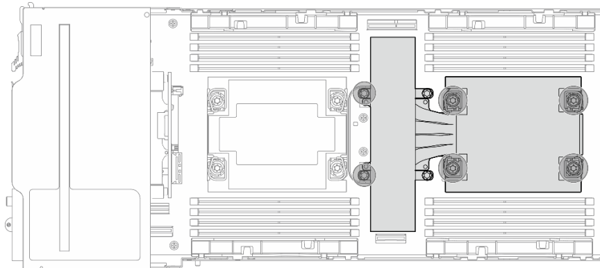
图 80. 双处理器配置的 PHM 位置
