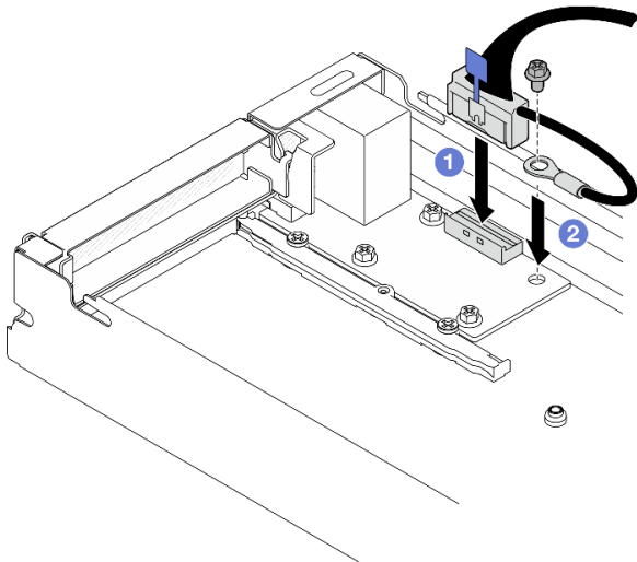
图 129. 安装背面 I/O 线缆和接地线缆
