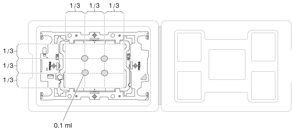
图 89. 为装运托盘中的处理器涂抹导热油脂
