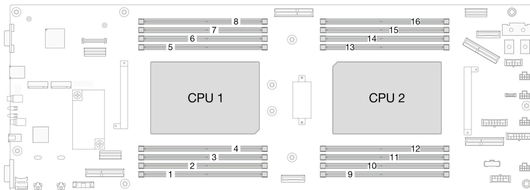
图 1. 内存条和处理器布局
