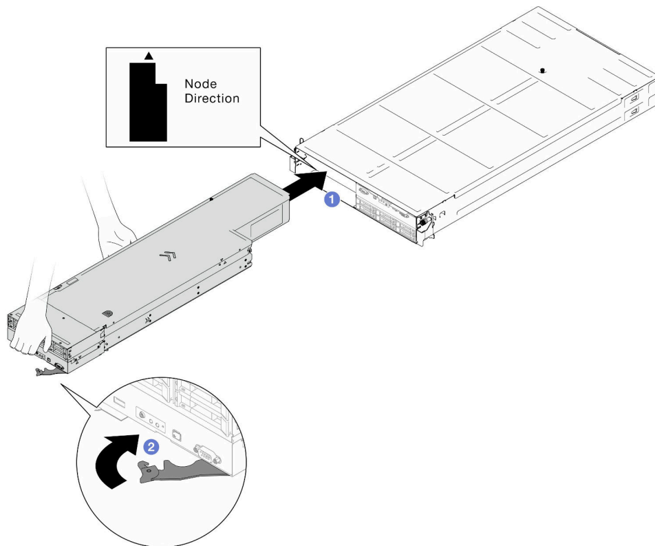
图 26. 将节点安装到左侧托盘
