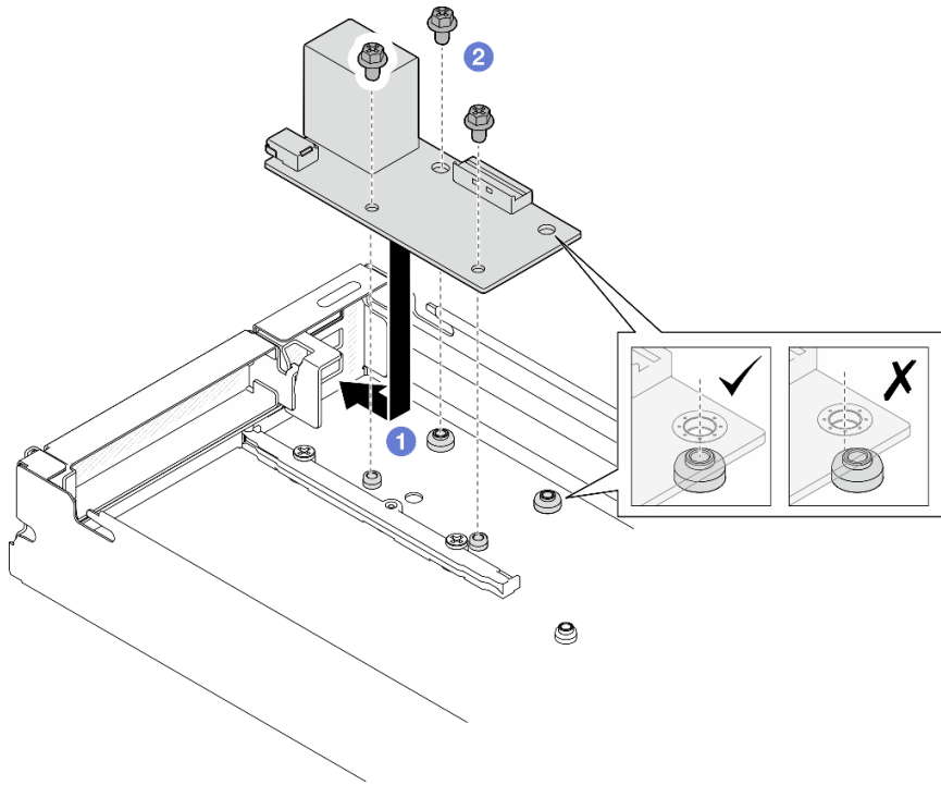
图 99. 安装背面 I/O 模块
