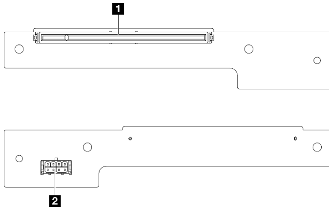
图 121. PCIe 转接卡接口
