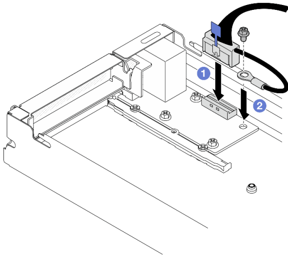
图 100. 安装背面 I/O 线缆和接地线缆
