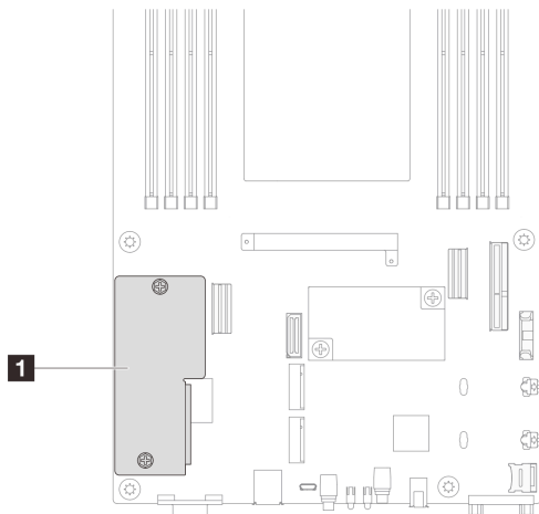
图 103. 固件和 RoT 安全模块位置
