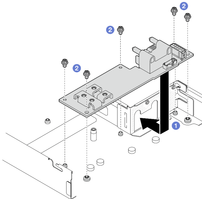
图 77. 安装配电板
