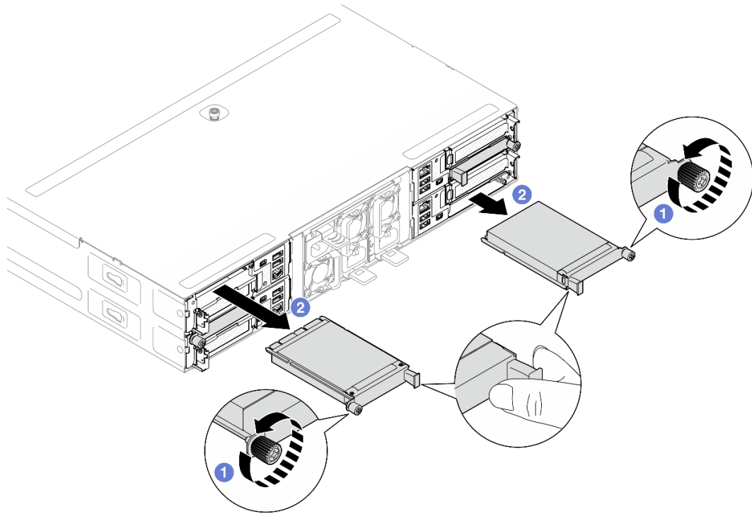
图 63. 卸下背面 OCP 模块
