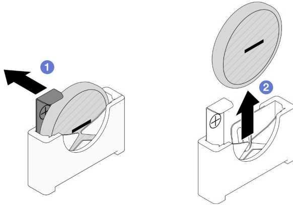
图 33. 卸下 CMOS 电池
