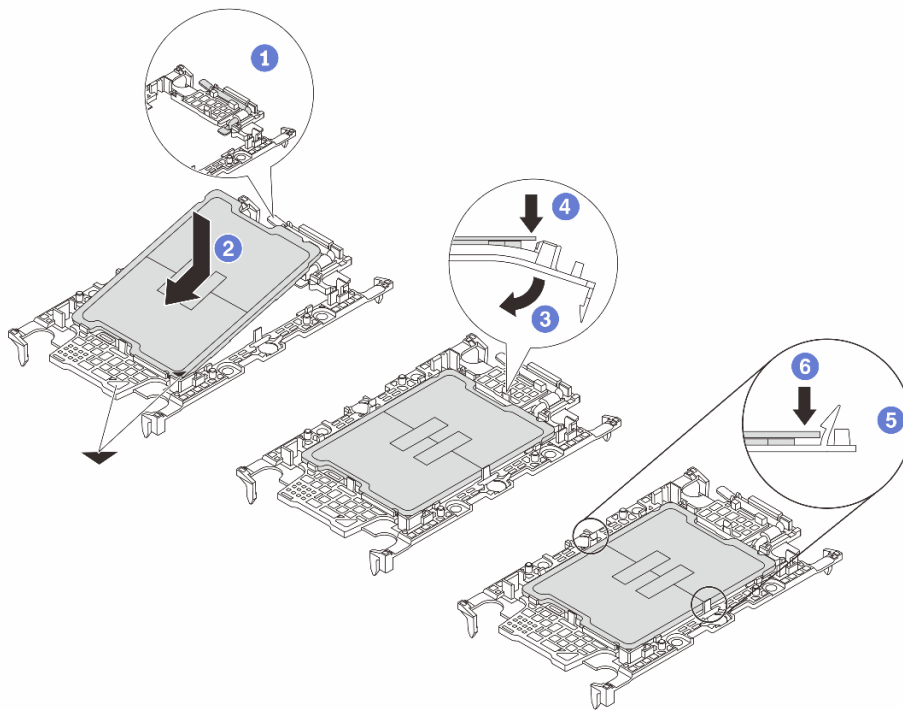
图 88. 安装处理器支架
