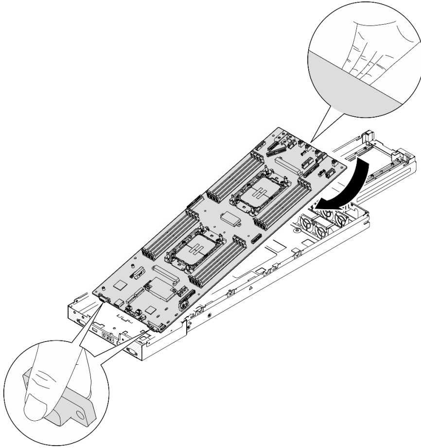
图 111. 安装主板
