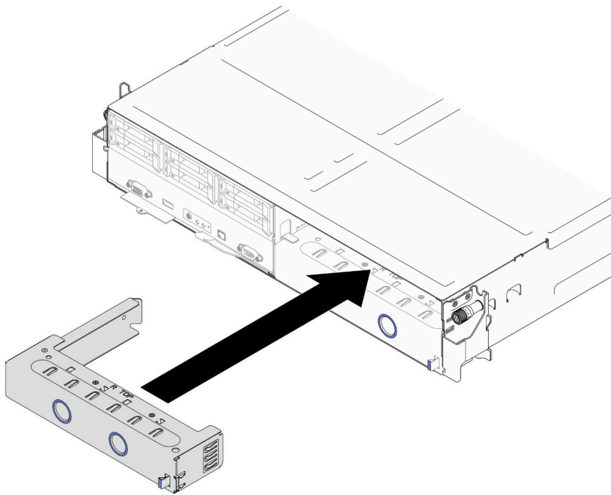
图 22. 安装正面节点托盘填充件
