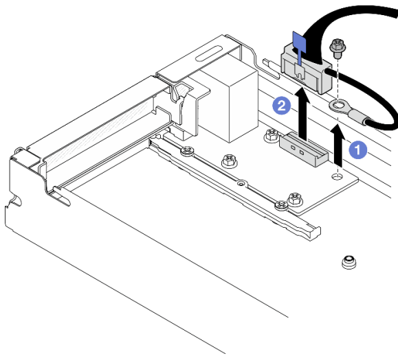
图 97. 卸下背面 I/O 线缆和接地线缆
