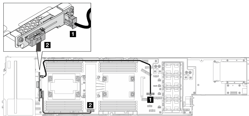
图 123. E3.S 硬盘背板的线缆布放
