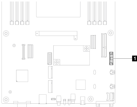
图 32. CMOS 电池插槽位置
