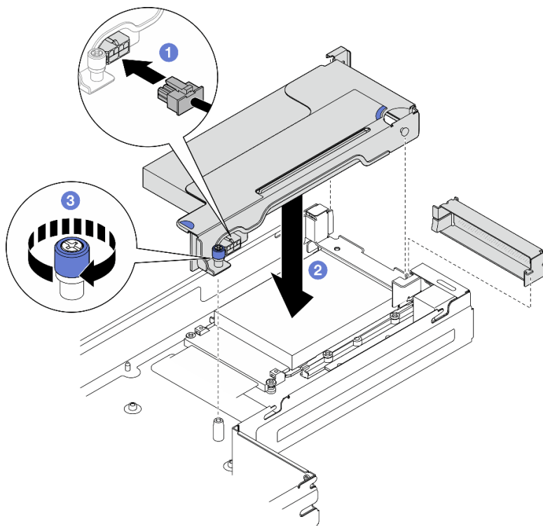
图 71. 安装 PCIe 转接卡组合件
