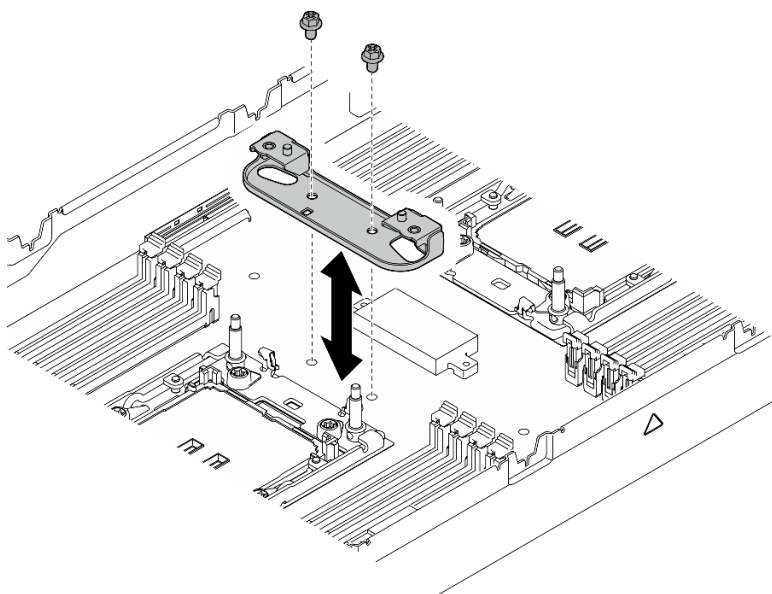
图 84. 更换散热器支撑架
