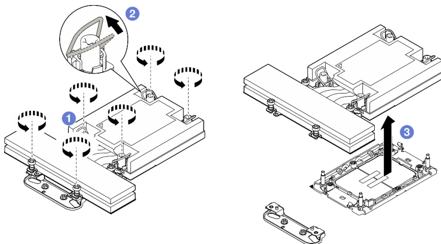
图 83. 从处理器 2 上卸下 1U 高性能 PHM
