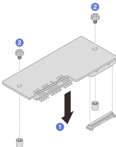
图 104. 安装固件和 RoT 安全模块
