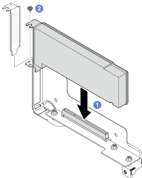
图 69. 安装 PCIe 适配器
