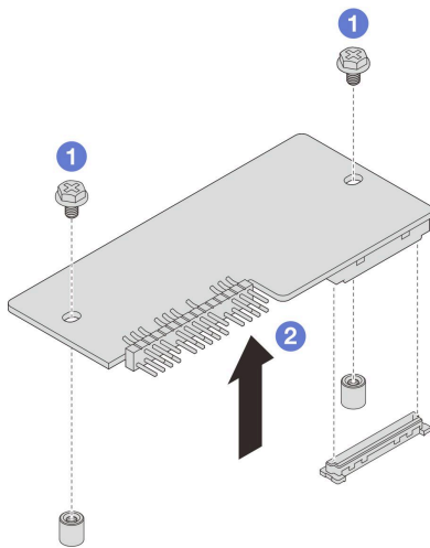
图 102. 卸下固件和 RoT 安全模块
