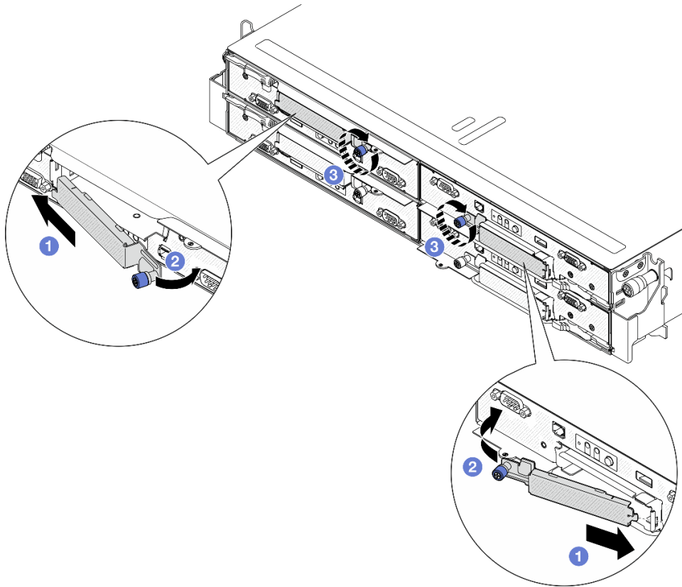
图 49. 安装 E3.S 硬盘仓盖
