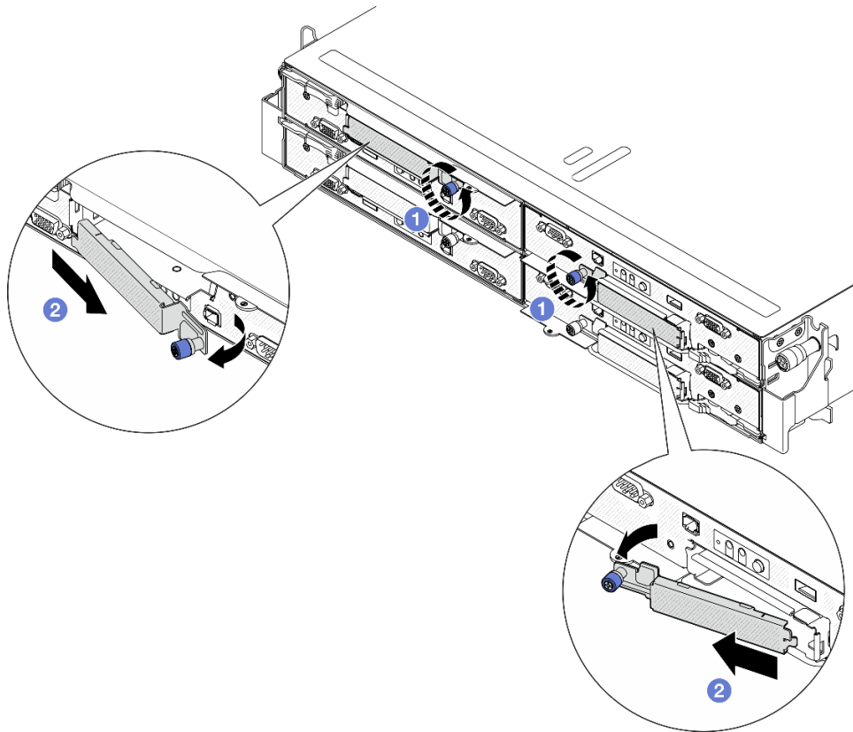
图 47. 卸下 E3.S 硬盘仓盖
