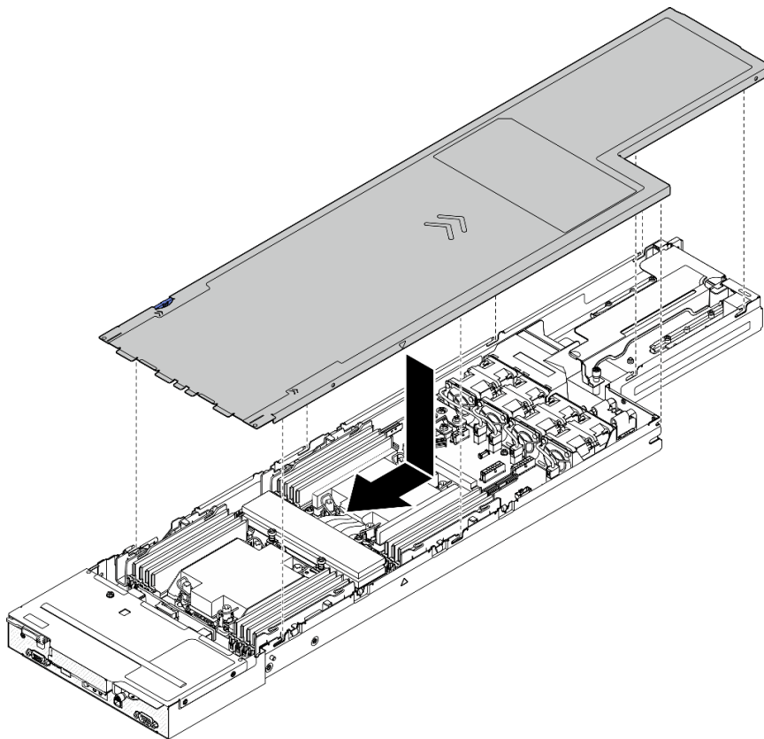
图 118. 安装顶盖
