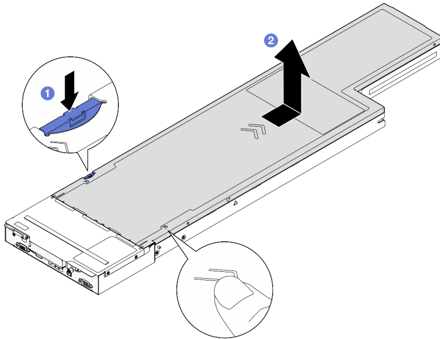
图 117. 卸下顶盖
