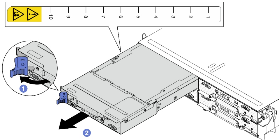
图 17. 将节点从左侧托盘卸下
