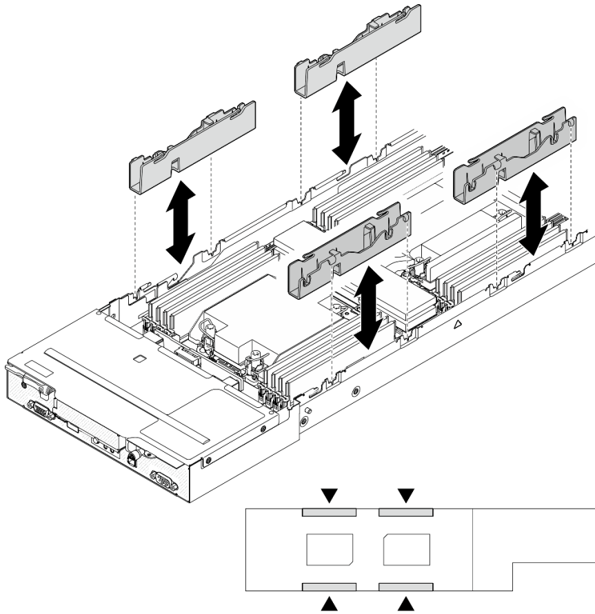
图 107. 更换线缆槽 (双处理器配置)
