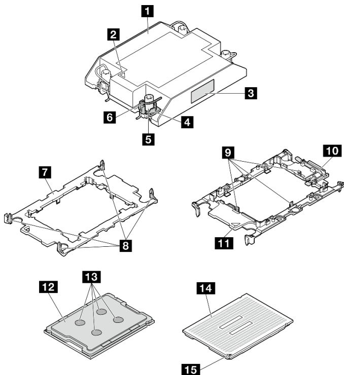
图 78. PHM 组件
