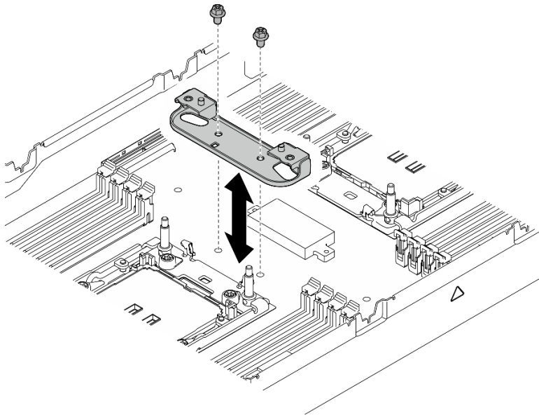
图 91. 更换散热器支撑架
