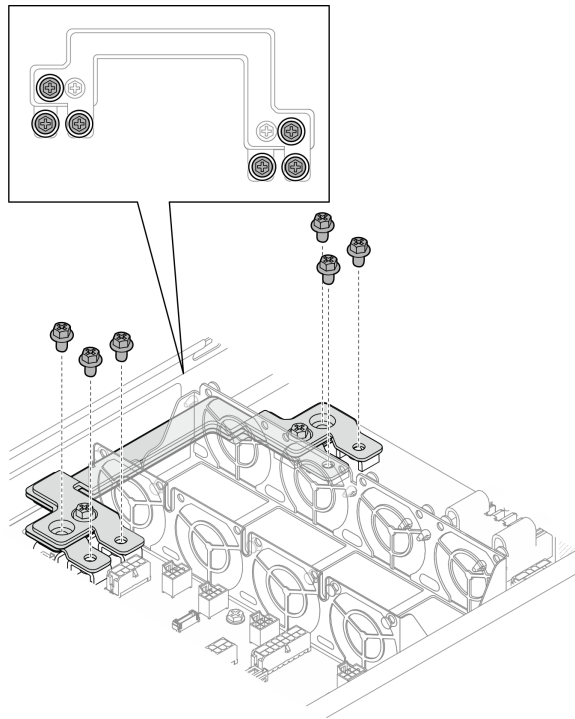
图 72. 卸下电源汇流条外侧螺钉
