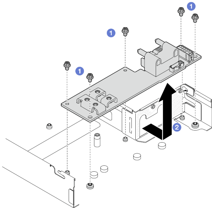
图 76. 卸下配电板
