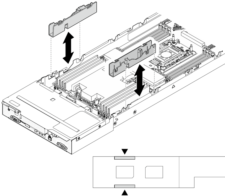
图 114. 更换线缆槽（单处理器配置）
