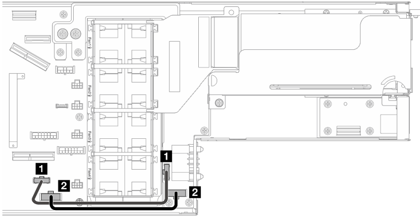
图 127. 配电板的线缆布放
