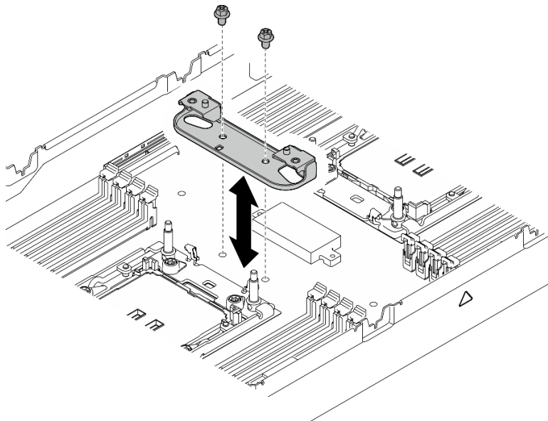
图 105. 更换散热器支撑架
