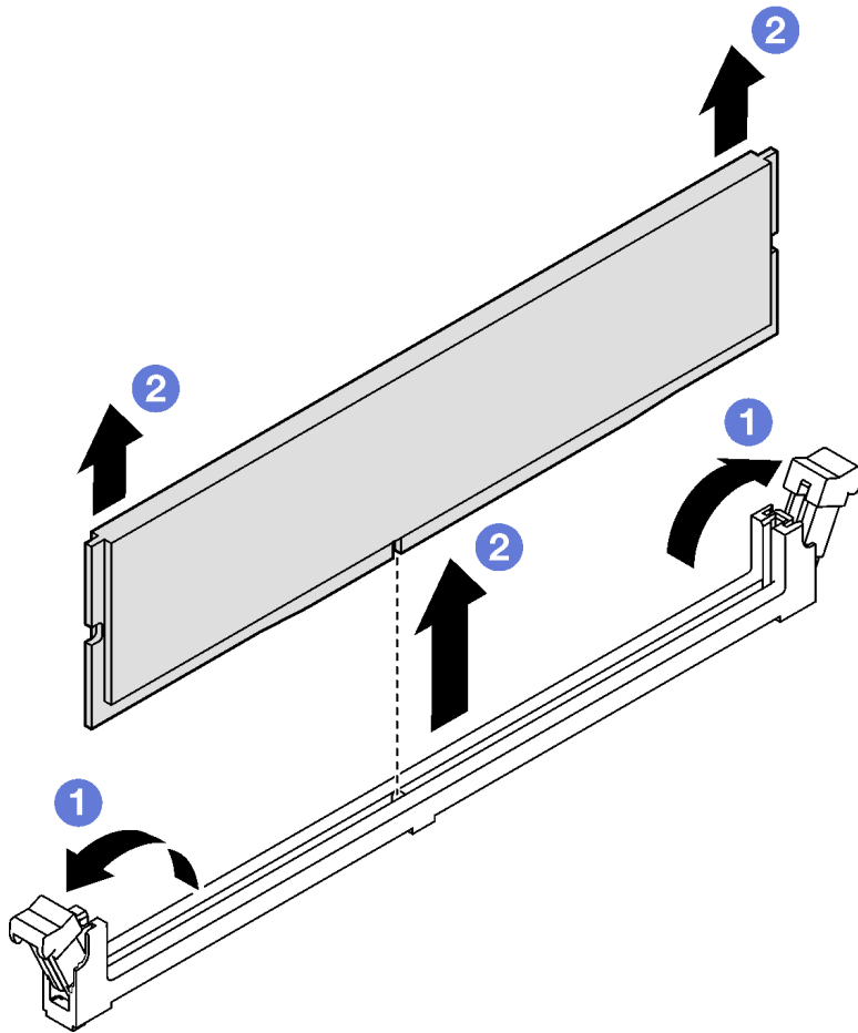
图 56. 卸下内存条
