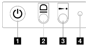
图 133. 正面操作员面板上的按钮和 LED
