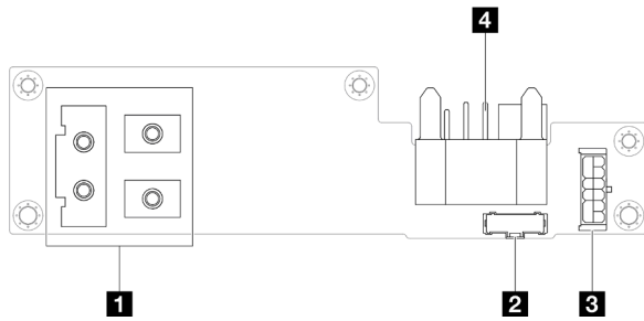
图 122. 配电板接口
