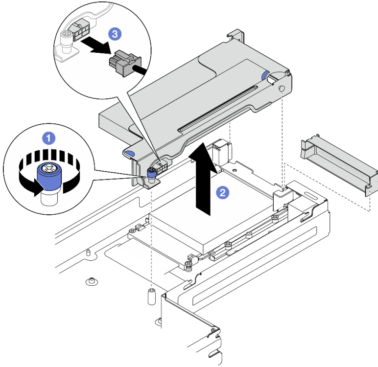
图 65. 卸下 PCIe 转接卡组合件
