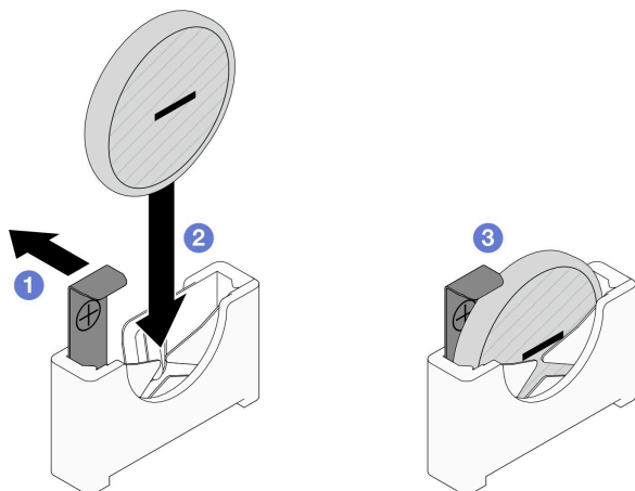
图 35. 安装 CMOS 电池
