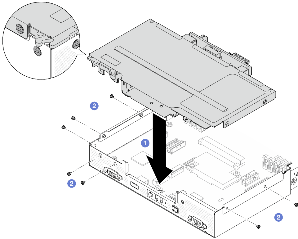
图 39. 安装硬盘仓组合件
