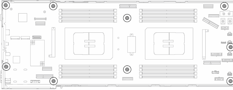
图 113. 安装主板上的螺钉
