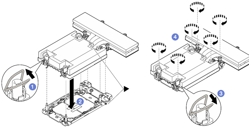
图 93. 为单处理器配置安装 1U 高性能 PHM
