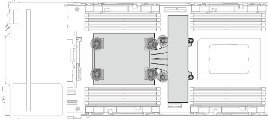
图 92. 单处理器配置的 PHM 位置
