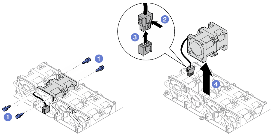
图 40. 卸下风扇
