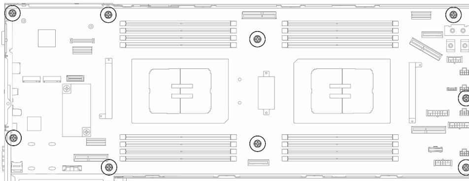
图 109. 卸下螺钉
