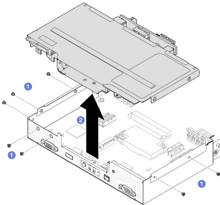
图 36. 卸下硬盘仓组合件
