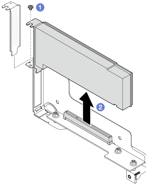
图 67. 卸下 PCIe 适配器
