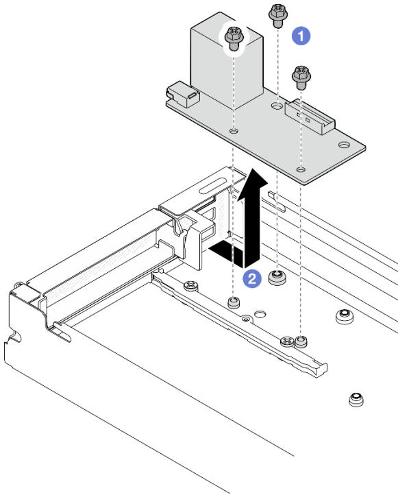
图 98. 卸下背面 I/O 模块
