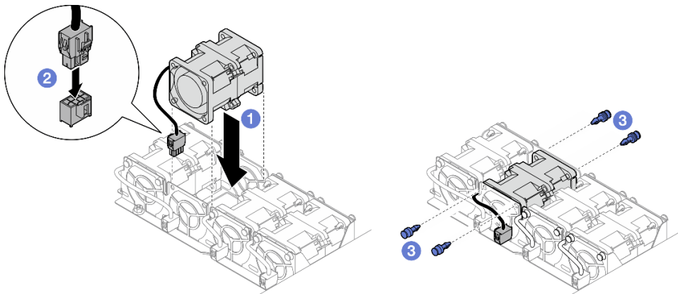
图 41. 安装风扇
