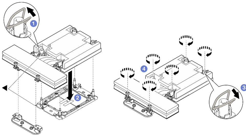
图 96. 为双处理器配置安装 1U 高性能 PHM
