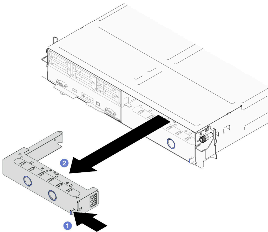
图 24. 卸下正面节点托盘填充件
