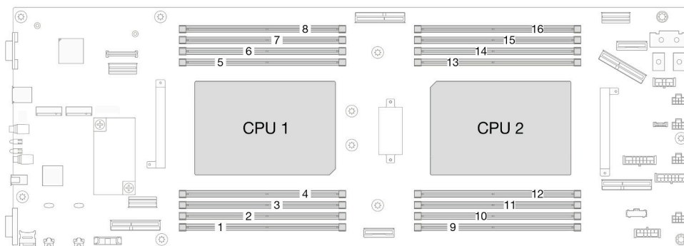
图 57. 内存条和处理器布局
