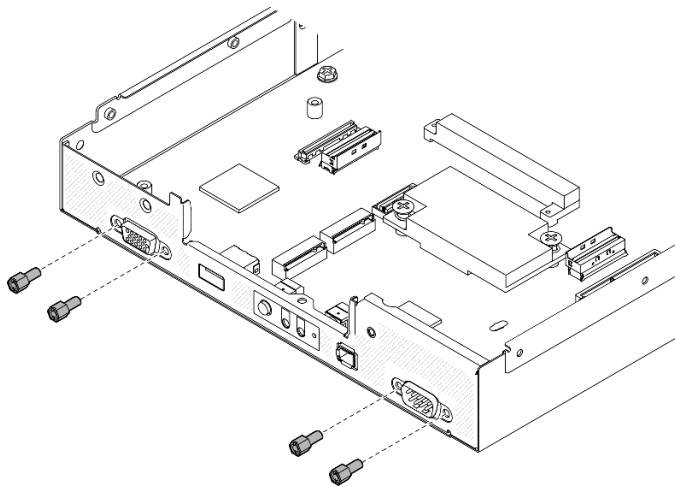
图 112. 安装正面的主板螺钉
