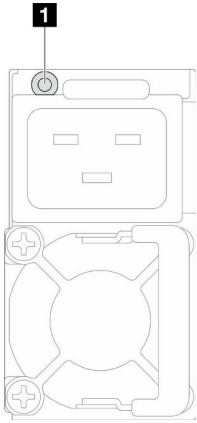
图 13. 电源模块 LED
