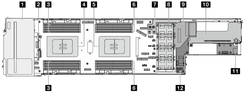
图 8. SD530 V3 俯视图
