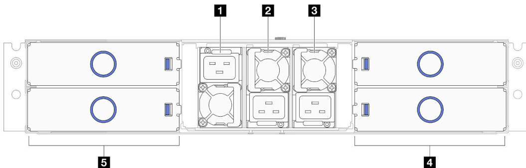
图 4. 机箱后视图
