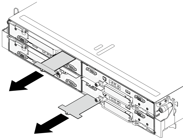
图 19. 抽取式信息卡上的 Lenovo XClarity Controller 网络访问标签
