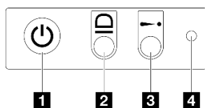
图 12. 正面操作员面板上的按钮和 LED
