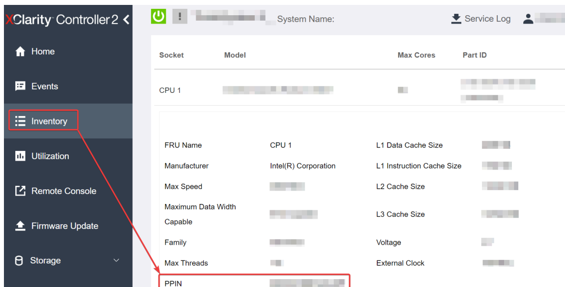
图 22. 通过 XCC Web GUI 读取 PPIN
