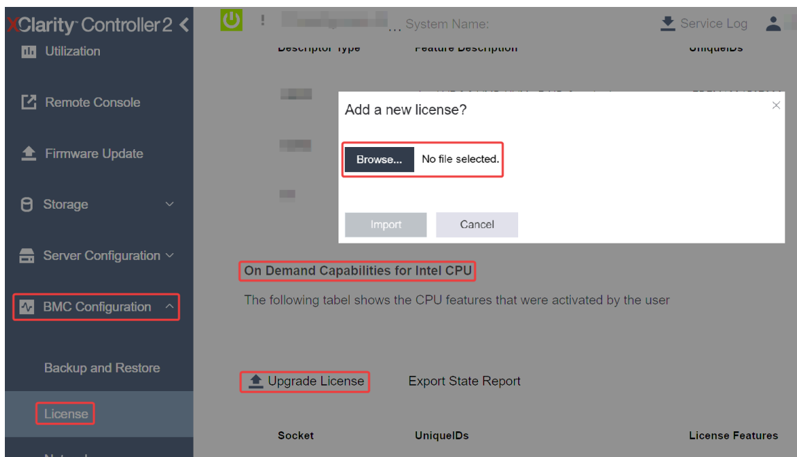
图 23. 通过 XCC Web GUI 上传激活密钥
