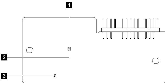
图 14. 固件和 RoT 安全模块上的 LED
