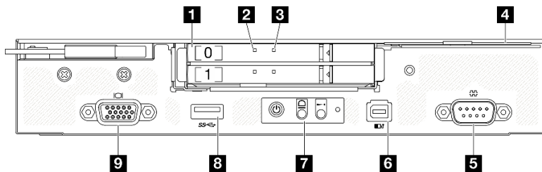
图 3. ThinkSystem SD530 V3 节点的前视图
