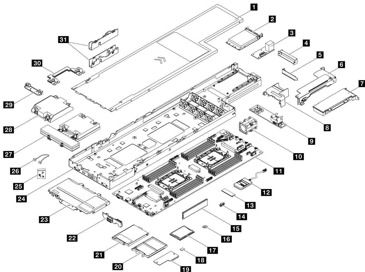
图 17. 节点组件
