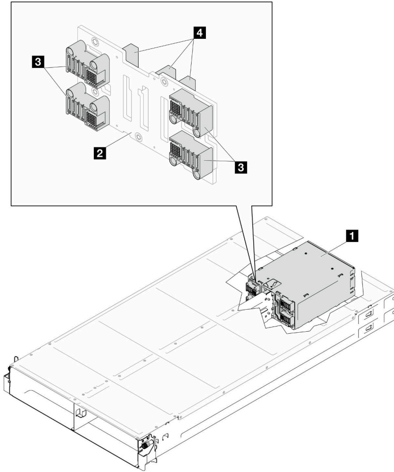
图 9. D3 机箱中面板位置和接口
