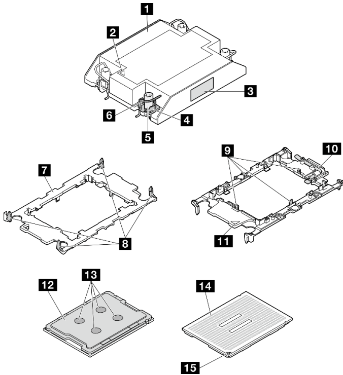
图 93. PHM 组件
