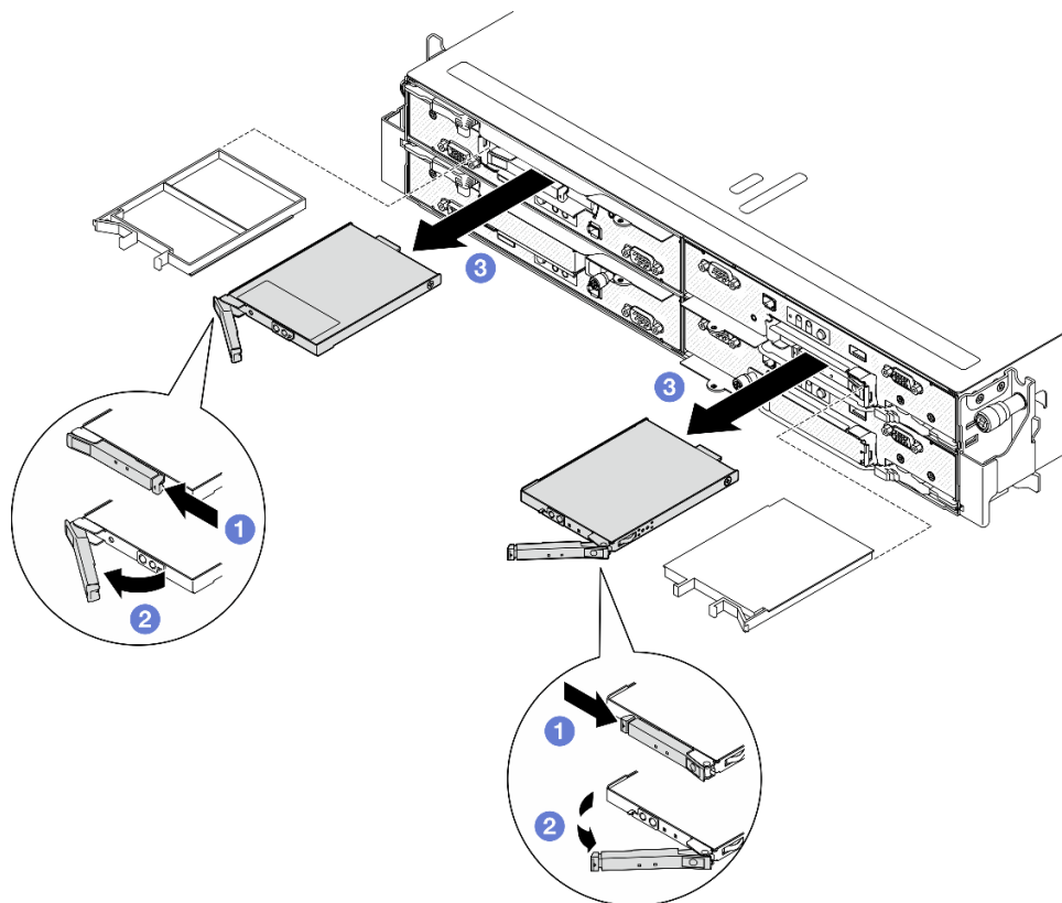
图 60. 卸下 E3.S 热插拔硬盘
