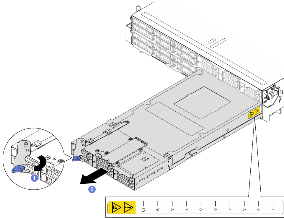
图 36. 将节点从右侧托盘卸下
