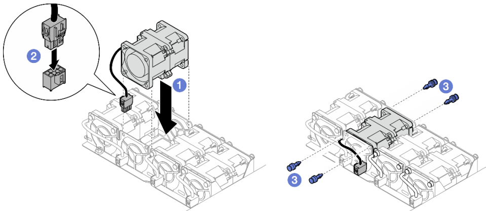
图 56. 安装风扇
