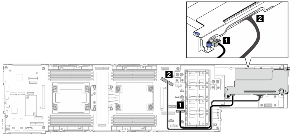
图 141. PCIe 转接卡线缆布放 - 两个处理器
