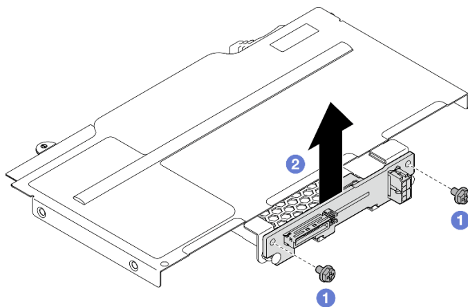
图 52. 卸下硬盘背板
