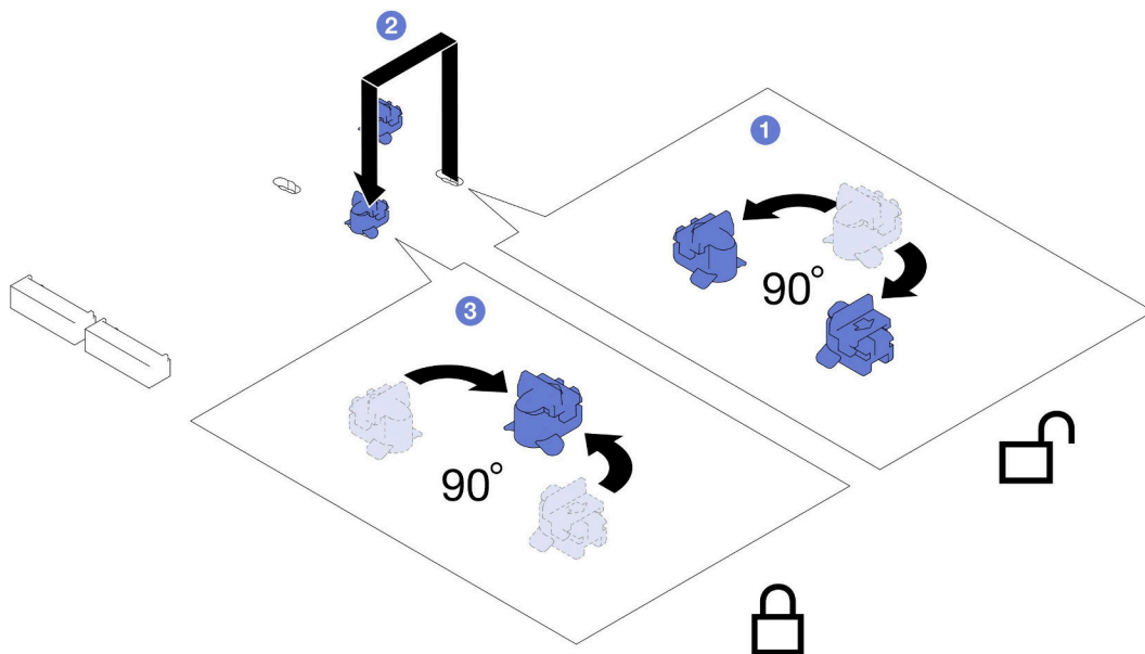
图 67. 调整 M.2 硬盘固定器
