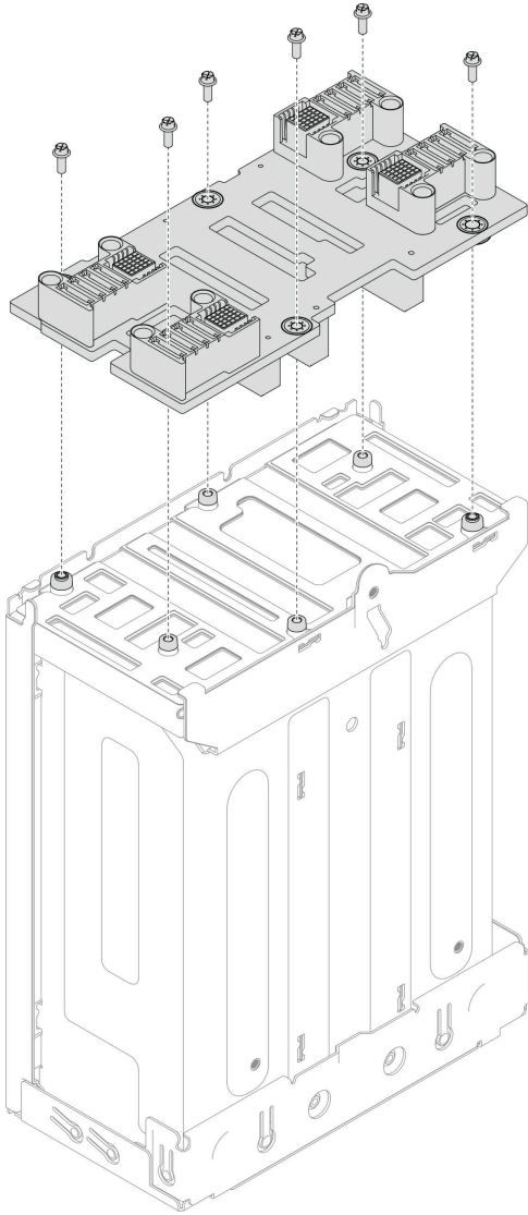
图 28. 卸下机箱中面板
