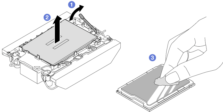
图 100. 将处理器与散热器和支架分开
