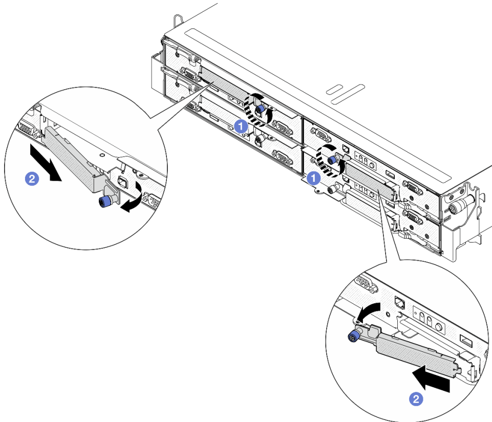
图 59. 卸下 E3.S 硬盘仓盖
