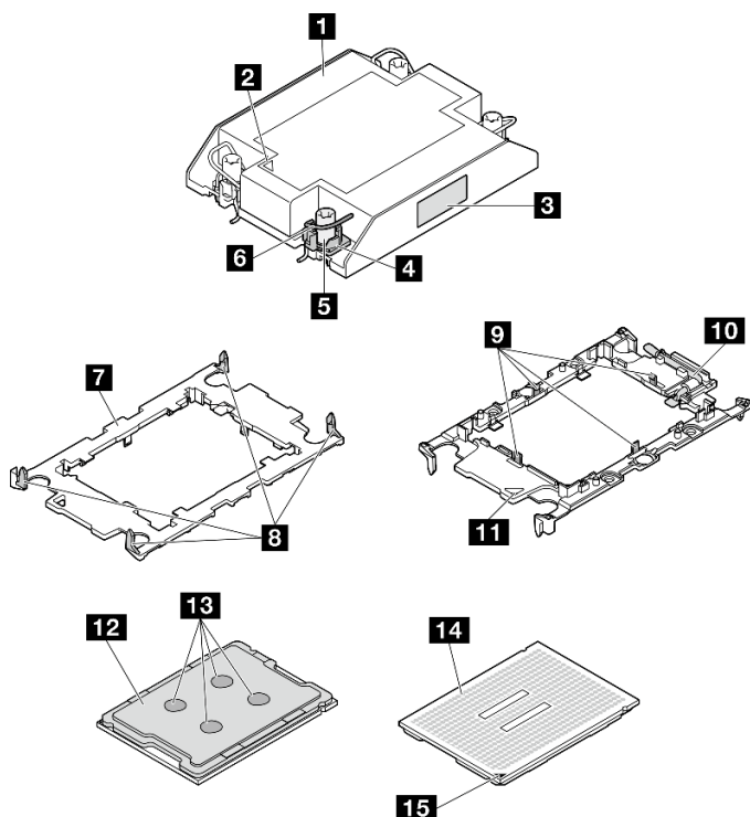
图 102. PHM 组件
