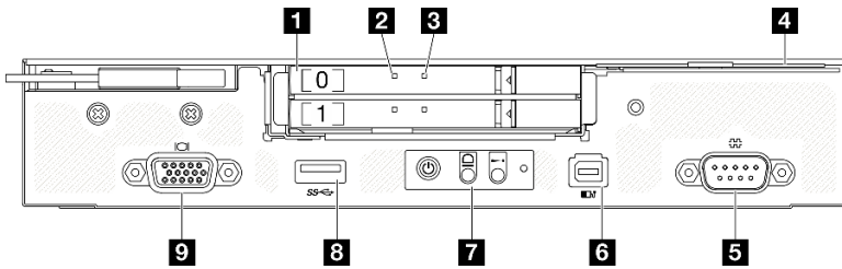
图 3. ThinkSystem SD530 V3 节点的前视图
