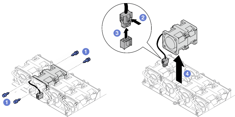
图 55. 卸下风扇
