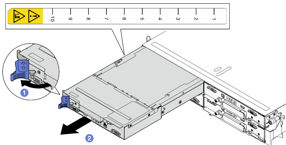
图 32. 将节点从左侧托盘卸下
