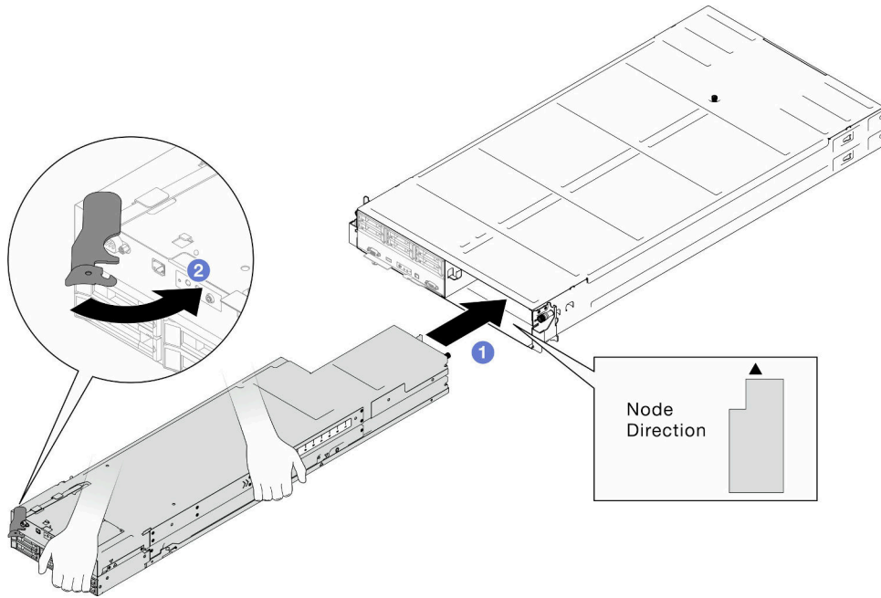
图 44. 将节点安装到右侧托盘
