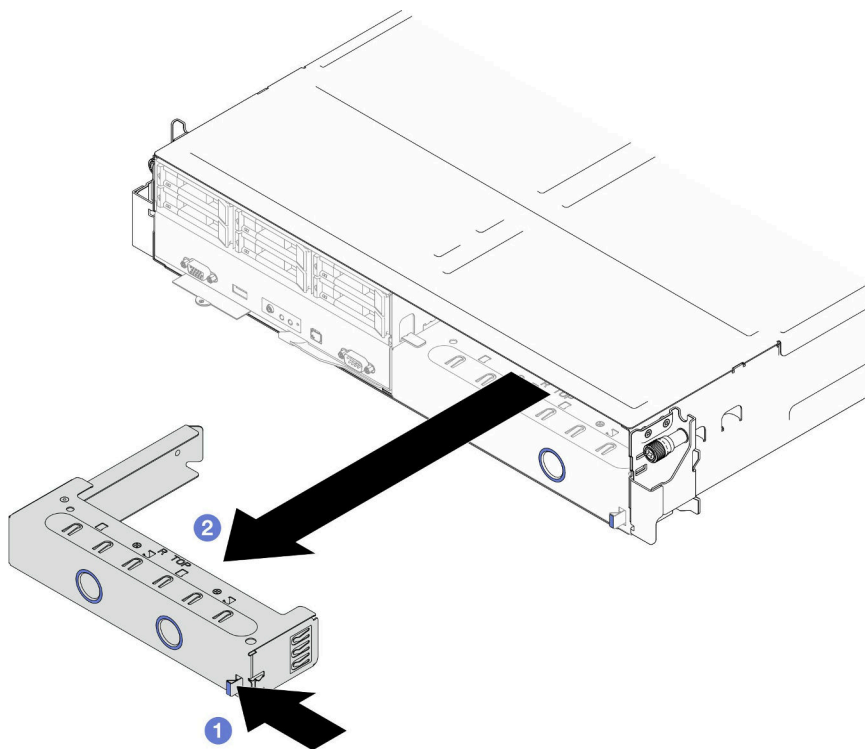
图 39. 卸下正面节点托盘填充件
