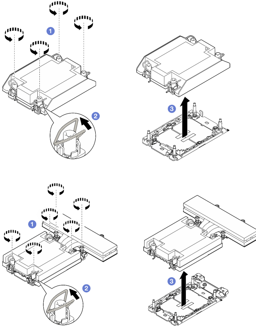
图 97. 从处理器 1 上卸下 1U 高性能 PHM
