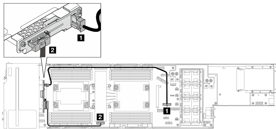
图 138. E3.S 硬盘背板的线缆布放
