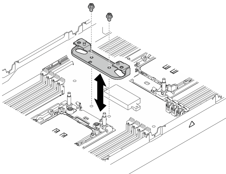
图 99. 更换散热器支撑架
