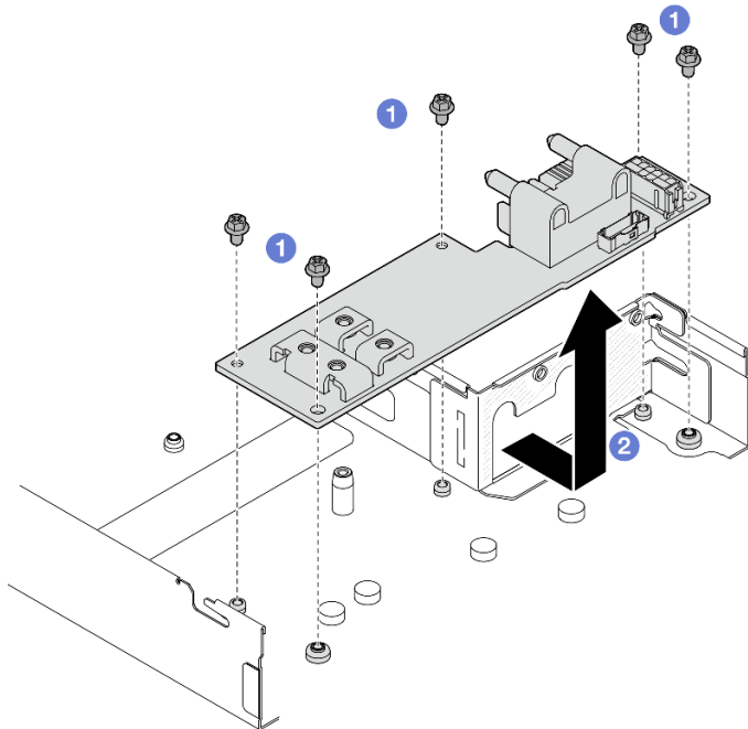
图 91. 卸下配电板
