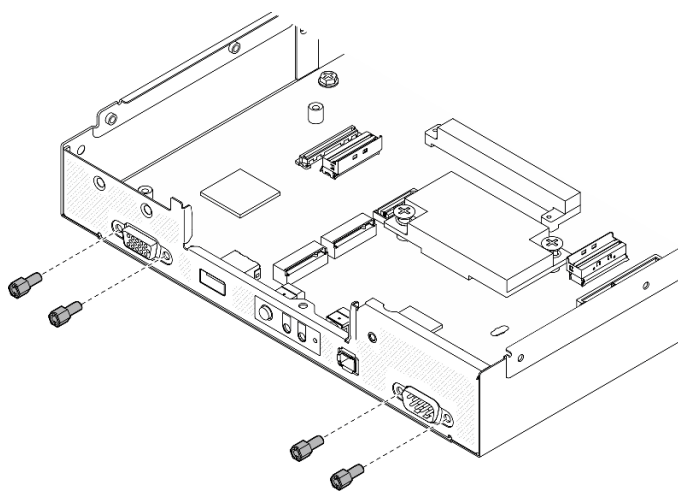
图 123. 卸下螺钉
