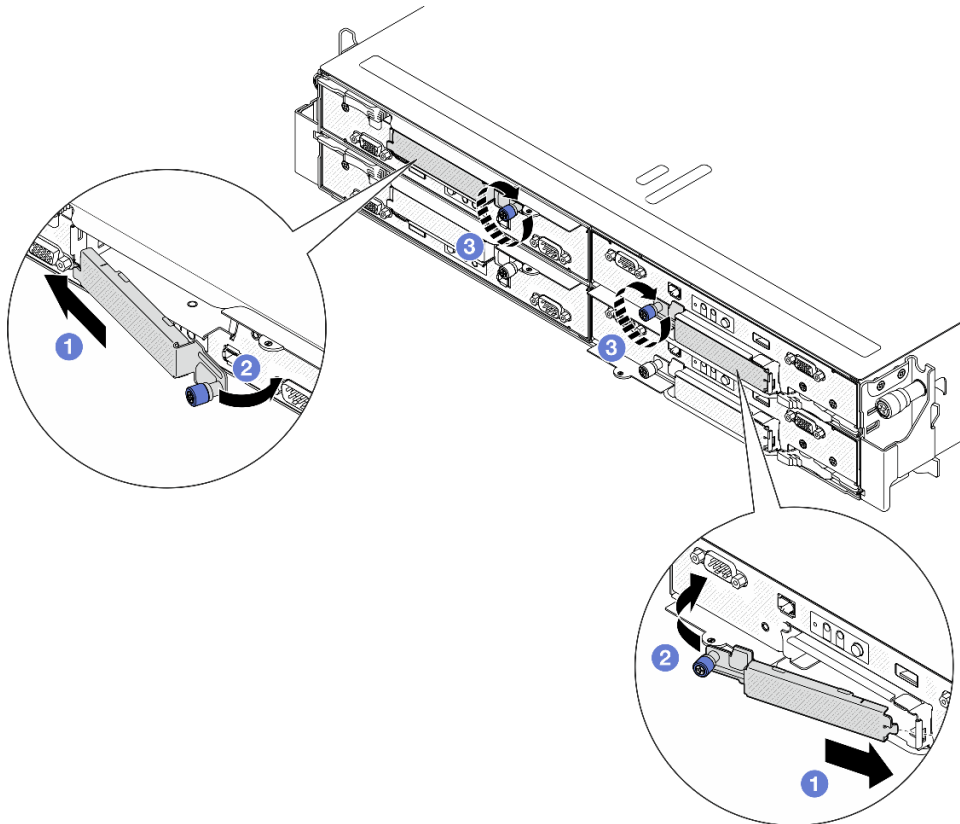
图 64. 安装 E3.S 硬盘仓盖
