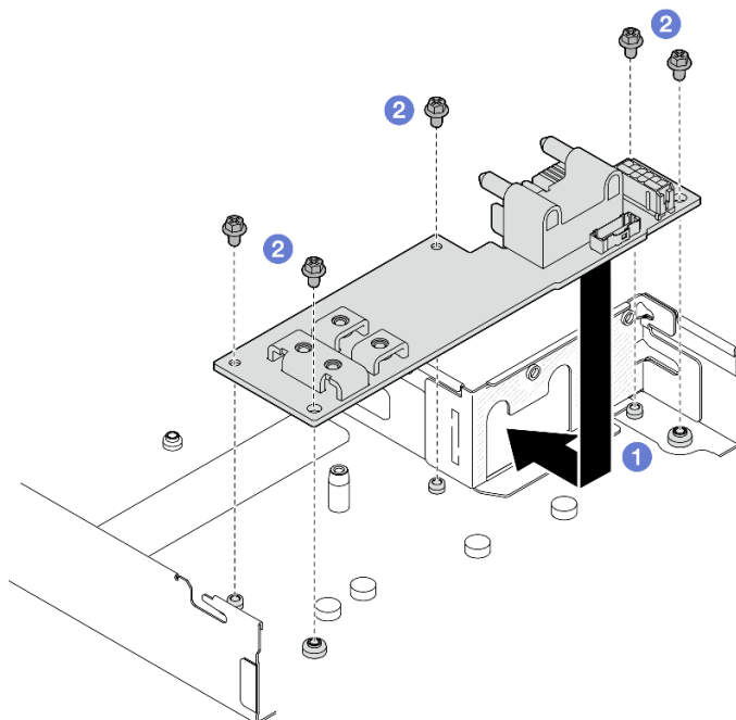
图 92. 安装配电板
