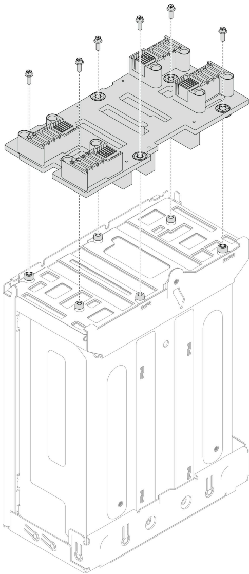
图 29. 安装机箱中面板
