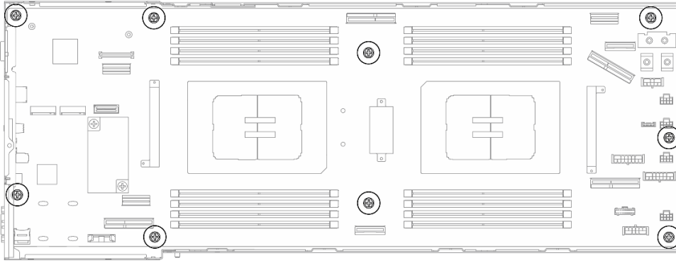
图 128. 安装主板上的螺钉
