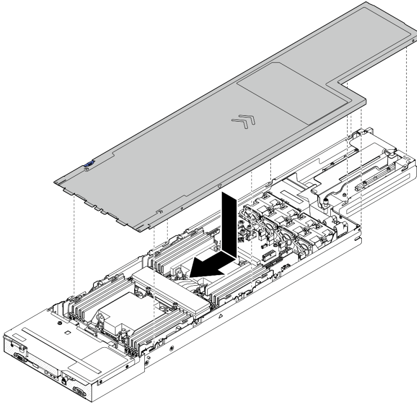
图 133. 安装顶盖
