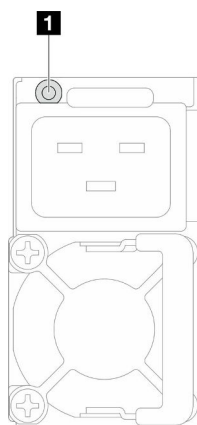
图 154. 电源模块 LED
