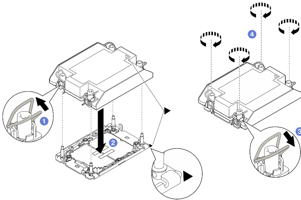
图 110. 为双处理器配置安装 1U 标准 PHM
