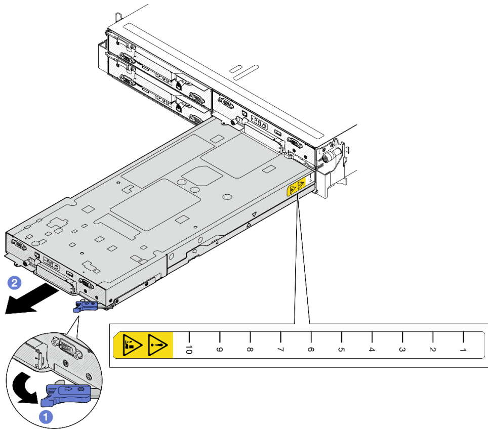
图 35. 将节点从右侧托盘卸下
