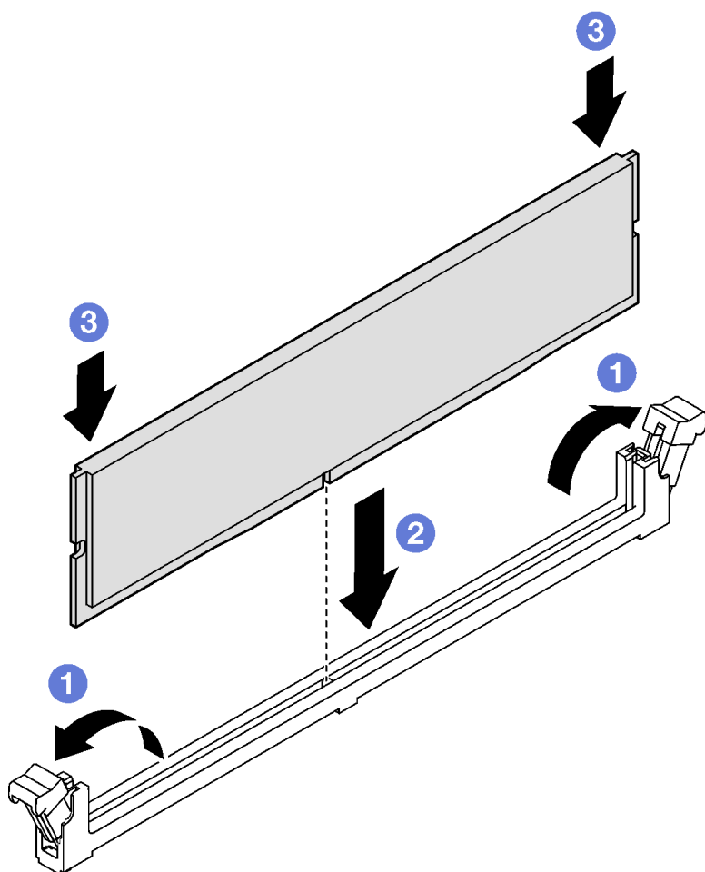
图 73. 安装内存条
