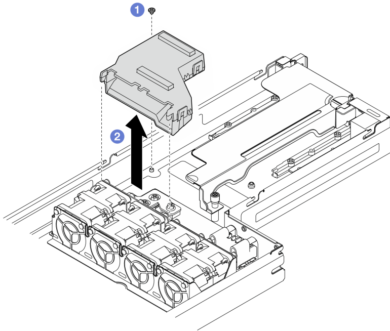
图 57. 卸下 GPU 导风管
