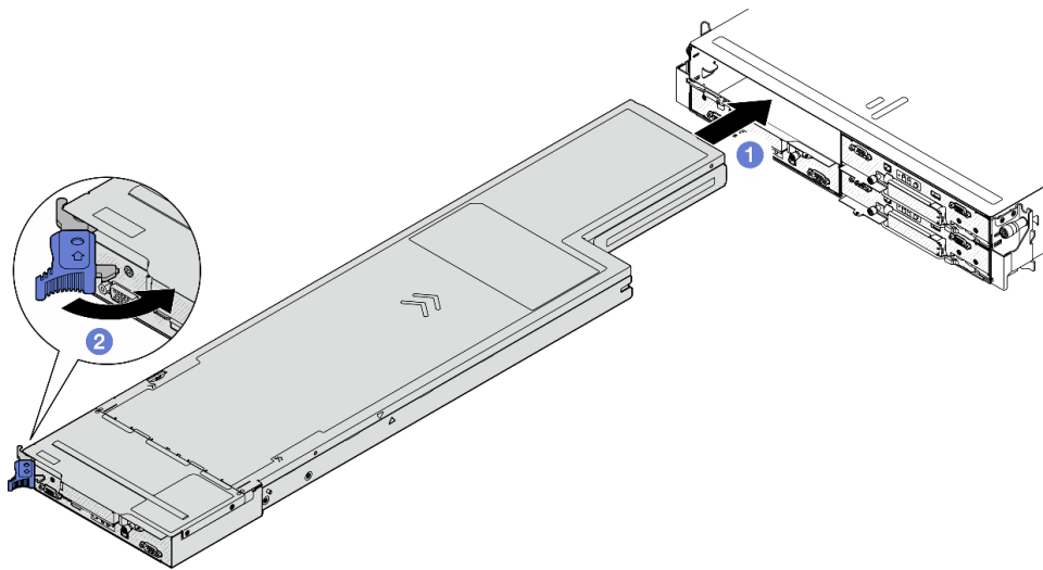
图 42. 将节点安装到左侧托盘
