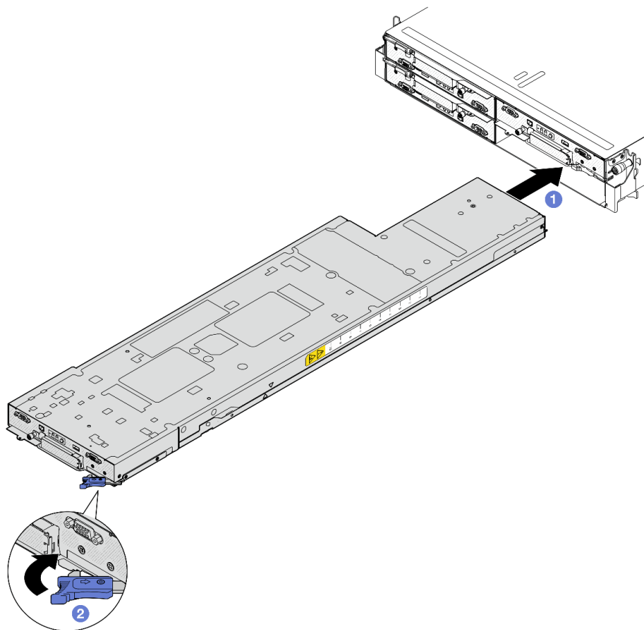
图 45. 将节点安装到右侧托盘
