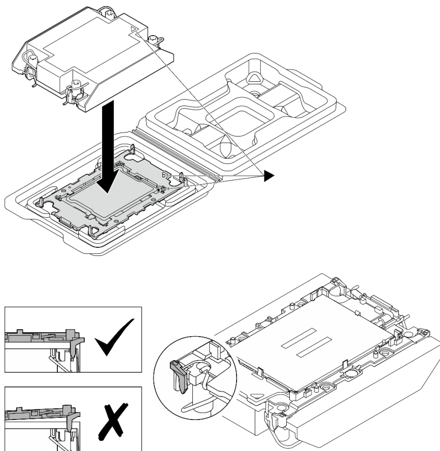
图 105. 在装运托盘中组装 PHM 和处理器
