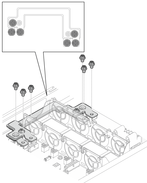
图 87. 卸下电源汇流条外侧螺钉
