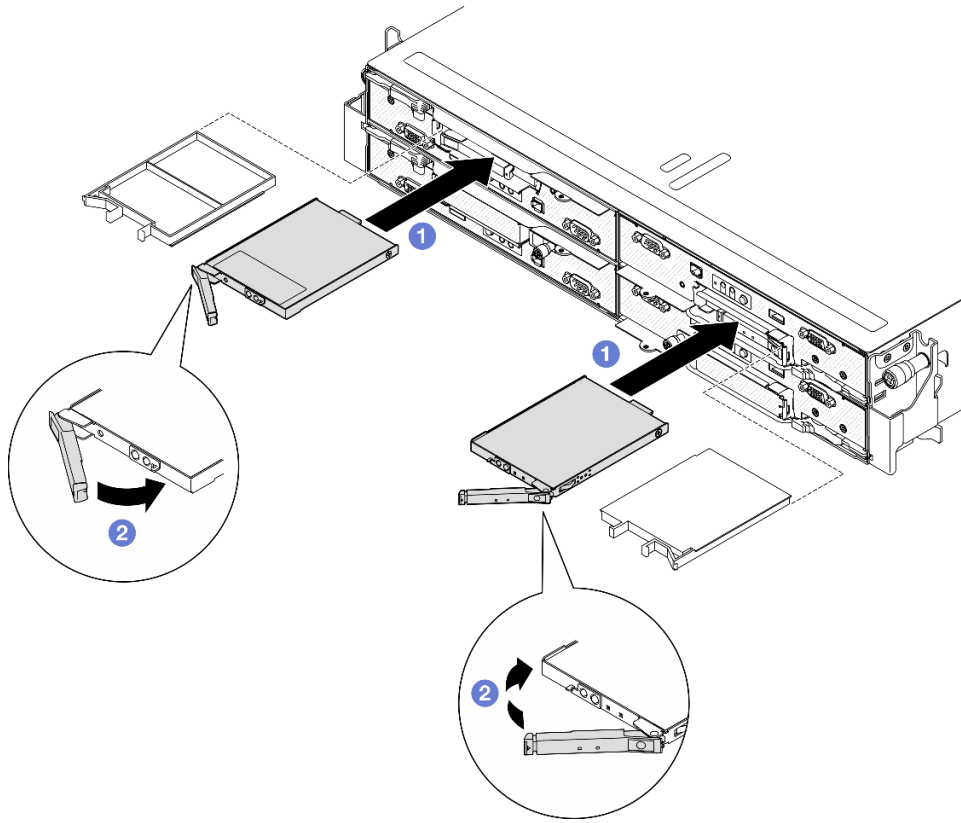
图 63. 安装 E3.S 热插拔硬盘
