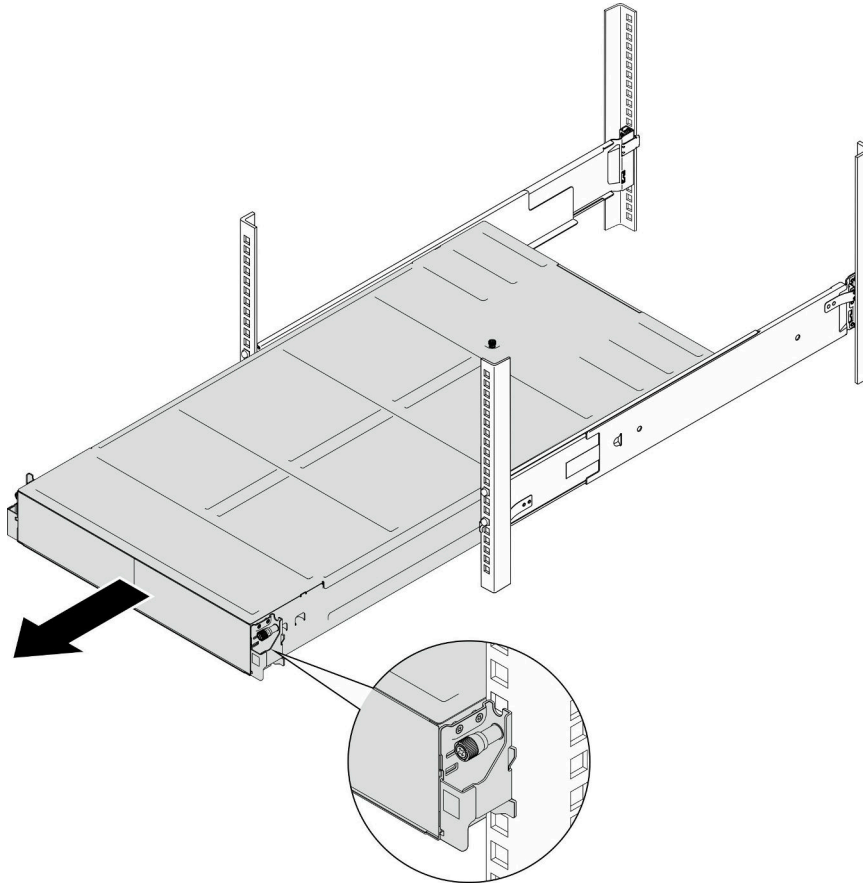
图 18. 卸下机箱
