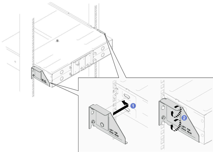
图 20. 安装装运支架
