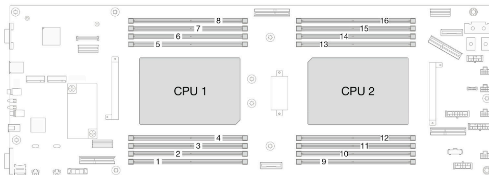
图 72. 内存条和处理器布局
