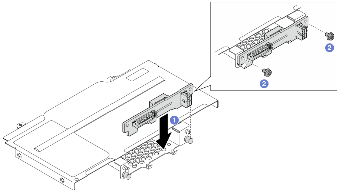
图 53. 安装硬盘背板
