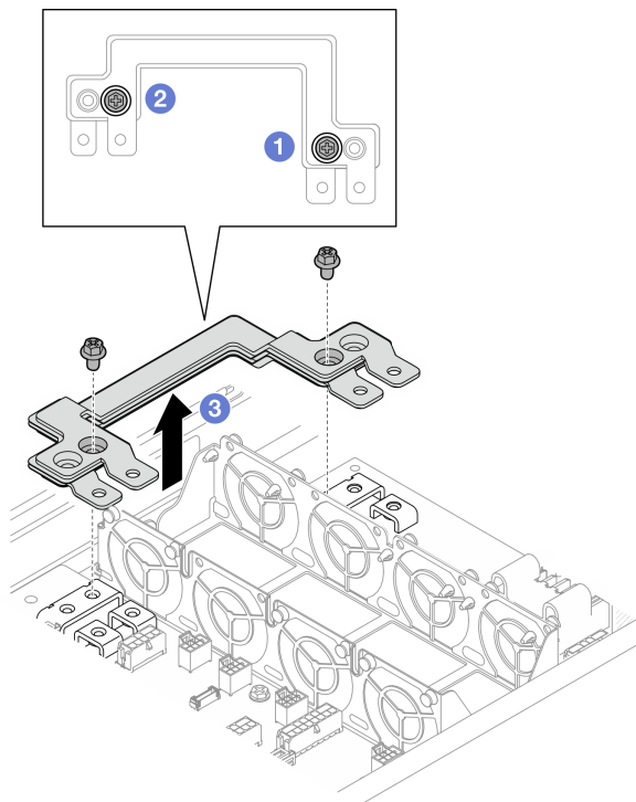
图 88. 卸下电源汇流条
