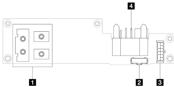
图 137. 配电板接口
