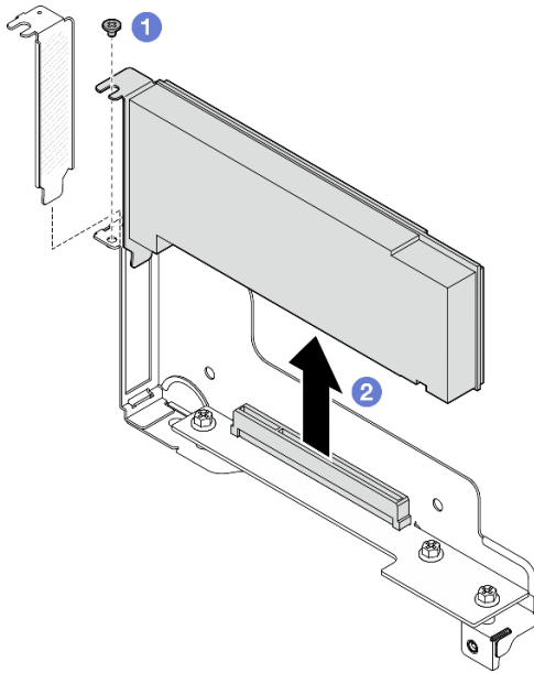
图 82. 卸下 PCIe 适配器
