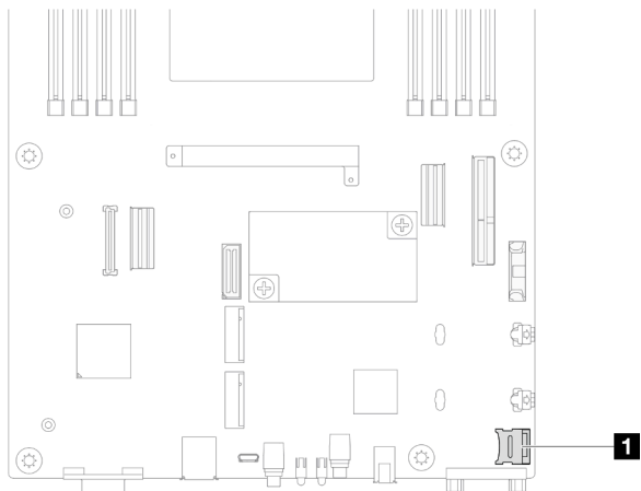
图 76. MicroSD 插槽位置
