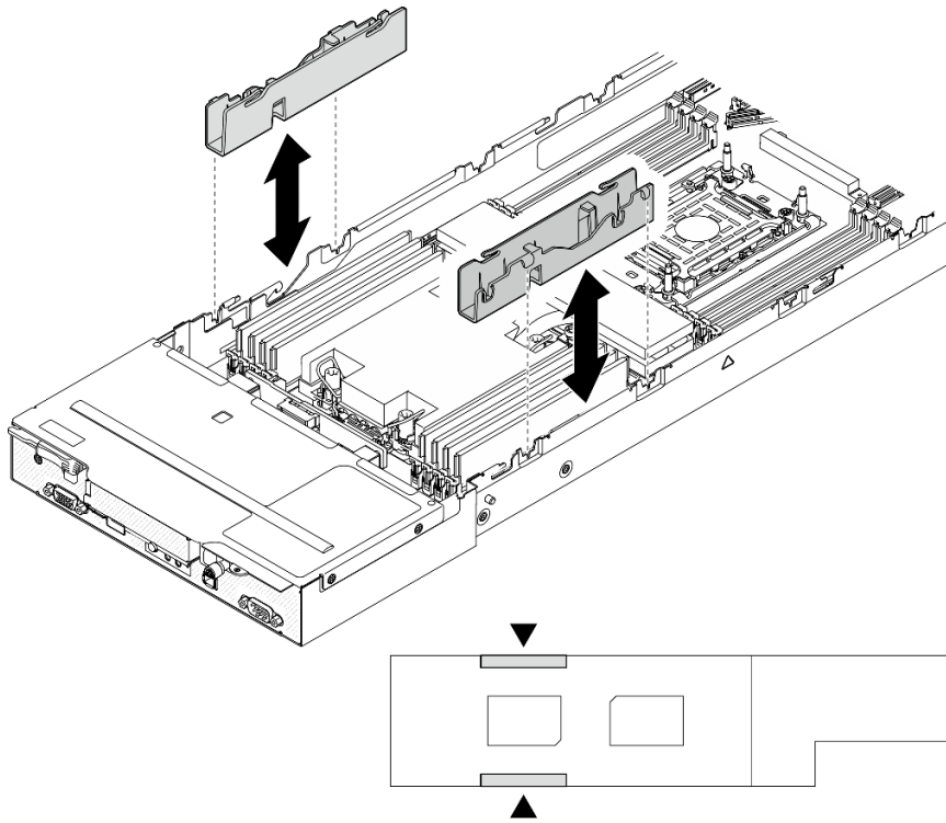
图 121. 更换线缆槽（单处理器配置）
