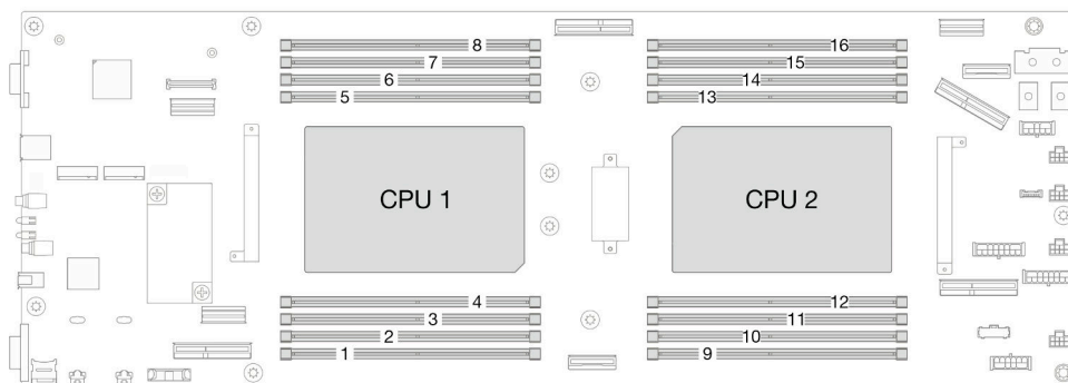
图 70. 内存条和处理器布局
