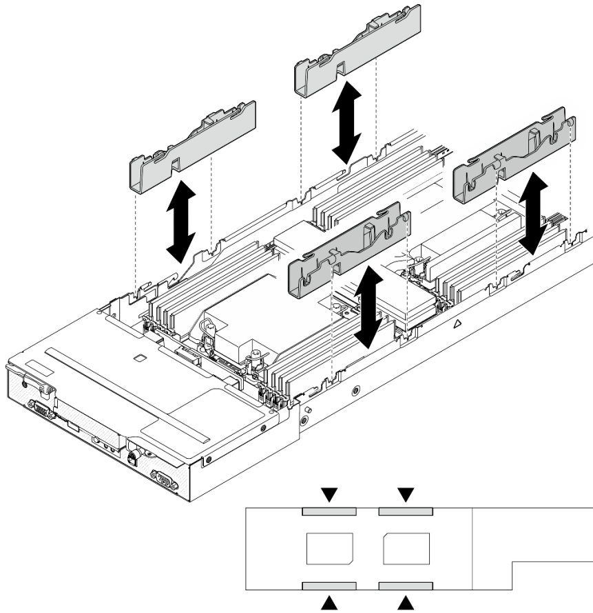
图 130. 更换线缆槽（双处理器配置）
