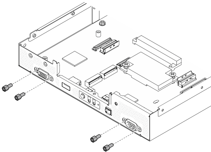
图 127. 安装正面的主板螺钉
