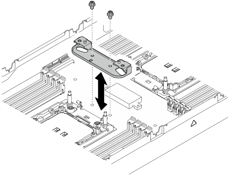
图 120. 更换散热器支撑架
