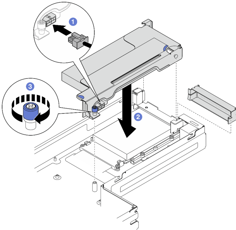
图 86. 安装 PCIe 转接卡组合件
