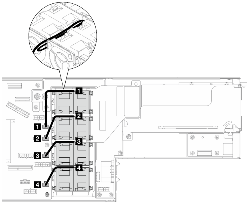
图 139. 风扇线缆布放
