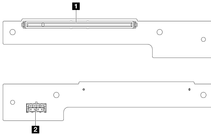
图 136. PCIe 转接卡接口
