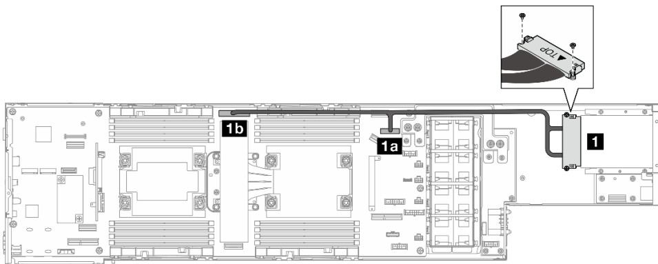
图 143. 背面 I/O 模块和 OCP 模块的线缆
