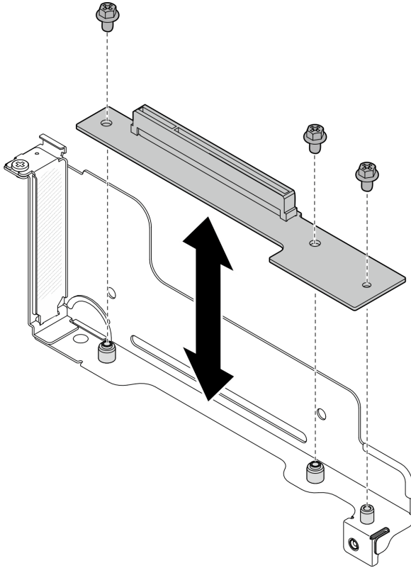
图 85. 更换 PCIe 转接卡
