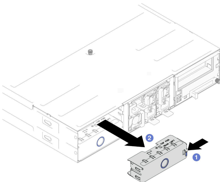
图 40. 卸下背面节点托盘填充件
