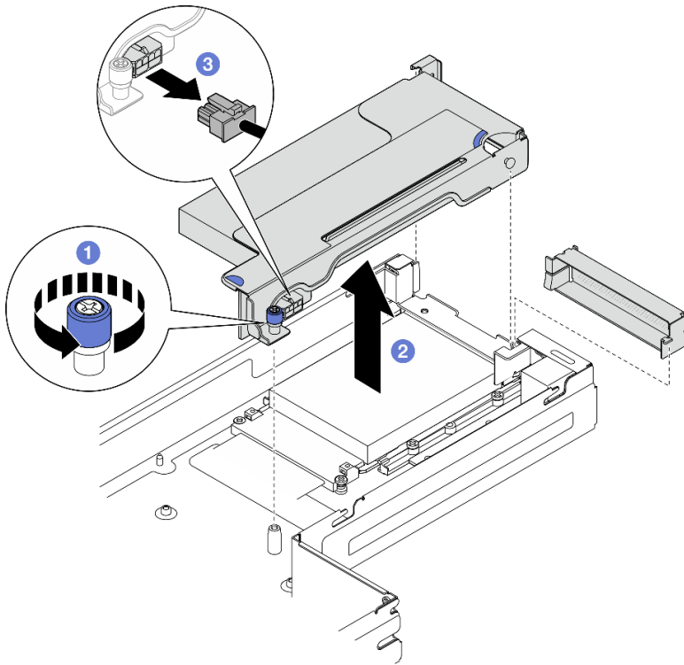
图 80. 卸下 PCIe 转接卡组合件
