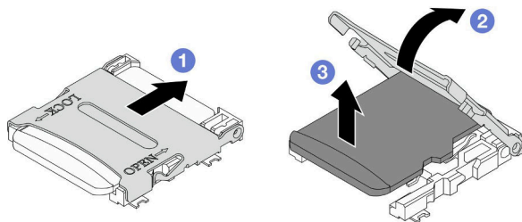
图 75. 卸下 MicroSD 卡
