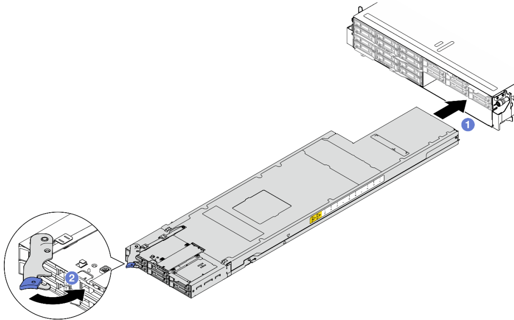
图 46. 将节点安装到右侧托盘
