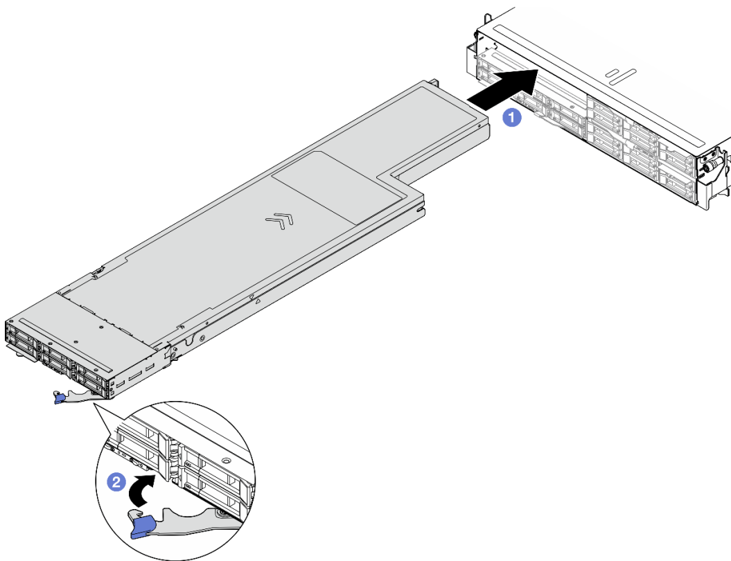
图 43. 将节点安装到左侧托盘
