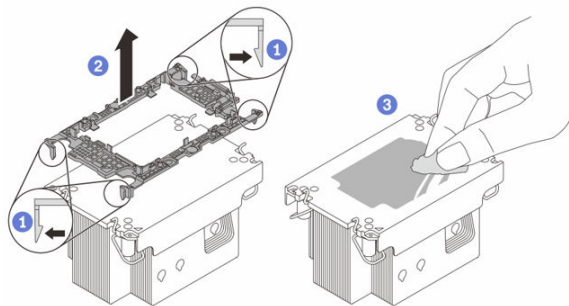
图 101. 将处理器支架与散热器分开
