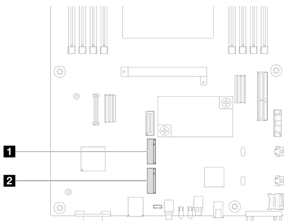
图 68. 主板上 M.2 插槽的位置
