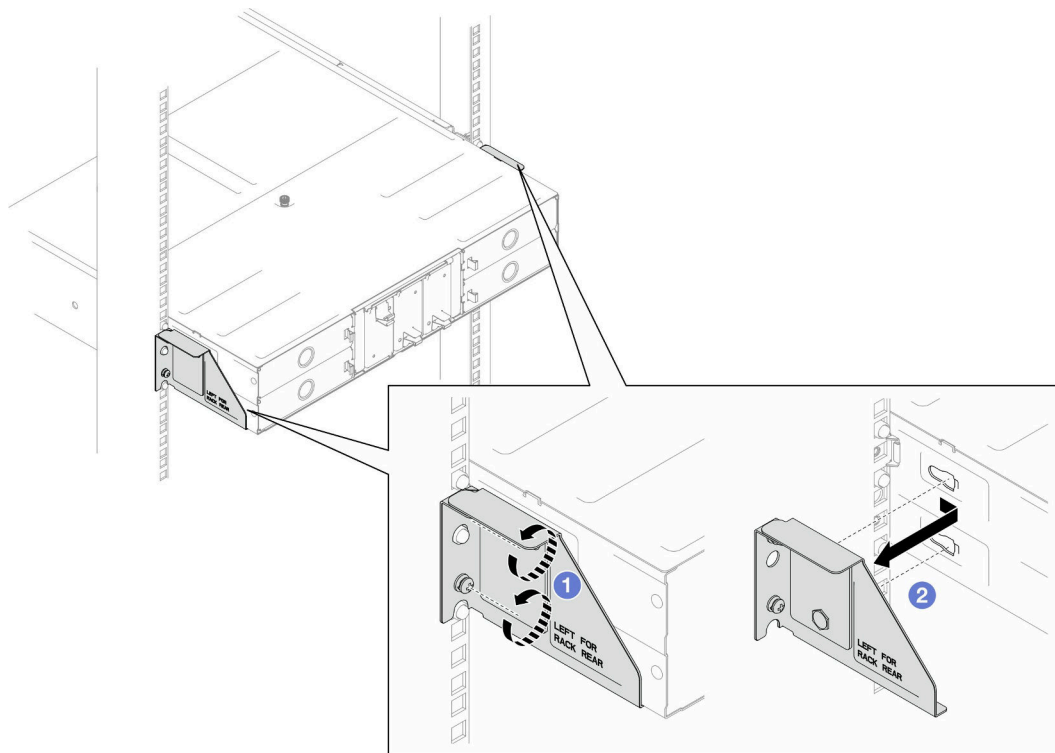
图 17. 卸下装运支架
