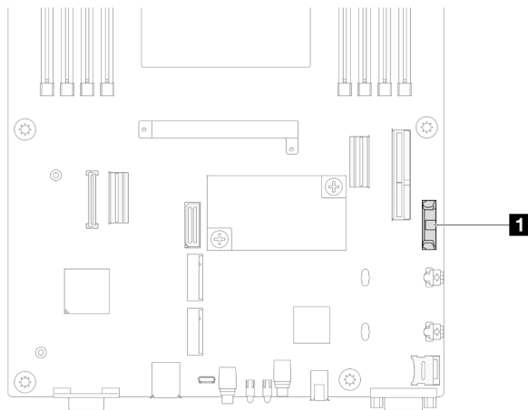
图 47. CMOS 电池插槽位置
