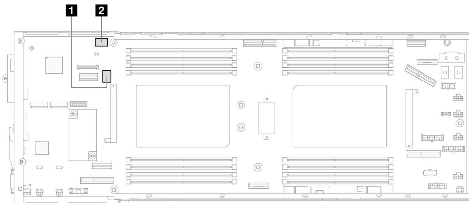
图 10. 主板开关
