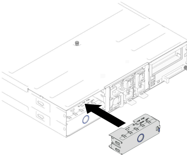
图 38. 安装背面节点托盘填充件
