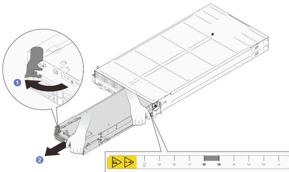
图 34. 将节点从右侧托盘卸下
