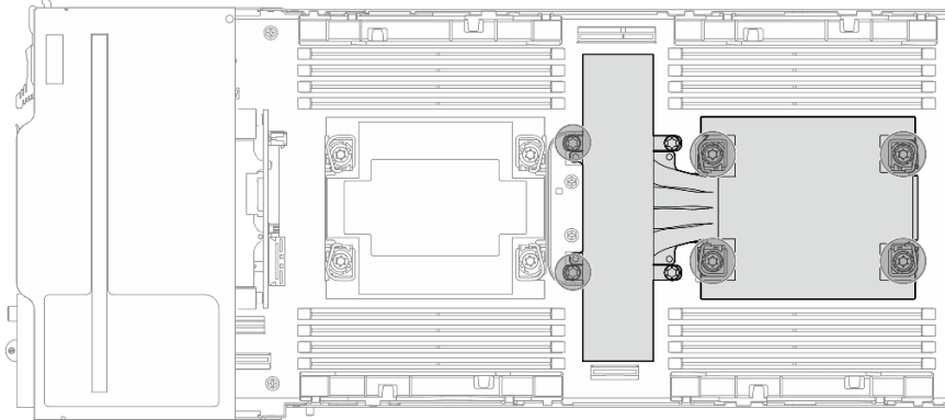
图 109. 双处理器配置的 PHM 位置
