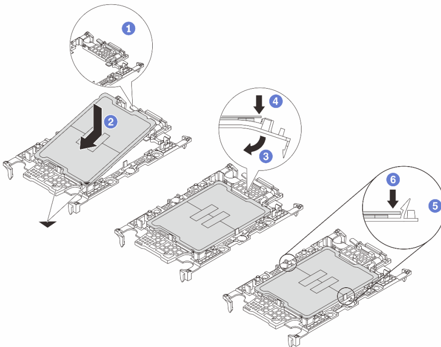
图 103. 安装处理器支架
