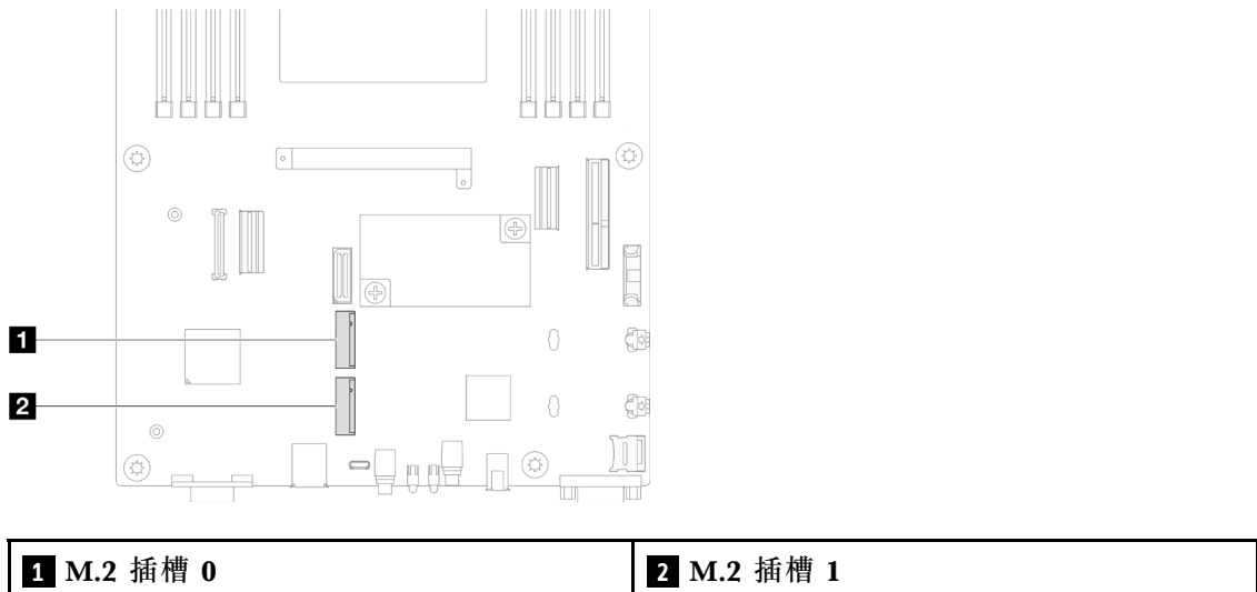
图 65. 主板上 M.2 插槽的位置
