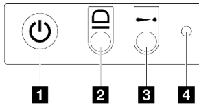
图 153. 正面操作员面板上的按钮和 LED
