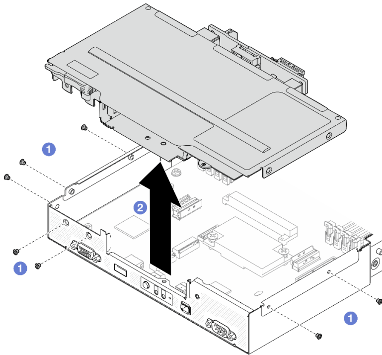
图 51. 卸下硬盘仓组合件
