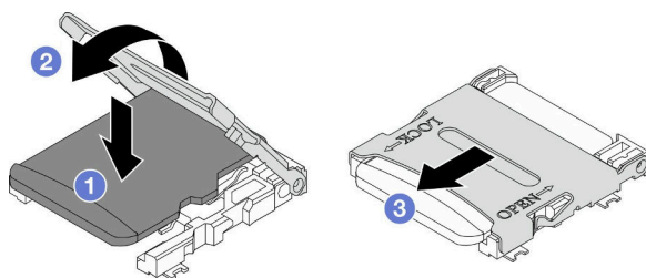
图 77. 安装 MicroSD 卡
