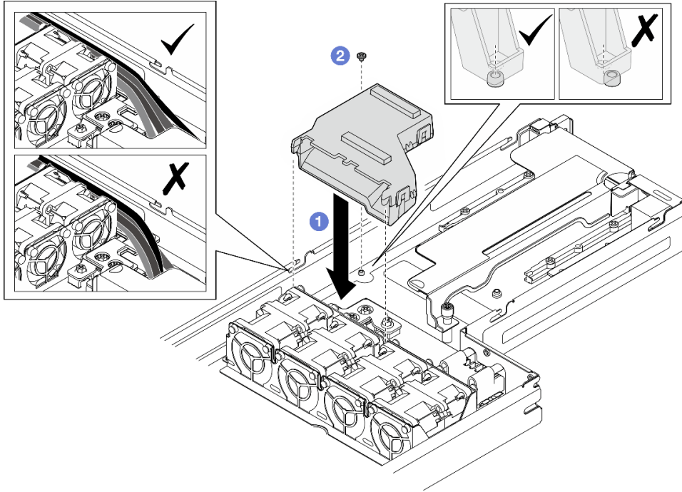
图 58. 安装 GPU 导风管
