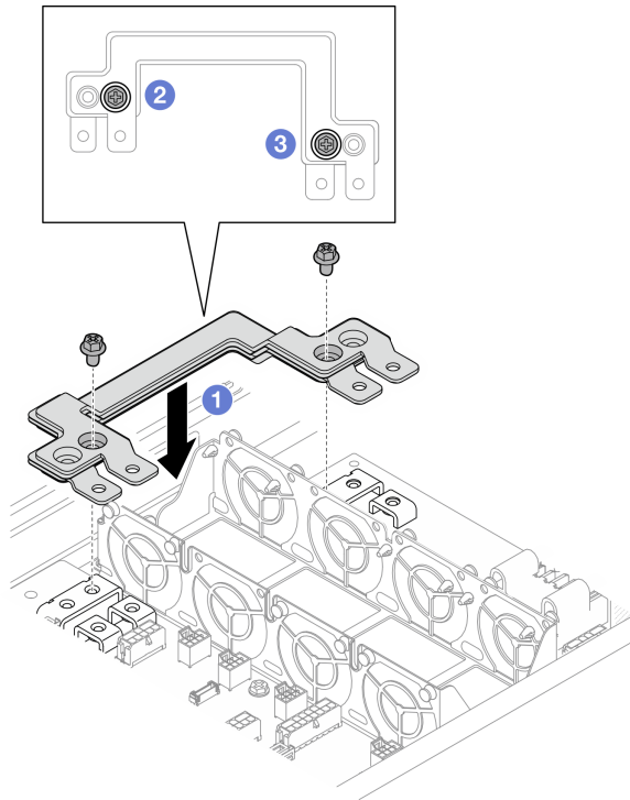
图 89. 安装电源汇流条
