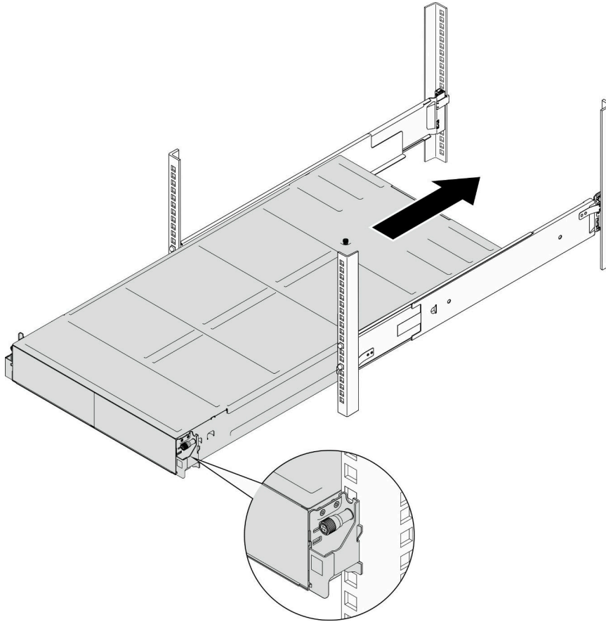
图 19. 安装机箱
