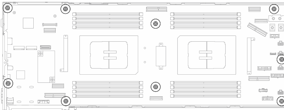
图 124. 卸下螺钉
