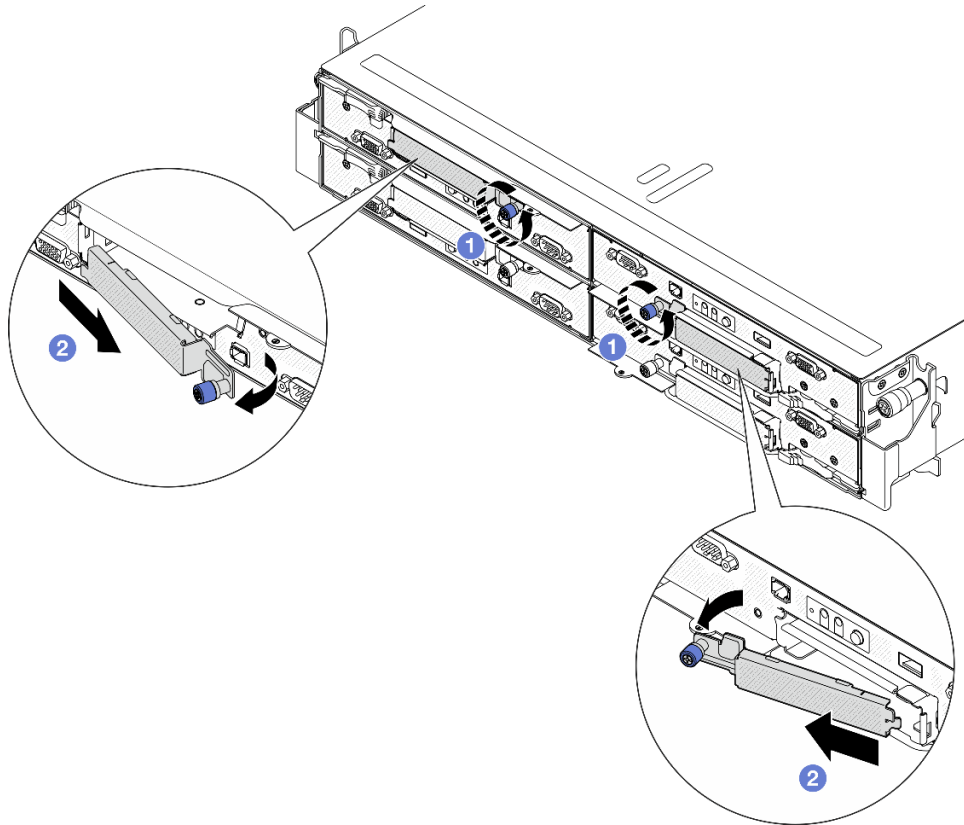
图 62. 卸下 E3.S 硬盘仓盖
