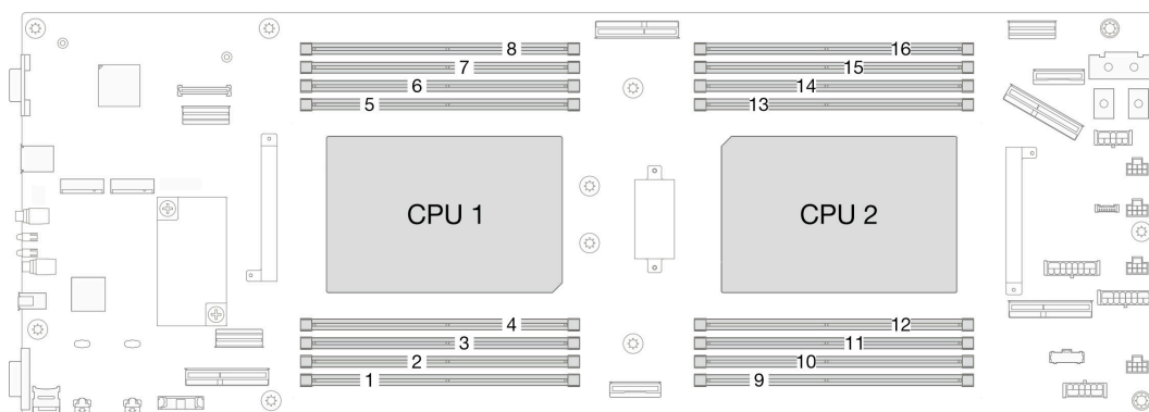
图 16. 内存条和处理器布局
