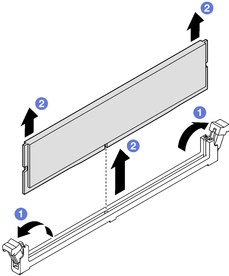
图 71. 卸下内存条
