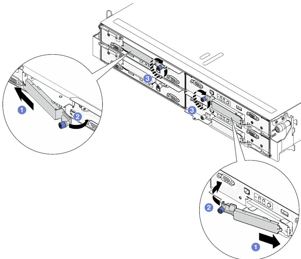
图 61. 安装 E3.S 硬盘仓盖
