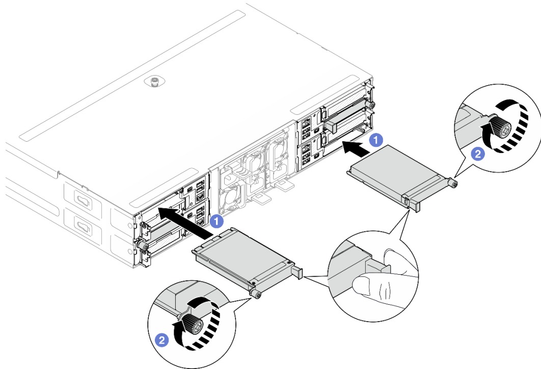
图 79. 安装背面 OCP 模块
