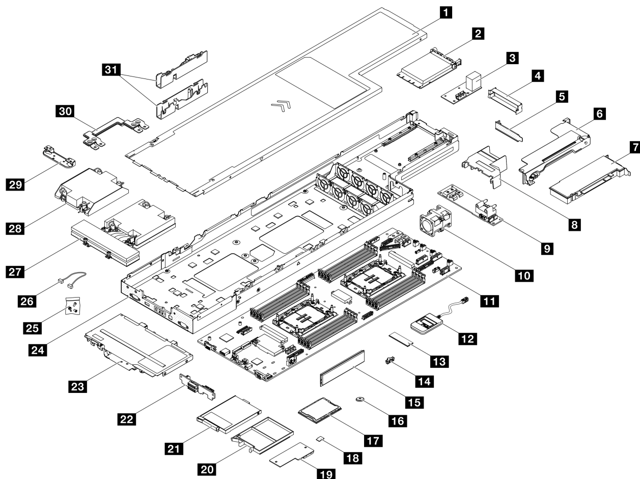
图 12. 节点组件
