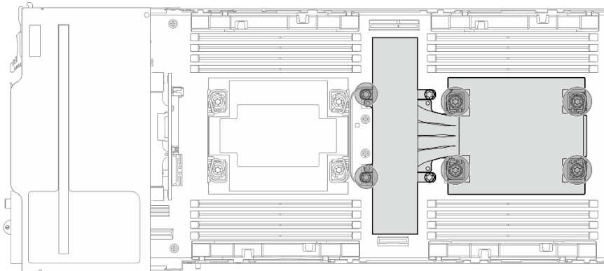
图 95. 双处理器配置的 PHM 位置
