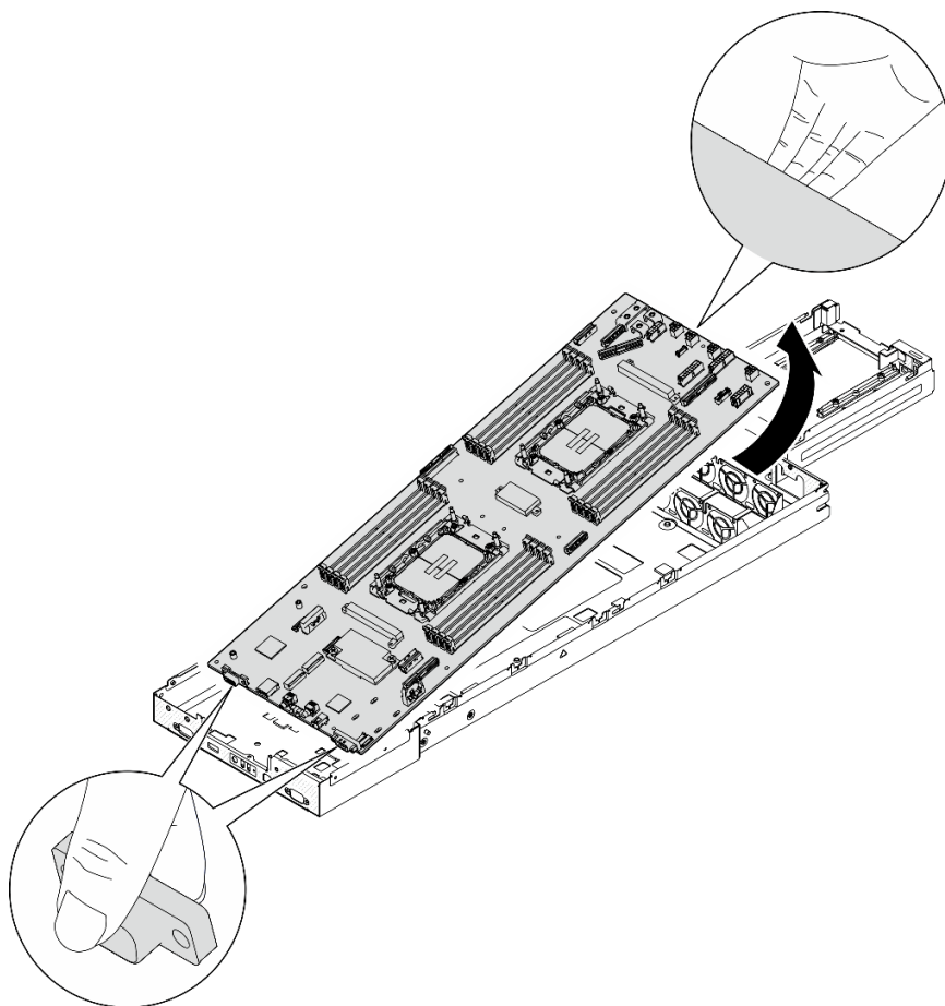
图 125. 卸下主板
