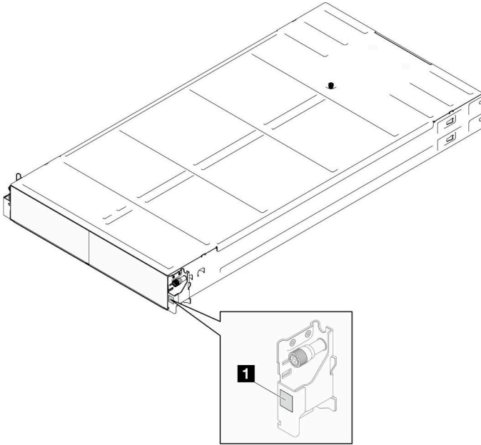
图 13. 机箱上的标识标签位置
