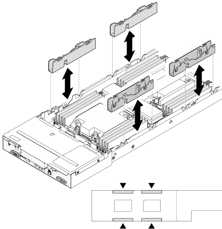
图 122. 更换线缆槽（双处理器配置）
