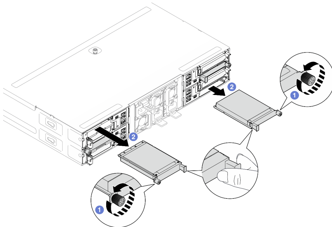
图 78. 卸下背面 OCP 模块
