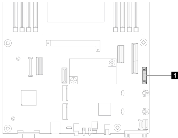
图 49. CMOS 电池插槽位置
