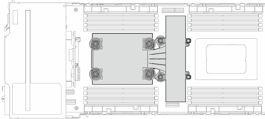
图 94. 单处理器配置的 PHM 位置
