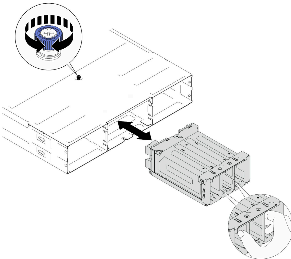
图 27. 卸下 PSU 仓
