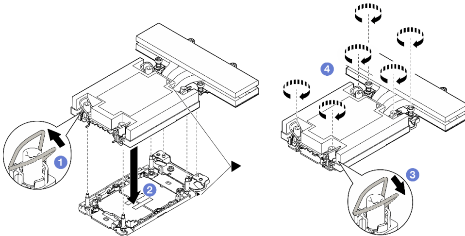
图 108. 为单处理器配置安装 1U 高性能 PHM
