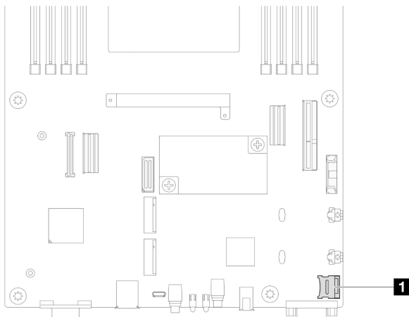
图 74. MicroSD 插槽位置
