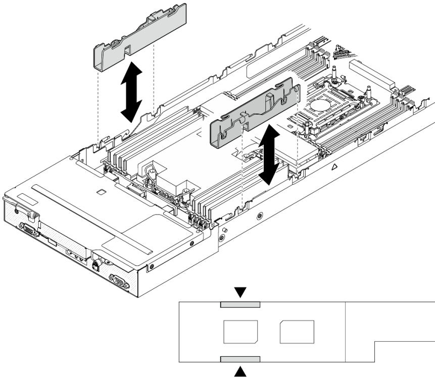
图 129. 更换线缆槽（单处理器配置）
