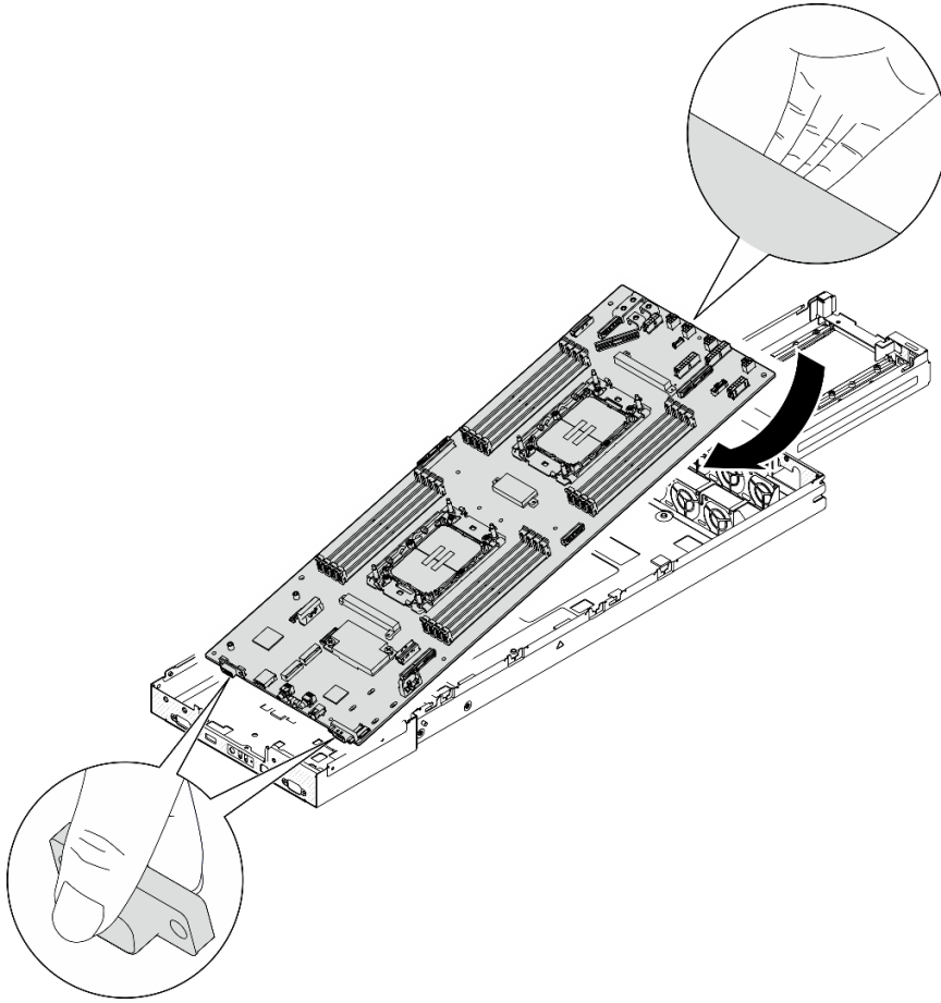
图 126. 安装主板
