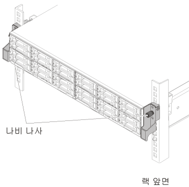
그림 12. 나비 나사
