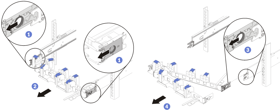
그림 11. 내부 마운팅 클립
