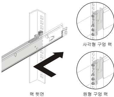
그림 3. 왼쪽 슬라이드 뒷면 설치
