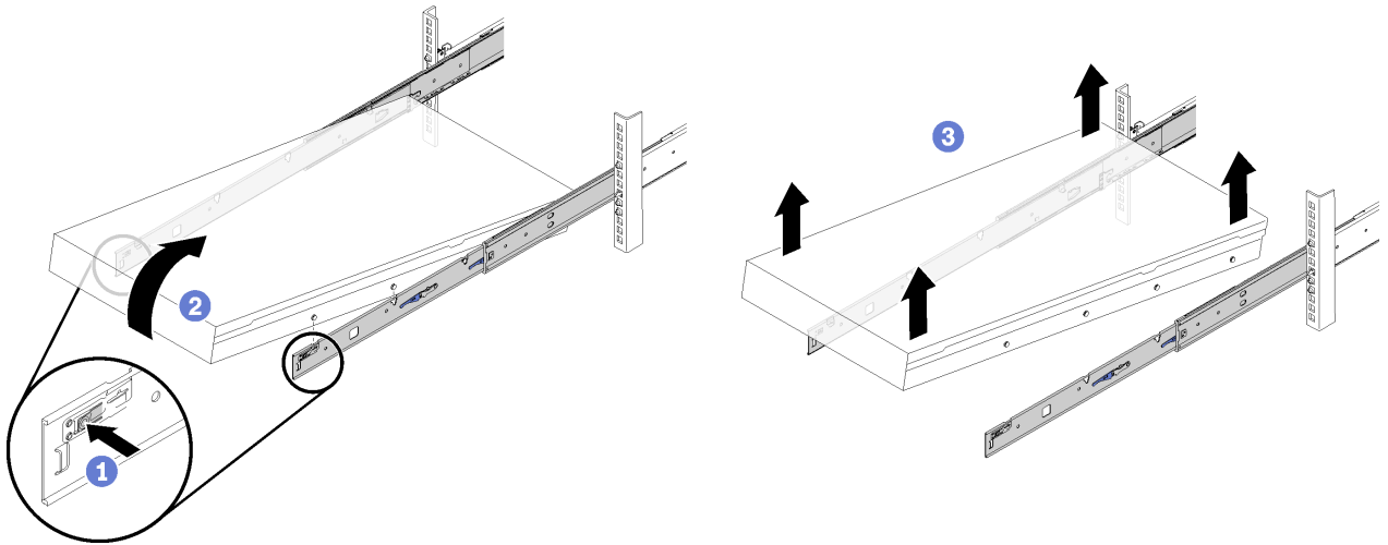
그림 14. 엔클로저 제거
