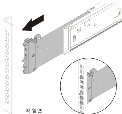
그림 4. 왼쪽 슬라이드 앞면 설치
