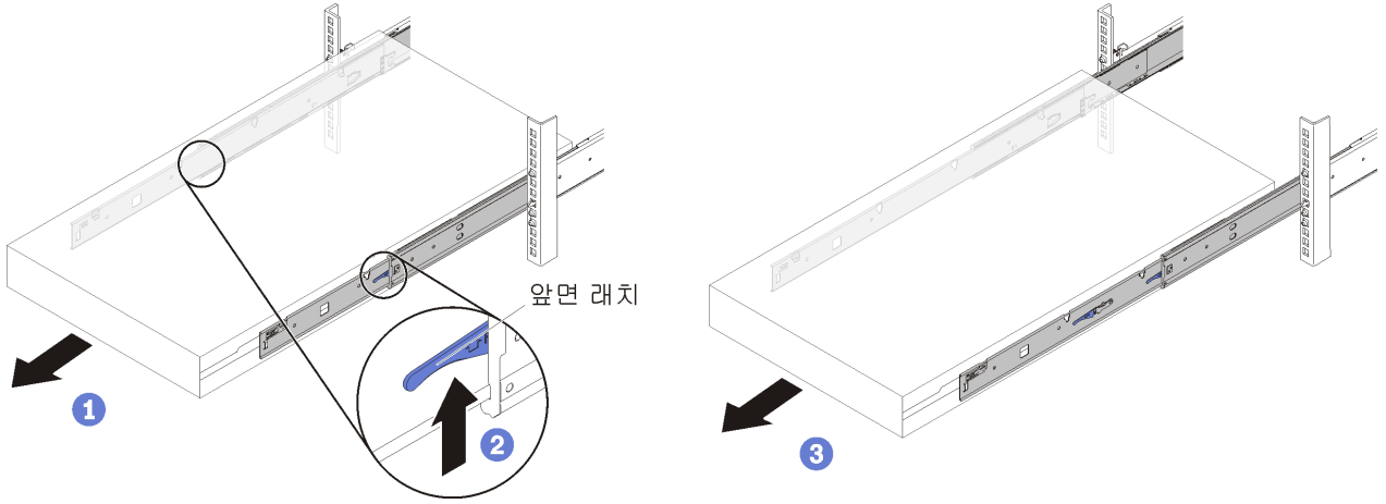
그림 13. 엔클로저 제거
