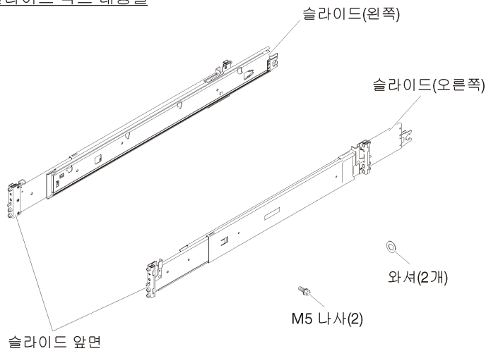
그림 1. 슬라이드 박스 내용물
