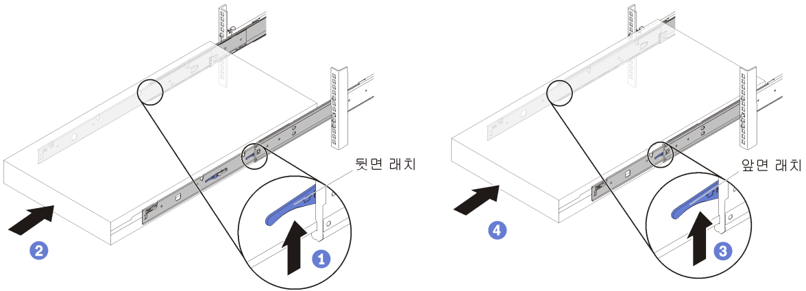
그림 8. 엔클로저 설치
