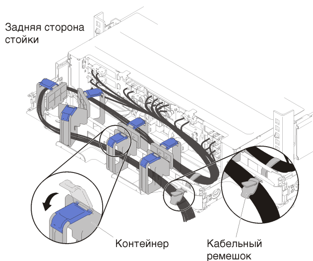
Рис. 3. Прокладка кабелей
