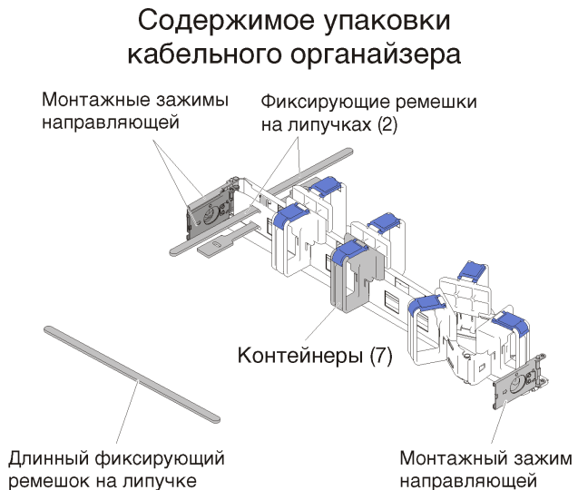
Рис. 1. Содержимое упаковки кабельного органайзера
