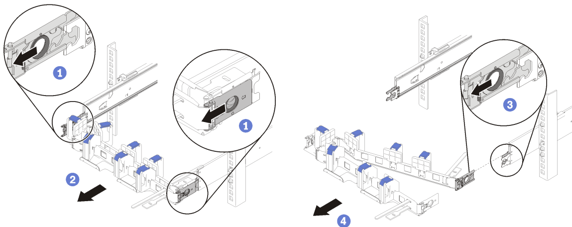
Рис. 4. Снятие кабельного органайзера
