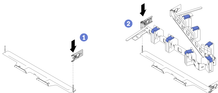
Рис. 6. Установка монтажного зажима
