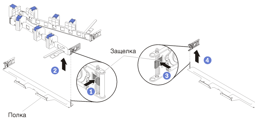
Рис. 5. Снятие монтажного зажима
