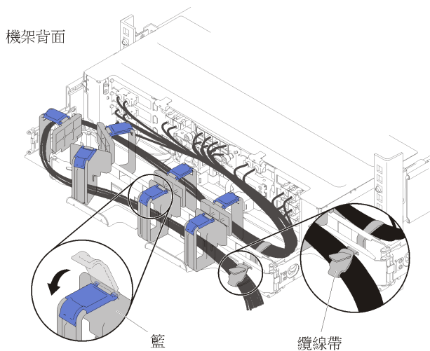
圖例 3. 纜線佈線
