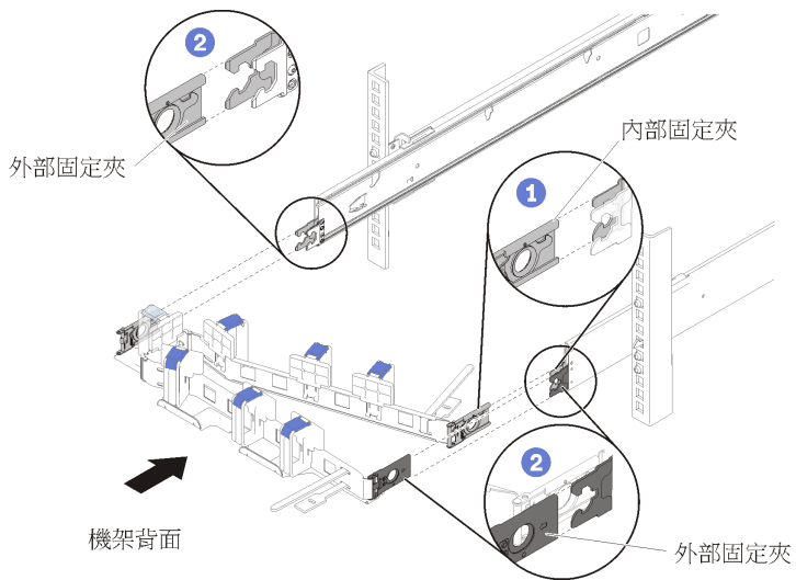
圖例 2. 纜線整理臂安裝
