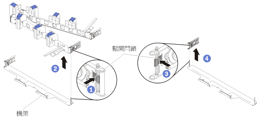
圖例 5. 卸下固定夾
