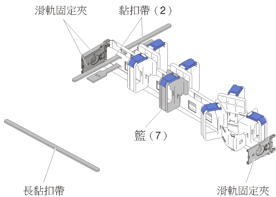
圖例 1. 纜線整理臂包裝內容物
