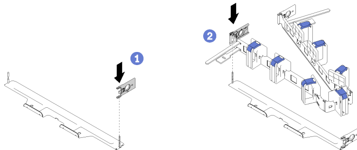
圖例 6. 安裝固定夾
