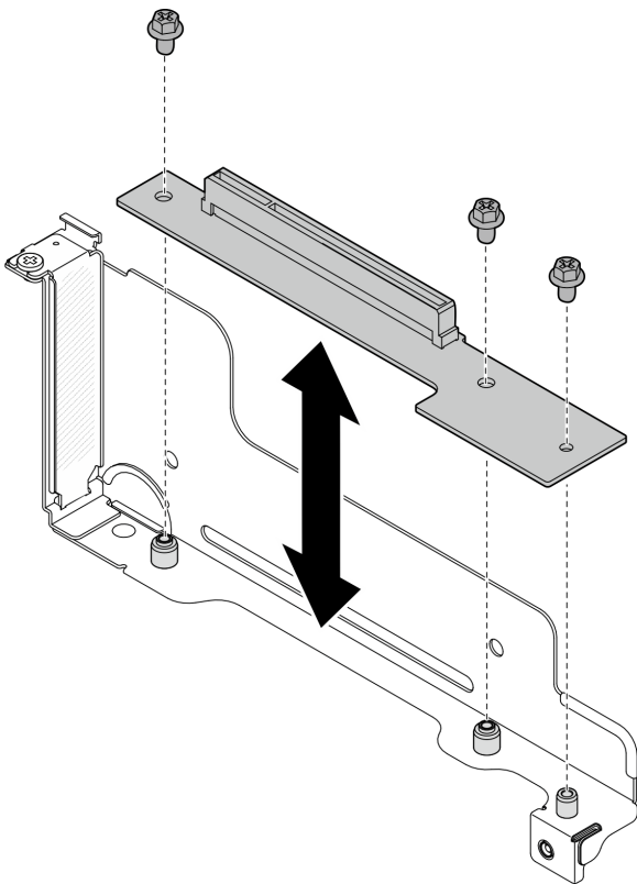
Abbildung 93. Austausch der PCIe-Adapterkarte
