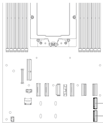
Abbildung 62. Positionen der M.2-Steckplätze auf der Systemplatine
