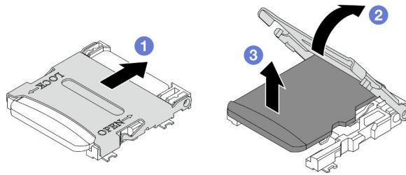
Abbildung 87. Entfernen der microSD-Karte
