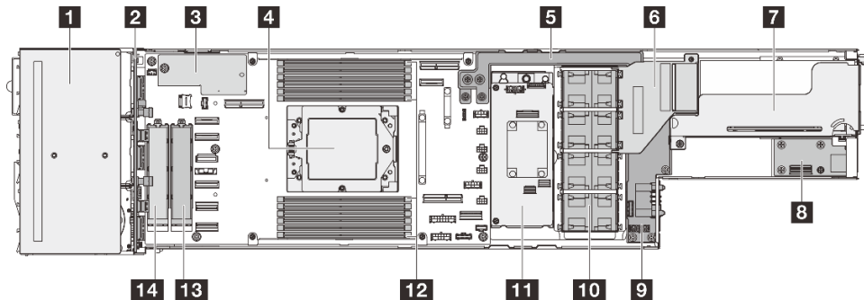
Abbildung 7. Ansicht von oben beim SD535 V3
