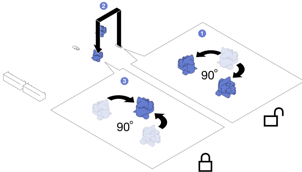
Abbildung 74. Anpassung einer M.2-Laufwerkhalterung
