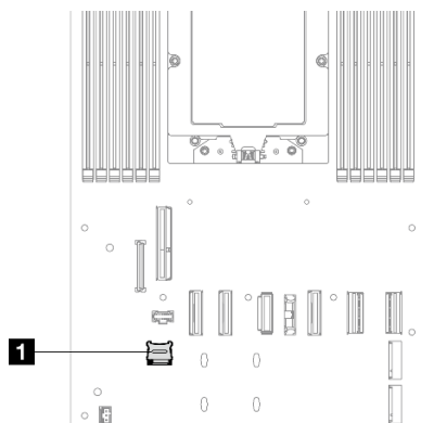
Abbildung 88. Position des microSD-Steckplatzes
