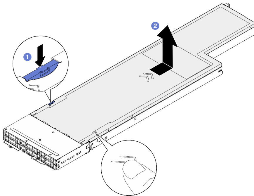
Abbildung 126. Entfernen der oberen Abdeckung
