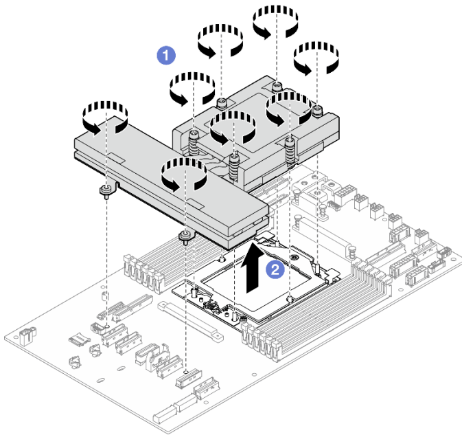
Abbildung 106. Entfernen eines Kühlkörpers
