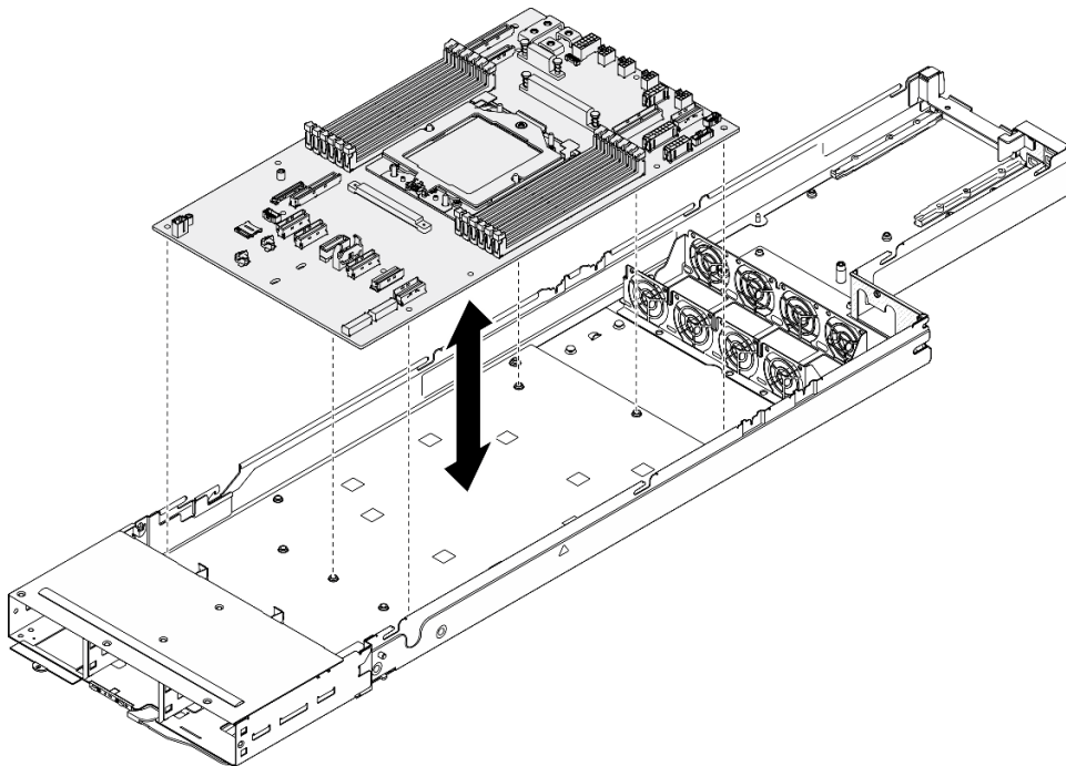
Abbildung 122. Entfernen der Systemplatine
