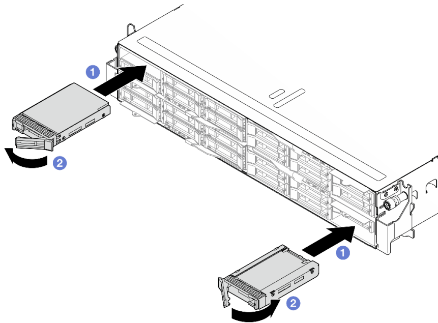
Abbildung 61. Installation eines Solid-State-Laufwerks
