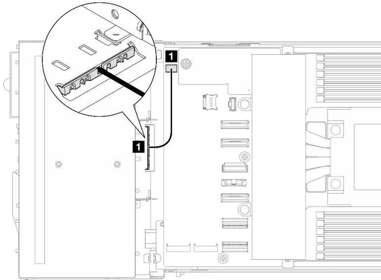
Abbildung 148. Kabelführung für den Temperatursensor an der Vorderseite
