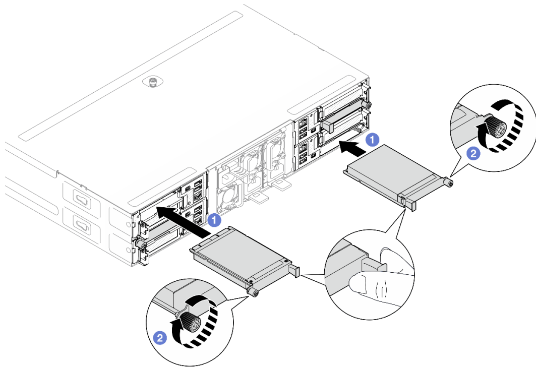
Abbildung 91. Installation des hinteren OCP-Moduls
