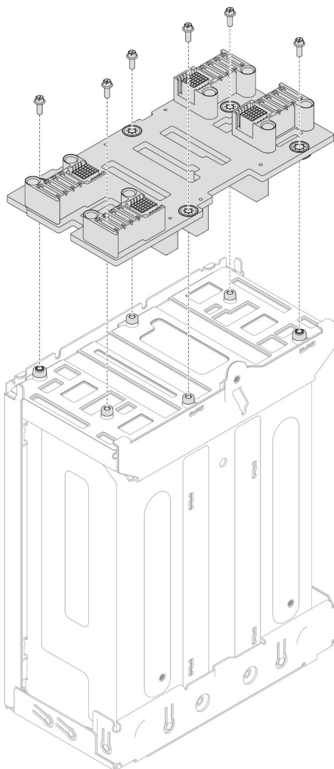
Abbildung 28. Installation der Gehäusemittelplatte
