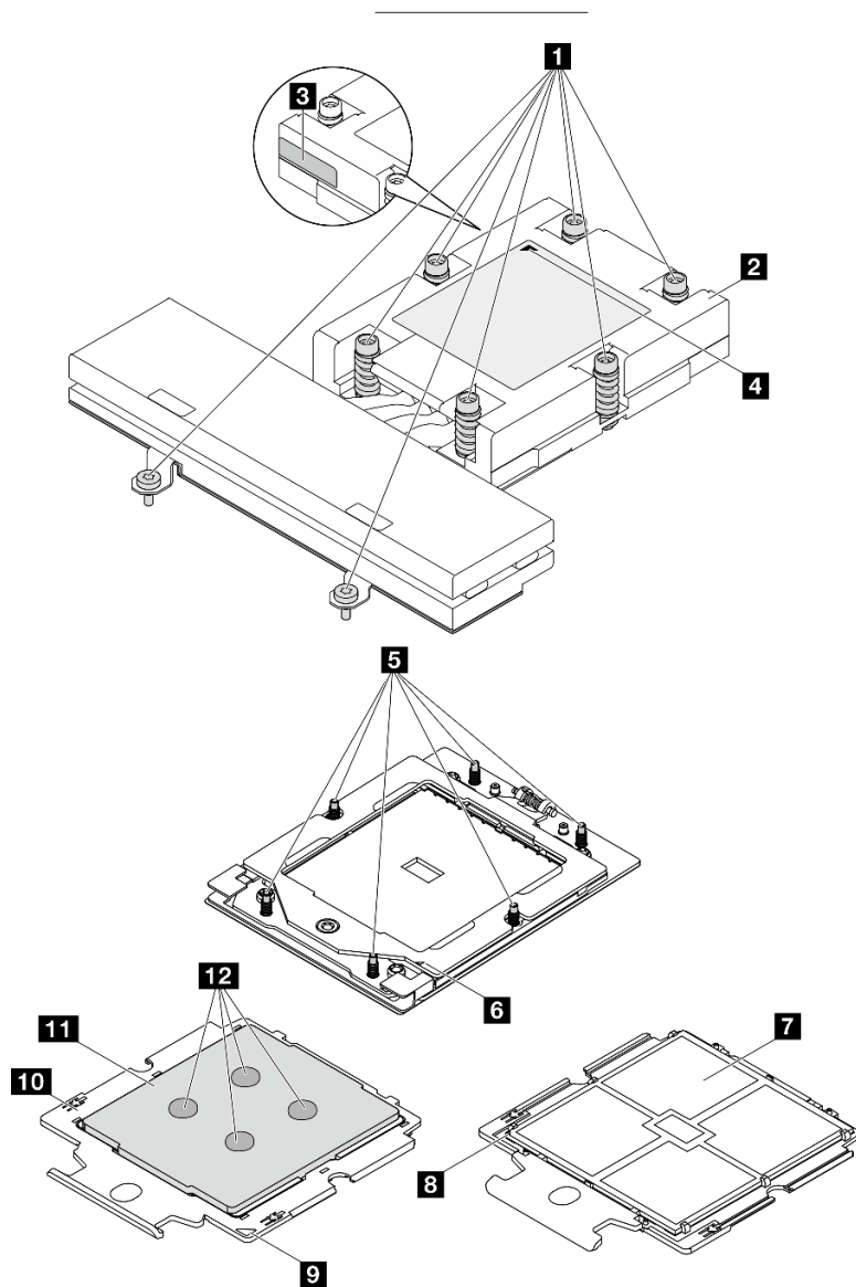
Abbildung 105. Prozessor- und Kühlkörperkomponenten
