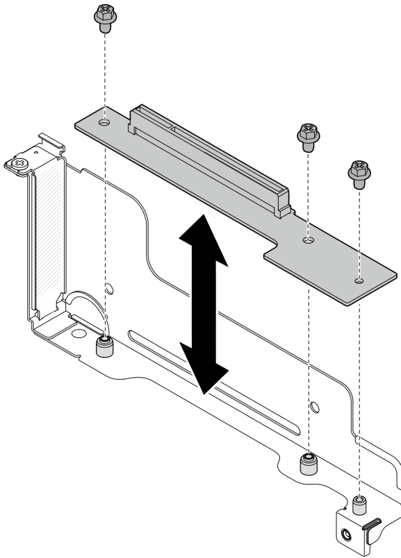
Abbildung 95. Austausch der PCIe-Adapterkarte
