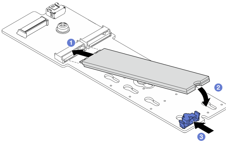
Abbildung 81. Installation eines M.2-Laufwerks
