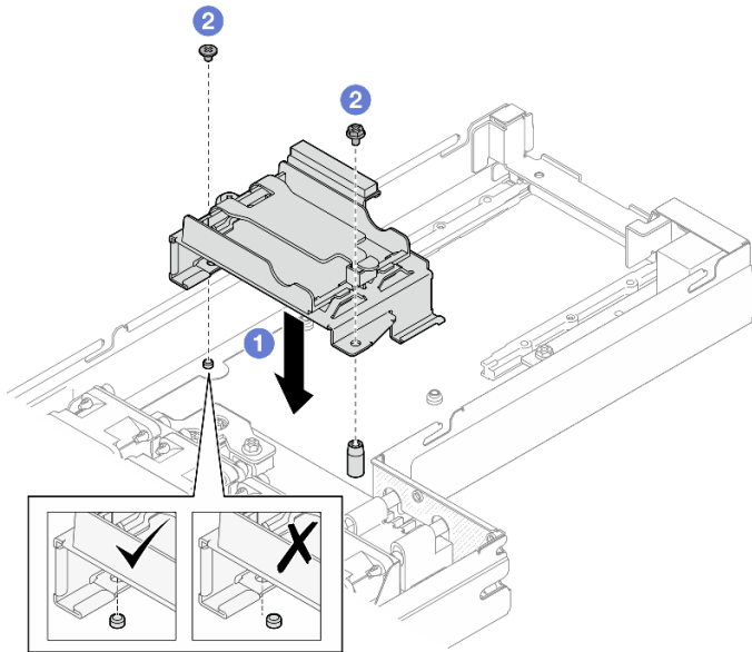
Abbildung 50. Installation der Halterung für das Flash-Stromversorgungsmodul
