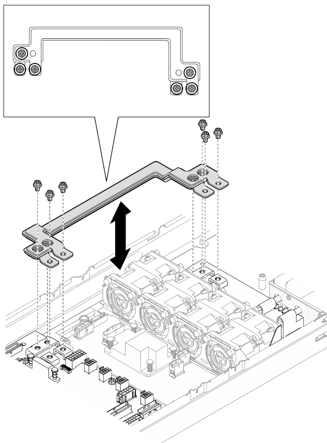
Abbildung 99. Entfernen der äußeren Schrauben der Sammelschiene
