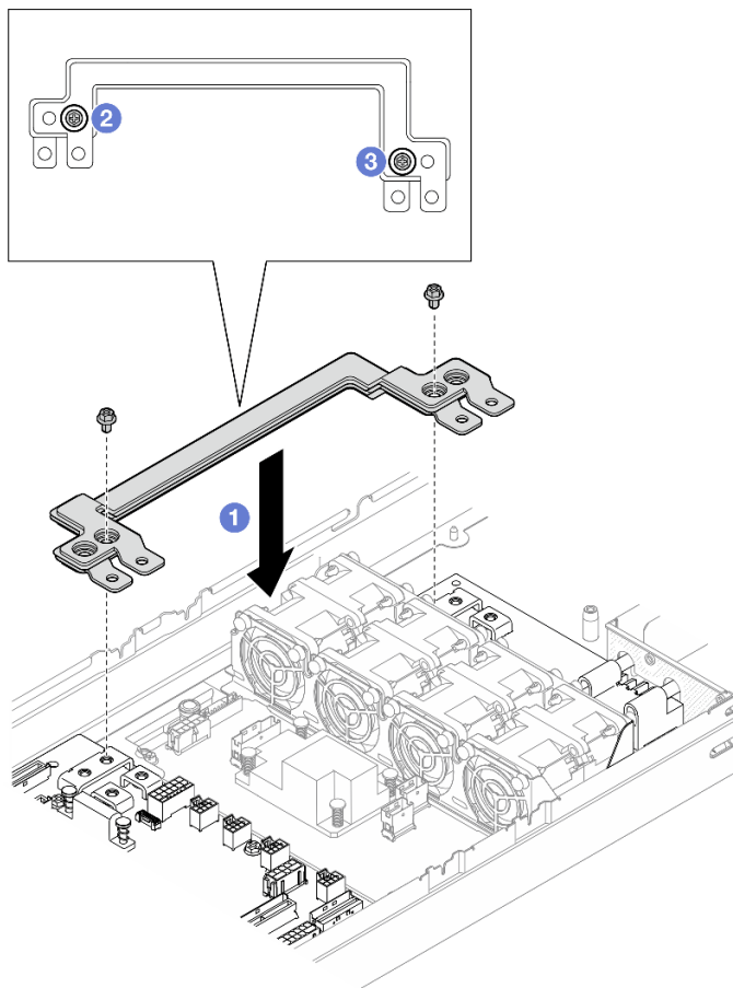
Abbildung 101. Installation der Sammelschiene
