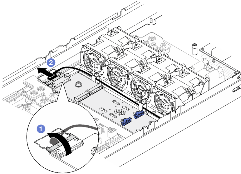
Abbildung 67. Abziehen des Kabels vom SATA/NVMe M.2-Bootadapter
