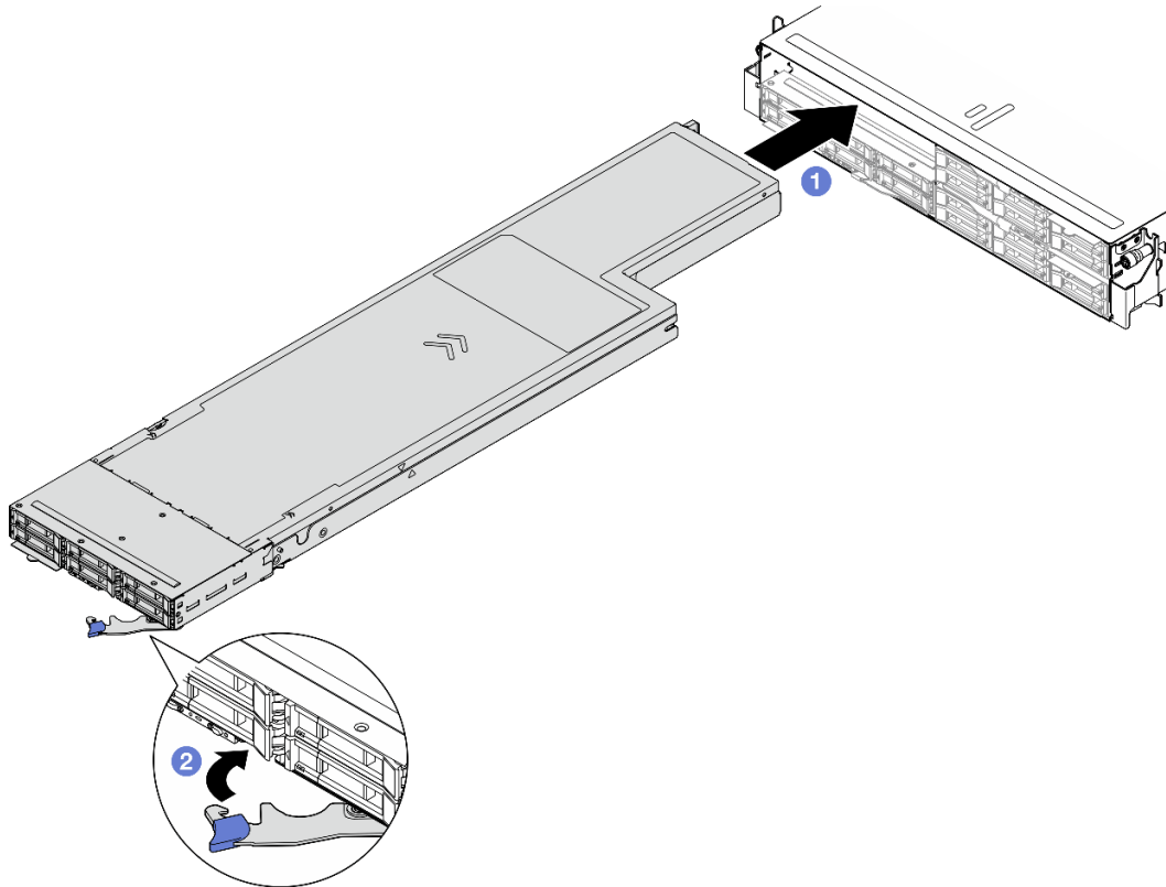
Abbildung 36. Knoteninstallation in einem linken Rahmen
