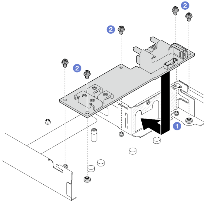
Abbildung 104. Installation einer Stromversorgungsplatine
