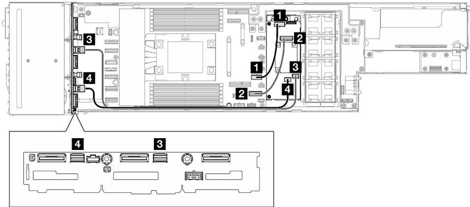
Abbildung 137. CFF RAID-Kabelführung
