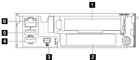
Abbildung 4. Rückansicht
