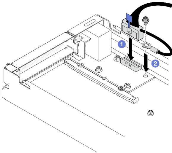
Abbildung 147. Installation des hinteren E/A-Kabels und des Erdungskabels
