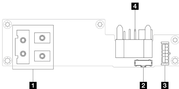
Abbildung 133. Anschlüsse für Stromversorgungsplatine
