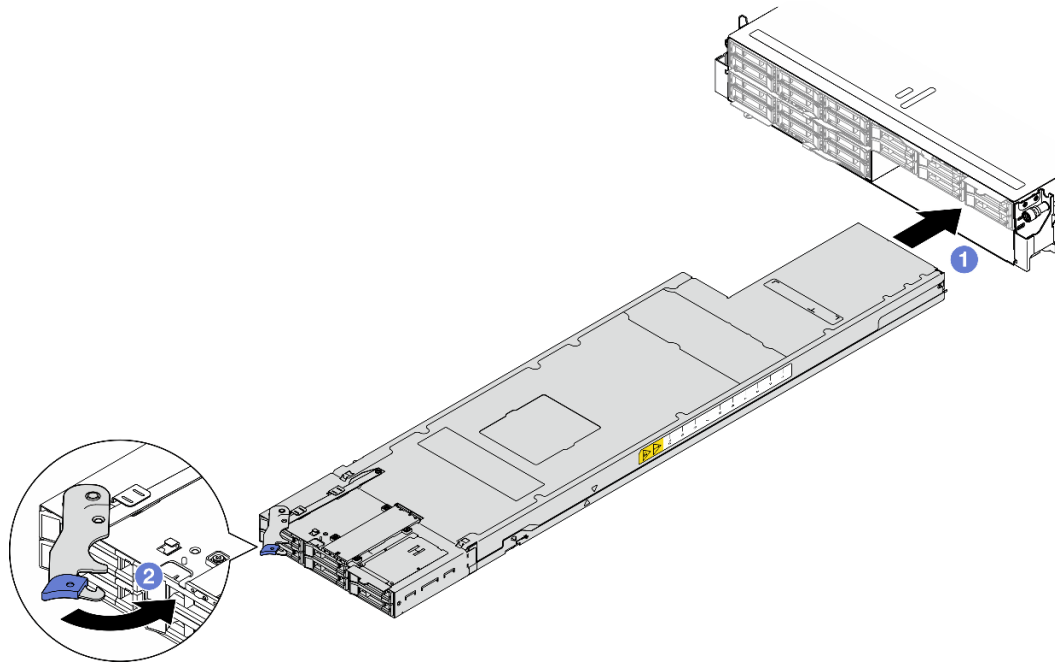
Abbildung 37. Knoteninstallation in einem rechten Rahmen
