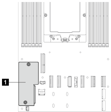
Abbildung 116. Position des Firmware- und RoT-Sicherheitsmodul
