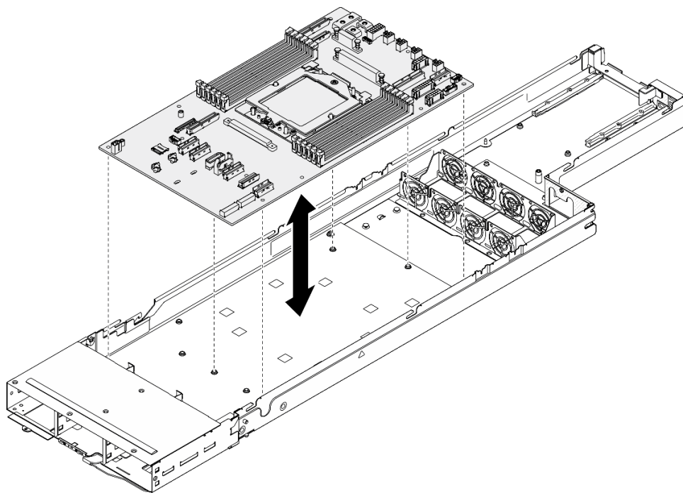
Abbildung 123. Installation der Systemplatine
