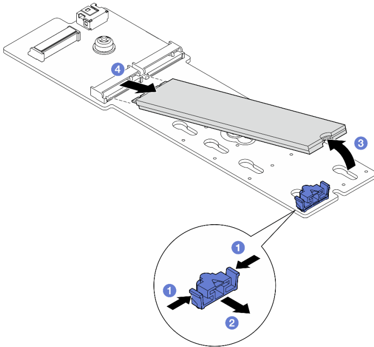
Abbildung 65. Entfernen eines M.2-Laufwerks
