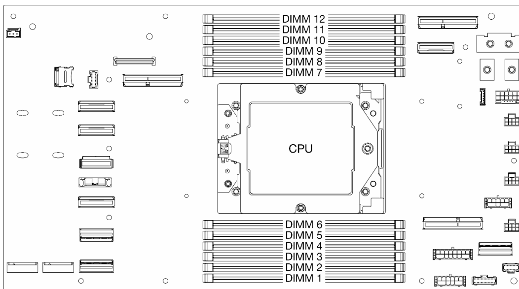
Abbildung 84. Layout für Speichermodule und Prozessoren
