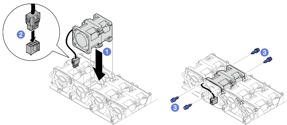
Abbildung 47. Lüftereinbau
