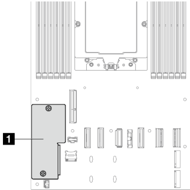
Abbildung 118. Position des Firmware- und RoT-Sicherheitsmodul
