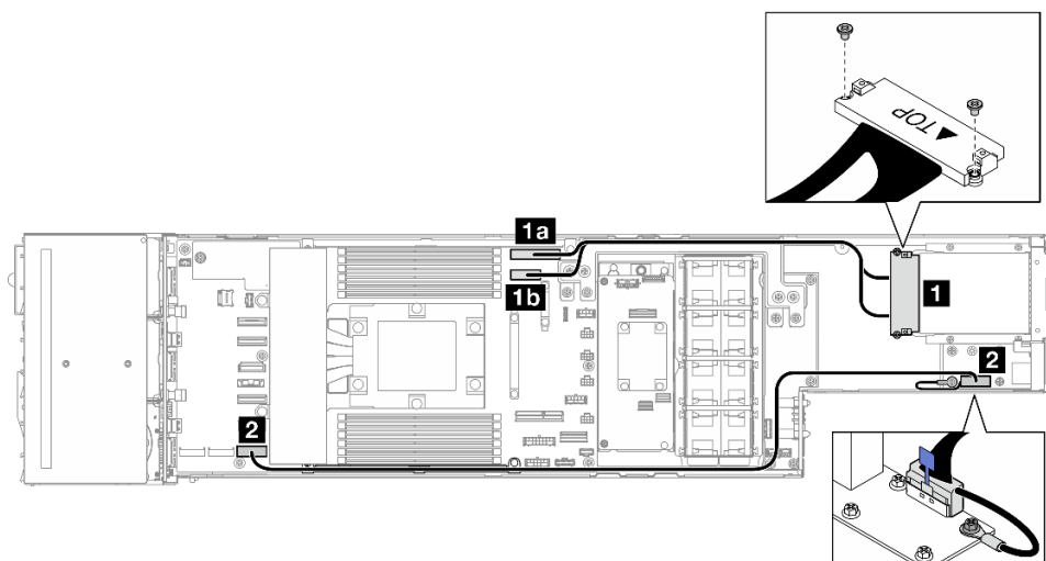
Abbildung 146. Kabel für das E/A-Modul an der Rückseite und das OCP-Modul
