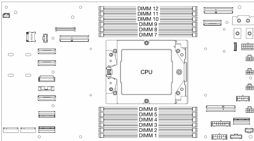
Abbildung 82. Layout für Speichermodule und Prozessoren
