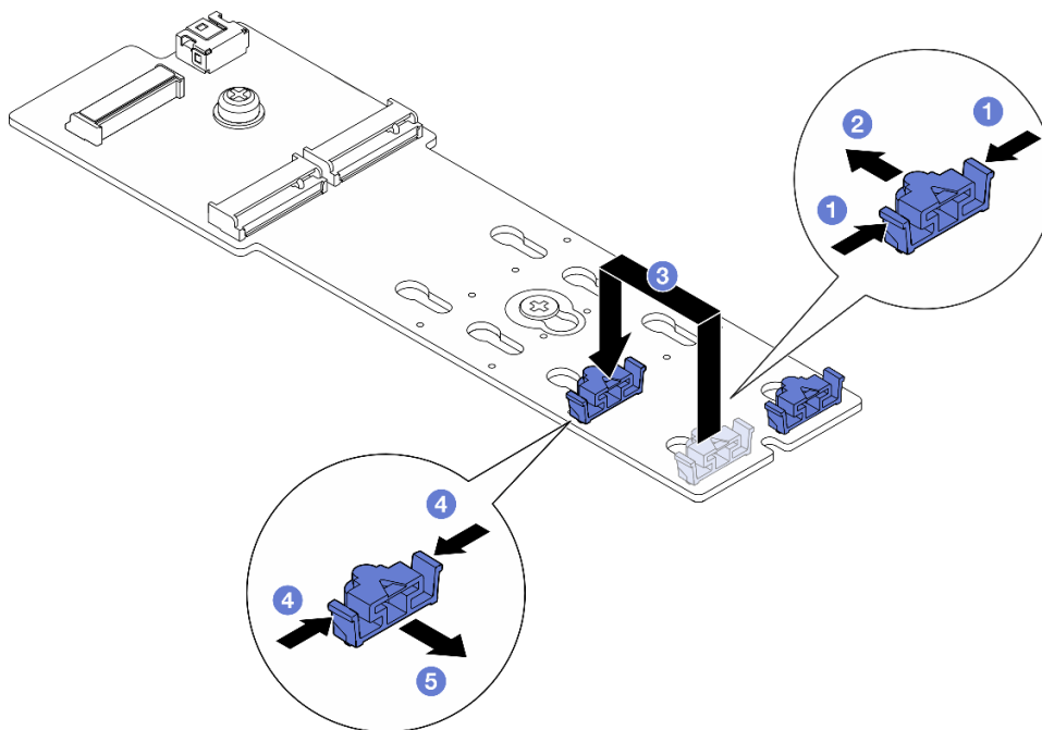
Abbildung 75. Positionsanpassung der M.2-Halterung
