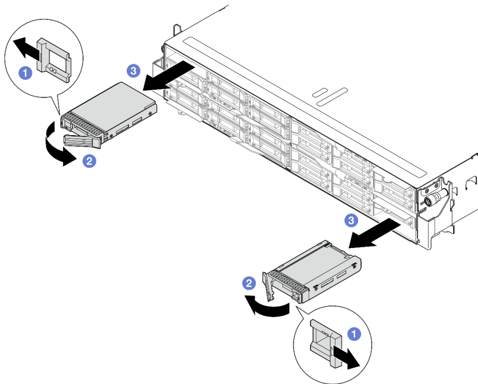
Abbildung 58. Entfernen eines Solid-State-Laufwerks
