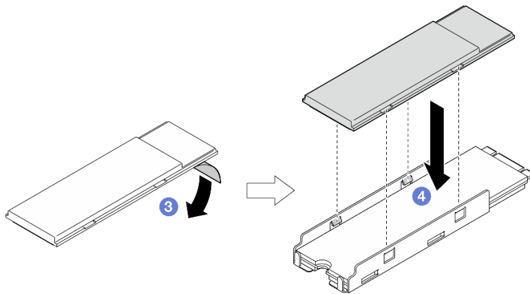
Abbildung 78. Installieren eines M.2-Kühlkörpers im M.2-Einbaurahmen
