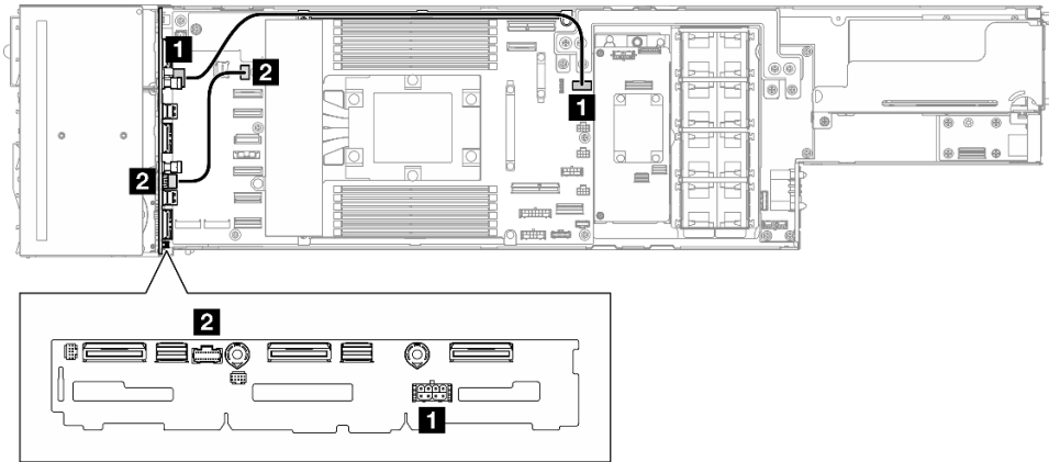
Abbildung 134. Seitenband und Netzkabelführung der Rückwandplatine für Laufwerke
