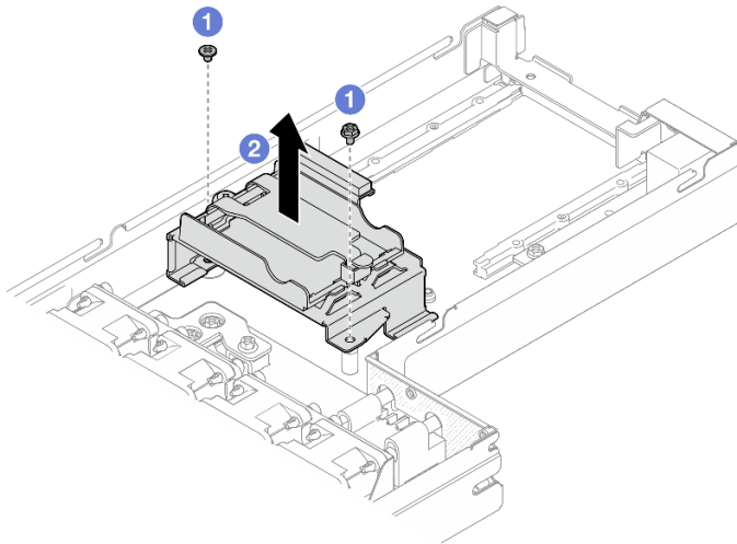
Abbildung 49. Entfernen der Halterung des Flash-Stromversorgungsmoduls
