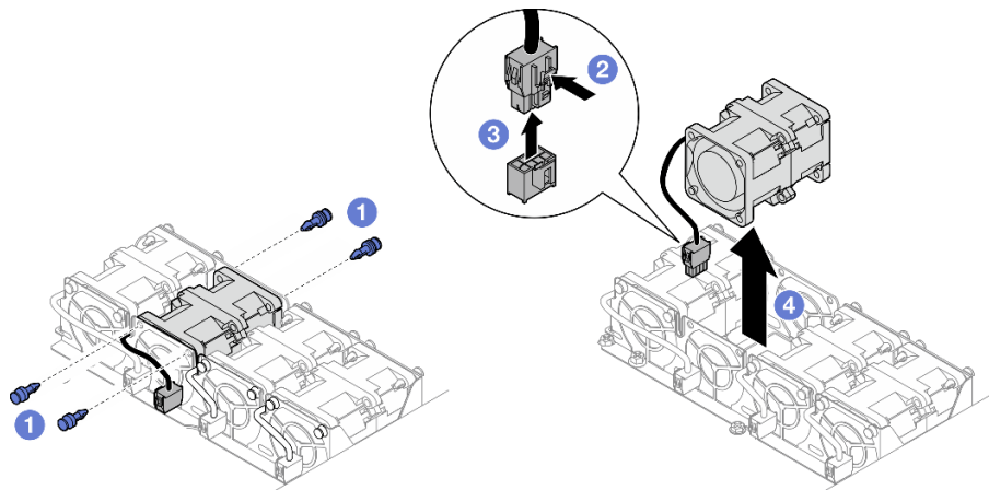
Abbildung 46. Entfernen des Lüfters
