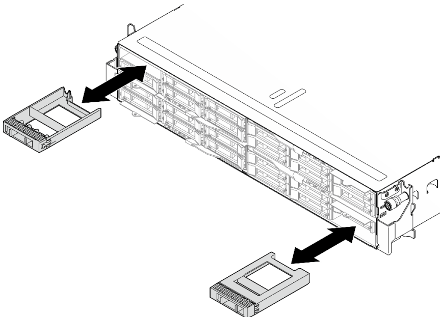
Abbildung 59. Austausch einer Abdeckblende für Laufwerke
