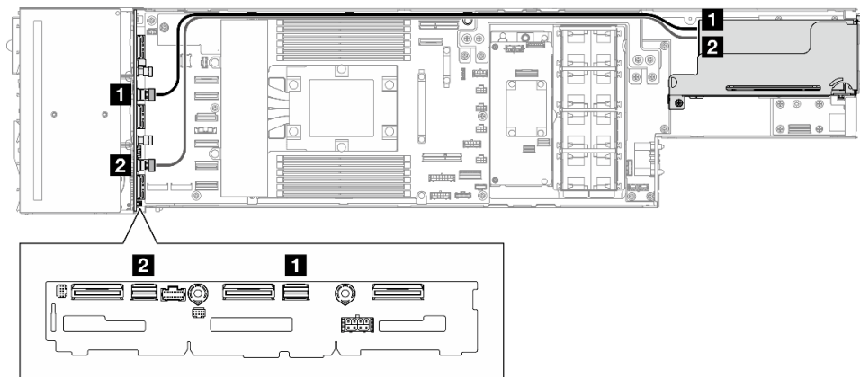
Abbildung 140. SATA/SAS-Kabelführung für 8i RAID PCIe-Adapter
