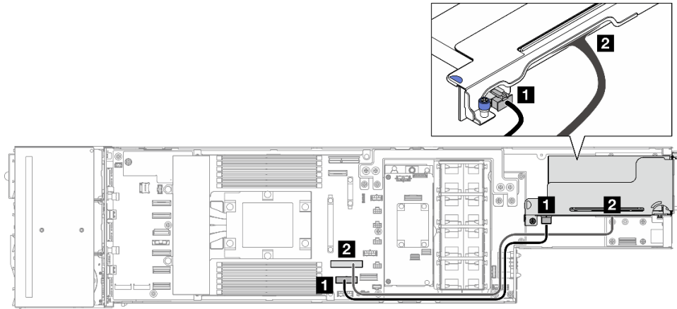
Abbildung 144. Kabelführung für PCIe-Adapterkarte
