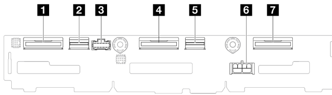
Abbildung 129. Rückwandplatine für 2,5-Zoll-Laufwerke
