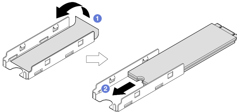
Abbildung 77. Installieren eines Wärmepads und M.2-Laufwerks im Einbaurahmen
