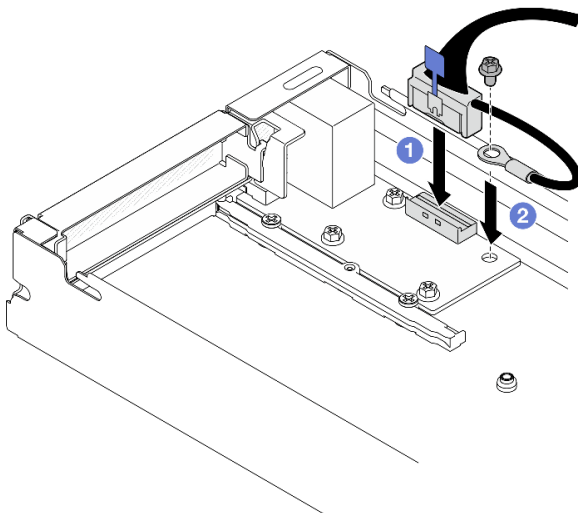
Abbildung 115. Installation des hinteren E/A-Kabels und des Erdungskabels
