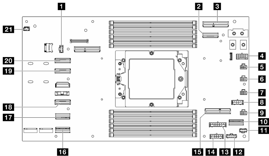
Abbildung 128. Anschlüsse auf der Systemplatine für die Kabelführung
