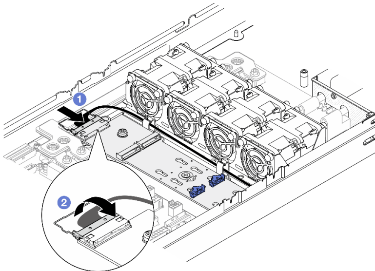
Abbildung 73. Anschließen des Kabels am SATA/NVMe M.2-Bootadapter
