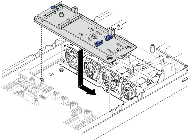
Abbildung 71. Installation eines M.2-Bootadaptersrahmens
