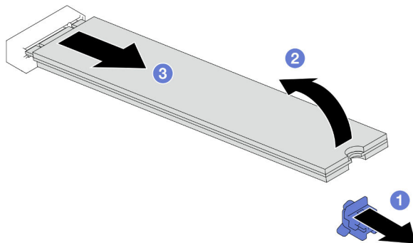
Abbildung 63. Entfernen eines M.2-Laufwerks
