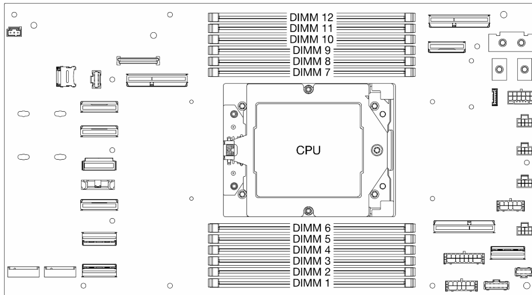
Abbildung 15. Layout für Speichermodule und Prozessor
