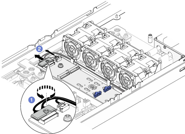
Abbildung 66. Abziehen des Kabels vom NVMe M.2-Bootadapter
