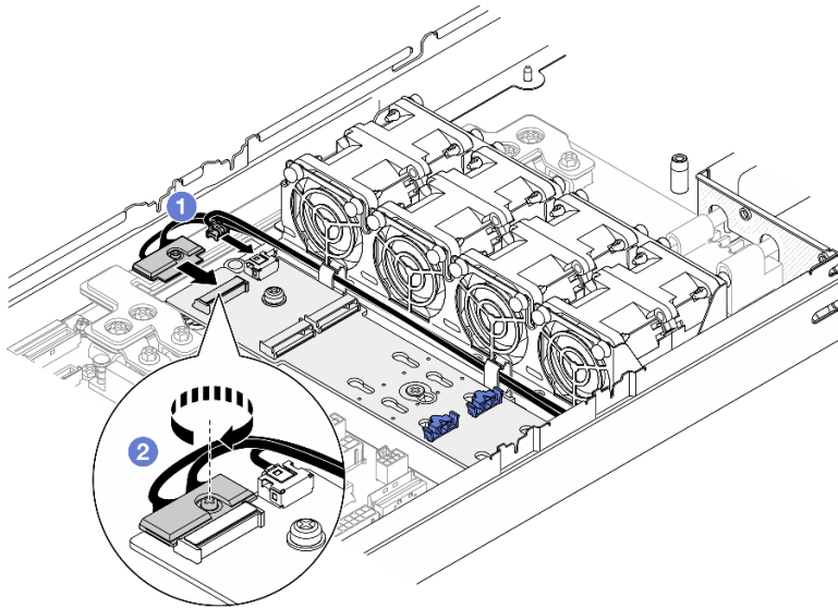
Abbildung 72. Anschließen des Kabels am NVMe M.2-Bootadapter
