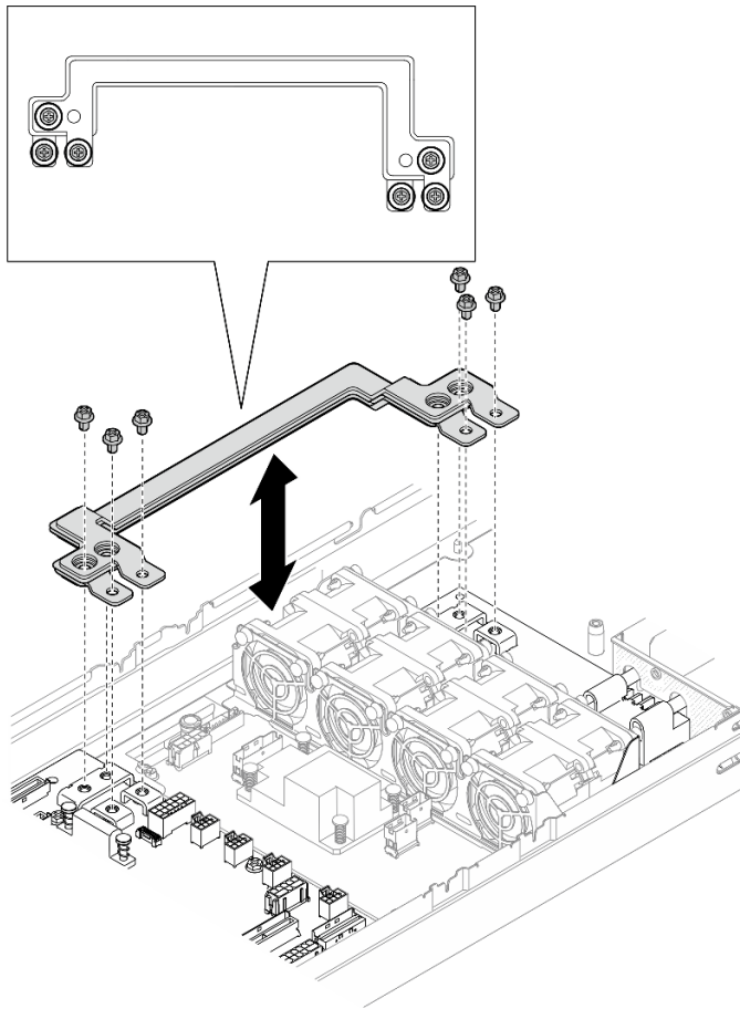
Abbildung 102. Anbringen der äußeren Schrauben der Sammelschiene
