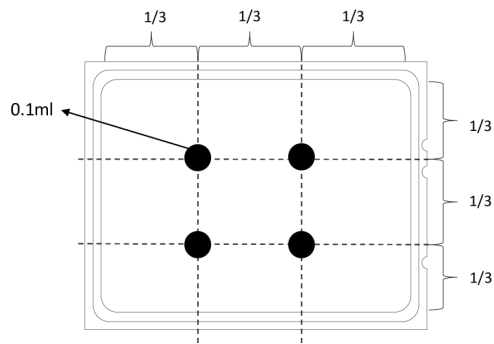
Abbildung 110. Wärmeleitpaste auftragen
