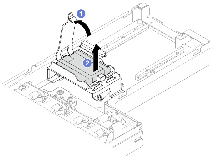
Abbildung 48. Entfernen des Flash-Stromversorgungsmoduls
