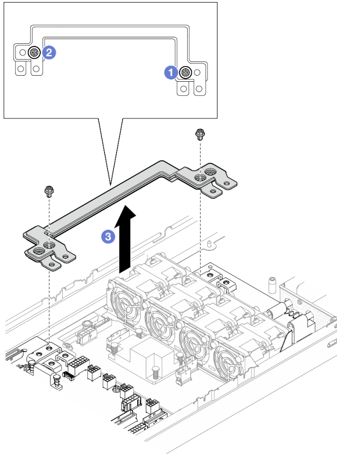
Abbildung 100. Entfernen der Sammelschiene
