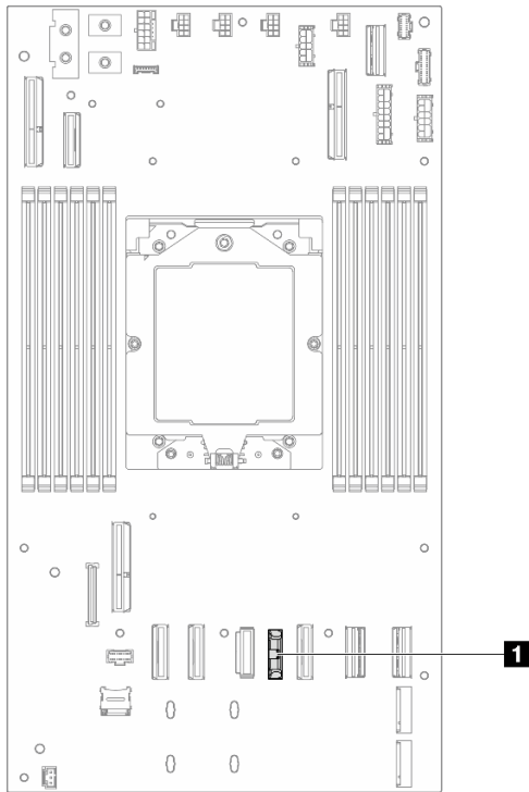
Abbildung 42. Position des CMOS-Batteriesockels
