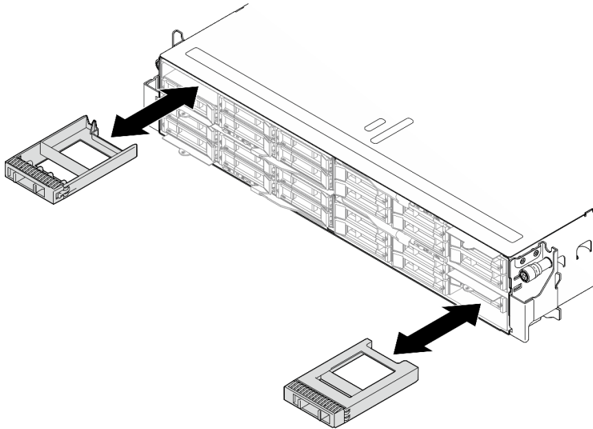
Abbildung 60. Austausch einer Abdeckblende für Laufwerke
