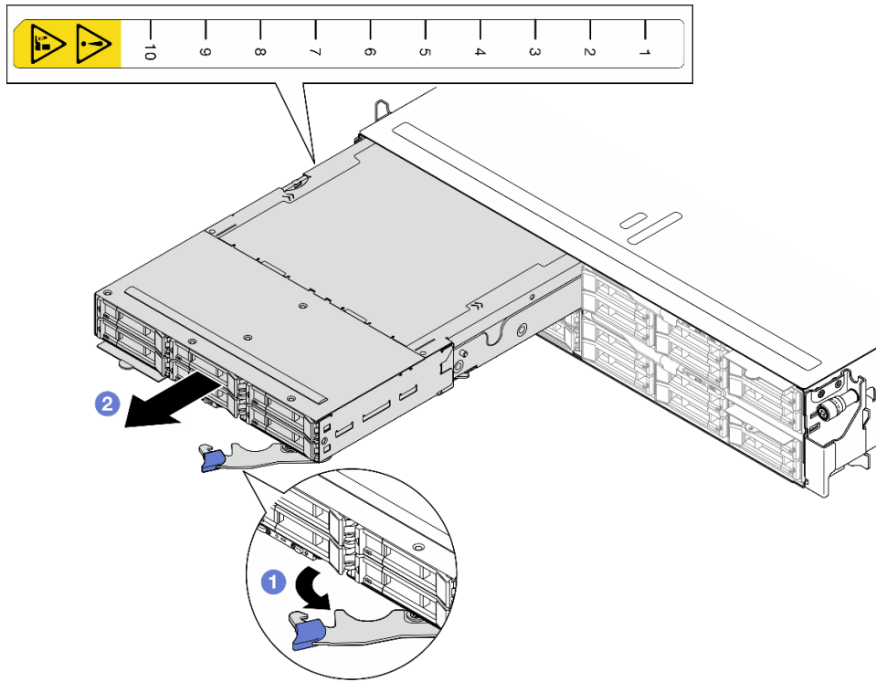
Abbildung 30. Knotenentfernung aus einem linken Rahmen
