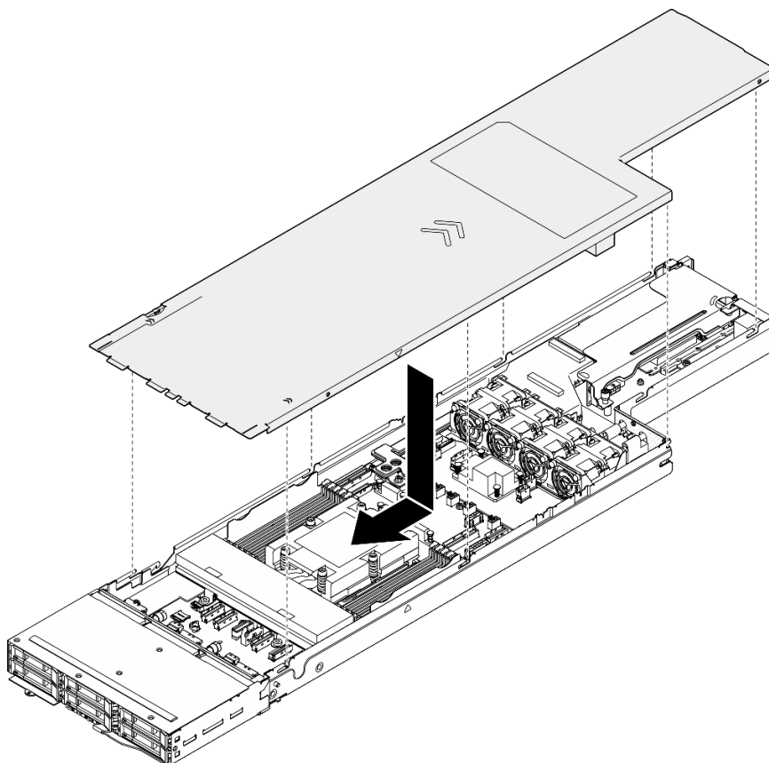
Abbildung 127. Installieren der oberen Abdeckung
