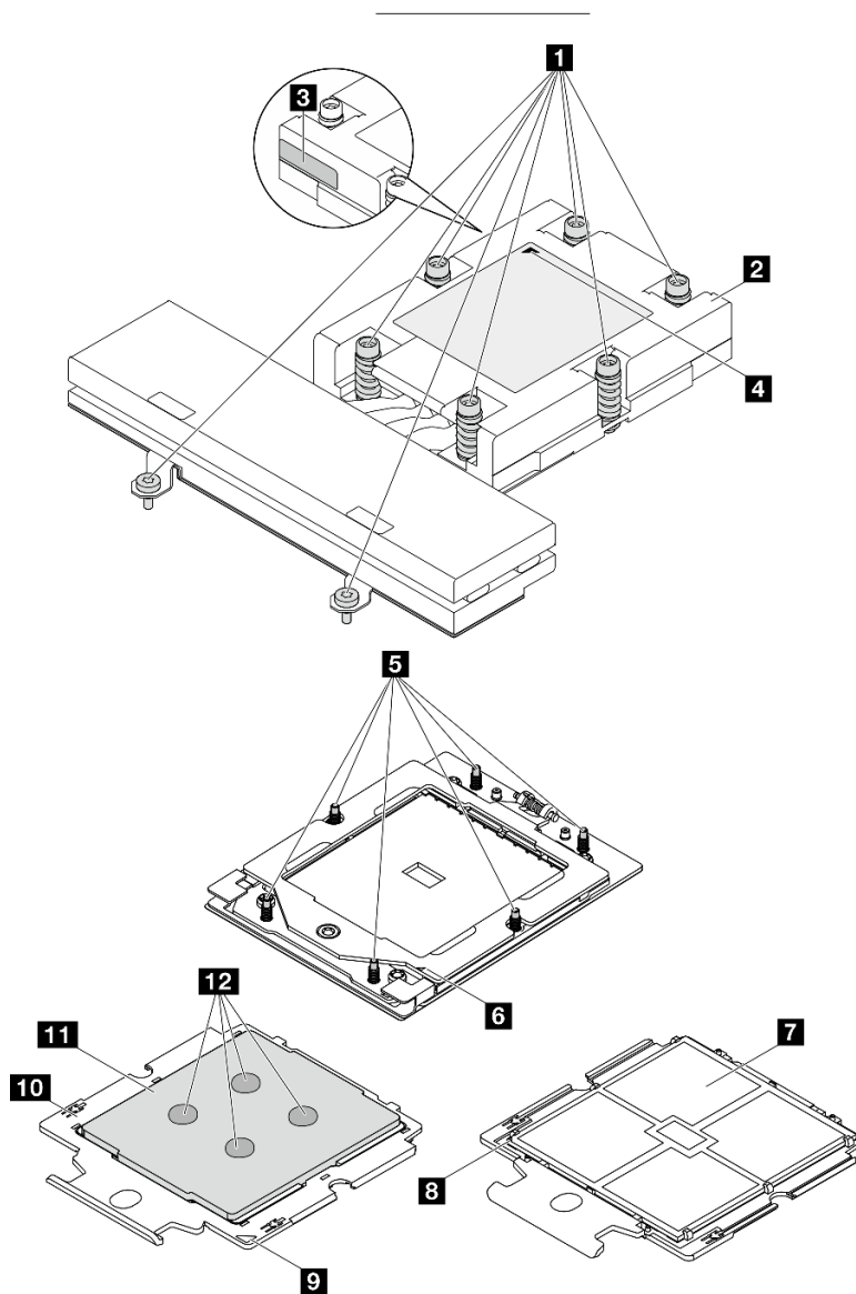
Abbildung 108. Prozessor- und Kühlkörperkomponenten
