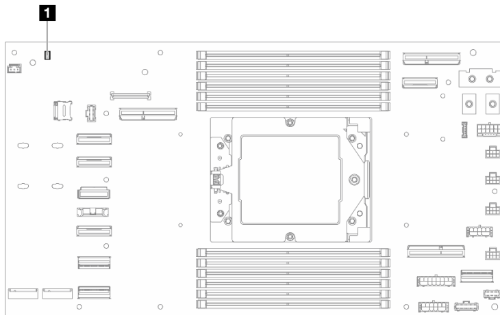
Abbildung 155. Anzeigen auf der Systemplatine
