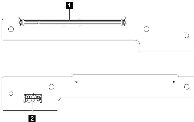
Abbildung 132. Anschlüsse an der PCIe-Adapterkarte
