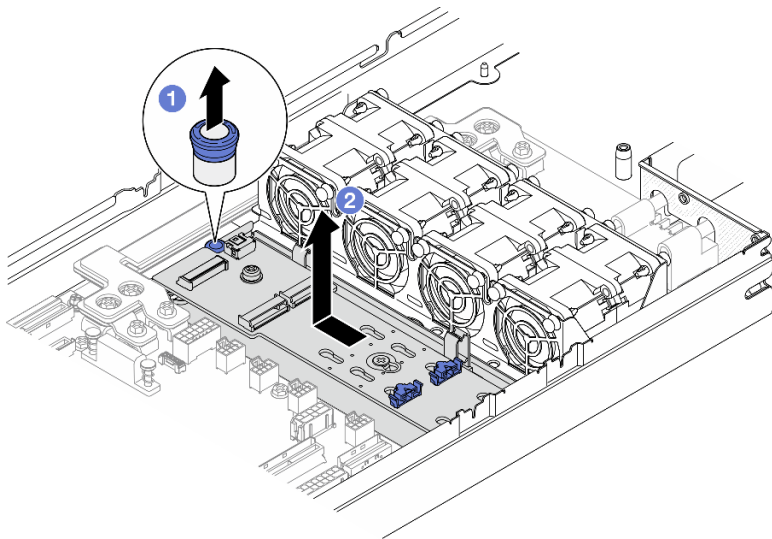
Abbildung 68. Entfernen des M.2-Bootadapterrahmens
