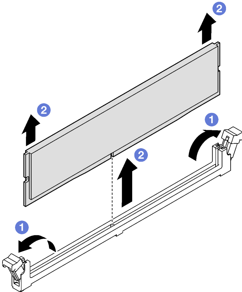
Abbildung 83. Entfernen eines Speichermoduls
