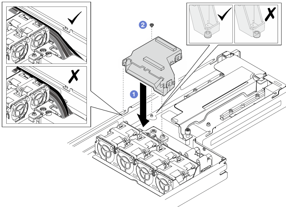
Abbildung 57. Installation des GPU-Luftkanals
