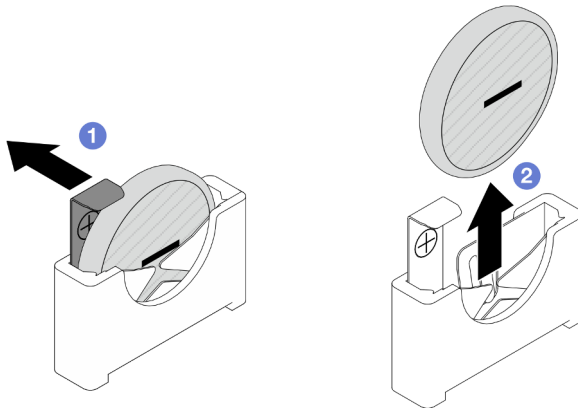
Abbildung 41. Entfernen der CMOS-Batterie
