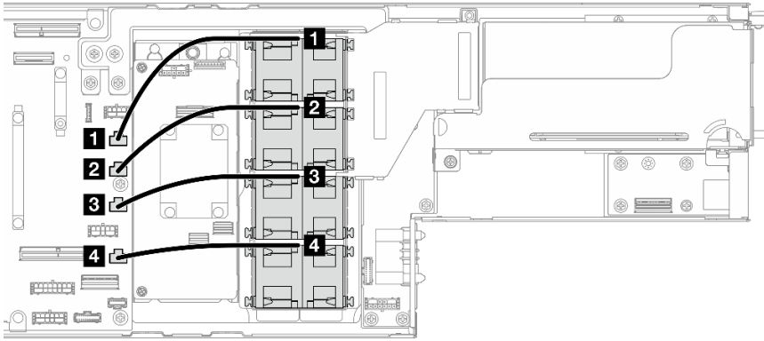
Abbildung 141. Lüfterkabelführung
