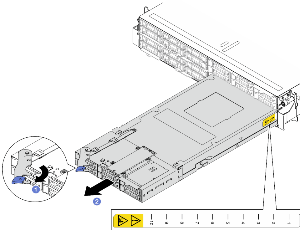
Abbildung 31. Knotenentfernung aus einem rechten Rahmen
