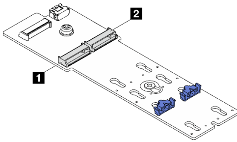
Abbildung 80. M.2-Laufwerksteckplätze
