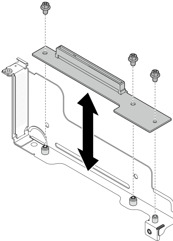
Abbildung 97. Austausch der PCIe-Adapterkarte
