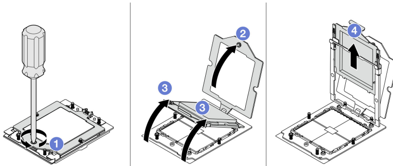
Abbildung 107. Entfernen eines Prozessors
