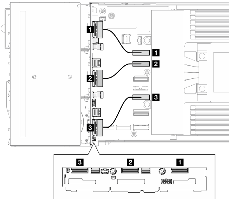
Abbildung 135. NVMe-Kabelführung
