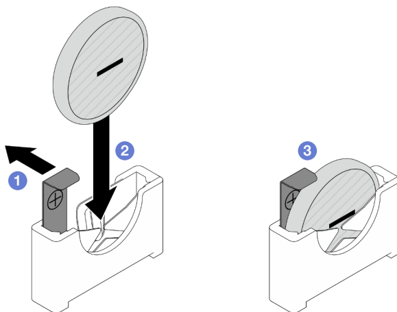
Abbildung 43. Installieren einer CMOS-Batterie
