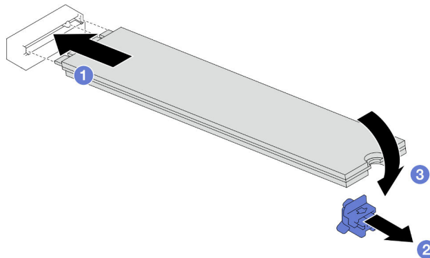
Abbildung 79. Installation eines M.2-Laufwerks
