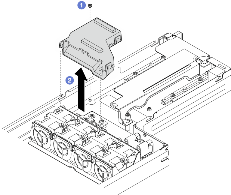
Abbildung 56. Entfernen des GPU-Luftkanals
