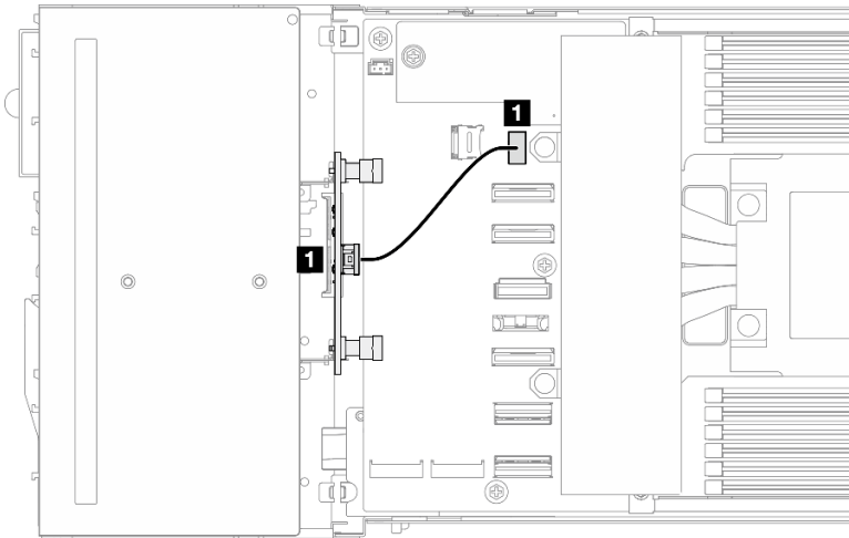
Abbildung 142. Kabelführung für E/A-Platine an der Vorderseite
