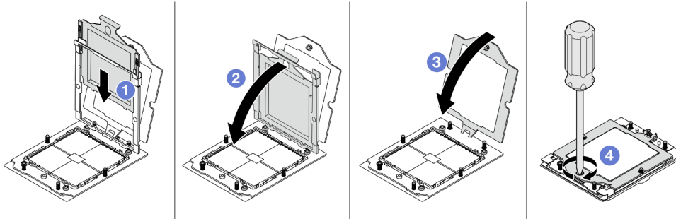
Abbildung 109. Installieren eines Prozessors
