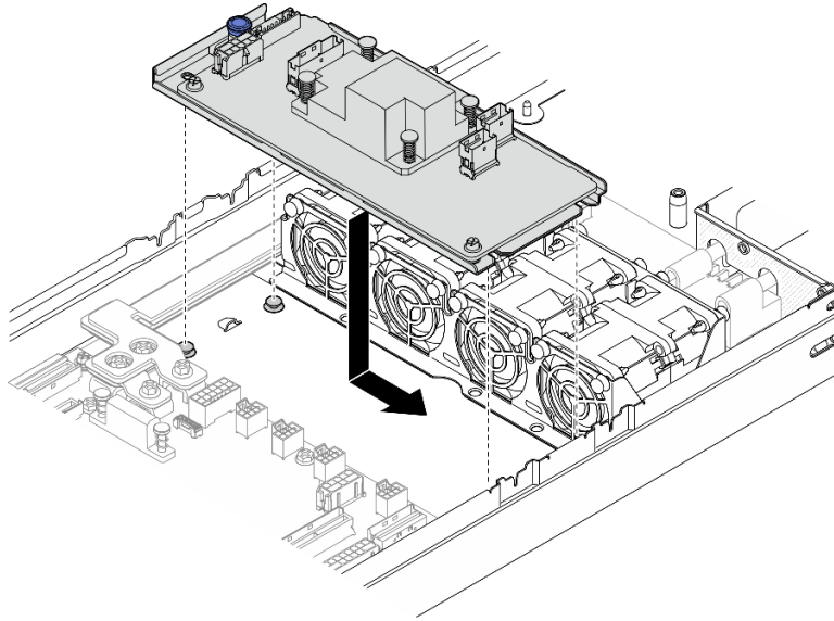
Abbildung 39. Installation eines internen CFF RAID-Adapters
