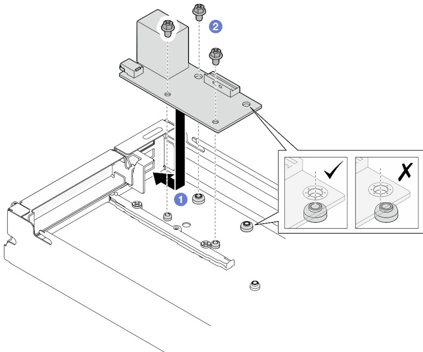
Abbildung 114. Installation des E/A-Moduls an der Rückseite
