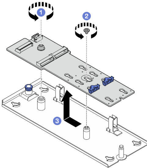
Abbildung 69. Entfernen des M.2-Bootadapters
