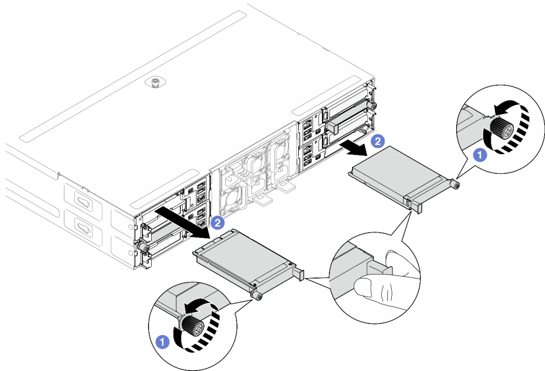
Abbildung 90. Entfernen des hinteren OCP-Moduls
