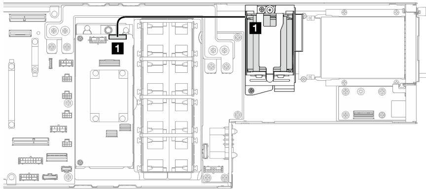
Abbildung 139. Kabelführung für Flash-Stromversorgungsmodul
