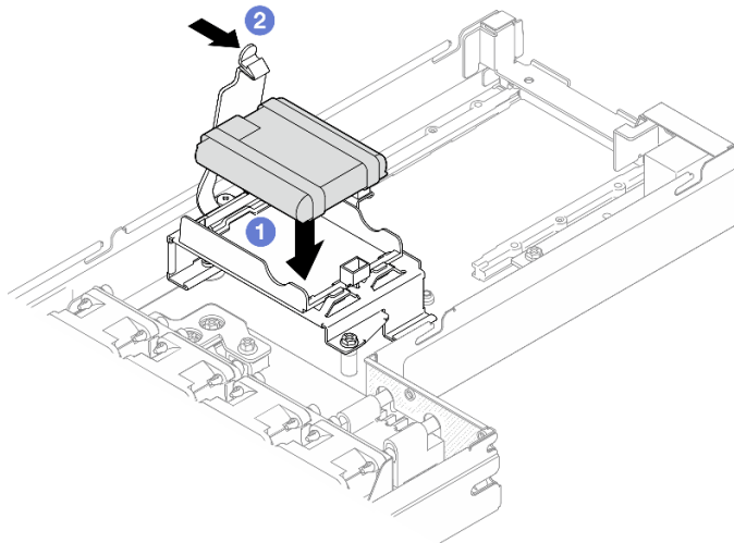
Abbildung 51. Installation des Flash-Stromversorgungsmoduls
