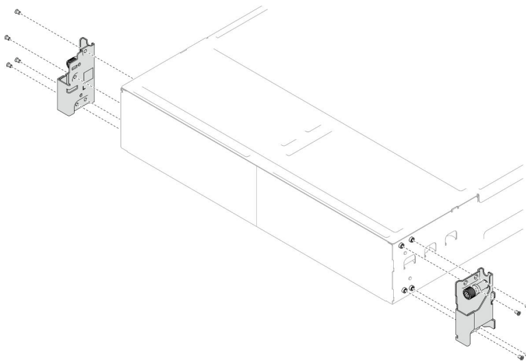
Abbildung 21. Installation der EIA-Halterung
