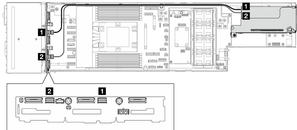
Figura 140. Disposición de los cables SATA/SAS del adaptador PCIe de RAID 8i
