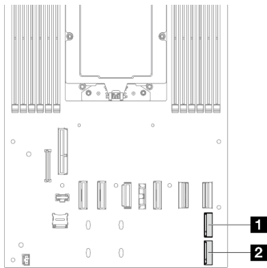
Figura 76. Ubicación de las bahías M.2 en la placa del sistema
