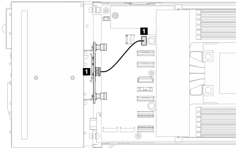
Figura 142. Disposición de los cables de la placa de E/S frontal
