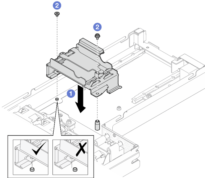
Figura 50. Instalación del soporte del módulo de alimentación flash
