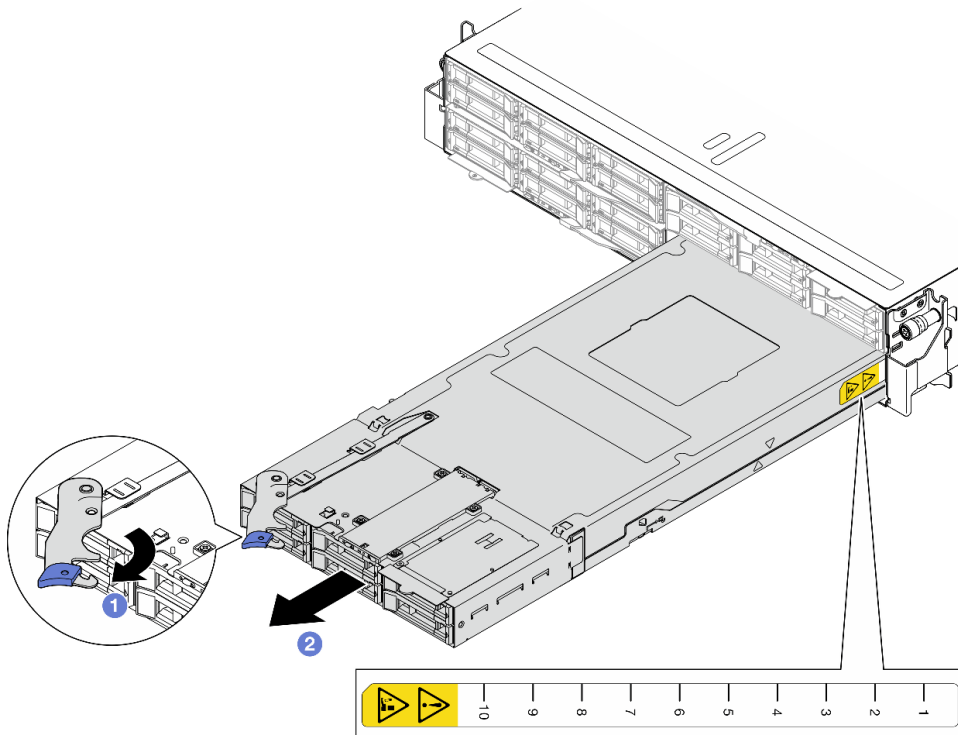
Figura 31. Extracción del nodo de una bandeja derecha
