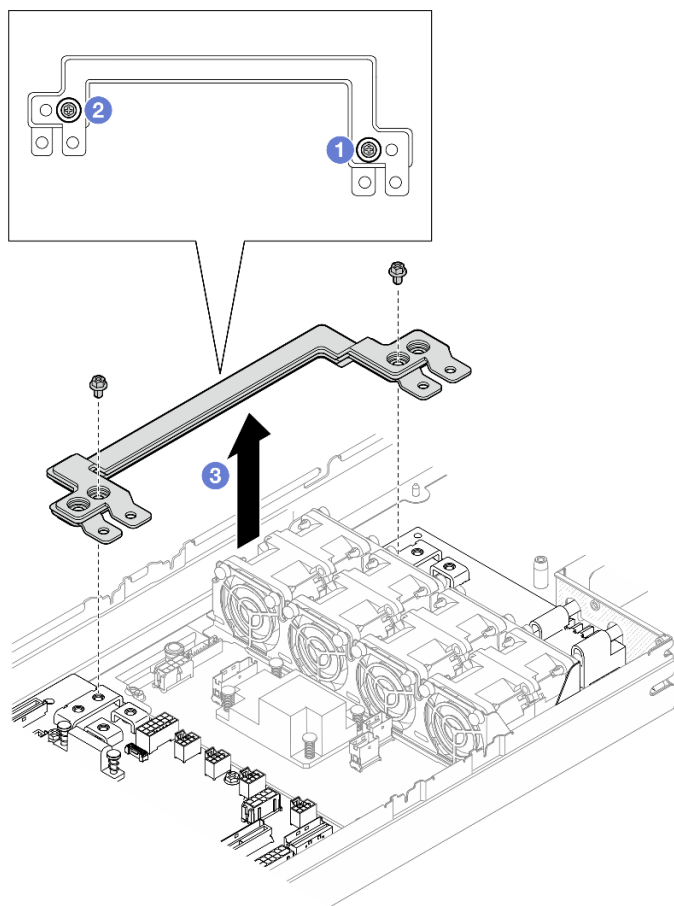
Figura 100. Extracción de la barra de bus de alimentación
