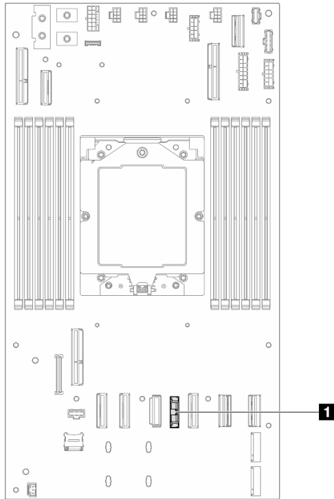
Figura 40. Ubicación del zócalo de la batería CMOS
