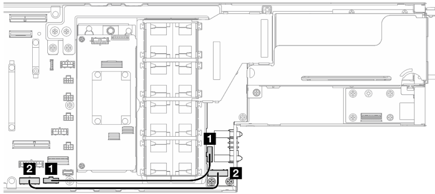
Figura 145. Disposición de los cables para la placa de la distribución de alimentación
