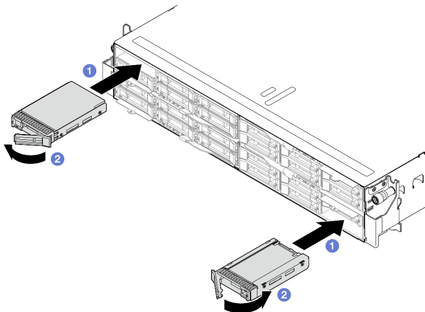
Figura 61. Instalación de una unidad de estado sólido
