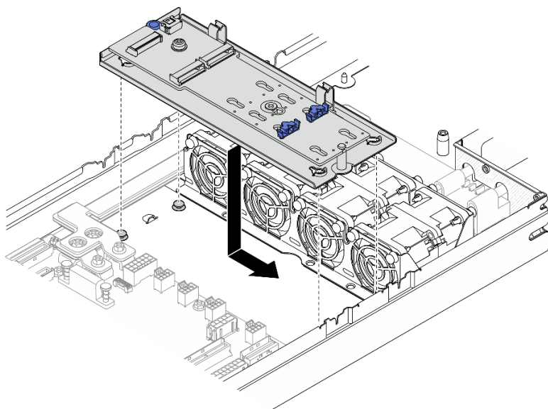
Figura 71. Instalación de la bandeja del adaptador de arranque M.2
