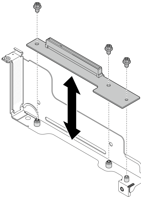
Figura 97. Sustitución de la tarjeta de expansión PCIe
