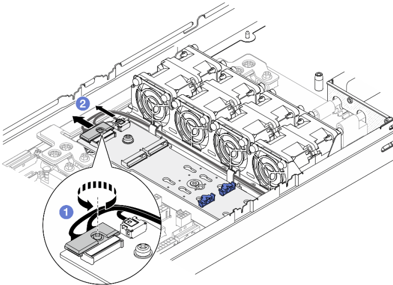
Figura 66. Desconexión del cable del adaptador de arranque M.2 NVMe
