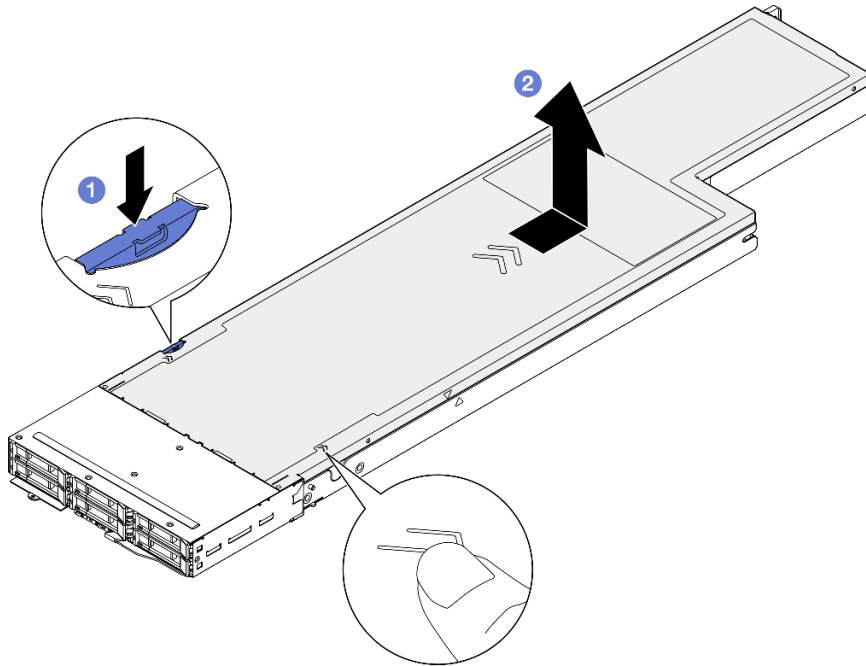
Figura 126. Extracción de la cubierta superior
