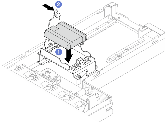
Figura 51. Instalación del módulo de alimentación flash
