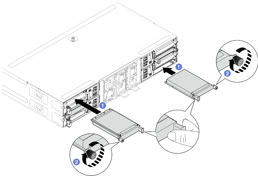
Figura 91. Instalación del módulo de OCP posterior
