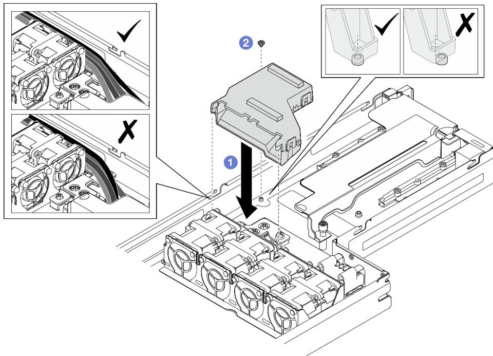
Figura 57. Instalación del conducto de aire de GPU
