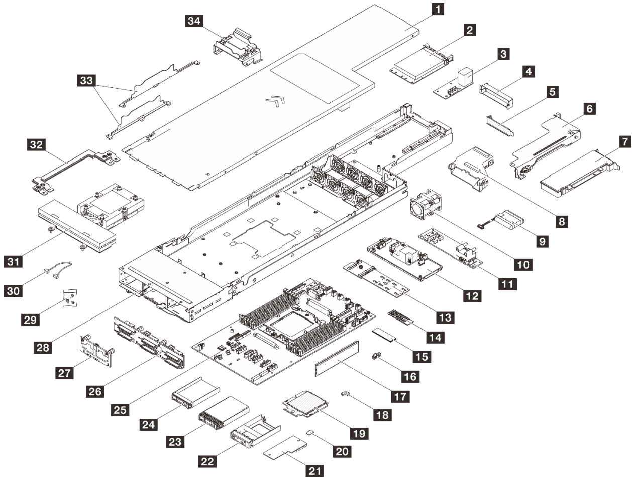
Figura 11. Componentes del nodo
