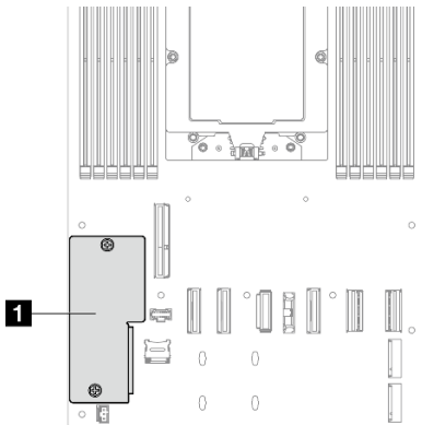
Figura 118. Ubicación del Firmware y módulo de seguridad de RoT
