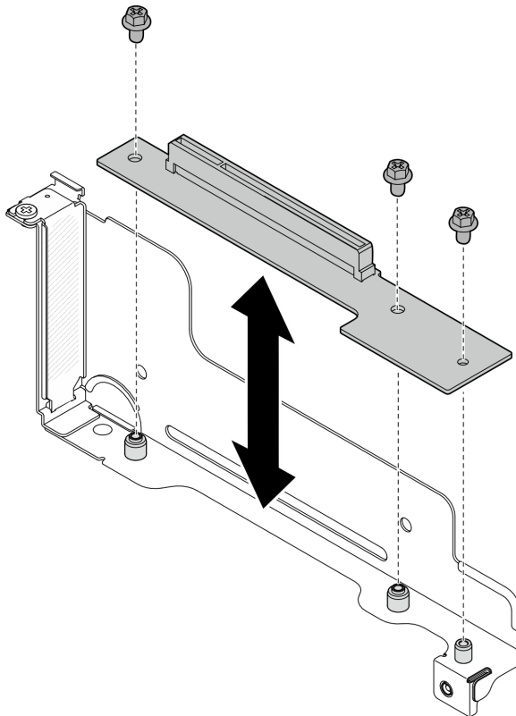
Figura 95. Sustitución de la tarjeta de expansión PCIe
