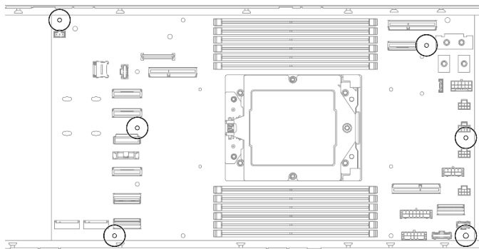
Figura 124. Instalación de los tornillos
