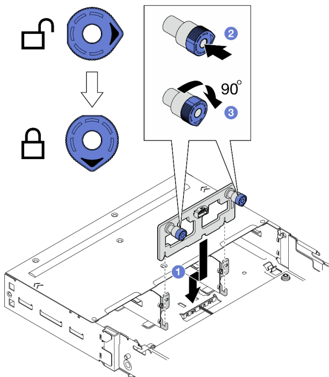
Figura 55. Instalación de la placa posterior de E/S frontal
