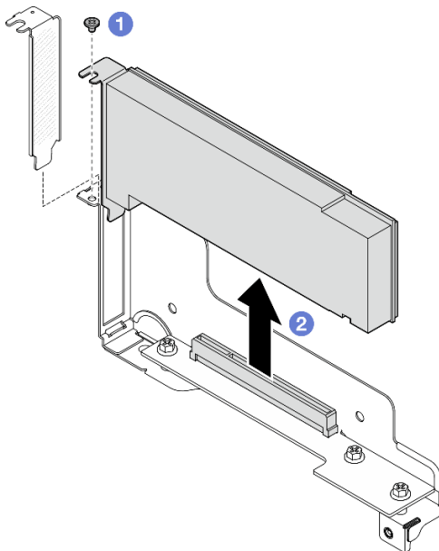
Figura 94. Extracción de un adaptador PCIe
