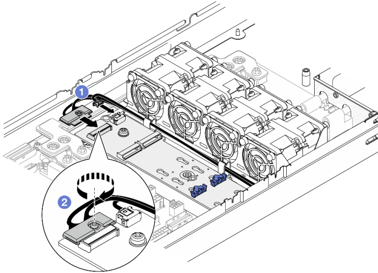
Figura 72. Conexión del cable al adaptador de arranque M.2 NVMe
