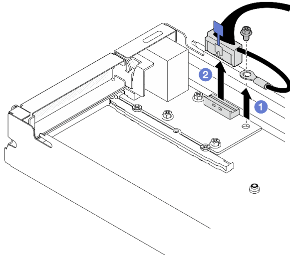
Figura 112. Extracción del cable de E/S posterior y del cable de conexión a tierra
