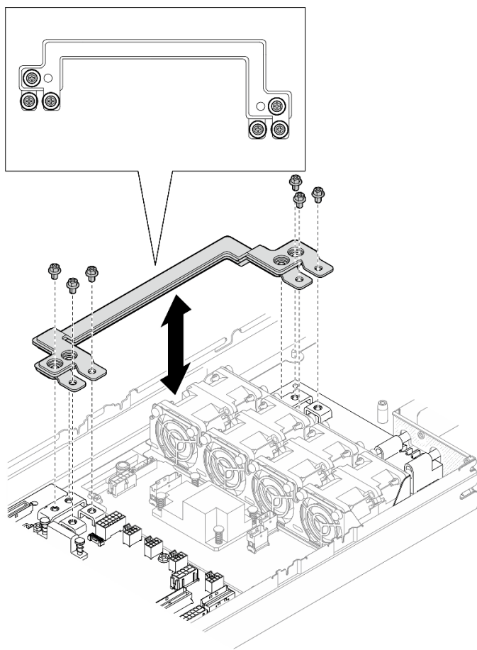
Figura 102. Instalación de los tornillos externos de la barra de bus de alimentación
