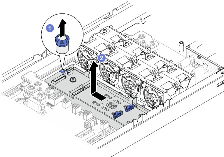
Figura 68. Extracción de la bandeja del adaptador de arranque M.2
