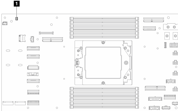
Figura 155. LED de la placa del sistema
