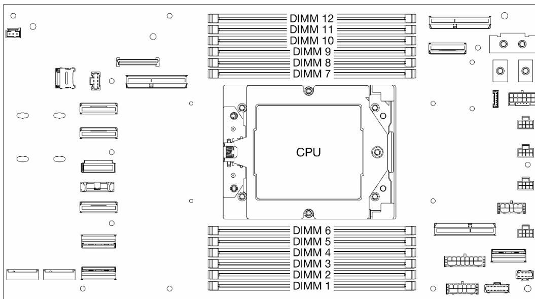
Figura 82. Diseño de los módulos de memoria y el procesador
