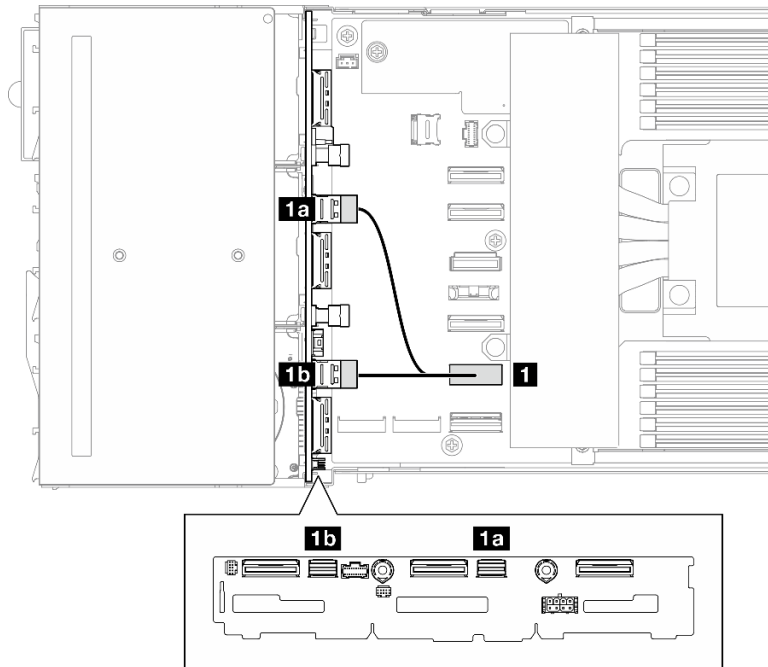
Figura 136. Disposición de los cables SATA incorporados
