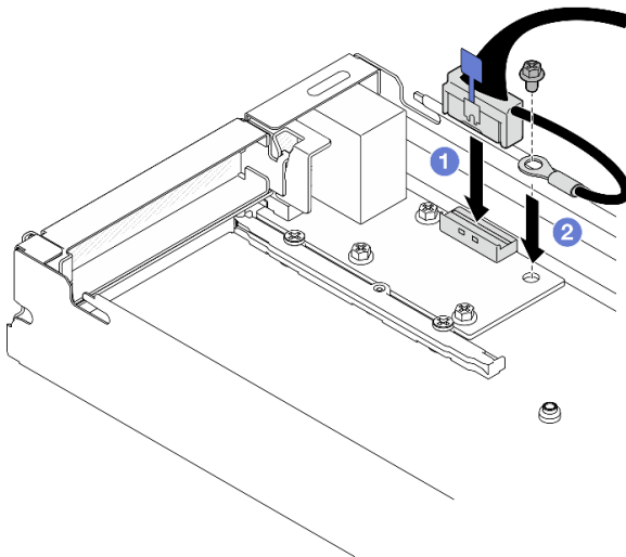
Figura 147. Instalación del cable de E/S posterior y del cable de conexión a tierra
