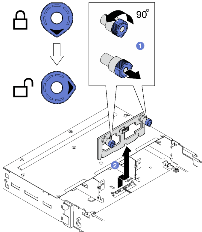
Figura 54. Extracción de la placa posterior de E/S frontal
