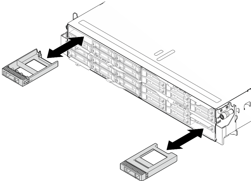
Figura 60. Sustitución de un relleno de unidad
