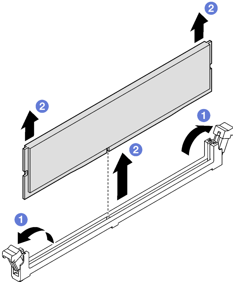
Figura 83. Extracción de un módulo de memoria
