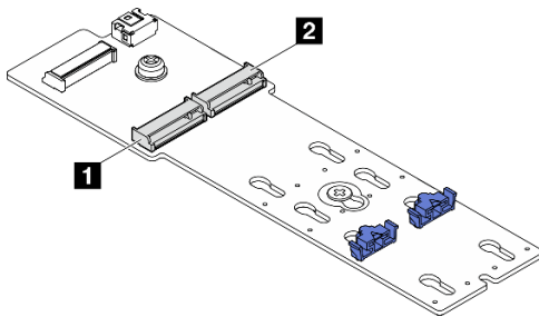
Figura 80. Ranuras de unidad M.2
