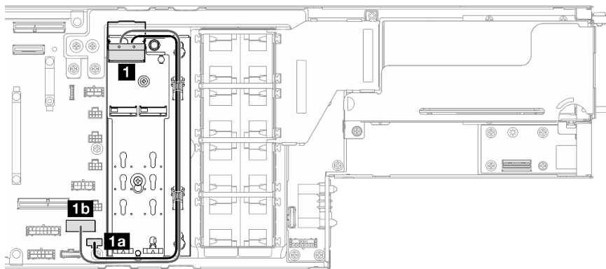
Figura 143. Disposición de los cables para el adaptador de arranque M.2 SATA/NVMe
