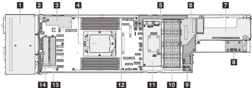
Figura 7. Vista superior de SD535 V3
