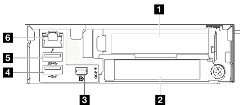
Figura 4. Vista posterior
