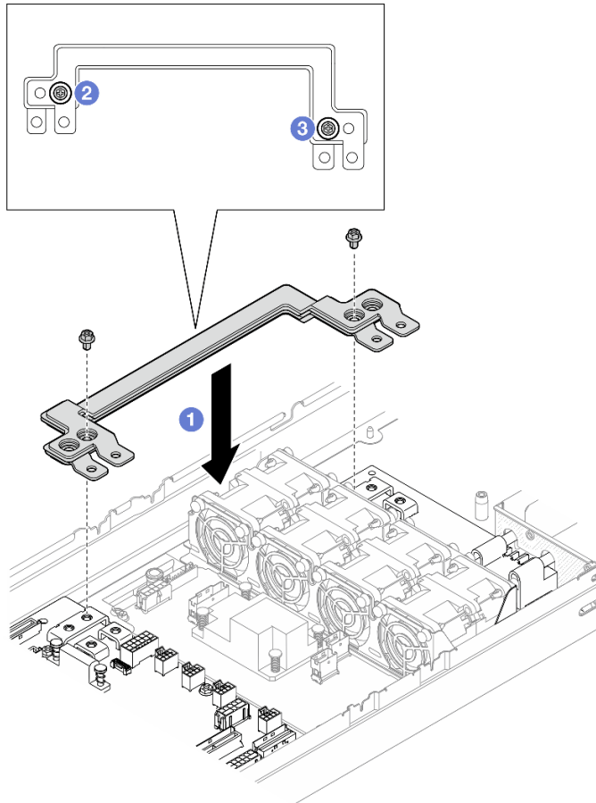
Figura 101. Instalación de la barra de bus de alimentación
