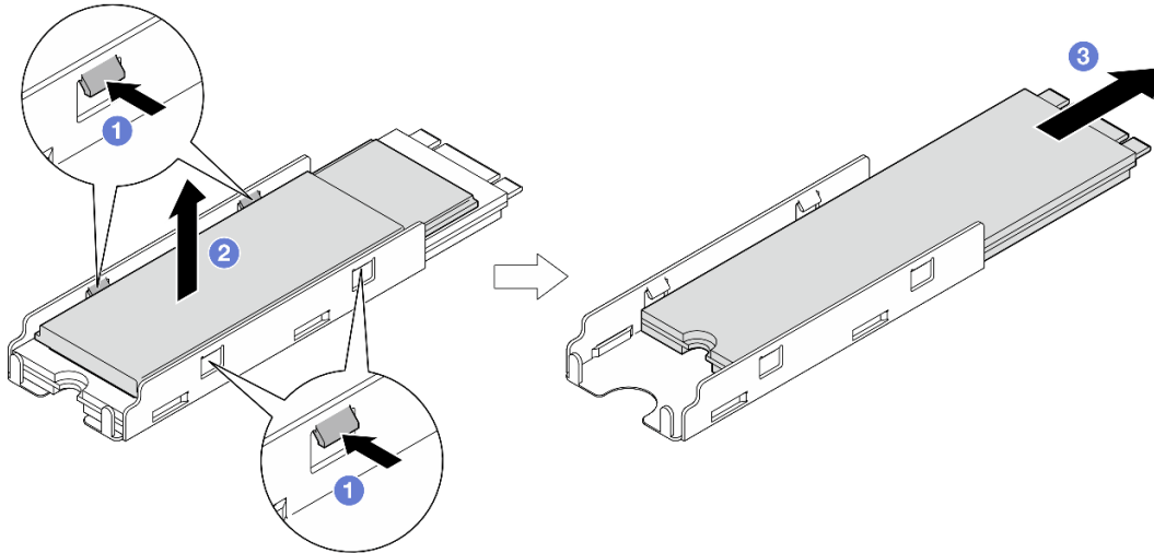
Figura 64. Extracción del dissipador de calor M.2
