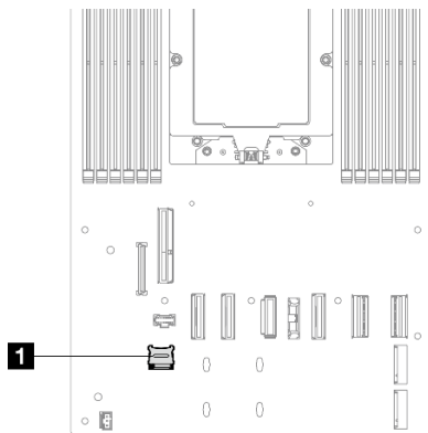
Figura 86. Ubicación del zócalo de MicroSD
