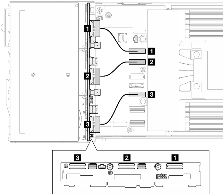
Figura 135. Disposición de los cables NVMe
