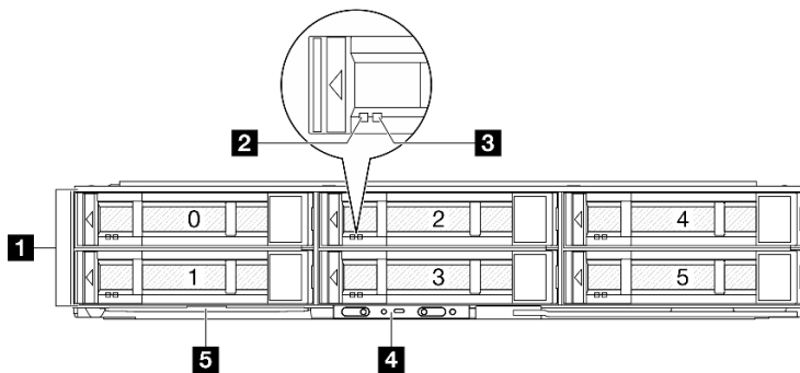
Figura 2. Configuración con seis SSD SAS/SATA/NVMe 2,5 pulgadas
