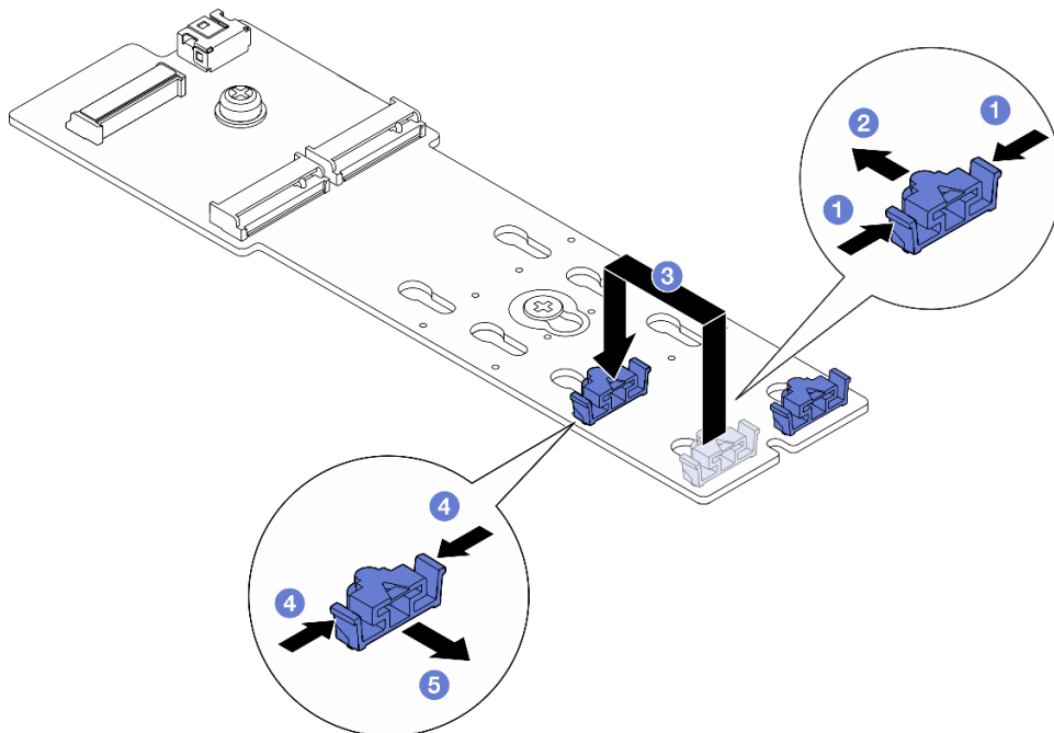
Figura 75. Ajuste del elemento de sujeción M.2
