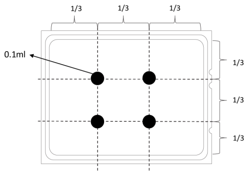
Figura 110. Aplicación de grasa térmica
