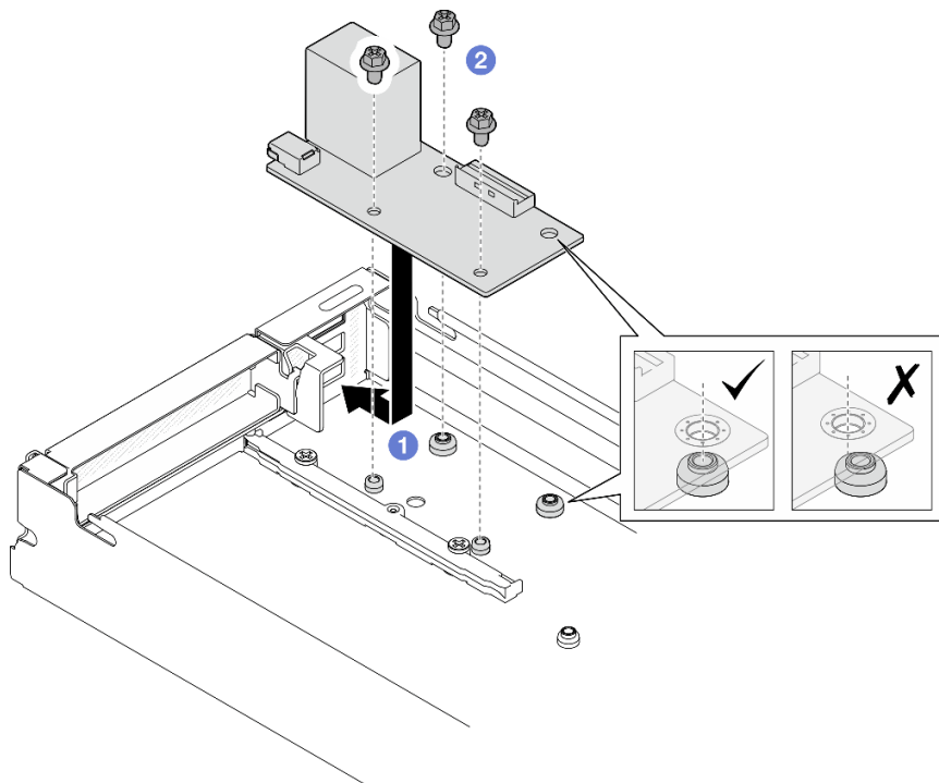
Figura 114. Instalación del módulo de E/S posterior
