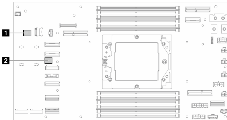
Figura 9. Conmutadores de la placa del sistema
