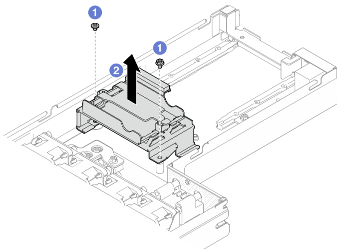
Figura 49. Extracción del soporte del módulo de alimentación flash
