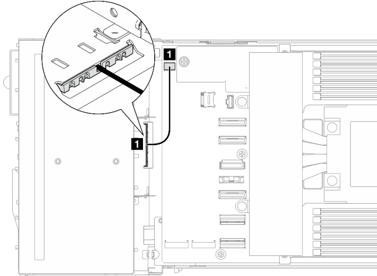
Figura 148. Disposición de los cables del sensor térmico frontal
