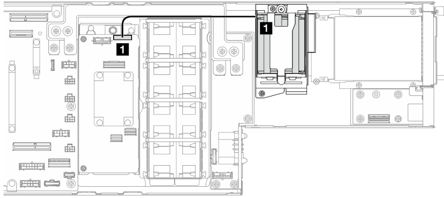
Figura 139. Disposición de cables del módulo de alimentación flash
