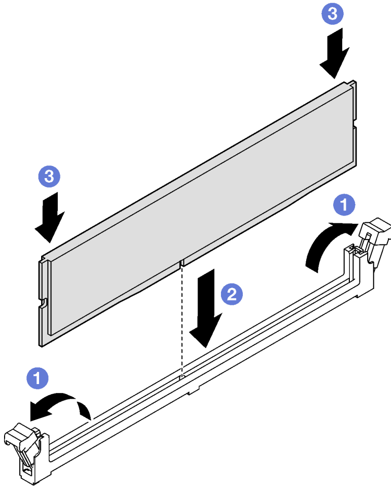
Figura 85. Instalación de un módulo de memoria
