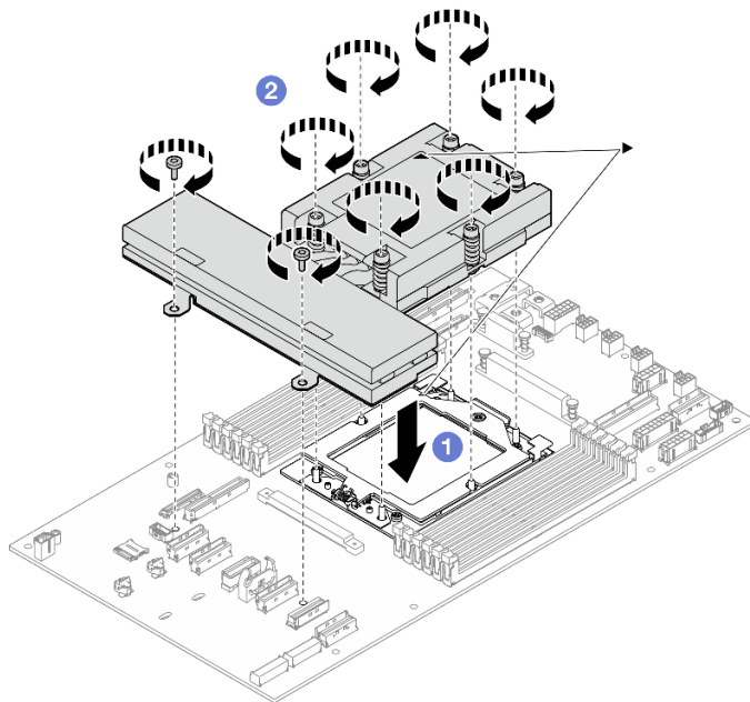
Figura 111. Instalar un disipador de calor
