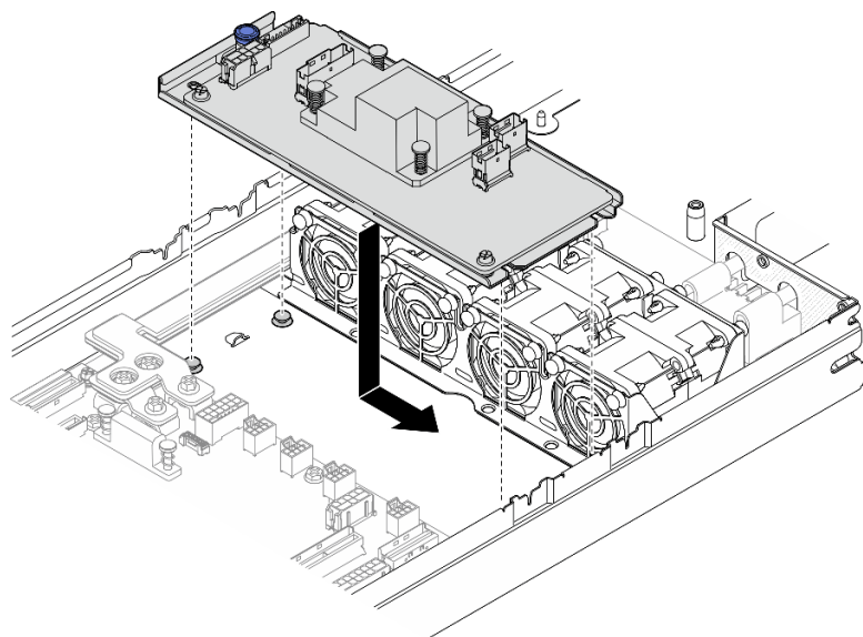
Figura 39. Instalación del adaptador RAID CFF interno
