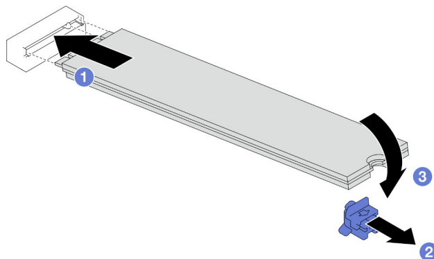
Figura 79. Instalación de una unidad M.2
