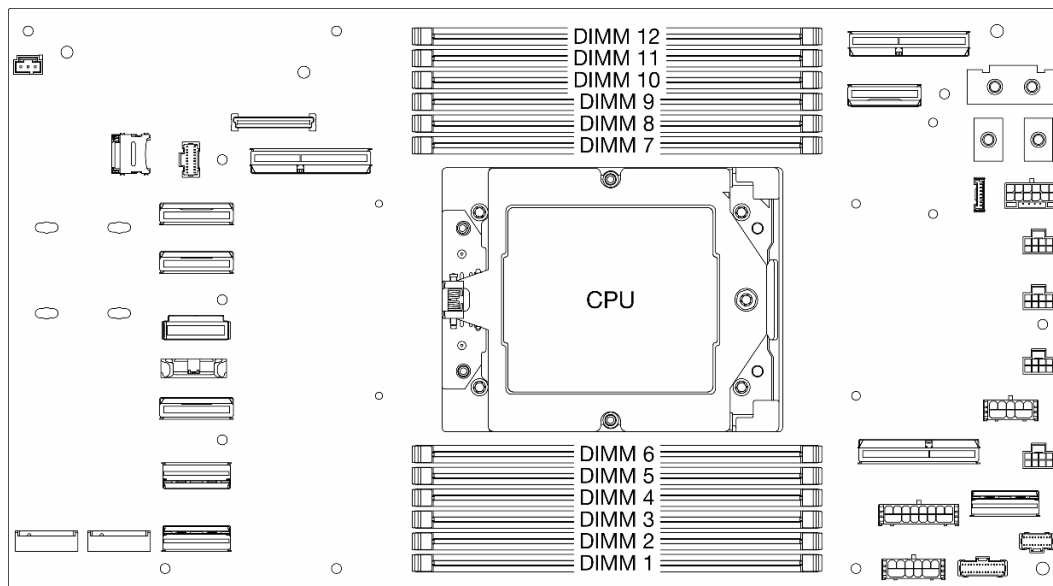
Figura 15. Diseño de los módulos de memoria y el procesador
