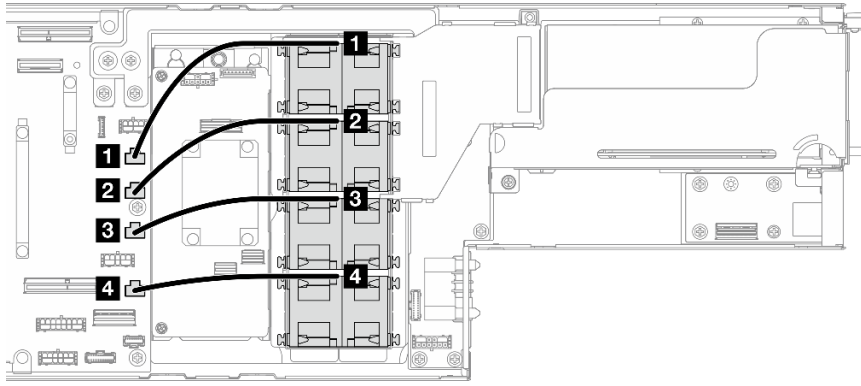
Figura 141. Disposición de los cables del ventilador
