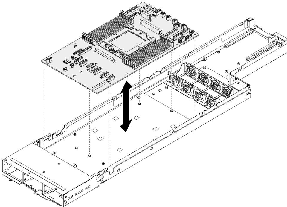
Figura 122. Extracción de la placa de sistema
