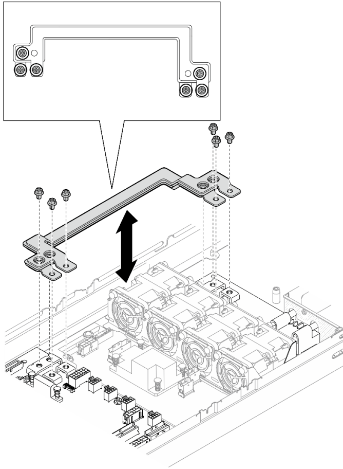
Figura 99. Extracción de los tornillos externos de la barra de bus de alimentación
