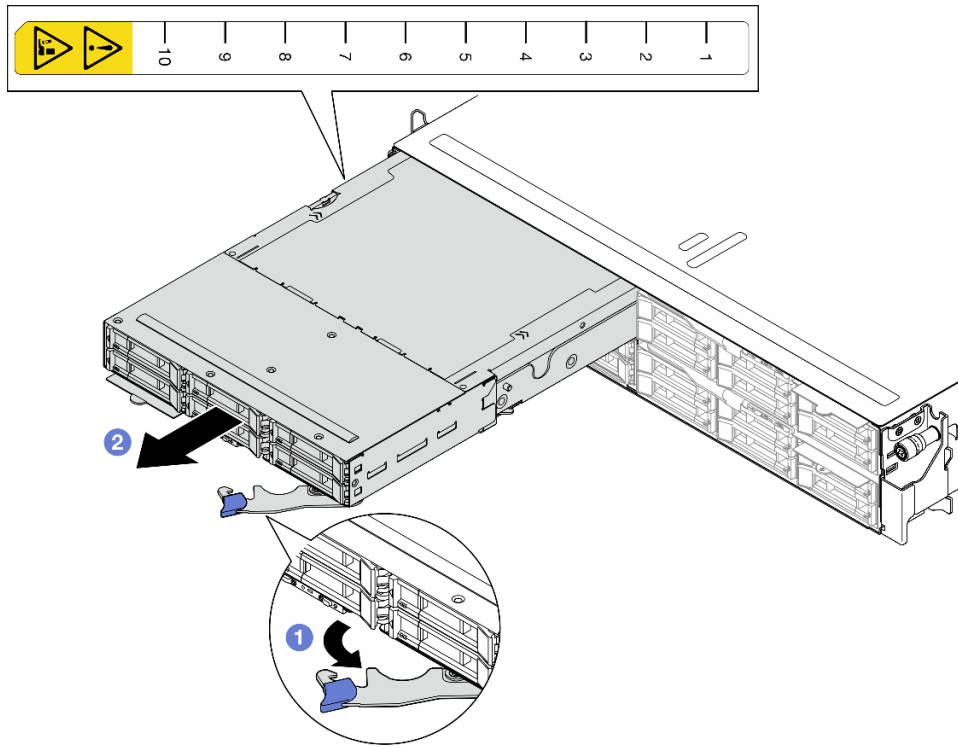
Figura 30. Extracción del nodo de una bandeja izquierda
