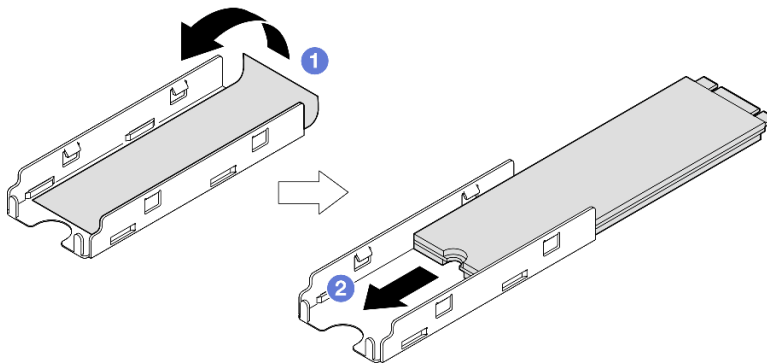
Figura 77. Instalación de una almohadilla térmica y una unidad M.2 en la bandeja
