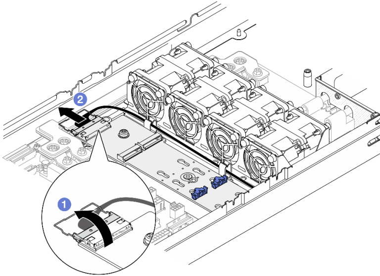
Figura 67. Desconexión del cable del adaptador de arranque M.2 SATA/NVMe
