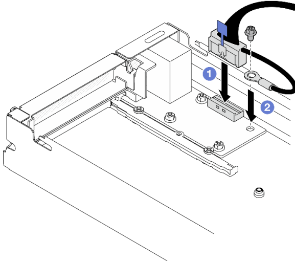
Figura 115. Instalación del cable de E/S posterior y del cable de conexión a tierra
