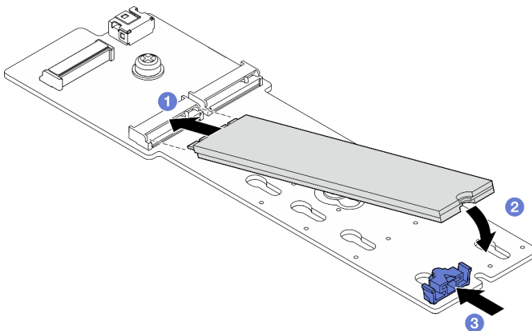
Figura 81. Instalación de una unidad M.2
