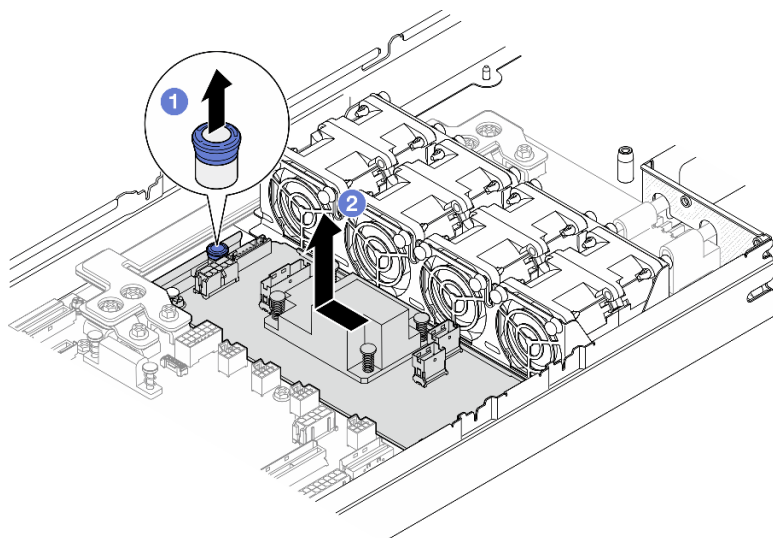
Figura 38. Extracción del adaptador RAID CFF interno
