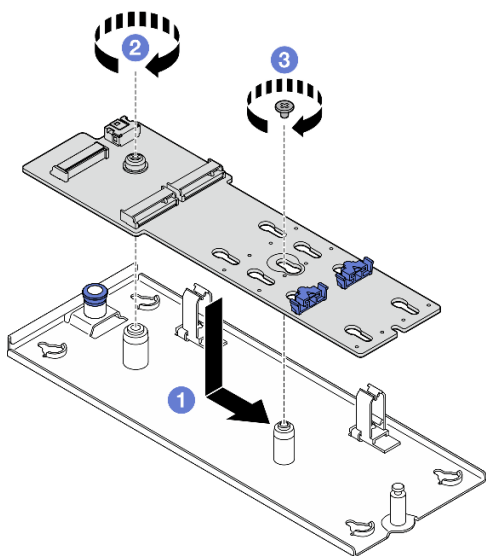
Figura 70. Instalación del adaptador de arranque M.2
