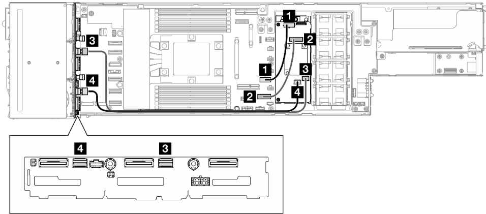
Figura 137. Disposición de los cables de RAID CFF
