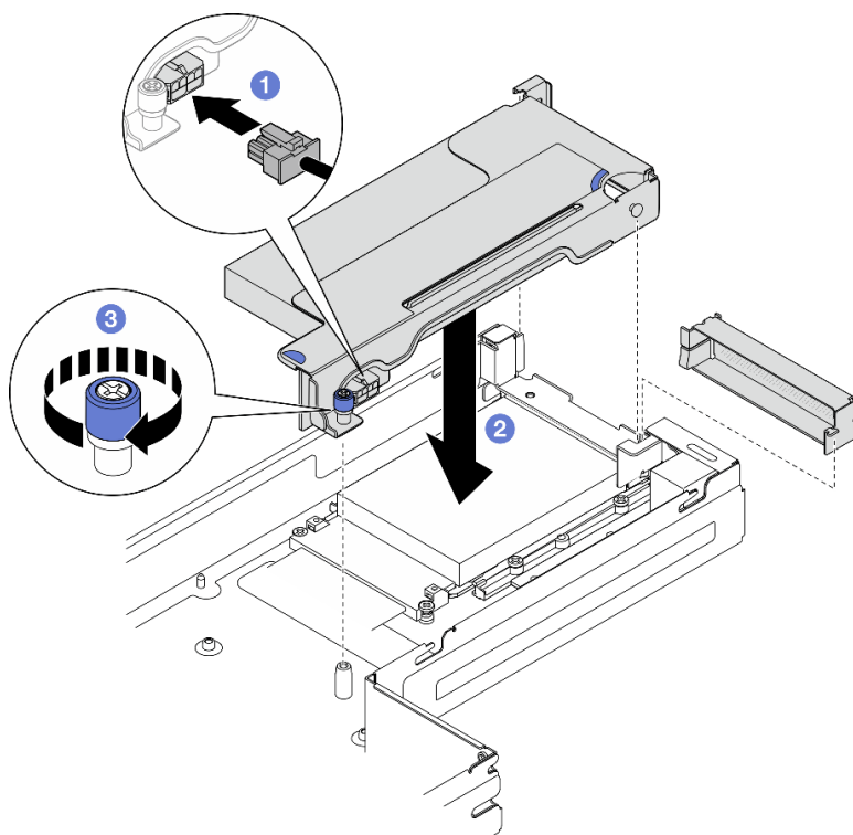
Figura 98. Instalación del conjunto de expansión PCIe
