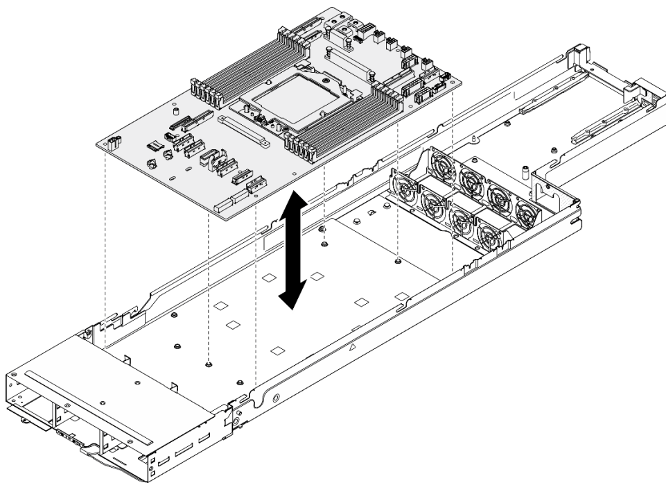
Figura 123. Instalación de la placa del sistema
