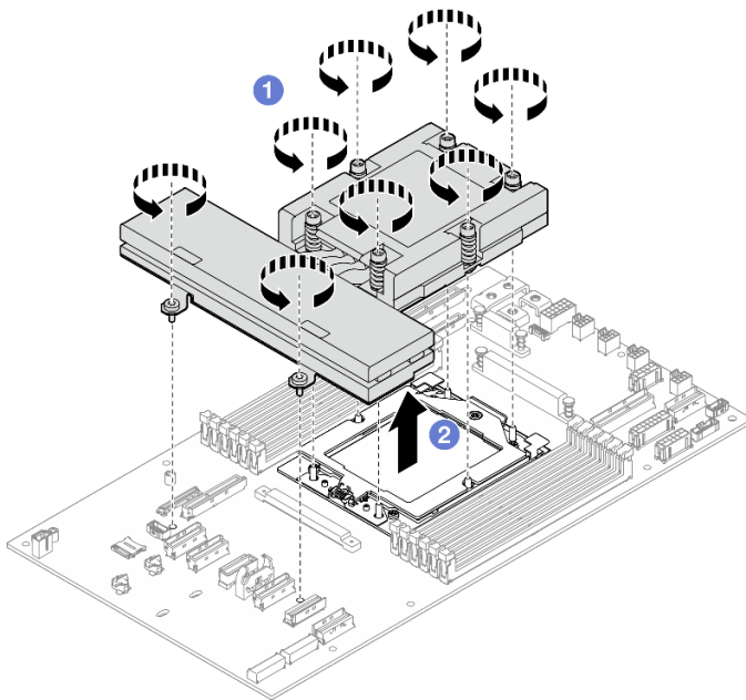
Figura 106. Extracción de un disipador de calor
