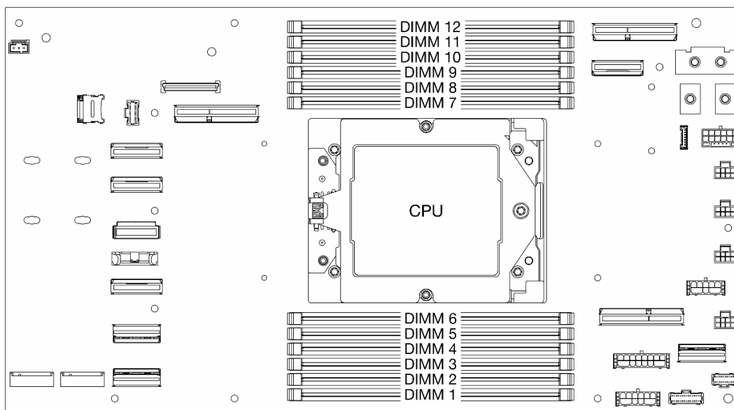
Figura 84. Diseño de los módulos de memoria y el procesador
