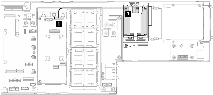
Figura 53. RAID CFF y cable del módulo de alimentación flash
