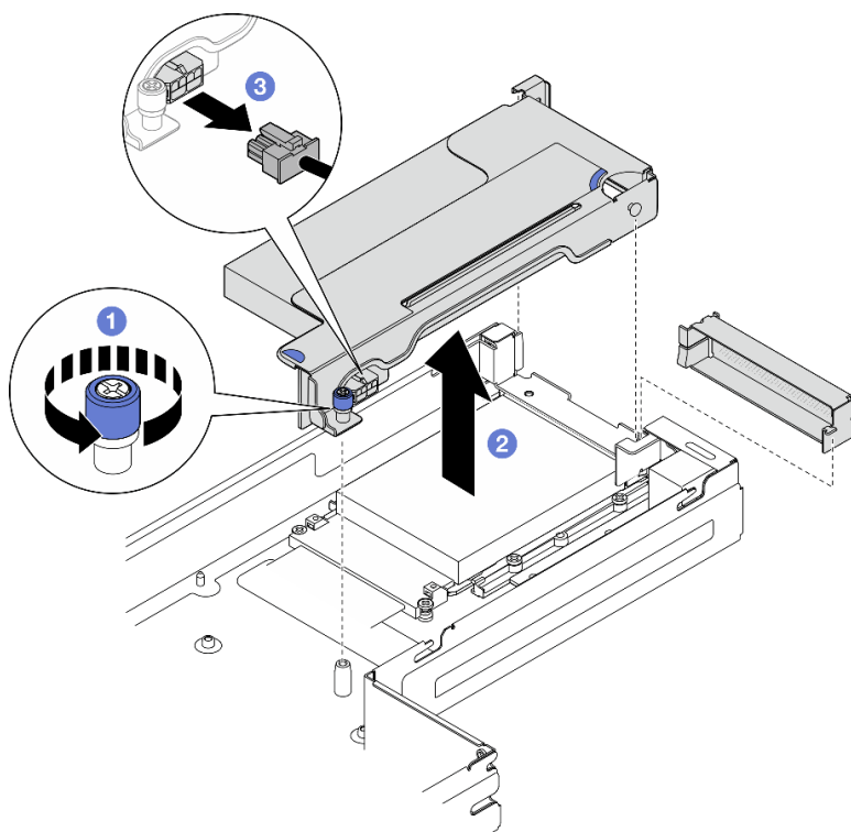
Figura 92. Extracción del conjunto de expansión PCIe
