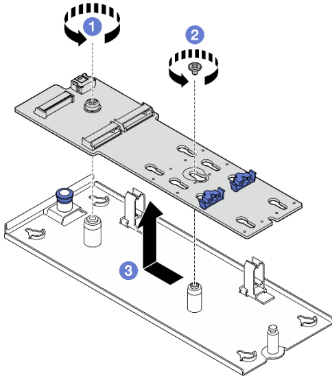
Figura 69. Extracción del adaptador de arranque M.2
