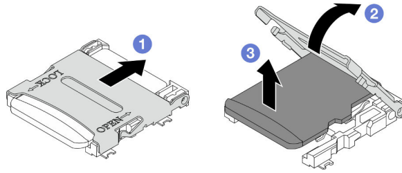
Figura 87. Extracción de la tarjeta MicroSD
