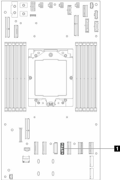
Figura 42. Ubicación del zócalo de la batería CMOS
