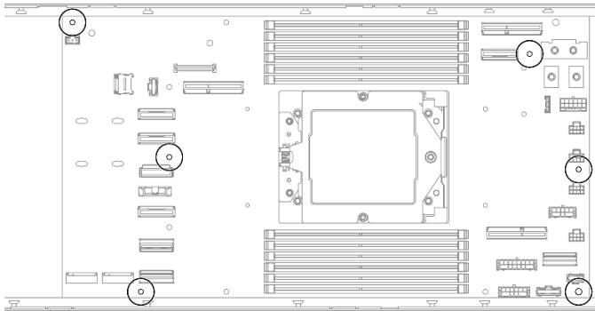
Figura 121. Extracción de los tornillos
