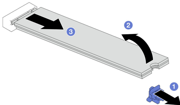
Figura 63. Extracción de una unidad M.2
