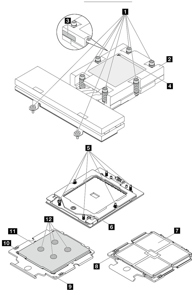
Figura 108. Componentes del procesador y el disipador de calor
