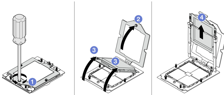
Figura 107. Extracción de un procesador
