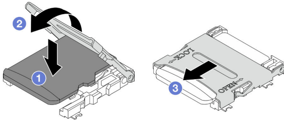
Figura 89. Instalación de una tarjeta MicroSD
