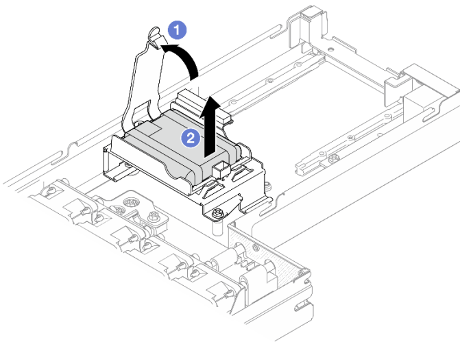
Figura 48. Extracción del módulo de alimentación flash
