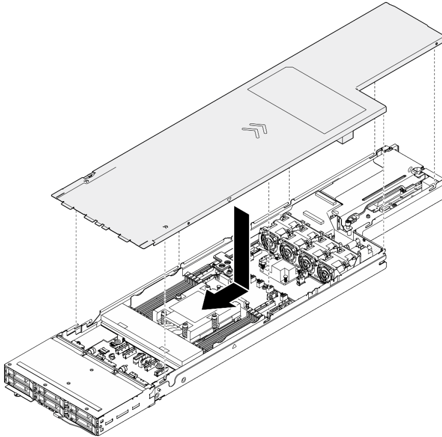
Figura 127. Instalación de la cubierta superior
