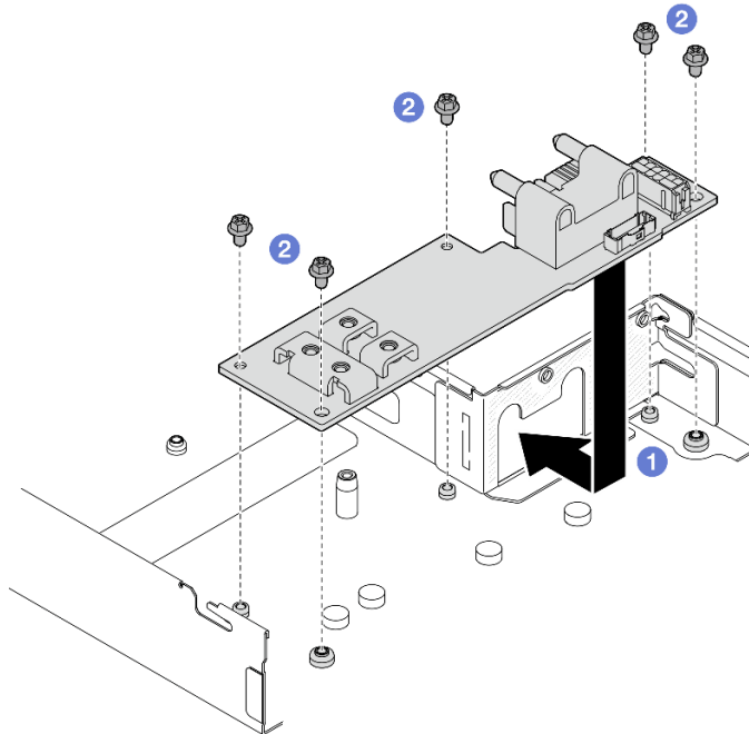
Figura 104. Instalación de una placa de distribución de alimentación
