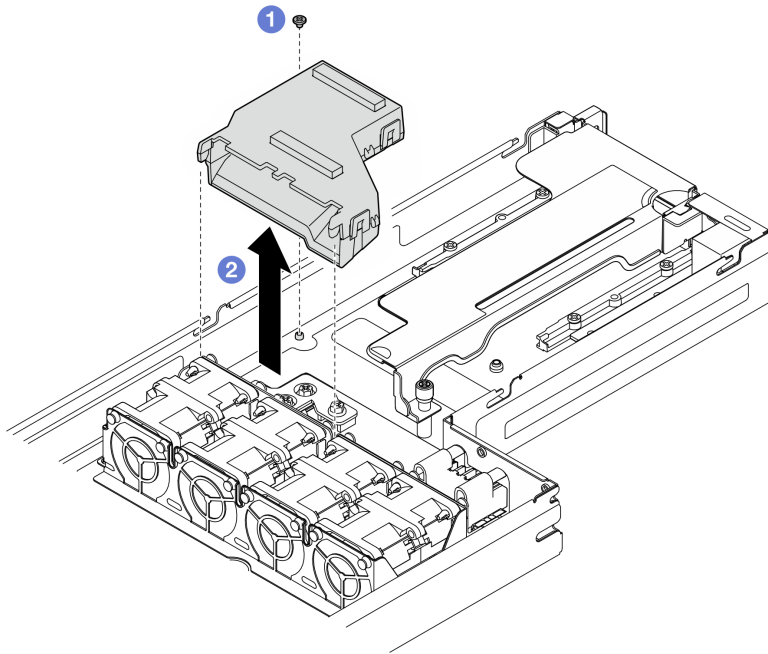
Figura 56. Extracción del conducto de aire de GPU
