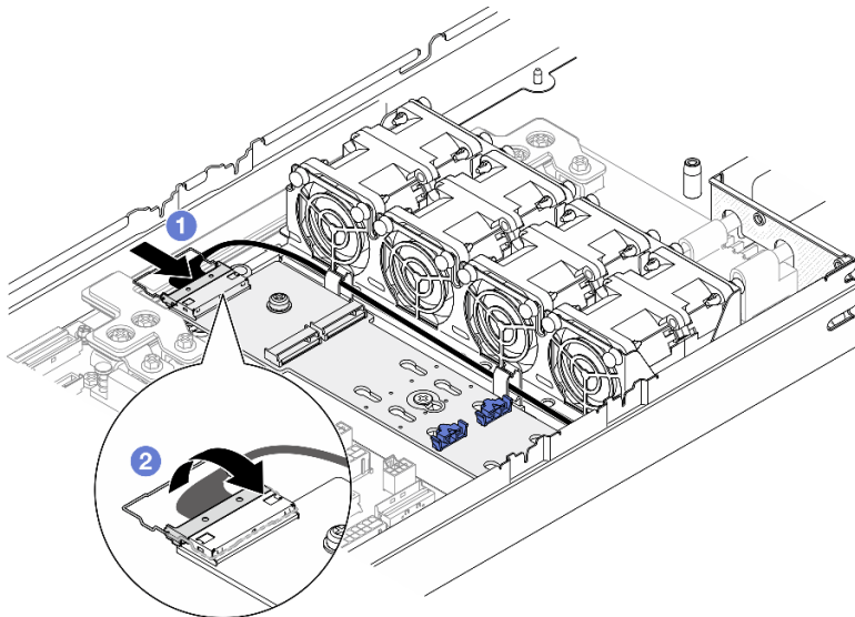
Figura 73. Conexión del cable al adaptador de arranque M.2 SATA/NVMe
