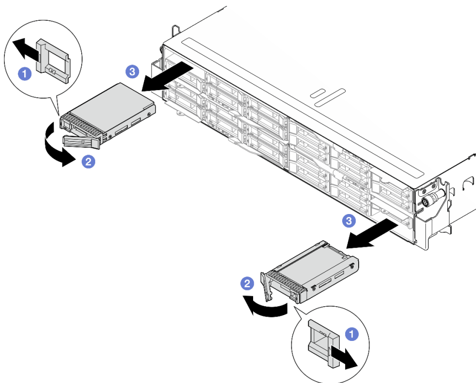
Figura 58. Extracción de la unidad de estado sólido
