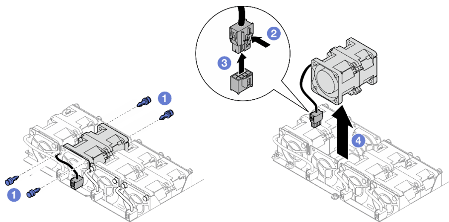
Figura 46. Extracción del ventilador
