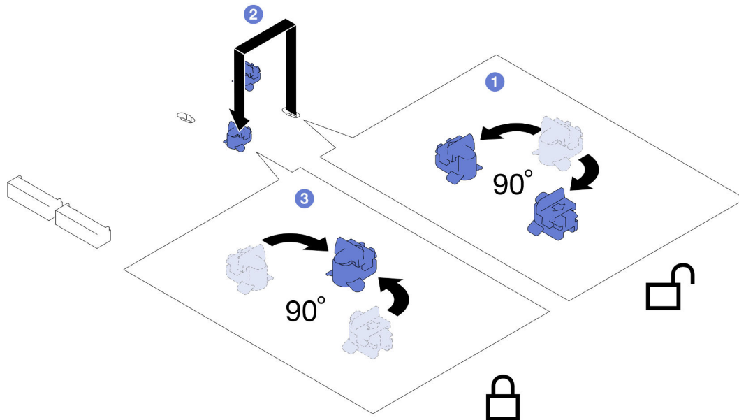
Figura 74. Ajuste de un elemento de sujeción de la unidad M.2
