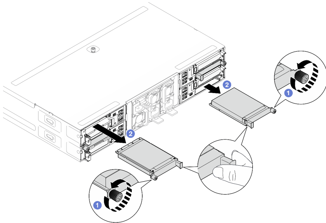
Figura 90. Extracción del módulo de OCP posterior
