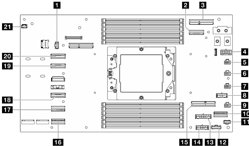
Figura 128. Conectores de la placa del sistema para la disposición de los cables
