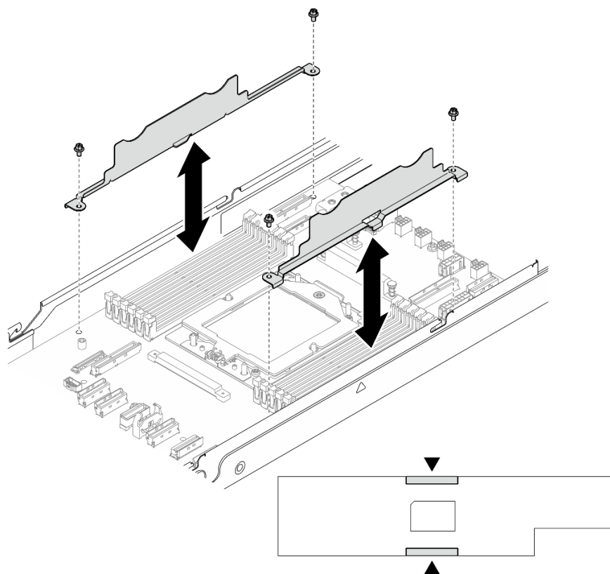
Figura 125. Sustitución de pared para cable
