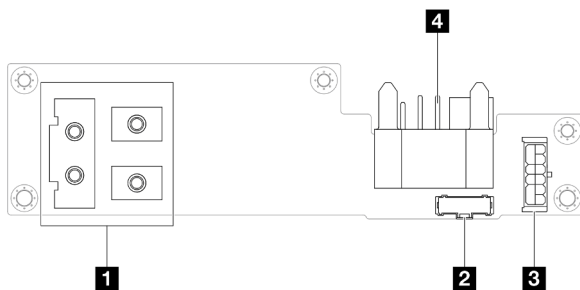
Figura 133. Conectores de placa de distribución de alimentación
