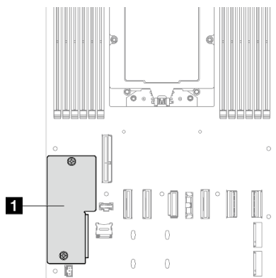
Figura 116. Ubicación del Firmware y módulo de seguridad de RoT
