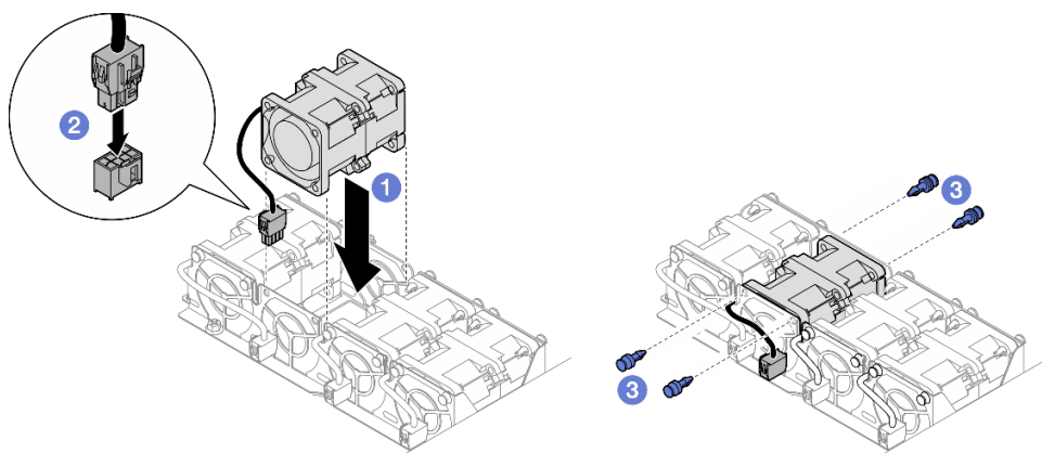
Figura 47. Instalación de ventilador
