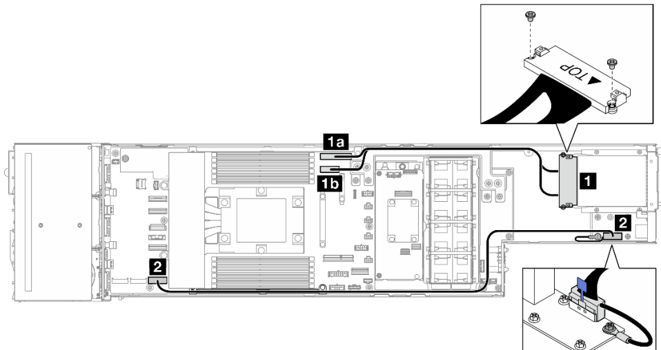
Figura 146. Cables para el módulo de E/S posterior y el módulo OCP
