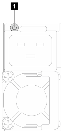
Figura 153. LED de fuente de alimentación
