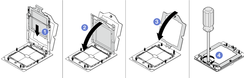
Figura 109. Instalación de un procesador
