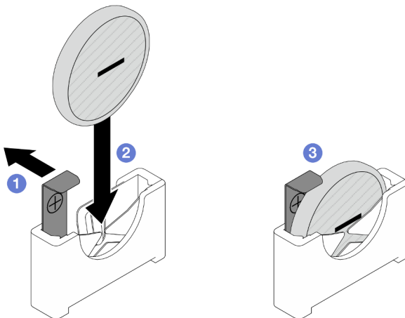
Figura 43. Instalación de una batería CMOS
