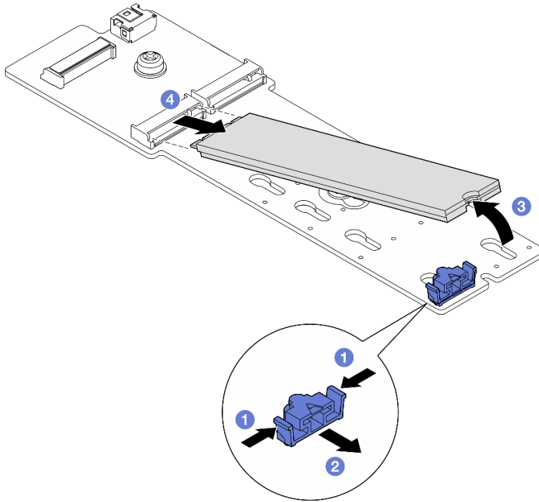
Figura 65. Extracción de una unidad M.2
