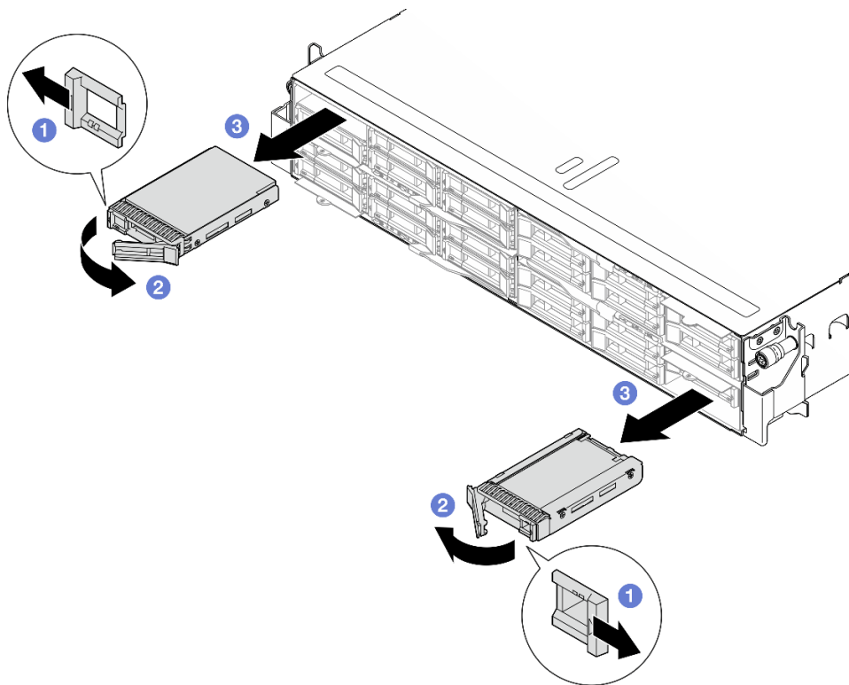
Figure 44. Retrait d'une unité SSD
