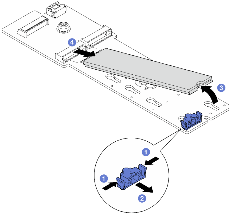
Figure 51. Retrait d'une unité M.2
