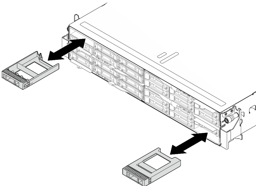
Figure 46. Remplacement d'un obturateur d'unité
