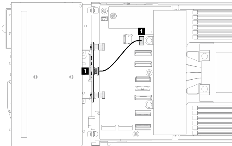
Figure 128. Cheminement des câbles de la carte d'E-S avant
