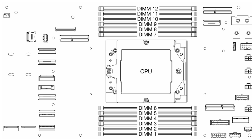
Figure 1. Disposition des modules de mémoire et des processeurs
