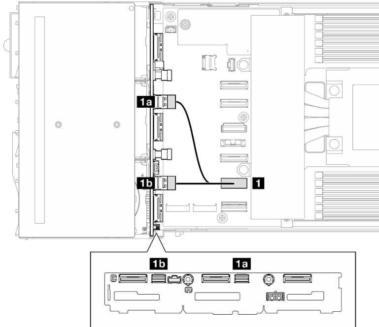
Figure 122. Cheminement des câbles SATA intégré
