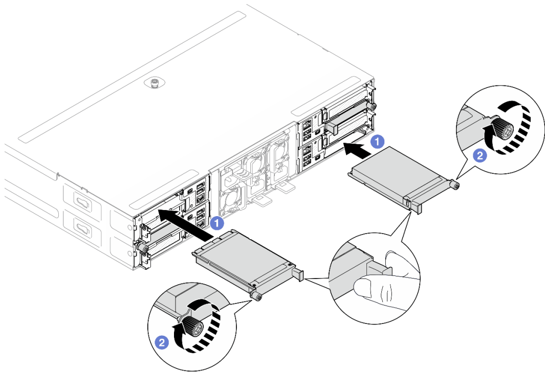
Figure 77. Installation du module OCP arrière
