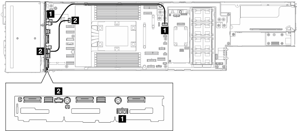
Figure 120. Bande latérale du fond de panier d'unité et cheminement des câbles d'alimentation
