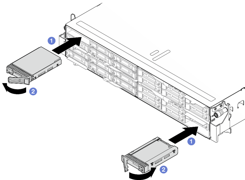
Figure 47. Installation d'un disque SSD
