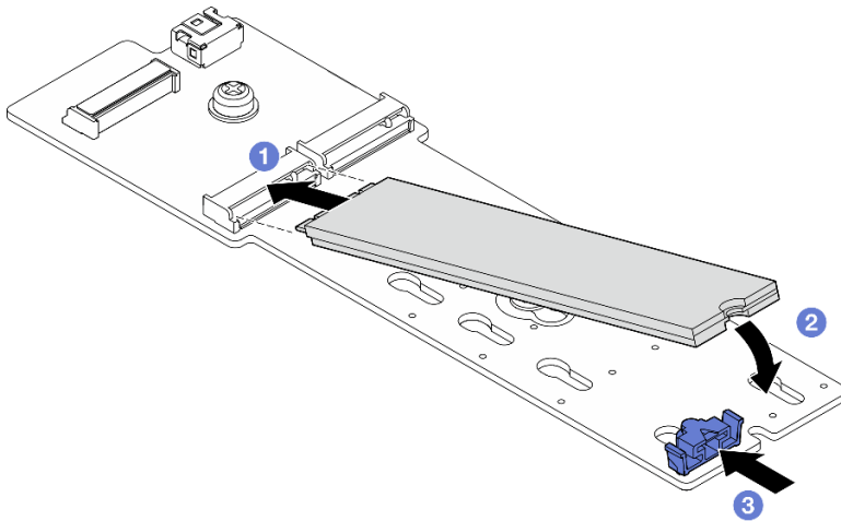
Figure 67. Installation d'une unité M.2
