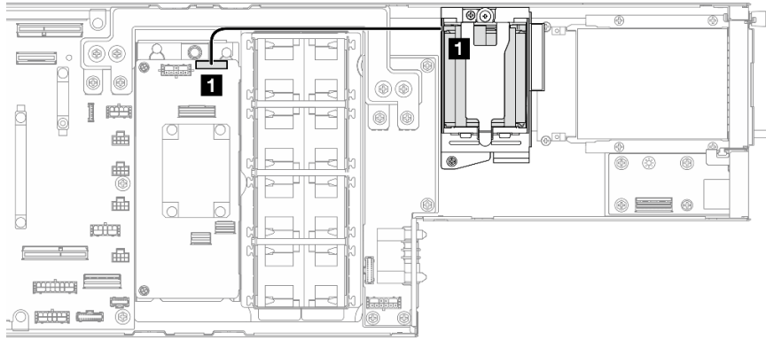
Figure 125. Cheminement du module d'alimentation flash
