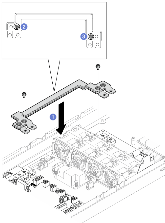
Figure 87. Installation de la barre-bus d'alimentation
