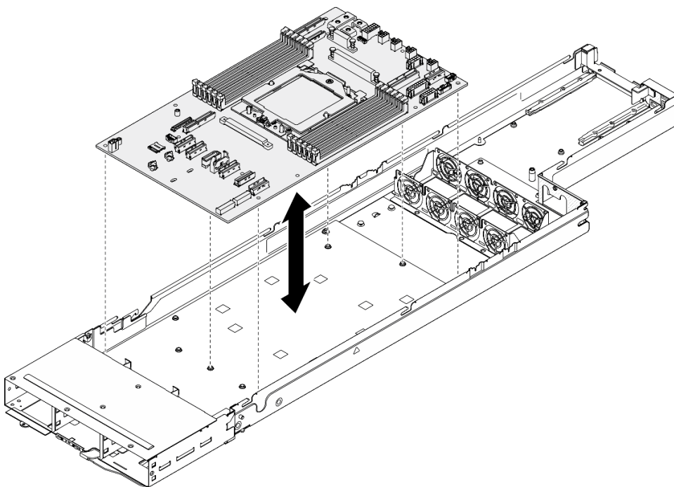
Figure 108. Retrait de la carte mère
