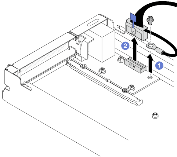
Figure 98. Retrait du câble d'E-S arrière et du câble de mise à la terre
