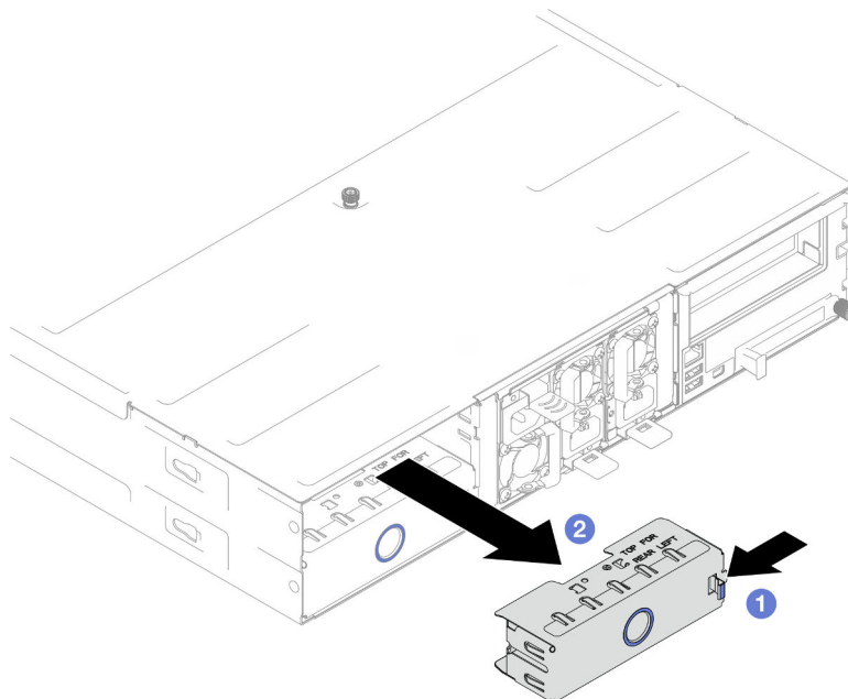
Figure 21. Retrait d'un obturateur de plateau de nœud arrière
