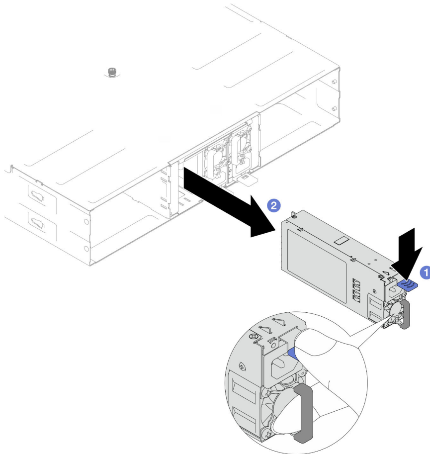
Figure 8. Retrait d'un PSU remplaçable à chaud
