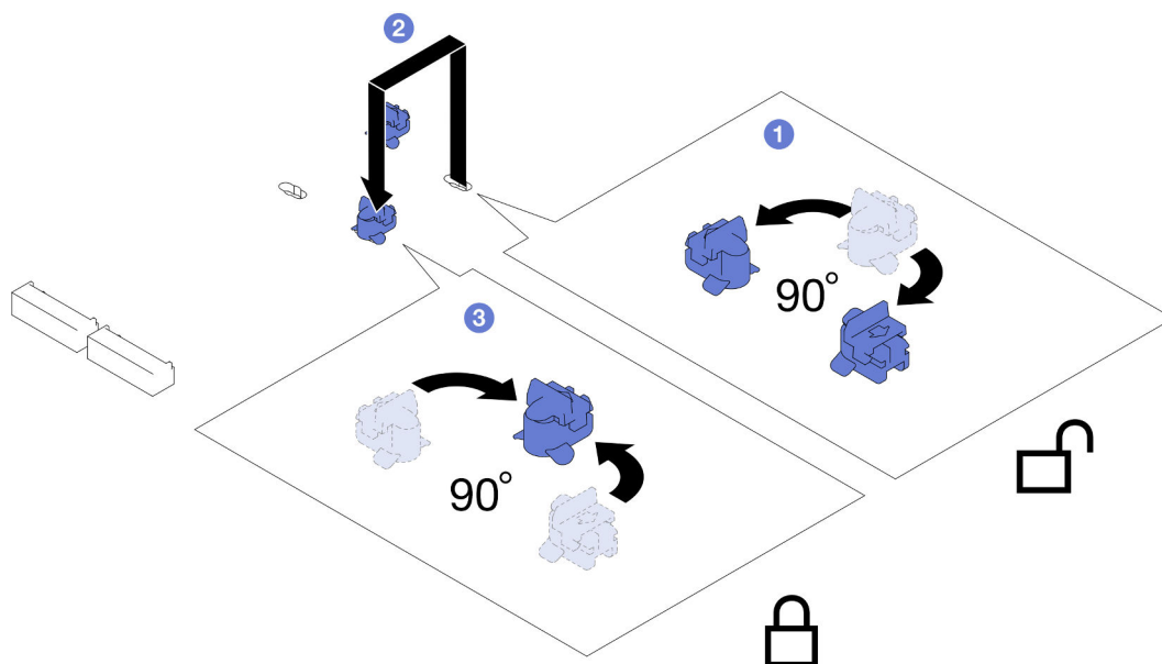
Figure 60. Ajustement d'un dispositif de retenue du disque M.2
