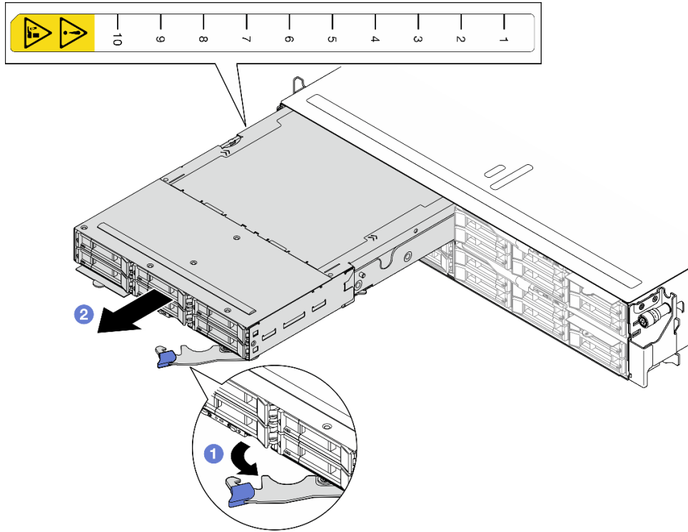
Figure 16. Retrait du nœud d'un plateau de gauche
