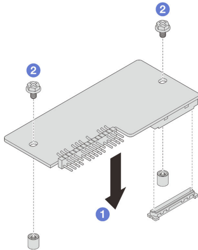
Figure 105. Installation du module de microprogramme et de sécurité RoT
