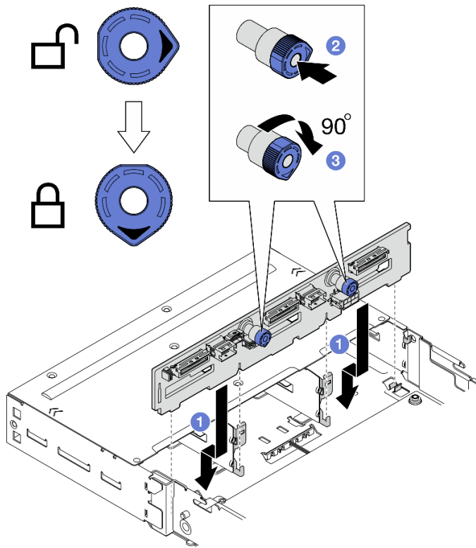
Figure 31. Installation du fond de panier d'unité
