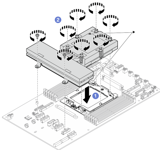
Figure 97. Installation d'un dissipateur thermique
