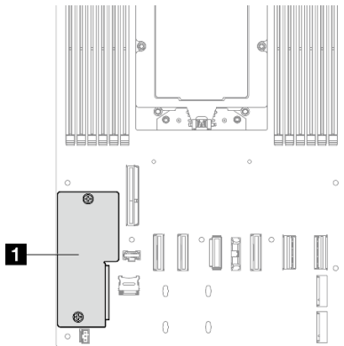
Figure 104. Emplacement du Module de microprogramme et de sécurité RoT
