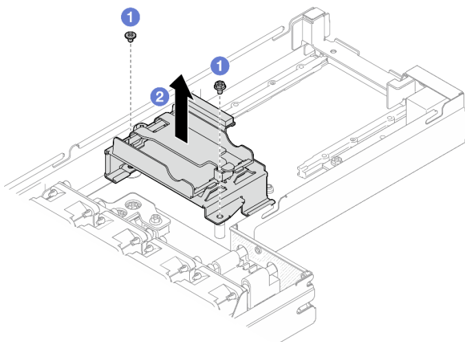
Figure 35. Retrait du support du module d'alimentation flash
