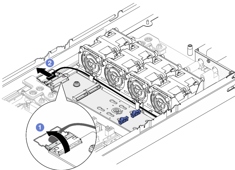
Figure 53. Déconnexion du câble de l'adaptateur d'amorçage SATA/NVMe M.2
