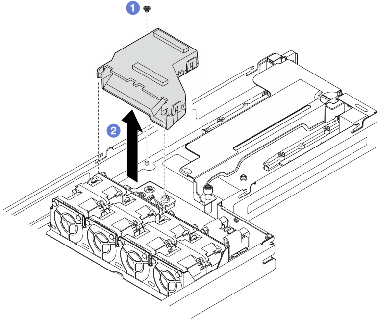
Figure 42. Retrait du conduit de ventilation du GPU
