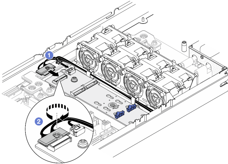
Figure 58. Connexion du câble à l'adaptateur d'amorçage NVMe M.2
