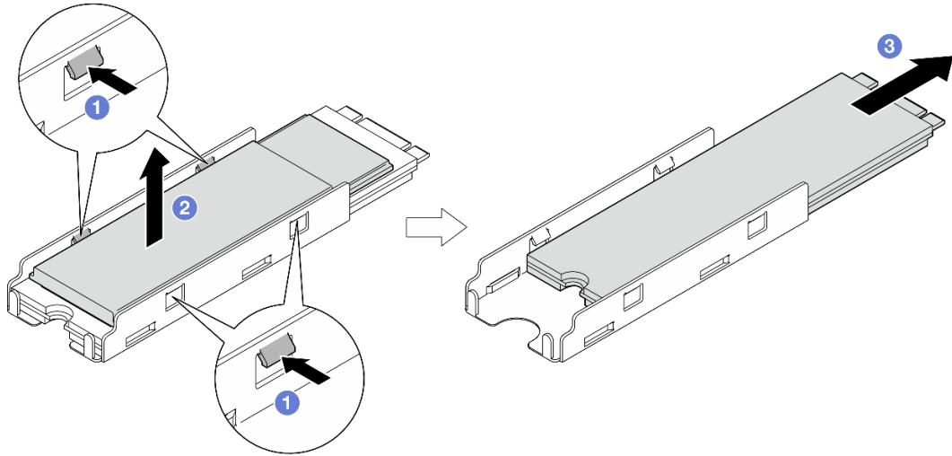
Figure 50. Retrait du dissipateur thermique M.2
