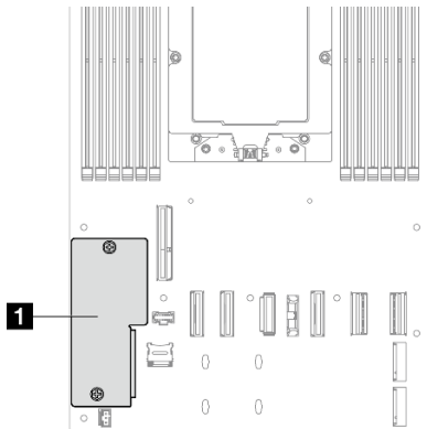
Figure 102. Emplacement du Module de microprogramme et de sécurité RoT
