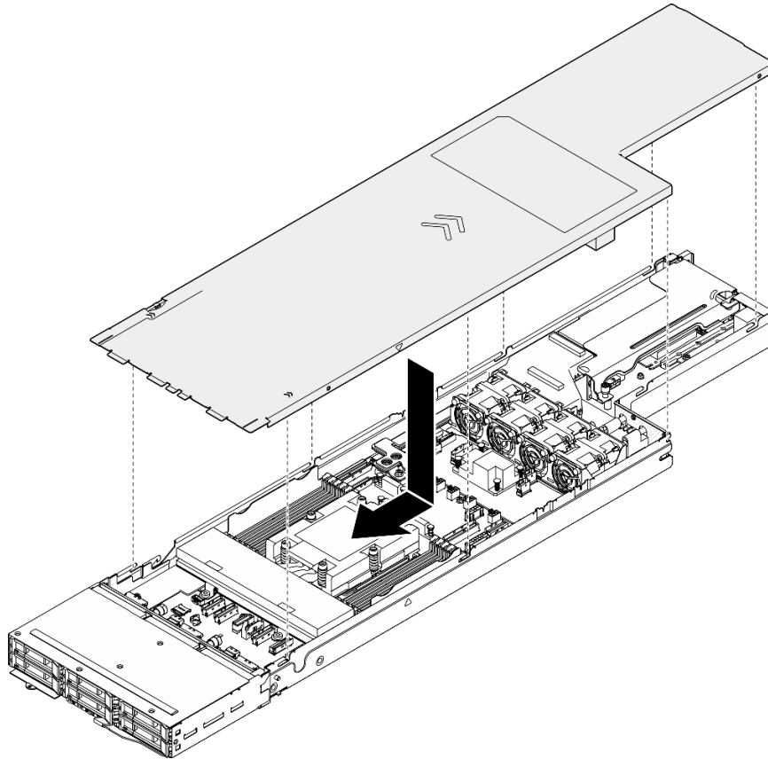
Figure 113. Installation du carter supérieur
