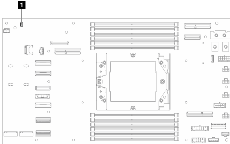
Figure 141. Voyants de la carte mère
