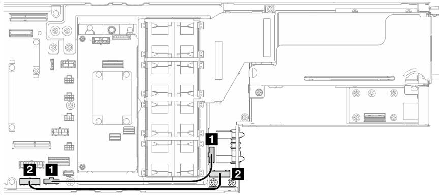
Figure 131. Cheminement des câbles pour le tableau de distribution
