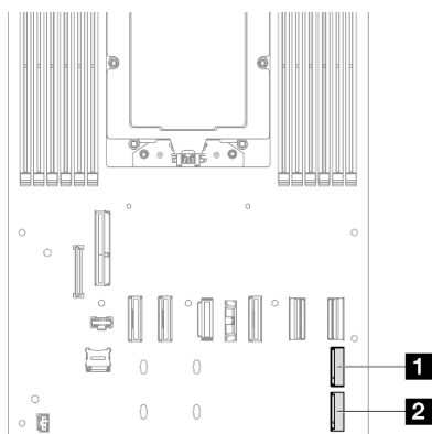
Figure 48. Emplacement des baies M.2 sur la carte mère
