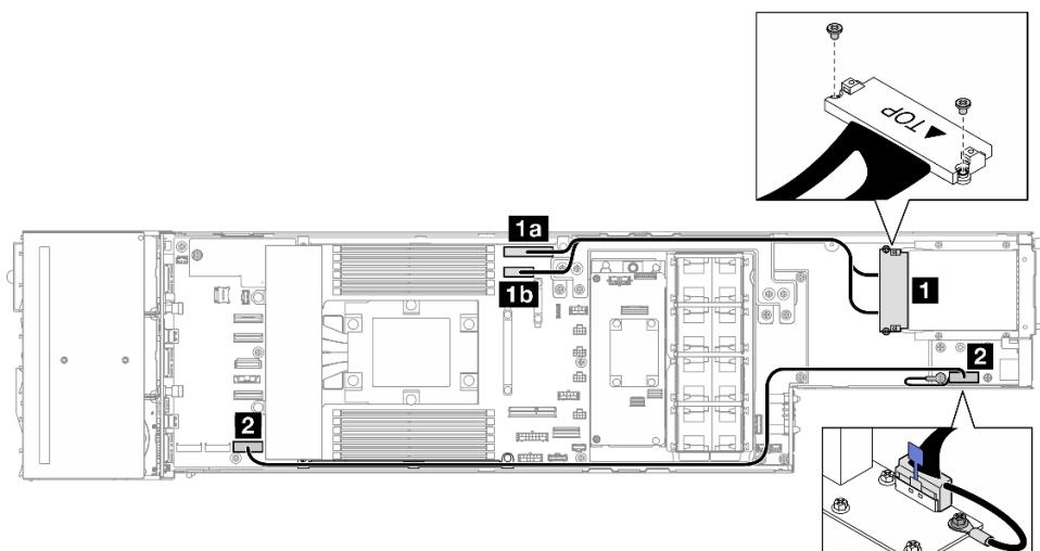
Figure 132. Câbles pour le module OCP et d'E-S arrière
