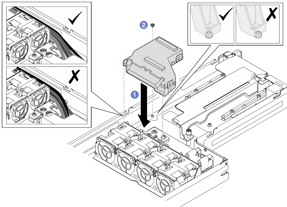
Figure 43. Installation du conduit de ventilation du GPU
