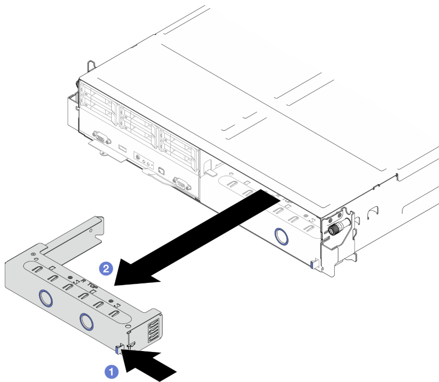
Figure 20. Retrait d'un obturateur de plateau de nœud avant
