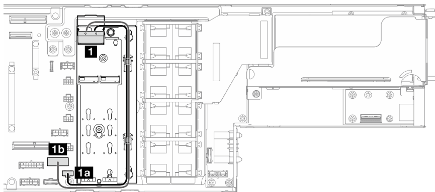
Figure 129. Cheminement des câbles pour l'adaptateur d'amorçage SATA/NVMe M.2
