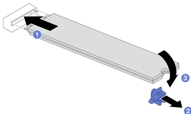
Figure 65. Installation d'une unité M.2
