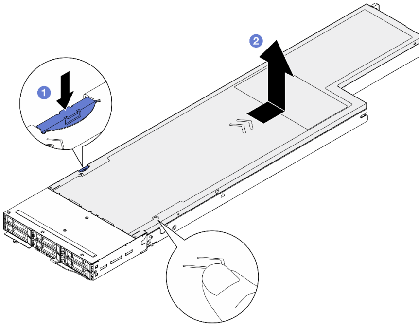
Figure 112. Retrait du carter supérieur
