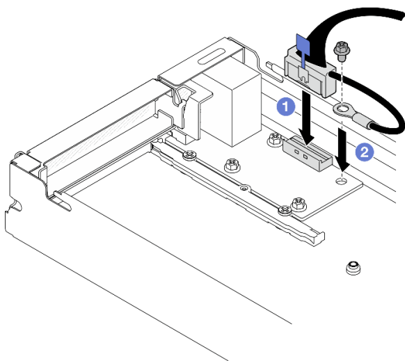
Figure 133. Installation du câble d'E-S arrière et du câble de mise à la terre
