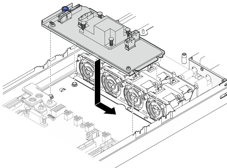
Figure 25. Installation de l'adaptateur RAID CFF interne
