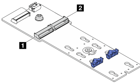
Figure 66. Emplacements des unités M.2
