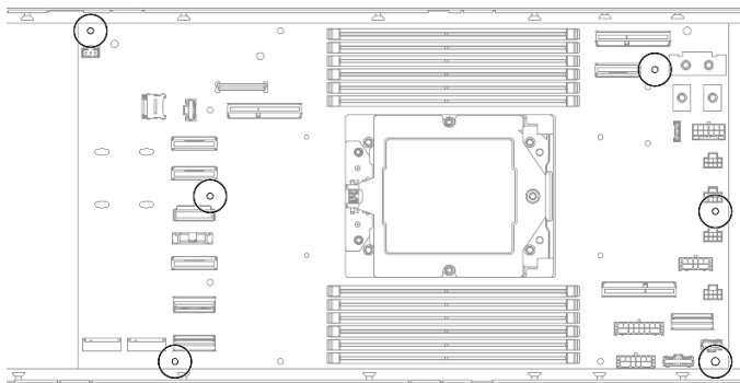
Figure 107. Retrait des vis
