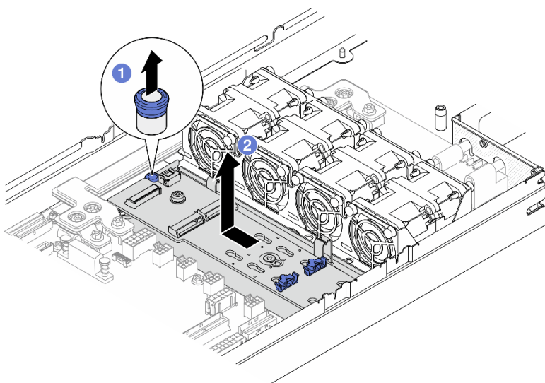
Figure 54. Retrait du plateau de l'adaptateur d'amorçage M.2
