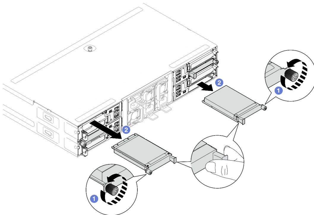
Figure 76. Retrait du module OCP arrière
