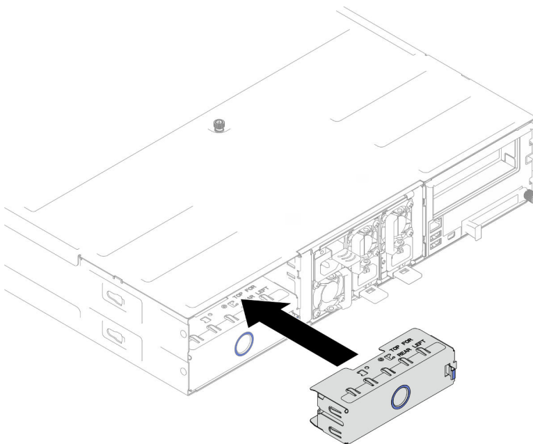
Figure 19. Installation d'un obturateur de plateau de nœud arrière
