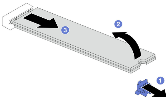
Figure 49. Retrait d'une unité M.2
