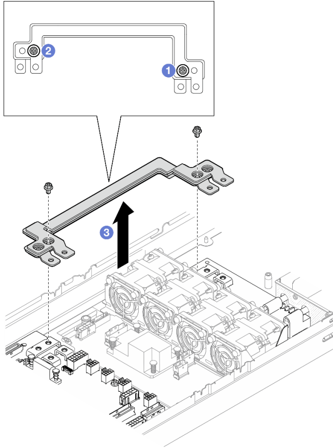
Figure 86. Retrait de la barre-bus d'alimentation
