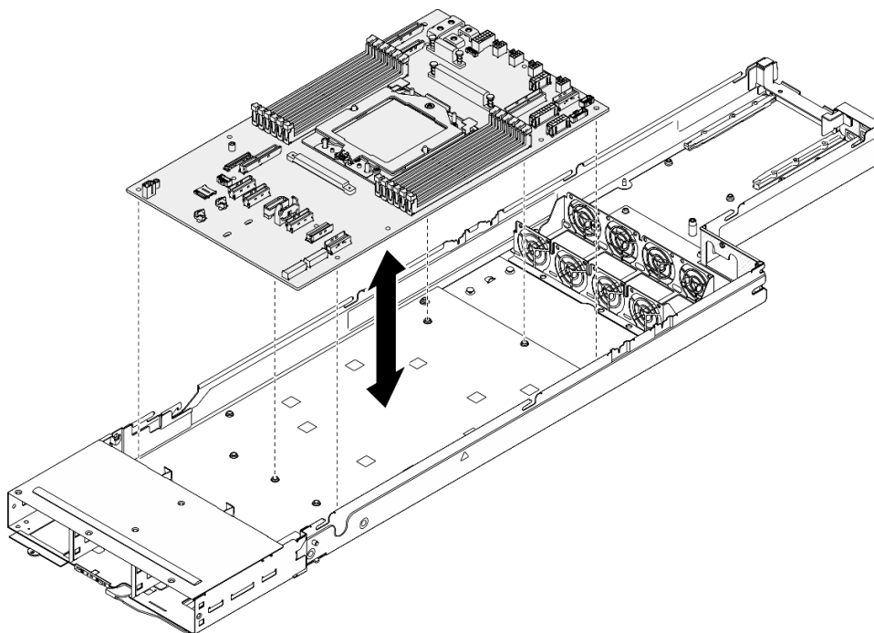
Figure 109. Installation de la carte mère
