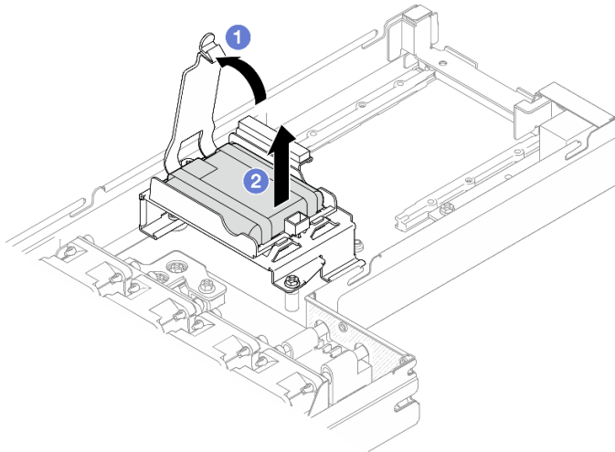
Figure 34. Retrait du module d'alimentation flash
