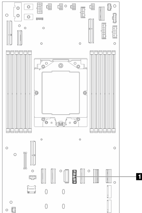
Figure 26. Emplacement du socket de la pile CMOS
