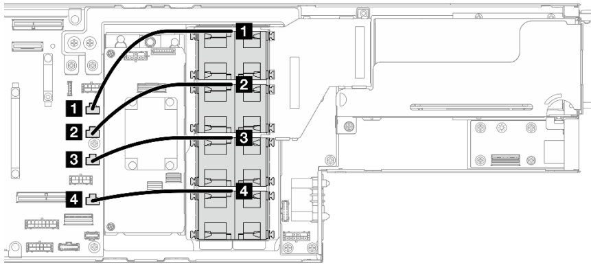
Figure 127. Cheminement des câbles de ventilateur
