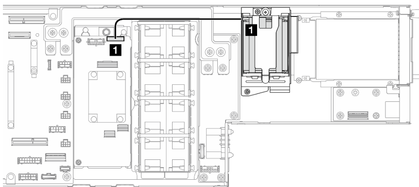
Figure 39. Câble du module d'alimentation flash et RAID CFF
