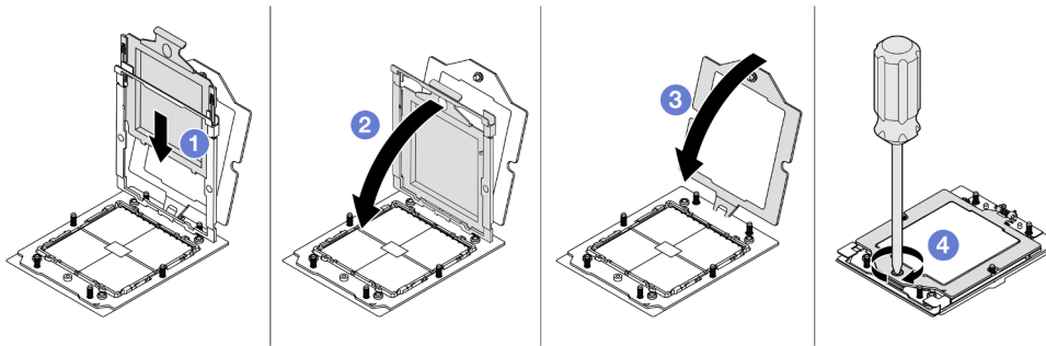
Figure 95. Installation d'un processeur
