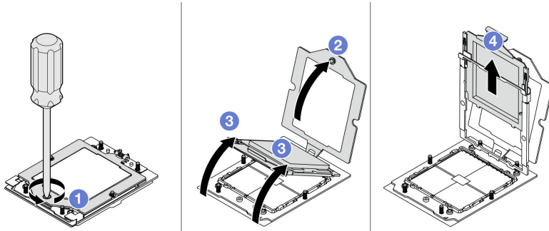
Figure 93. Retrait d'un processeur
