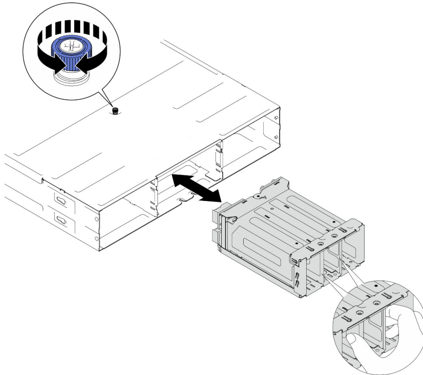
Figure 15. Installation du boîtier de PSU
