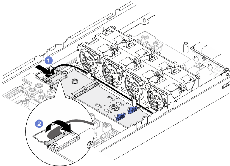
Figure 59. Connexion du câble à l'adaptateur d'amorçage SATA/NVMe M.2
