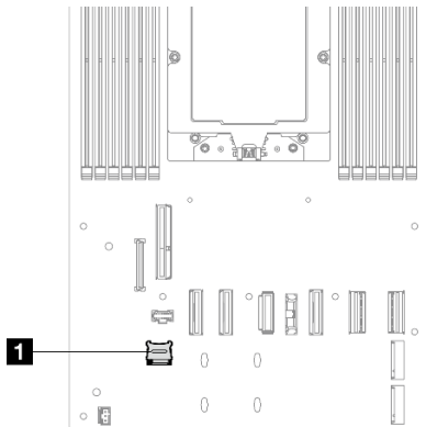
Figure 74. Emplacement du socket MicroSD
