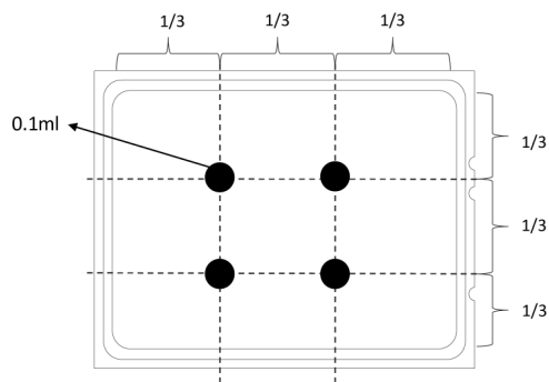
Figure 96. Application de pâte thermoconductrice
