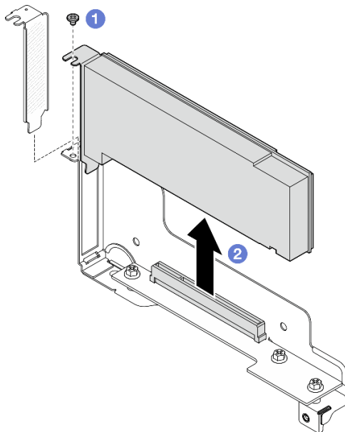
Figure 80. Retrait d'un adaptateur PCIe
