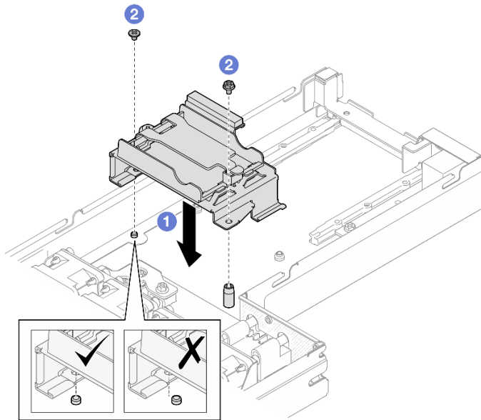
Figure 36. Installation du support du module d'alimentation flash
