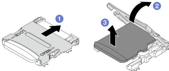
Figure 73. Retrait de la carte MicroSD
