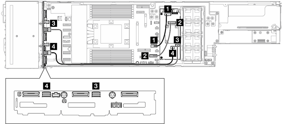
Figure 123. Cheminement des câbles RAID CFF
