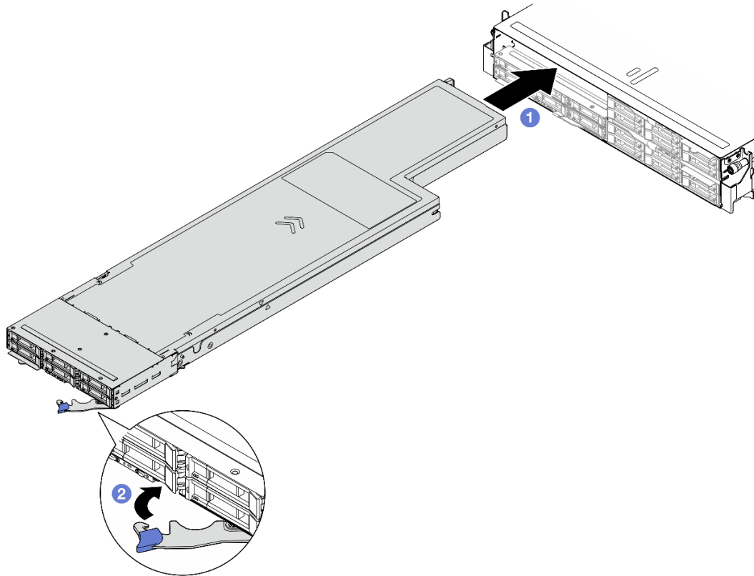
Figure 22. Installation du nœud dans un plateau de gauche
