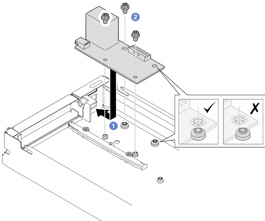
Figure 100. Installation du module d'E-S arrière
