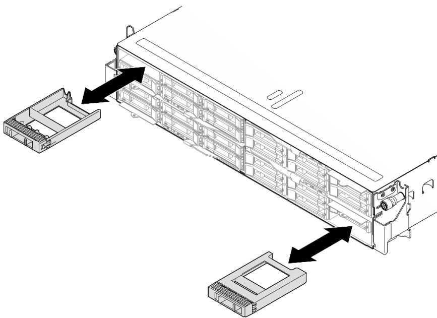
Figure 45. Remplacement d'un obturateur d'unité
