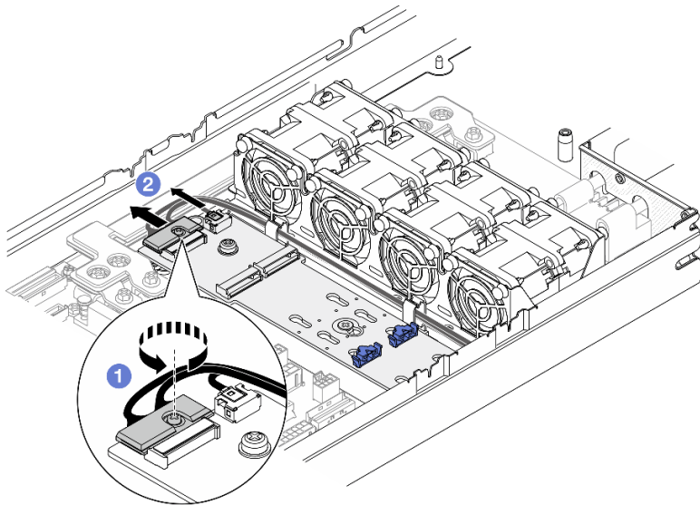
Figure 52. Déconnexion du câble de l'adaptateur d'amorçage NVMe M.2
