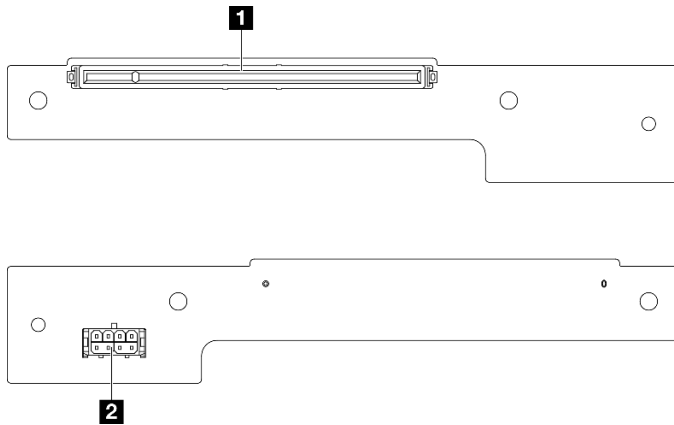
Figure 118. Connecteurs de carte mezzanine PCIe
