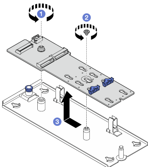
Figure 55. Retrait de l'adaptateur d'amorçage M.2
