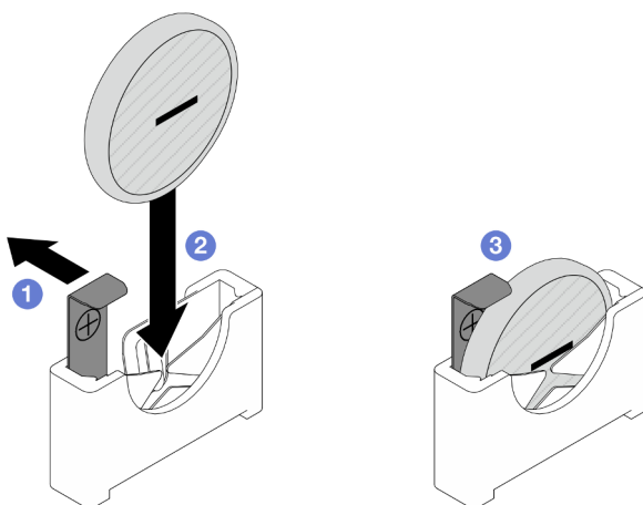
Figure 29. Installation d'une pile CMOS
