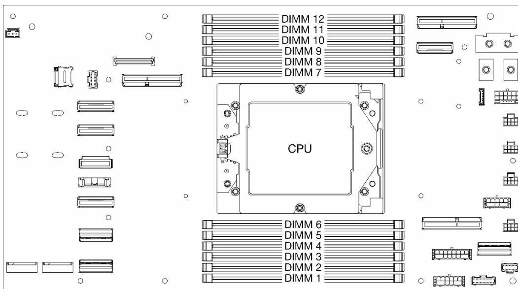
Figure 70. Disposition des modules de mémoire et des processeurs
