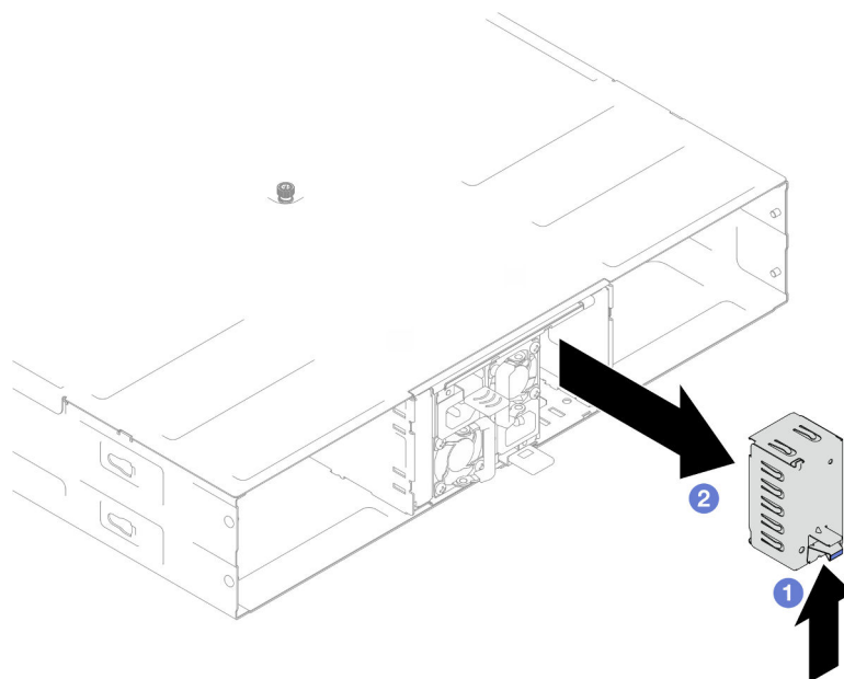
Figure 10. Retrait d'un obturateur de PSU
