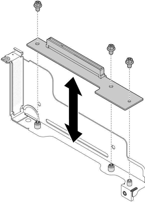
Figure 79. Remplacement de la carte mezzanine PCIe
