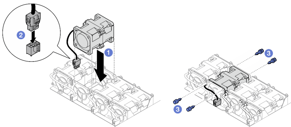
Figure 33. Installation du ventilateur
