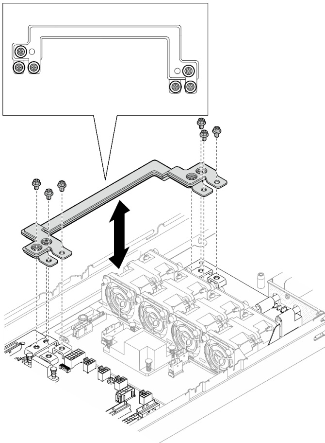
Figure 85. Retrait des vis externes de la barre-bus d'alimentation
