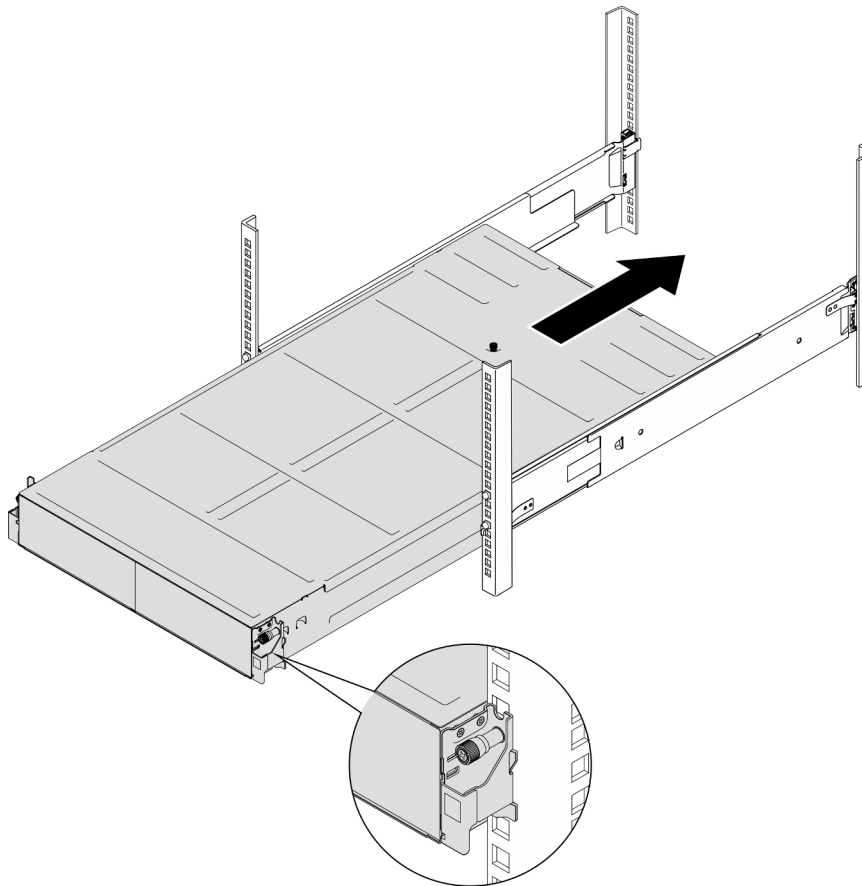
Figure 4. Installation du châssis
