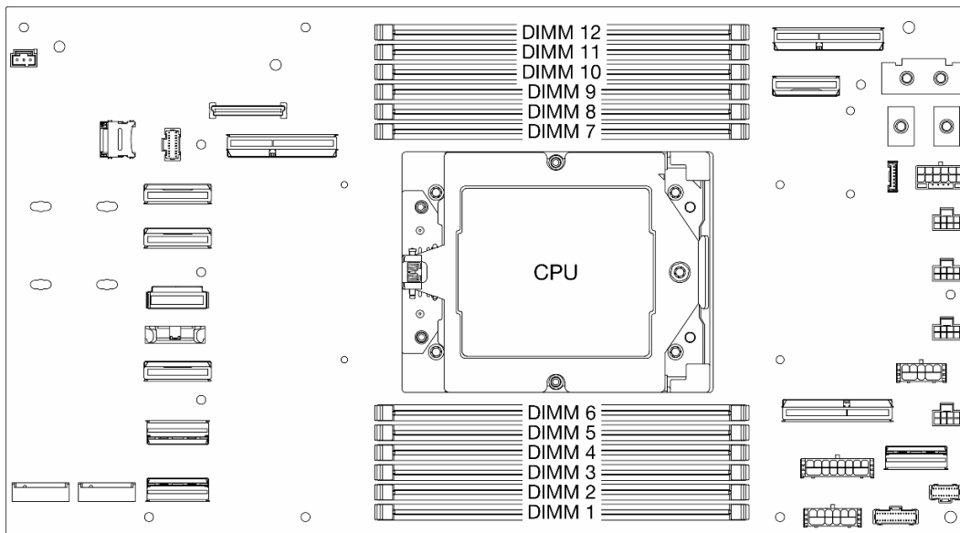
Figure 68. Disposition des modules de mémoire et des processeurs
