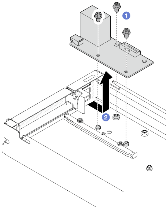
Figure 99. Retrait du module d'E-S arrière
