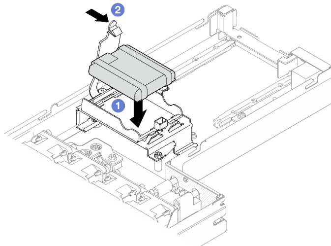
Figure 37. Installation du module d'alimentation flash
