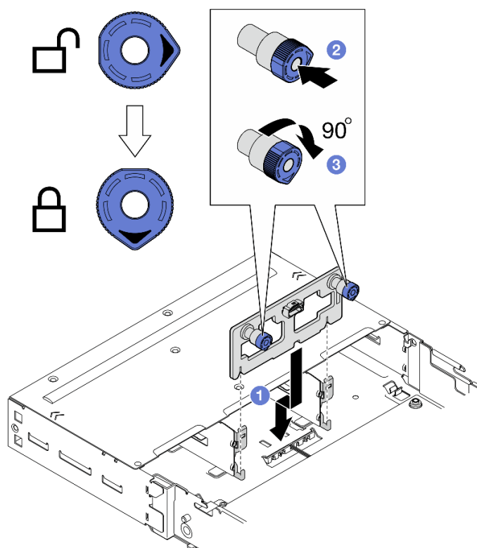
Figure 41. Installation du fond de panier d'E-S avant
