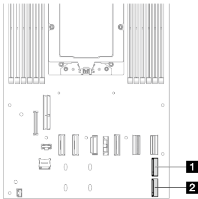
Figure 62. Emplacement des baies M.2 sur la carte mère
