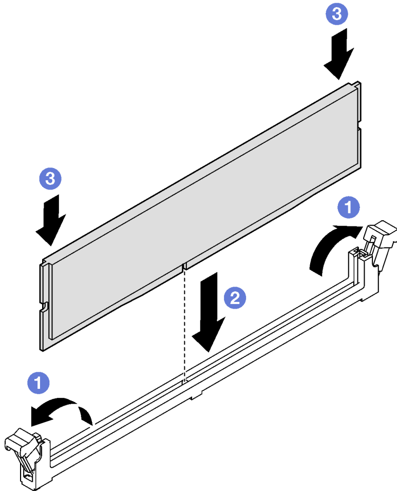
Figure 71. Installation d'un module de mémoire
