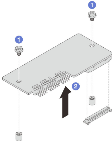
Figure 103. Retrait du Module de microprogramme et de sécurité RoT
