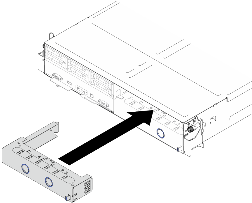
Figure 18. Installation d'un obturateur de plateau de nœud avant
