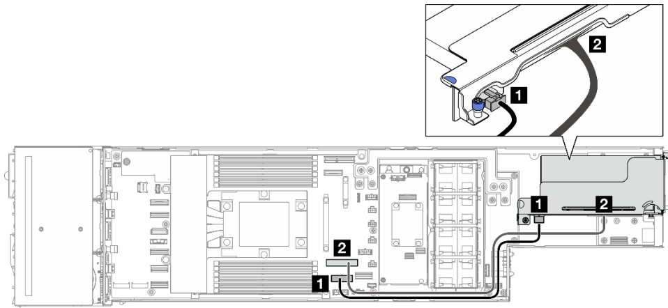
Figure 130. Cheminement des câbles de la carte mezzanine PCIe
