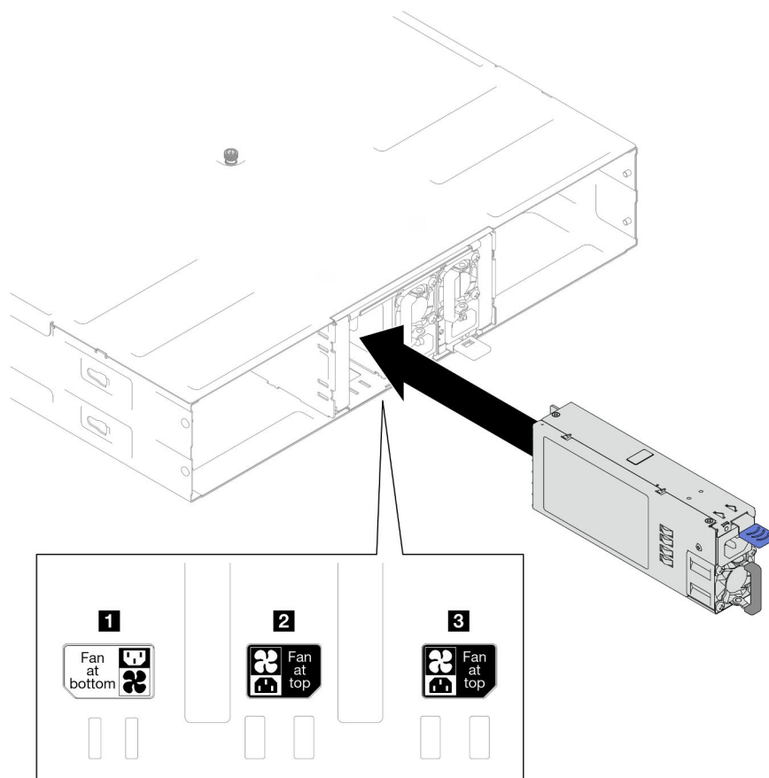
Figure 11. Installation d'un bloc d'alimentation remplaçable à chaud
