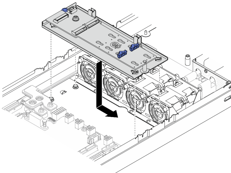
Figure 57. Installation du plateau de l'adaptateur d'amorçage M.2
