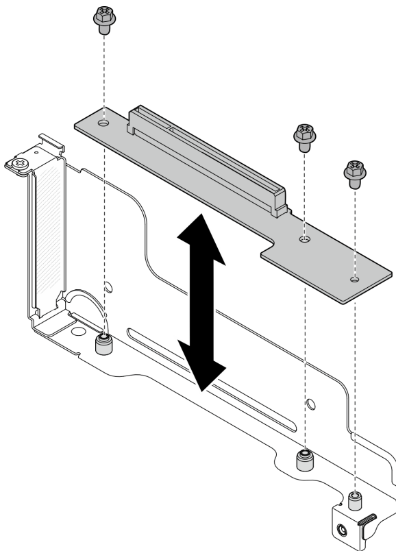
Figure 81. Remplacement de la carte mezzanine PCIe
