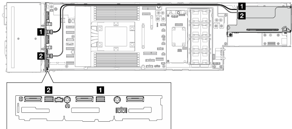
Figure 126. Cheminement des câbles SATA/SAS pour adaptateur PCIe RAID 8i
