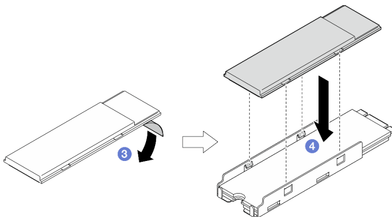
Figure 64. Installation d'un dissipateur thermique M.2 dans le plateau M.2
