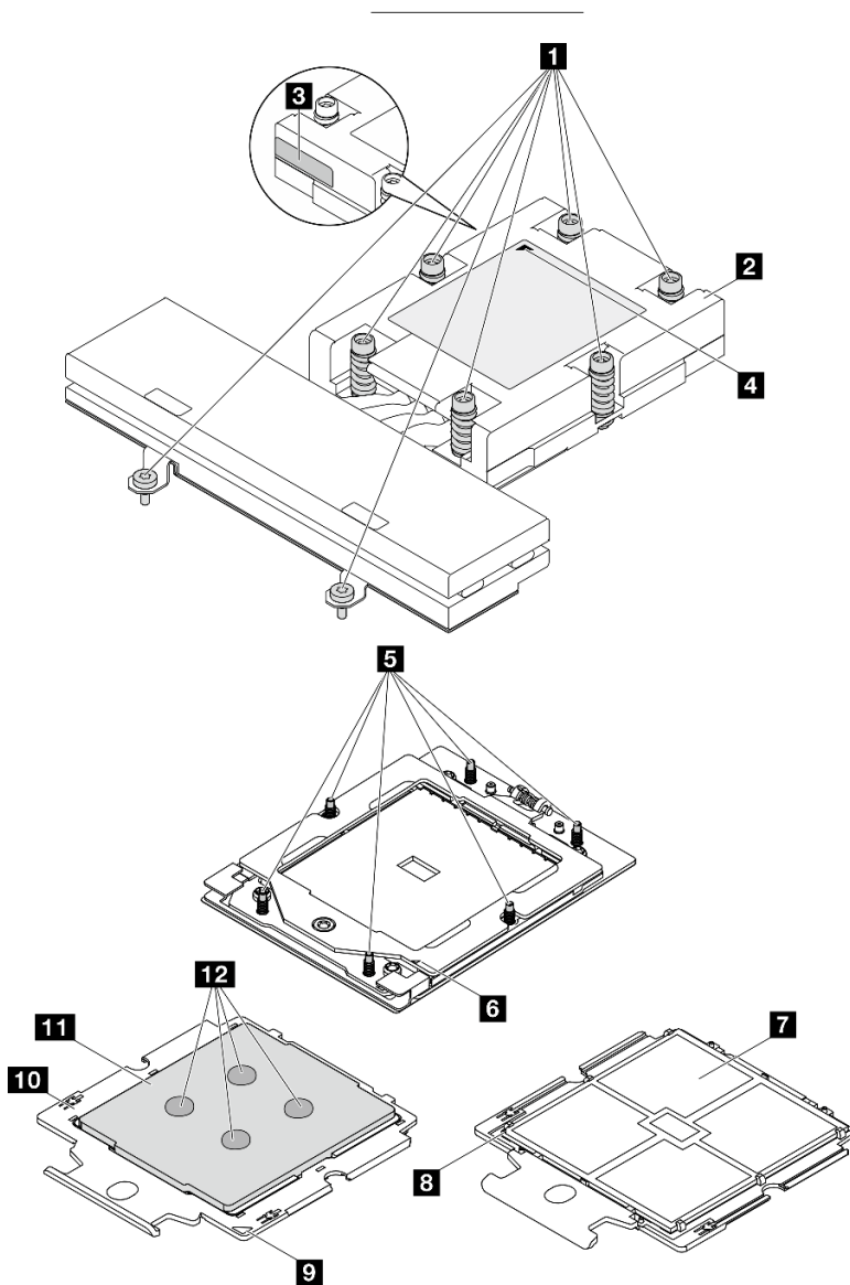
Figure 91. Composants du processeur et dissipateur thermique
