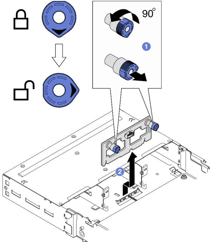
Figure 40. Retrait du fond de panier d'E-S avant
