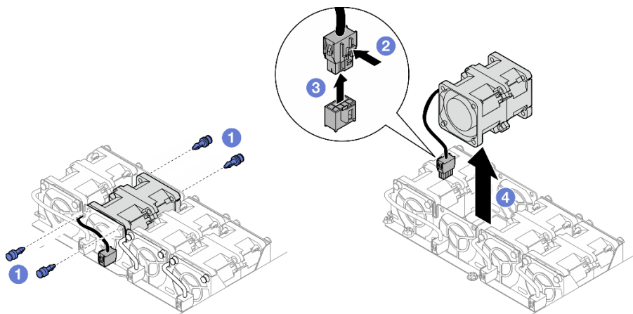
Figure 32. Retrait du ventilateur
