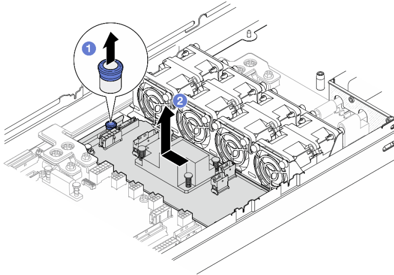
Figure 24. Retrait de l'adaptateur RAID CFF interne
