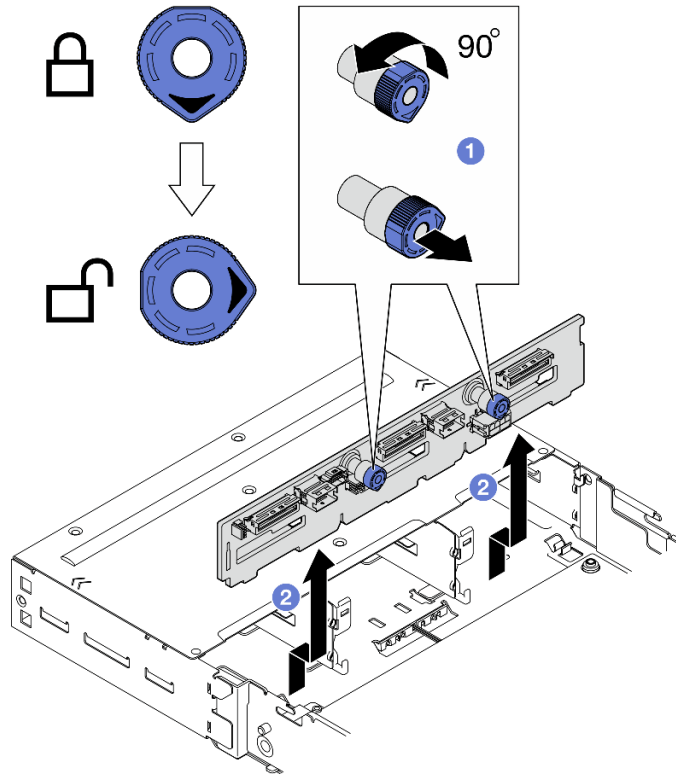
Figure 30. Retrait du fond de panier d'unité
