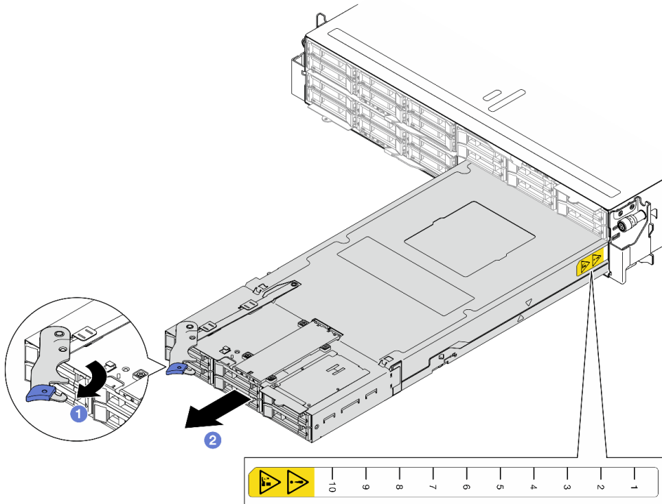
Figure 17. Retrait du nœud d'un plateau de droite
