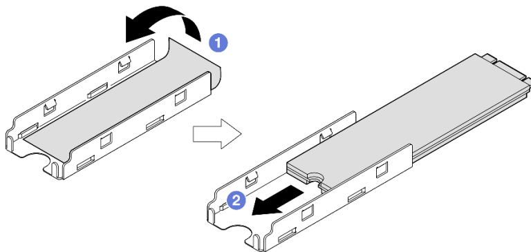
Figure 63. Installation d'un tampon thermique et d'une unité M.2 dans le plateau
