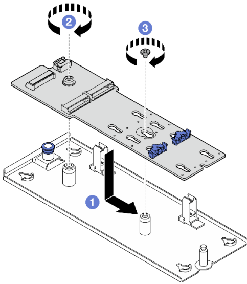
Figure 56. Installation de l'adaptateur d'amorçage M.2
