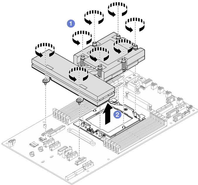
Figure 92. Retrait d'un dissipateur thermique
