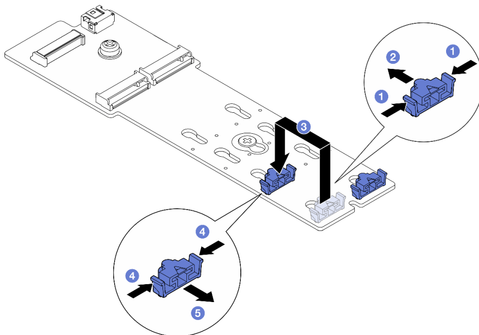
Figure 61. Ajustement du crochet de retenue M.2
