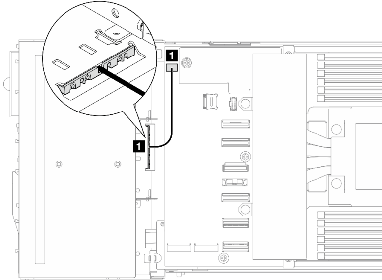
Figure 134. Cheminement des câbles du capteur thermique avant
