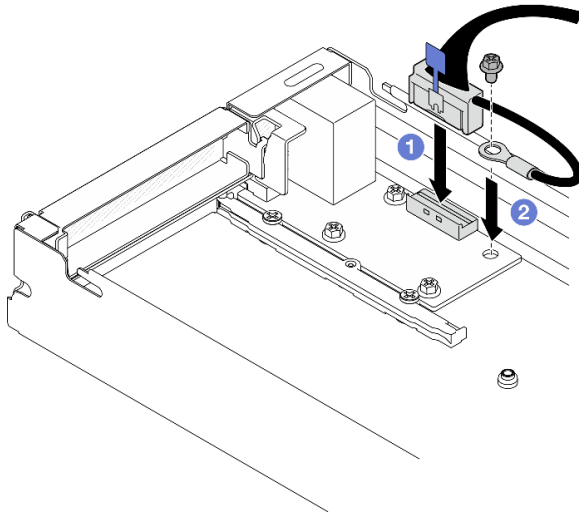
Figure 101. Installation du câble d'E-S arrière et du câble de mise à la terre
