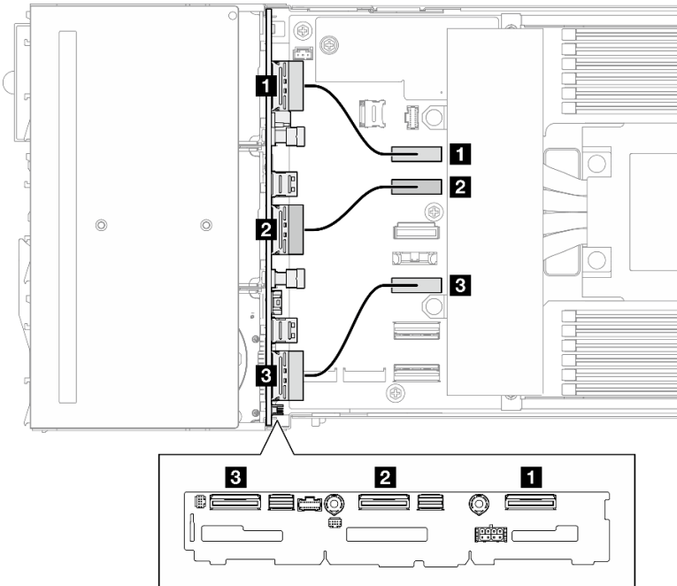
Figure 121. Cheminement des câbles NVMe
