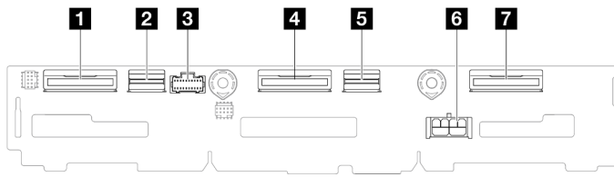
Figure 115. Fond de panier d'unité 2,5 pouces
