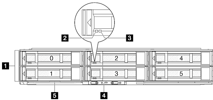
Figura 2. Configurazione con 6 unità SSD SAS/SATA/NVMe da 2,5"
