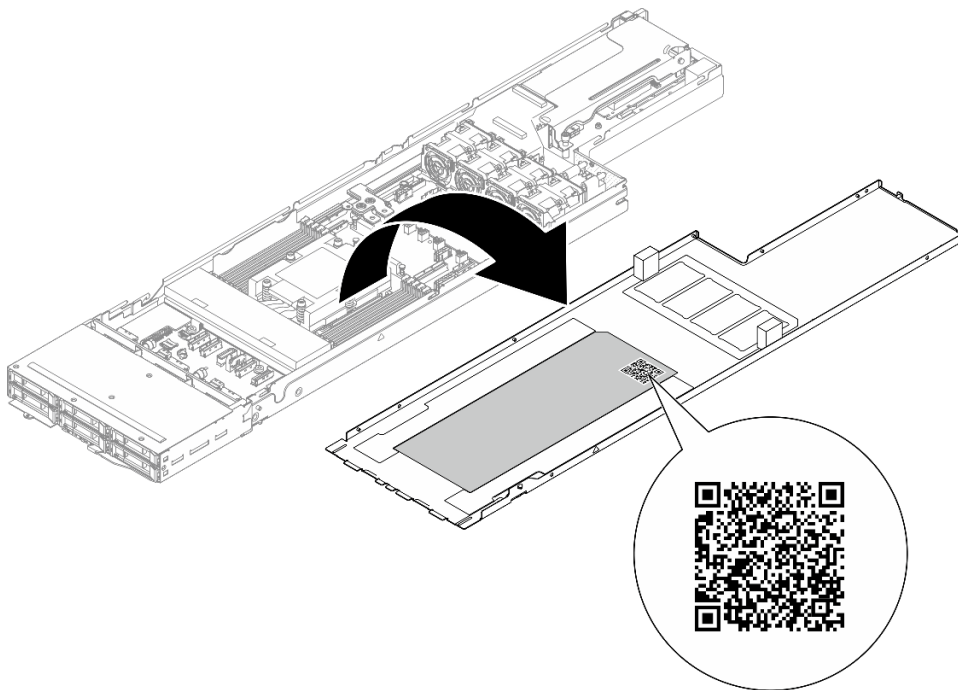
Figura 20. Etichetta di servizio e codice QR
