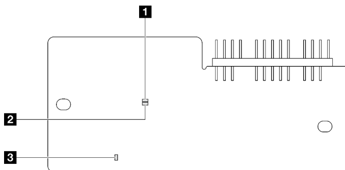
Figura 13. LED sul modulo firmware e sicurezza RoT
