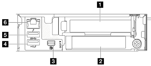
Figura 4. Vista posteriore
