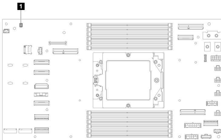
Figura 14. LED della scheda di sistema
