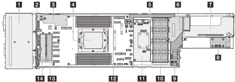
Figura 7. Vista superiore di SD535 V3
