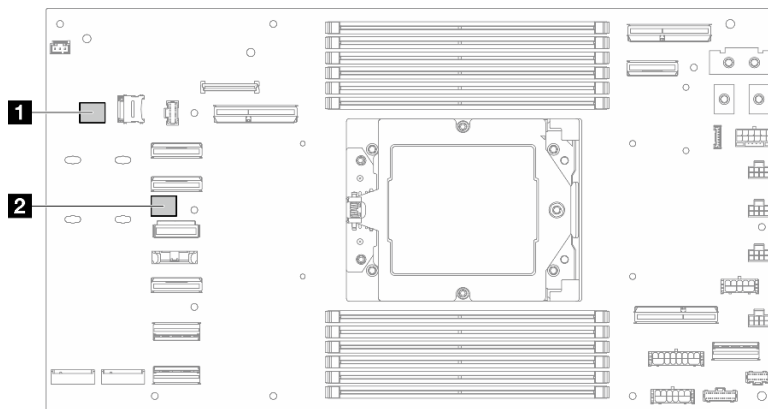
Figura 9. Switch della scheda di sistema
