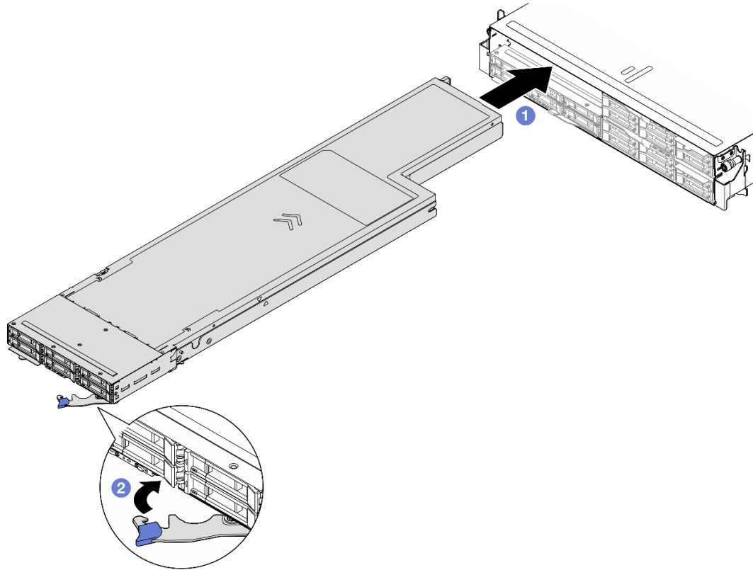
図22. 左トレイへのノードの取り付け
