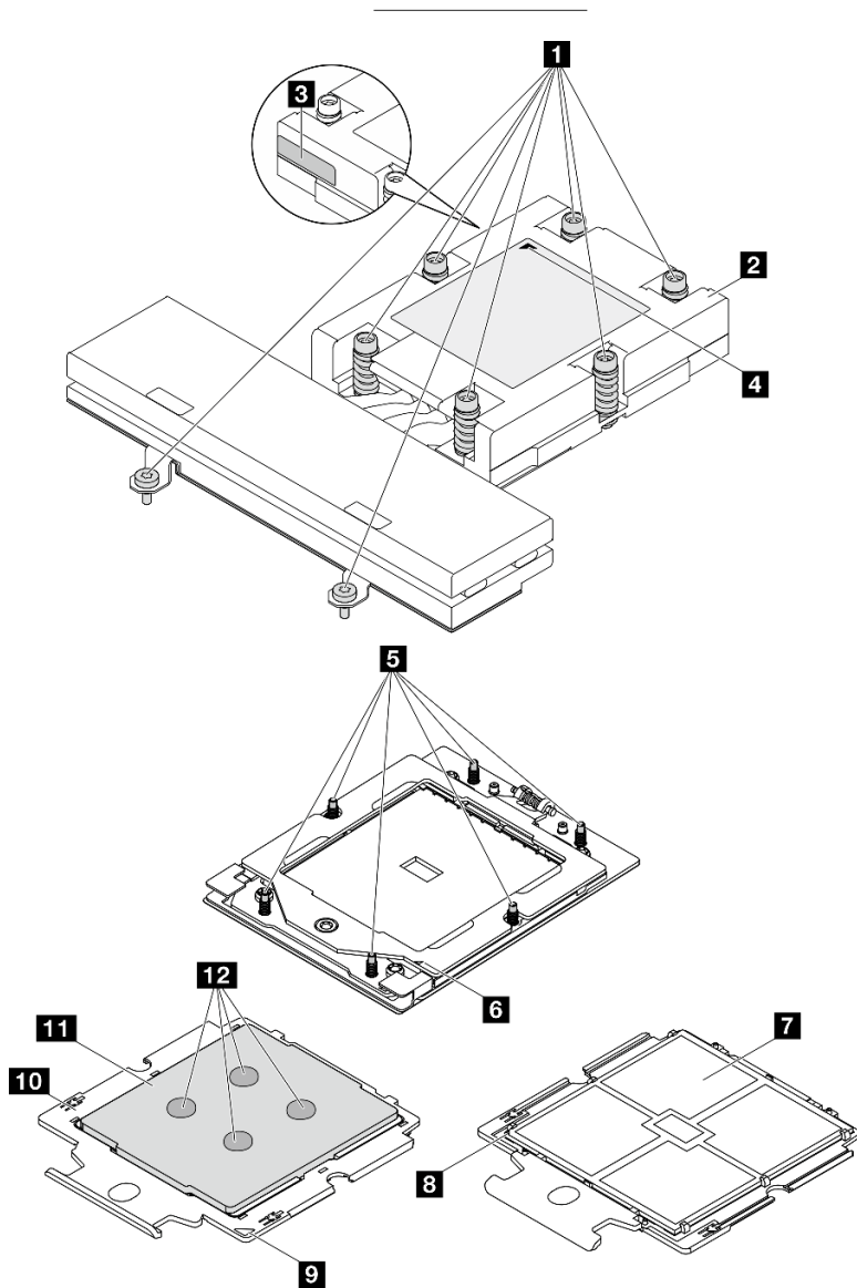
図94. プロセッサおよびヒートシンク・コンポーネント
