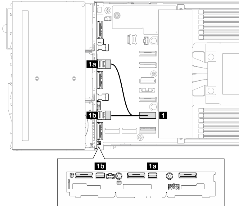
図 122. オンボード SATA ケーブル配線
