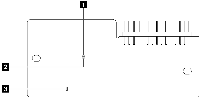
図 140. ファームウェアおよび RoT セキュリティー・モジュール上の LED
