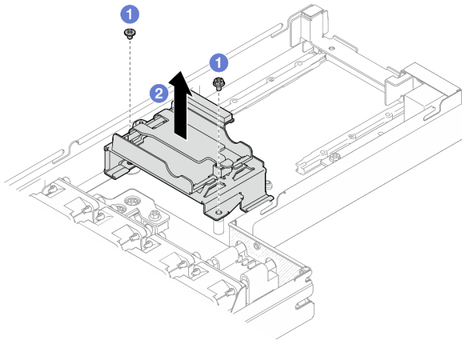
図35. フラッシュ電源モジュール・ホルダーの取り外し
