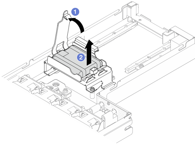
図34. フラッシュ電源モジュールの取り外し
