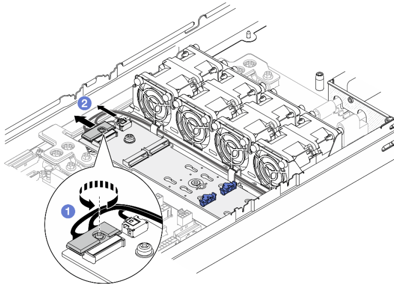
図 52. NVMe M.2 ブート・アダプターからケーブルを取り外す
