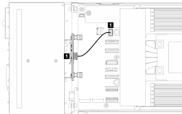
図 128. 前面 I/O ボード・ケーブル配線
