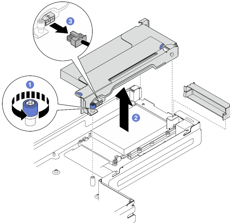
図 78. PCIe ライザー・アセンブリの取り外し
