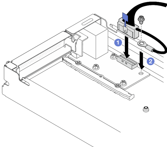
図 101. 背面 I/O ケーブルと接地用ケーブルの取り付け
