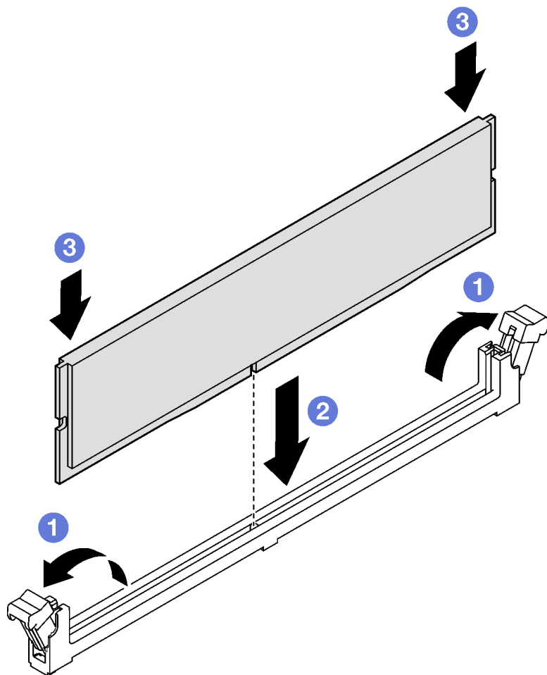
図71. メモリー・モジュールの取り付け
