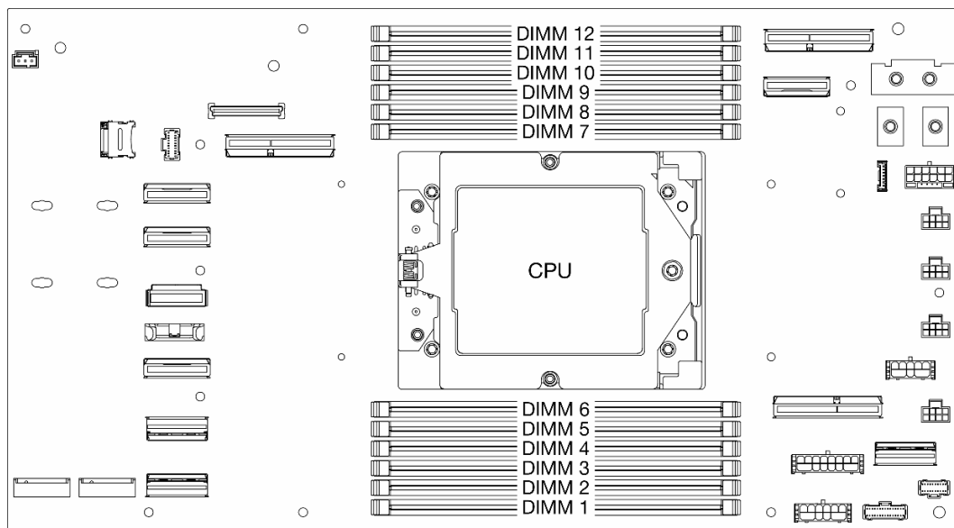
図 68. メモリー・モジュールおよびプロセッサのレイアウト
