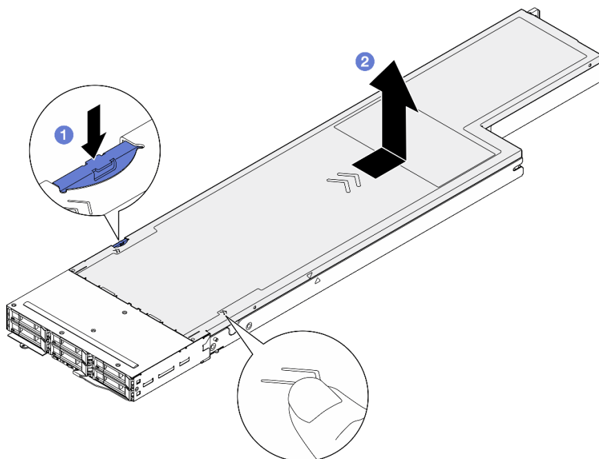
図 112. トップ・カバーの取り外し
