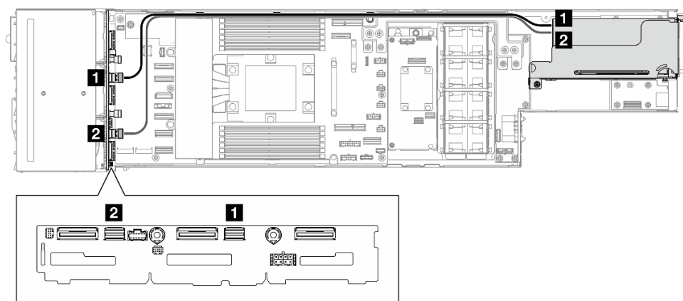
図 126. 8i RAID PCIe アダプター SATA/SAS ケーブル配線
