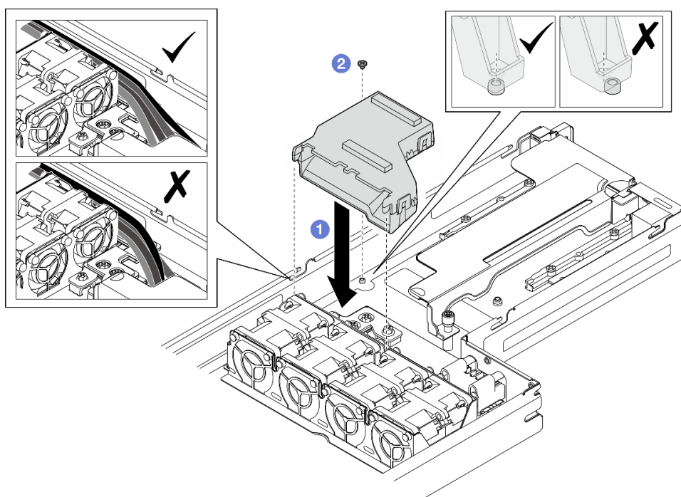
図 43. GPU エア・ダクトの取り付け
