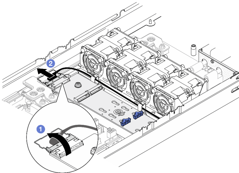
図 53. SATA/NVMe M.2 ブート・アダプターからケーブルを取り外す
