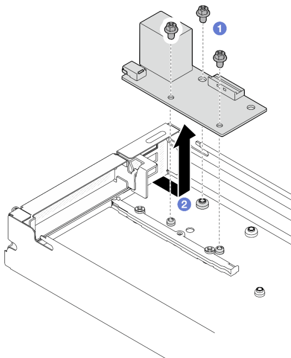
図99. 背面 I/O モジュールの取り外し
