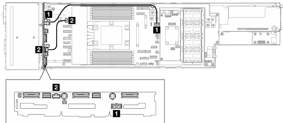
図 120. ドライブ・バックプレーンの側波帯と電源ケーブル配線
