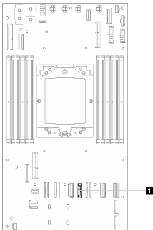
図 26. CMOS バッテリー・ソケットの位置
