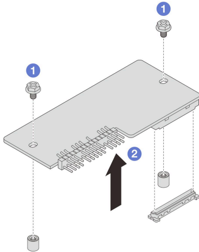
図 103. ファームウェアおよび RoT セキュリティー・モジュール の取り外し
