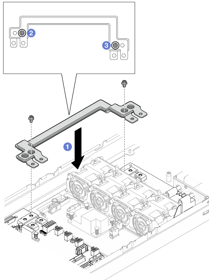
図 87. 電源バス・バーの取り付け
