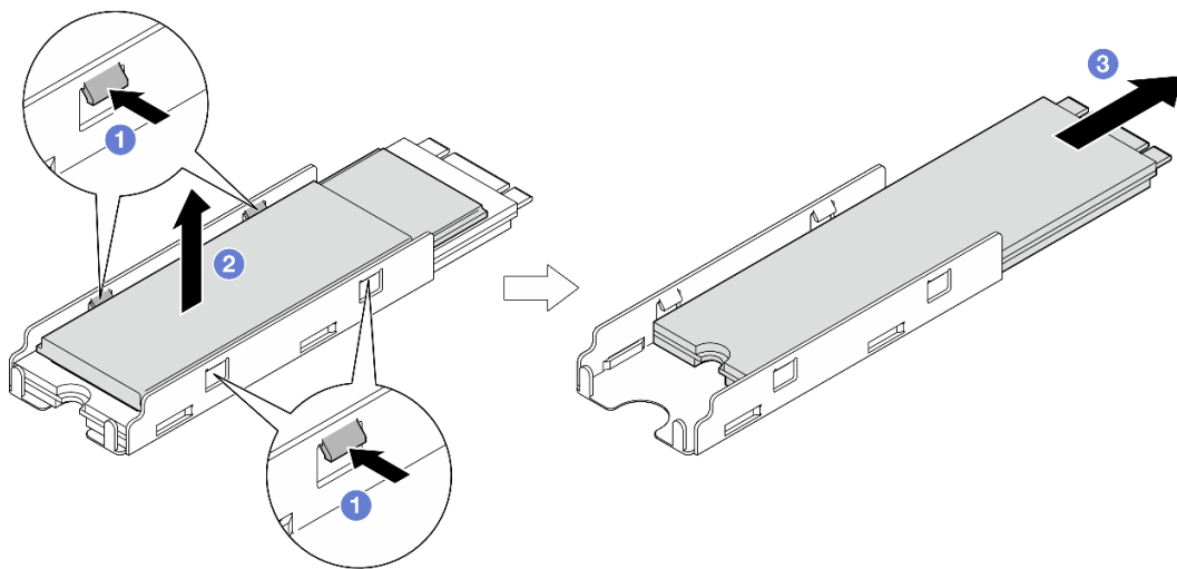
図50. M.2 ヒートシンクの取り外し
