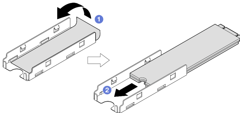
図 63. トレイへのサーマル・パッドおよび M.2 ドライブの取り付け
