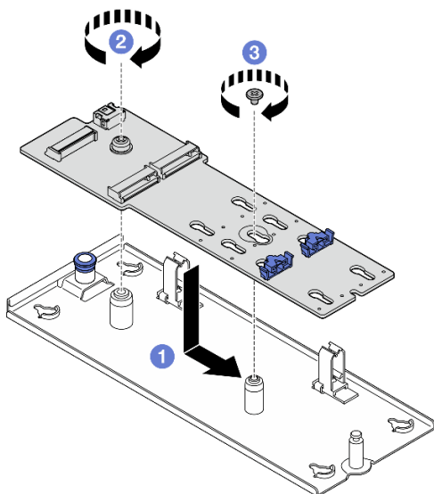
図 56. M.2 ブート・アダプターの取り付け
