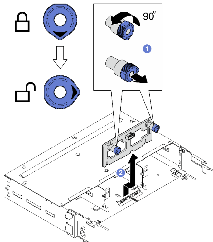
図40. 前面 I/O バックプレートの取り外し
