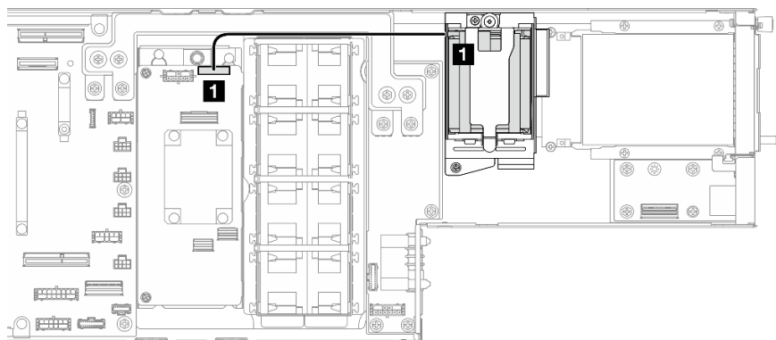
図 125. フラッシュ電源モジュールのケーブル配線
