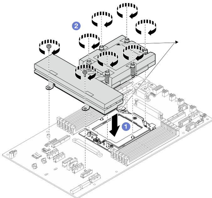
図97. ヒートシンクの取り付け
