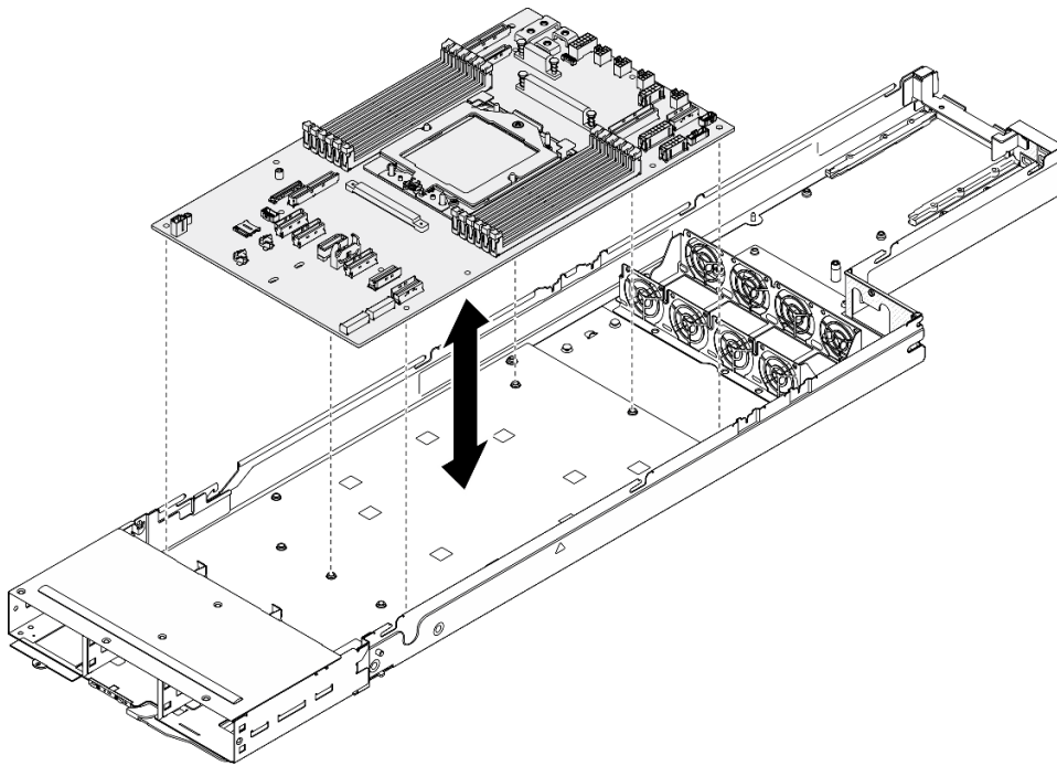
図108. システム・ボードの取り外し
