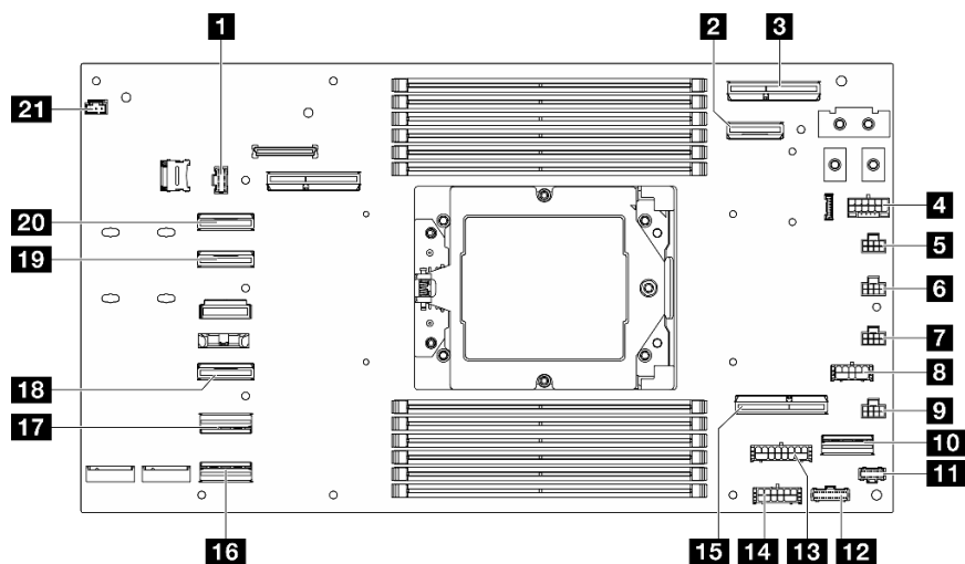
図 114. ケーブル配線用のシステム・ボード・コネクタ
