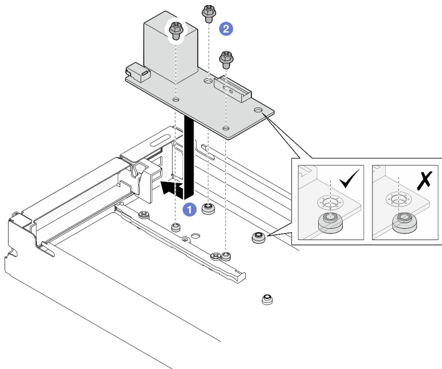
図 100. 背面 I/O モジュールの取り付け
