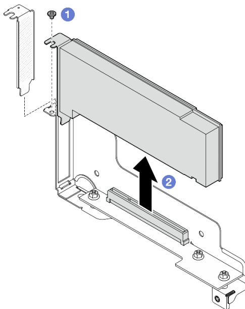
図 80. PCIe アダプターの取り外し
