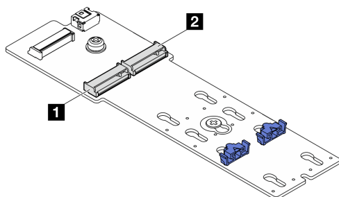
図 66. M.2 ドライブ・スロット
