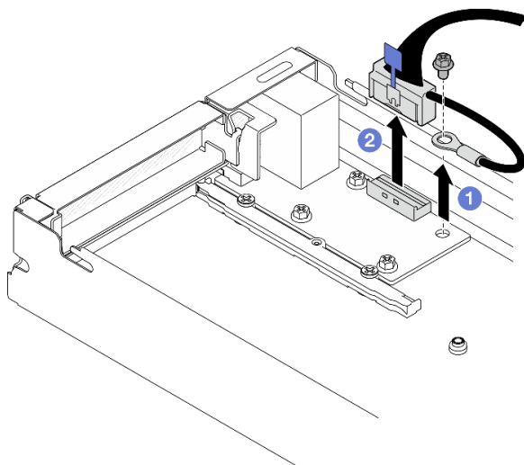
図98. 背面 I/O ケーブルと接地用ケーブルの取り外し
