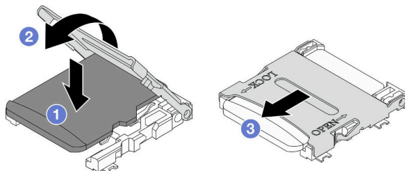
図 75. MicroSD カードの取り付け
