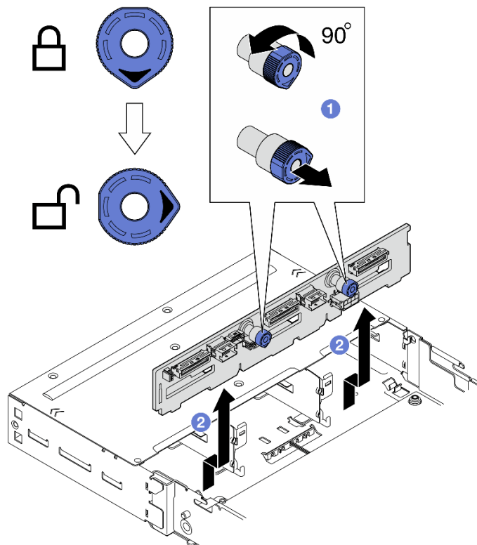
図30. ドライブ・バックプレーンの取り外し
