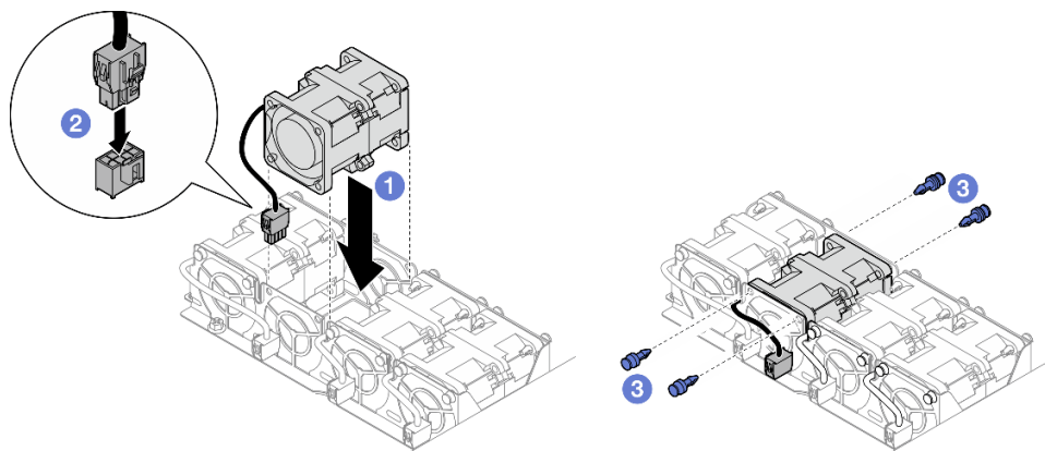
図 33. ファンの取り付け
