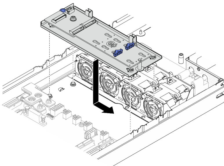
図 57. M.2 ブート・アダプター・トレイの取り付け
