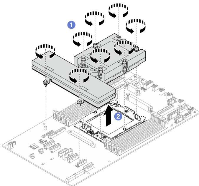
図92. ヒートシンクの取り外し
