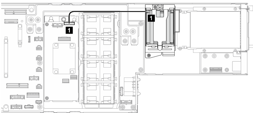
図 39. CFF RAID およびフラッシュ電源モジュール・ケーブル
