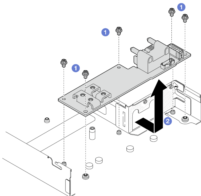
図 89. 分電盤の取り外し
