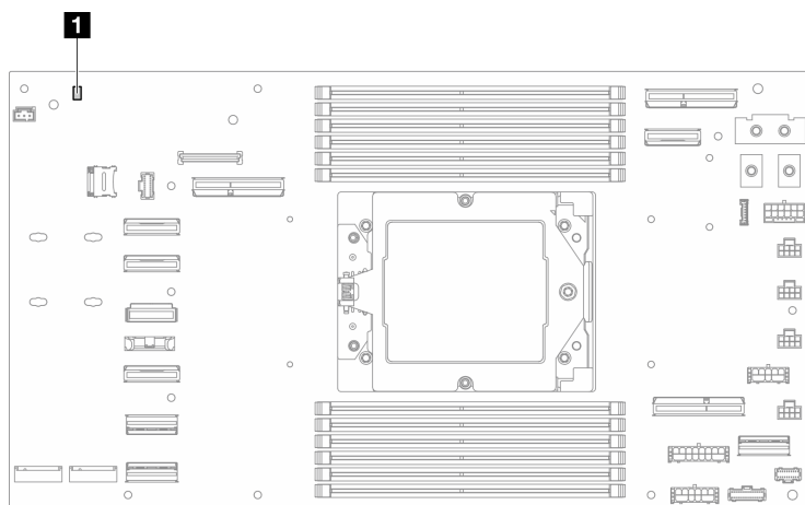
図 141. システム・ボード LED
