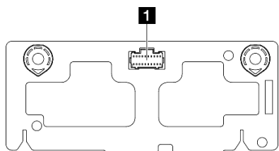
図 116. 前面 I/O ボード・コネクタ
