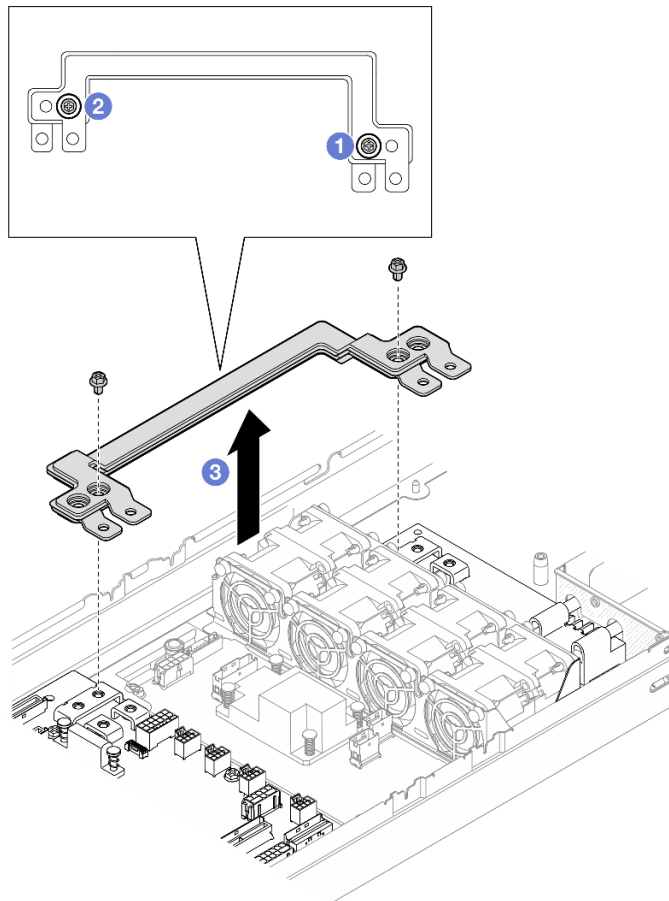
図86. 電源バス・バーの取り外し
