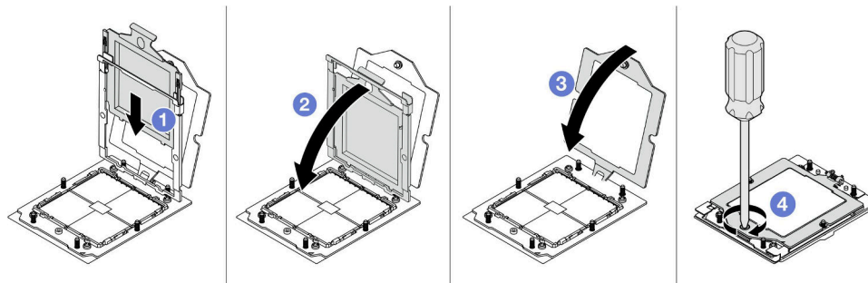
図95. プロセッサの取り付け
