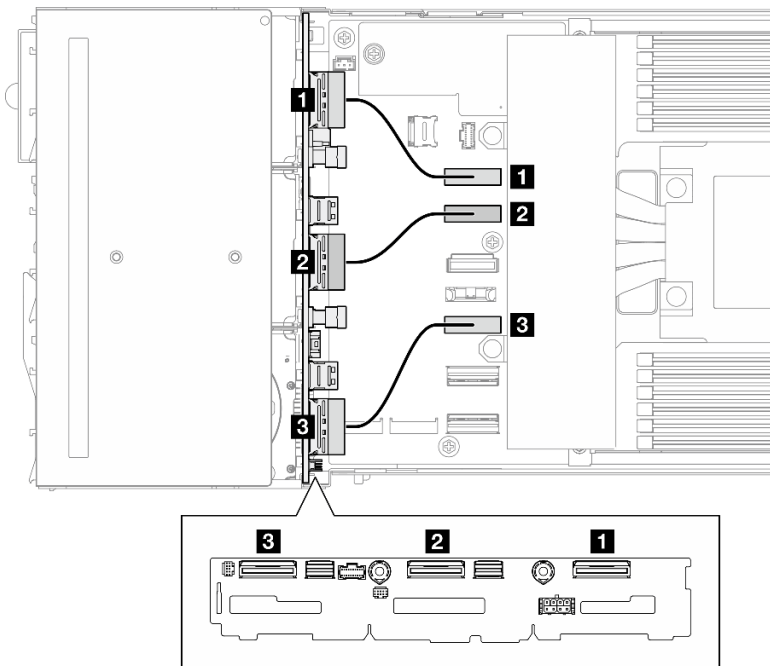
図 121. NVMe ケーブル配線
