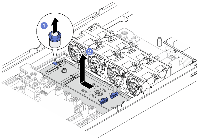
図 54. M.2 ブート・アダプター・トレイの取り外し
