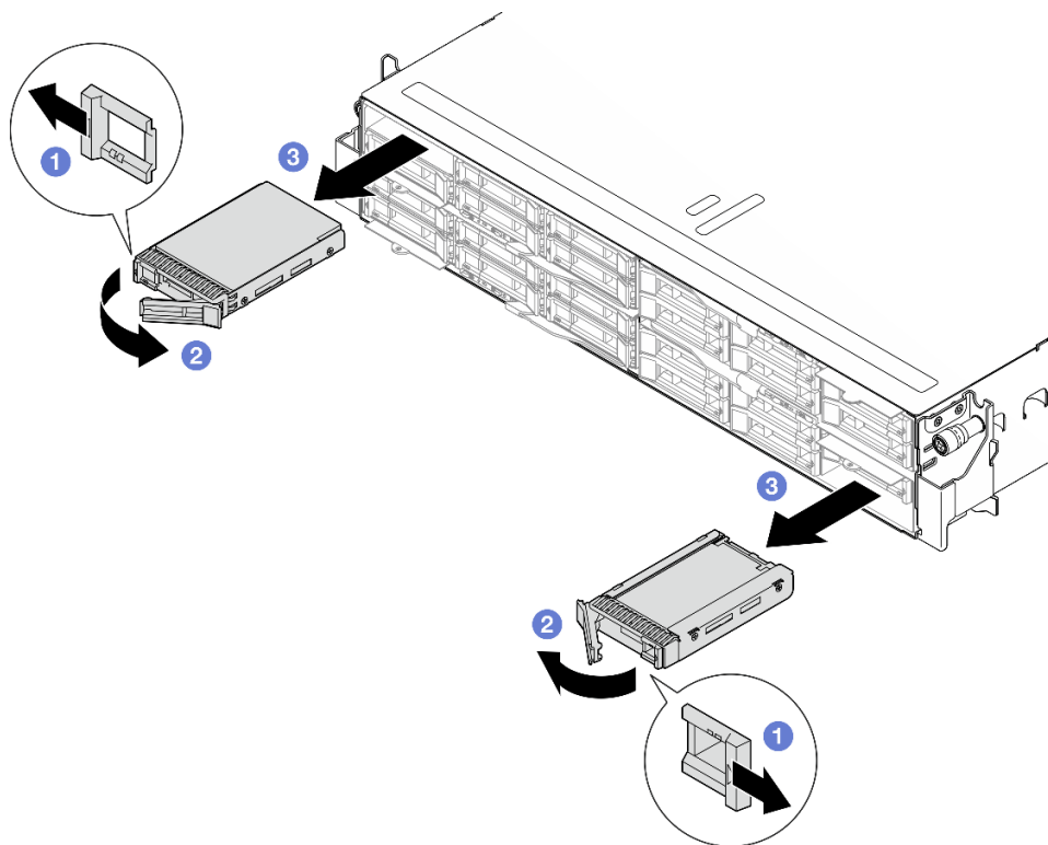
図44. ソリッド・ステート・ドライブの取り外し
