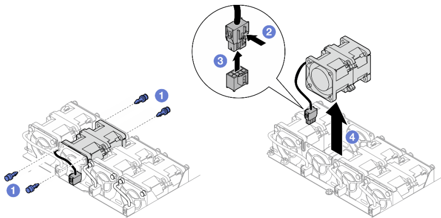
図32. ファンの取り外し
