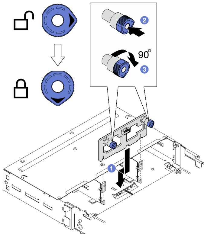
図 41. 前面 I/O バックプレーンの取り付け
