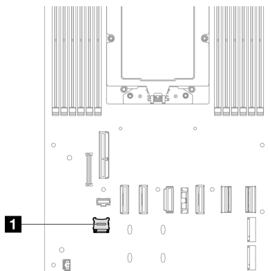
図 72. MicroSD ソケットの位置
