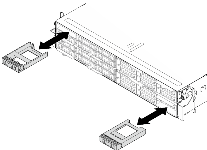
図 46. ドライブ・フィラーの交換
