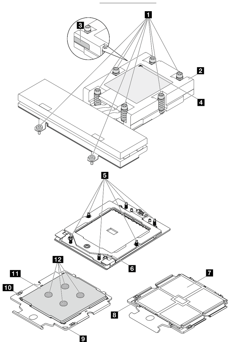
図91. プロセッサおよびヒートシンク・コンポーネント
