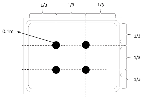
図96. 熱伝導グリースの塗布
