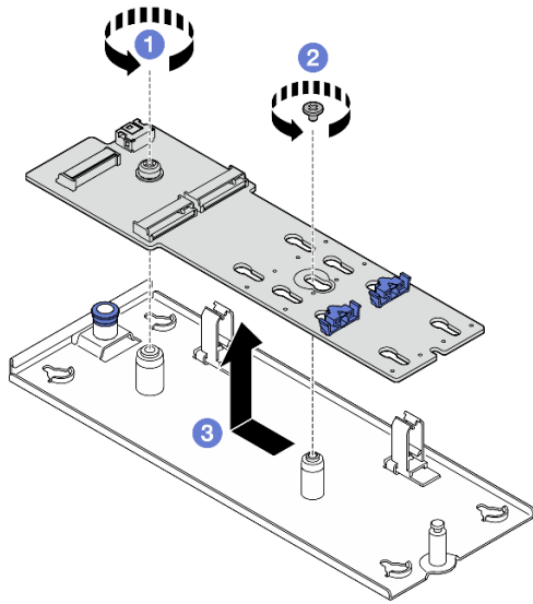
図 55. M.2 ブート・アダプターの取り外し
