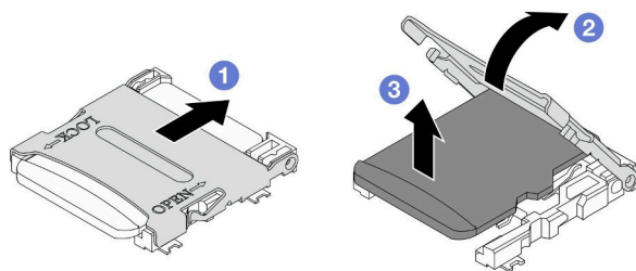
図 73. MicroSD カードの取り外し
