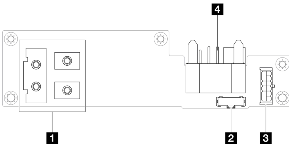
図 119. 分電盤コネクタ
