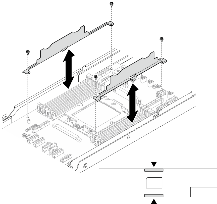
図111. ケーブル壁の交換
