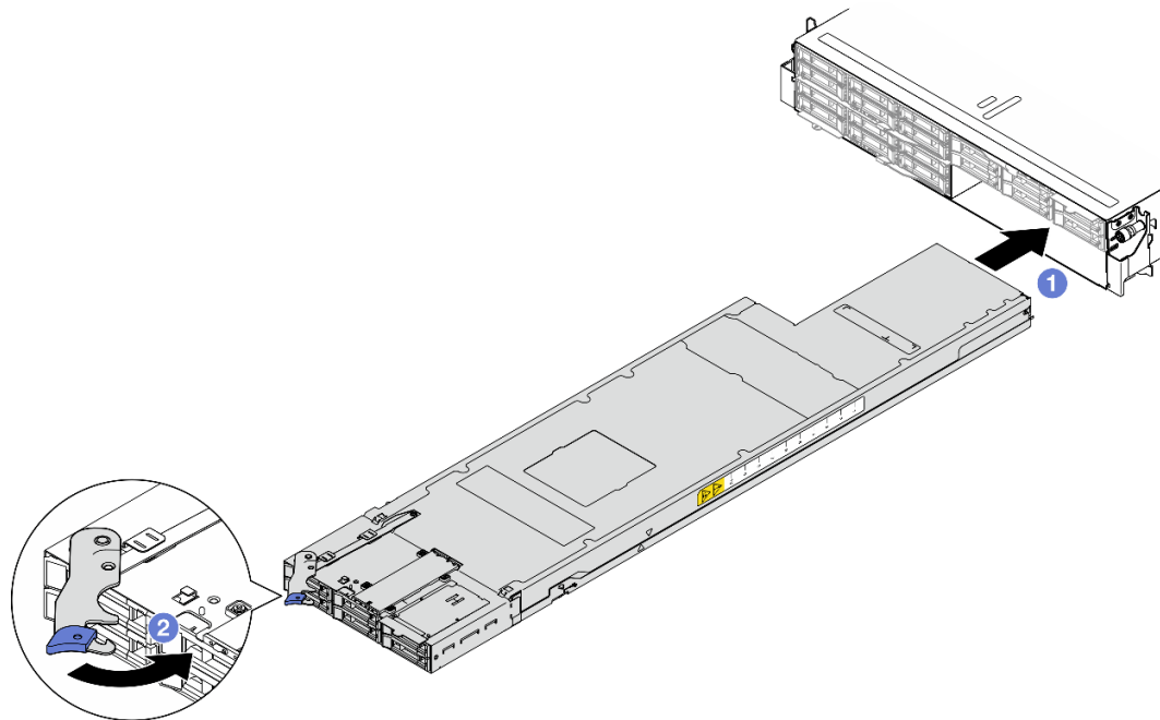
図23. 右トレイへのノードの取り付け
