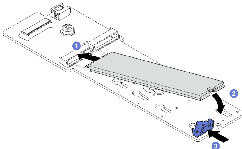
図 67. M.2 ドライブの取り付け
