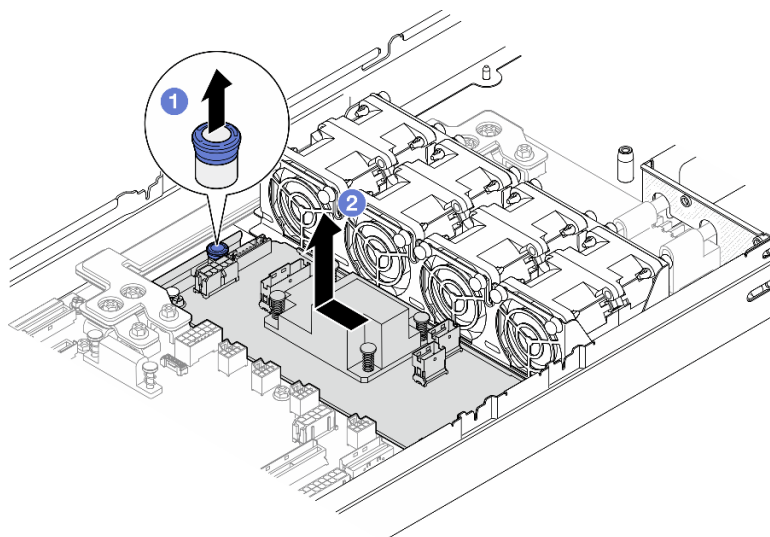
図 24. 内部 CFF RAID アダプターの取り外し
