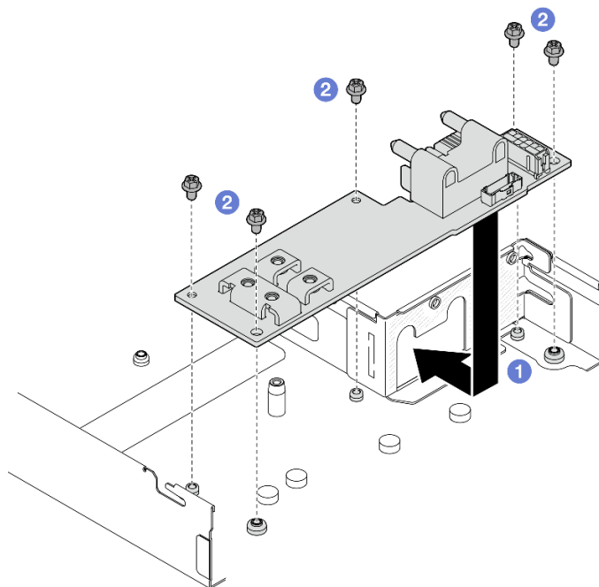
図 90. 分電盤の取り付け
