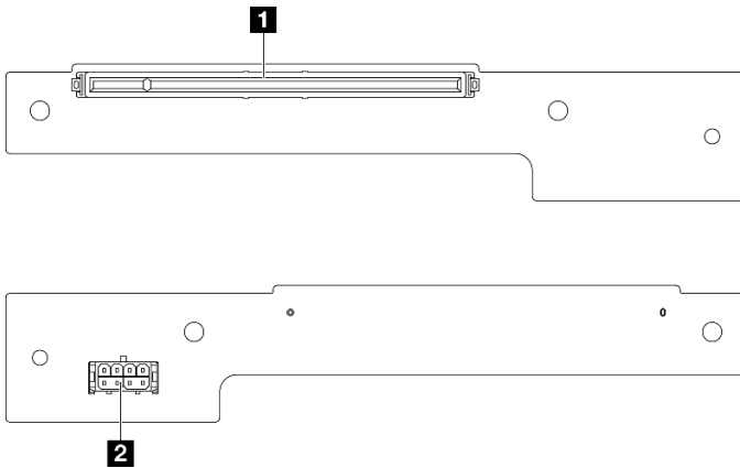
図 118. PCIe ライザー・カード・コネクタ
