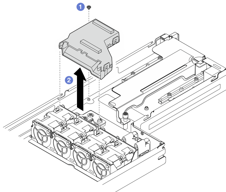
図 42. GPU エアークラウドの取り外し
