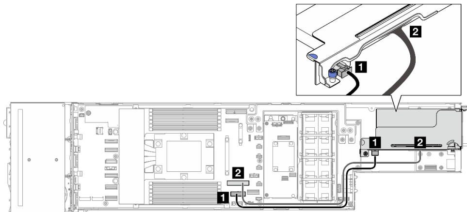
図 130. PCIe ライザーのケーブル配線
