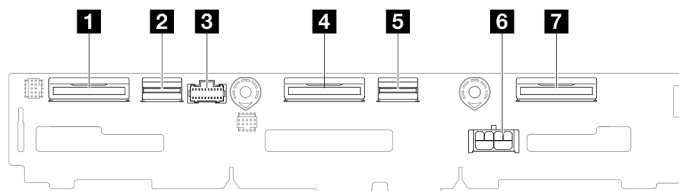
図 115. 2.5 型ドライブバック・プレーン
