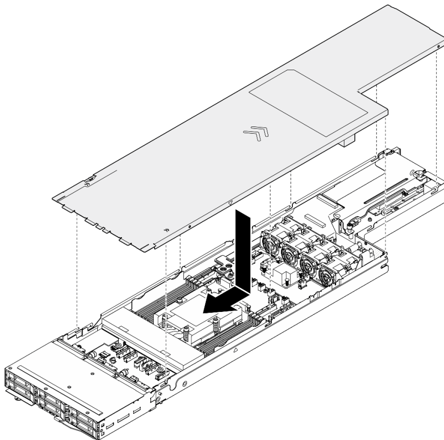
図113. トップ・カバーの取り付け
