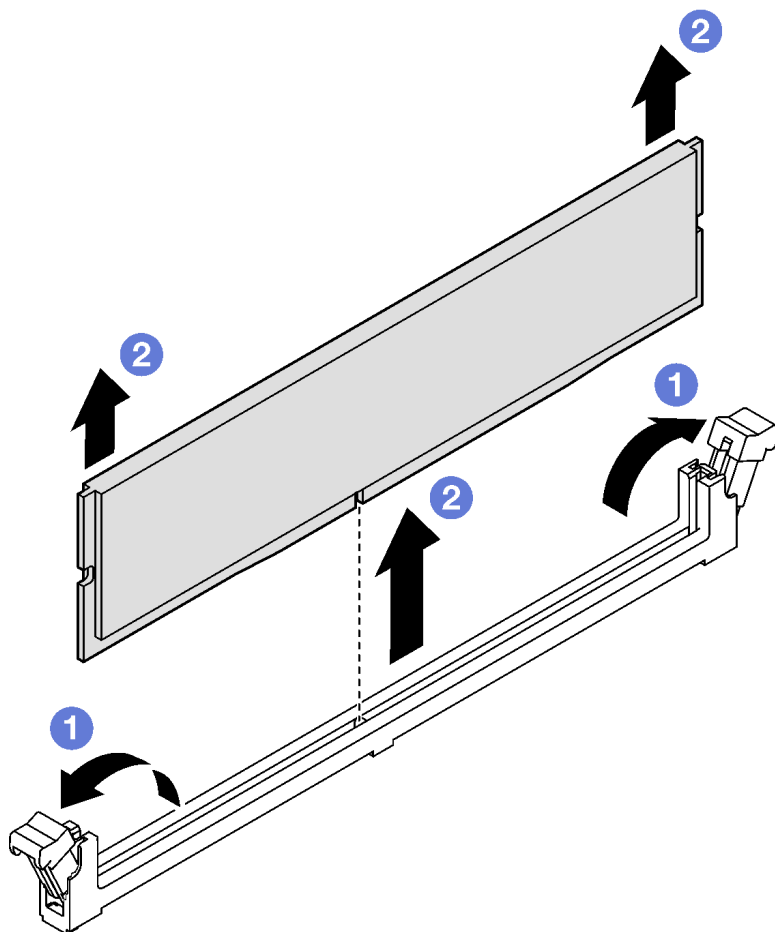
図 69. メモリー・モジュールの取り外し
