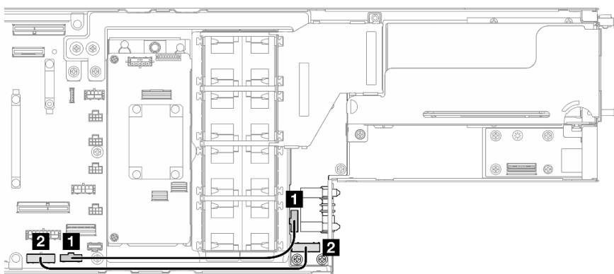
図 131. 分電盤のケーブル配線
