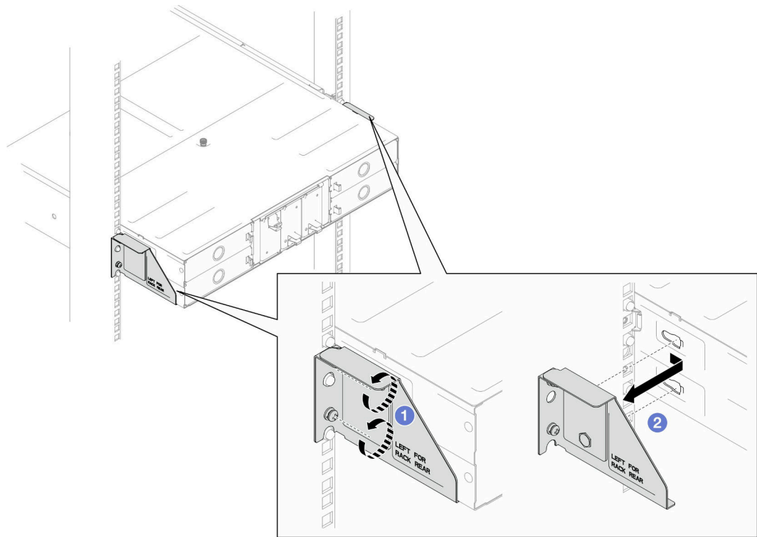
図2. 配送用ブラケットの取り外し
