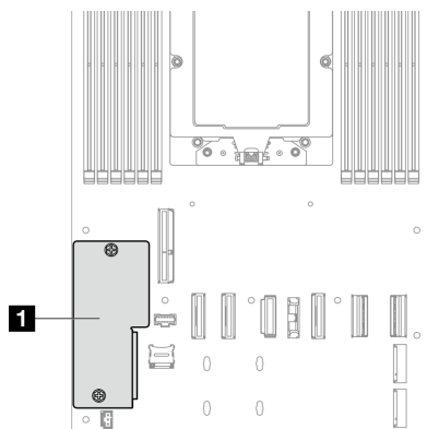
図 102. ファームウェアおよび RoT セキュリティー・モジュール の位置
