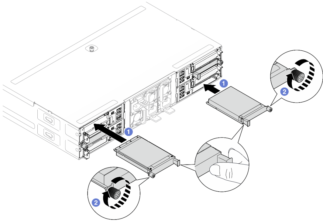
그림 77. 뒷면 OCP 모듈 설치
