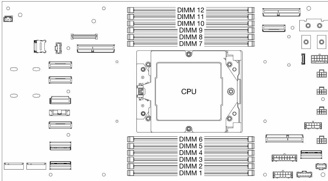
그림 68. 메모리 모듈 및 프로세서 레이아웃
