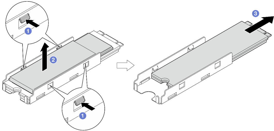
그림 50. M.2 방열판 제거
