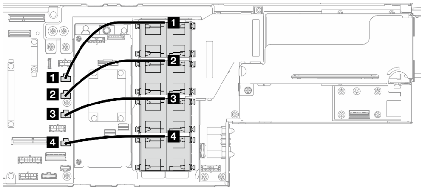
그림 127. 팬 케이블 배선
