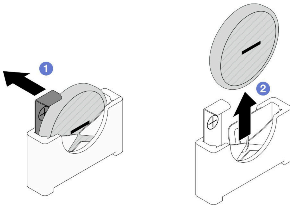
그림 27. CMOS 배터리 제거
