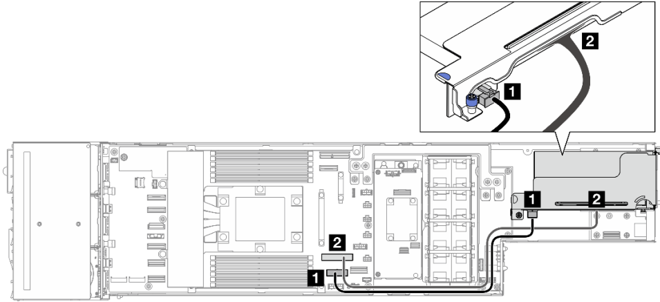
그림 130. PCIe 라이저 케이블 배선
