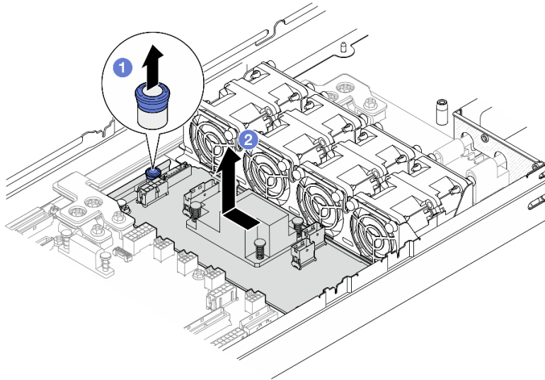
그림 24. 내부 CFF RAID 어댑터 제거
