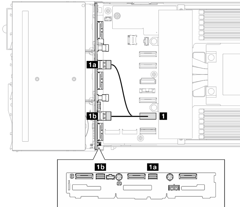
그림 122. 온보드 SATA 케이블 배선
