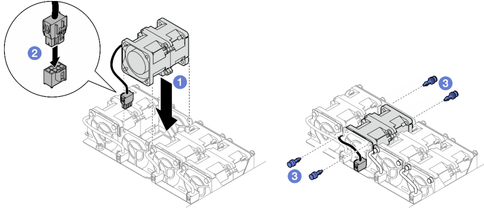
그림 33. 팬 설치
