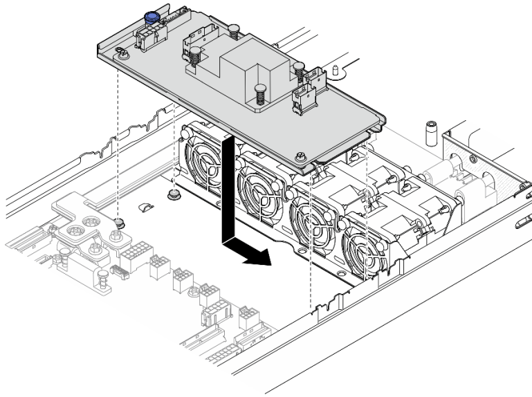
그림 25. 내부 CFF RAID 어댑터 설치
