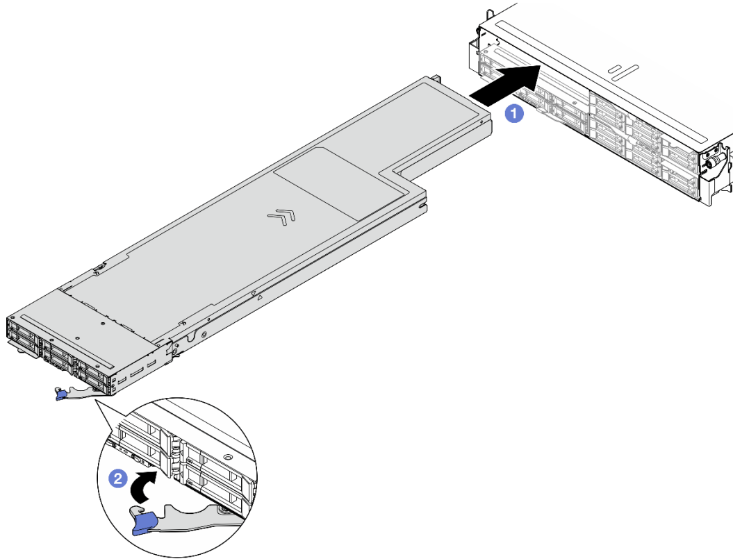
그림 22. 왼쪽 트레이에 노드 설치
