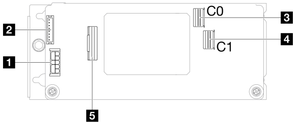
그림 117. 내부 CFF RAID 어댑터 커넥터
