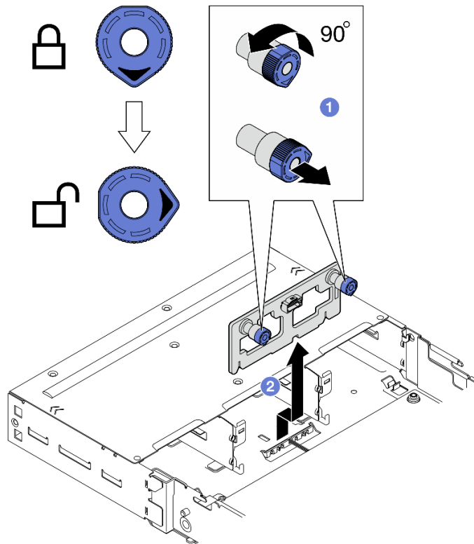
그림 40. 앞면 I/O 백플레인 제거
