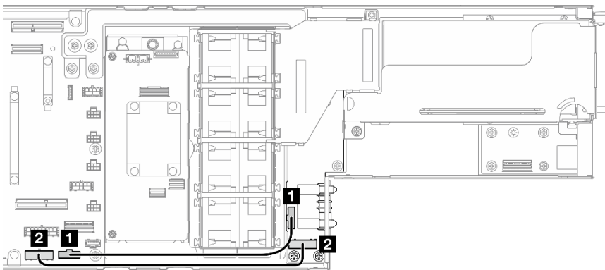
그림 131. 전원 분배 보드의 케이블 배선
