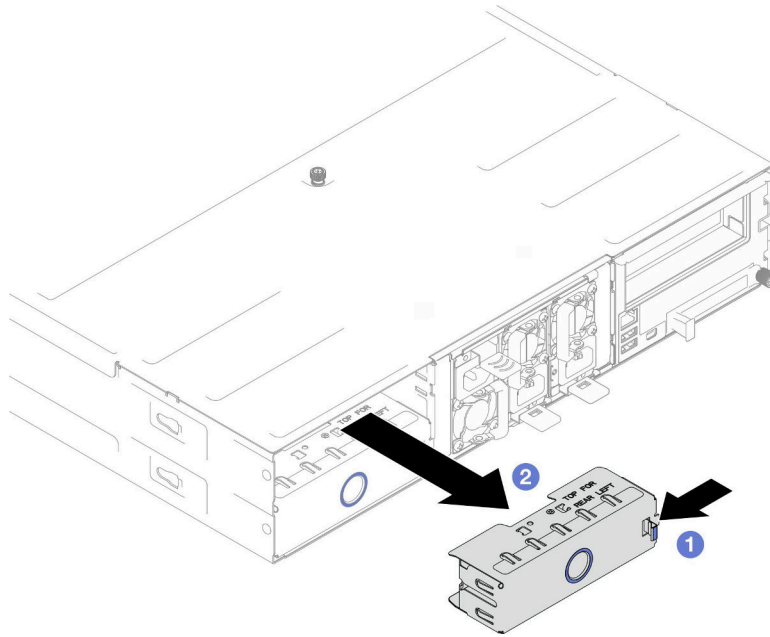
그림 21. 뒷면 노드 트레이 필러 제거
