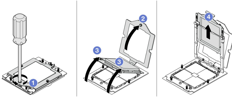
그림 93. 프로세서 제거
