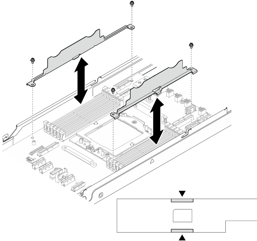
그림 106. 케이블 벽 교체
