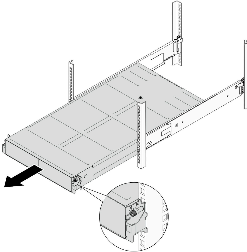
그림 3. 새시 제거
