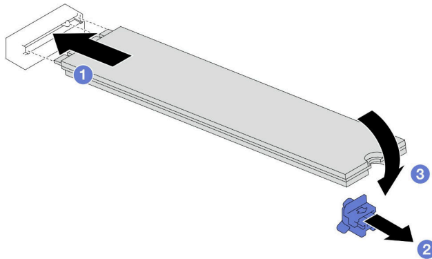
그림 65. M.2 드라이브 설치
