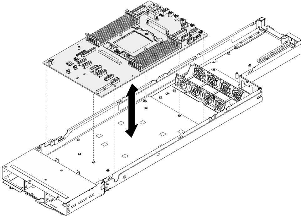
그림 109. 시스템 보드 설치
