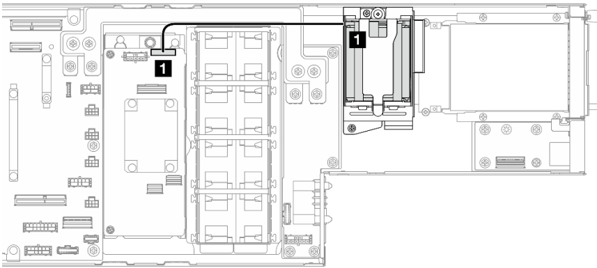
그림 39. CFF RAID 및 플래시 전원 모듈 케이블
