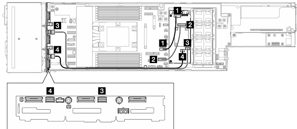
그림 123. CFF RAID 케이블 배선
