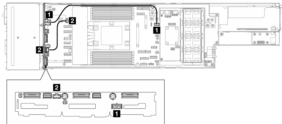
그림 120. 드라이브 백플레인 사이드밴드 및 전원 케이블 배선
