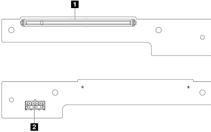
그림 118. PCIe 라이저 카드 커넥터
