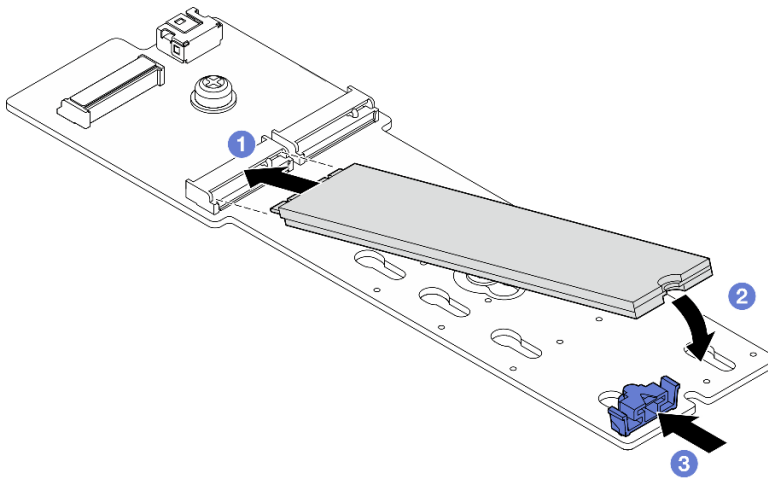
그림 67. M.2 드라이브 설치
