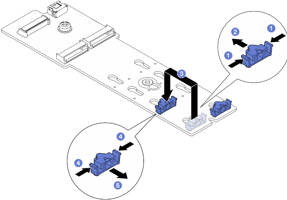
그림 61. M.2 고정장치 조정
