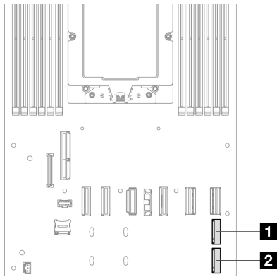
그림 48. 시스템 보드에서 M.2 베이의 위치
