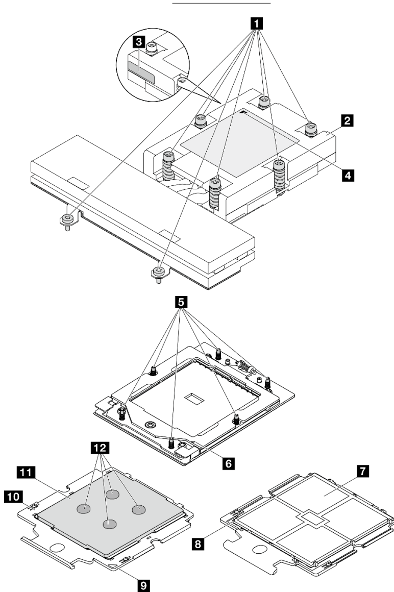
그림 91. 프로세서 및 방열판 구성 요소
