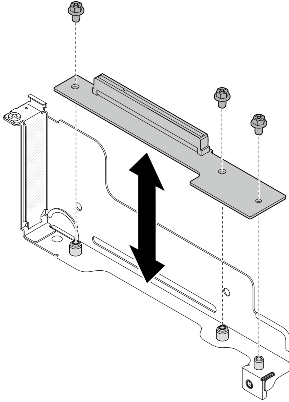
그림 83. PCIe 라이저 카드 교체
