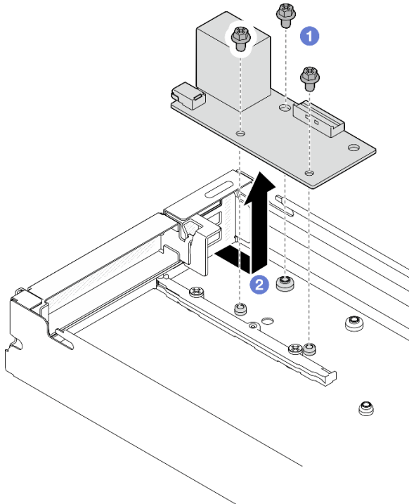
그림 99. 뒷면 I/O 모듈 제거
