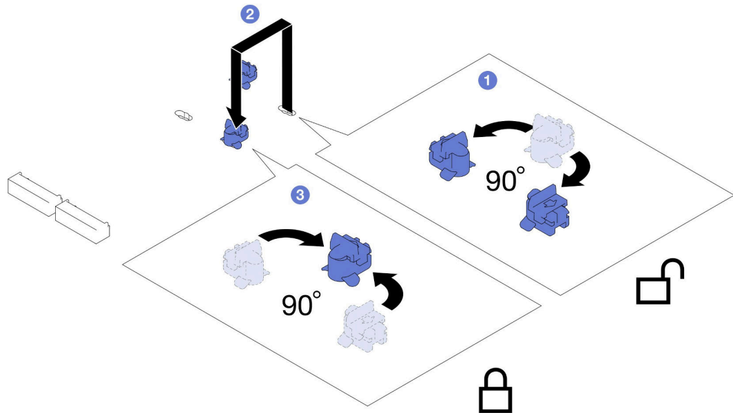
그림 60. M.2 드라이브 고정장치 조정
