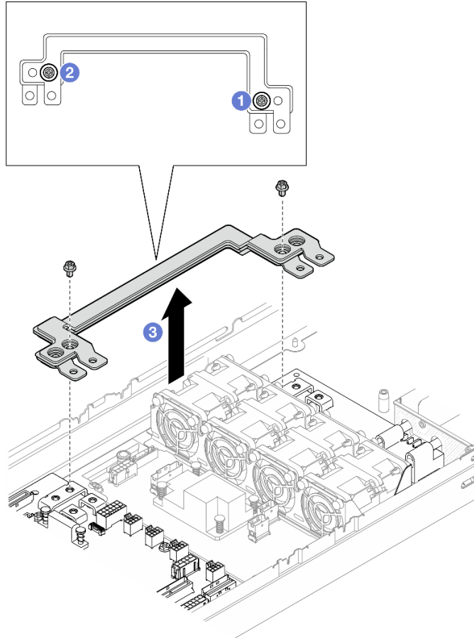
그림 86. 전원 버스 바 제거
