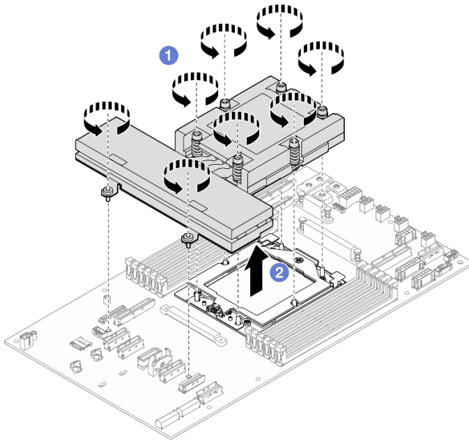
그림 92. 방열판 제거
