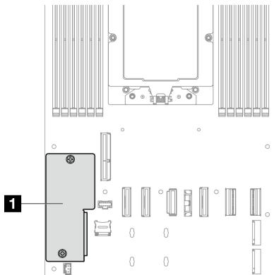
그림 104. 펌웨어 및 RoT 보안 모듈의 위치
