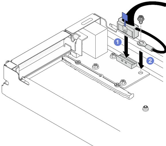
그림 101. 뒷면 I/O 케이블 및 접지 케이블 설치
