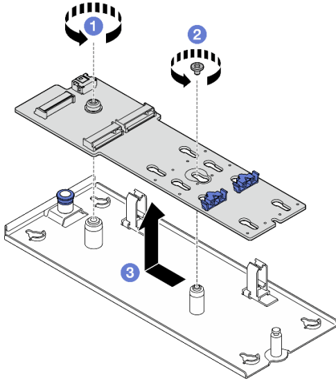
그림 55. M.2 부트 어댑터 제거
