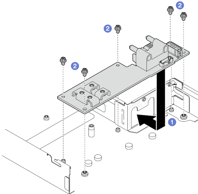
그림 90. 전원 분배 보드 설치
