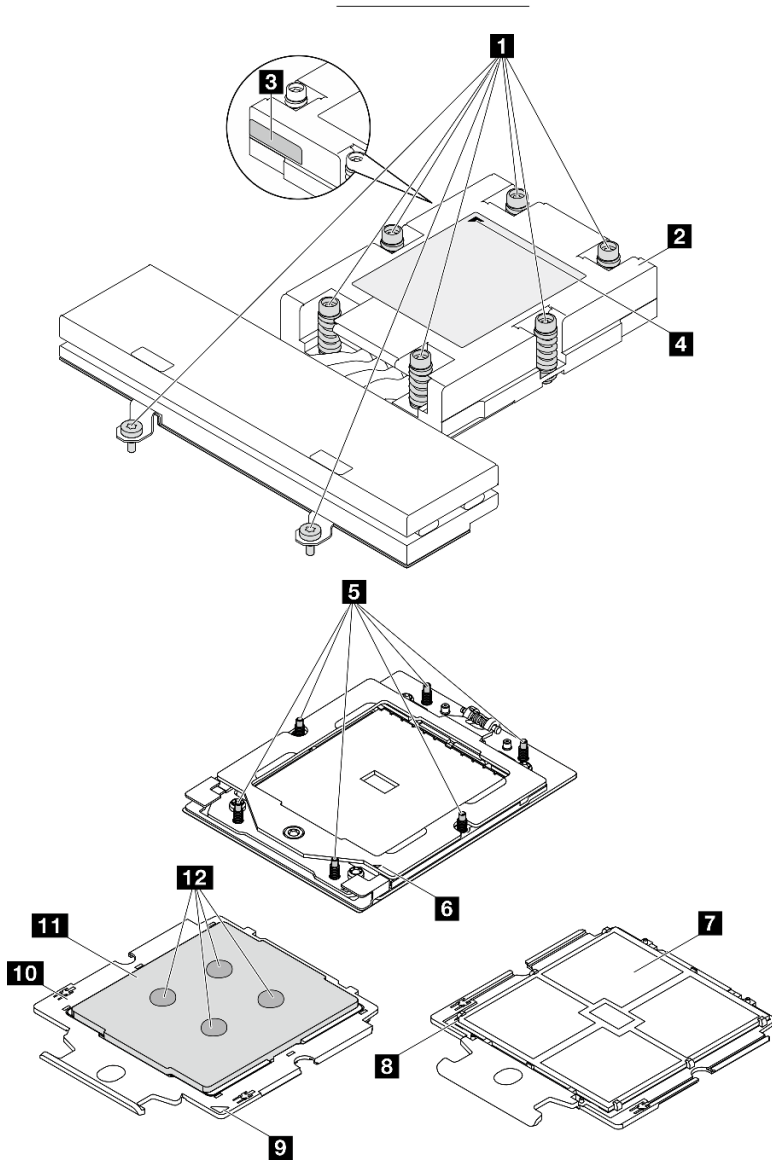
그림 94. 프로세서 및 방열판 구성 요소
