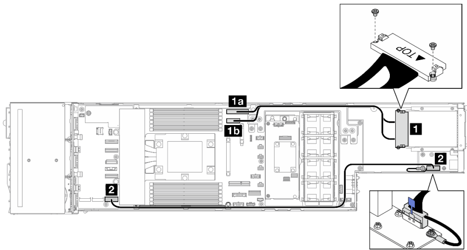
그림 132. 뒷면 I/O 모듈 및 OCP 모듈의 케이블
