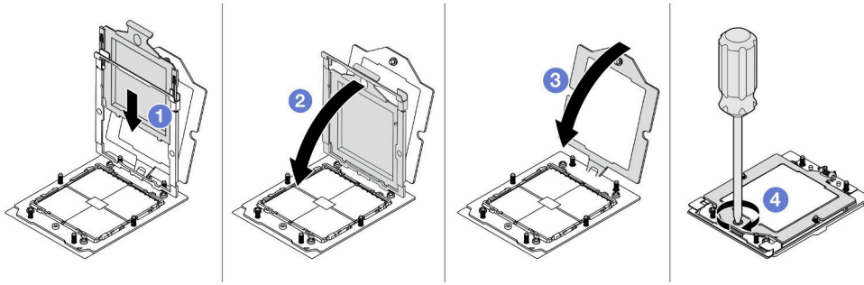
그림 95. 프로세서 설치
