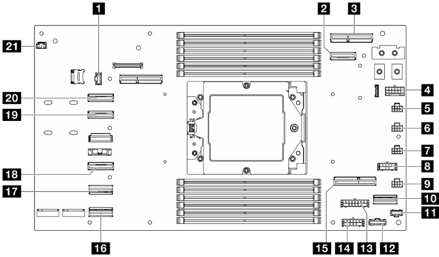
그림 114. 케이블 배선용 시스템 보드 커넥터
