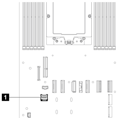
그림 72. MicroSD 소켓의 위치
