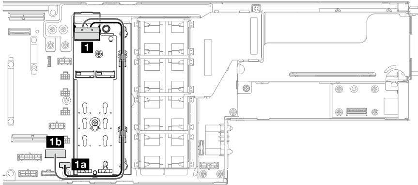
그림 129. SATA/NVMe M.2 부트 어댑터 케이블 배선
