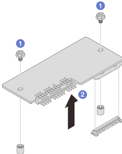
그림 103. 펌웨어 및 RoT 보안 모듈 제거
