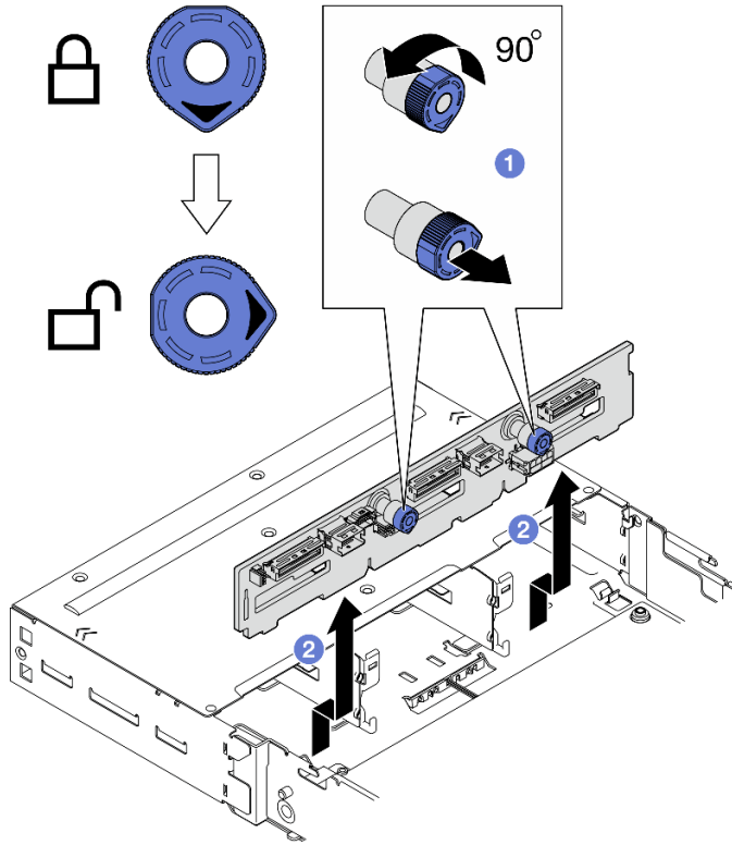
그림 30. 드라이브 백플레인 제거
