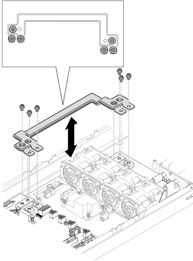
그림 88. 전원 버스 바 외부 나사 설치
