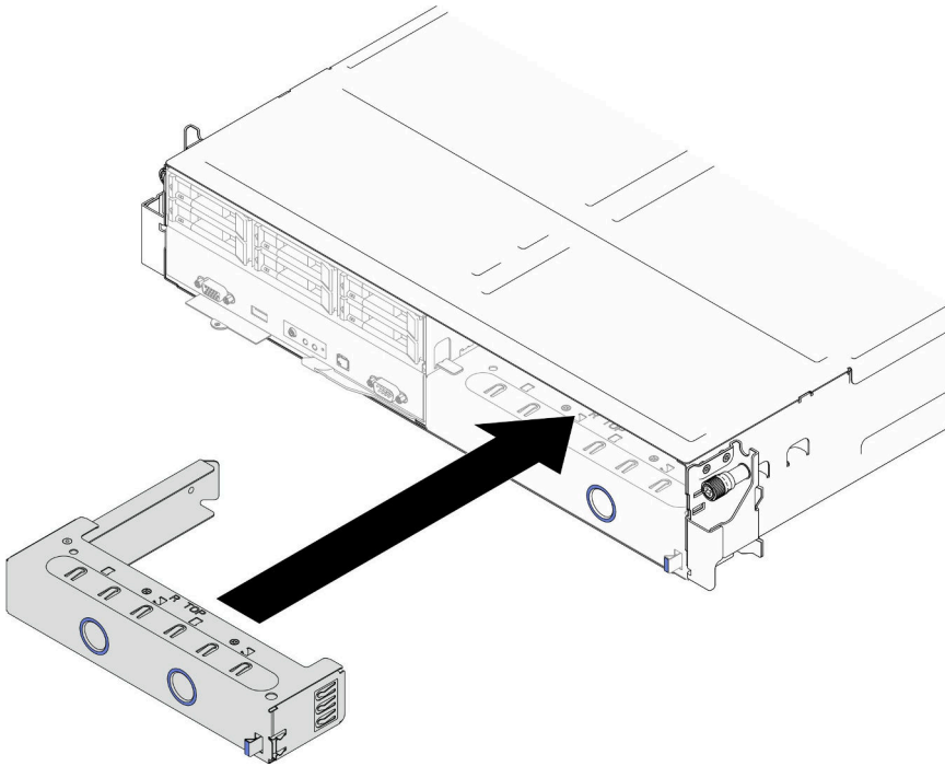
그림 18. 앞면 노드 트레이 필러 설치
