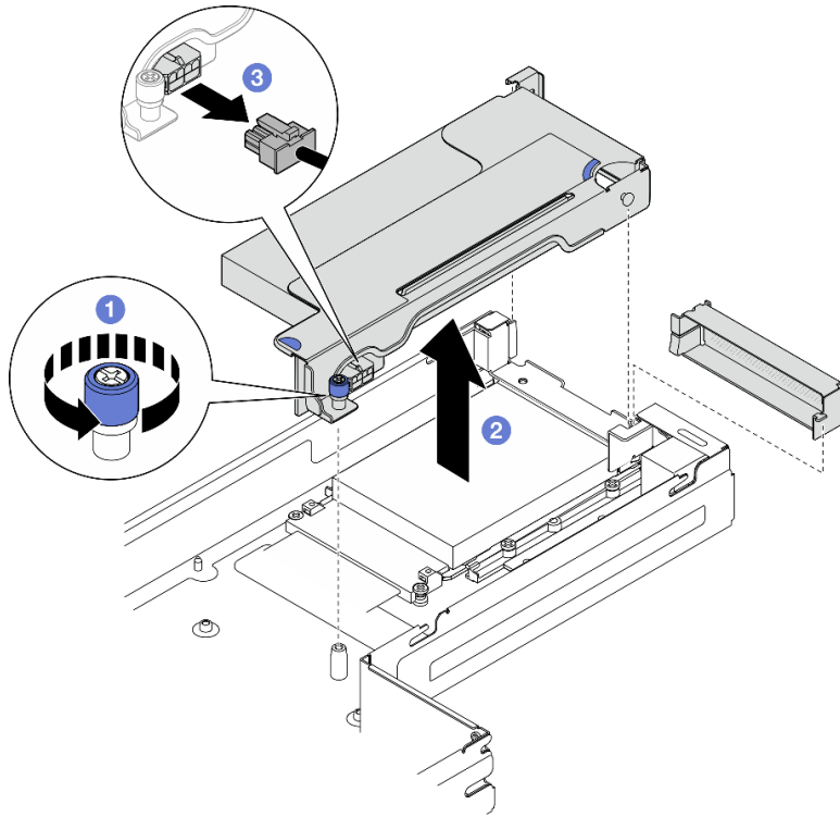
그림 78. PCIe 라이저 어셈블리 제거
