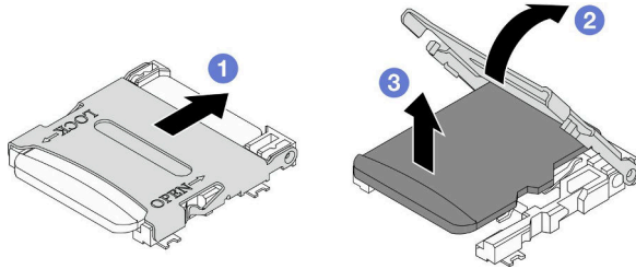
그림 73. MicroSD 카드 제거
