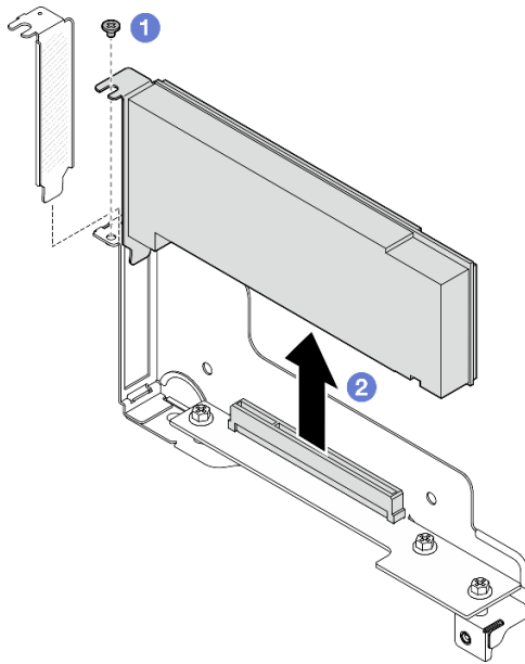
그림 80. PCIe 어댑터 제거
