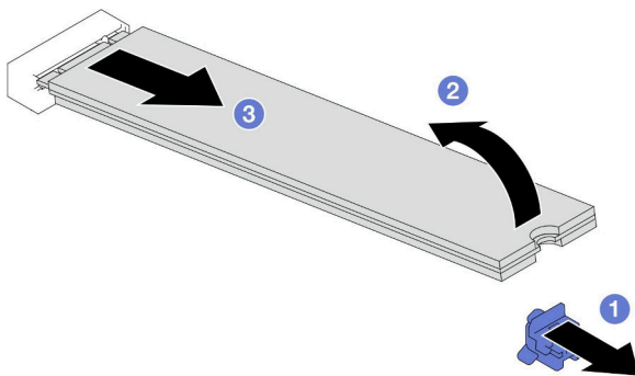
그림 49. M.2 드라이브 제거
