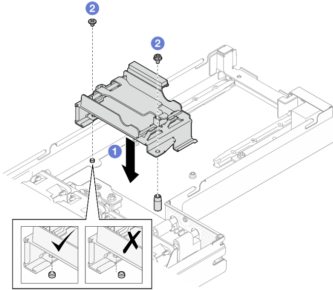
그림 36. 플래시 전원 모듈 홀더 설치
