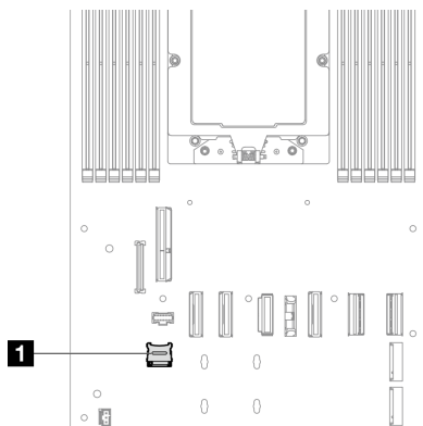
그림 74. MicroSD 소켓의 위치
