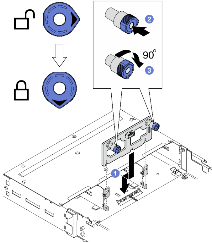
그림 41. 앞면 I/O 백플레인 설치
