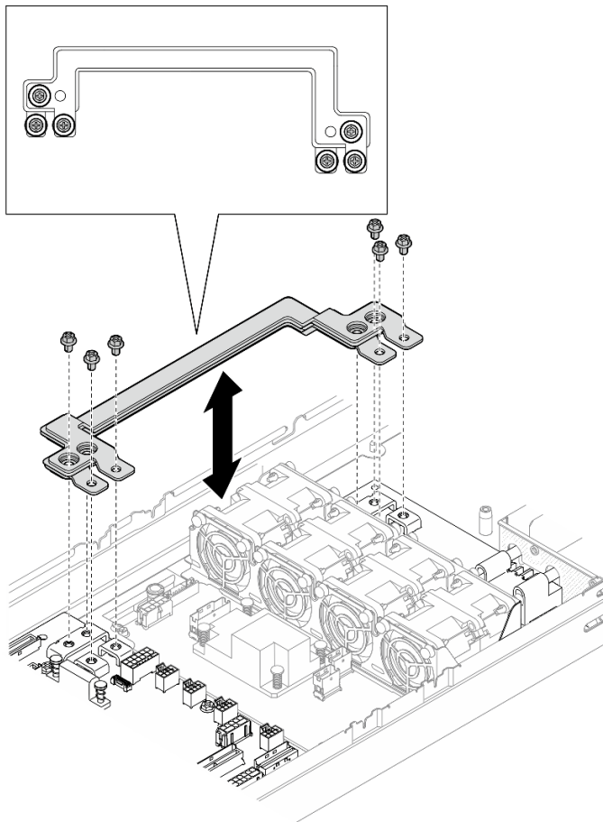
그림 85. 전원 버스 바의 외부 나사 제거
