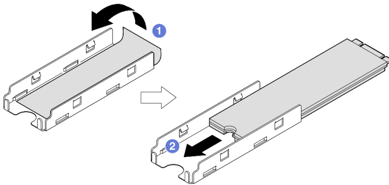
그림 63. 열 패드 및 M.2 드라이브를 트레이에 설치
