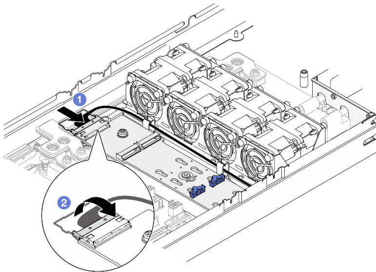
그림 59. SATA/NVMe M.2 부트 어댑터에 케이블 연결
