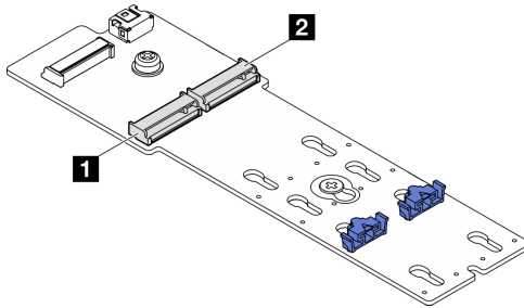
그림 66. M.2 드라이브 슬롯
