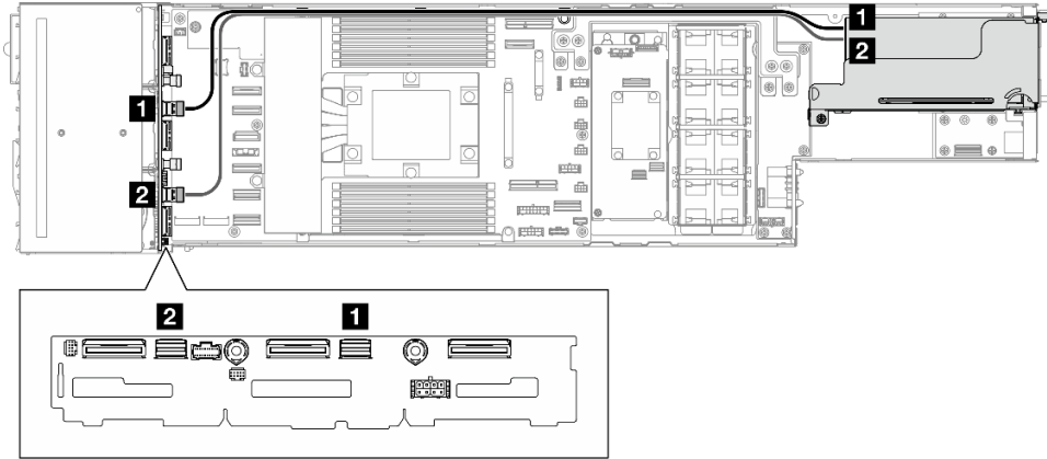
그림 126. 8i RAID PCIe 어댑터 SATA/SAS 케이블 배선
