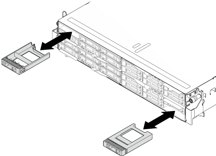
그림 46. 드라이브 필터 교체
