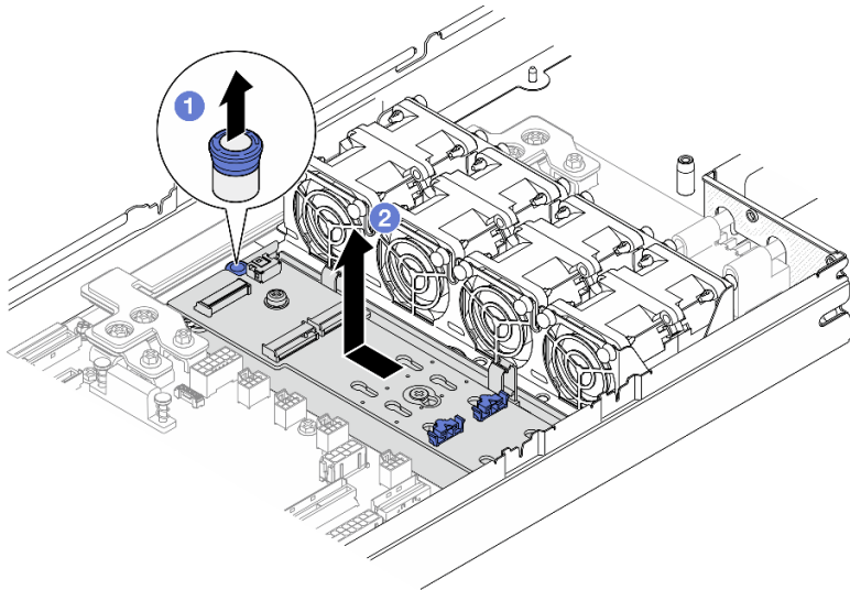
그림 54. M.2 부트 어댑터 트레이 제거
