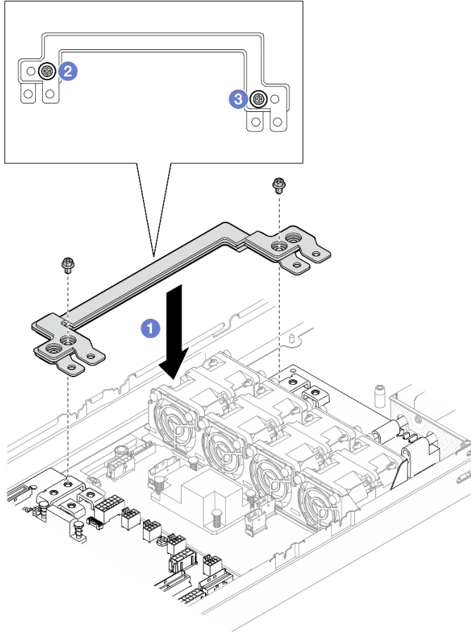
그림 87. 전원 버스 바 설치
