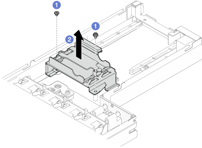
그림 35. 플래시 전원 모듈 홀더 제거
