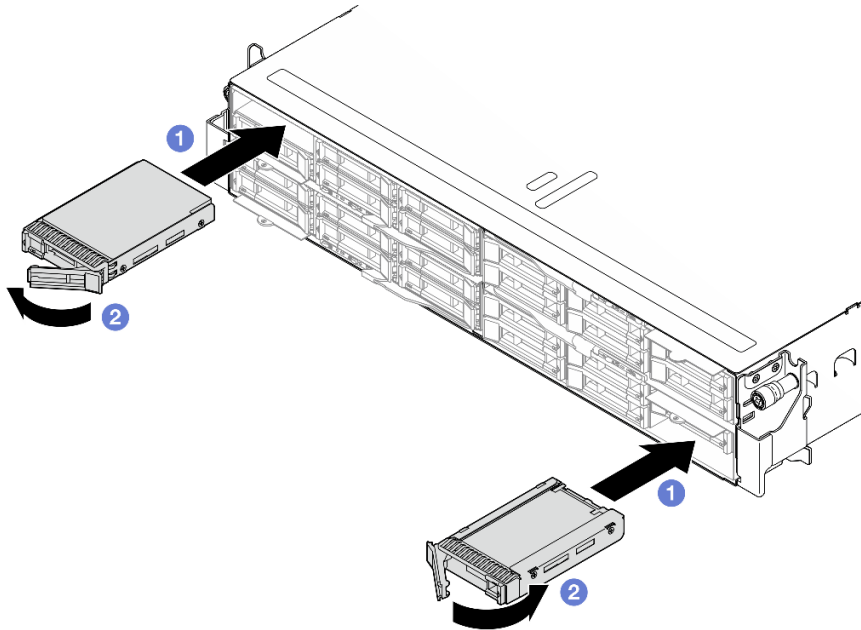
그림 47. 솔리드 스테이트 드라이브 설치
