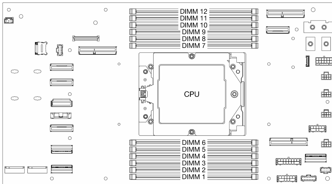
그림 70. 메모리 모듈 및 프로세서 레이아웃
