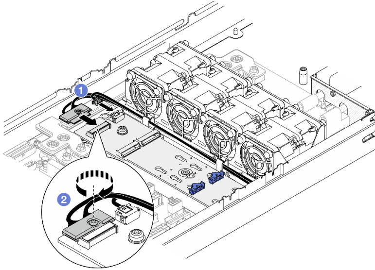
그림 58. NVMe M.2 부트 어댑터에 케이블 연결
