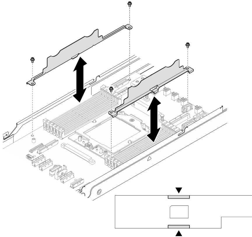
그림 111. 케이블 벽 교체
