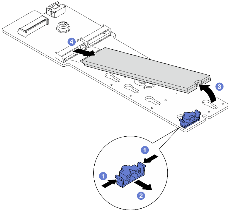
그림 51. M.2 드라이브 제거
