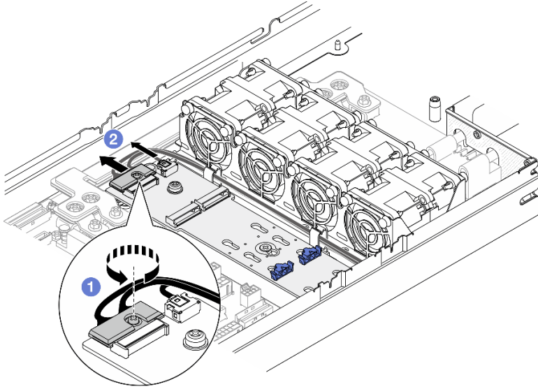
그림 52. NVMe M.2 부트 어댑터에서 케이블 분리
