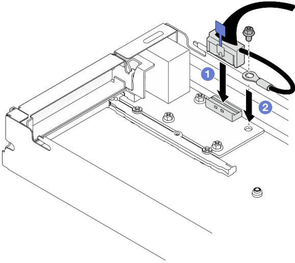
그림 133. 뒷면 I/O 케이블 및 접지 케이블 설치
