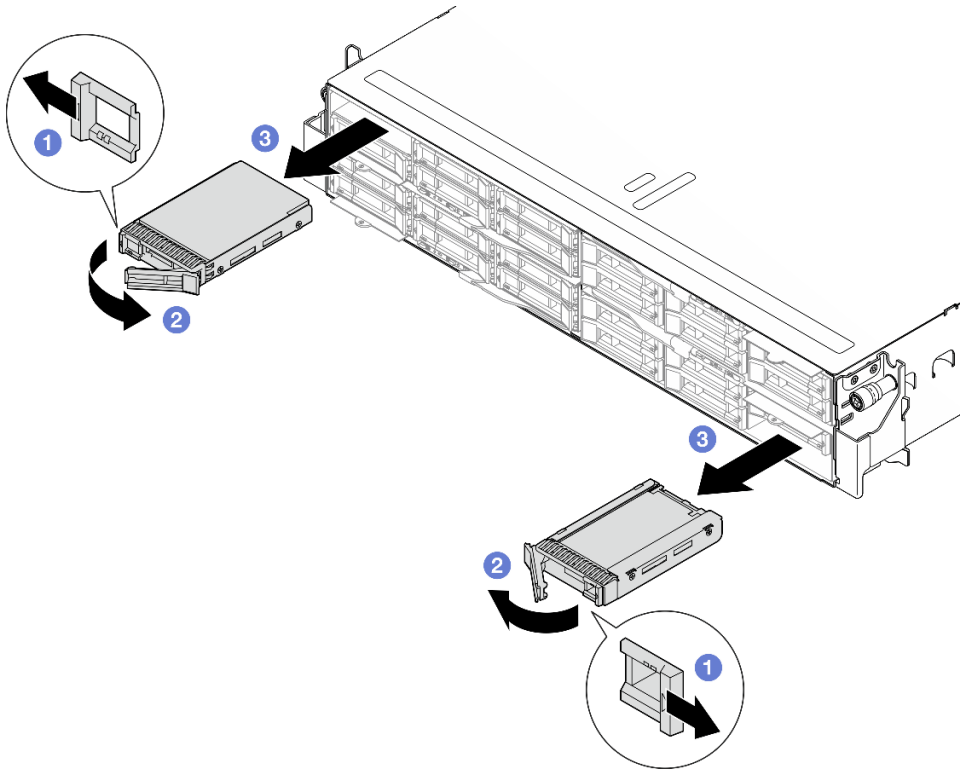
그림 44. 솔리드 스테이트 드라이브 제거
