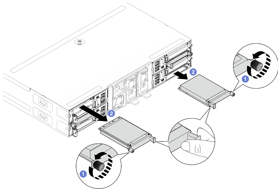
그림 76. 뒷면 OCP 모듈 제거
