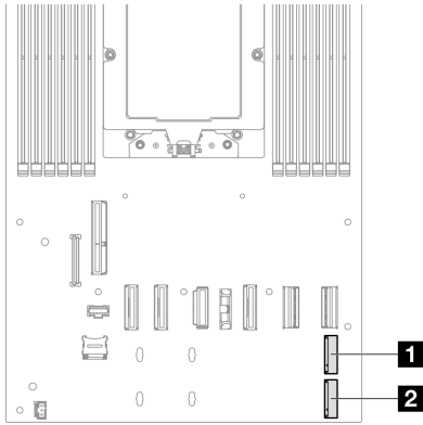
그림 62. 시스템 보드에서 M.2 베이의 위치
