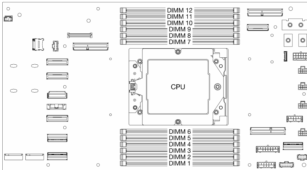
그림 1. 메모리 모듈 및 프로세서 레이아웃
