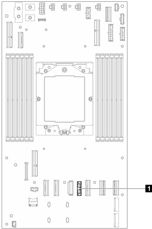
그림 28. CMOS 배터리 소켓의 위치
