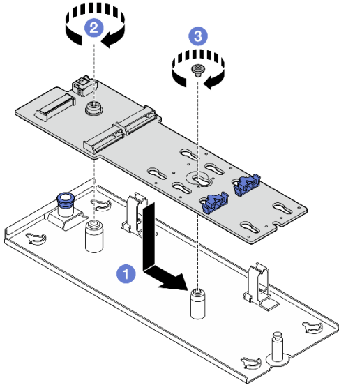
그림 56. M.2 부트 어댑터 설치
