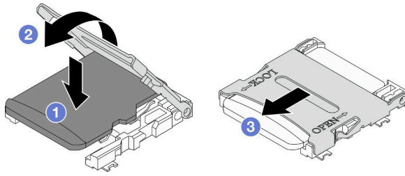
그림 75. MicroSD 카드 설치
