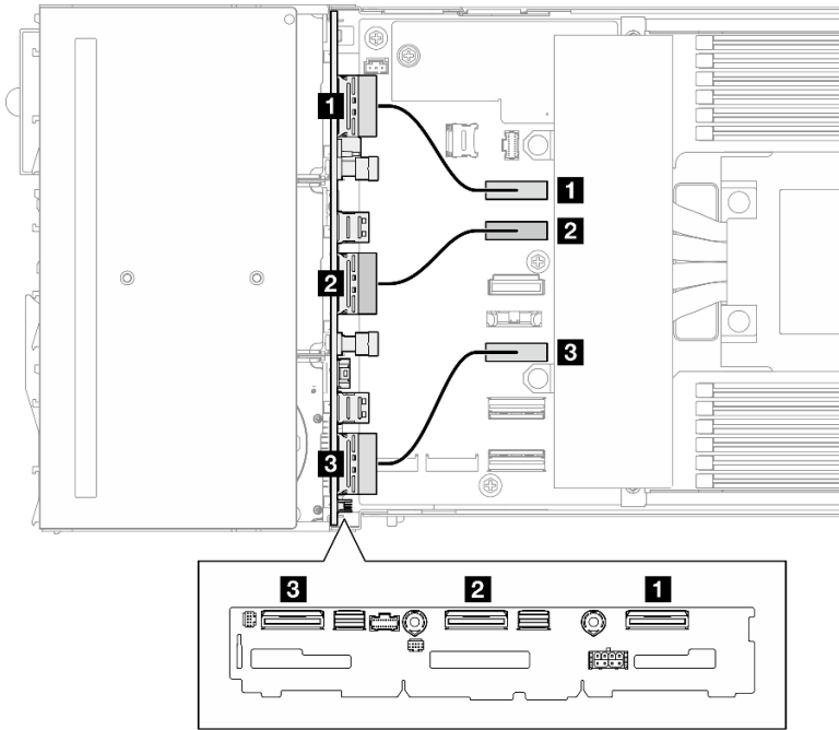
그림 121. NVMe 케이블 배선
