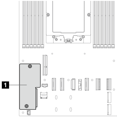
그림 102. 펌웨어 및 RoT 보안 모듈의 위치
