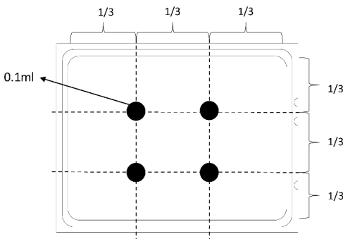
그림 96. 열전도 그리스 도포
