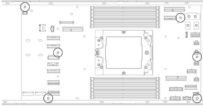
그림 107. 나사 제거
