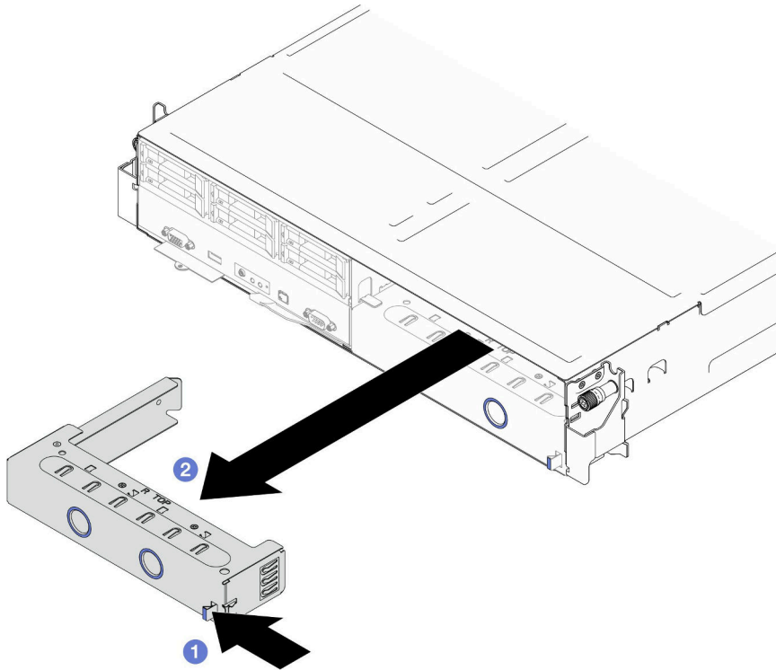
그림 20. 앞면 노드 트레이 필터 제거
