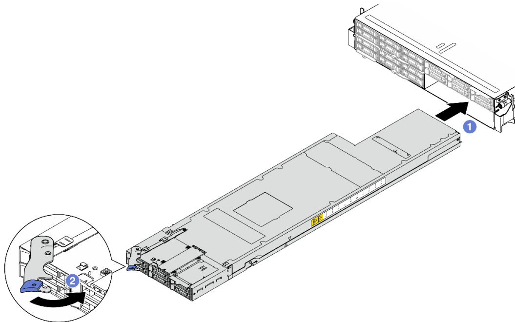
그림 23. 오른쪽 트레이에 노드 설치
