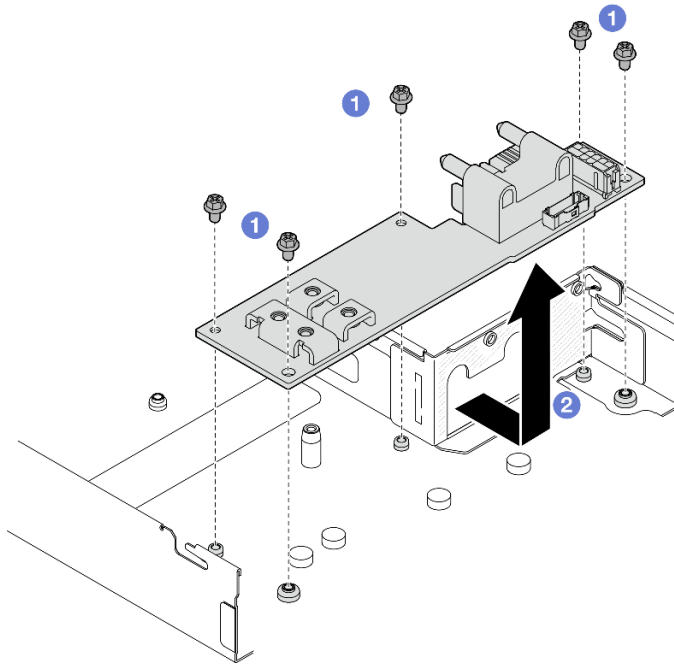
그림 89. 전원 분배 보드 제거
