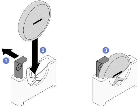
그림 29. CMOS 배터리 설치
