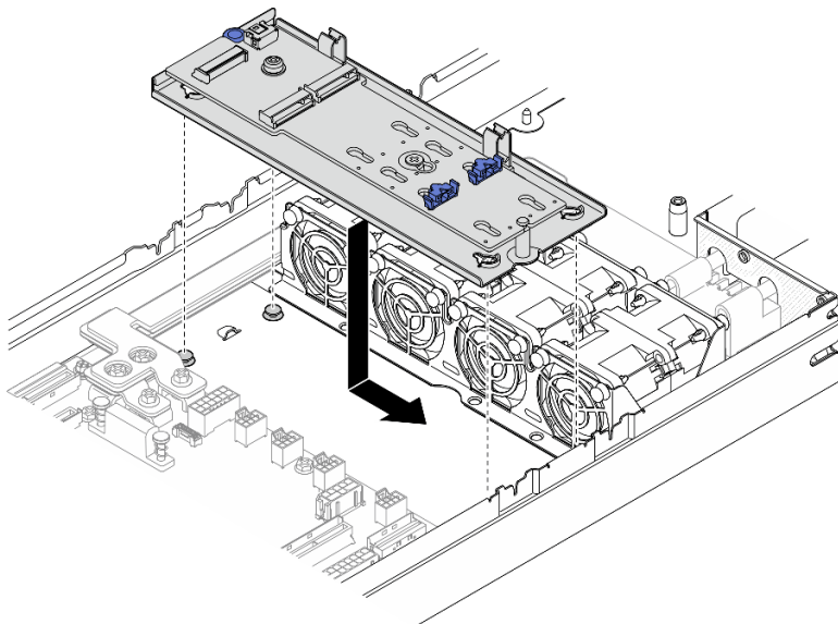
그림 57. M.2 부트 어댑터 트레이 설치
