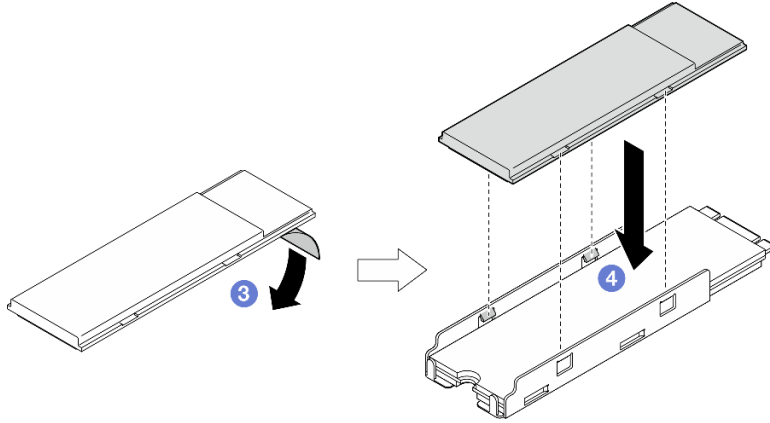
그림 64. M.2 트레이에 M.2 방열판 설치
