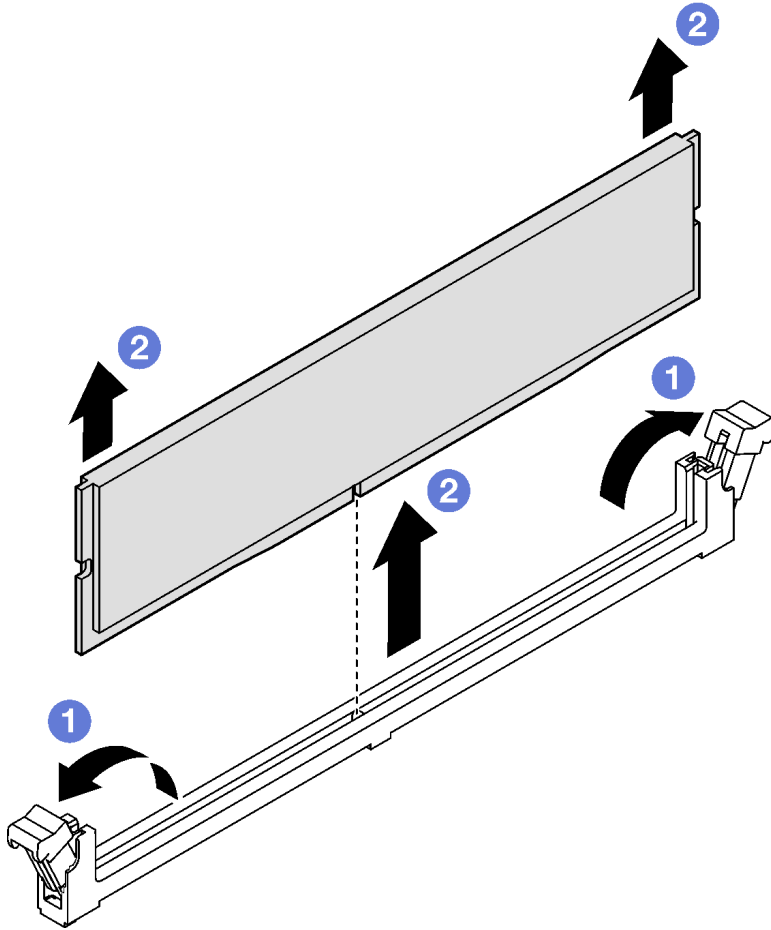
그림 69. 메모리 모듈 제거
