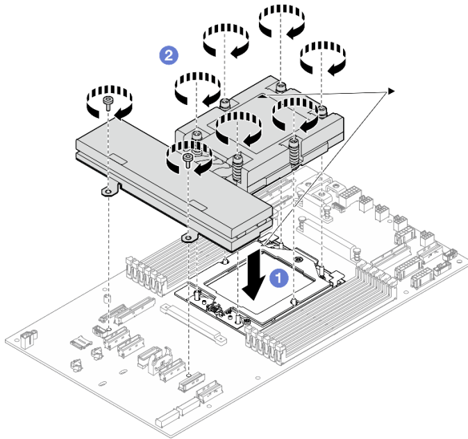
그림 97. 방열판 설치
