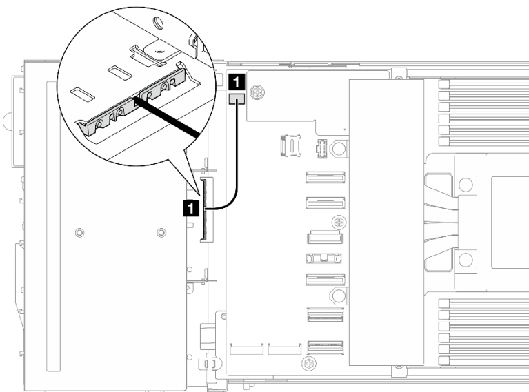
그림 134. 앞면 열 센서 케이블 배선
