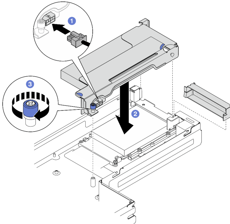
그림 84. PCIe 라이저 어셈블리 설치
