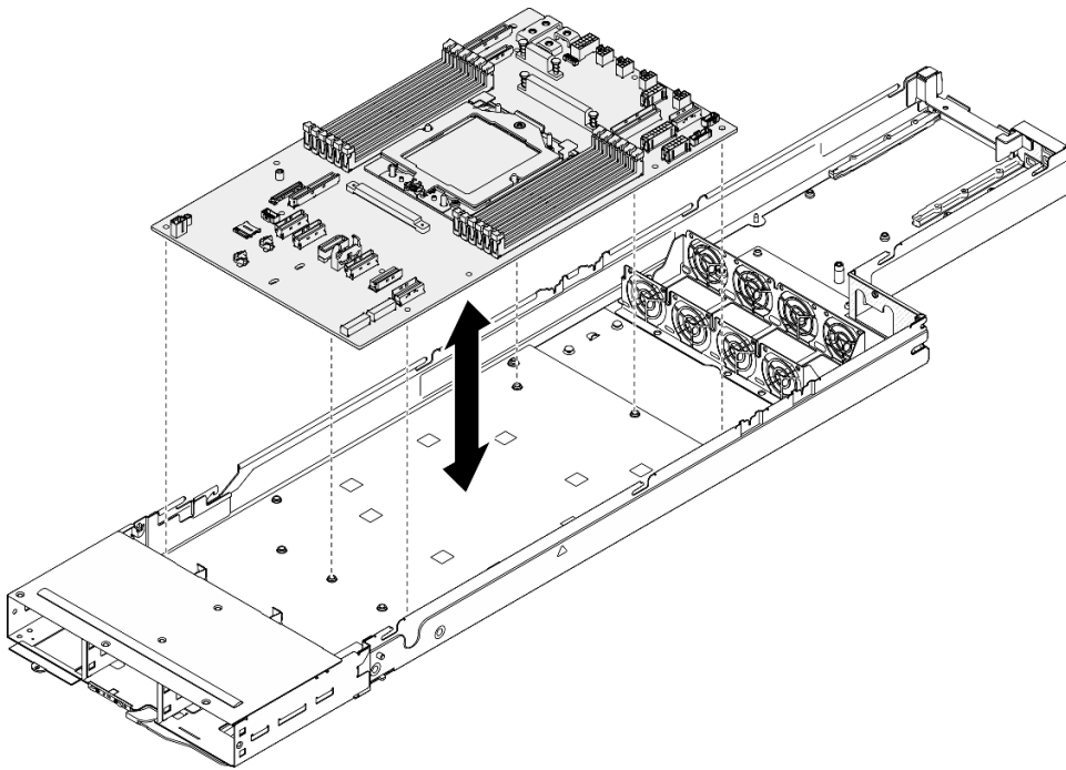
그림 108. 시스템 보드 제거
