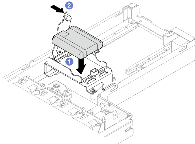
그림 37. 플래시 전원 모듈 설치
