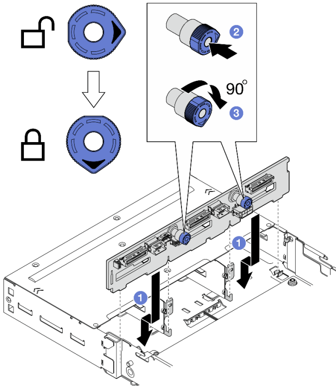
그림 31. 드라이브 백플레인 설치
