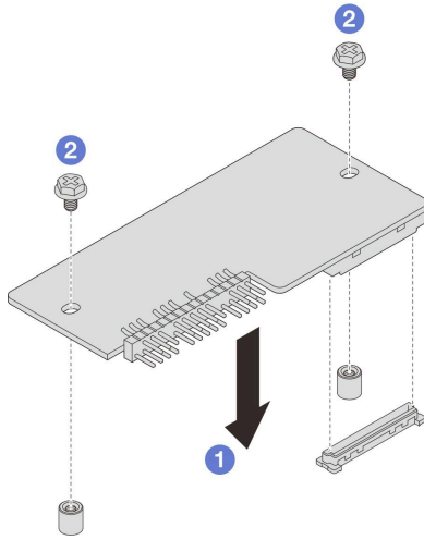
그림 105. 펌웨어 및 RoT 보안 모듈 설치
