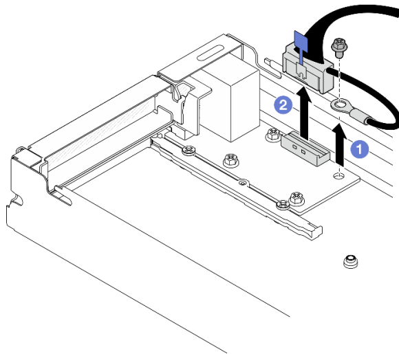
그림 98. 뒷면 I/O 케이블 및 접지 케이블 제거
