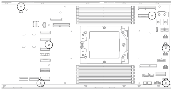
그림 110. 나사 설치
