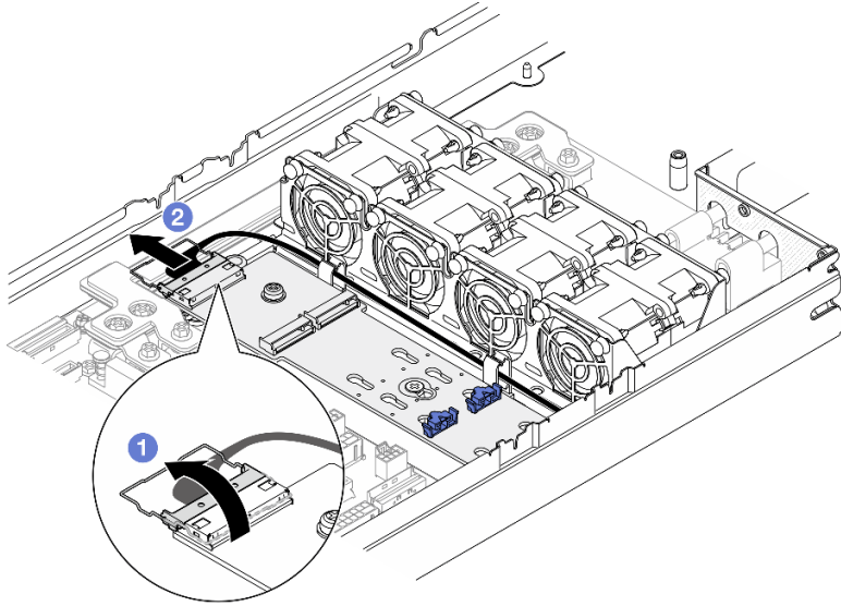
그림 53. SATA/NVMe M.2 부트 어댑터에서 케이블 분리
