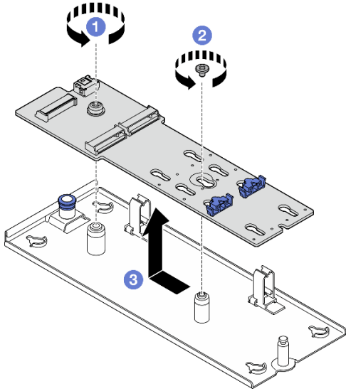
그림 69. M.2 부트 어댑터 제거
