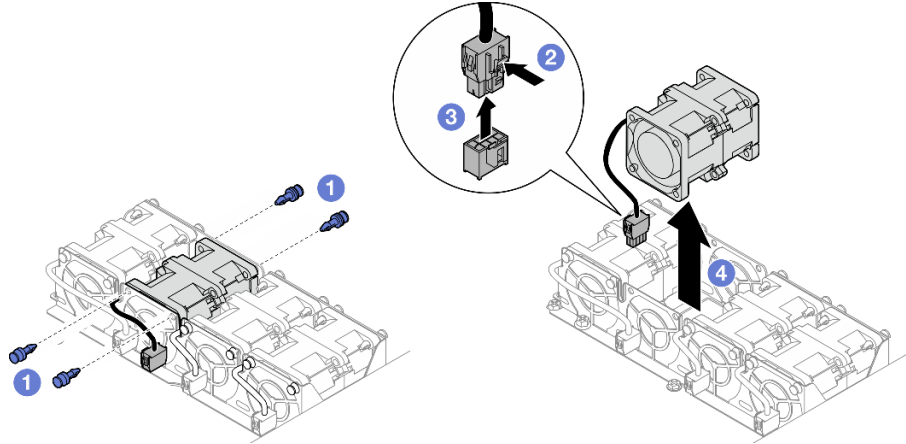
그림 46. 팬 제거
