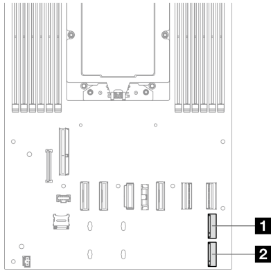
그림 76. 시스템 보드에서 M.2 베이의 위치
