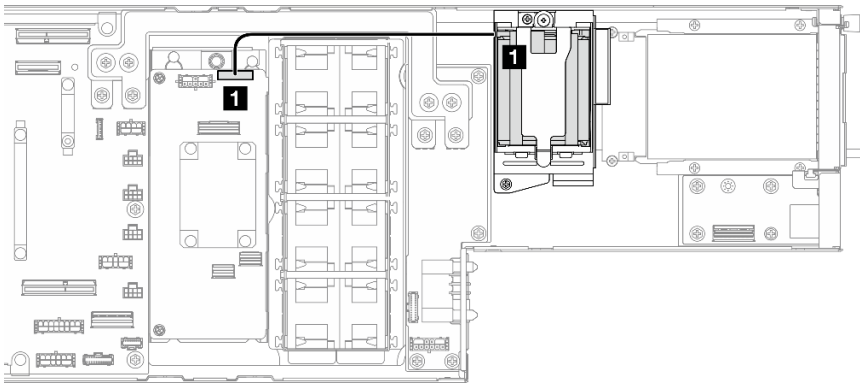
그림 139. 플래시 전원 모듈 케이블 배선
