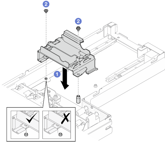
그림 50. 플래시 전원 모듈 홀더 설치
