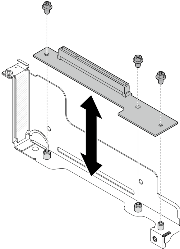
그림 95. PCIe 라이저 카드 교체
