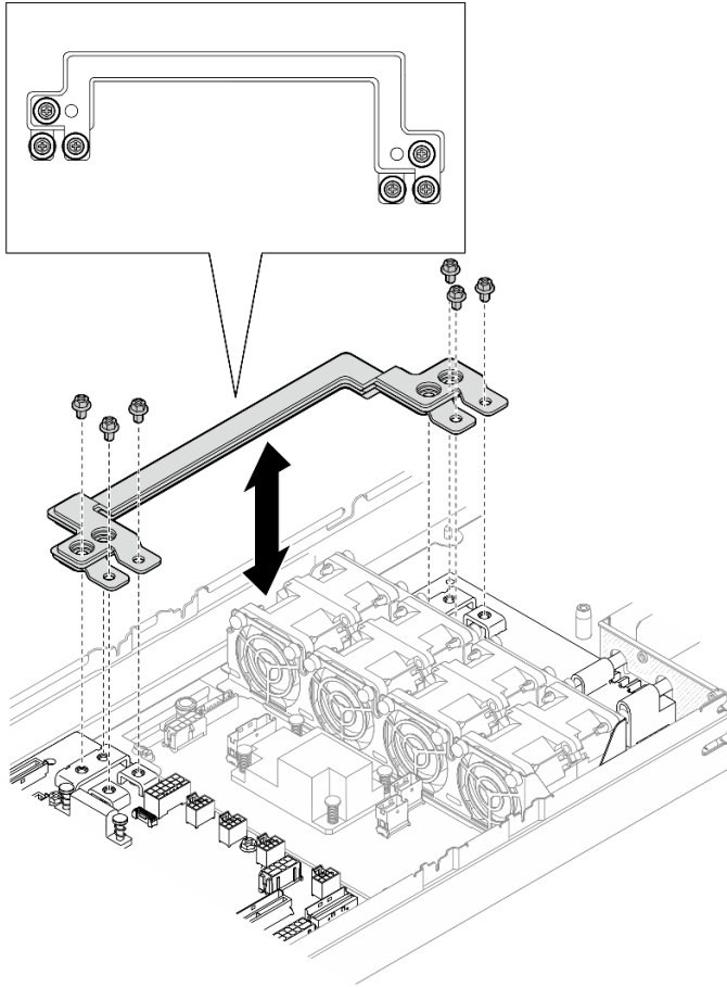
그림 102. 전원 버스 바 외부 나사 설치
