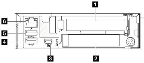
그림 4. 뒷면 보기
