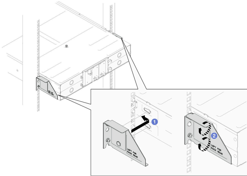
그림 19. 운반 브래킷 설치
