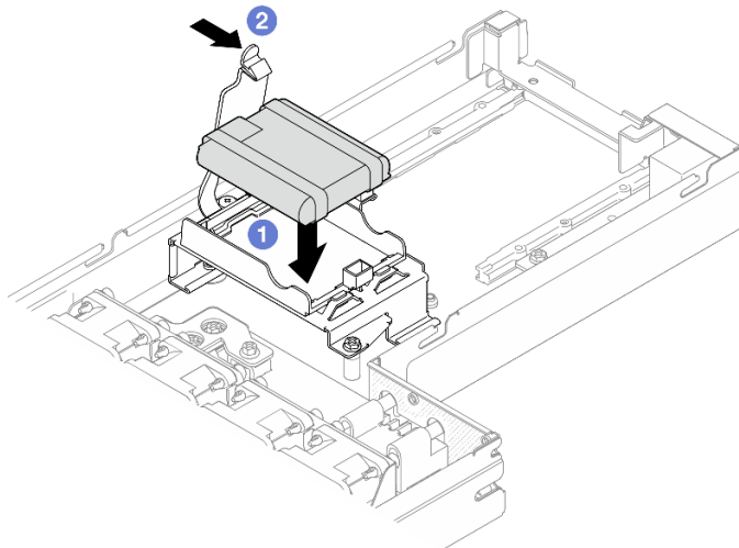
그림 51. 플래시 전원 모듈 설치
