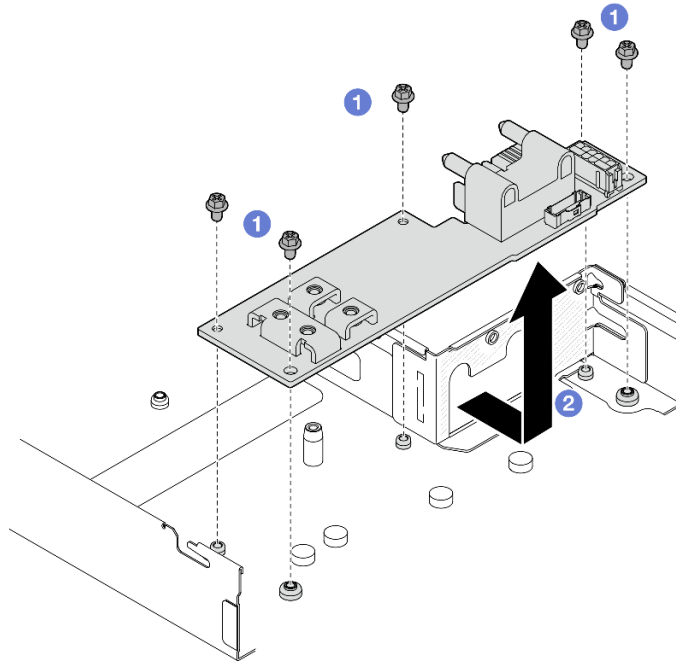
그림 103. 전원 분배 보드 제거
