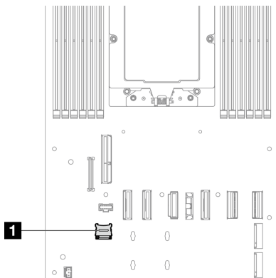
그림 86. MicroSD 소켓의 위치
