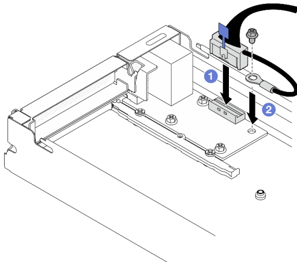
그림 115. 뒷면 I/O 케이블 및 접지 케이블 설치
