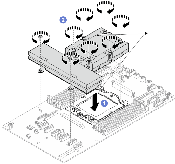
그림 111. 방열판 설치
