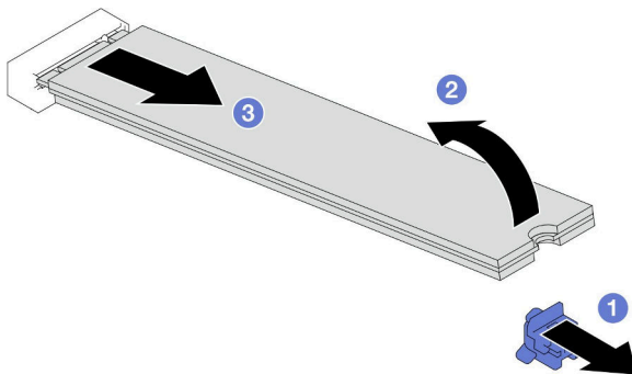
그림 63. M.2 드라이브 제거
