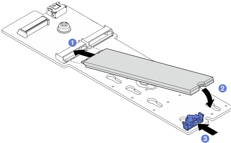
그림 81. M.2 드라이브 설치
