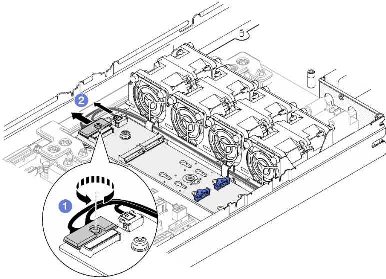
그림 66. NVMe M.2 부트 어댑터에서 케이블 분리
