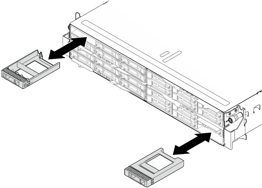
그림 59. 드라이브 필터 교체
