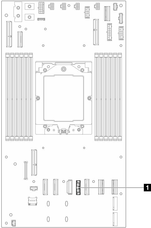
그림 42. CMOS 배터리 소켓의 위치
