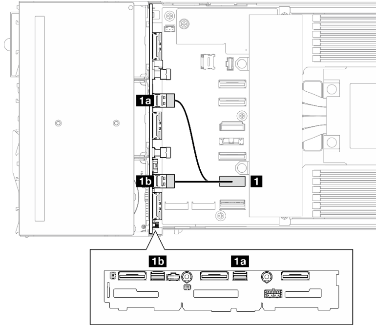
그림 136. 온보드 SATA 케이블 배선
