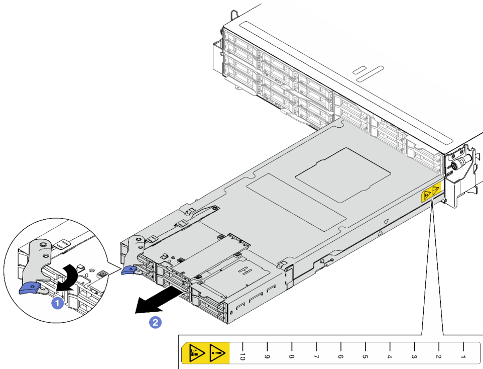
그림 31. 오른쪽 트레이에서 노드 제거
