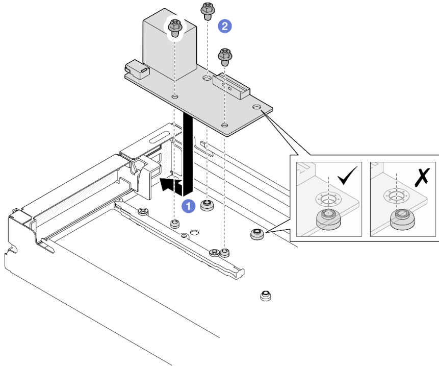
그림 114. 뒷면 I/O 모듈 설치
