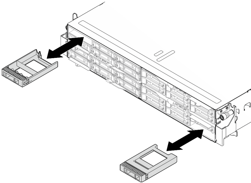
그림 60. 드라이브 필터 교체
