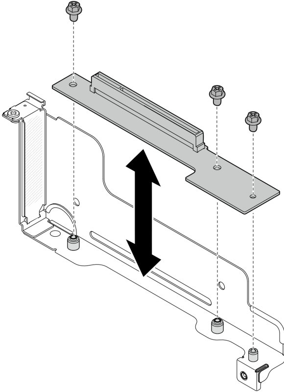
그림 93. PCIe 라이저 카드 교체
