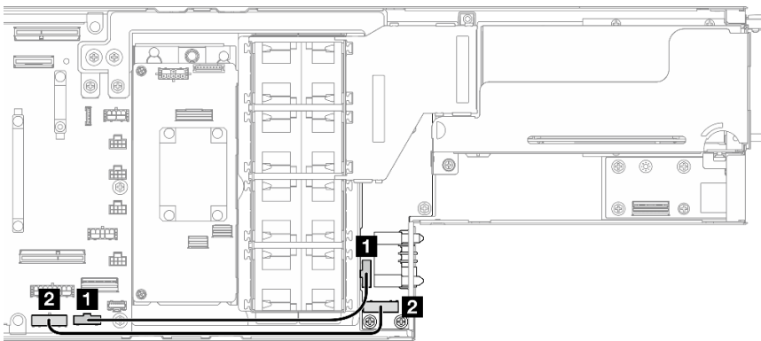
그림 145. 전원 분배 보드의 케이블 배선
