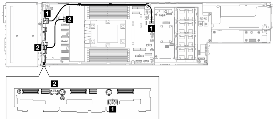
그림 134. 드라이브 백플레인 사이드밴드 및 전원 케이블 배선
