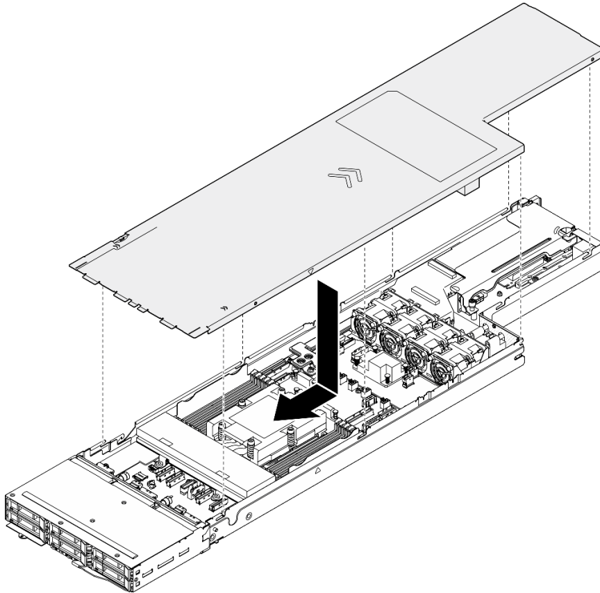
그림 127. 윗면 덮개 설치
