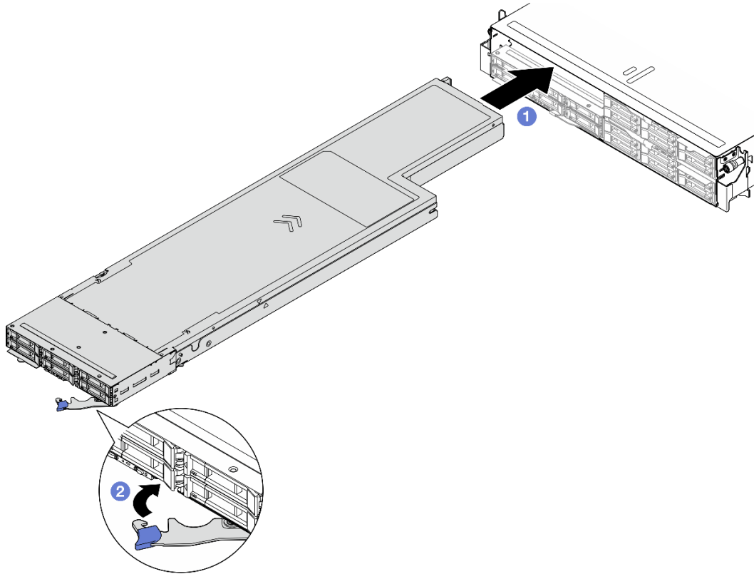
그림 36. 왼쪽 트레이에 노드 설치
