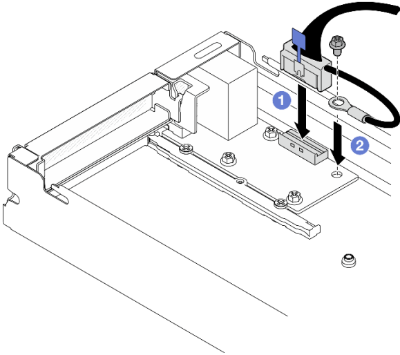
그림 147. 뒷면 I/O 케이블 및 접지 케이블 설치
