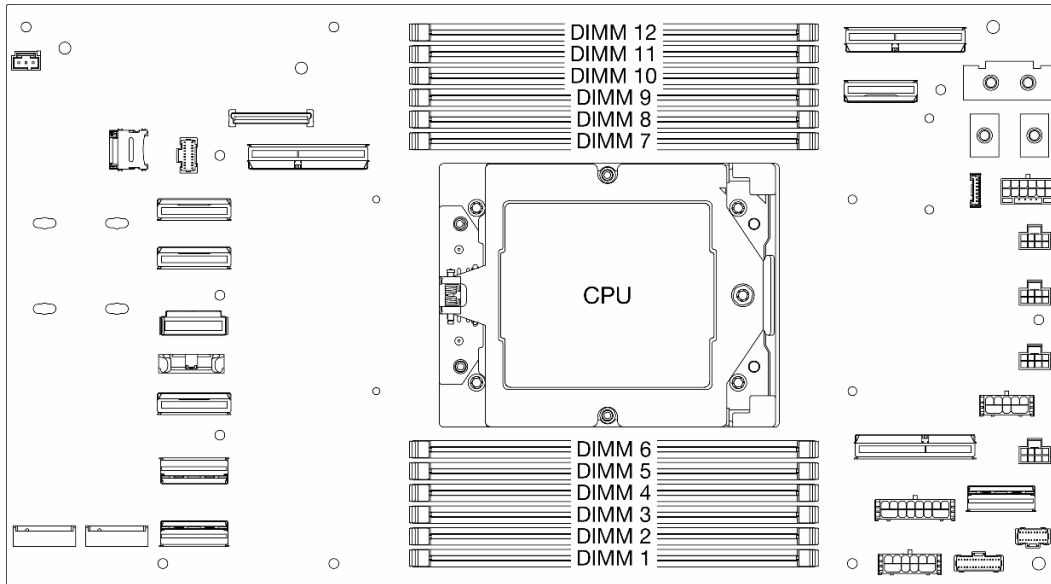
그림 82. 메모리 모듈 및 프로세서 레이아웃
