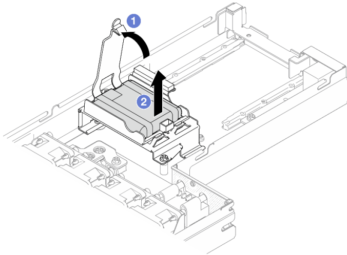
그림 48. 플래시 전원 모듈 제거
