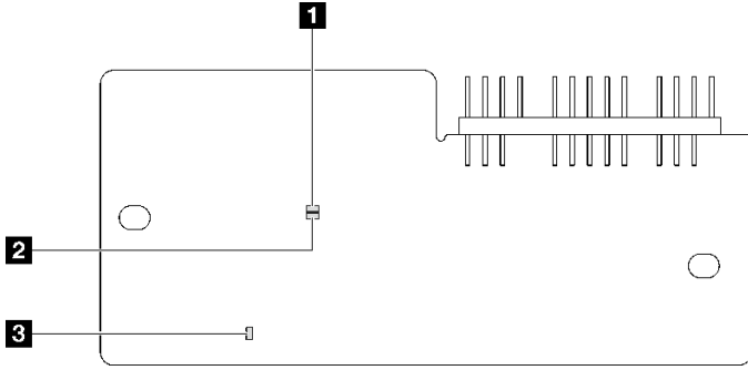
그림 154. 펌웨어 및 RoT 보안 모듈의 LED
