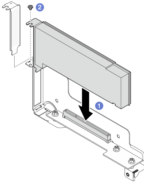
그림 96. PCIe 어댑터 설치
