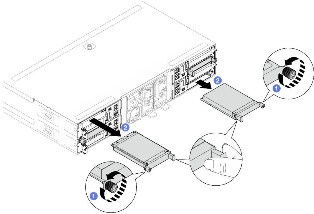
그림 90. 뒷면 OCP 모듈 제거
