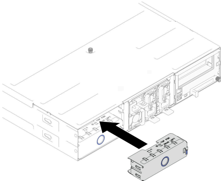
그림 33. 뒷면 노드 트레이 필러 설치
