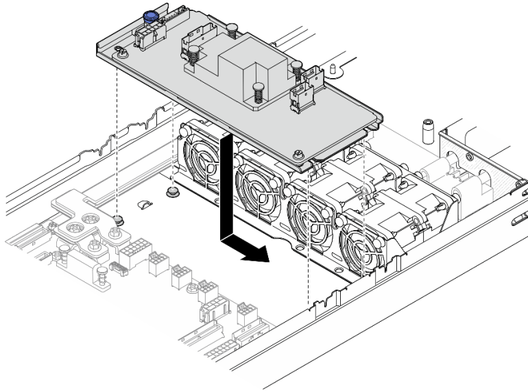
그림 39. 내부 CFF RAID 어댑터 설치
