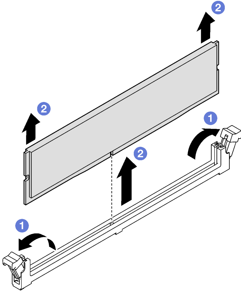
그림 83. 메모리 모듈 제거
