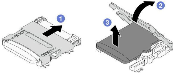
그림 87. MicroSD 카드 제거
