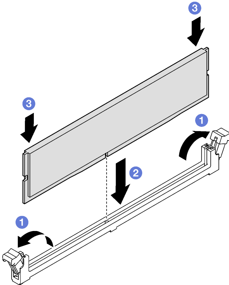
그림 85. 메모리 모듈 설치
