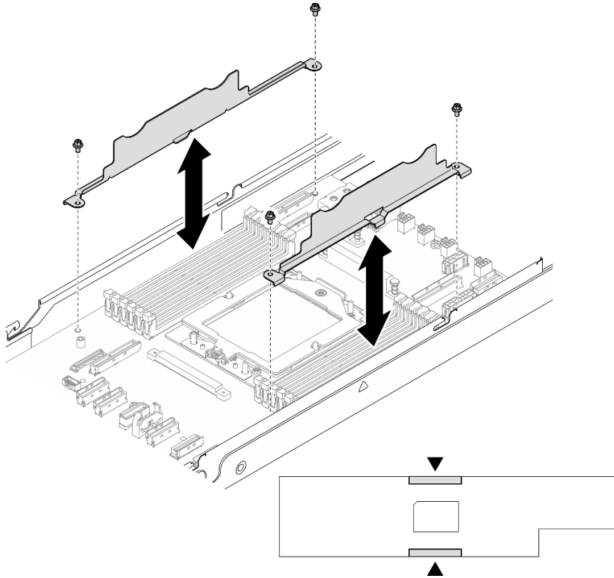
그림 120. 케이블 벽 교체
