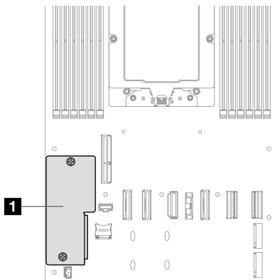
그림 118. 펌웨어 및 RoT 보안 모듈의 위치
