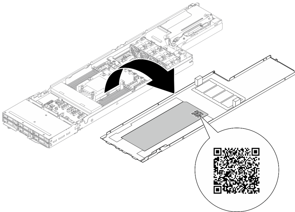
그림 14. 서비스 레이블 및 QR 코드
