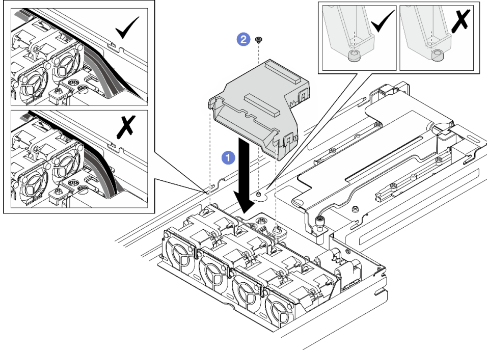
그림 57. GPU 통풍관 설치
