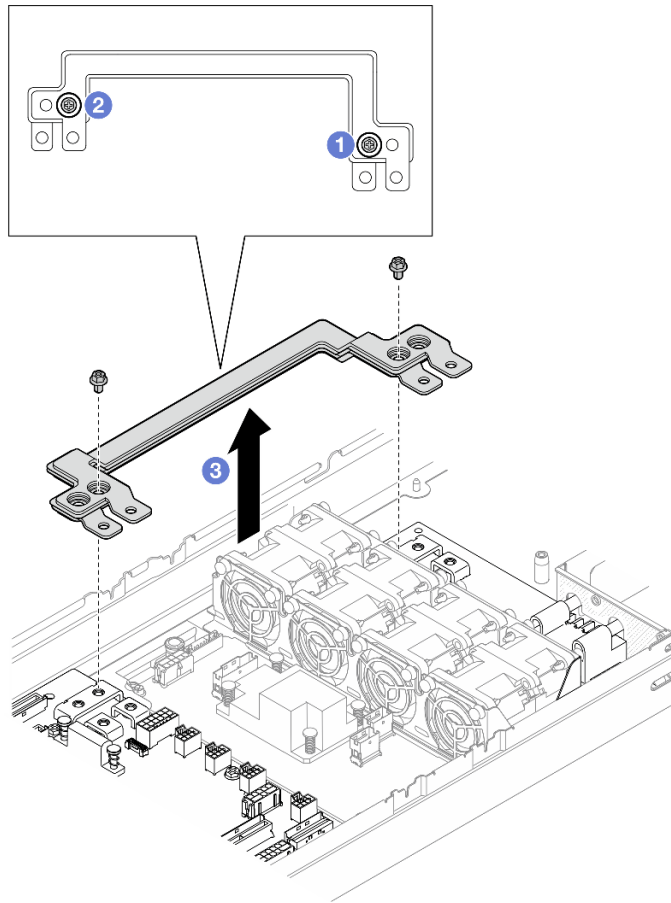
그림 100. 전원 버스 바 제거
