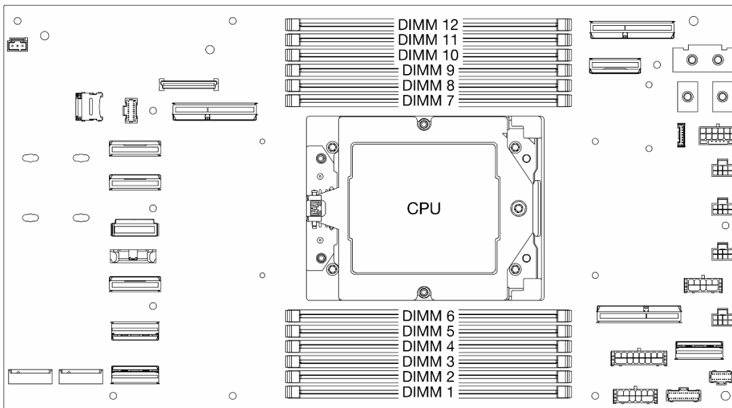
그림 15. 메모리 모듈 및 프로세서 레이아웃
