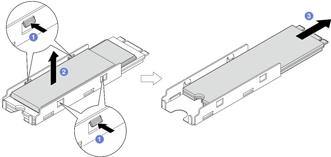
그림 64. M.2 방열판 제거
