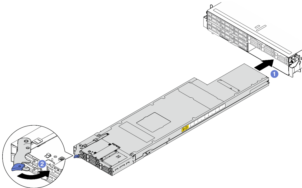
그림 37. 오른쪽 트레이에 노드 설치
