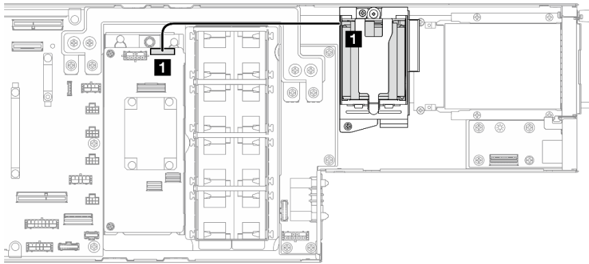
그림 53. CFF RAID 및 플래시 전원 모듈 케이블
