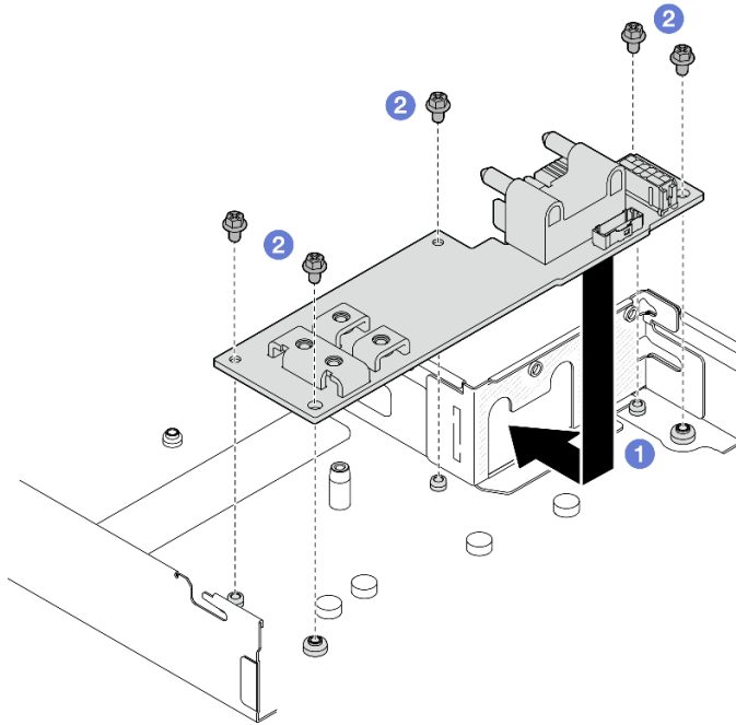
그림 104. 전원 분배 보드 설치
