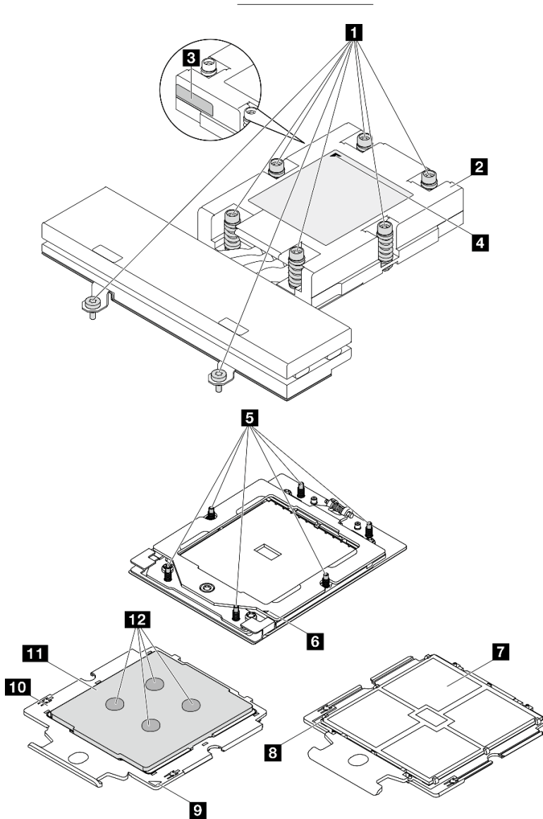
그림 108. 프로세서 및 방열판 구성 요소
