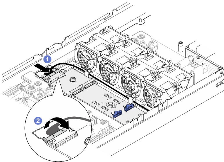
그림 73. SATA/NVMe M.2 부트 어댑터에 케이블 연결
