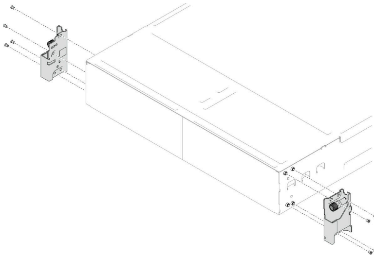
그림 20. EIA 브래킷 제거
