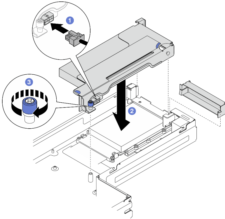
그림 98. PCIe 라이저 어셈블리 설치
