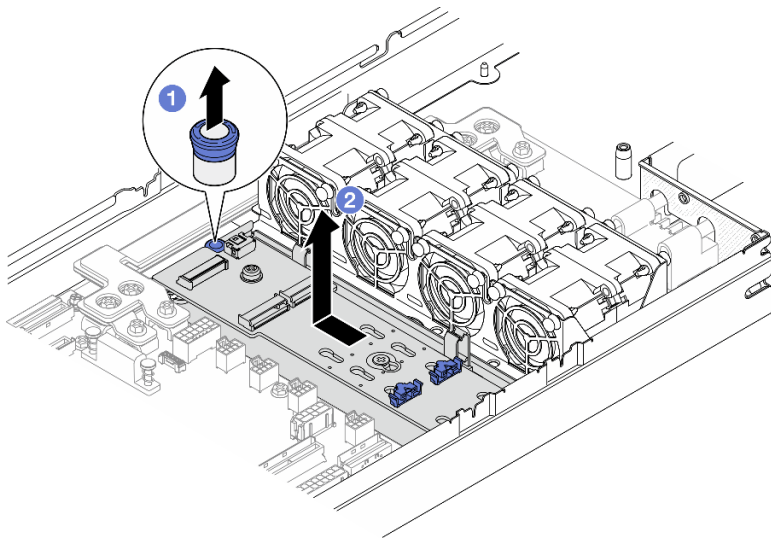
그림 68. M.2 부트 어댑터 트레이 제거
