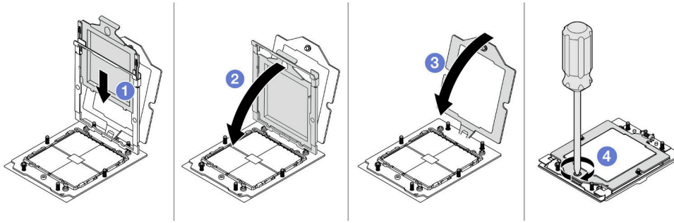
그림 109. 프로세서 설치
