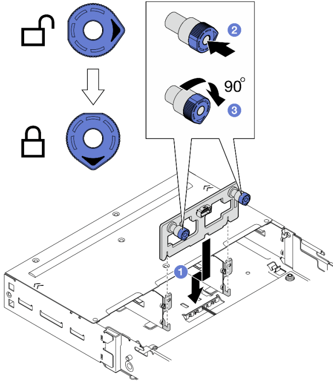
그림 55. 앞면 I/O 백플레인 설치
