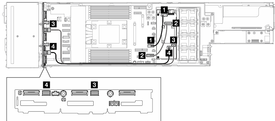
그림 137. CFF RAID 케이블 배선
