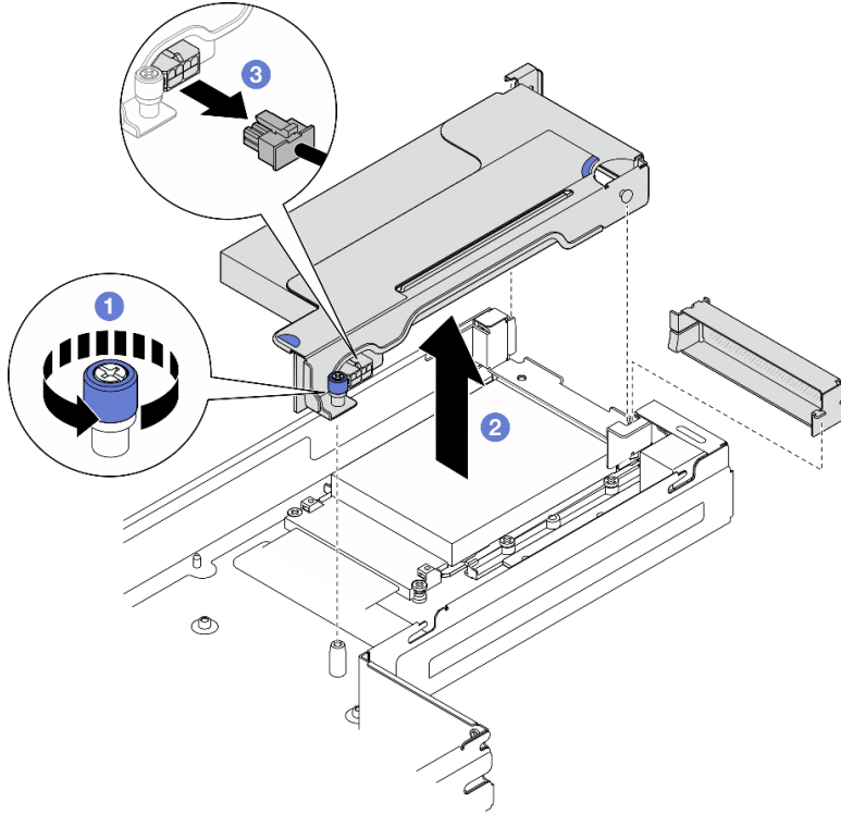
그림 92. PCIe 라이저 어셈블리 제거
