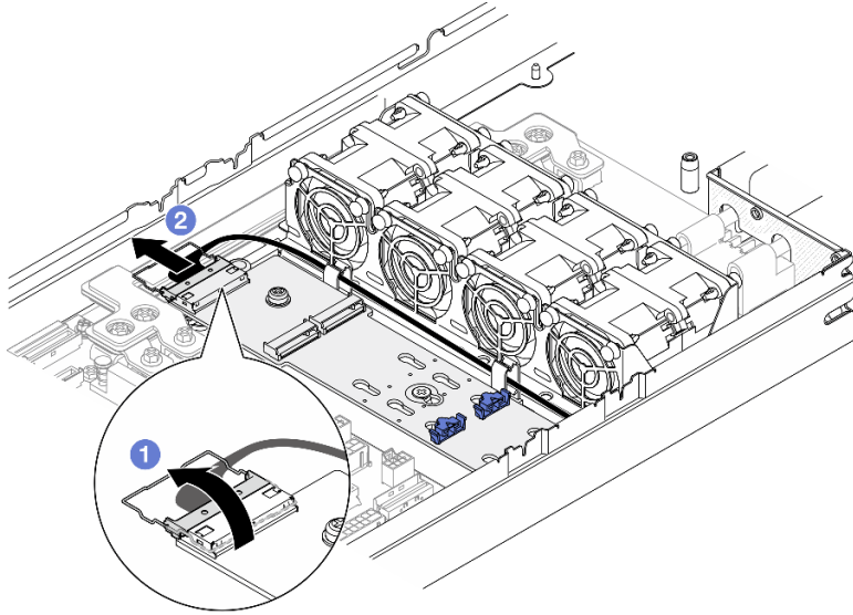
그림 67. SATA/NVMe M.2 부트 어댑터에서 케이블 분리
