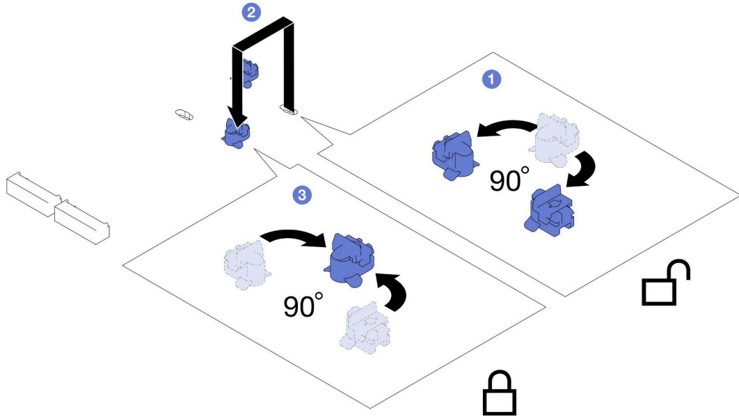
그림 74. M.2 드라이브 고정장치 조정
