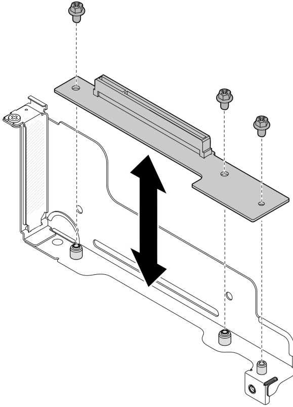
그림 97. PCIe 라이저 카드 교체
