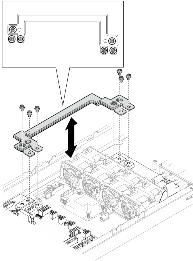
그림 99. 전원 버스 바의 외부 나사 제거
