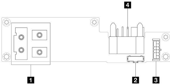
그림 133. 전원 분배 보드 커넥터
