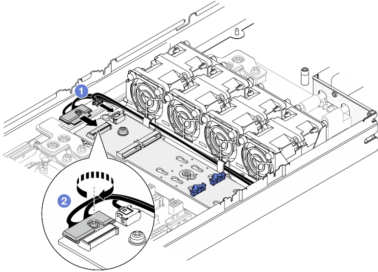
그림 72. NVMe M.2 부트 어댑터에 케이블 연결
