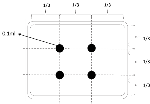
그림 110. 열전도 그리스 도포
