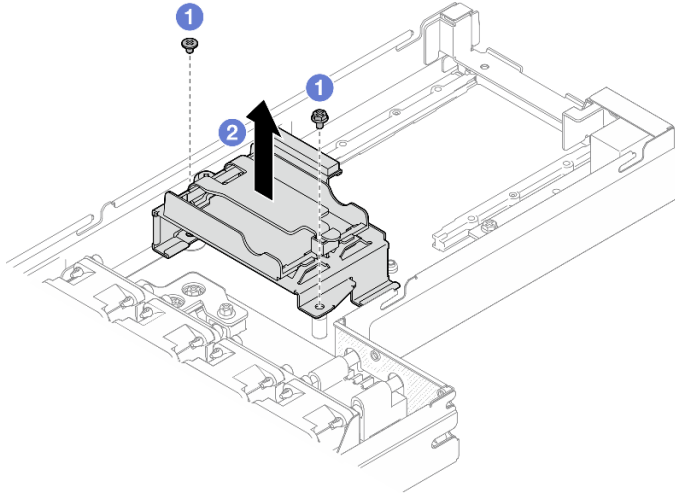
그림 49. 플래시 전원 모듈 홀더 제거
