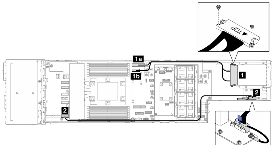
그림 146. 뒷면 I/O 모듈 및 OCP 모듈의 케이블
