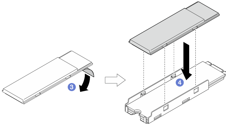
그림 78. M.2 트레이에 M.2 방열판 설치
