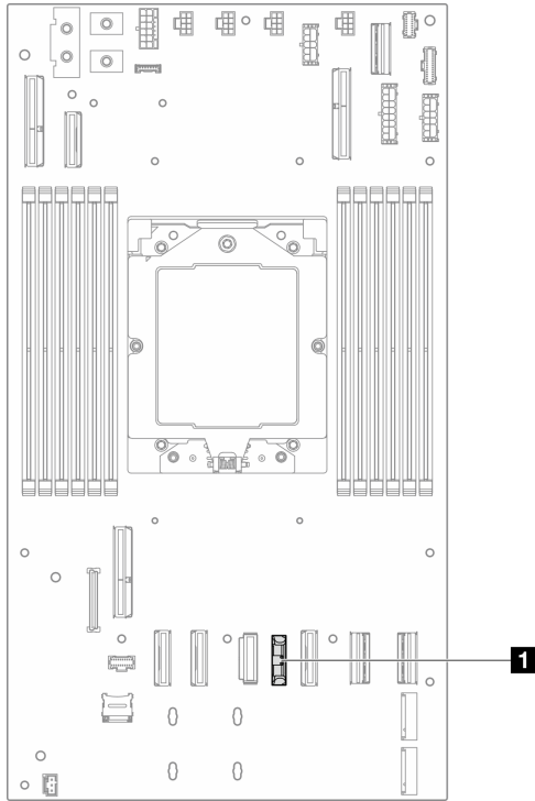
그림 40. CMOS 배터리 소켓의 위치
