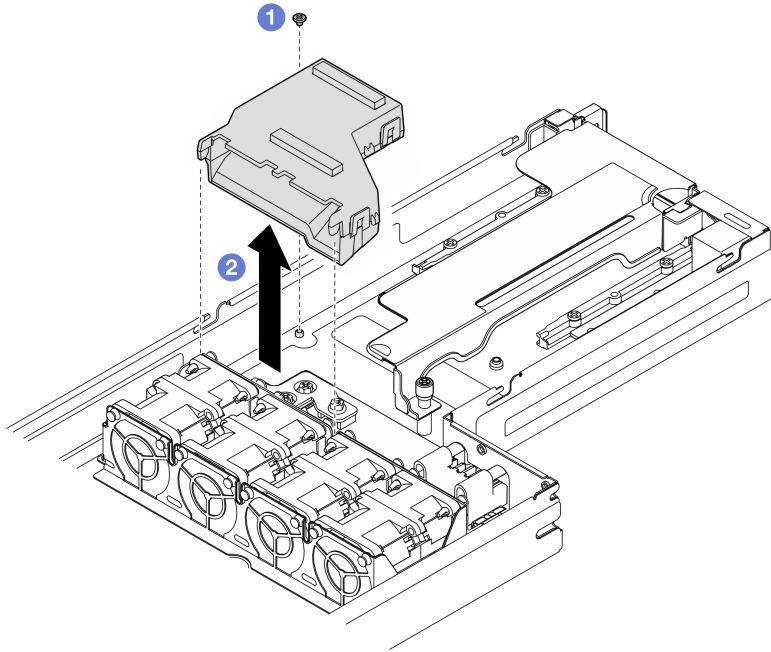
그림 56. GPU 통풍관 제거
