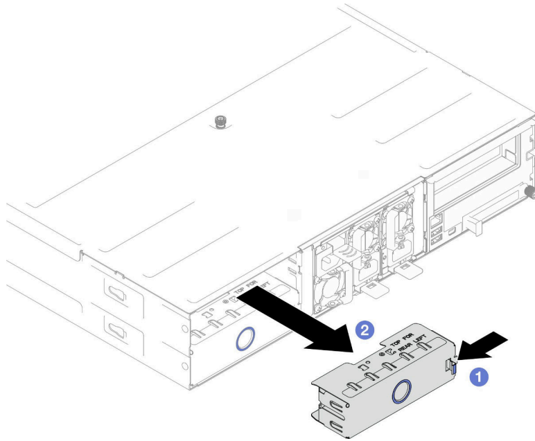
그림 35. 뒷면 노드 트레이 필러 제거
