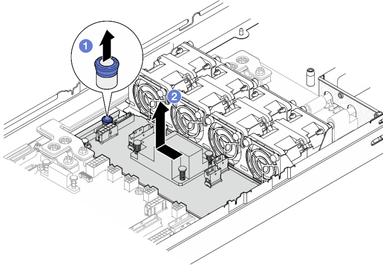
그림 38. 내부 CFF RAID 어댑터 제거
