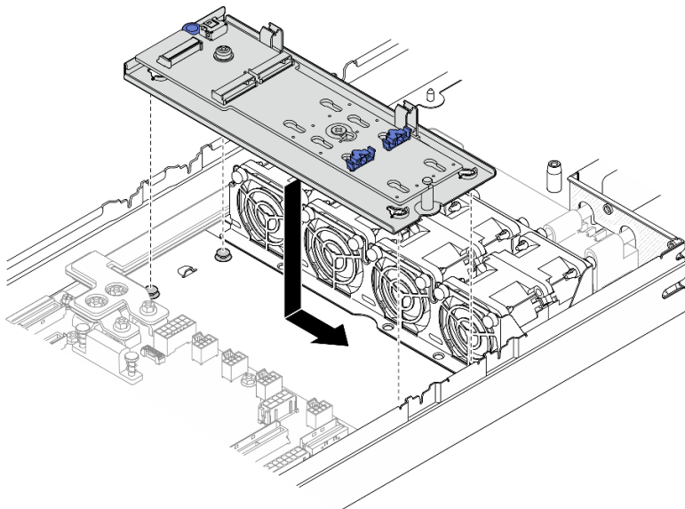
그림 71. M.2 부트 어댑터 트레이 설치
