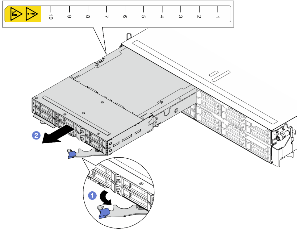
그림 30. 왼쪽 트레이에서 노드 제거
