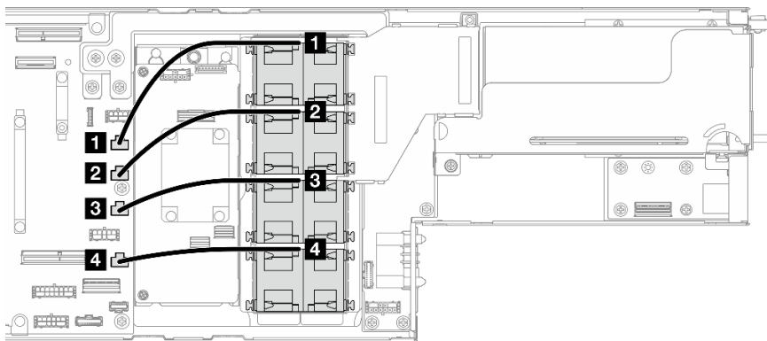
그림 141. 팬 케이블 배선
