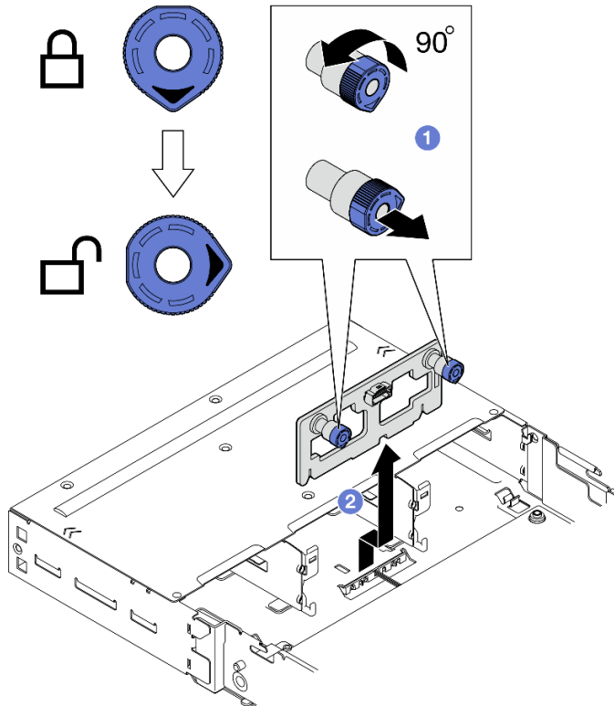
그림 54. 앞면 I/O 백플레인 제거
