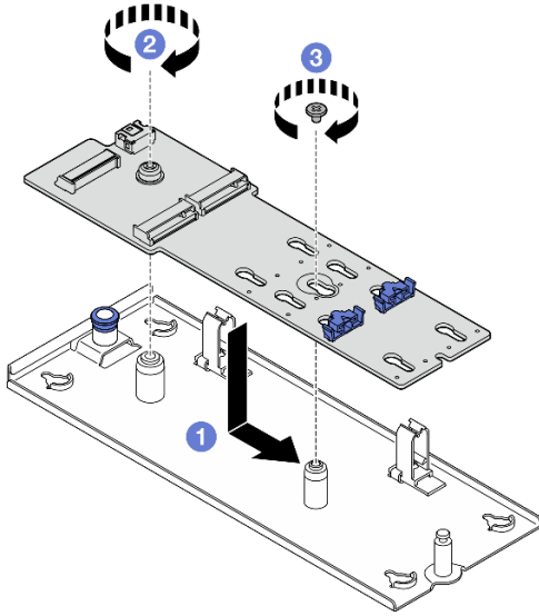
그림 70. M.2 부트 어댑터 설치
