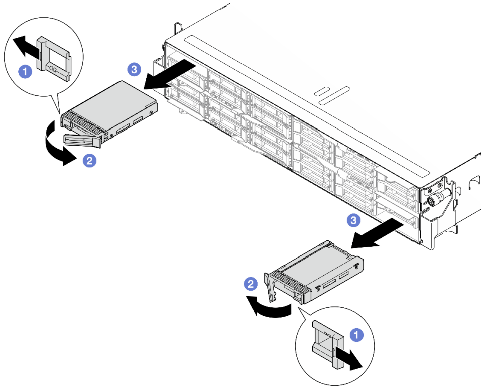
그림 58. 솔리드 스테이트 드라이브 제거
