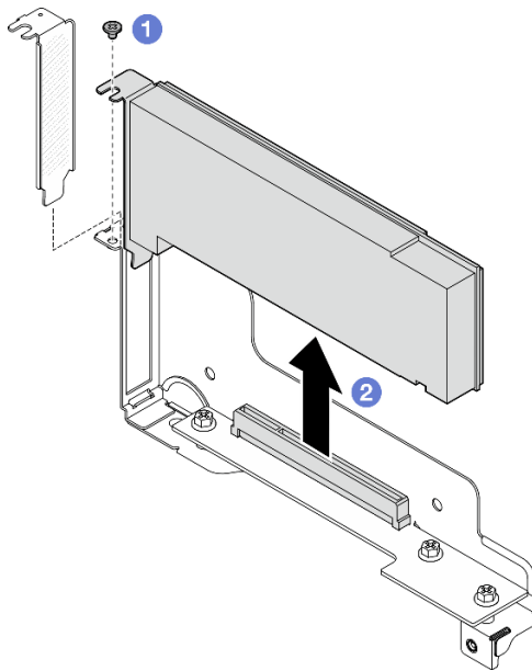
그림 94. PCIe 어댑터 제거
