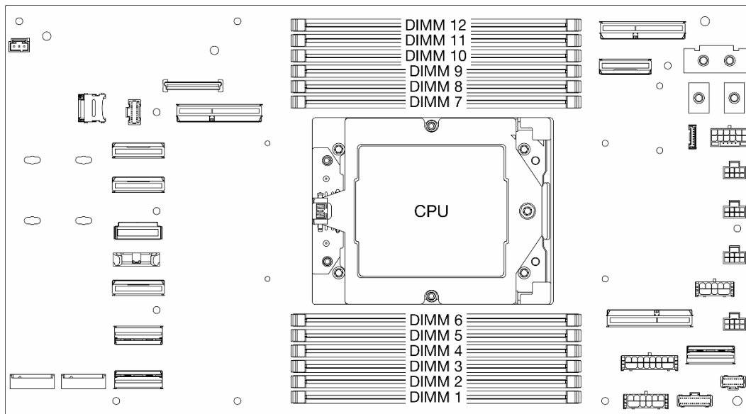
그림 84. 메모리 모듈 및 프로세서 레이아웃
