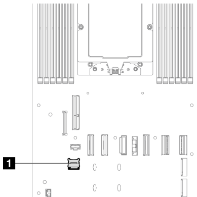
그림 88. MicroSD 소켓의 위치
