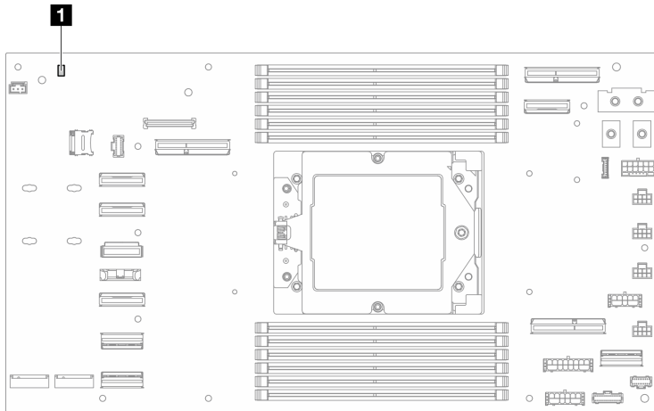
그림 155. 시스템 보드 LED
