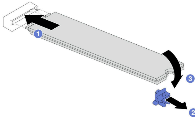
그림 79. M.2 드라이브 설치
