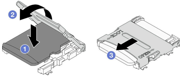
그림 89. MicroSD 카드 설치
