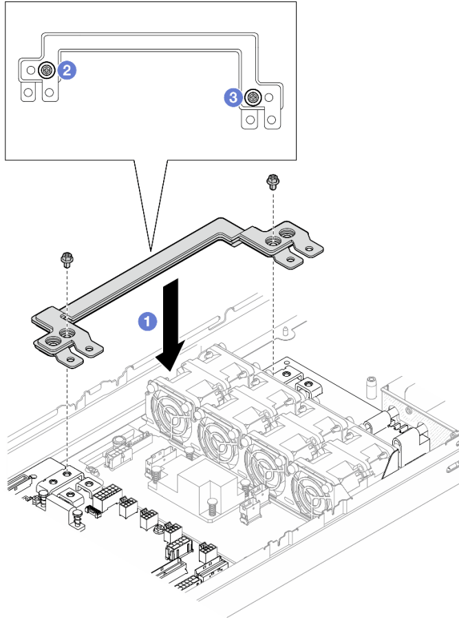
그림 101. 전원 버스 바 설치
