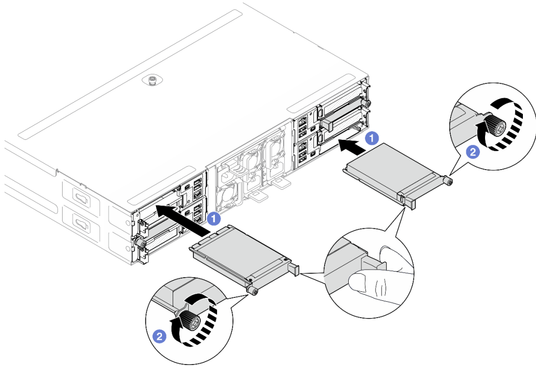
그림 91. 뒷면 OCP 모듈 설치
