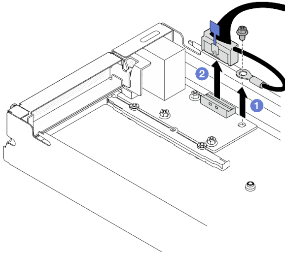
그림 112. 뒷면 I/O 케이블 및 접지 케이블 제거
