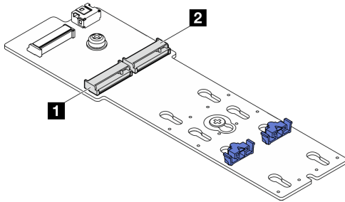
그림 80. M.2 드라이브 슬롯
