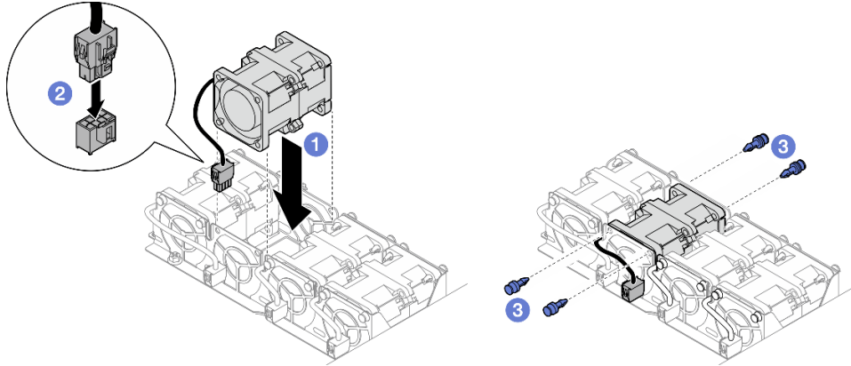
그림 47. 팬 설치
