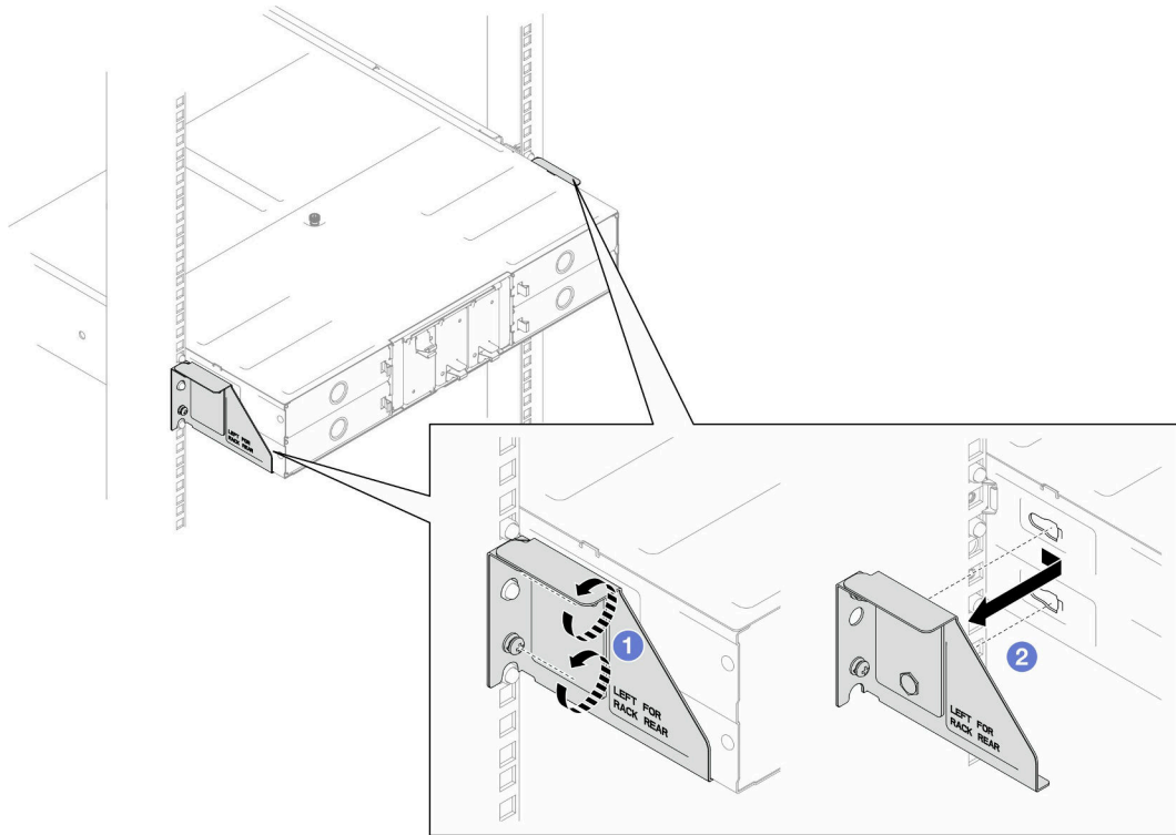
그림 16. 운반 브래킷 제거
