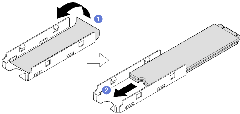
그림 77. 열 패드 및 M.2 드라이브를 트레이에 설치
