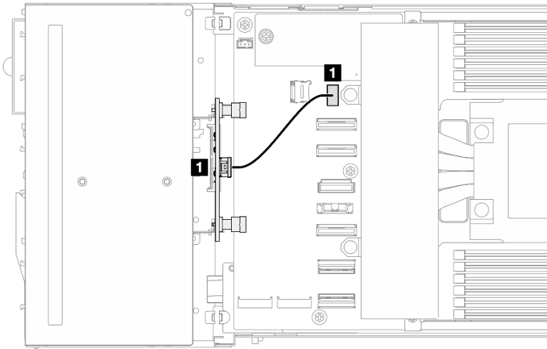
그림 142. 앞면 I/O 보드 케이블 배선
