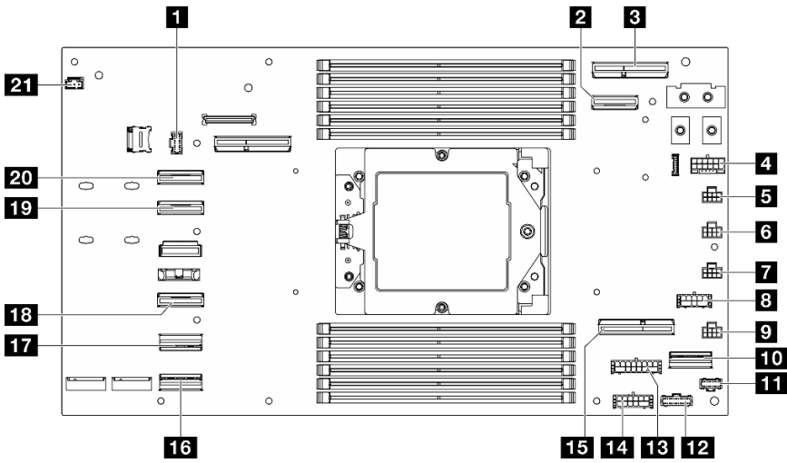
그림 128. 케이블 배선용 시스템 보드 커넥터
