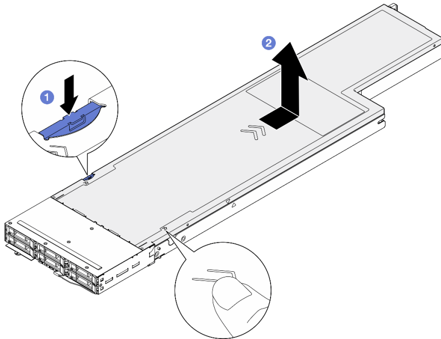
그림 126. 윗면 덮개 제거
