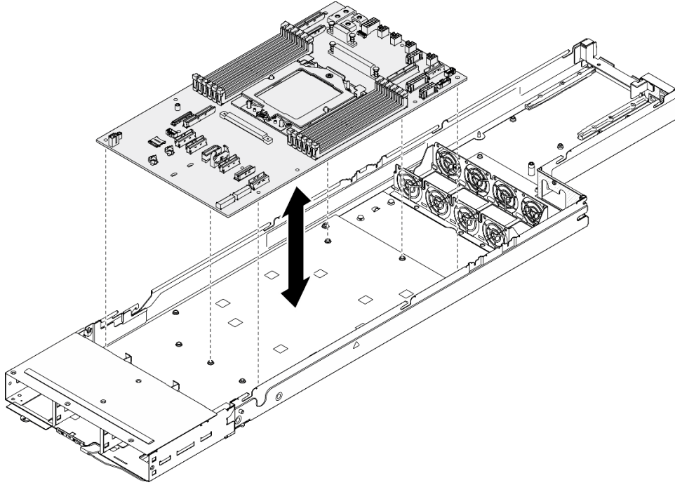
그림 123. 시스템 보드 설치
