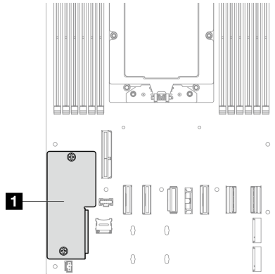
그림 116. 펌웨어 및 RoT 보안 모듈의 위치
