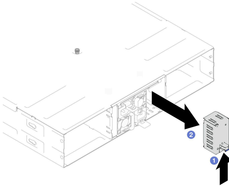
图 10. 卸下 PSU 填充件
