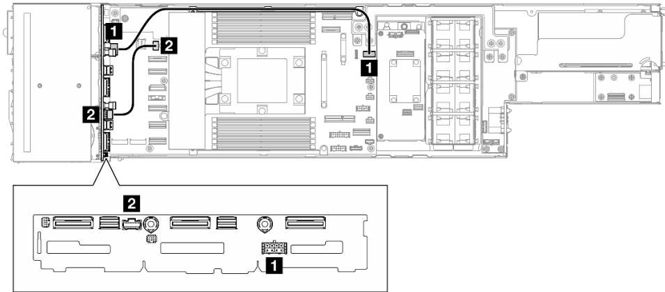
图 120. 硬盘背板边带及电源线布放
