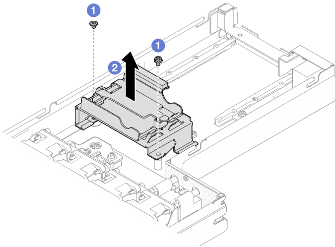
图 35. 卸下快速充电模块夹持器
