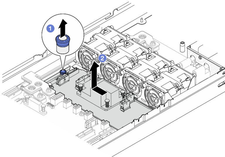
图 24. 卸下内部 CFF RAID 适配器
