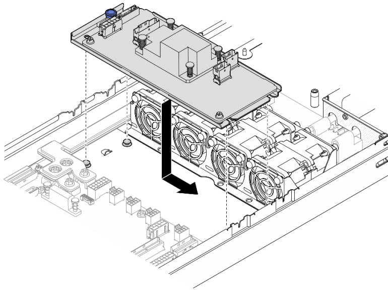
图 25. 安装内部 CFF RAID 适配器
