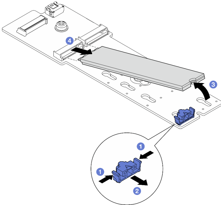
图 51. 卸下 M.2 硬盘
