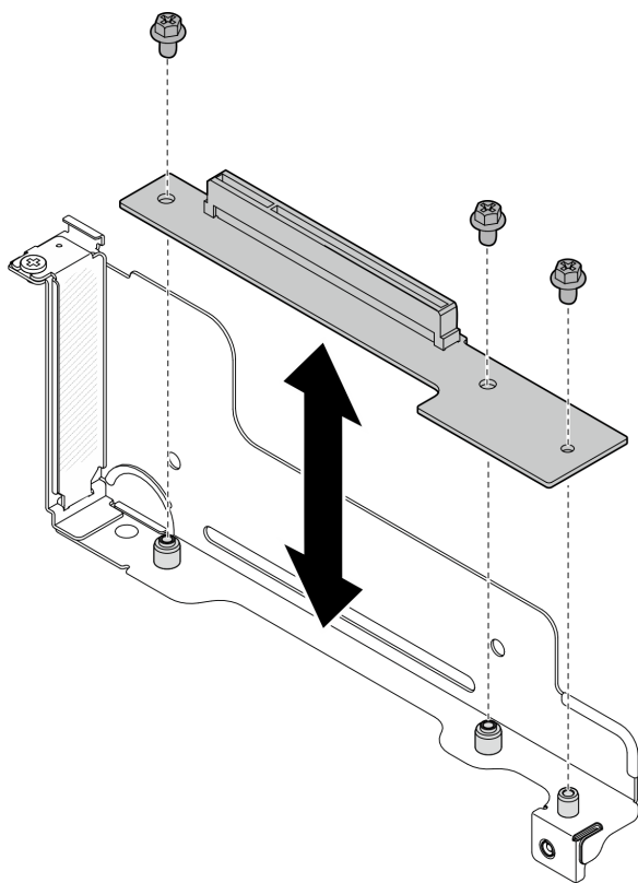
图 81. 更换 PCIe 转接卡
