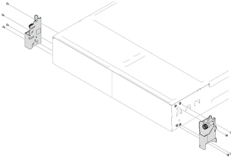
图 7. 安装 EIA 支架
