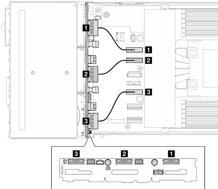
图 121. NVMe 线缆布放
