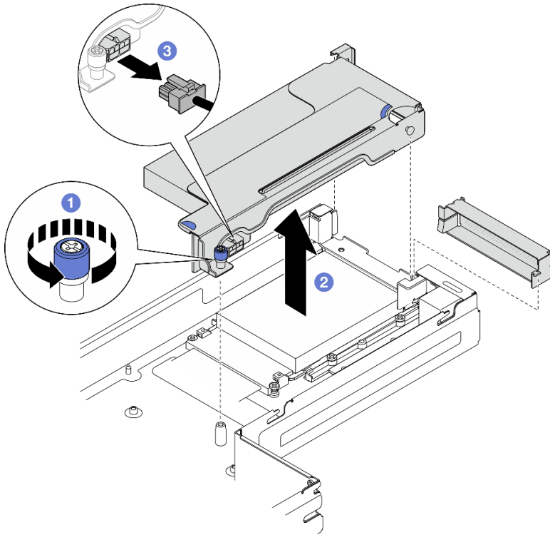
图 78. 卸下 PCIe 转接卡组合件
