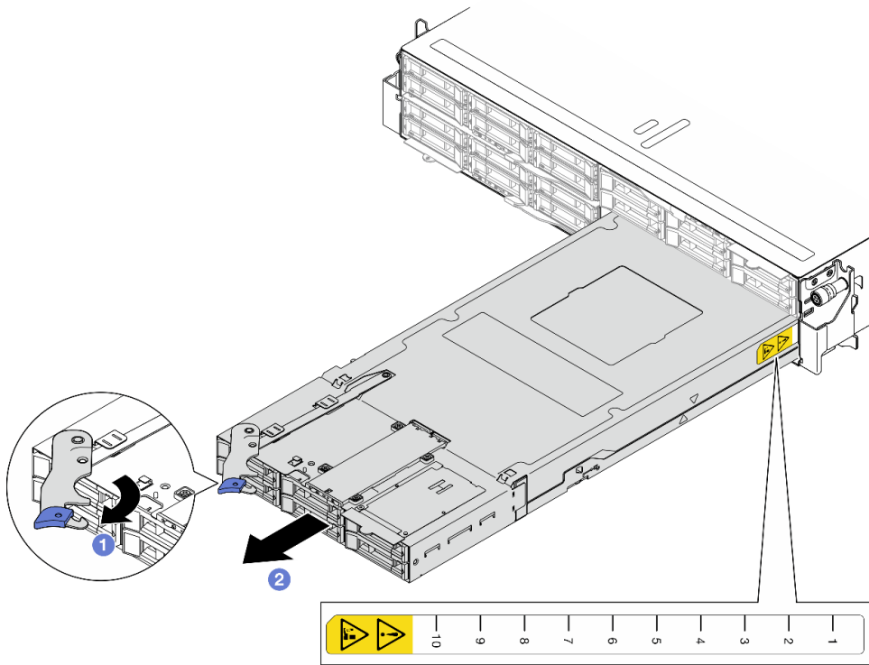
图 17. 将节点从右侧托盘卸下
