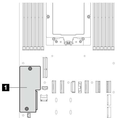
图 102. 固件和 RoT 安全模块位置
