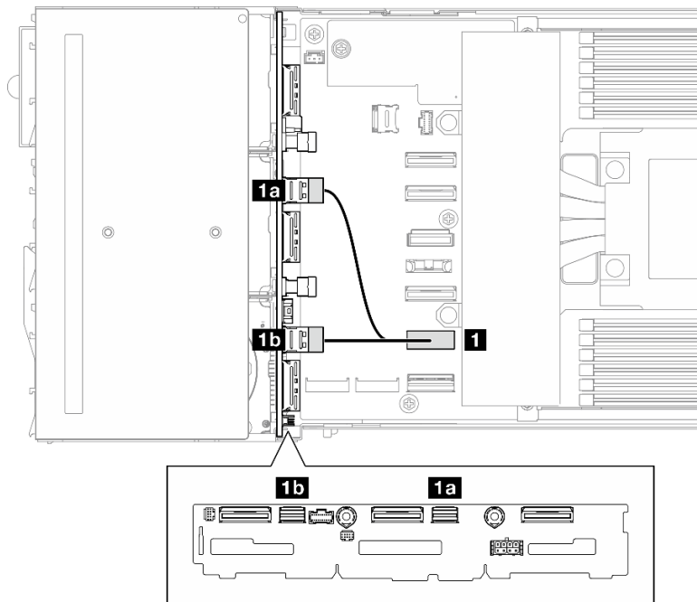
图 122. 板载 SATA 线缆布放
