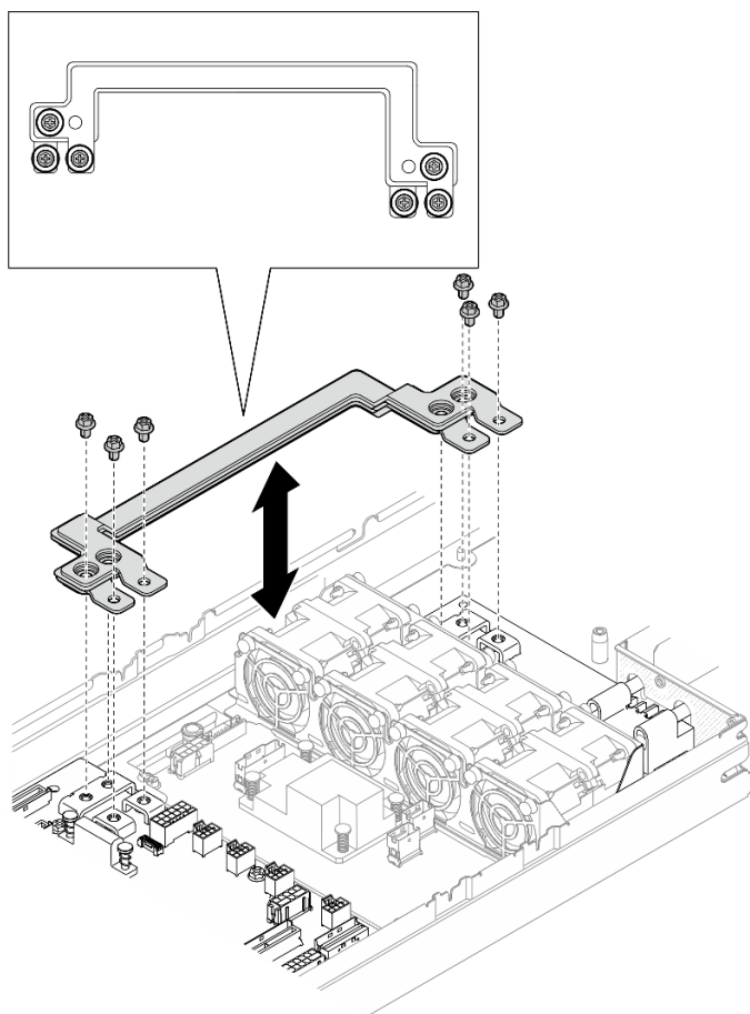
图 88. 安装电源汇流条外侧螺钉
