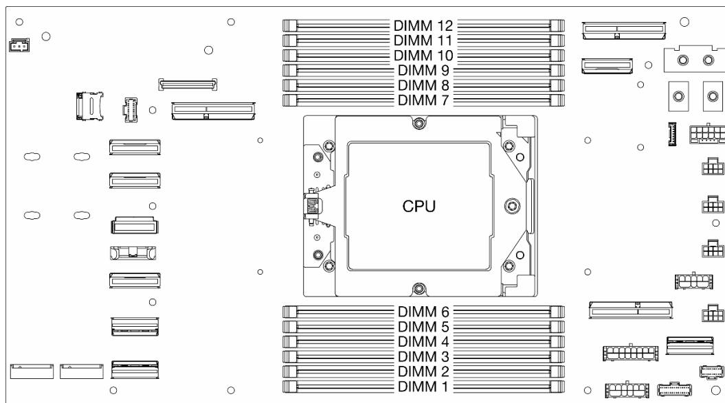
图 1. 内存条和处理器布局
