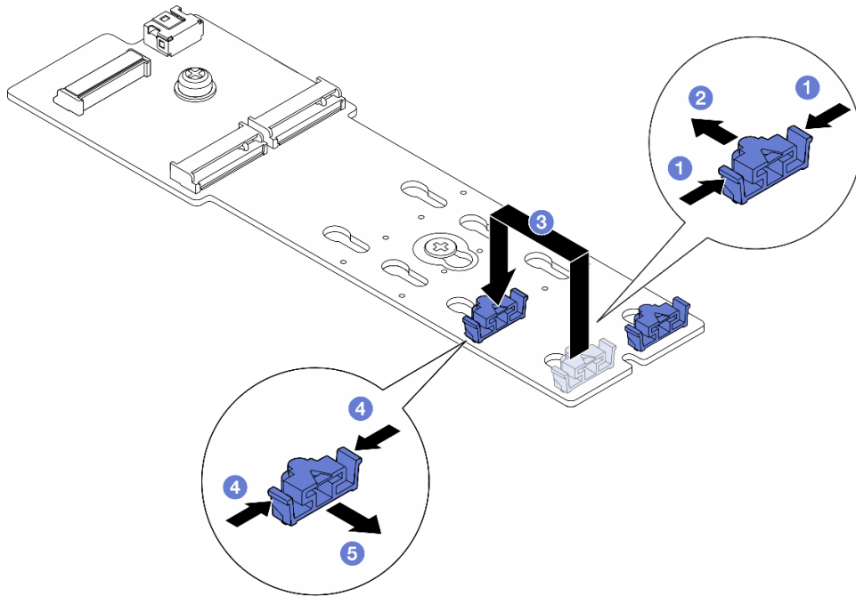
图 61. 调整 M.2 固定器
