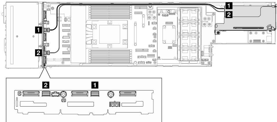
图 126. 8i RAID PCIe 适配器 SATA/SAS 线缆布放
