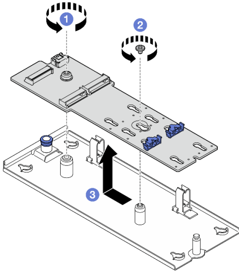
图 55. 卸下 M.2 引导适配器
