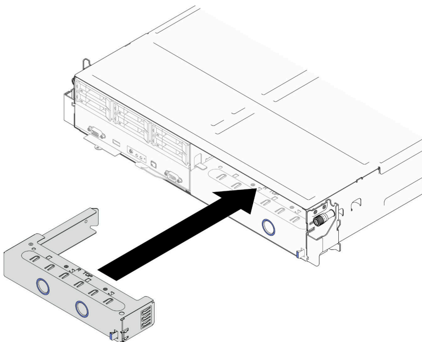
图 18. 安装正面节点托盘填充件
