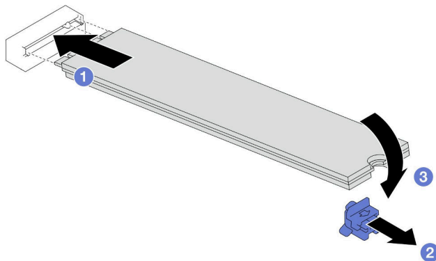
图 65. 安装 M.2 硬盘
