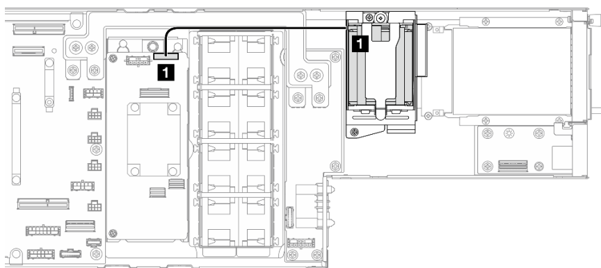
图 39. CFF RAID 和快速充电模块线缆
