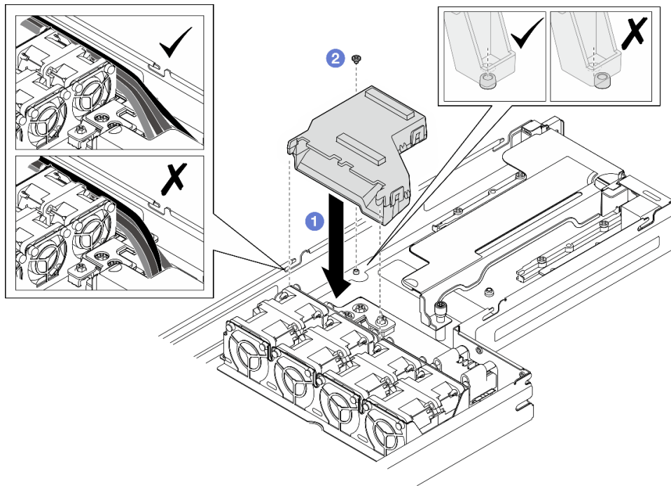
图 43. 安装 GPU 导风管
