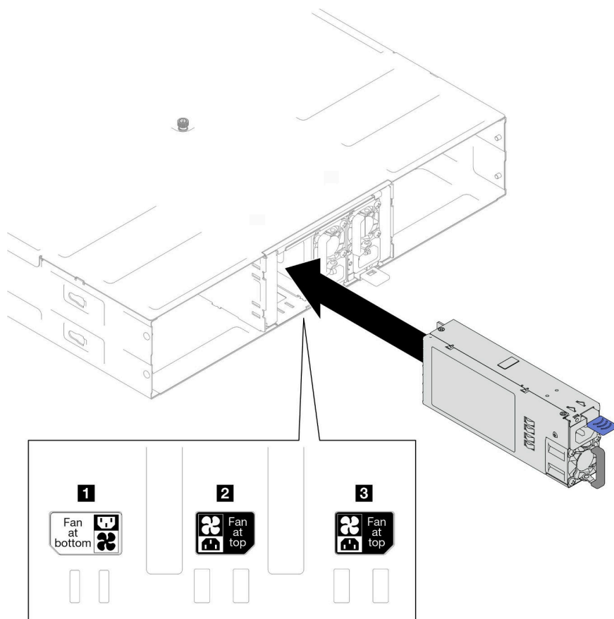
图 11. 安装热插拔电源模块
