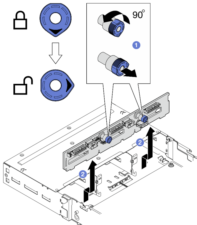
图 30. 卸下硬盘背板
