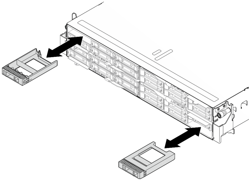
图 45. 更换硬盘填充件
