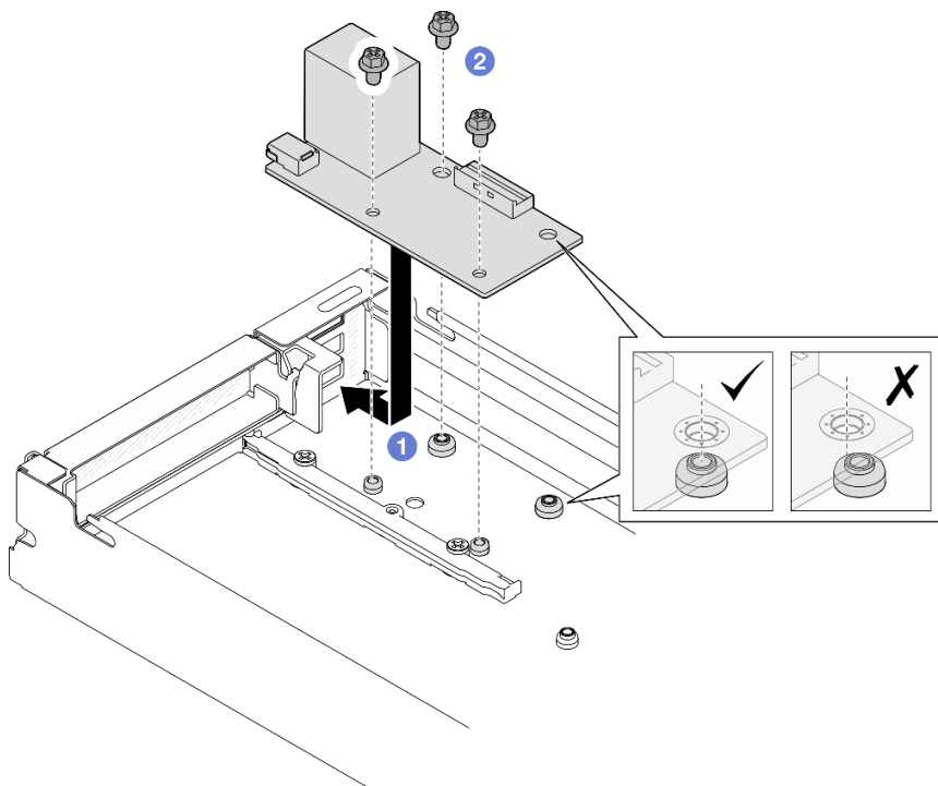
图 100. 安装背面 I/O 模块
