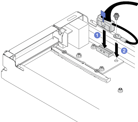
图 133. 安装背面 I/O 线缆和接地线缆
