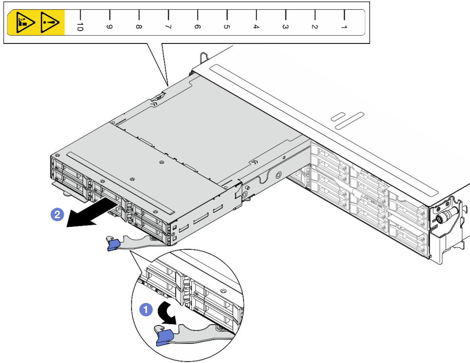
图 16. 将节点从左侧托盘卸下
