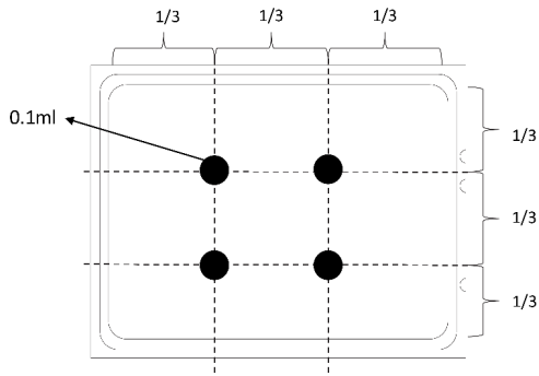
图 96. 涂抹导热油脂
