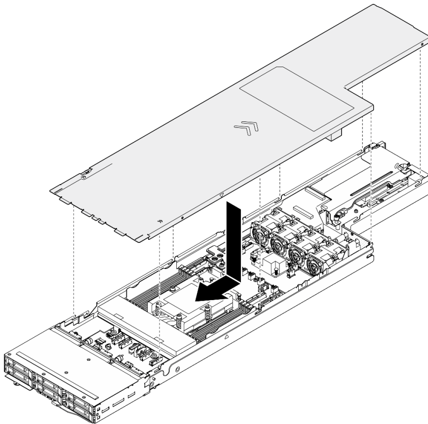
图 113. 安装顶盖
