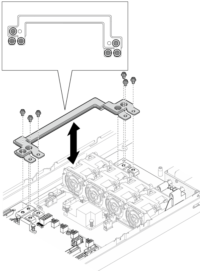
图 85. 卸下电源汇流条外侧螺钉
