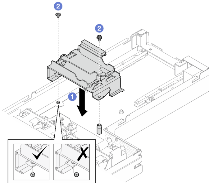
图 36. 安装快速充电模块夹持器
