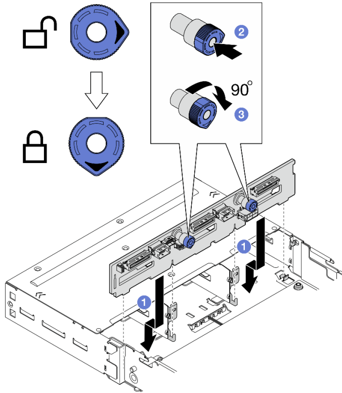
图 31. 安装硬盘背板
