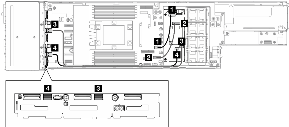
图 123. CFF RAID 线缆布放
