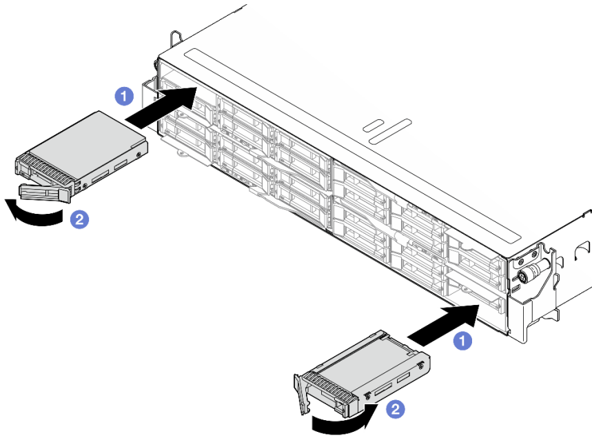
图 47. 安装固态硬盘
