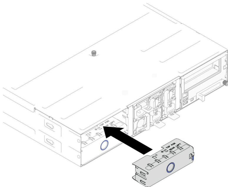
图 19. 安装背面节点托盘填充件
