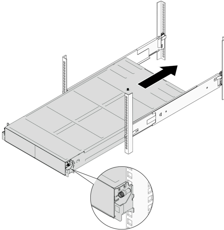
图 4. 安装机箱
