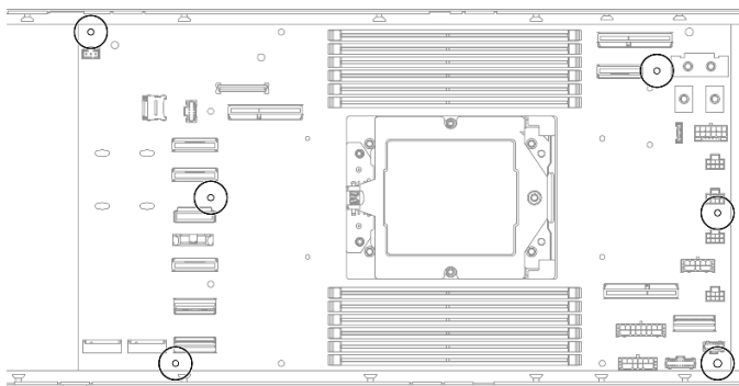
图 107. 卸下螺钉
