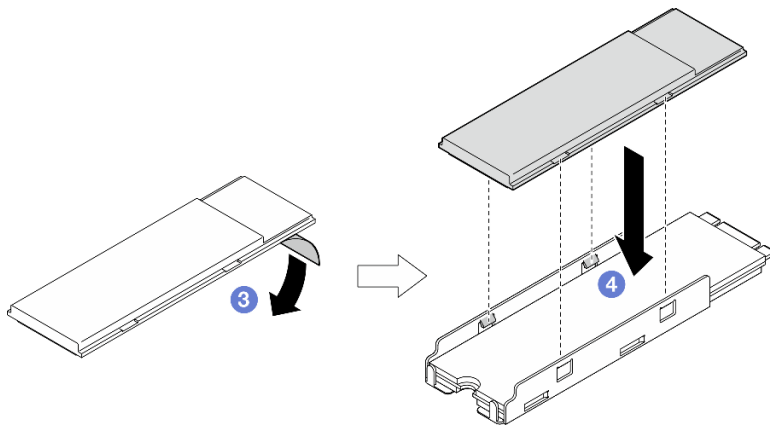
图 64. 将 M.2 散热器安装到 M.2 托盘中
