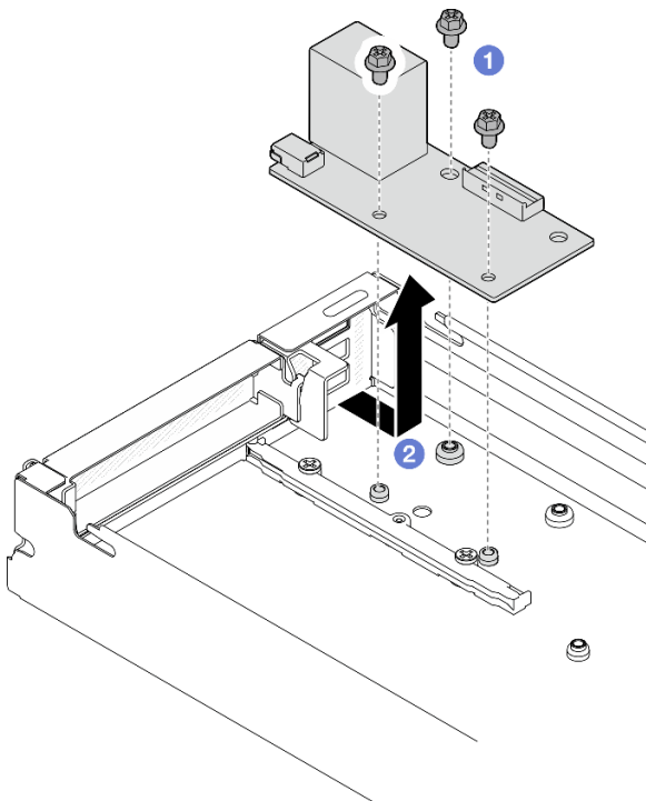
图 99. 卸下背面 I/O 模块
