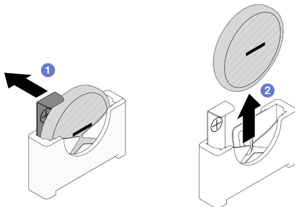
图 27. 卸下 CMOS 电池
