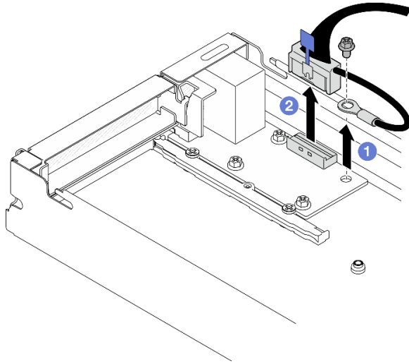
图 98. 卸下背面 I/O 线缆和接地线缆
