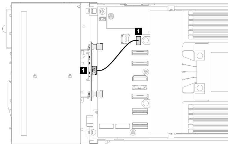
图 128. 正面 I/O 板线缆布放
