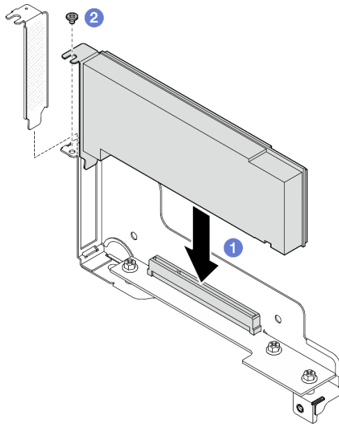
图 82. 安装 PCIe 适配器
