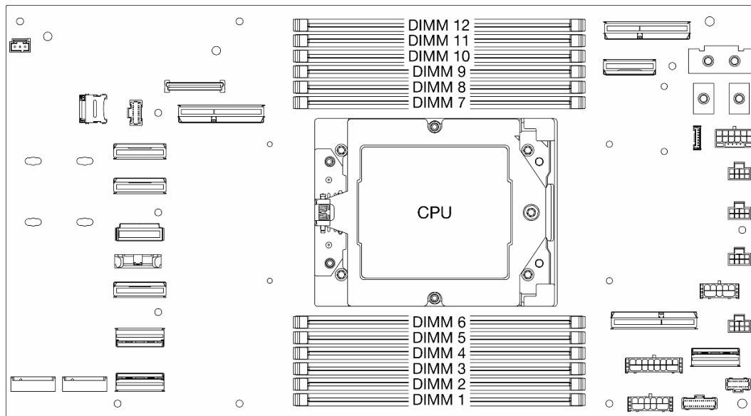
图 70. 内存条和处理器布局
