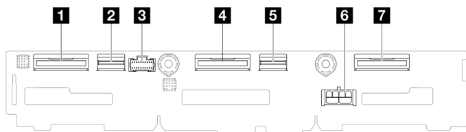
图 115. 2.5 英寸硬盘背板
