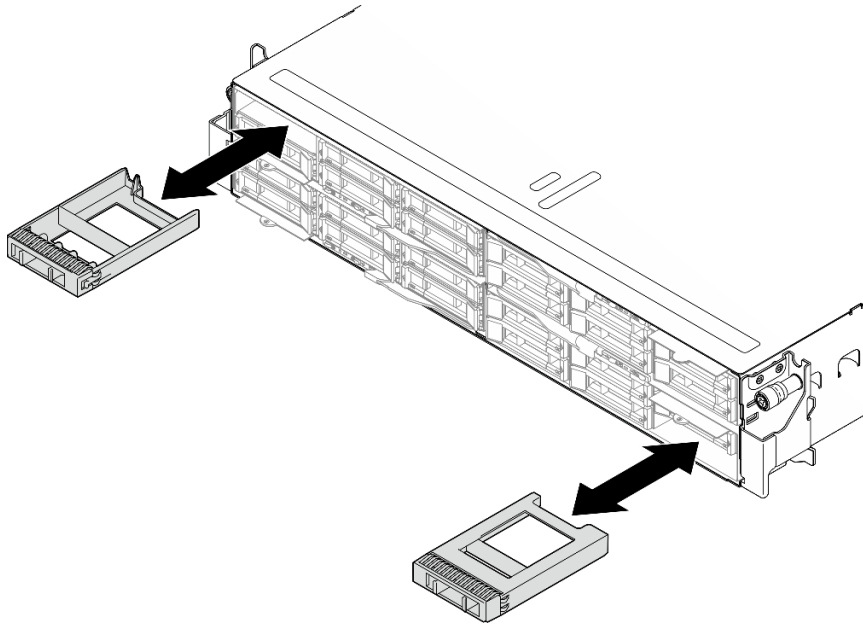
图 46. 更换硬盘填充件
