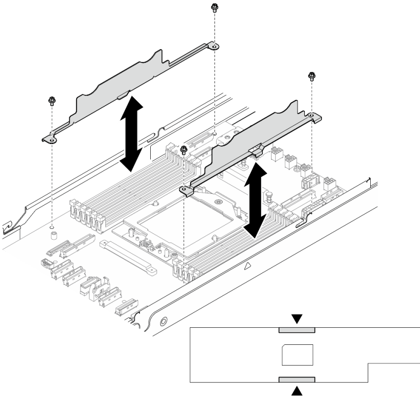
图 111. 更换线缆壁挂支架
