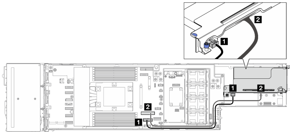
图 130. PCIe 转接卡线缆布放
