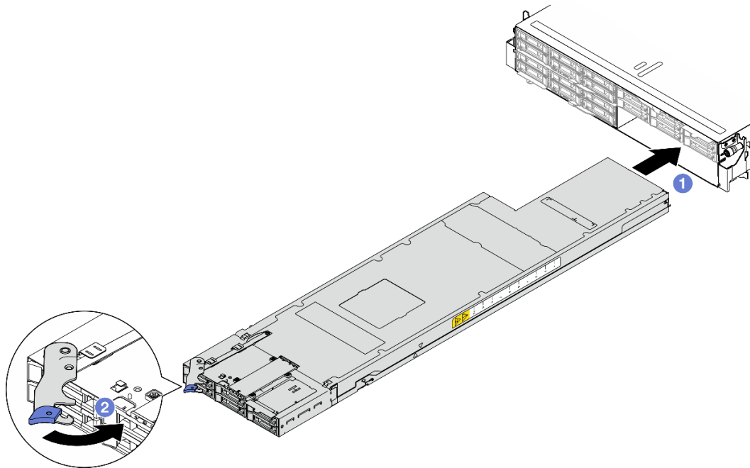
图 23. 将节点安装到右侧托盘
