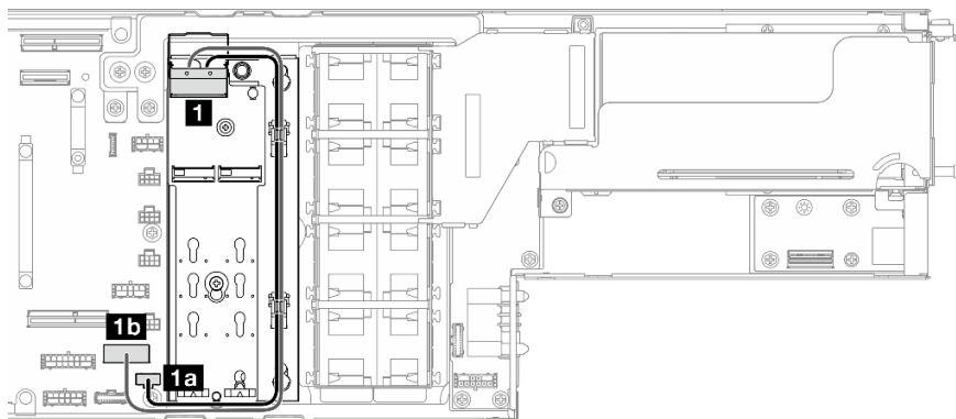
图 129. SATA/NVMe M.2 引导适配器线缆布放
