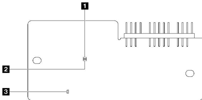
图 140. 固件和 RoT 安全模块上的 LED
