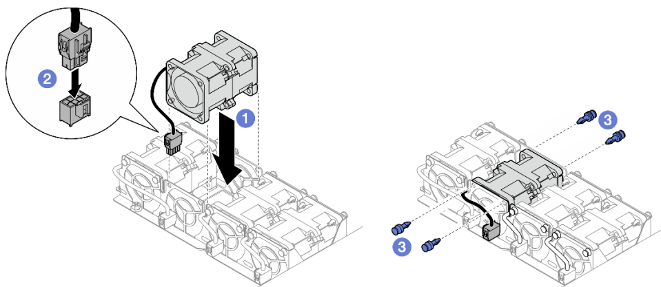
图 33. 安装风扇
