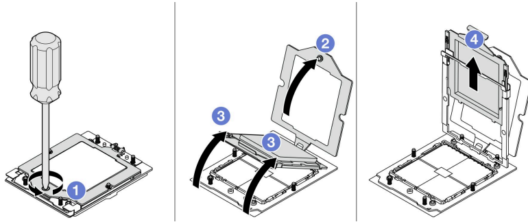
图 93. 卸下处理器
