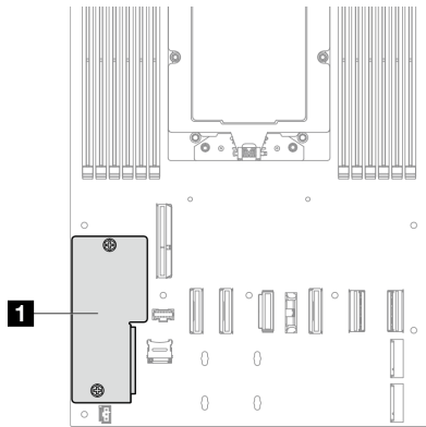
图 104. 固件和 RoT 安全模块位置
