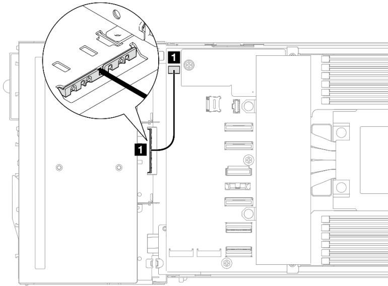
图 134. 正面热传感器线缆布放
