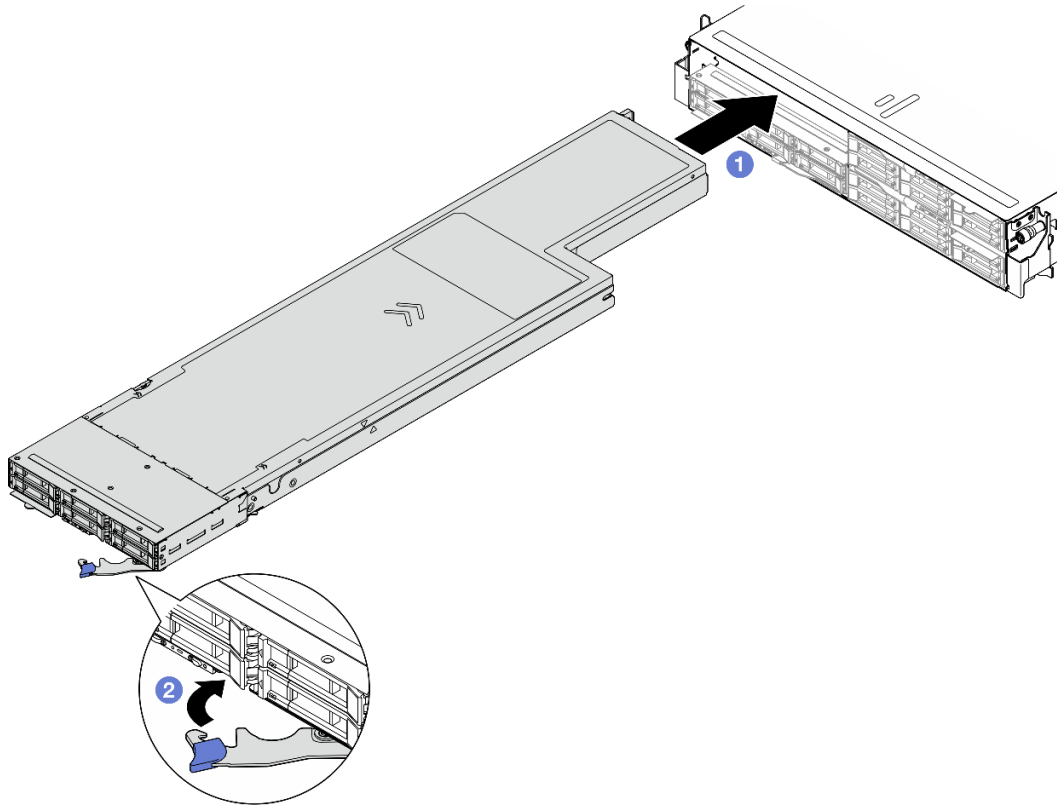
图 22. 将节点安装到左侧托盘
