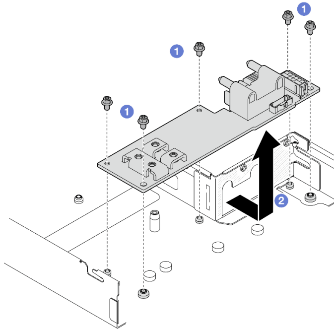
图 89. 卸下配电板
