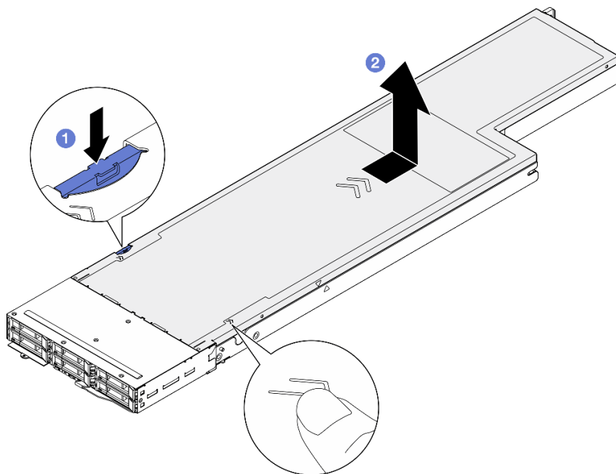
图 112. 卸下顶盖
