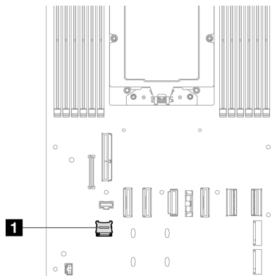
图 74. MicroSD 插槽位置
