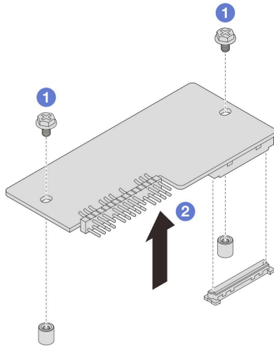
图 103. 卸下固件和 RoT 安全模块
