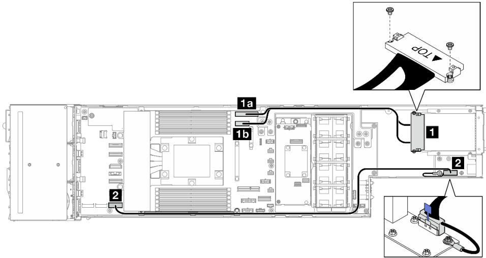
图 132. 背面 I/O 模块和 OCP 模块的线缆
