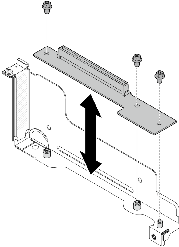
图 79. 更换 PCIe 转接卡
