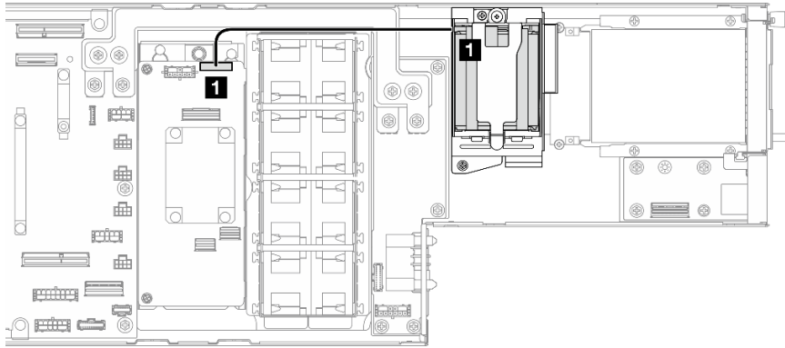
图 125. 快速充电模块线缆布放
