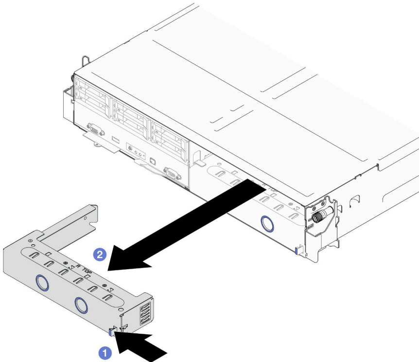
图 20. 卸下正面节点托盘填充件
