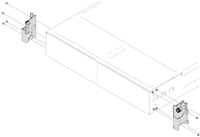
图 6. 卸下 EIA 支架
