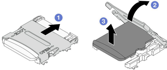
图 73. 卸下 MicroSD 卡
