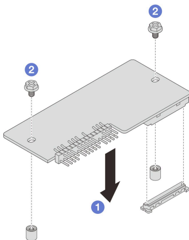
图 105. 安装固件和 RoT 安全模块
