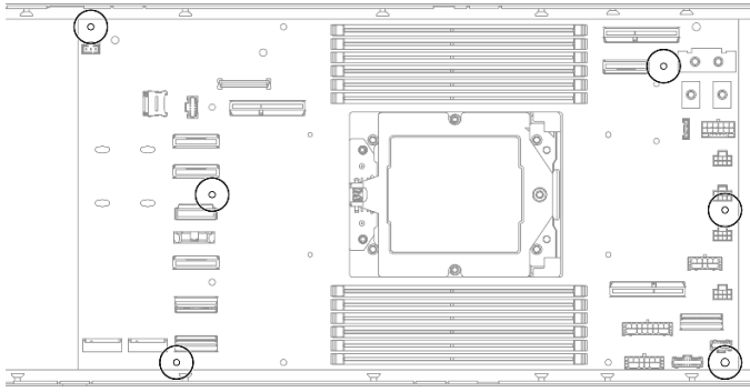
图 110. 安装螺钉
