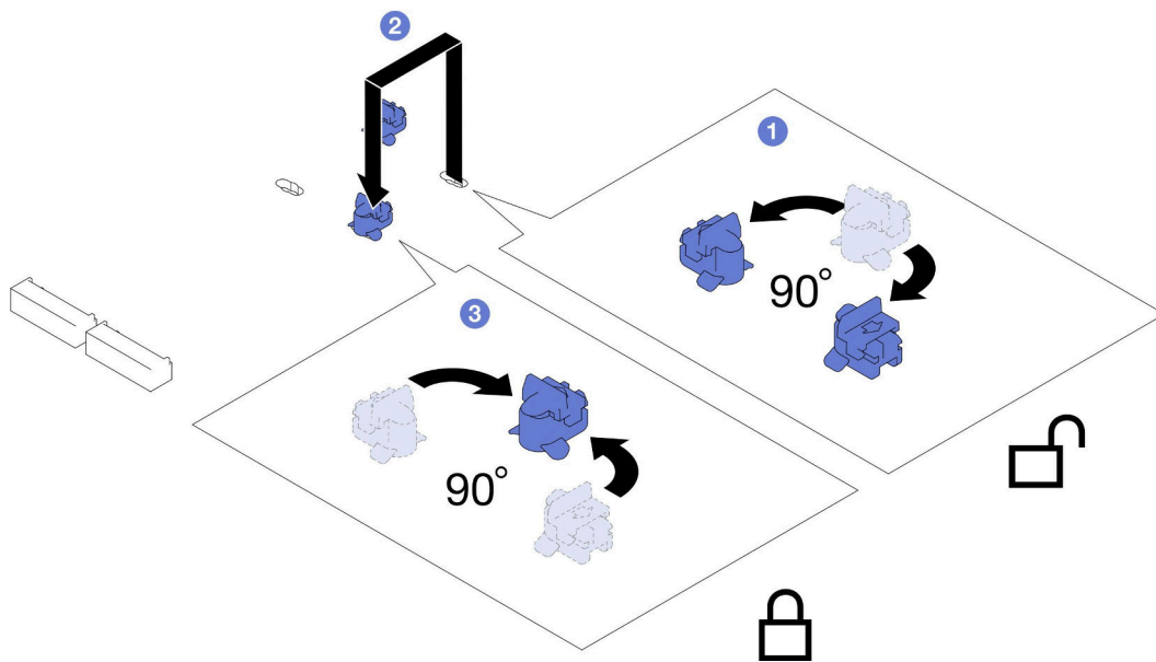
图 60. 调整 M.2 硬盘固定器
