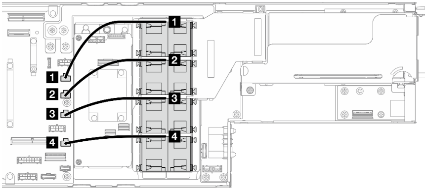
图 127. 风扇线缆布放
