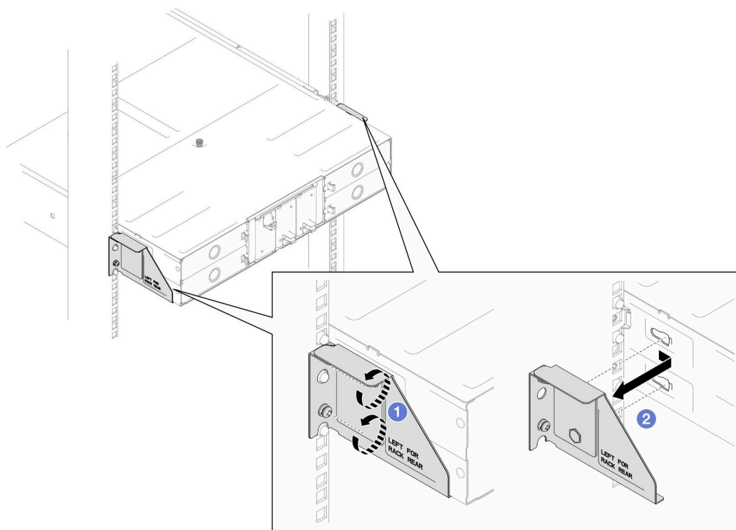
图 2. 卸下装运支架
