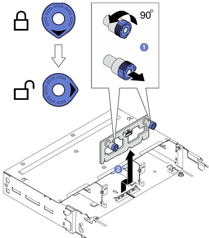
图 40. 卸下正面 I/O 背板
