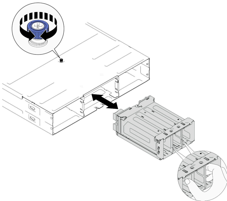
图 15. 安装 PSU 仓
