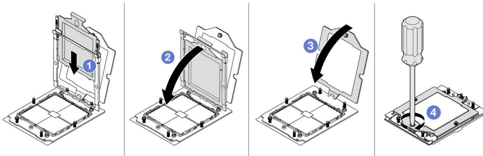
图 95. 安装处理器
