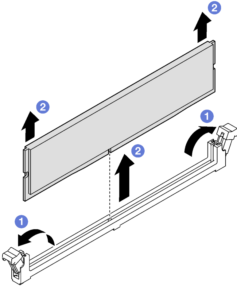
图 69. 卸下内存条
