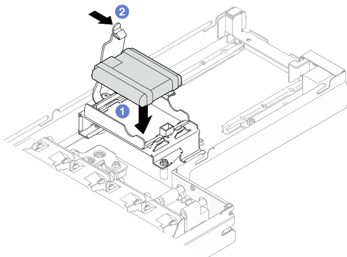
图 37. 安装快速充电模块
