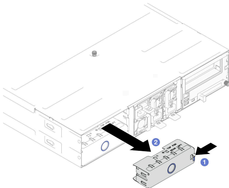
图 21. 卸下背面节点托盘填充件
