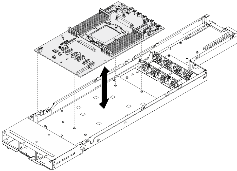
图 108. 卸下主板
