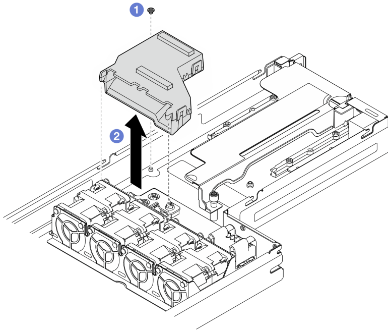
图 42. 卸下 GPU 导风管
