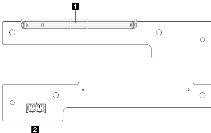
图 118. PCIe 转接卡接口
