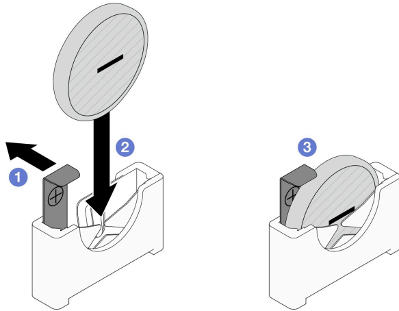
图 29. 安装 CMOS 电池
