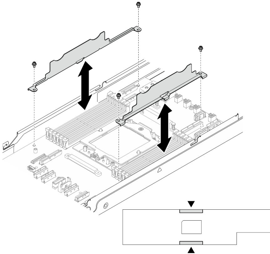
图 106. 更换线缆壁挂支架
