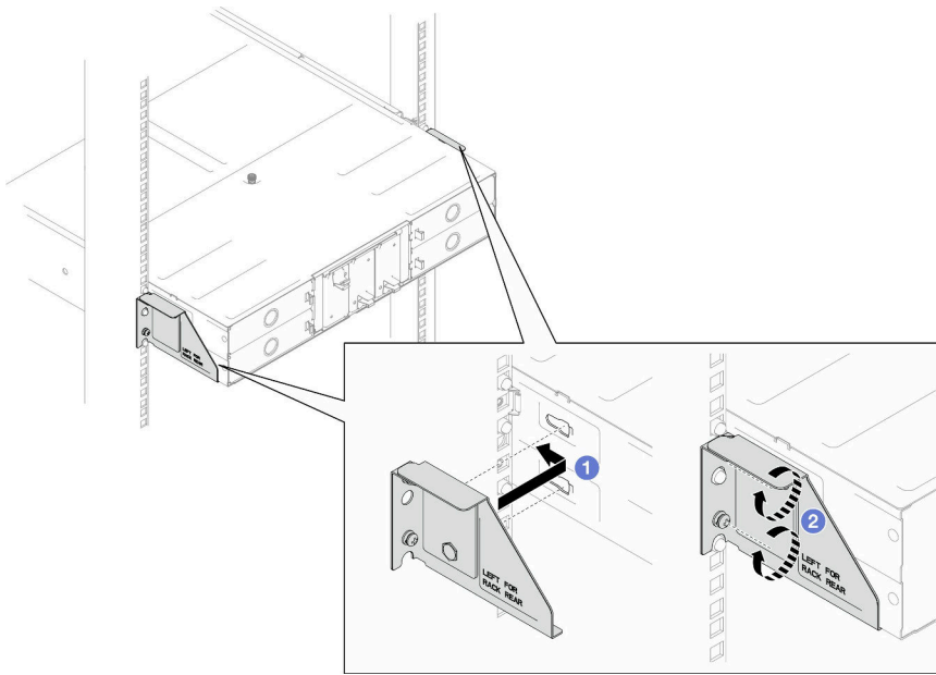
图 5. 安装装运支架
