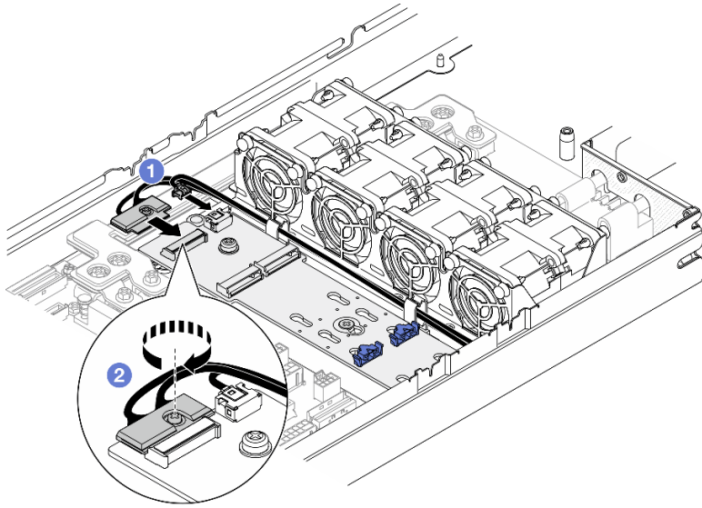
图 58. 将线缆连接到 NVMe M.2 引导适配器
