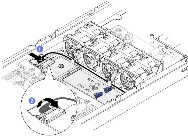
图 59. 将线缆连接到 SATA/NVMe M.2 引导适配器
