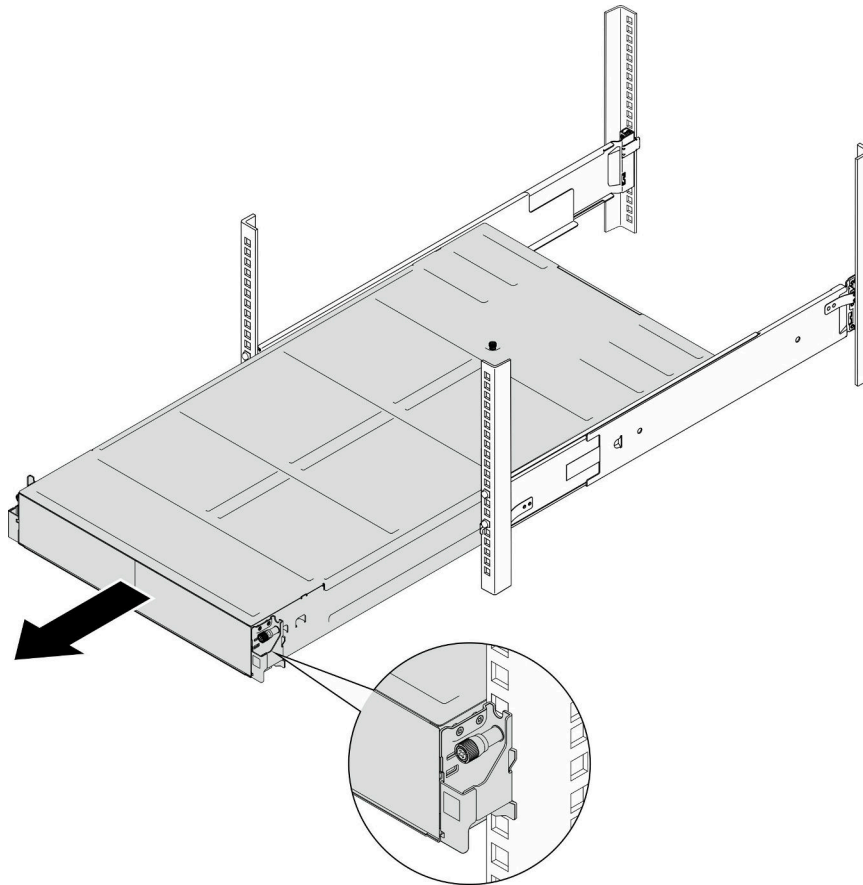
图 3. 卸下机箱
