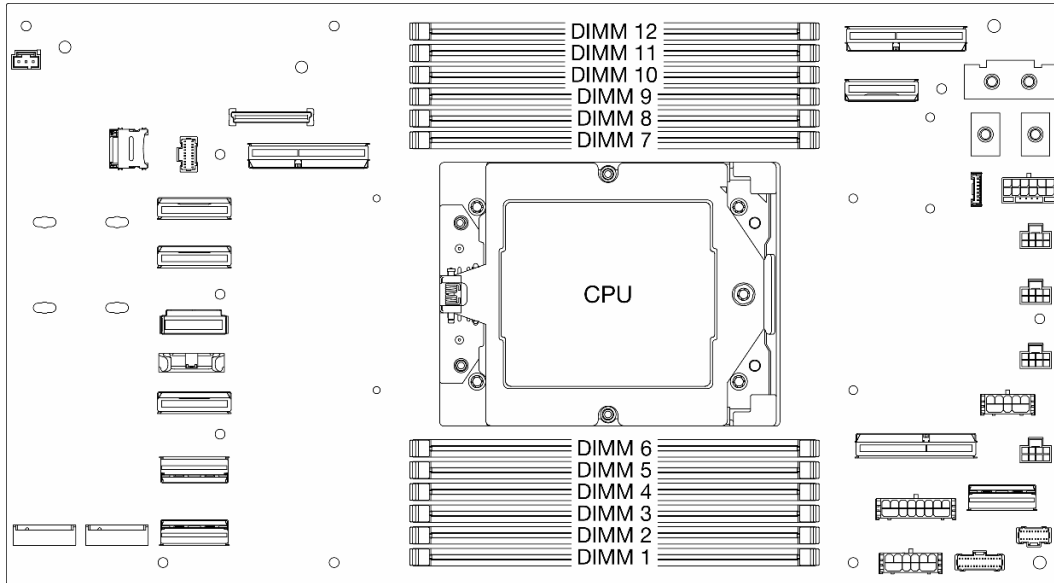
图 68. 内存条和处理器布局
