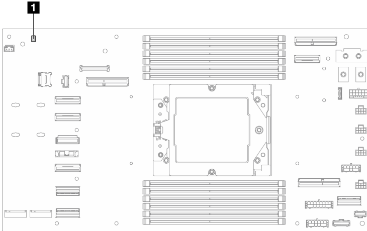
图 141. 主板 LED
