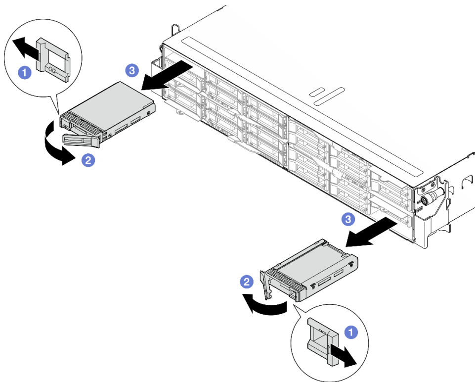
图 44. 卸下固态硬盘
