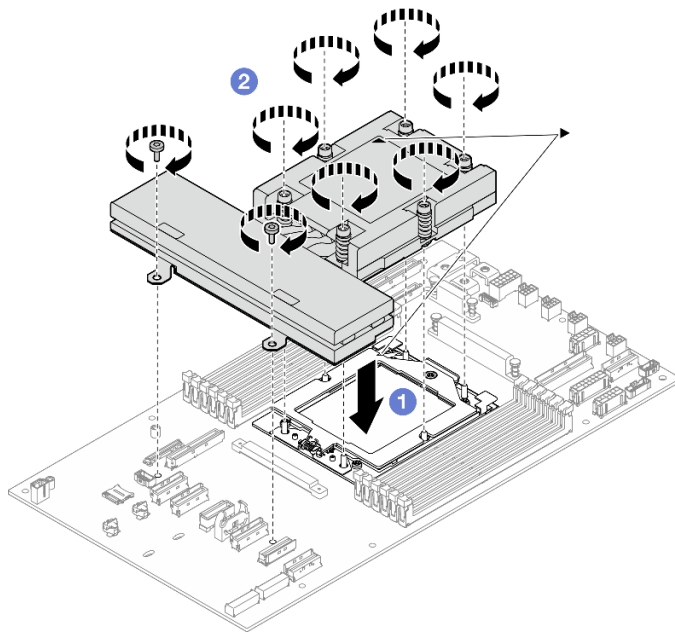
图 97. 安装散热器
