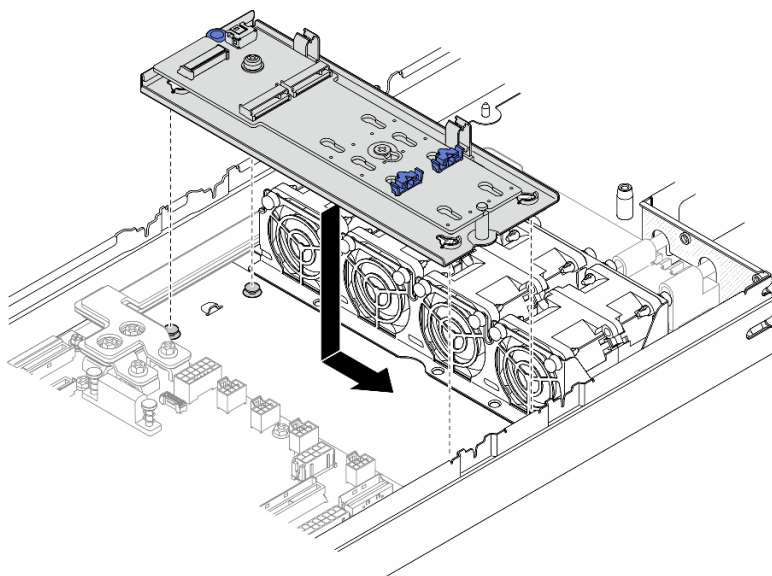
图 57. 安装 M.2 引导适配器托盘
