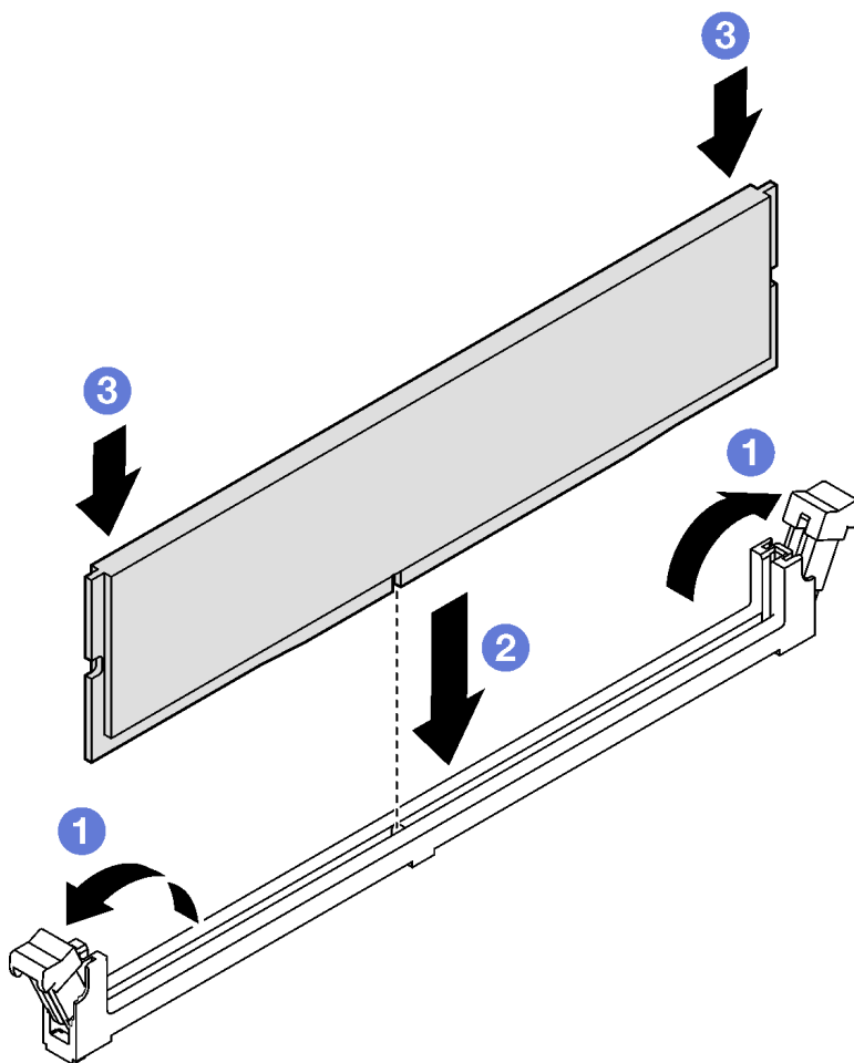
图 71. 安装内存条
