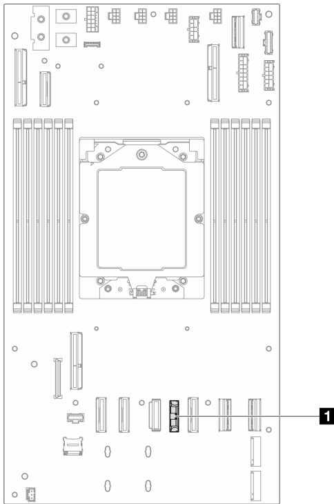
图 26. CMOS 电池插槽位置
