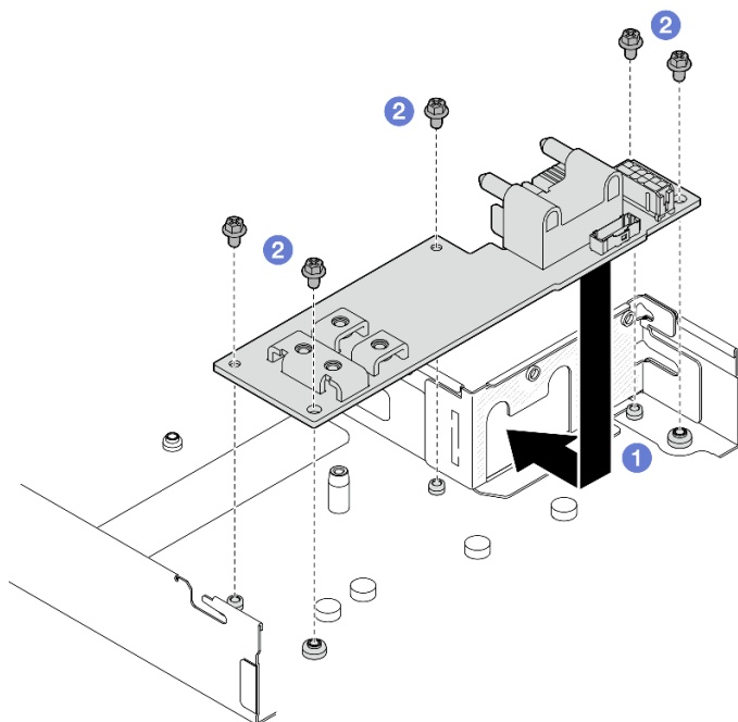
图 90. 安装配电板
