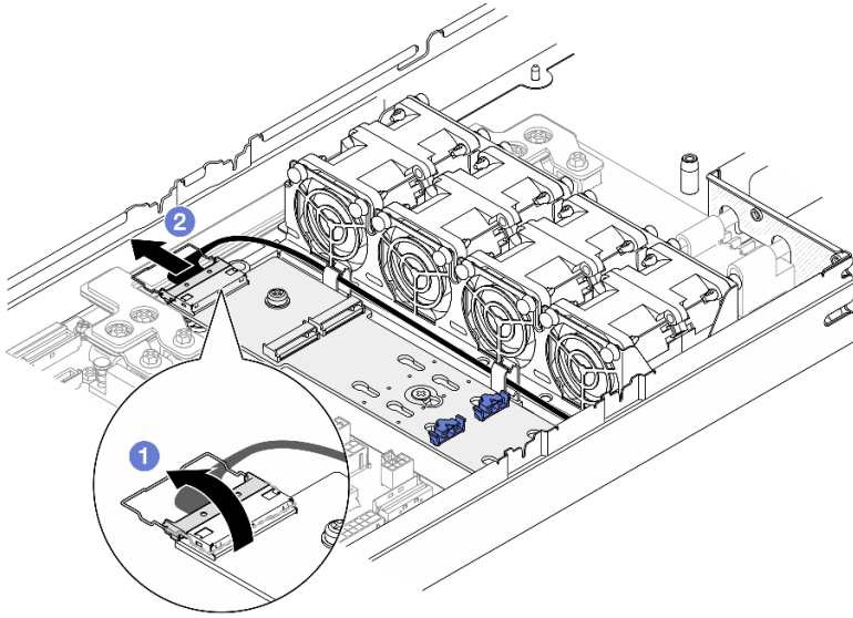
图 53. 从 SATA/NVMe M.2 引导适配器上拔下线缆
