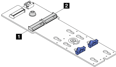
图 66. M.2 硬盘插槽
