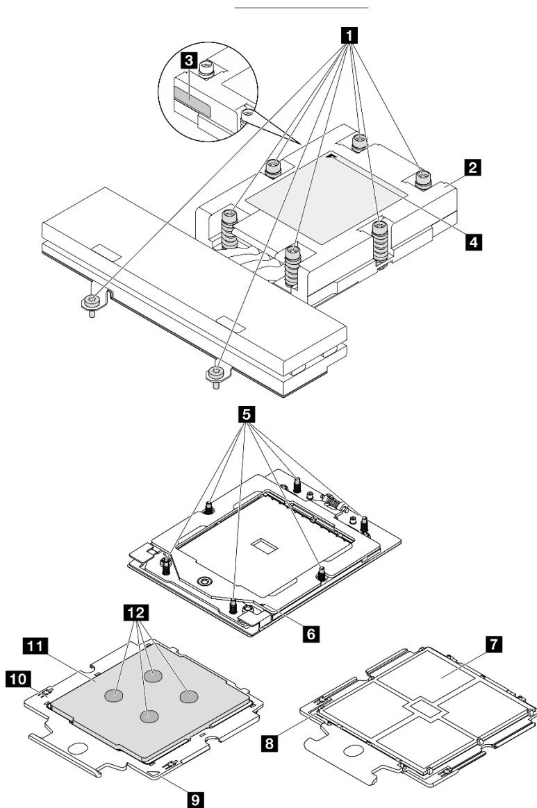
图 94. 处理器和散热器组件
