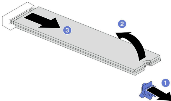
图 49. 卸下 M.2 硬盘
