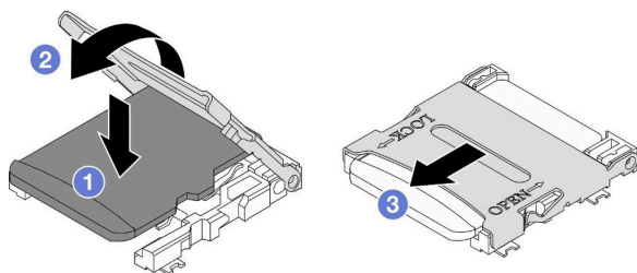
图 75. 安装 MicroSD 卡
