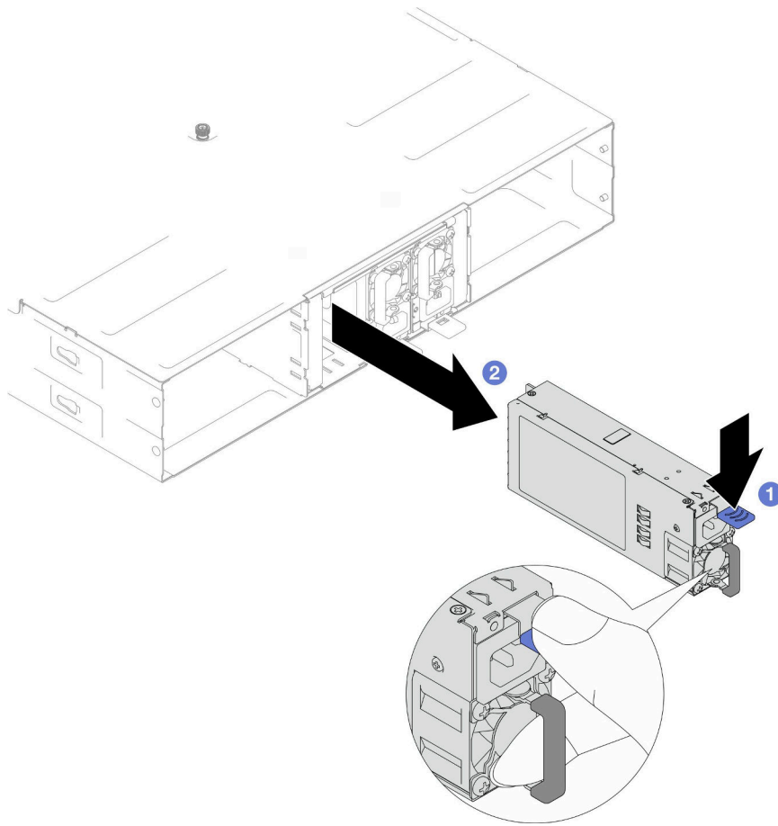
图 8. 卸下热插拔 PSU
