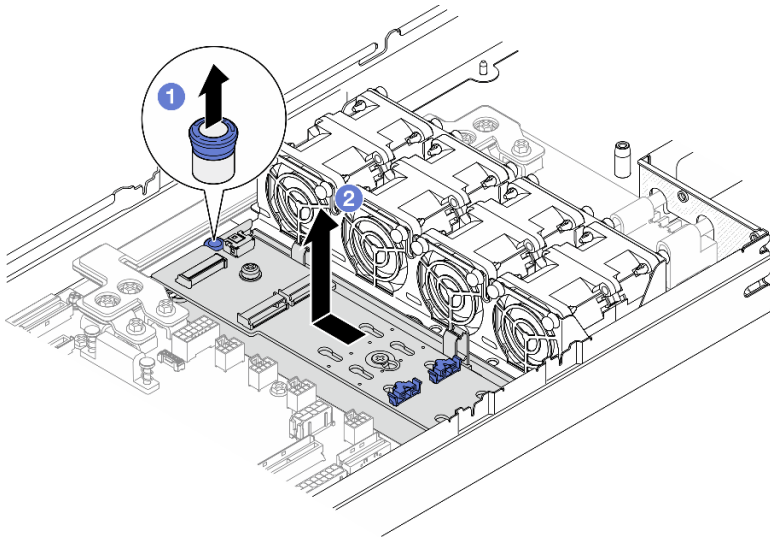
图 54. 卸下 M.2 引导适配器托盘
