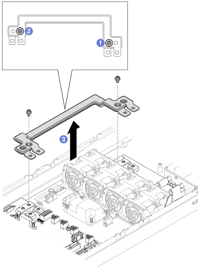
图 86. 卸下电源汇流条
