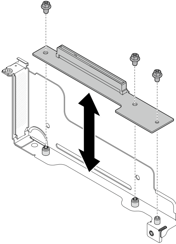
图 83. 更换 PCIe 转接卡
