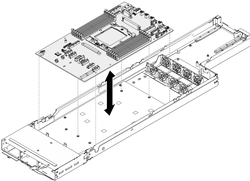
图 109. 安装主板
