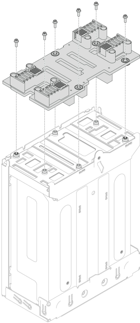
图 13. 卸下机箱中面板
