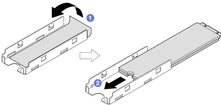
图 63. 将导热垫和 M.2 硬盘安装到托盘中
