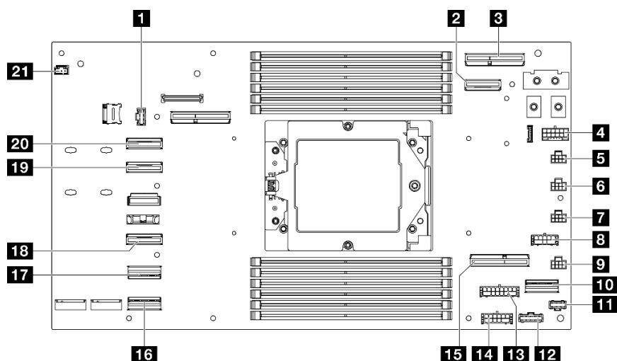
图 114. 用于线缆布放的主板接口
