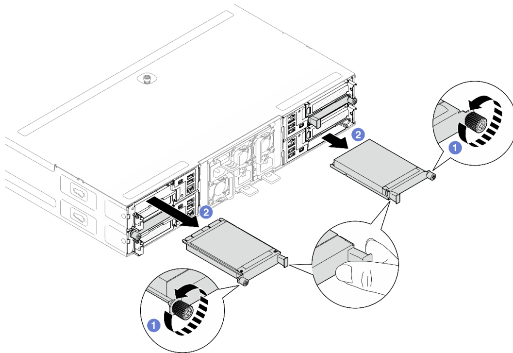
图 76. 卸下背面 OCP 模块
