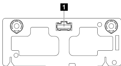
图 116. 正面 I/O 板接口
