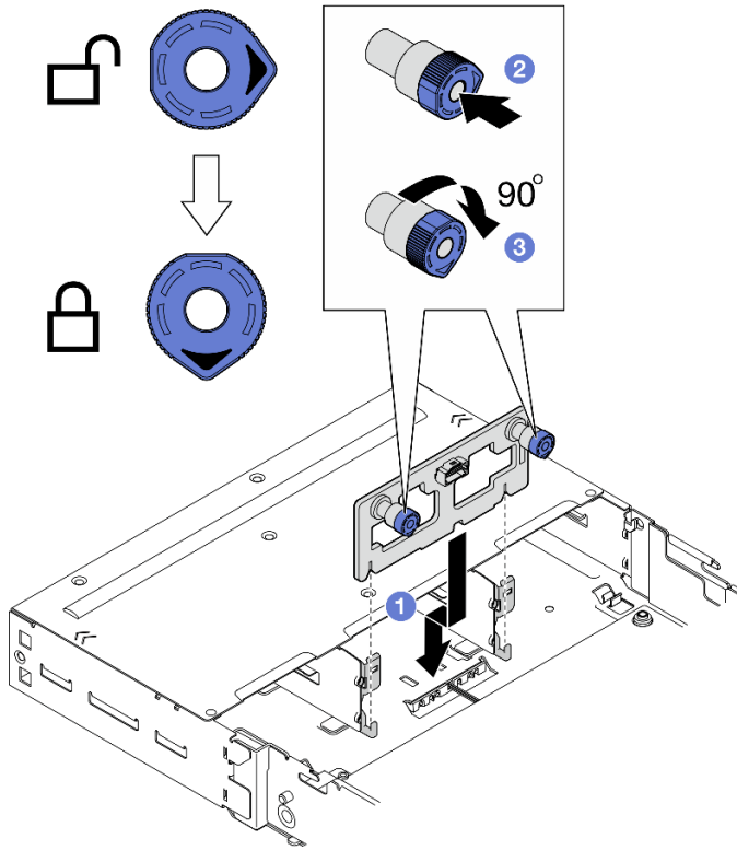
图 41. 安装正面 I/O 背板
