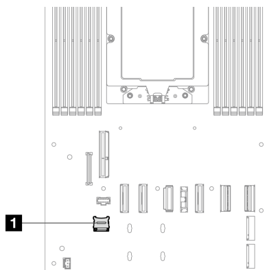
图 72. MicroSD 插槽位置
