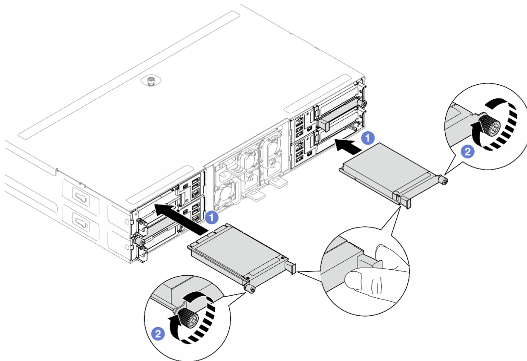
图 77. 安装背面 OCP 模块
