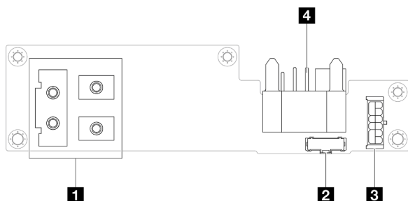
图 119. 配电板接口
