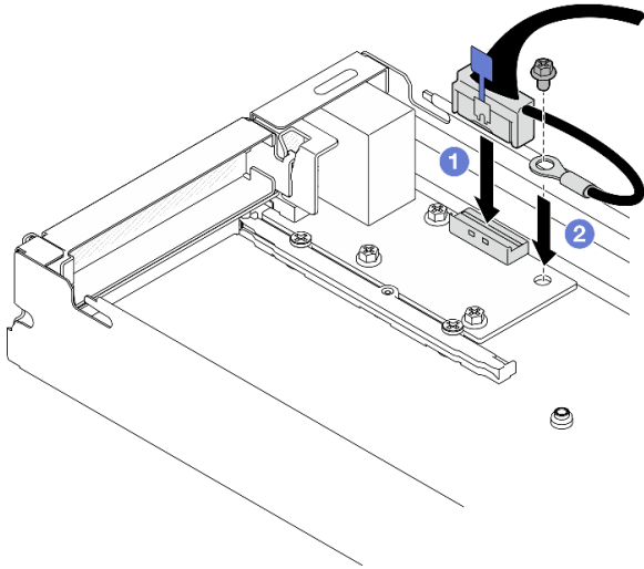
图 101. 安装背面 I/O 线缆和接地线缆
