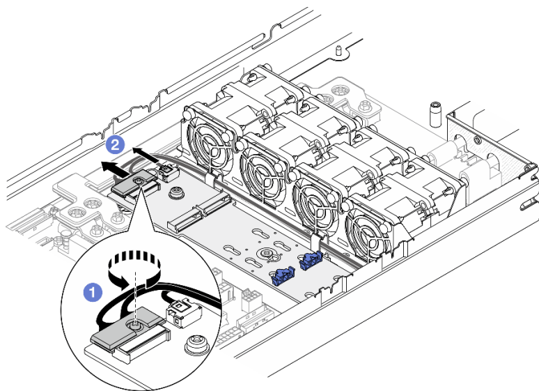
图 52. 从 NVMe M.2 引导适配器上拔下线缆
