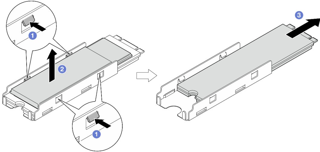
图 50. 卸下 M.2 散热器
