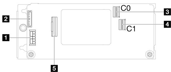
图 117. 内部 CFF RAID 适配器接口
