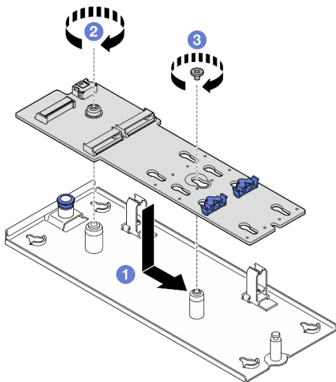
图 56. 安装 M.2 引导适配器
