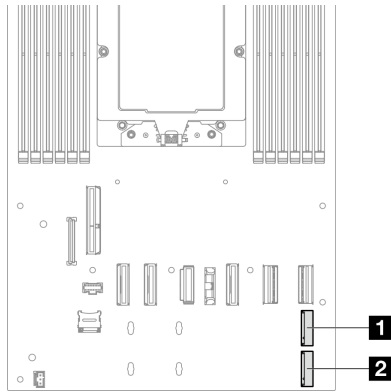
图 48. 主板上 M.2 插槽的位置
