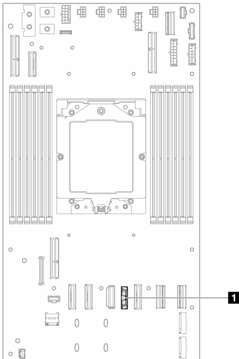
图 28. CMOS 电池插槽位置
