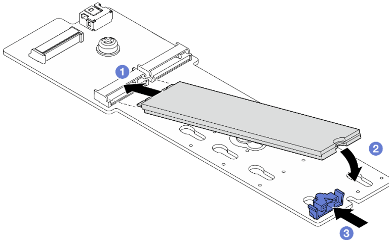
图 67. 安装 M.2 硬盘
