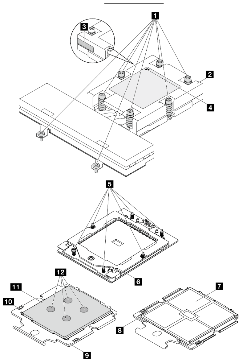
图 91. 处理器和散热器组件
