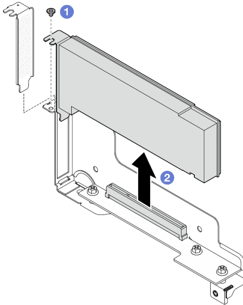
图 80. 卸下 PCIe 适配器
