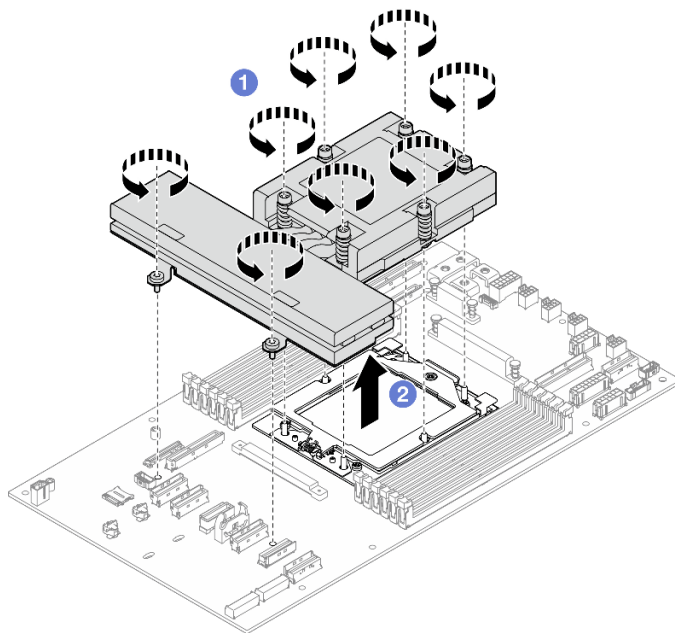
图 92. 卸下散热器
