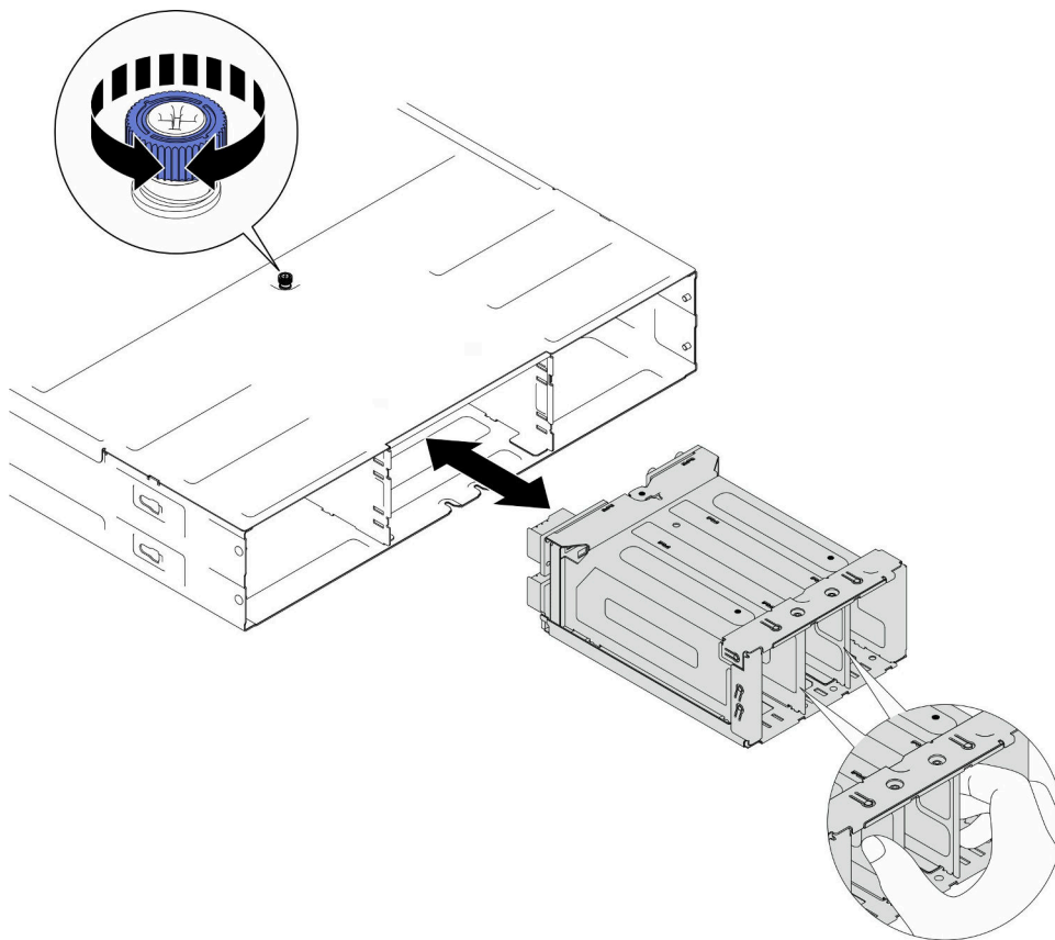
图 12. 卸下 PSU 仓
