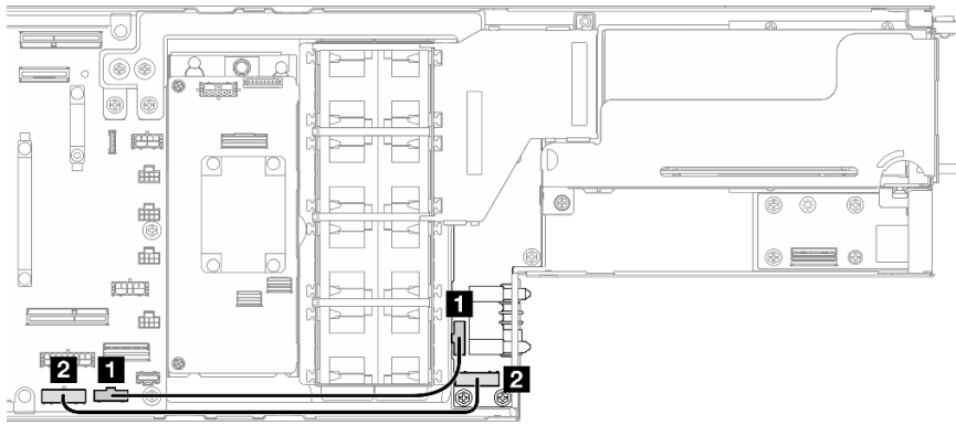
图 131. 配电板的线缆布放
