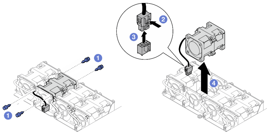
图 32. 卸下风扇
