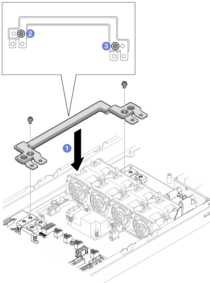
图 87. 安装电源汇流条
