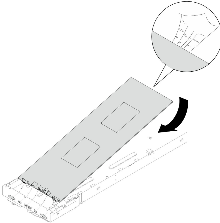
Figura 110. Instalación de la placa del sistema
