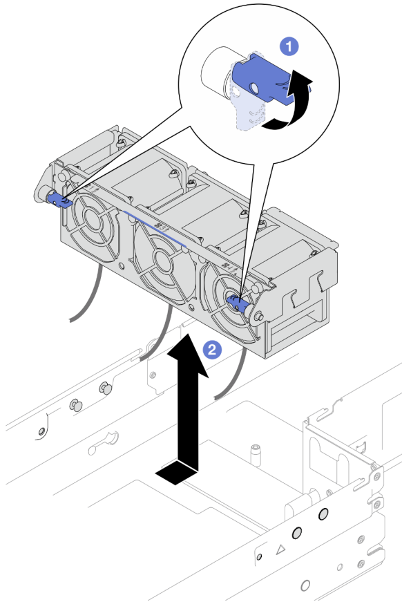
Figura 39. Extracción del compartimiento del ventilador
