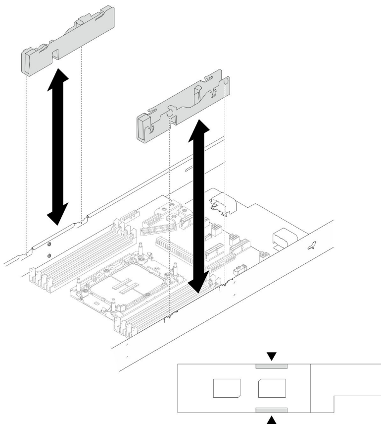
Figura 106. Sustitución del conducto de cable
