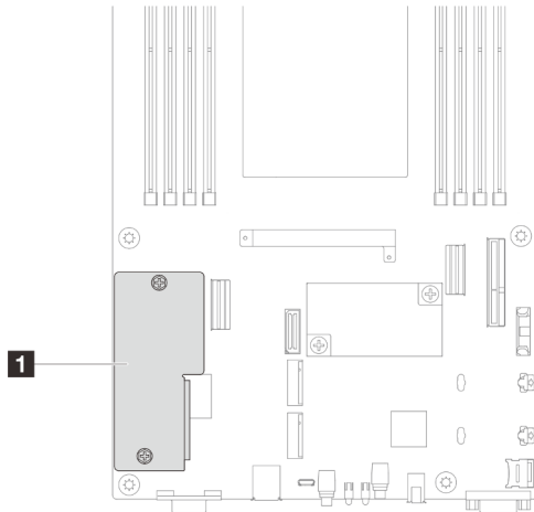
Figura 102. Ubicación del Firmware y módulo de seguridad de RoT
