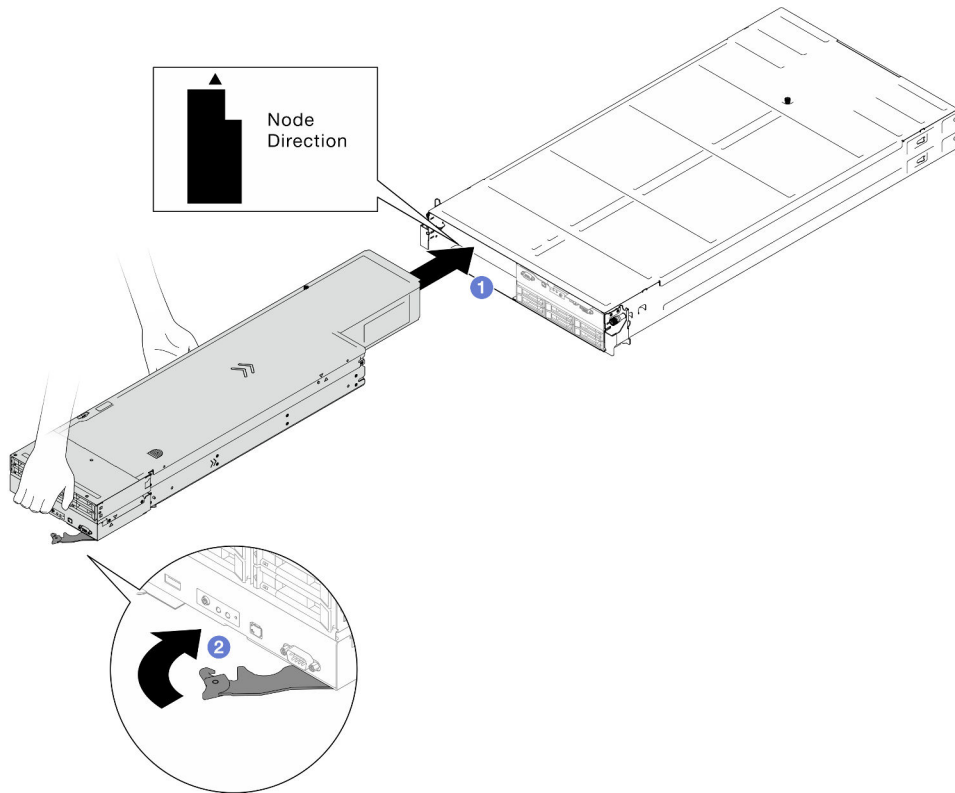
Figura 22. Instalación de un nodo en la bandeja izquierda
