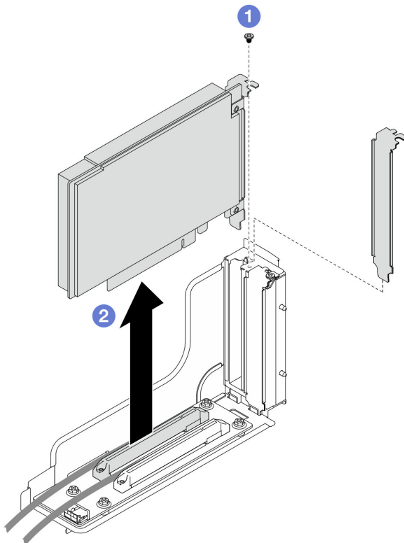
Figura 74. Extracción de un adaptador PCIe
