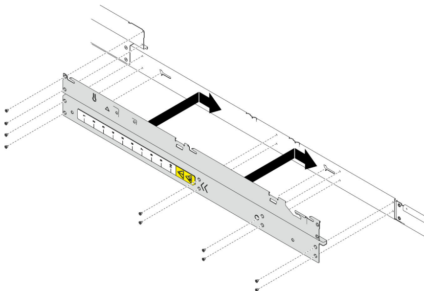
Figura 101. Instalación del soporte lateral
