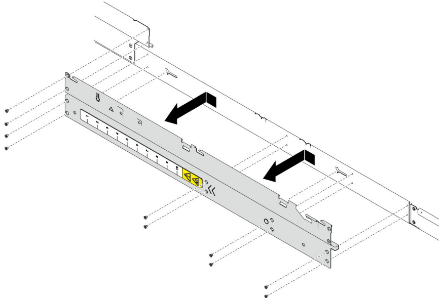
Figura 100. Extracción del soporte lateral
