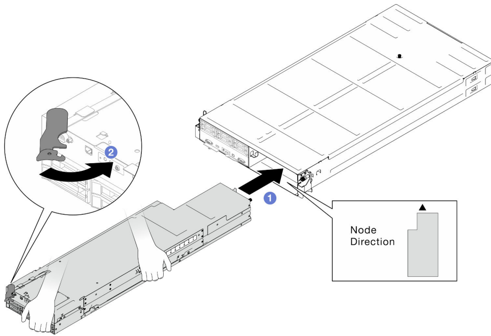
Figura 23. Instalación de un nodo en la bandeja derecha
