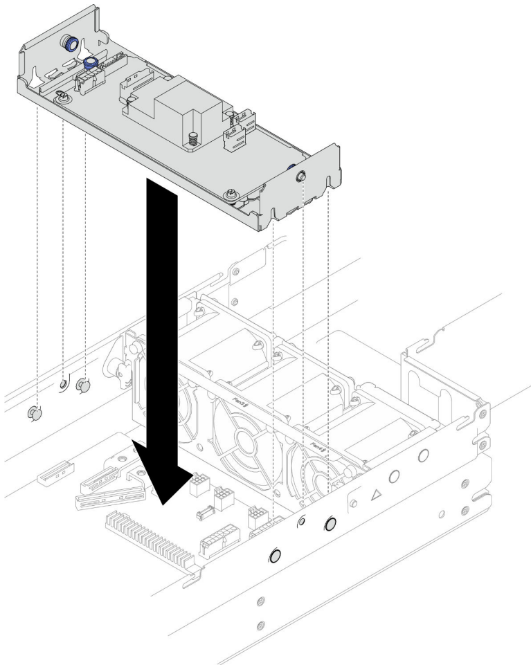
Figura 56. Instalación del soporte del adaptador interno
