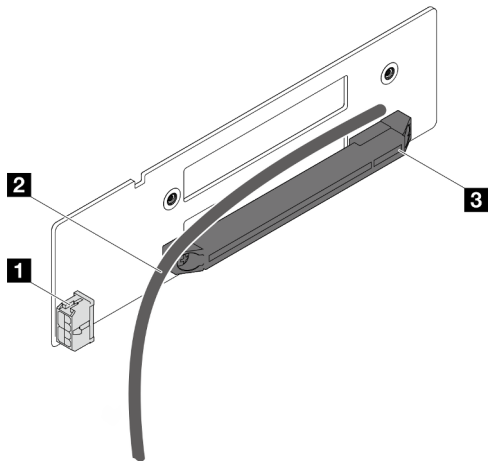
Figura 118. Conectores y cable de la tarjeta de expansión PCIe de una ranura
