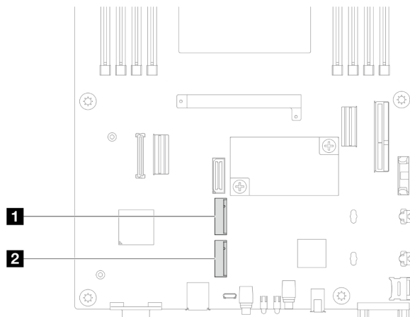
Figura 60. Ubicación de las bahías M.2 en la placa del sistema
