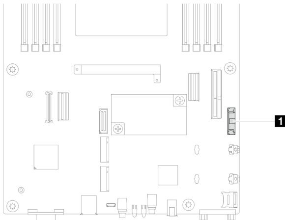
Figura 31. Ubicación del zócalo de la batería CMOS
