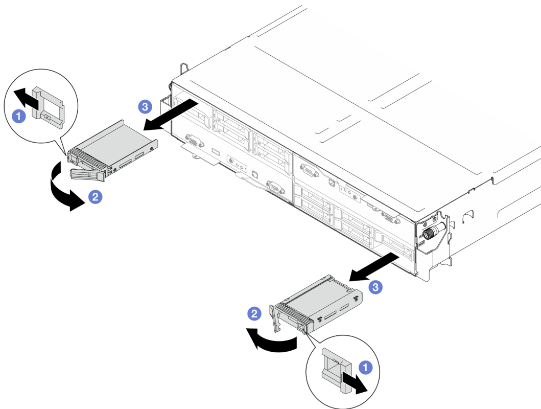
Figura 49. Extracción de una unidad de estado sólido de 7 mm
