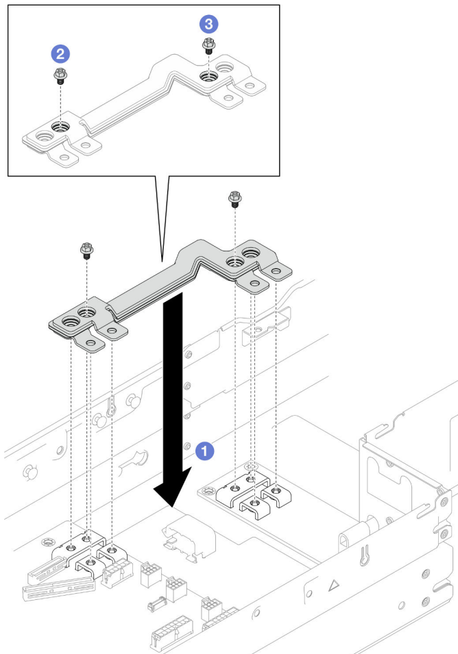
Figura 81. Instalación de la barra de bus de alimentación
