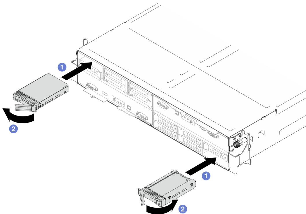
Figura 54. Instalación de una unidad de estado sólido de 15 mm
