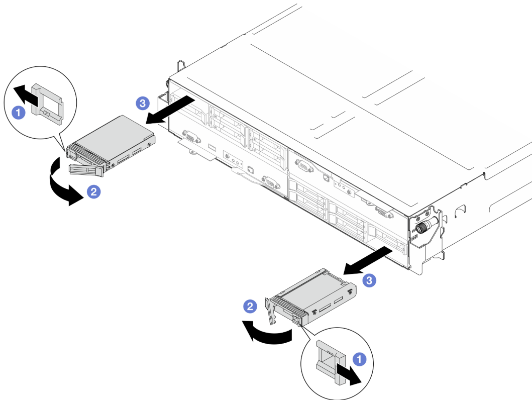
Figura 50. Extracción de una unidad de estado sólido de 15 mm
