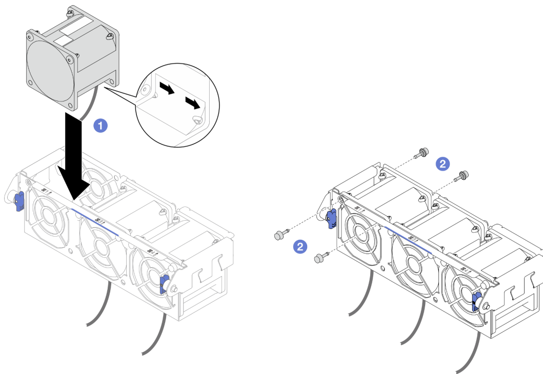
Figura 41. Instalación de ventilador
