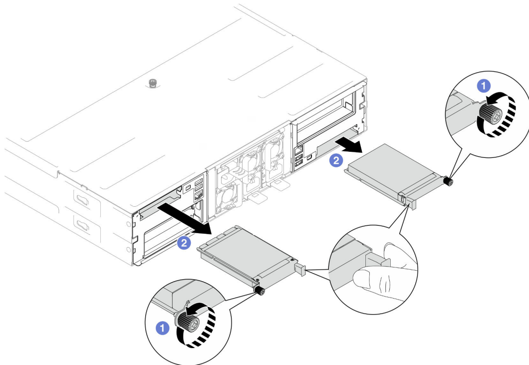
Figura 70. Extracción del módulo de OCP posterior
