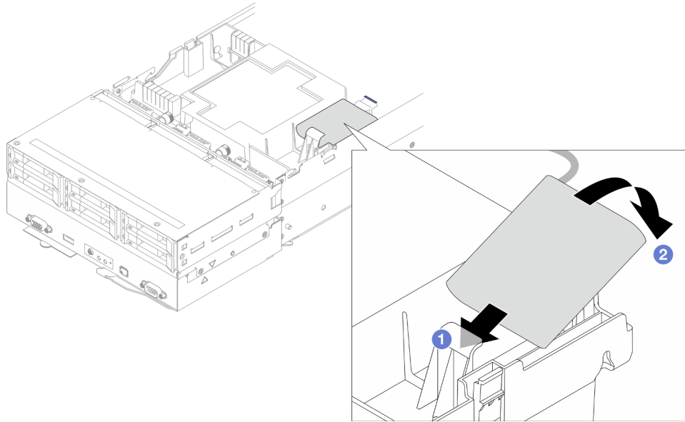
Figura 44. Instalación del módulo de alimentación flash
