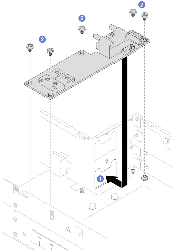
Figura 84. Instalación de una placa de distribución de alimentación
