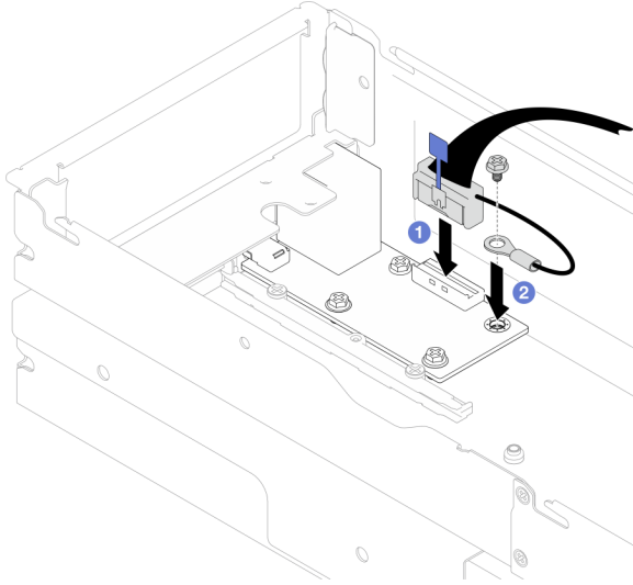
Figura 99. Instalación del cable de E/S posterior y del cable de conexión a tierra
