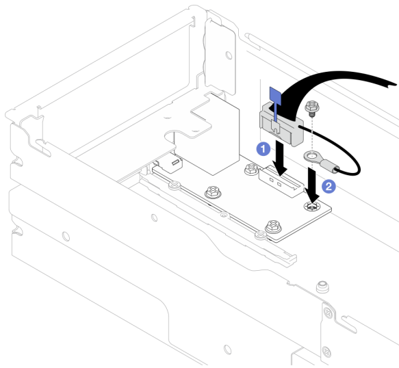
Figura 134. Instalación del cable de E/S posterior y del cable de conexión a tierra
