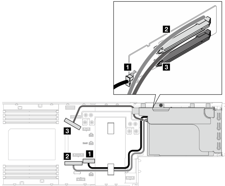
Figura 131. Disposición de cables de la expansión PCIe – dos procesadores
