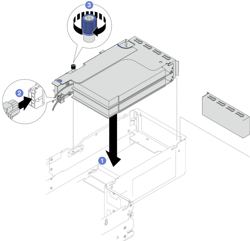
Figura 78. Instalación del conjunto de expansión PCIe
