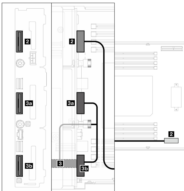
Figura 125. Disposición de los cables NVMe
