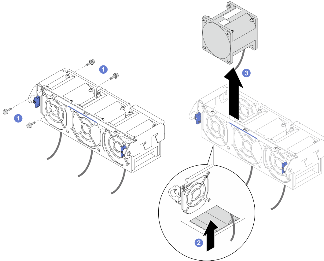
Figura 40. Extracción del ventilador
