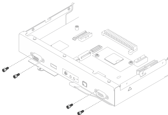
Figura 107. Extracción de los tornillos
