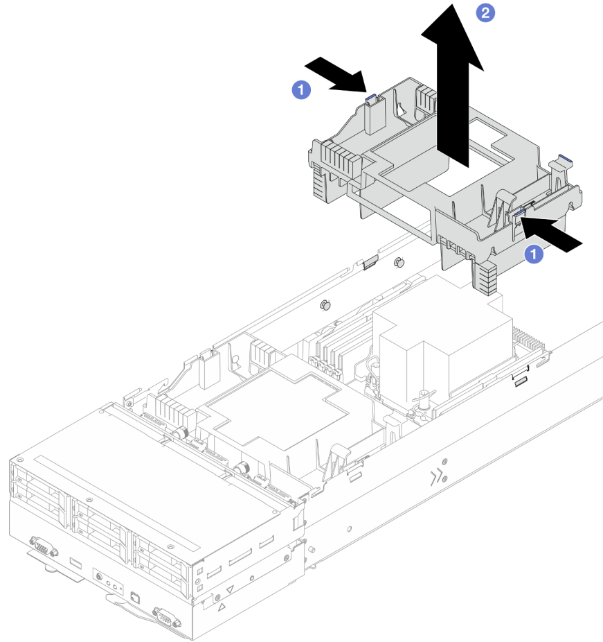
Figura 25. Extracción del deflector de aire posterior
