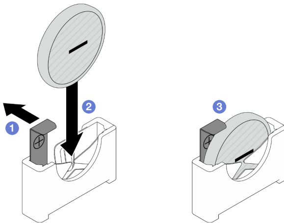
Figura 34. Instalación de una batería CMOS
