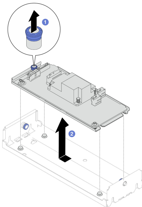
Figura 28. Extracción del adaptador CFF interno
