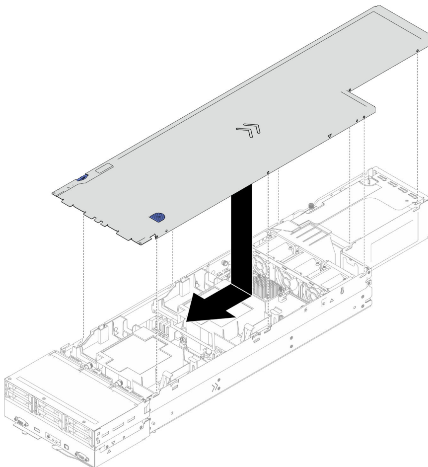
Figura 115. Instalación de la cubierta superior
