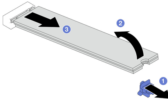
Figura 58. Extracción de una unidad M.2
