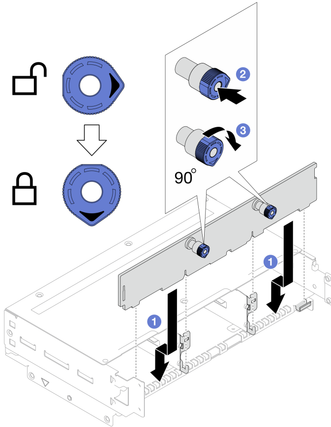
Figura 37. Instalación de la placa posterior de la unidad
