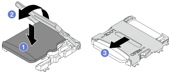
Figura 69. Instalación de una tarjeta MicroSD
