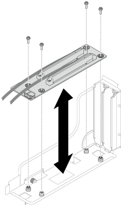
Figura 77. Sustitución de la tarjeta de expansión PCIe
