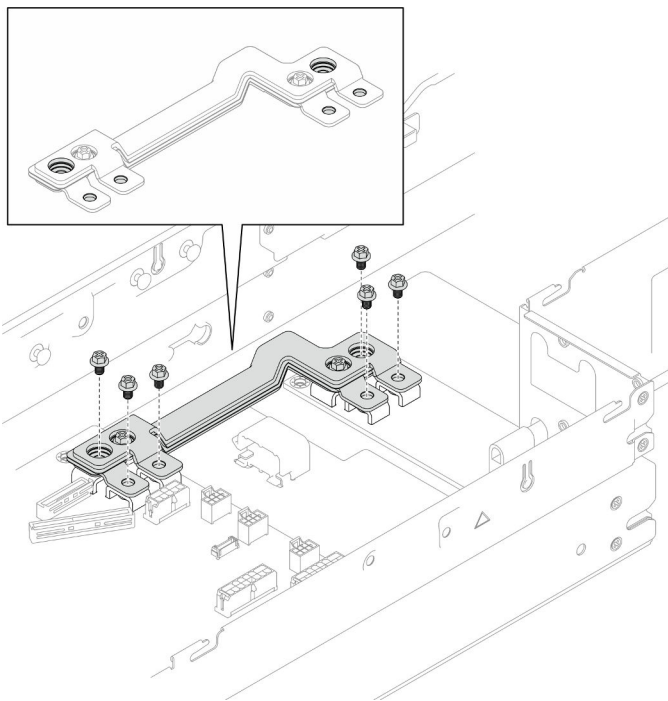
Figura 79. Extracción de los tornillos externos de la barra de bus de alimentación
