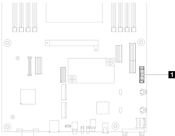
Figura 33. Ubicación del zócalo de la batería CMOS
