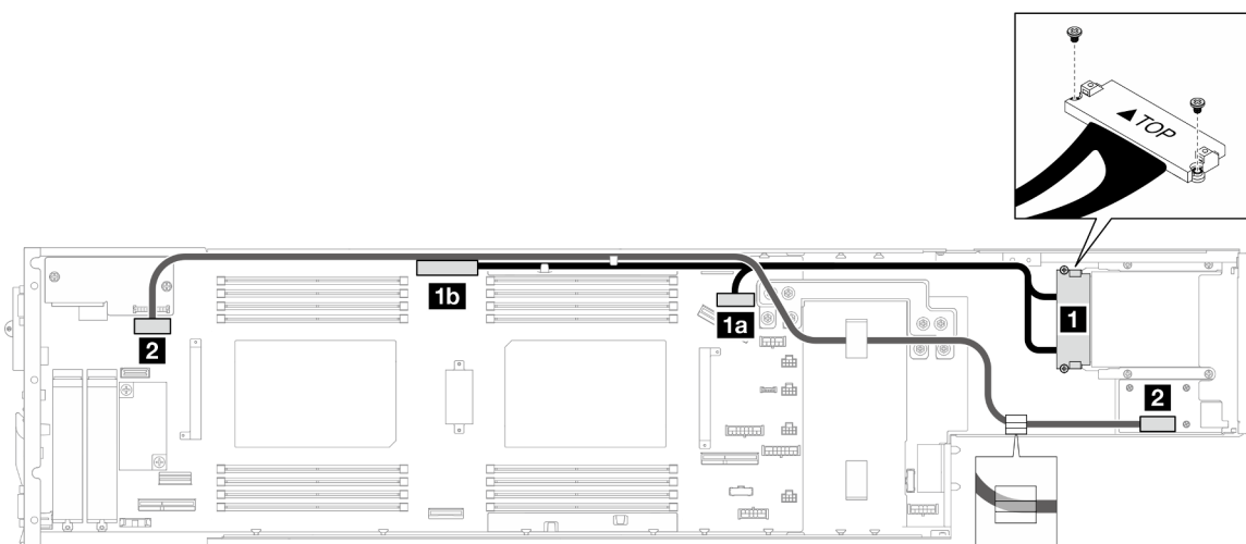
Figura 133. Cables para el módulo de E/S posterior y el módulo OCP
