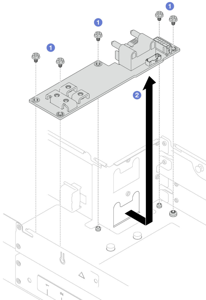
Figura 83. Extracción de la placa de distribución de alimentación
