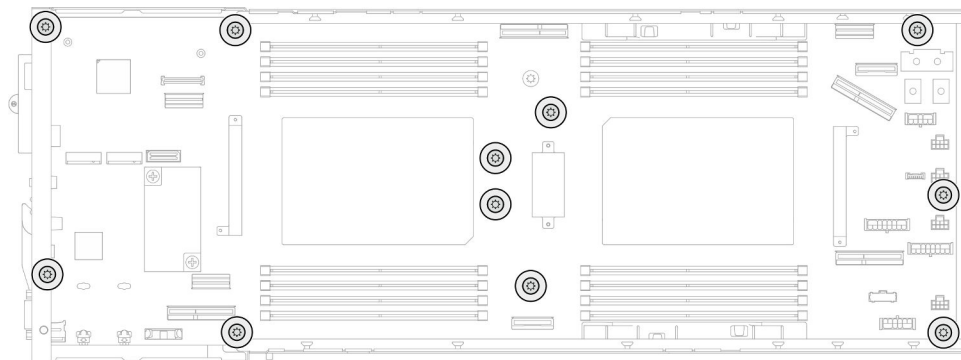
Figura 112. Instalación de los tornillos en la placa del sistema
