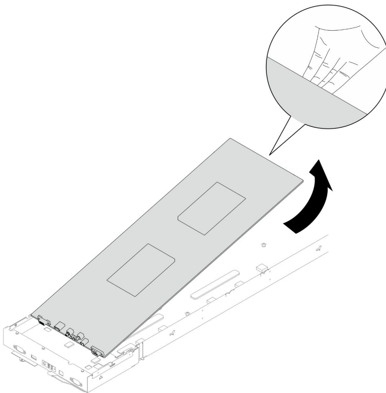
Figura 109. Extracción de la placa de sistema
