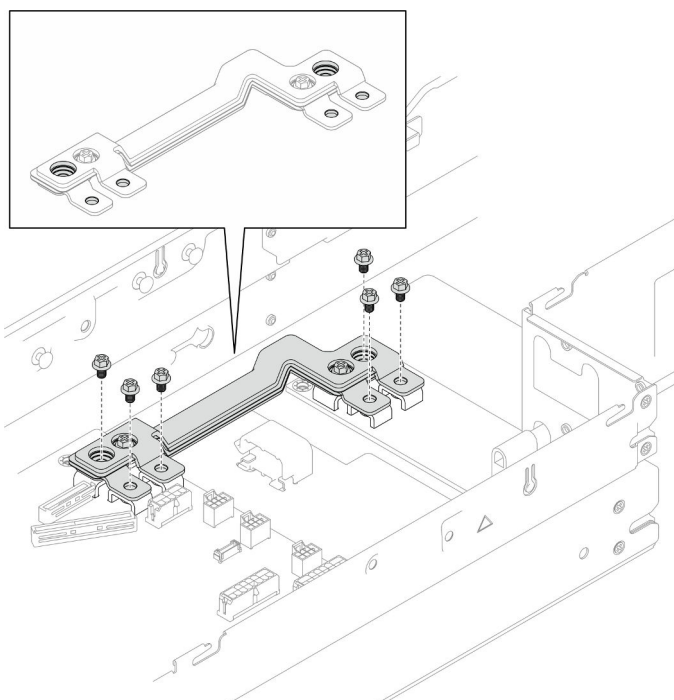
Figura 82. Instalación de los tornillos externos de la barra de bus de alimentación
