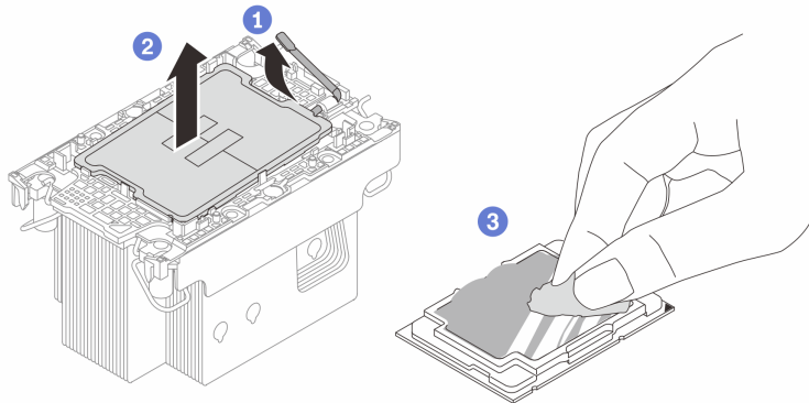
Figura 88. Separación de un procesador del disipador de calor y del transportador
