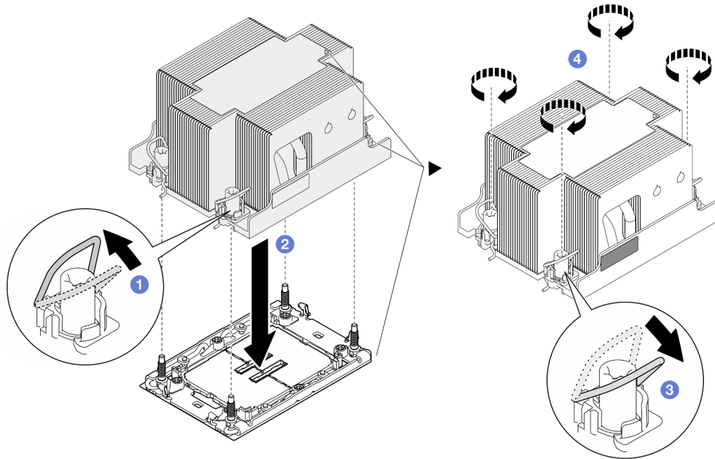
Figura 94. Instalación de un PHM estándar 2U
