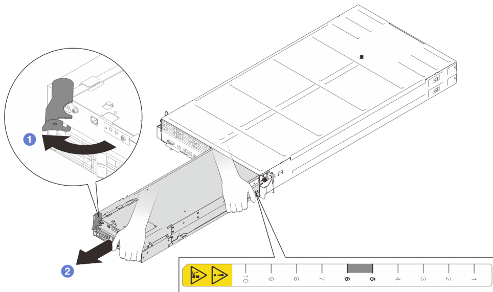
Figura 17. Extracción del nodo de la bandeja derecha
