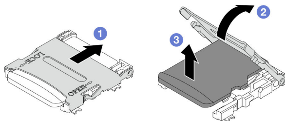
Figura 67. Extracción de la tarjeta MicroSD
