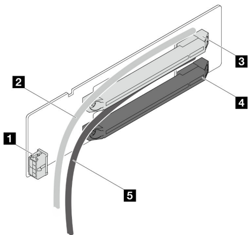
Figura 119. Conectores y cables de la tarjeta de expansión PCIe de dos ranuras
