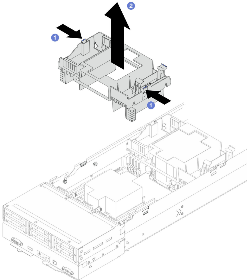
Figura 24. Extracción del deflector de aire frontal
