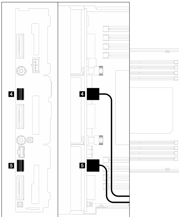
Figura 126. Cables SATA en la placa posterior de la unidad
