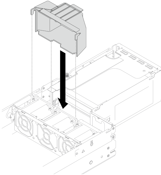
Figura 48. Instalación del conducto de aire de GPU
