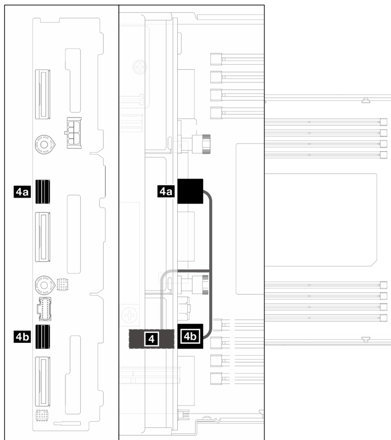
Figura 123. Disposición de los cables SATA - Configuración sin RAID CFF
