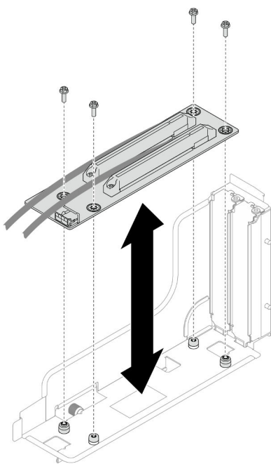
Figura 73. Sustitución de la tarjeta de expansión PCIe
