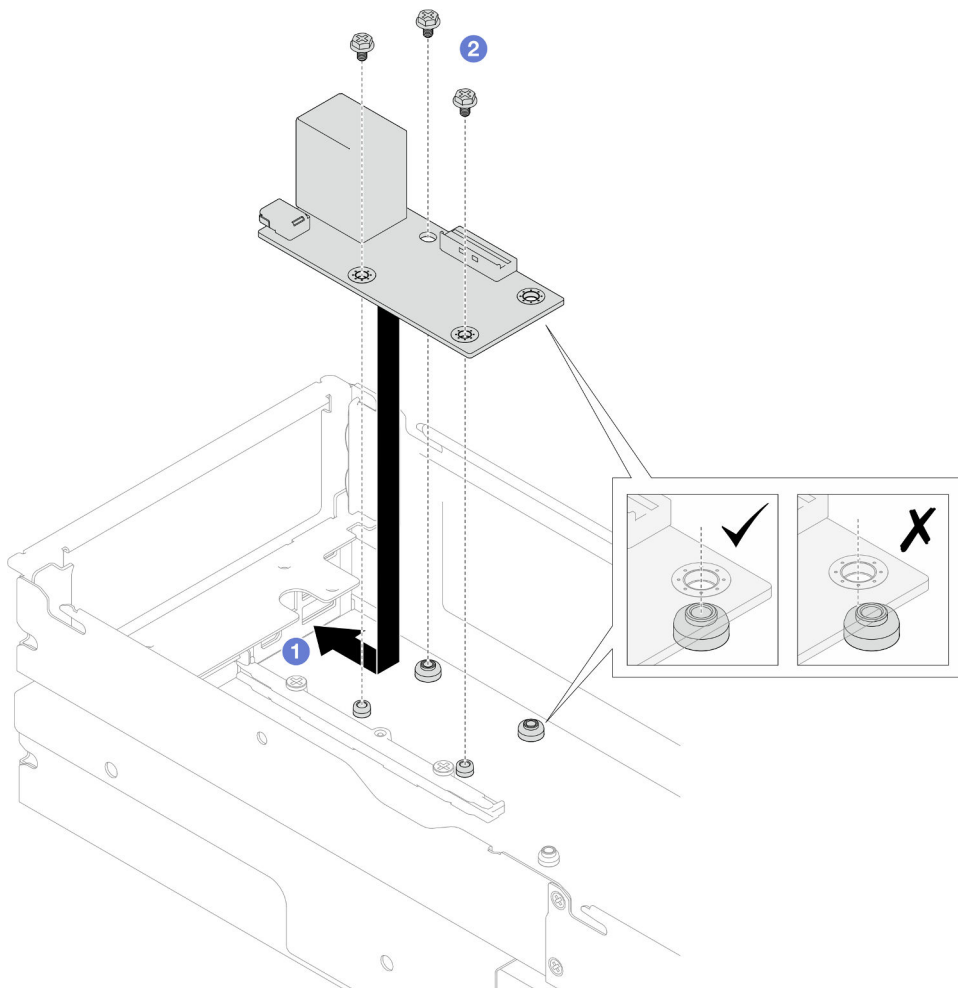
Figura 98. Instalación del módulo de E/S posterior
