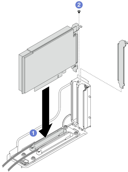
Figura 76. Instalación de un adaptador PCIe
