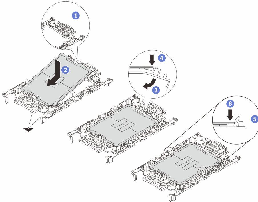
Figura 91. Instalación del transportador del procesador
