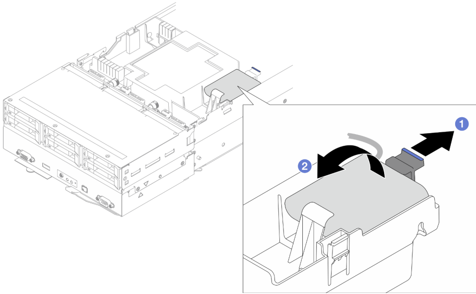
Figura 43. Extracción del módulo de alimentación flash
