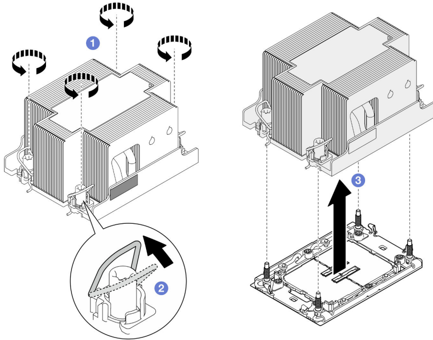
Figura 86. Extracción del PHM estándar 2U
