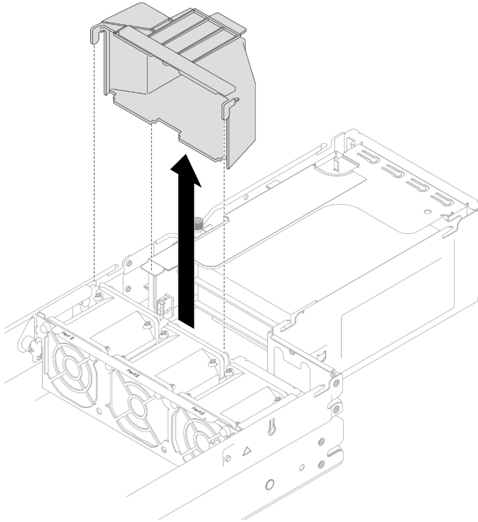
Figura 47. Extracción del conducto de aire de GPU
