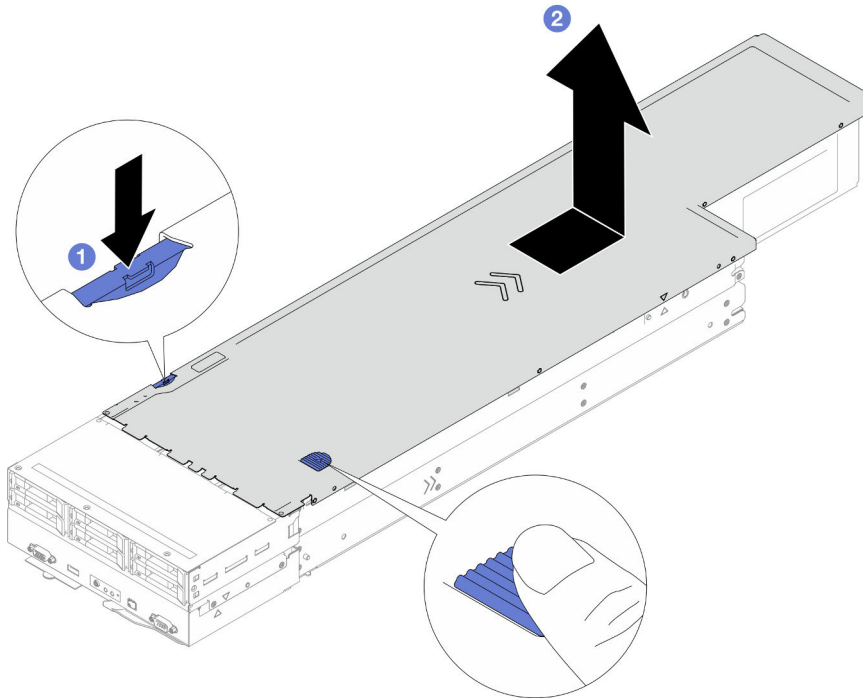
Figura 114. Extracción de la cubierta superior
