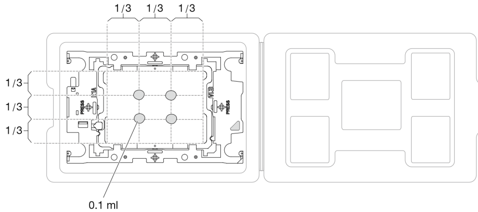
Figura 92. Aplicación de grasa térmica con el procesador en la bandeja de envío
