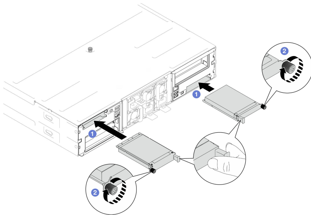
Figura 71. Instalación del módulo de OCP posterior
