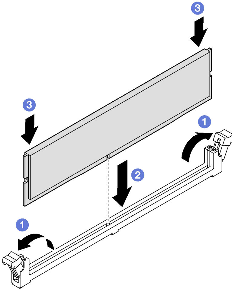
Figura 65. Instalación de un módulo de memoria
