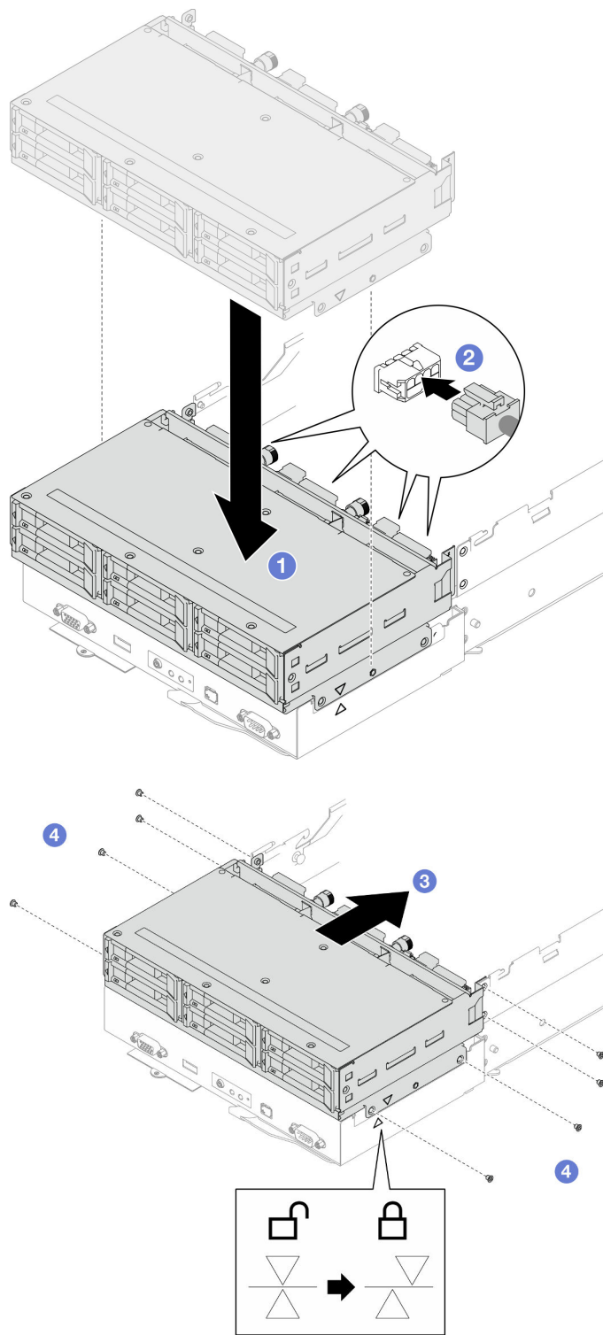
Figura 38. Instalación del conjunto del compartimiento de la unidad
