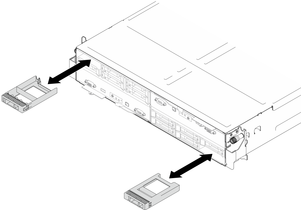
Figura 51. Sustitución de un relleno de unidad
