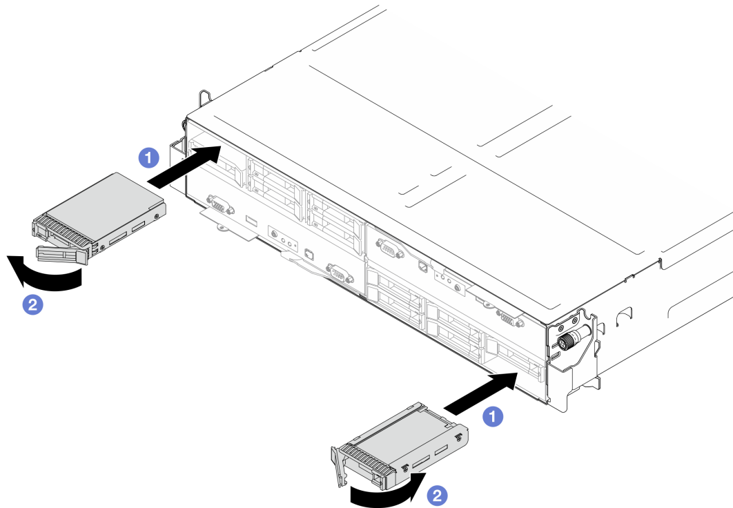
Figura 53. Instalación de una unidad de estado sólido de 7 mm
