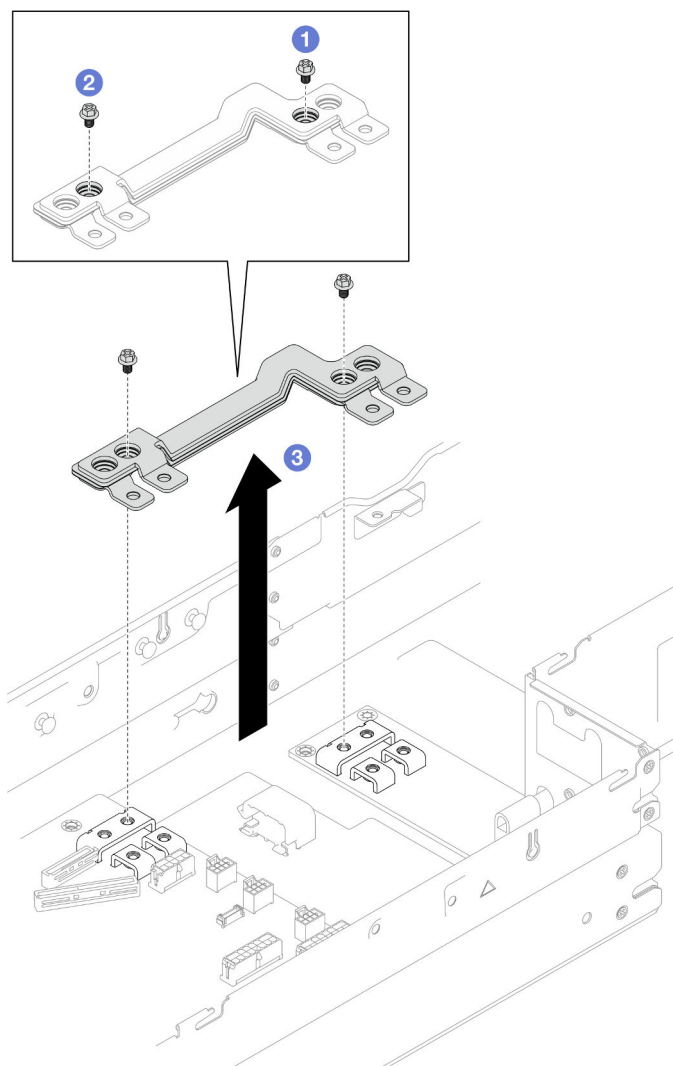
Figura 94. Extracción de la barra de bus de alimentación
