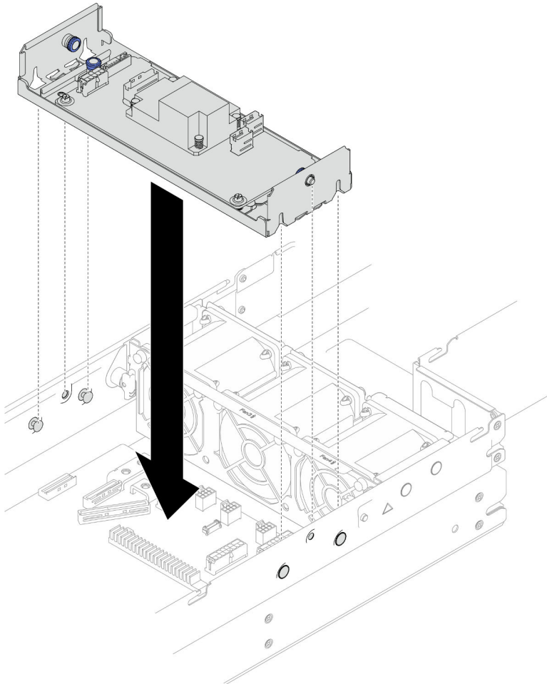
Figura 70. Instalación del soporte del adaptador interno
