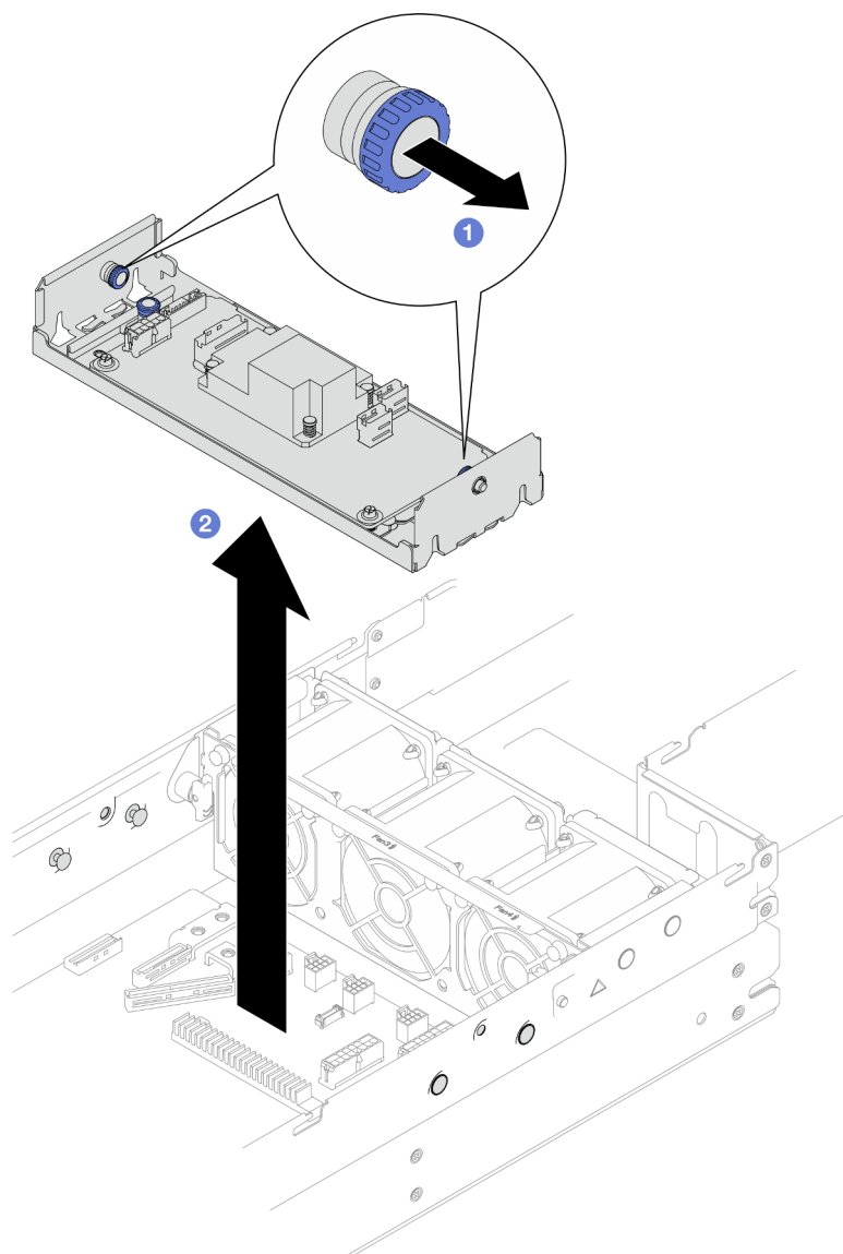
Figura 69. Extracción del soporte del adaptador interno
