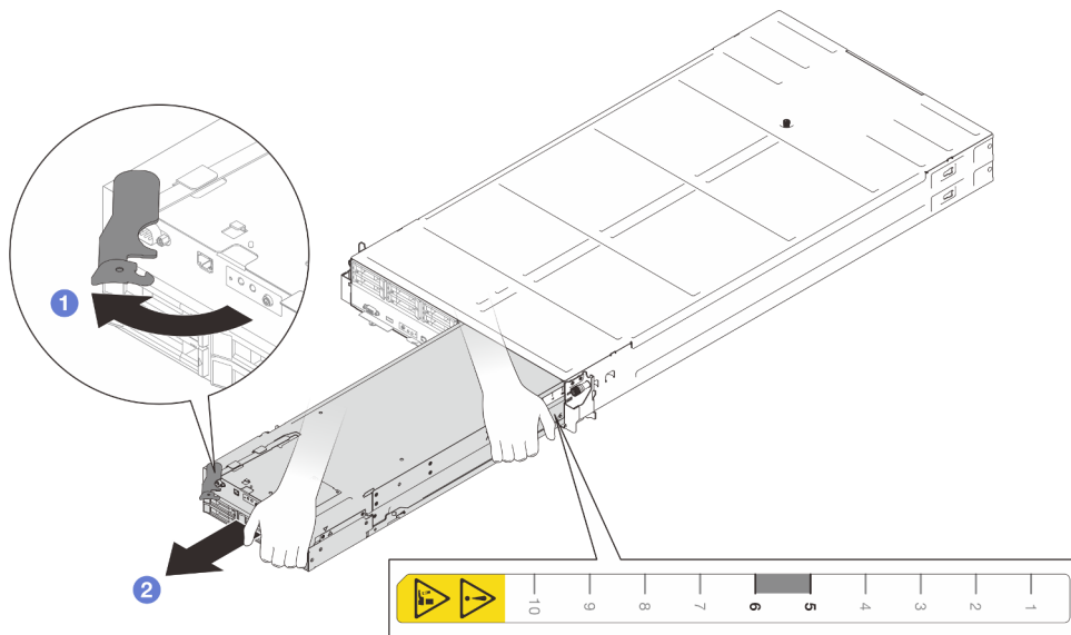
Figura 31. Extracción del nodo de la bandeja derecha
