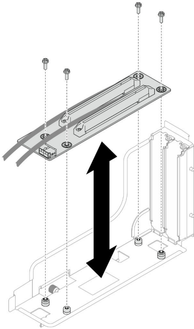
Figura 89. Sustitución de la tarjeta de expansión PCIe
