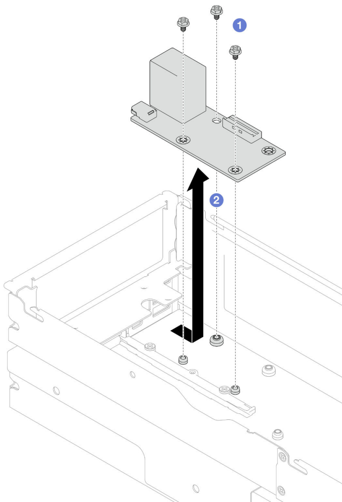
Figura 111. Extracción del módulo de E/S posterior
