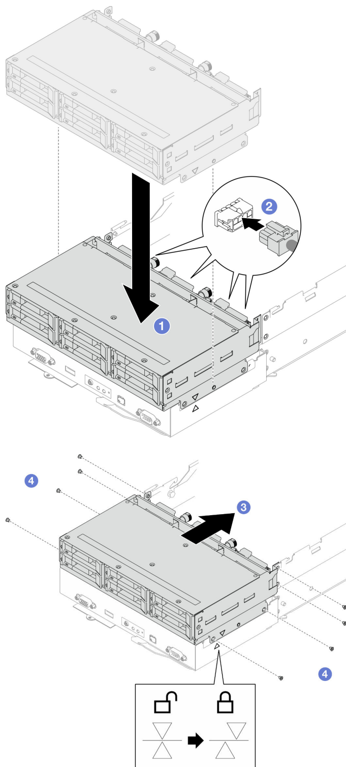
Figura 52. Instalación del conjunto del compartimiento de la unidad
