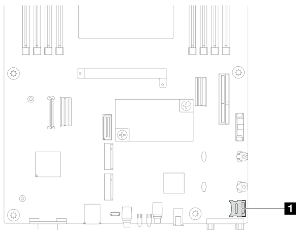
Figura 80. Ubicación del zócalo de MicroSD
