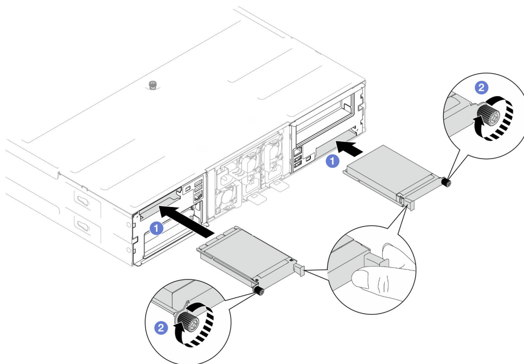
Figura 85. Instalación del módulo de OCP posterior
