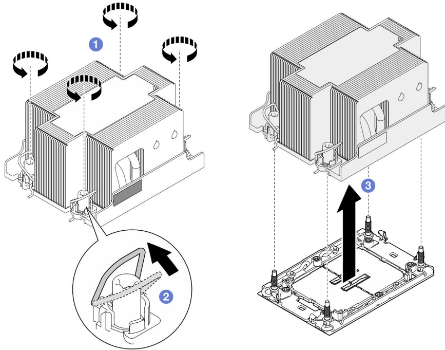
Figura 100. Extracción del PHM estándar 2U
