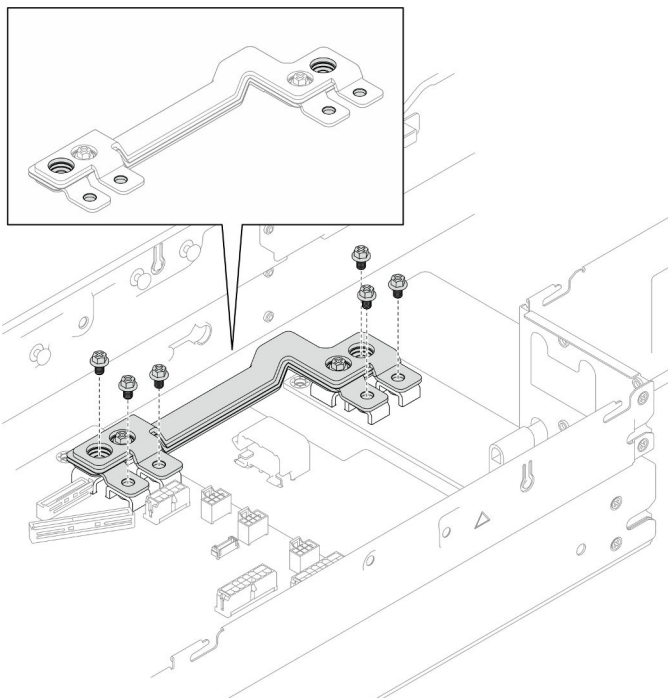
Figura 93. Extracción de los tornillos externos de la barra de bus de alimentación
