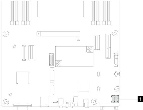
Figura 82. Ubicación del zócalo de MicroSD
