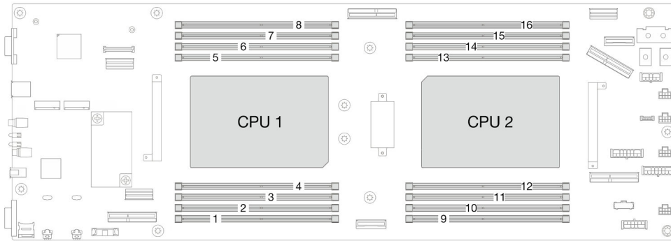
Figura 78. Diseño de los módulos de memoria y el procesador
