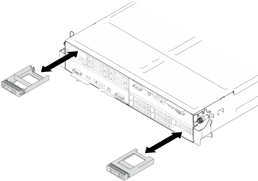
Figura 65. Sustitución de un relleno de unidad
