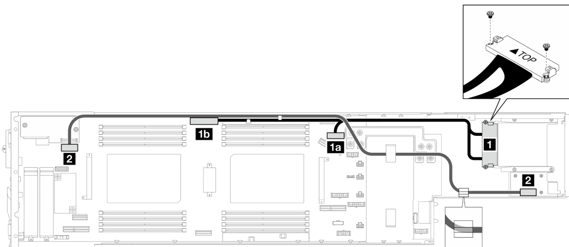
Figura 147. Cables para el módulo de E/S posterior y el módulo OCP
