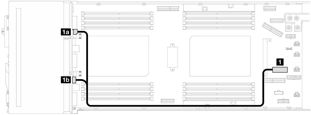
Figura 135. Disposición de los cables de alimentación de la placa posterior de la unidad
