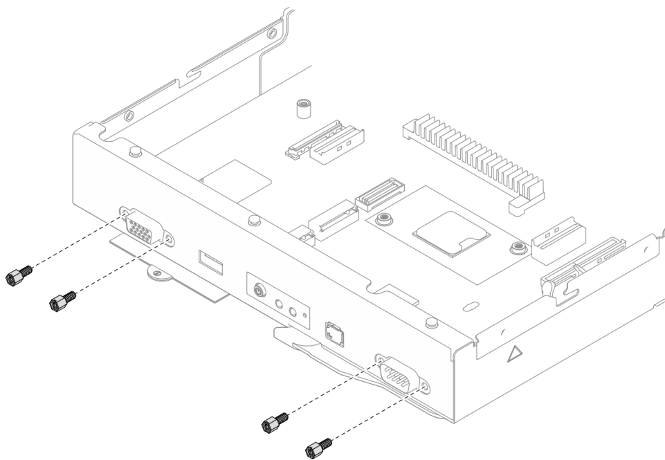
Figura 125. Instalación de los tornillos de la placa del sistema en la parte frontal
