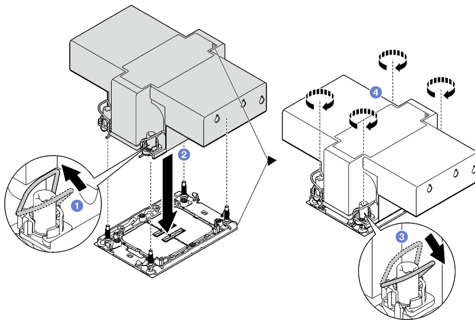
Figura 109. Instalación de un PHM de rendimiento 2U
