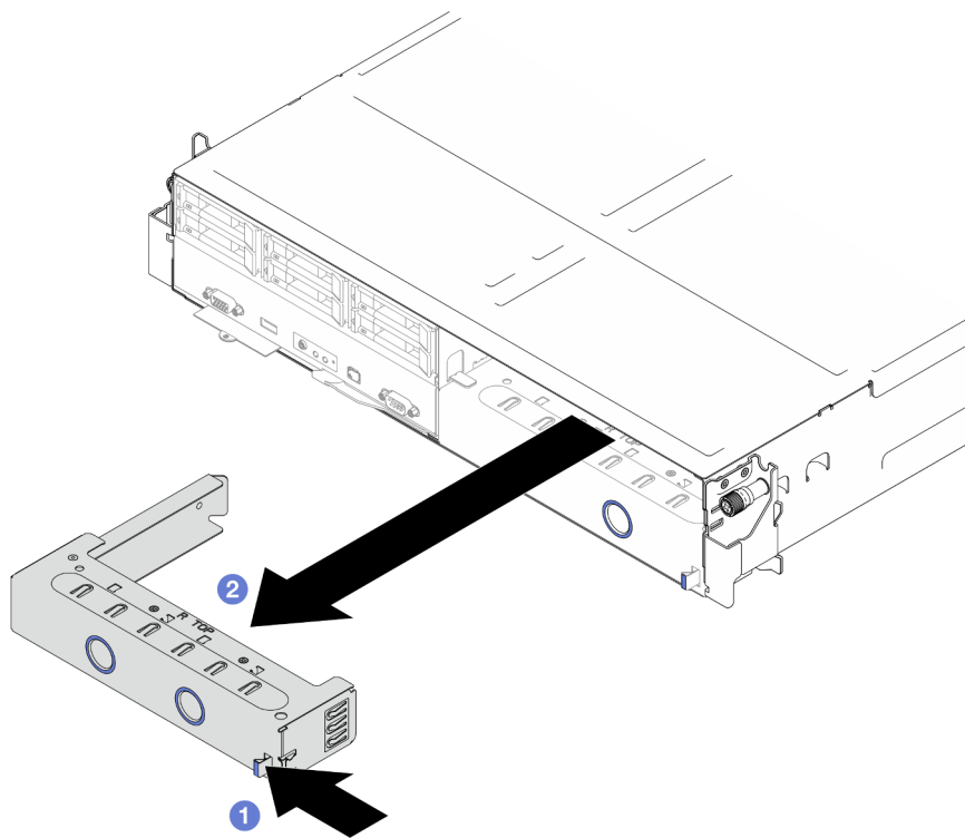
Figura 34. Extracción de un relleno de la bandeja del nodo frontal
