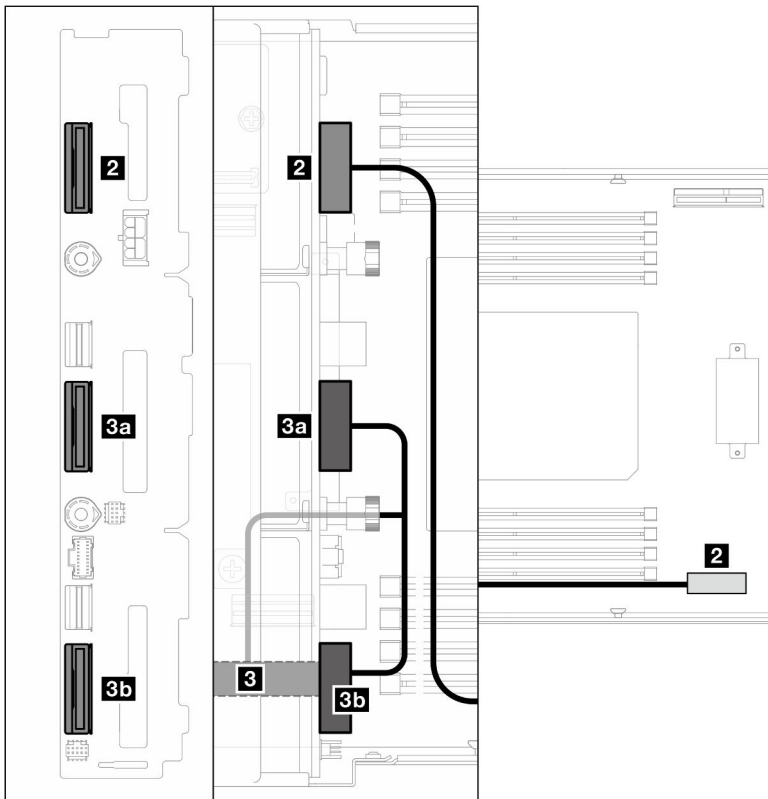
Figura 136. Disposición de los cables NVMe
