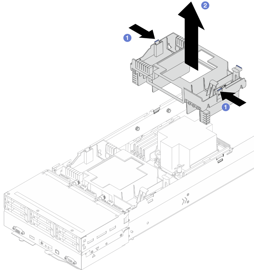
Figura 39. Extracción del deflector de aire posterior
