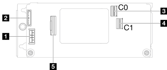
Figura 131. Conectores del adaptador RAID CFF interno
