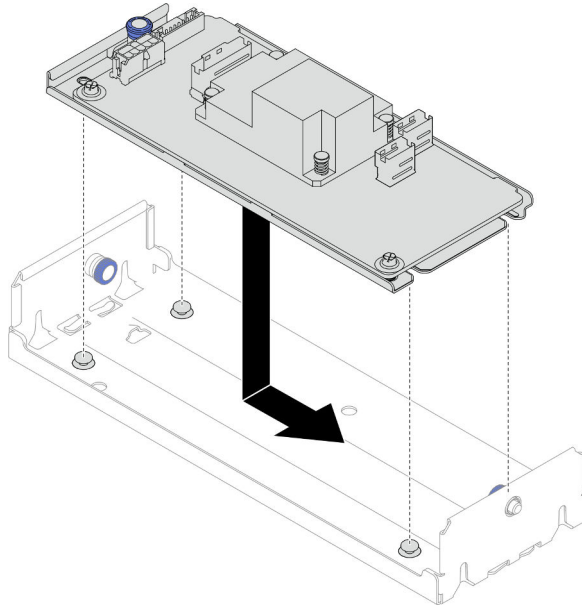
Figura 44. Instalación del adaptador RAID CFF interno en el soporte
