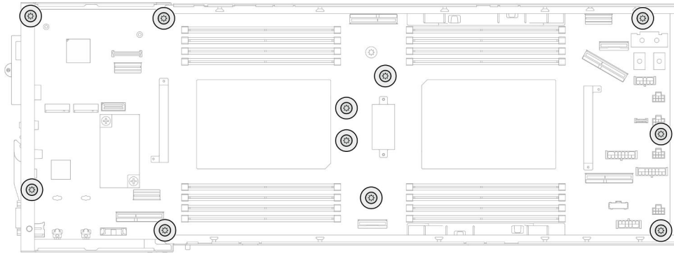
Figura 122. Extracción de los tornillos
