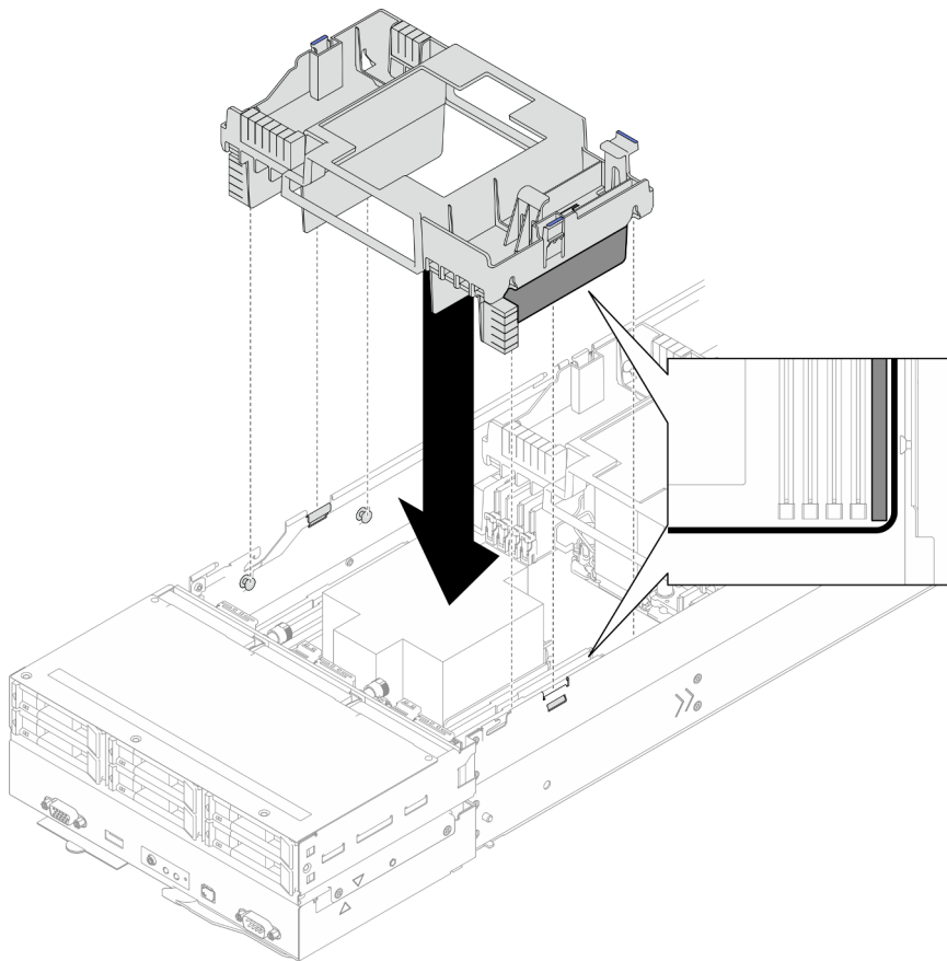
Figura 40. Instalación del deflector de aire frontal
