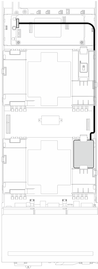
Figura 60. RAID CFF y cable del módulo de alimentación flash
