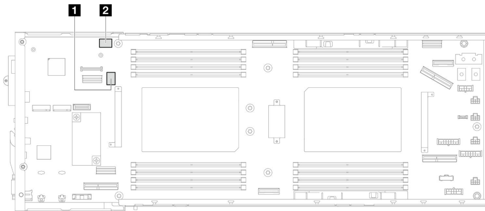
Figura 9. Conmutadores de la placa del sistema
