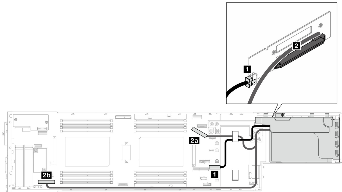
Figura 144. Disposición de cables de la expansión PCIe – un procesador
