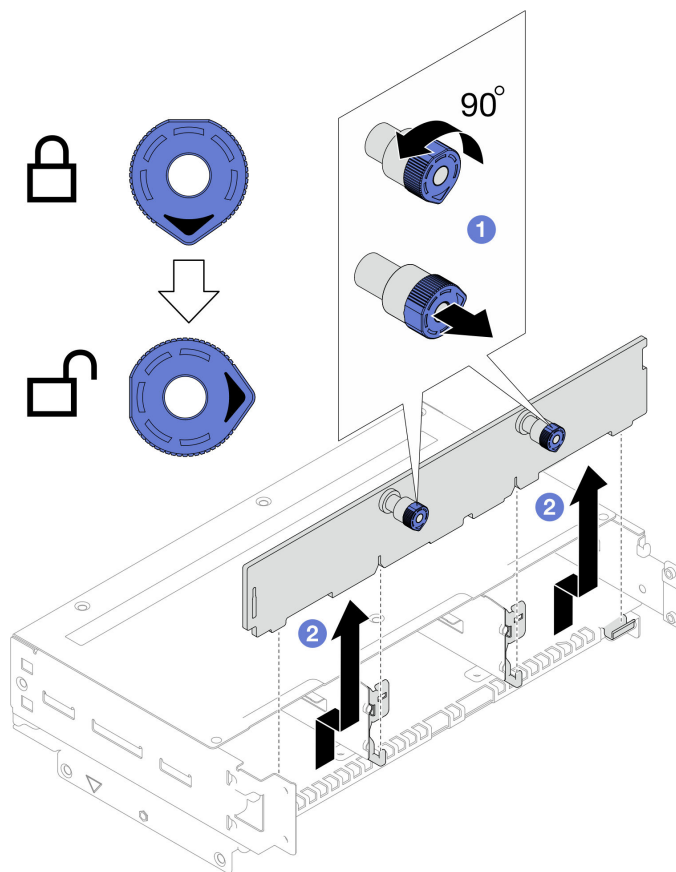
Figura 50. Extracción de la placa posterior de la unidad
