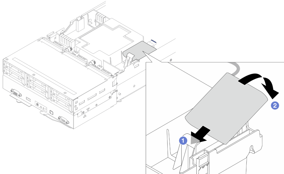
Figura 58. Instalación del módulo de alimentación flash
