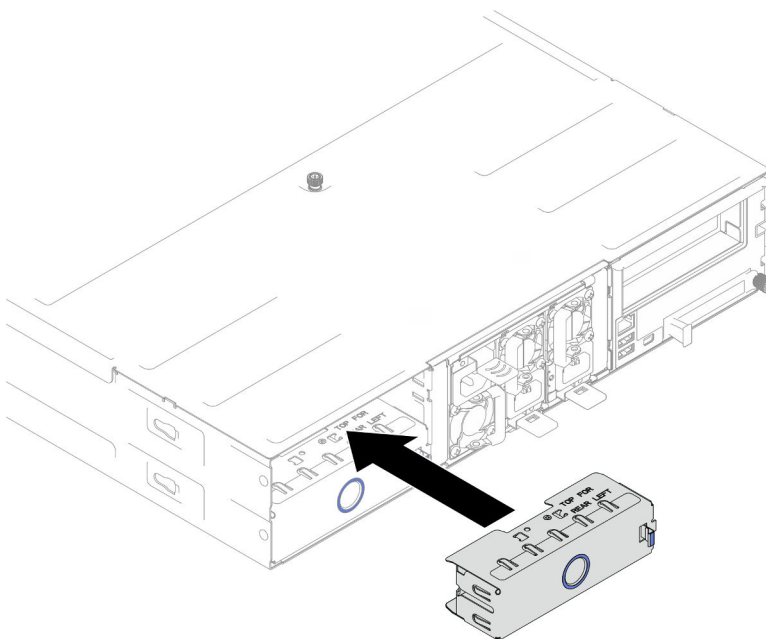
Figura 33. Instalación de un relleno de la bandeja del nodo posterior
