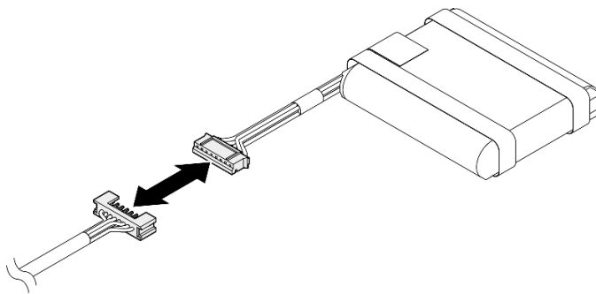
Figura 59. Cable de extensión del módulo de alimentación flash
