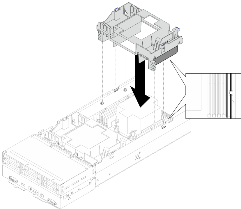
Figura 41. Instalación del deflector de aire posterior
