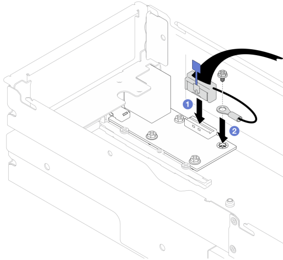
Figura 113. Instalación del cable de E/S posterior y del cable de conexión a tierra
