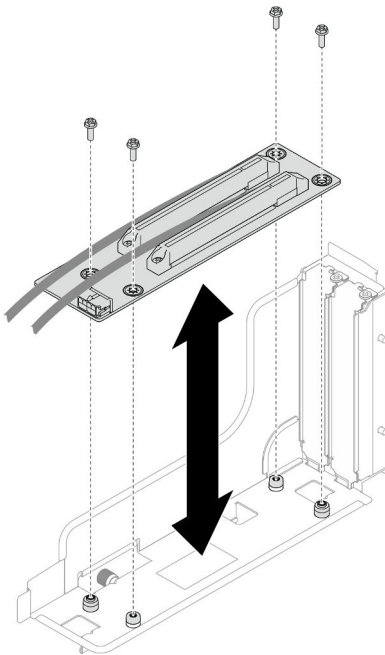
Figura 91. Sustitución de la tarjeta de expansión PCIe
