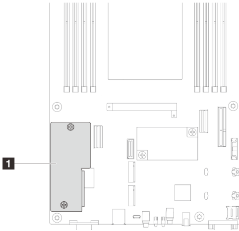
Figura 118. Ubicación del Firmware y módulo de seguridad de RoT
