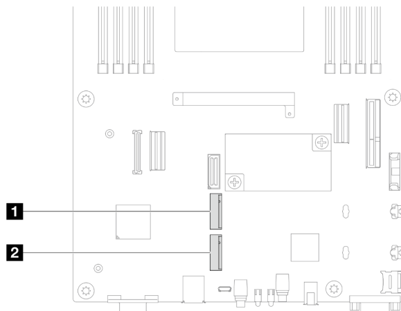
Figura 74. Ubicación de las bahías M.2 en la placa del sistema
