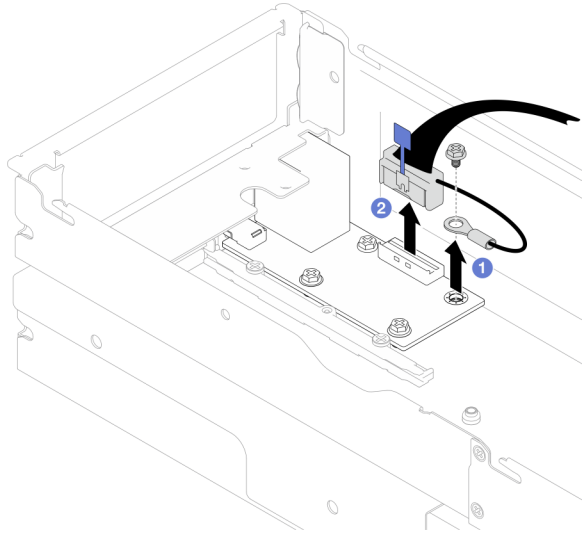
Figura 110. Extracción del cable de E/S posterior y del cable de conexión a tierra
