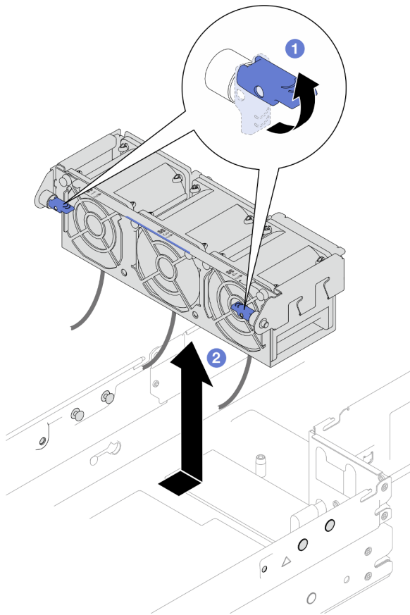
Figura 53. Extracción del compartimiento del ventilador
