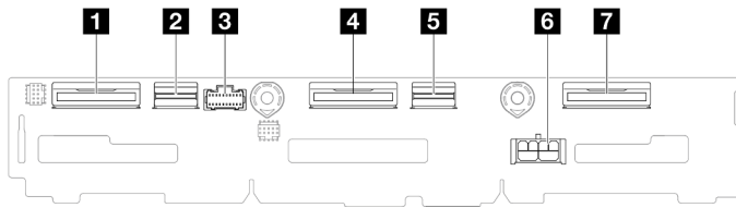
Figura 130. Placa posterior de la unidad de 2,5 pulgadas
