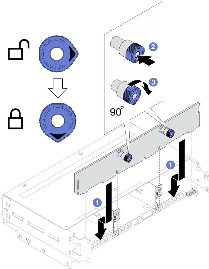
Figura 51. Instalación de la placa posterior de la unidad
