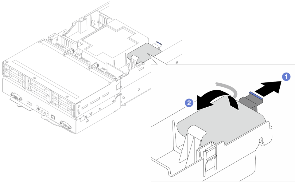
Figura 57. Extracción del módulo de alimentación flash
