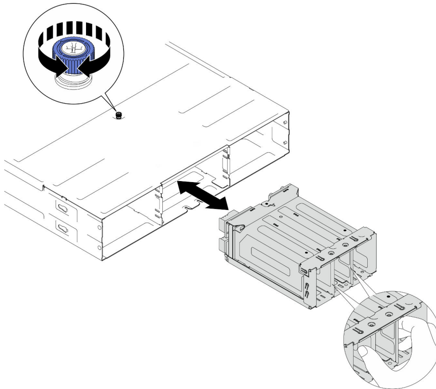
Figura 29. Instalación del compartimiento de PSU
