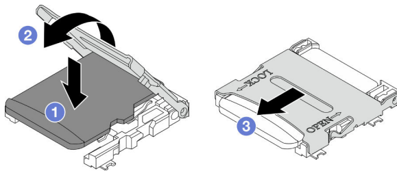
Figura 83. Instalación de una tarjeta MicroSD
