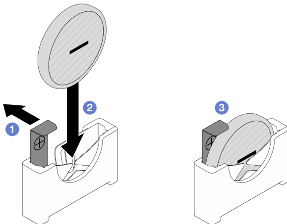
Figura 48. Instalación de una batería CMOS
