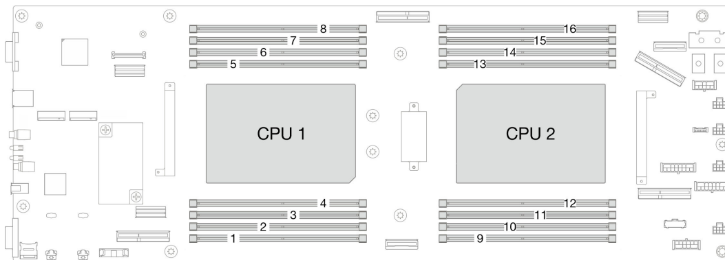
Figura 15. Diseño de los módulos de memoria y el procesador
