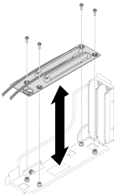
Figura 87. Sustitución de la tarjeta de expansión PCIe
