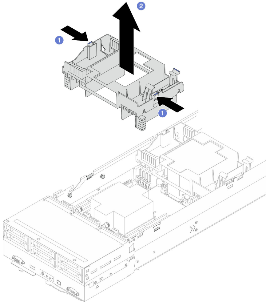
Figura 38. Extracción del deflector de aire frontal
