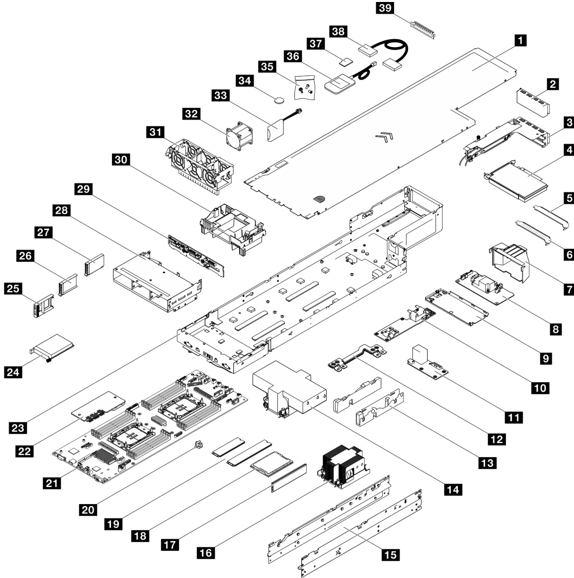
Figura 11. Componentes del nodo
