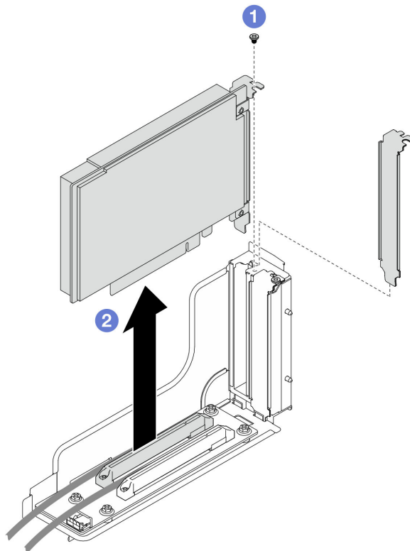
Figura 88. Extracción de un adaptador PCIe
