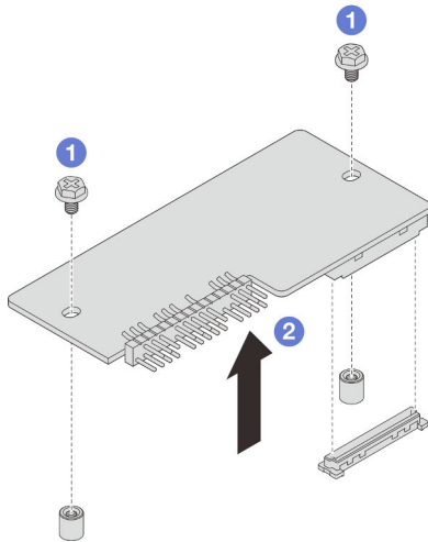
Figura 117. Extracción de la Firmware y módulo de seguridad de RoT
