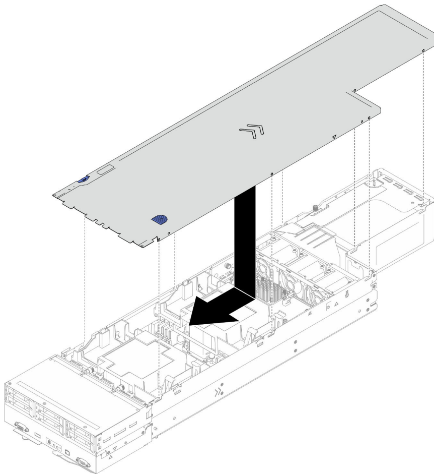
Figura 129. Instalación de la cubierta superior
