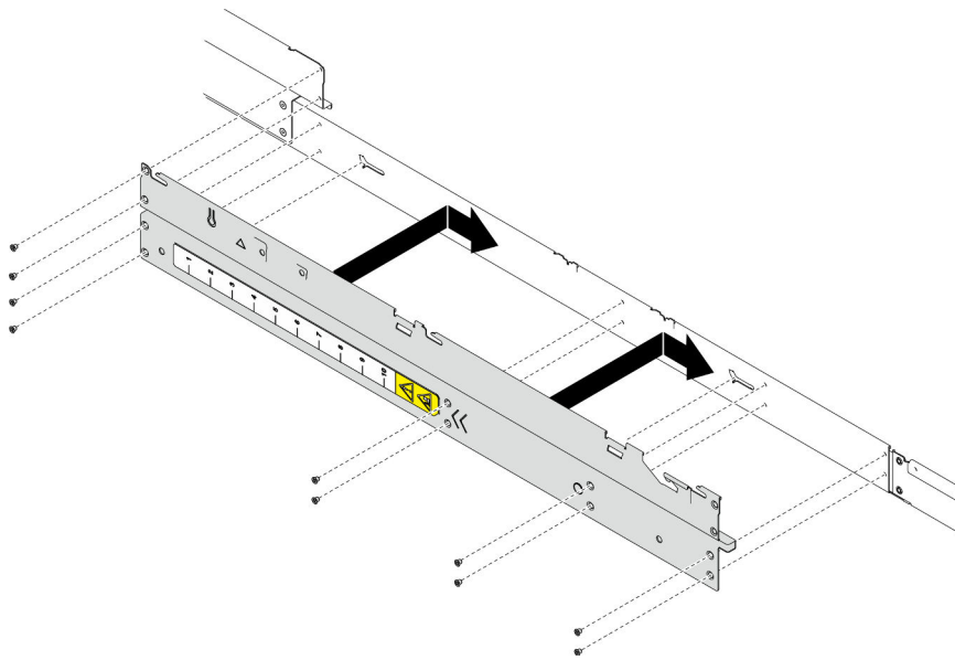
Figura 115. Instalación del soporte lateral
