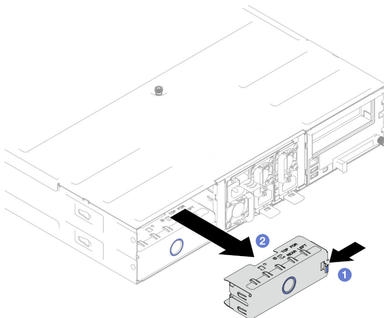
Figura 35. Extracción de un relleno de la bandeja del nodo posterior
