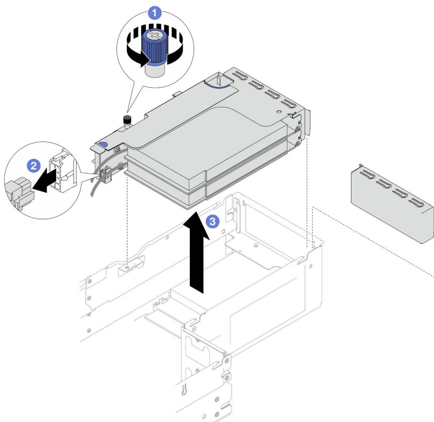
Figura 86. Extracción del conjunto de expansión PCIe
