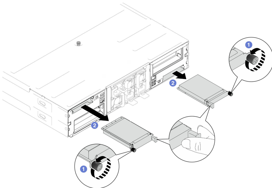
Figura 84. Extracción del módulo de OCP posterior
