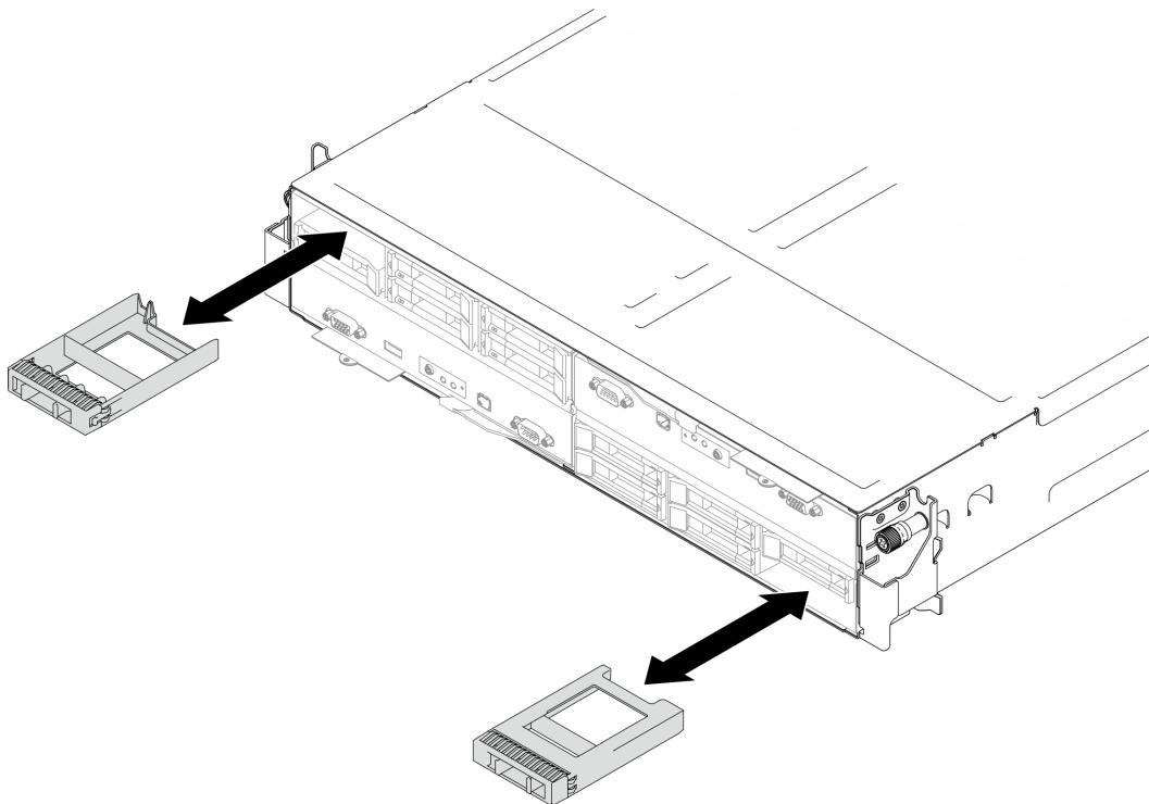
Figura 66. Sustitución de un relleno de unidad
