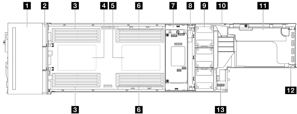
Figura 7. Vista superior de SD550 V3
