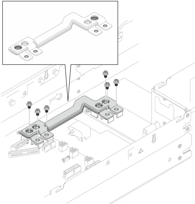
Figura 96. Instalación de los tornillos externos de la barra de bus de alimentación
