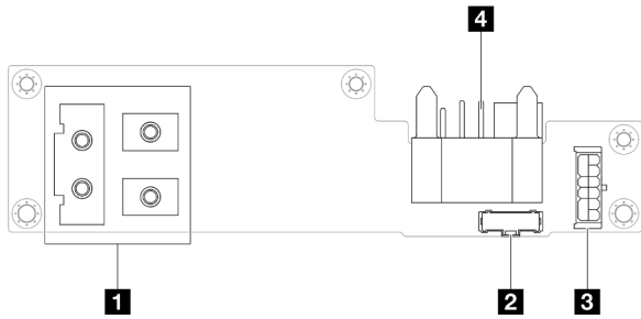
Figura 134. Conectores de placa de distribución de alimentación
