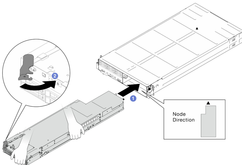
Figura 37. Instalación de un nodo en la bandeja derecha
