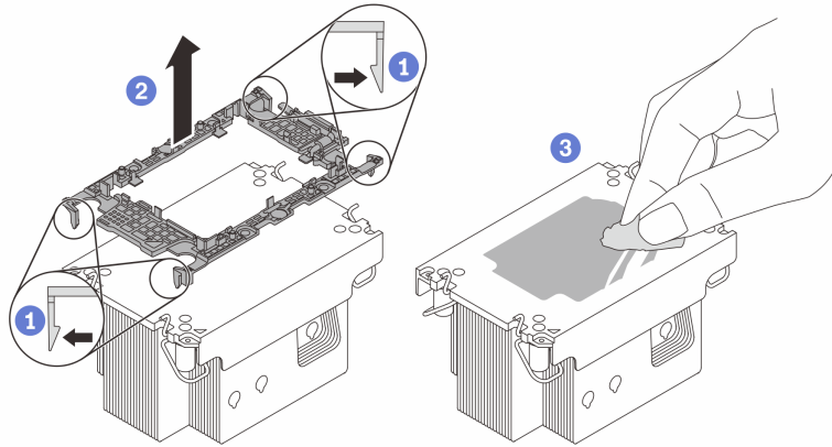
Figura 103. Separación de un transportador de procesador del disipador de calor
