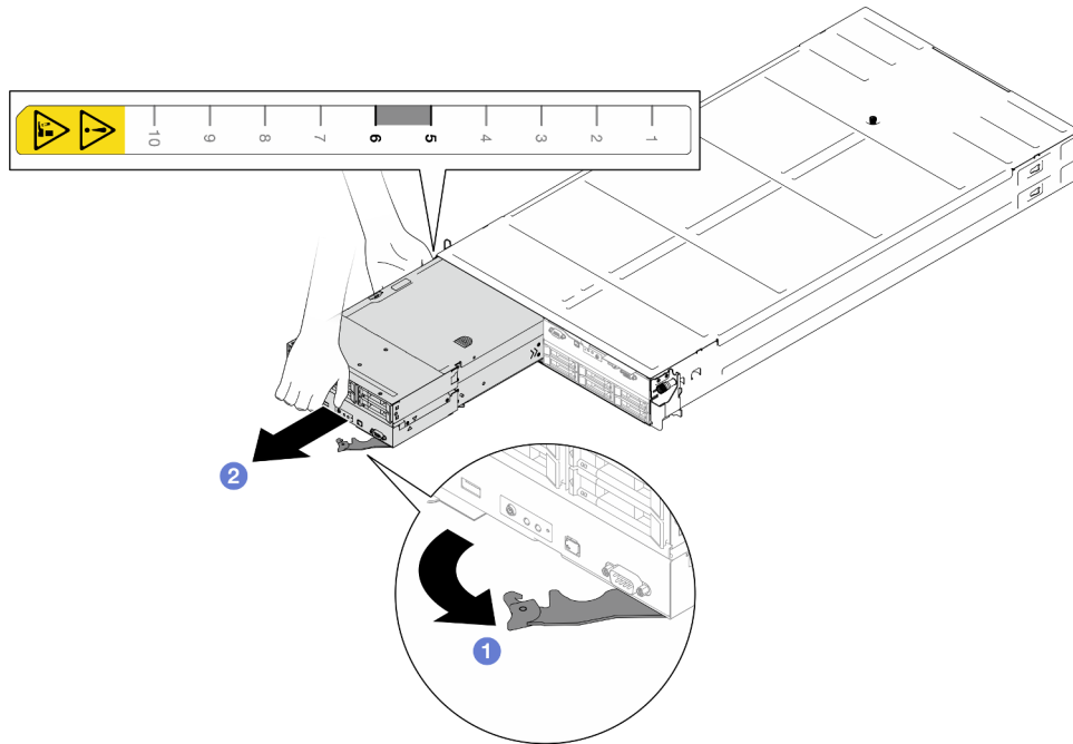
Figura 30. Extracción del nodo de la bandeja izquierda
