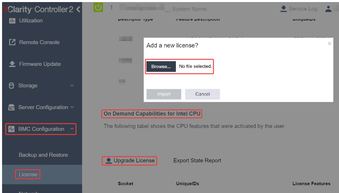
Figura 151. Carga de la clave de activación a través de la GUI web de XCC
