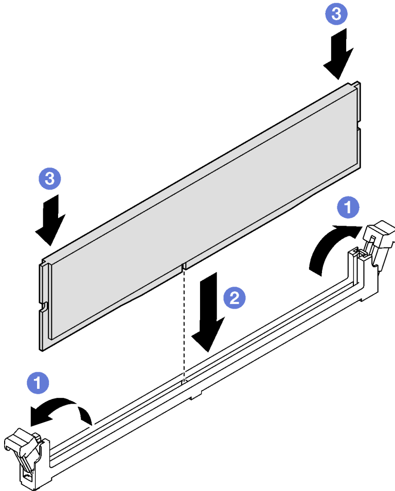
Figura 79. Instalación de un módulo de memoria
