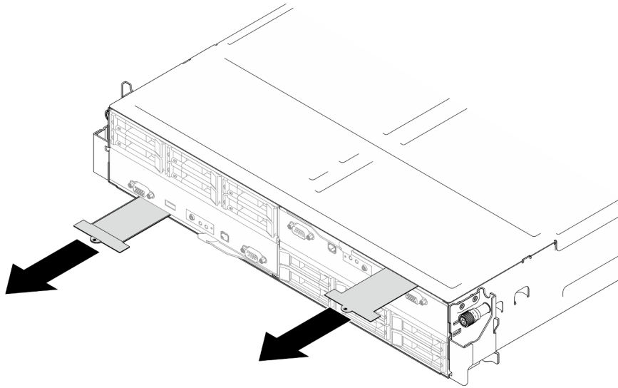
Figura 13. Etiqueta de acceso de red de Lenovo XClarity Controller en la pestaña de información extraíble.
