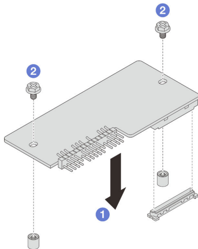
Figura 119. Instalación de la firmware y módulo de seguridad de RoT
