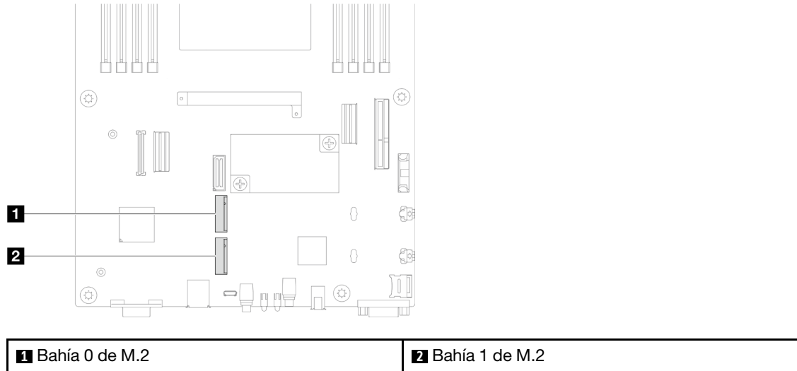
Figura 71. Ubicación de las bahías M.2 en la placa del sistema
