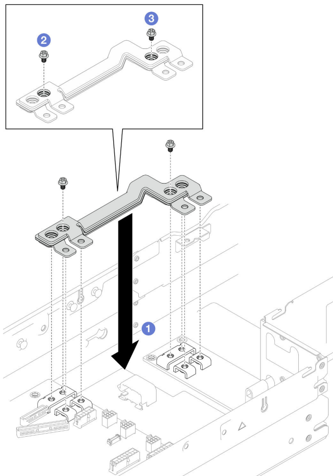
Figura 95. Instalación de la barra de bus de alimentación
