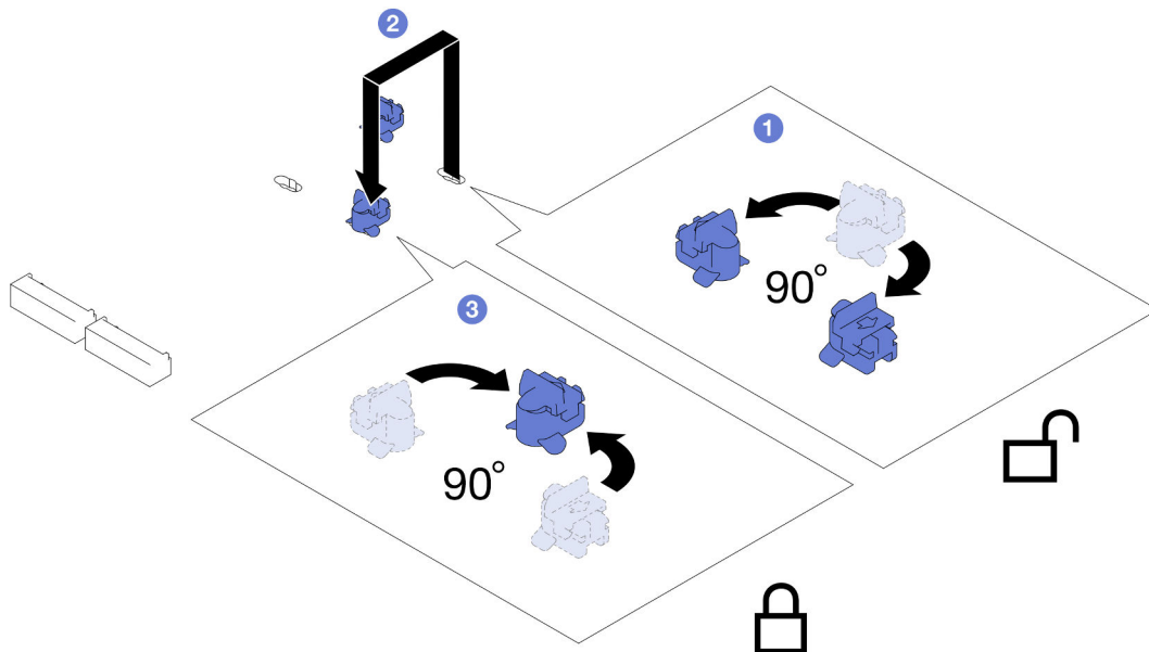
Figura 73. Ajuste de un elemento de sujeción de la unidad M.2
