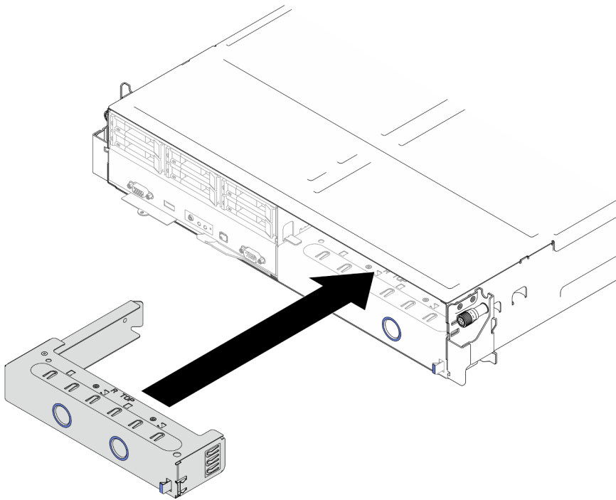
Figura 32. Instalación de un relleno de la bandeja del nodo frontal
