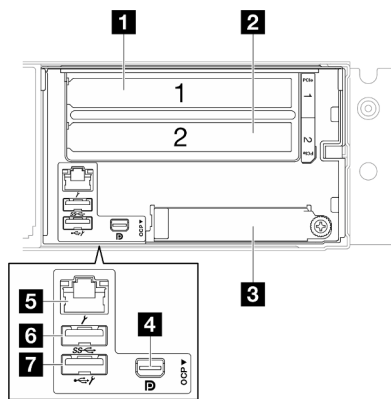
Figura 4. Vista posterior del nodo de ThinkSystem SD550 V3
