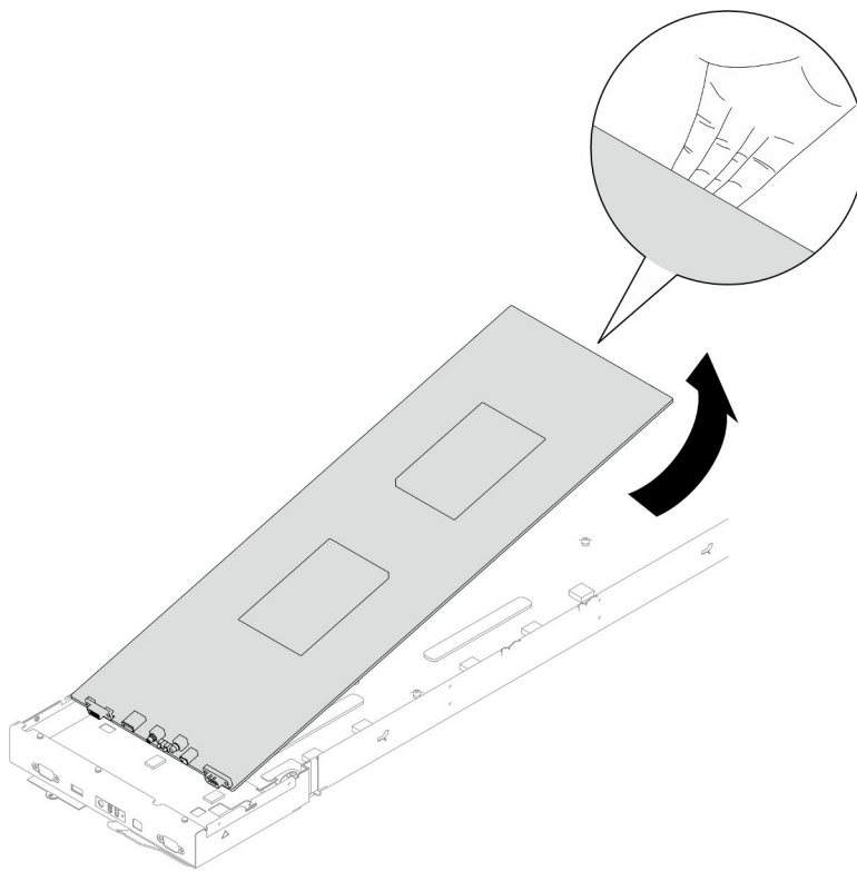
Figura 123. Extracción de la placa de sistema
