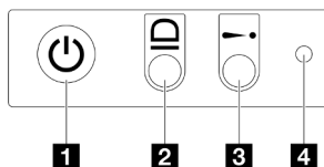
Figure 138. Boutons et voyants du panneau opérateur avant
