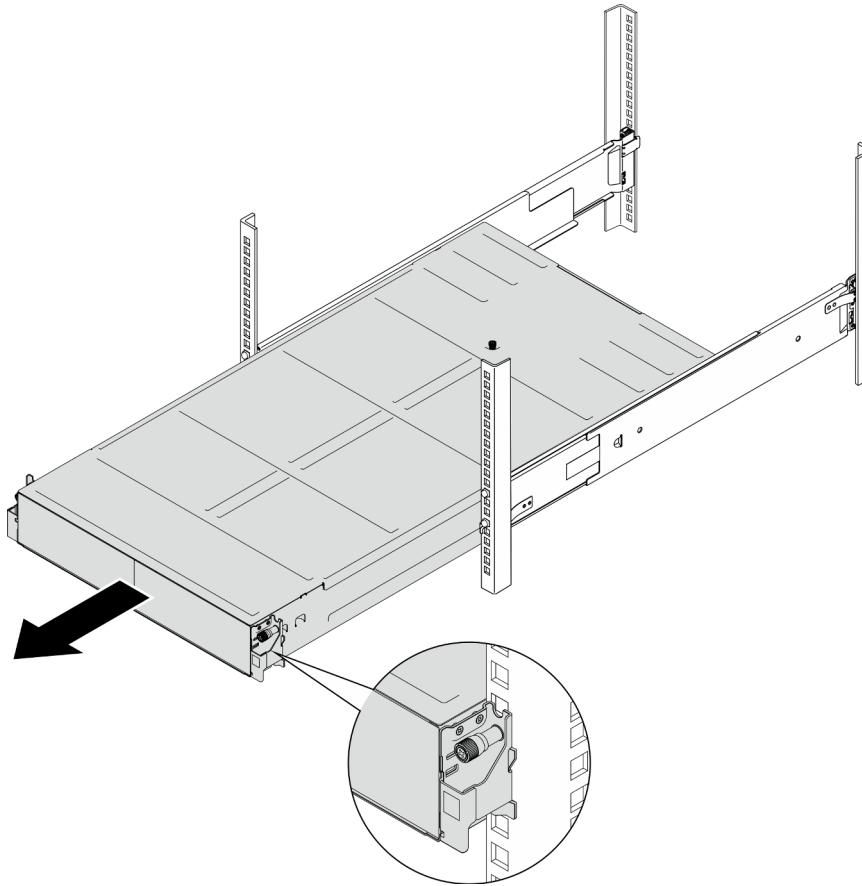
Figure 3. Retrait du châssis
