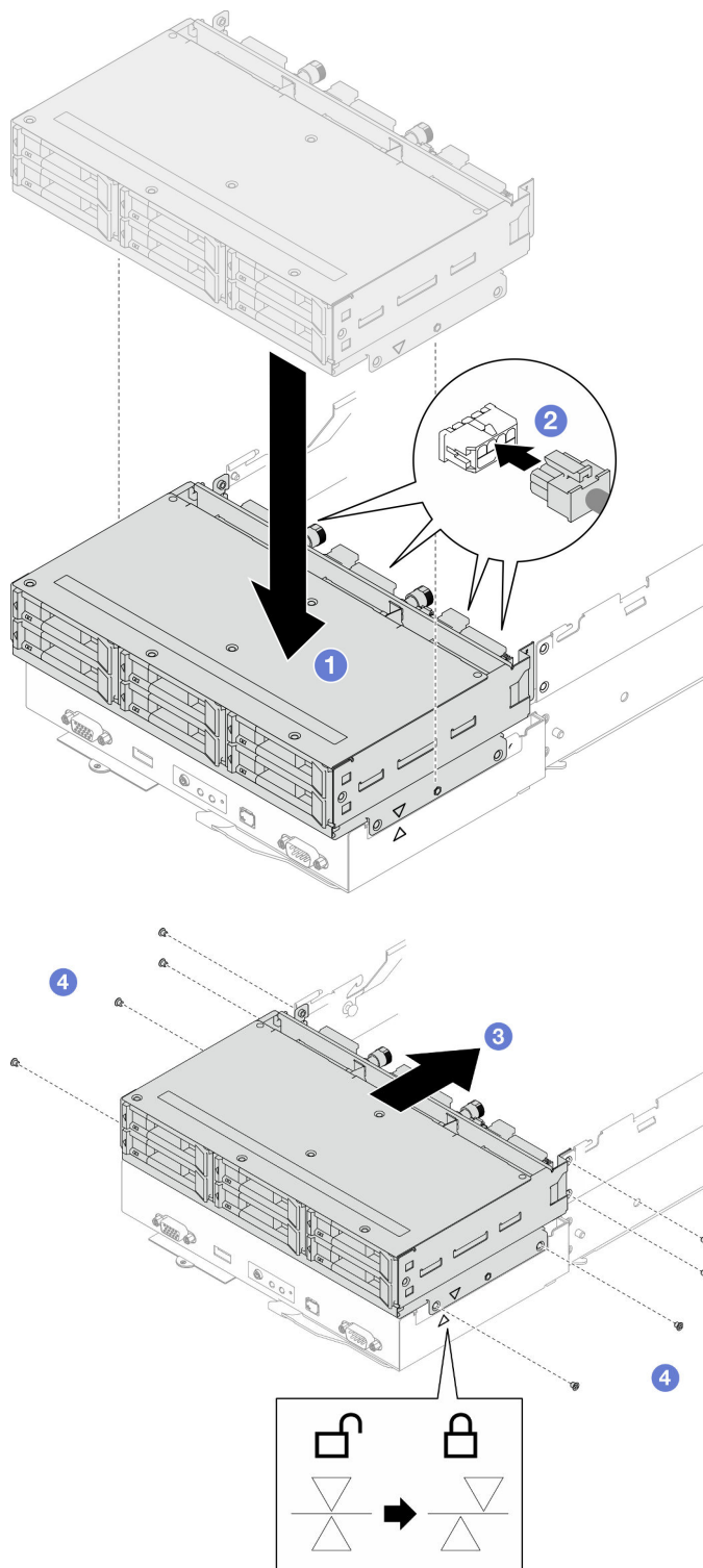
Figure 38. Installation du bloc boîtier d'unités de disque dur
