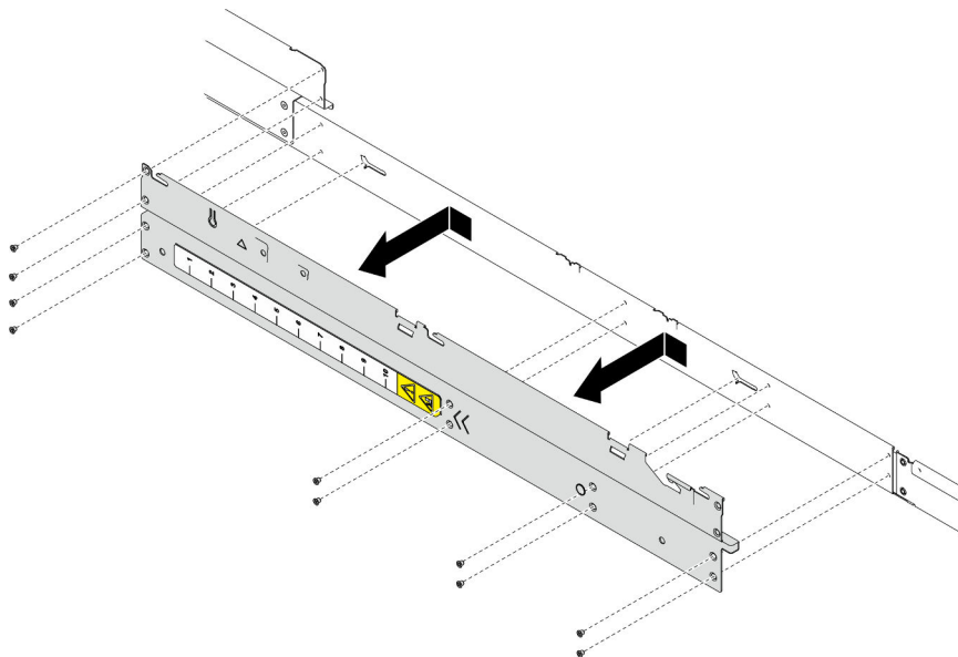
Figure 100. Retrait du support latéral
