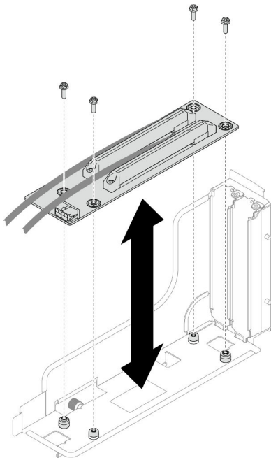
Figure 77. Remplacement de la carte mezzanine PCIe
