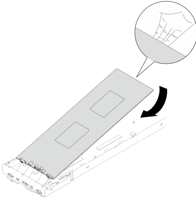
Figure 110. Installation de la carte mère
