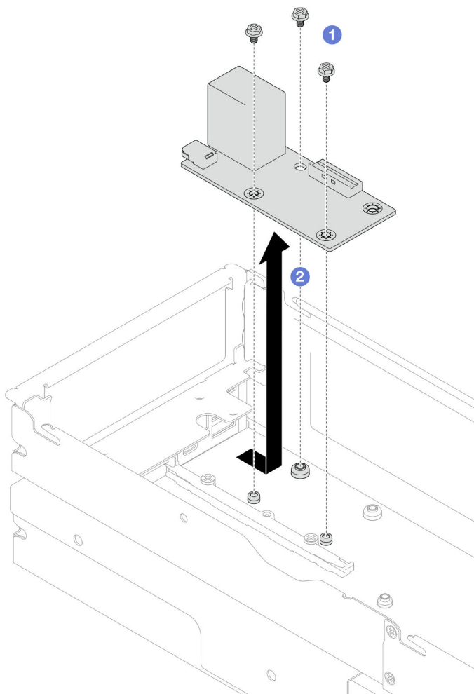
Figure 97. Retrait du module d'E-S arrière
