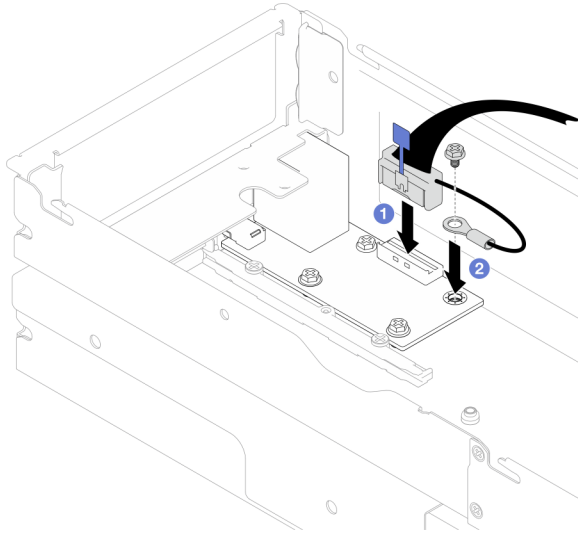
Figure 99. Installation du câble d'E-S arrière et du câble de mise à la terre
