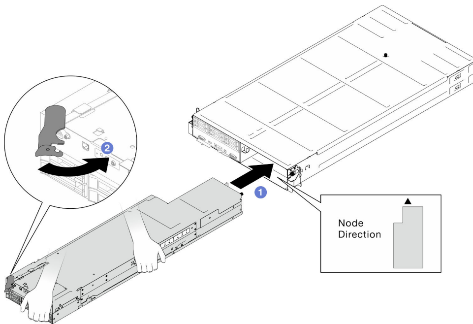
Figure 23. Installation du nœud dans le plateau de droite
