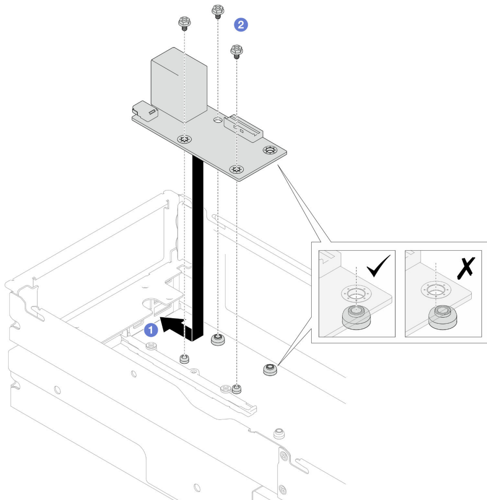
Figure 98. Installation du module d'E-S arrière
