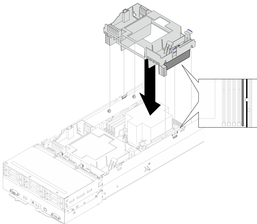
Figure 27. Installation de la grille d'aération arrière
