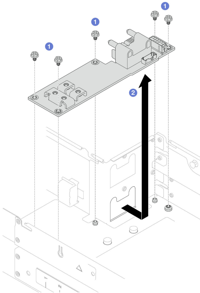
Figure 83. Retrait du tableau de distribution
