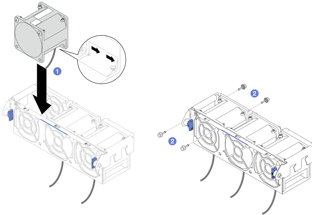
Figure 41. Installation du ventilateur
