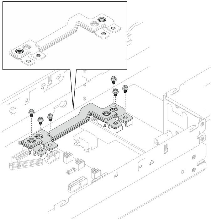
Figure 79. Retrait des vis externes de la barre-bus d'alimentation
