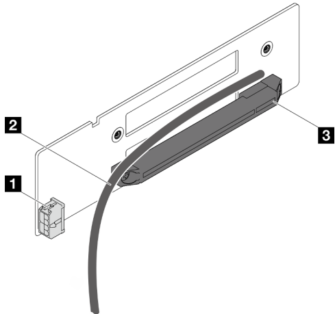
Figure 118. Câble et connecteurs de carte mezzanine PCIe à un emplacement
