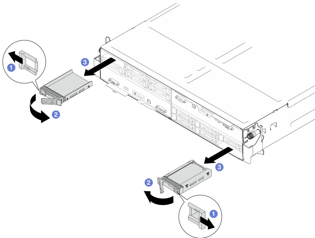
Figure 49. Retrait d'une unité SSD 7 mm
