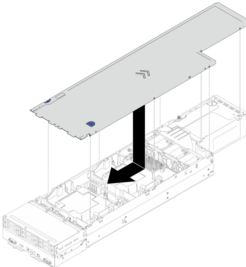
Figure 115. Installation du carter supérieur
