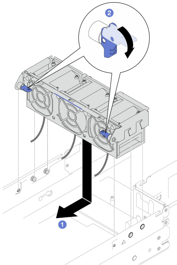
Figure 42. Installation du boîtier de ventilation
