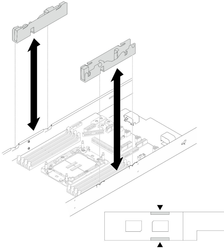
Figure 106. Remplacement d'un conduit de câbles
