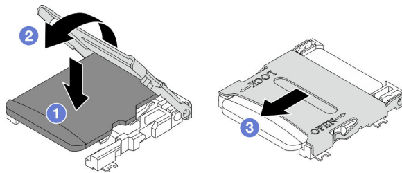
Figure 69. Installation d'une carte MicroSD
