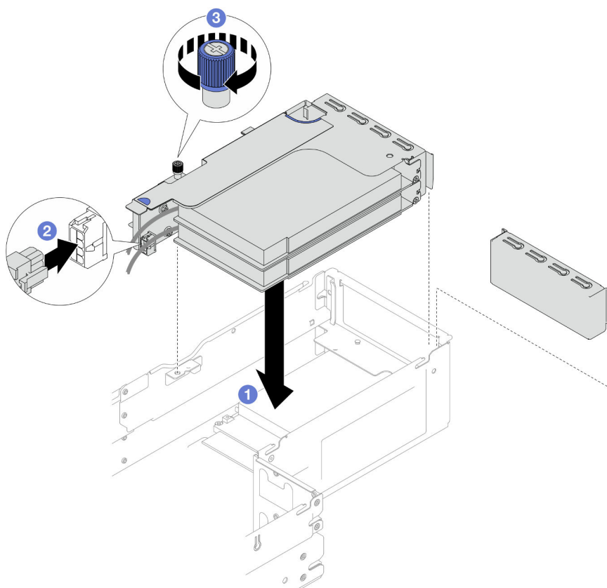
Figure 78. Installation de l'assemblage de cartes mezzanines PCIe
