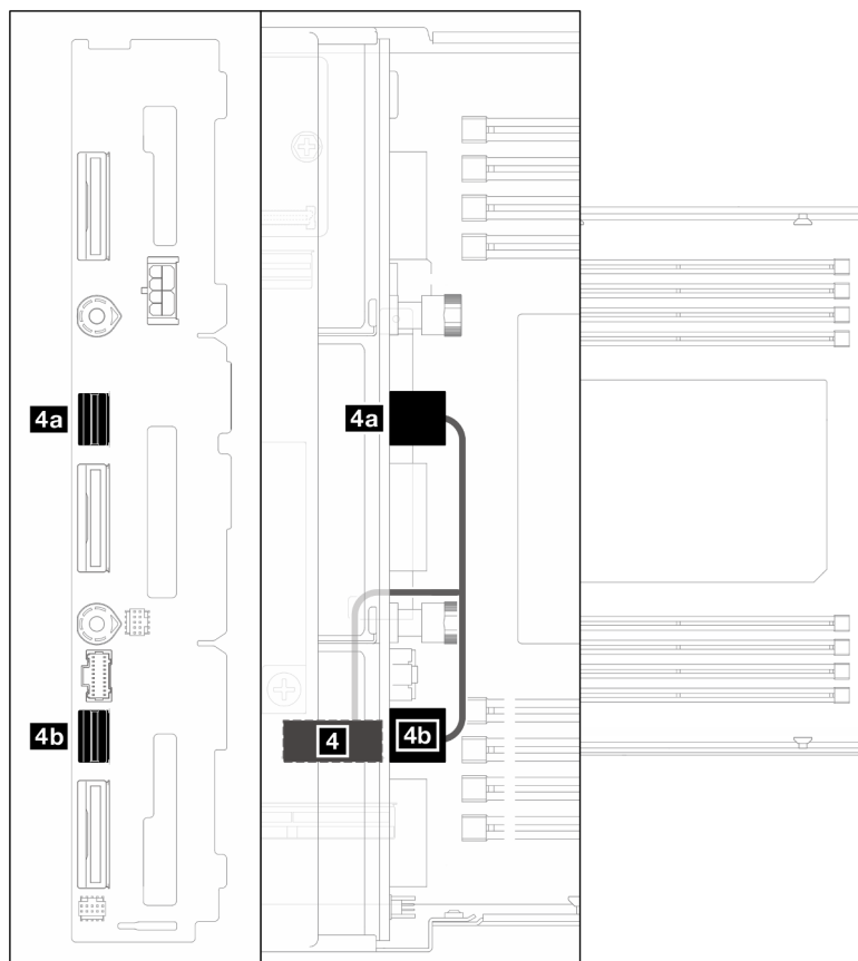
Figure 123. Cheminement des câbles SATA – Configuration sans RAID CFF
