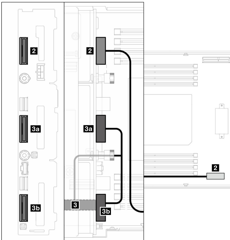
Figure 125. Cheminement des câbles NVMe
