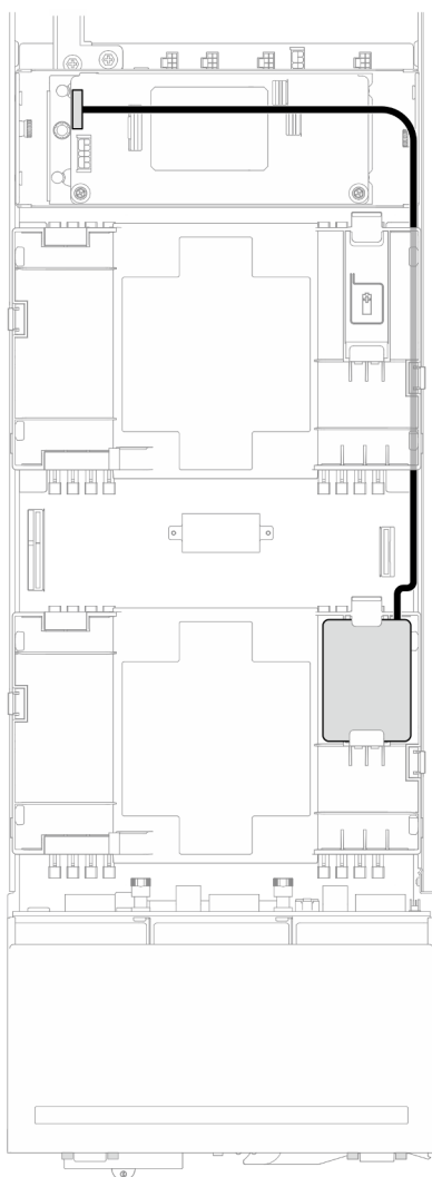
Figure 46. Câble du module d'alimentation flash et RAID CFF
