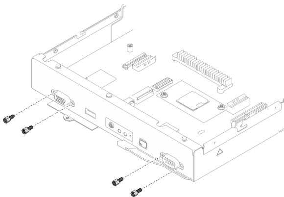
Figure 107. Retrait des vis
