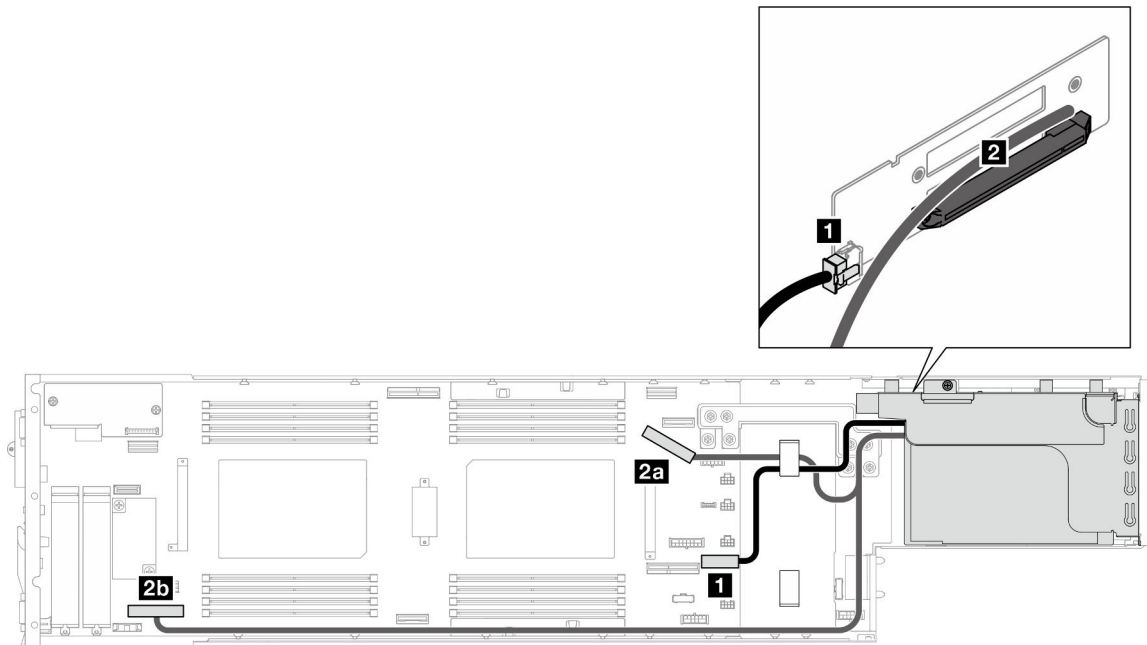
Figure 130. Cheminement des câbles de la carte mezzanine PCIe – un processeur
