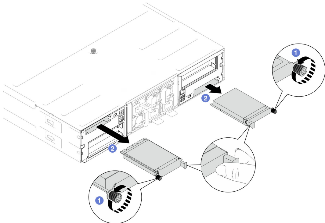
Figure 70. Retrait du module OCP arrière
