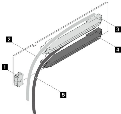
Figure 119. Câbles et connecteurs de carte mezzanine PCIe à deux emplacements
