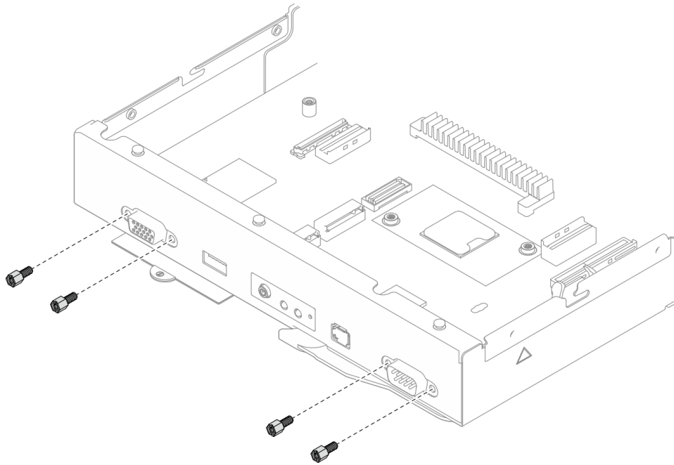
Figure 111. Installation des vis de la carte mère sur le devant
