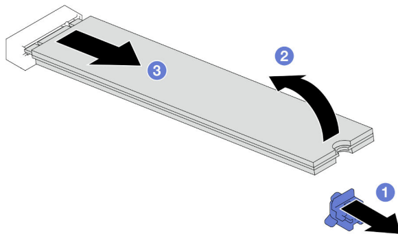
Figure 58. Retrait d'une unité M.2
