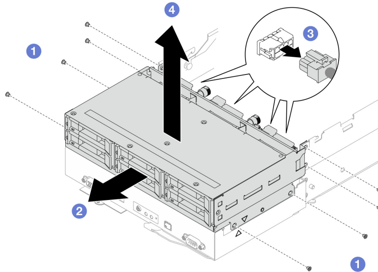
Figure 35. Retrait du bloc boîtier d'unités de disque dur
