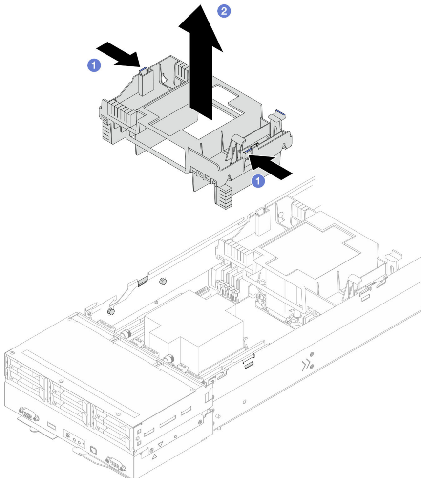
Figure 24. Retrait de grille d'aération avant
