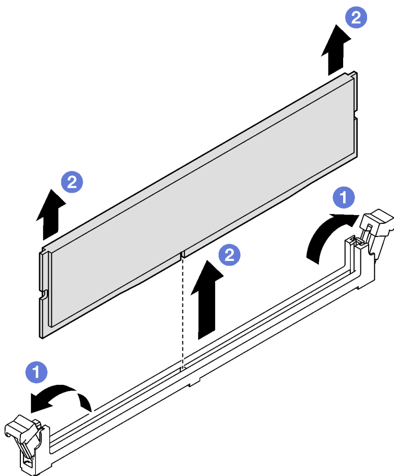
Figure 63. Retrait d'un module de mémoire
