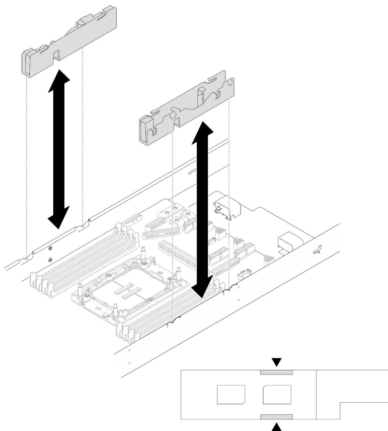
Figure 113. Remplacement d'un conduit de câbles
