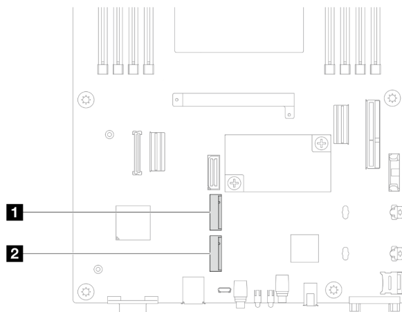
Figure 60. Emplacement des baies M.2 sur la carte mère
