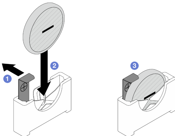
Figure 34. Installation d'une pile CMOS
