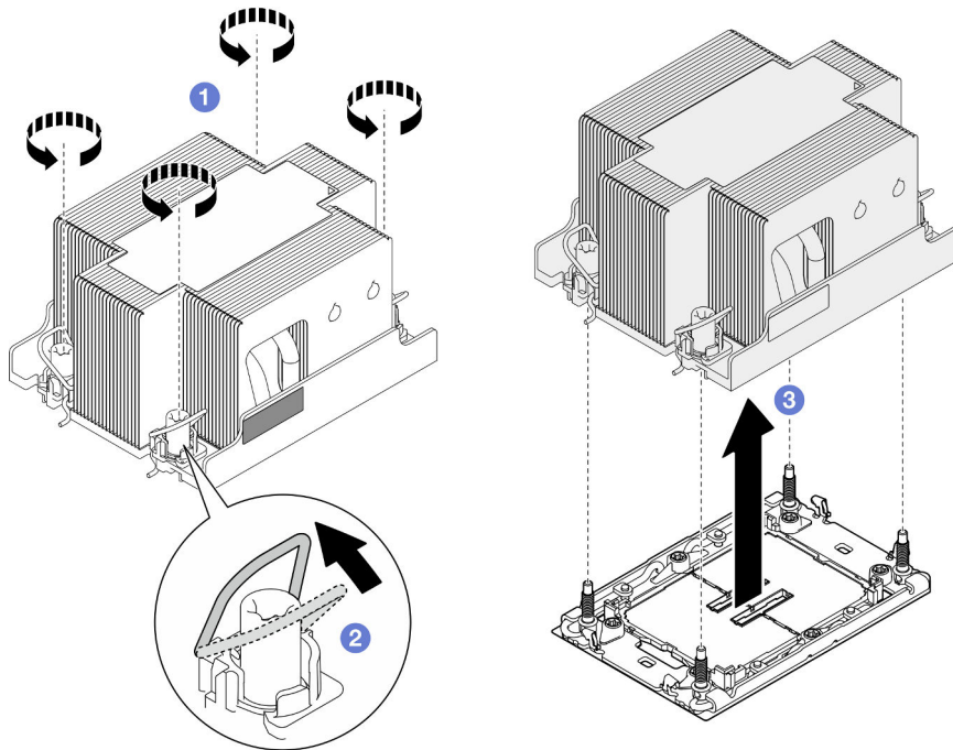
Figure 86. Retrait du PHM standard 2U
