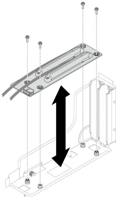
Figure 75. Remplacement de la carte mezzanine PCIe
