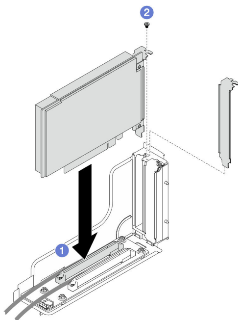
Figure 76. Installation d'un adaptateur PCIe
