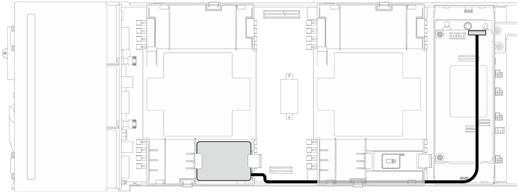
Figure 129. Câble du module d'alimentation flash et RAID CFF
