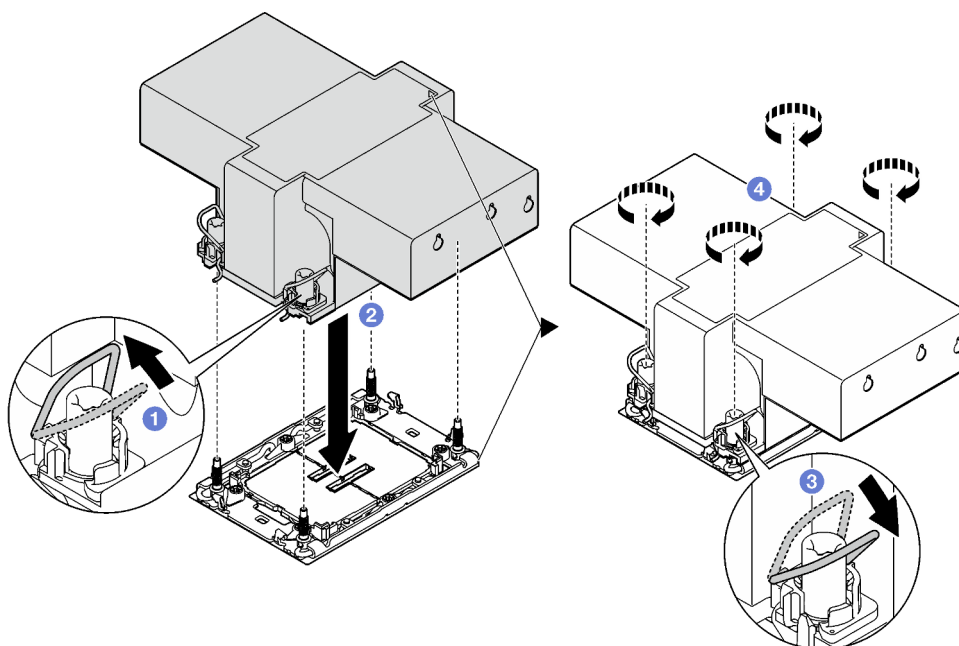
Figure 95. Installation d'un PHM de performances 2U
