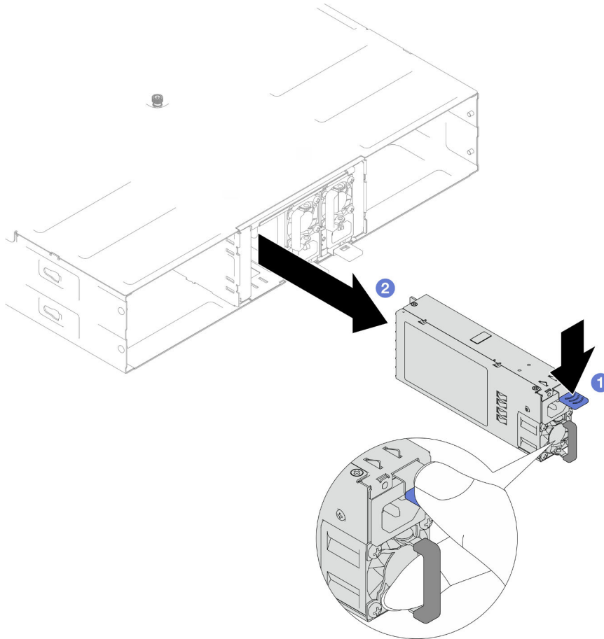
Figure 8. Retrait d'un PSU remplaçable à chaud
