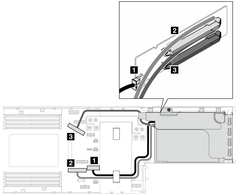
Figure 131. Cheminement des câbles de la carte mezzanine PCIe – deux processeurs
