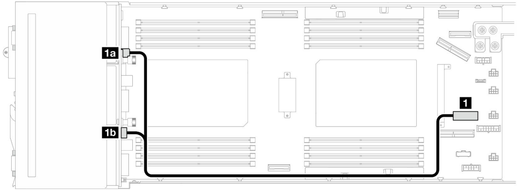
Figure 121. Cheminement des câbles d'alimentation du fond de panier d'unité
