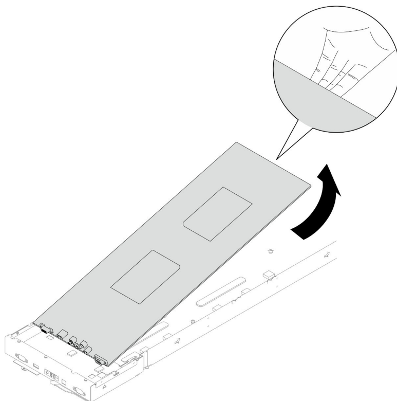
Figure 109. Retrait de la carte mère
