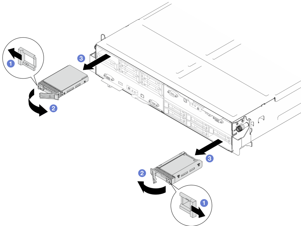
Figure 50. Retrait d'une unité SSD 15 mm
