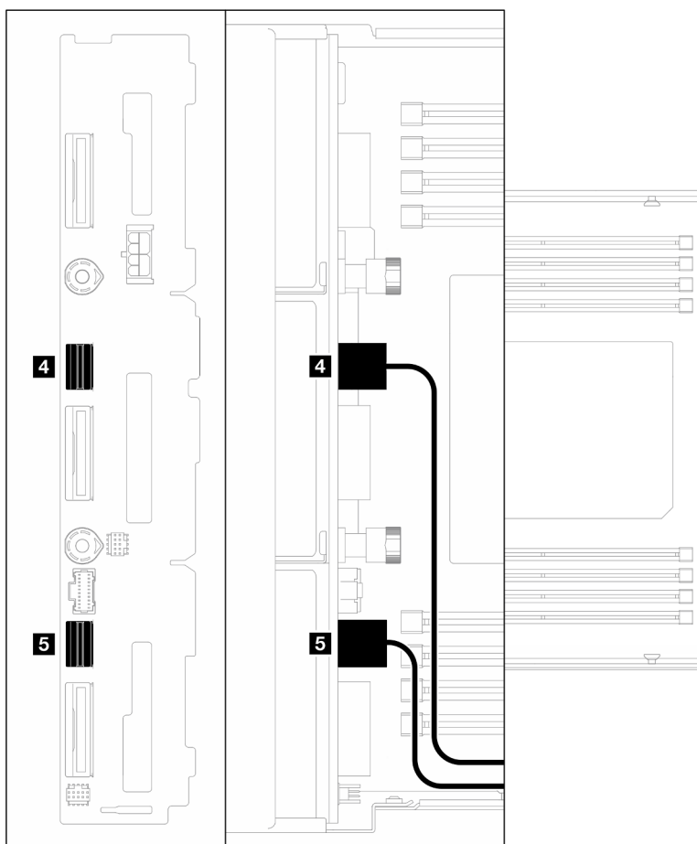
Figure 126. Câbles SATA sur le fond de panier d'unité
