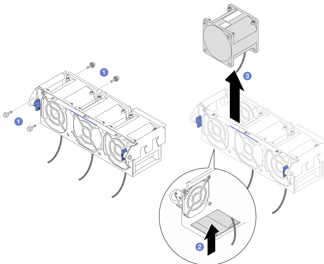
Figure 40. Retrait du ventilateur
