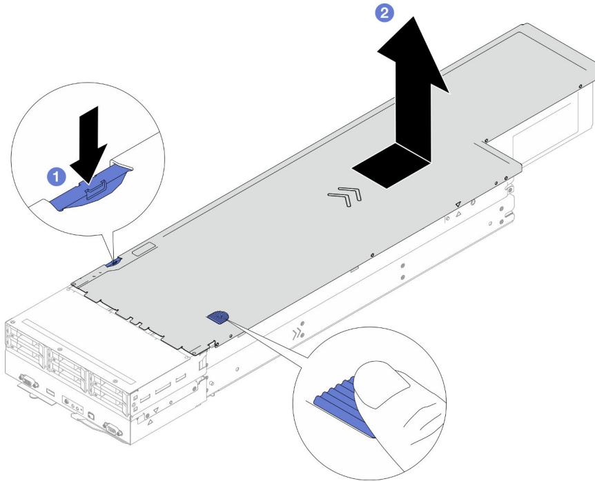
Figure 114. Retrait du carter supérieur
