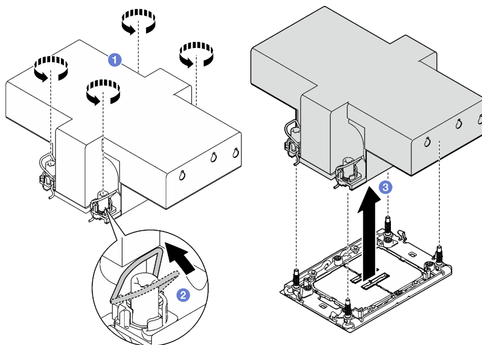
Figure 87. Retrait d'un PHM 2U de performance
