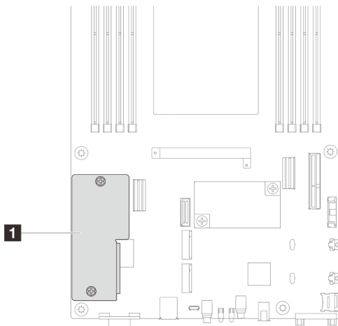
Figure 104. Emplacement du Module de microprogramme et de sécurité RoT
