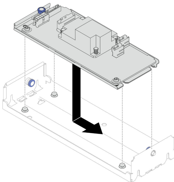
Figure 30. Installation de l'adaptateur RAID CFF interne sur le support
