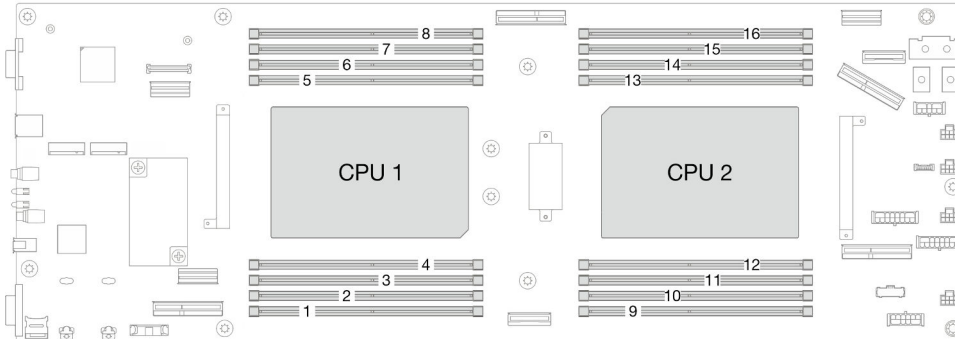
Figure 62. Disposition des modules de mémoire et des processeurs
