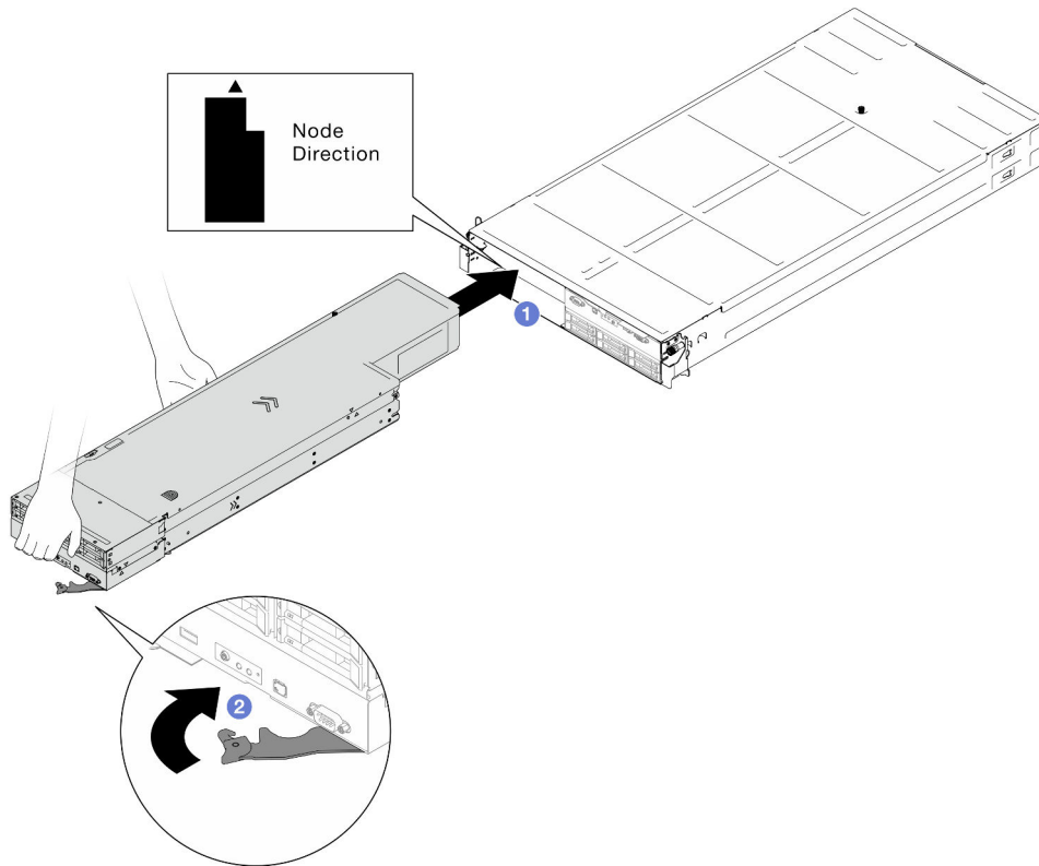
Figure 22. Installation du nœud dans le plateau de gauche
