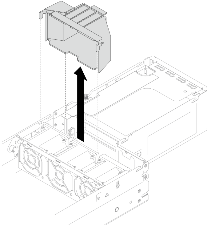
Figure 47. Retrait du conduit de ventilation du GPU
