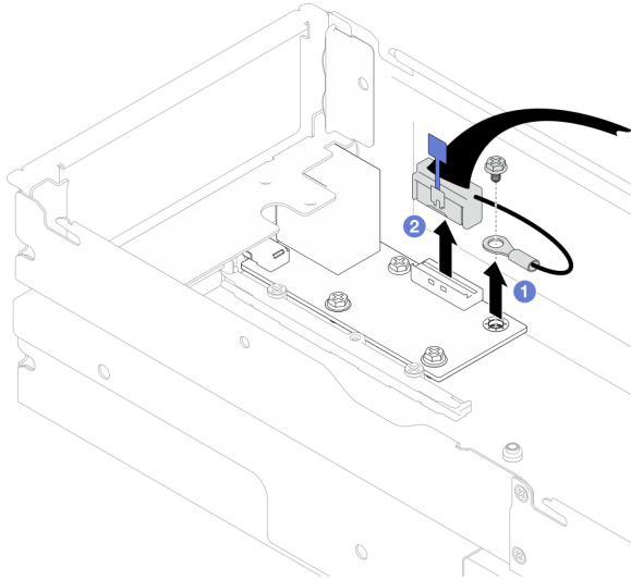
Figure 96. Retrait du câble d'E-S arrière et du câble de mise à la terre
