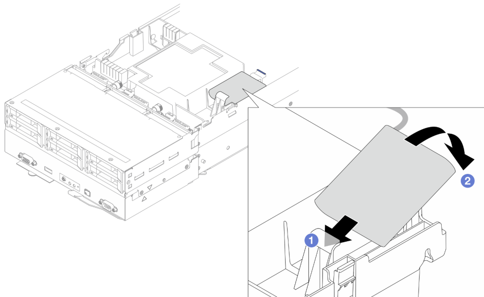
Figure 44. Installation du module d'alimentation flash
