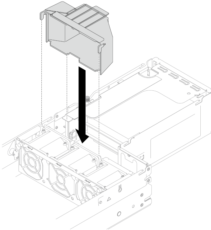
Figure 48. Installation du conduit de ventilation du GPU
