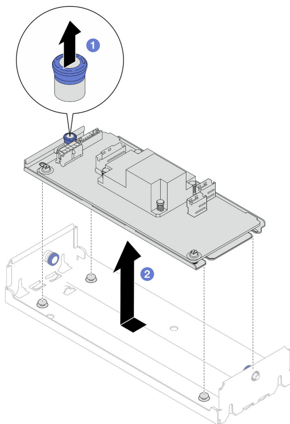
Figure 28. Retrait de l'adaptateur CFF interne
