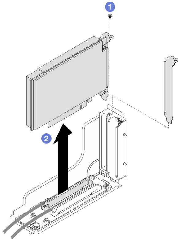
Figure 74. Retrait d'un adaptateur PCIe
