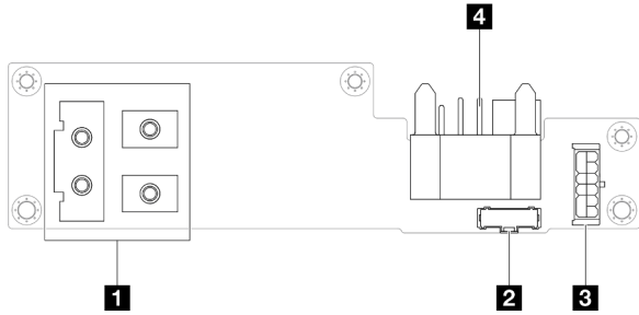
Figure 120. Connecteurs du tableau de distribution
