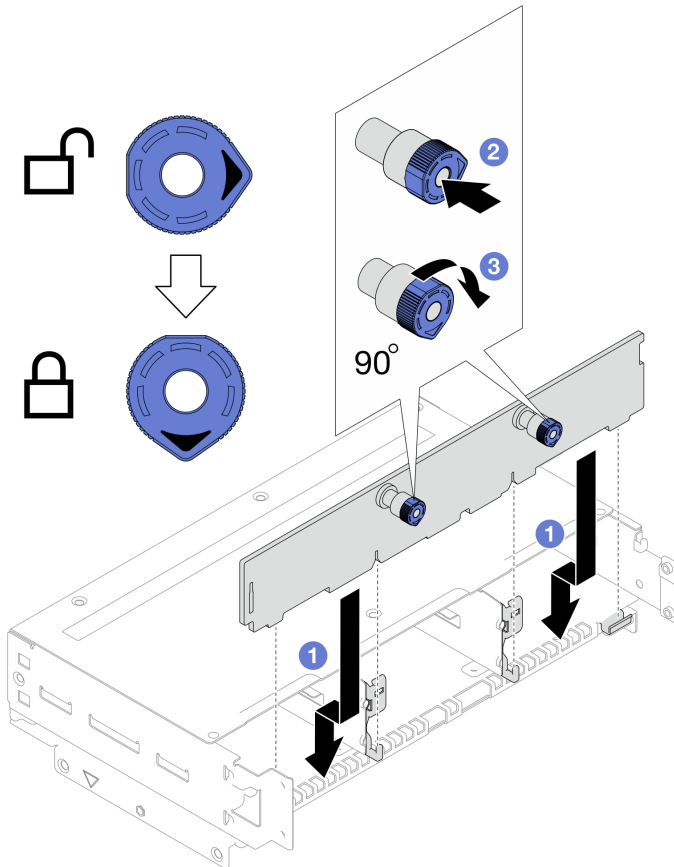
Figure 37. Installation du fond de panier d'unité
