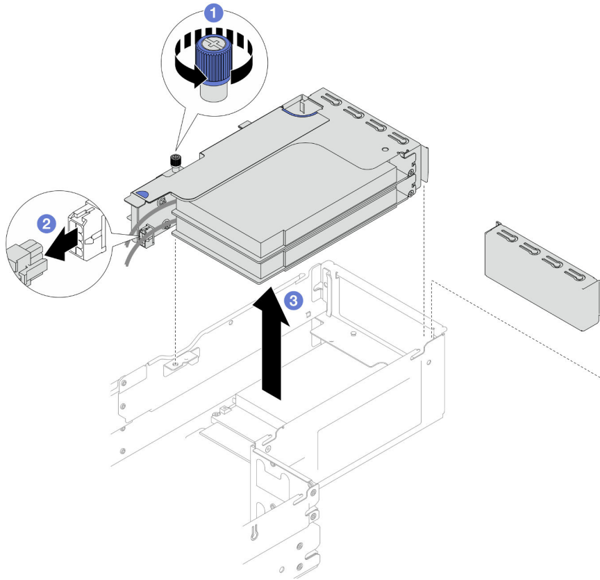
Figure 72. Retrait de l'assemblage de cartes mezzanines PCIe
