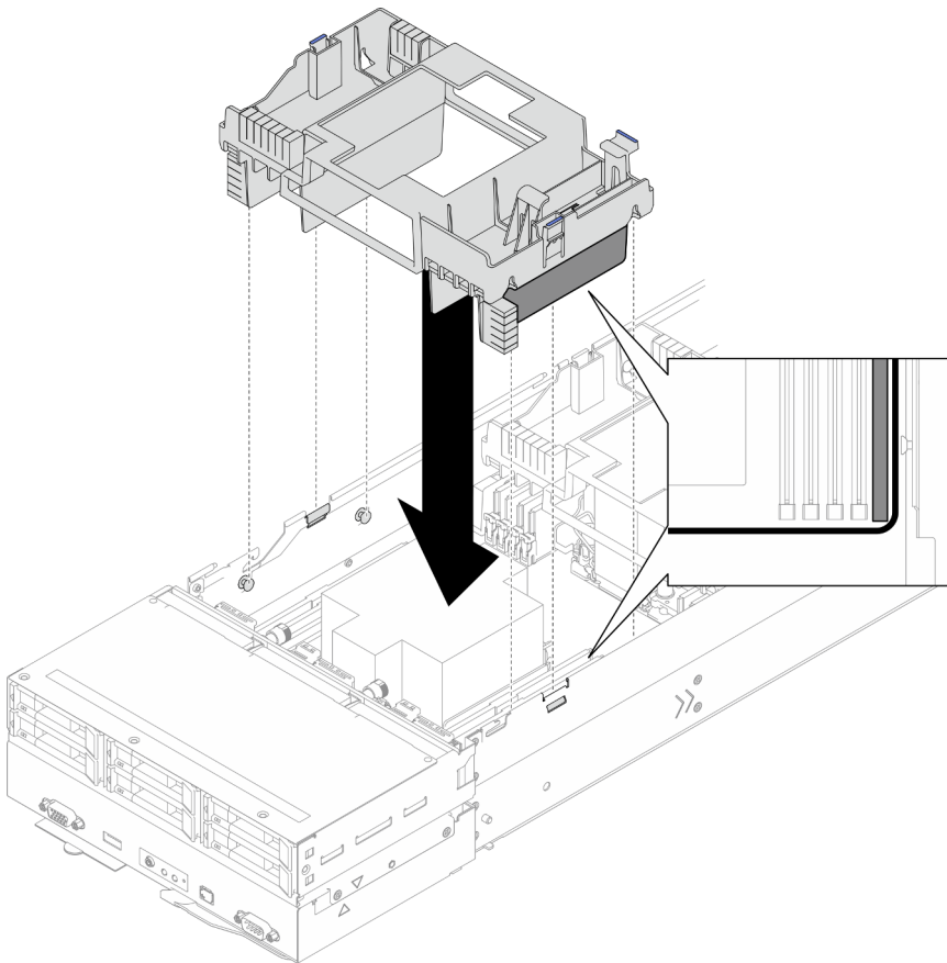
Figure 26. Installation de la grille d'aération avant
