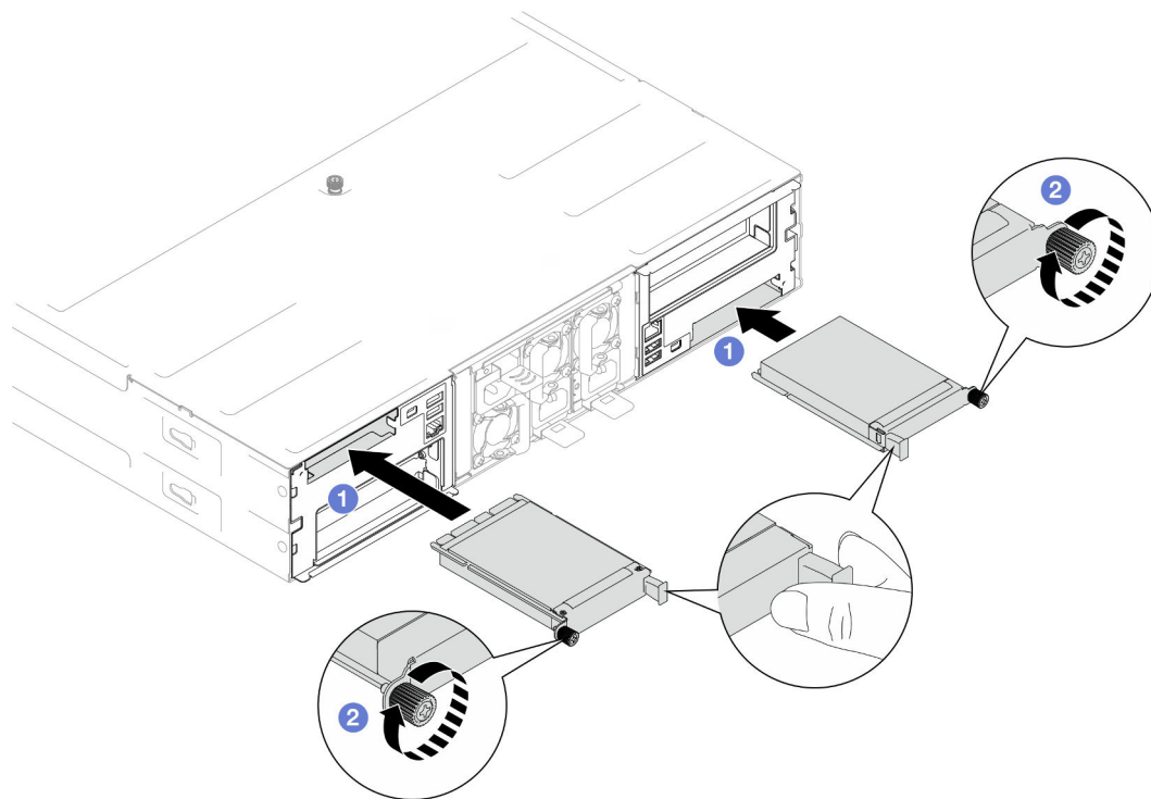
Figure 71. Installation du module OCP arrière
