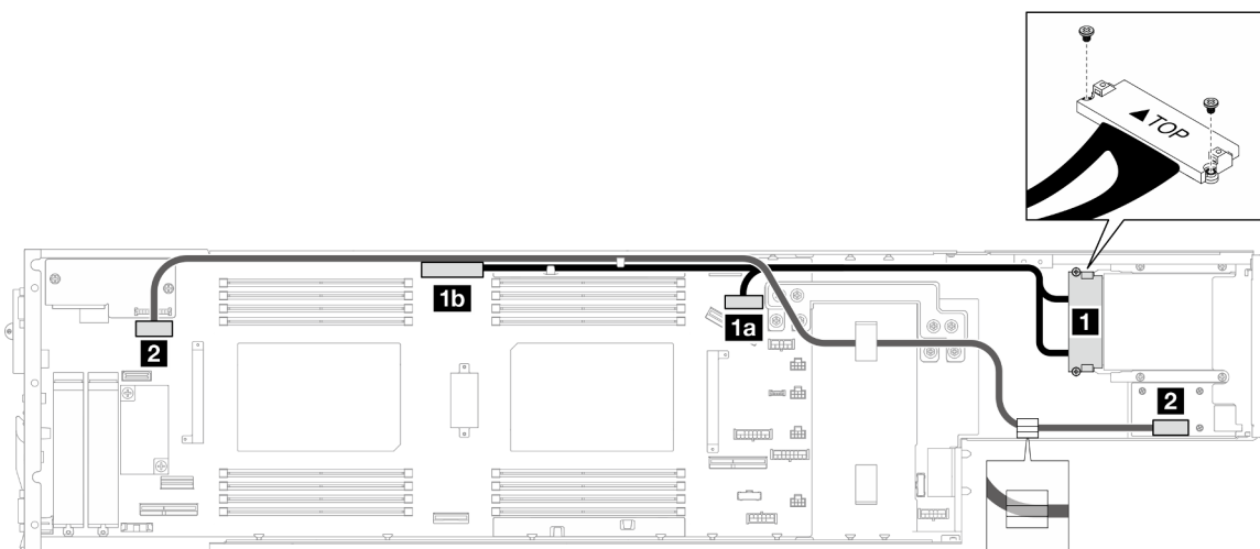
Figure 133. Câbles pour le module OCP et d'E-S arrière
