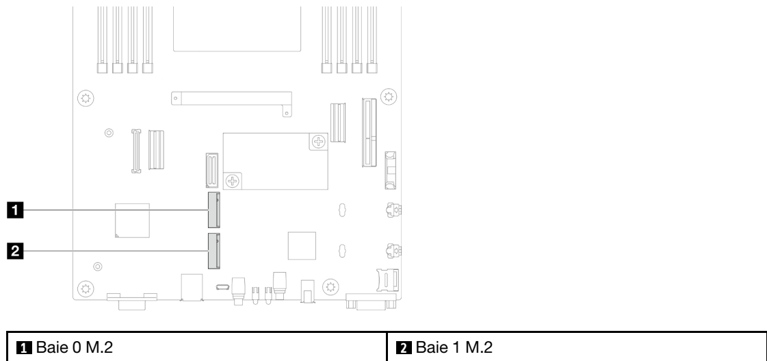
Figure 57. Emplacement des baies M.2 sur la carte mère
