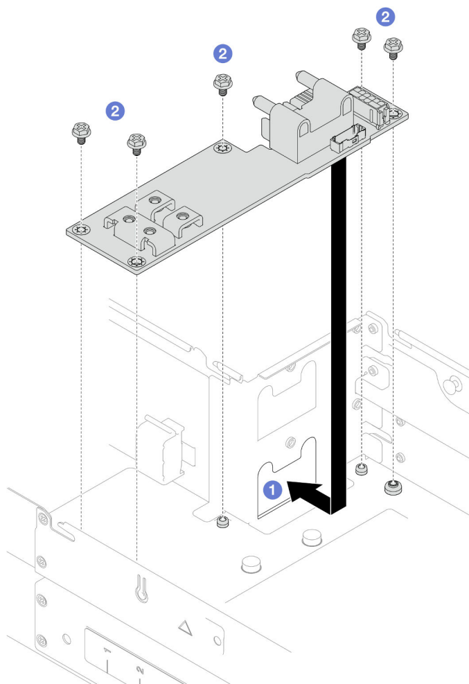
Figure 84. Installation du tableau de distribution
