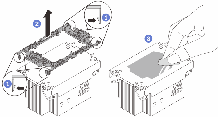
Figure 89. Dissociation d'un support de processeur du dissipateur thermique
