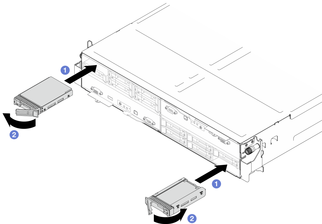
Figure 53. Installation d'un disque SSD 7 mm
