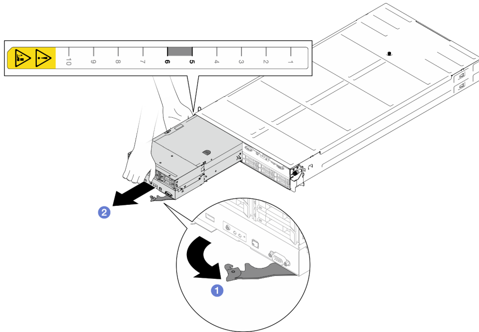
Figure 16. Retrait du nœud du plateau de gauche
