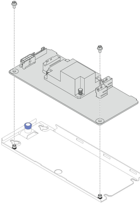
Figure 29. Séparation de l'adaptateur RAID CFF interne du plateau
