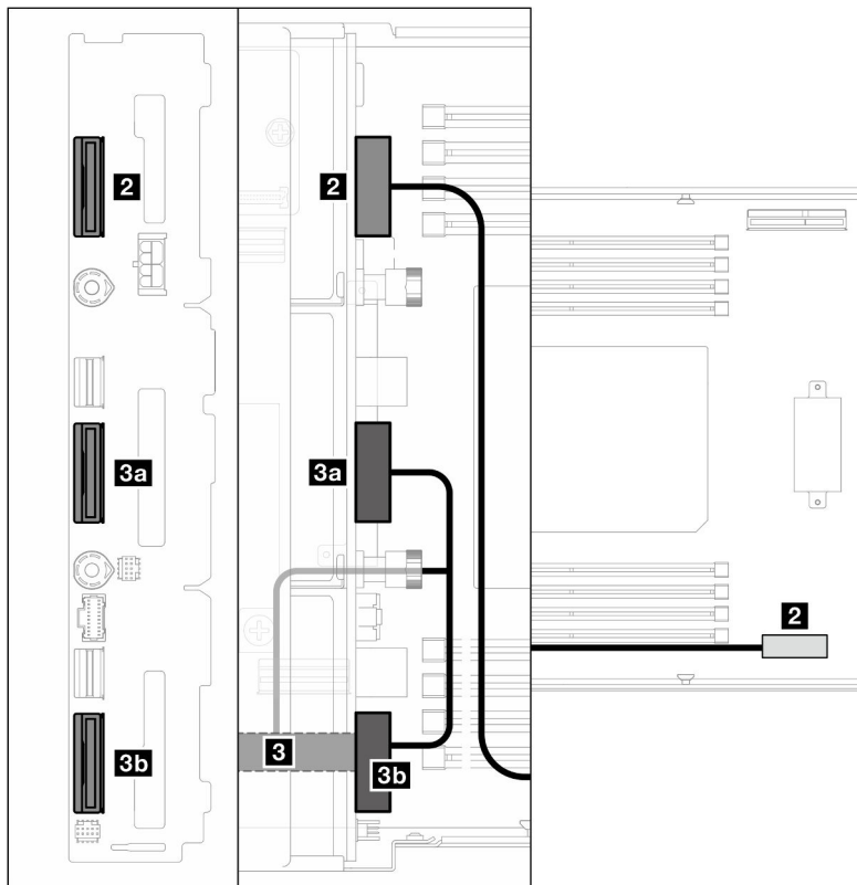
Figure 122. Cheminement des câbles NVMe
