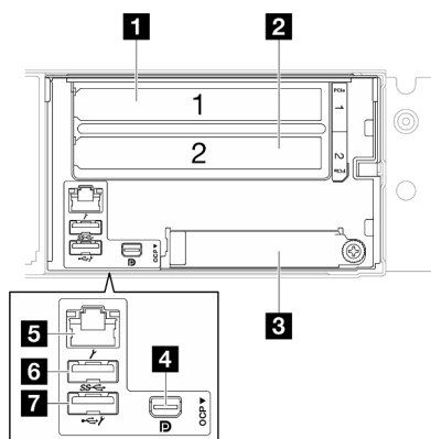
Figura 4. Vista posteriore del nodo ThinkSystem SD550 V3
