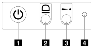
Figura 11. Pulsanti e LED sul pannello anteriore dell'operatore
