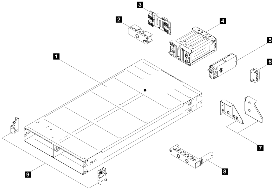
Figura 15. Componenti dello chassis
