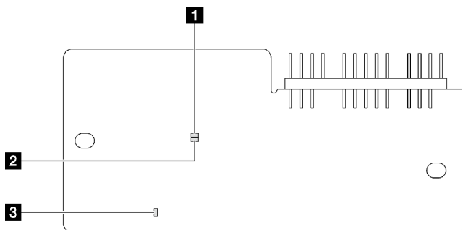
Figura 13. LED sul modulo firmware e sicurezza RoT
