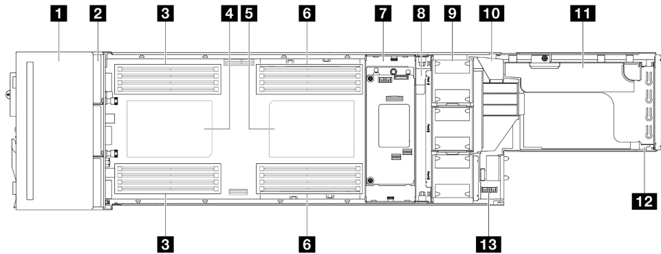
Figura 7. Vista superiore di SD550 V3
