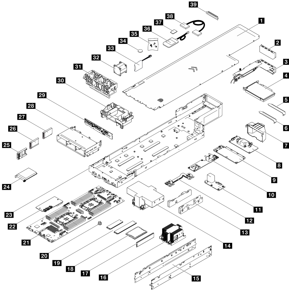
Figura 16. Componenti del nodo
