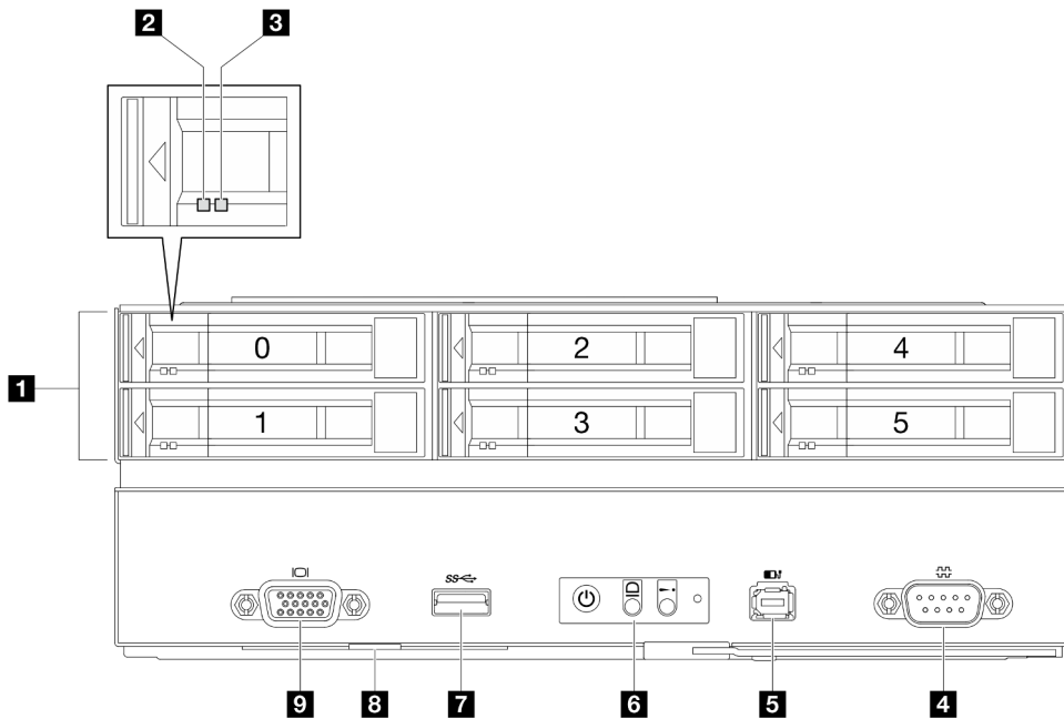
Figura 2. Configurazione con massimo sei unità da 2,5"
