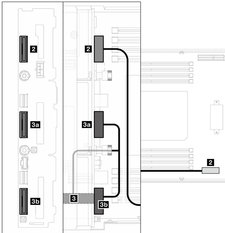
Figura 136. Instradamento dei cavi NVMe
