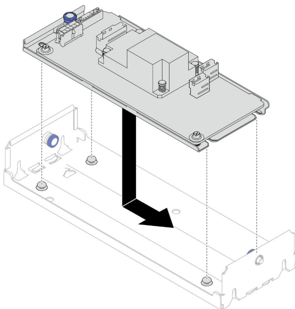
Figura 44. Installazione dell'adattatore RAID CFF interno sulla staffa
