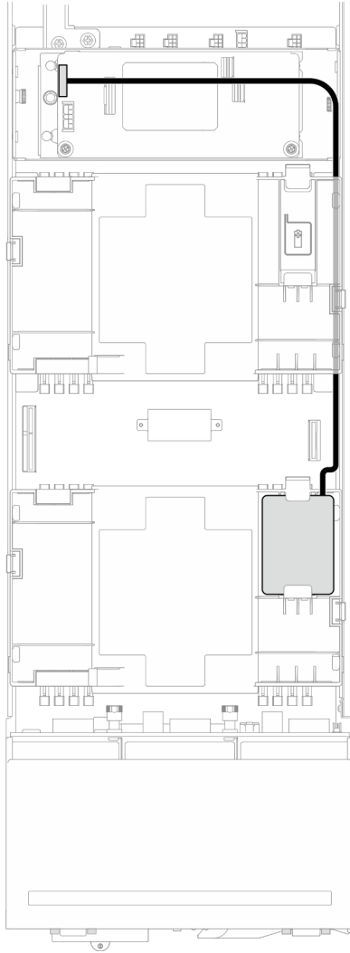
Figura 60. Cavo del modulo di alimentazione flash e RAID CFF
