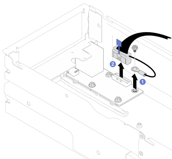
Figura 110. Rimozione del cavo I/O posteriore e del cavo di messa a terra
