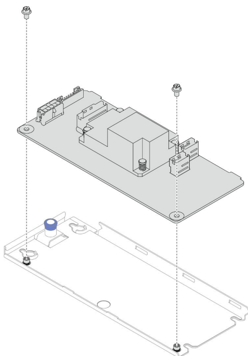
Figura 43. Separazione dell'adattatore RAID CFF interno dal vassoio
