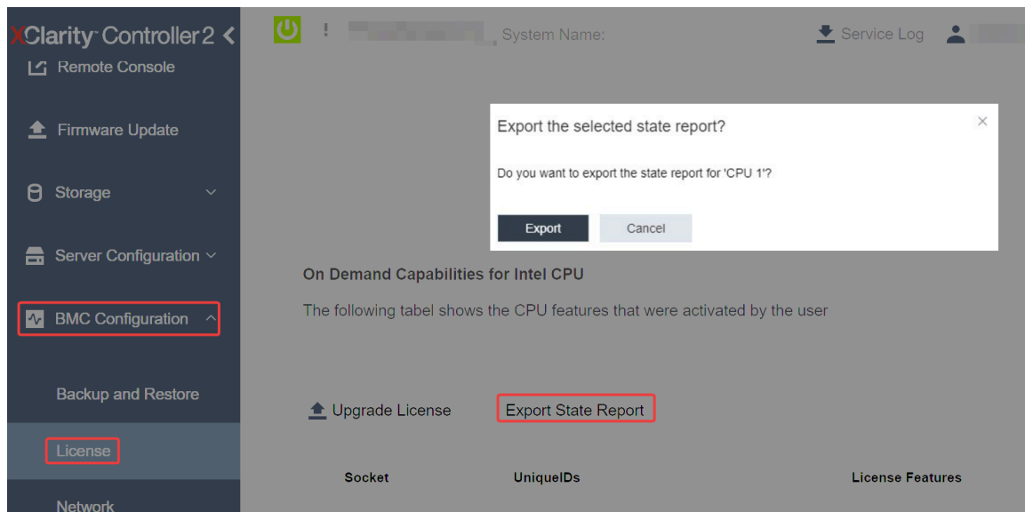
Figura 152. Esportare il report sullo stato tramite la GUI Web di XCC
