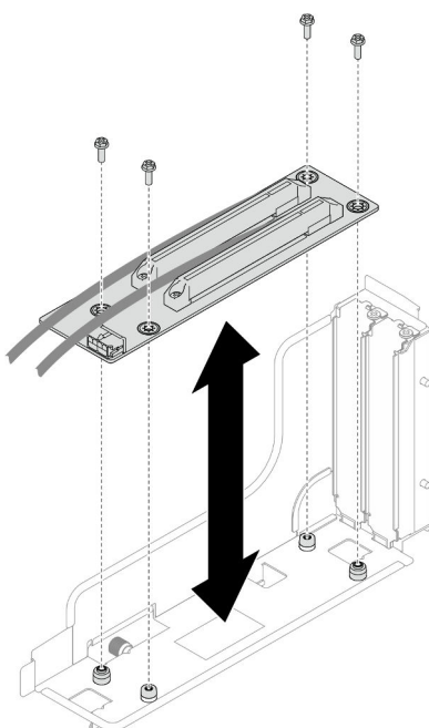
Figura 87. Sostituzione della scheda verticale PCIe
