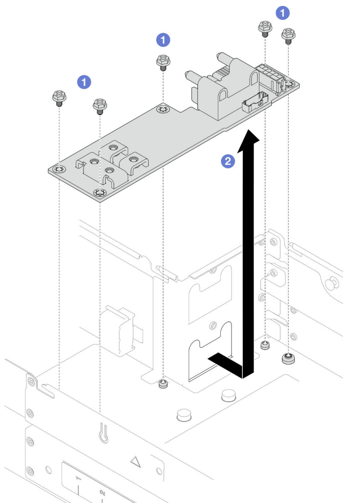
Figura 97. Rimozione della scheda di distribuzione dell'alimentazione
