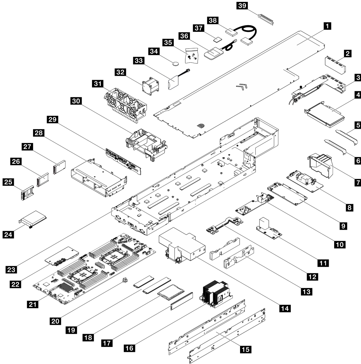
Figura 11. Componenti del nodo
