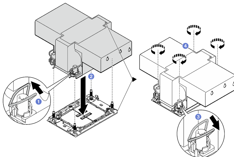
Figura 109. Installazione di un PHM 2U ad alte prestazioni
