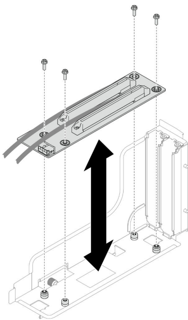
Figura 89. Sostituzione della scheda verticale PCIe
