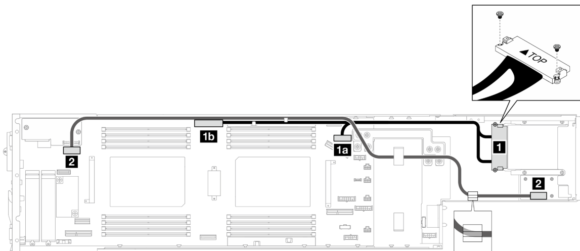
Figura 147. Cavi per i moduli I/O posteriore e OCP
