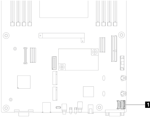
Figura 82. Posizione del socket MicroSD
