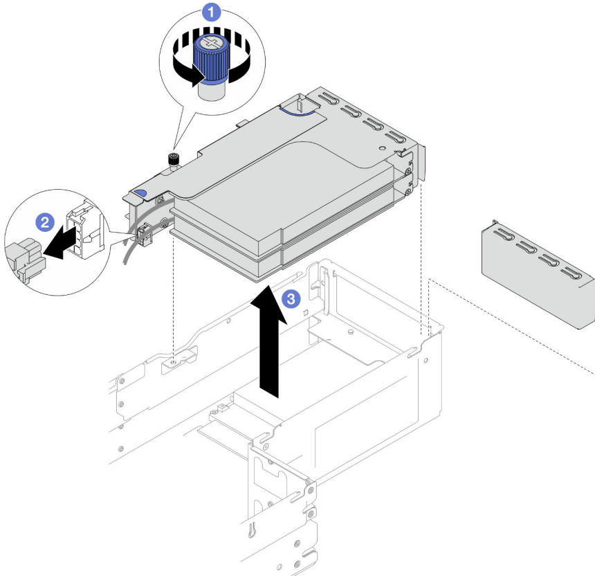
Figura 86. Rimozione dell'assieme verticale PCIe
