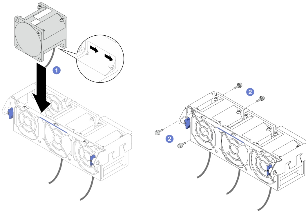
Figura 55. Installazione delle ventole
