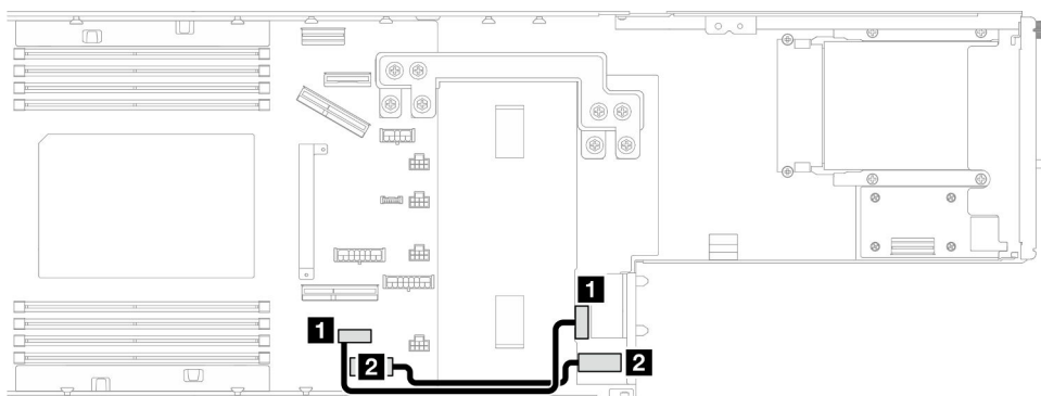
Figura 146. Instradamento dei cavi per la scheda di distribuzione dell'alimentazione
