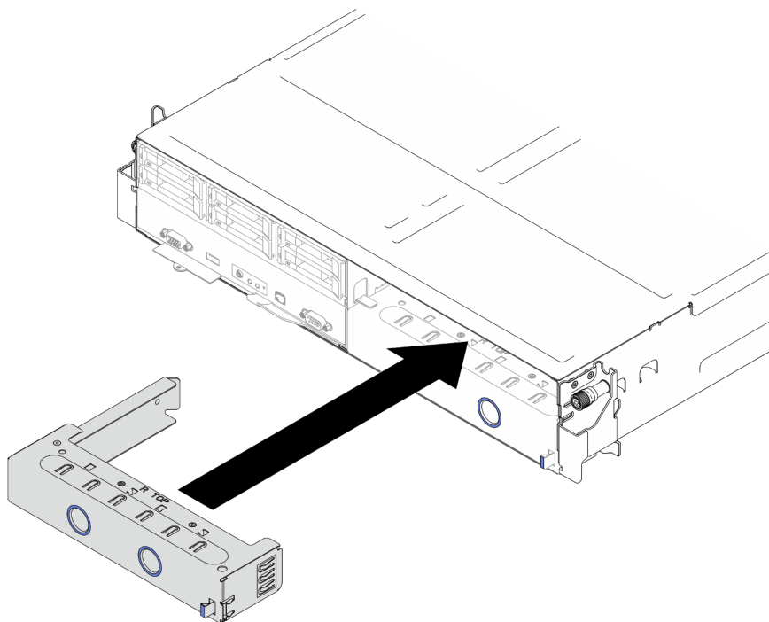
Figura 32. Installazione di un elemento di riempimento del vassoio del nodo anteriore
