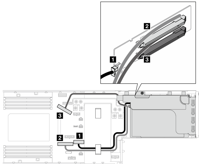
Figura 145. Instradamento dei cavi delle schede verticali PCIe – due processori
