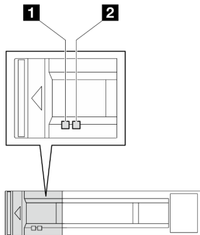
Figura 156. LED dell'unità da 2,5"
