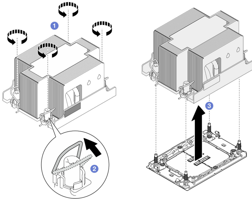
Figura 100. Rimozione del PHM 2U standard
