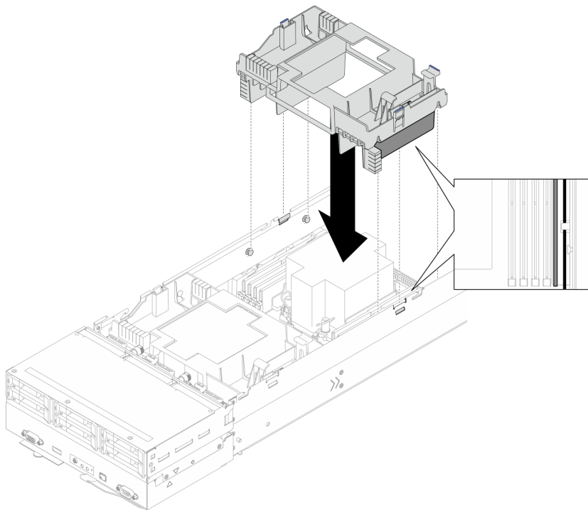
Figura 41. Installazione del deflettore d'aria posteriore
