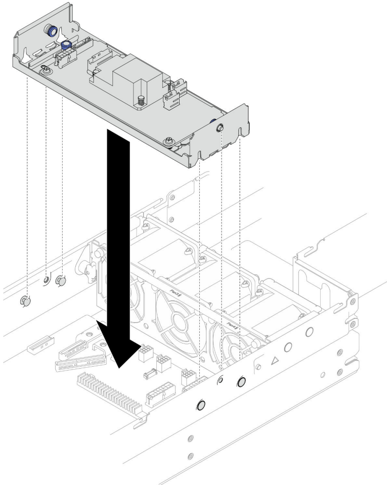
Figura 70. Installazione della staffa dell'adattatore interno
