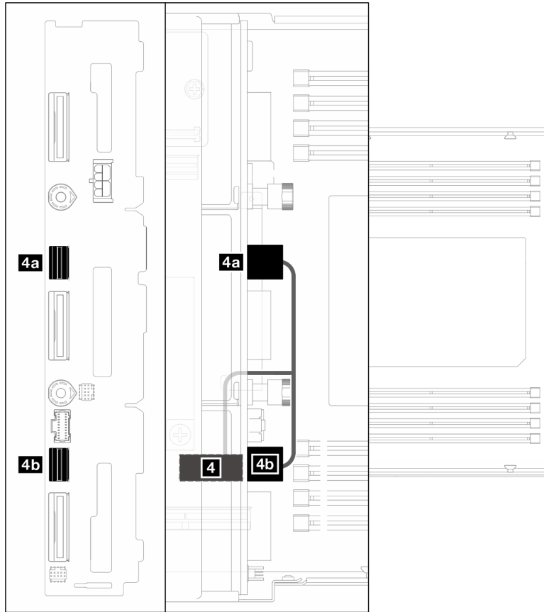
Figura 137. Instradamento dei cavi SATA - Configurazione senza RAID CFF
