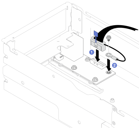
Figura 113. Installazione del cavo I/O posteriore e del cavo di messa a terra
