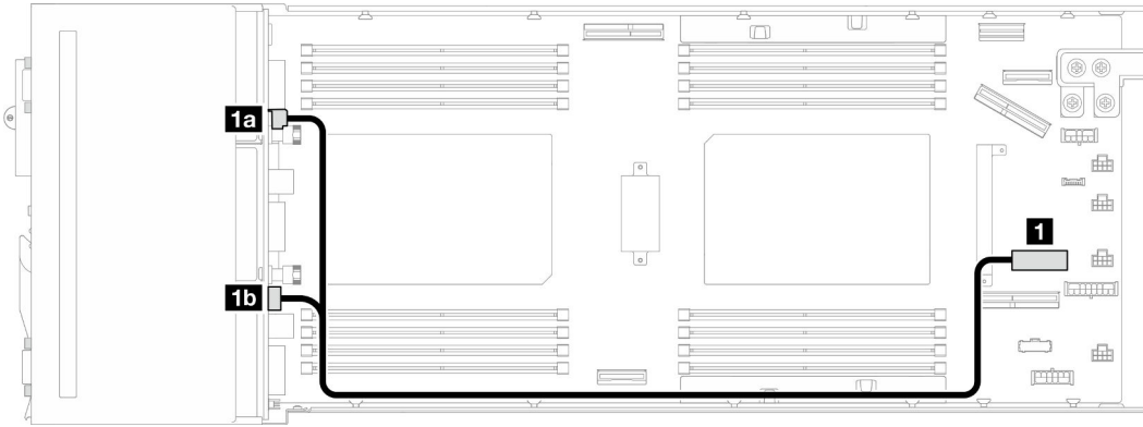
Figura 138. Instradamento dei cavi di alimentazione del backplane dell'unità
