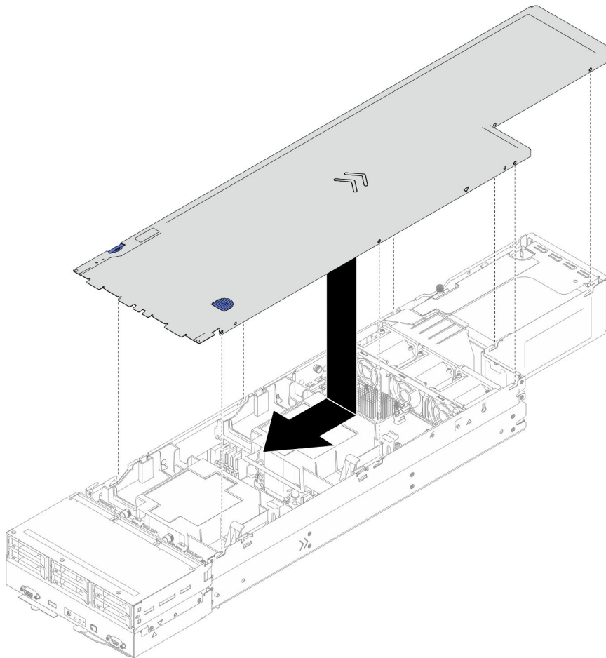
Figura 129. Installazione del coperchio superiore
