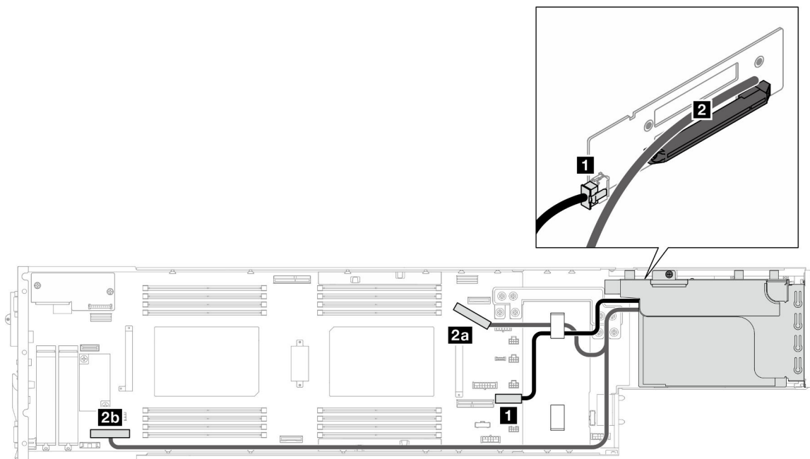
Figura 144. Instradamento dei cavi delle schede verticali PCIe – un processore
