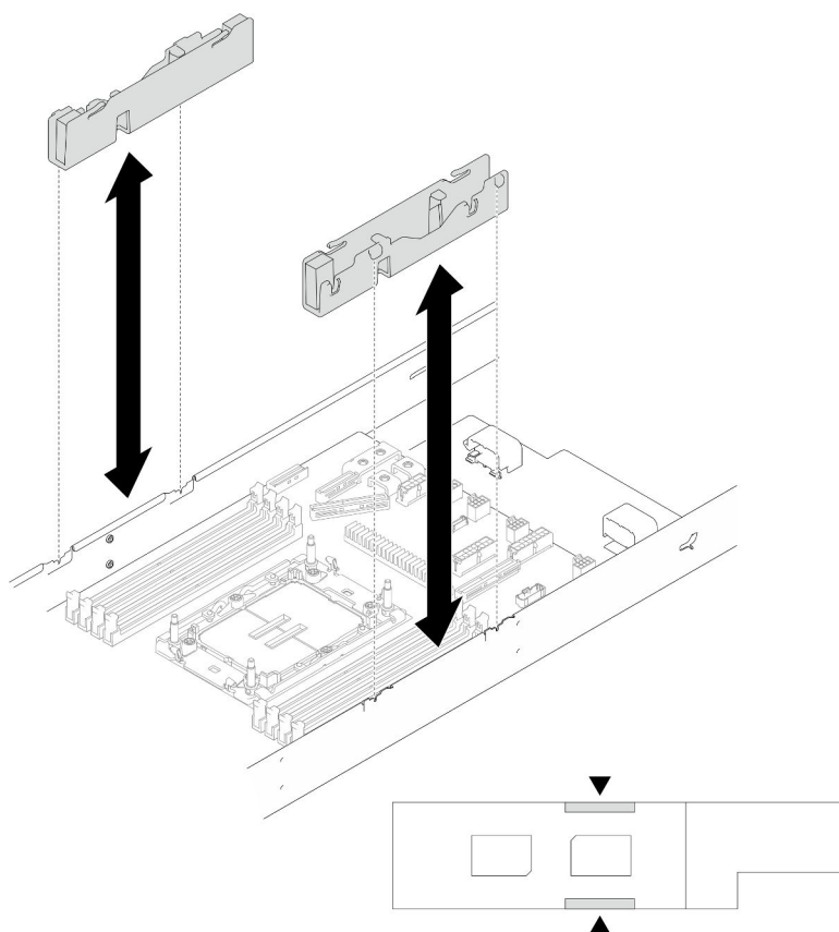
Figura 127. Sostituzione dei condotti dei cavi
