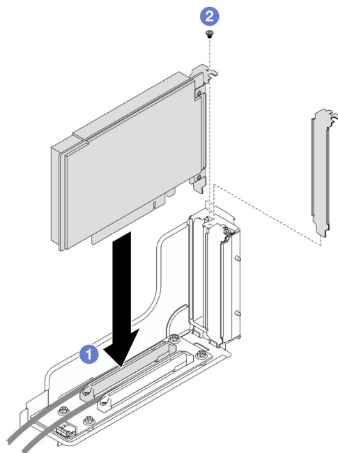
Figura 90. Installazione di un adattatore PCIe
