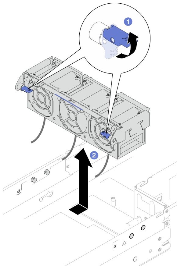
Figura 53. Rimozione dell'alloggiamento della ventola
