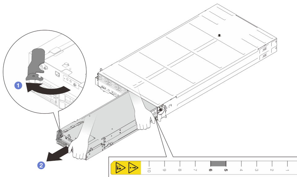
Figura 31. Rimozione del nodo dal vassoio destro
