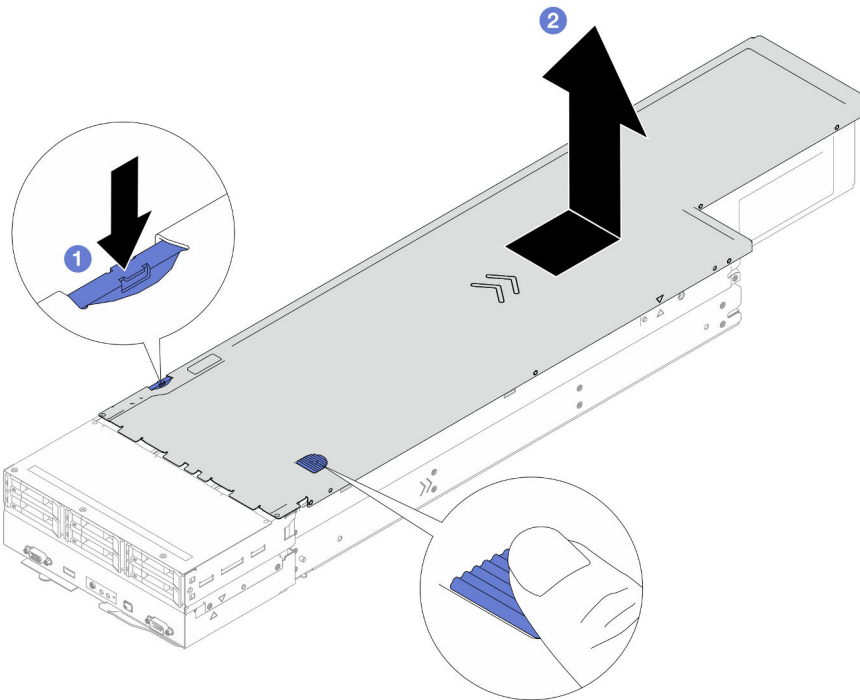
Figura 128. Rimozione del coperchio superiore
