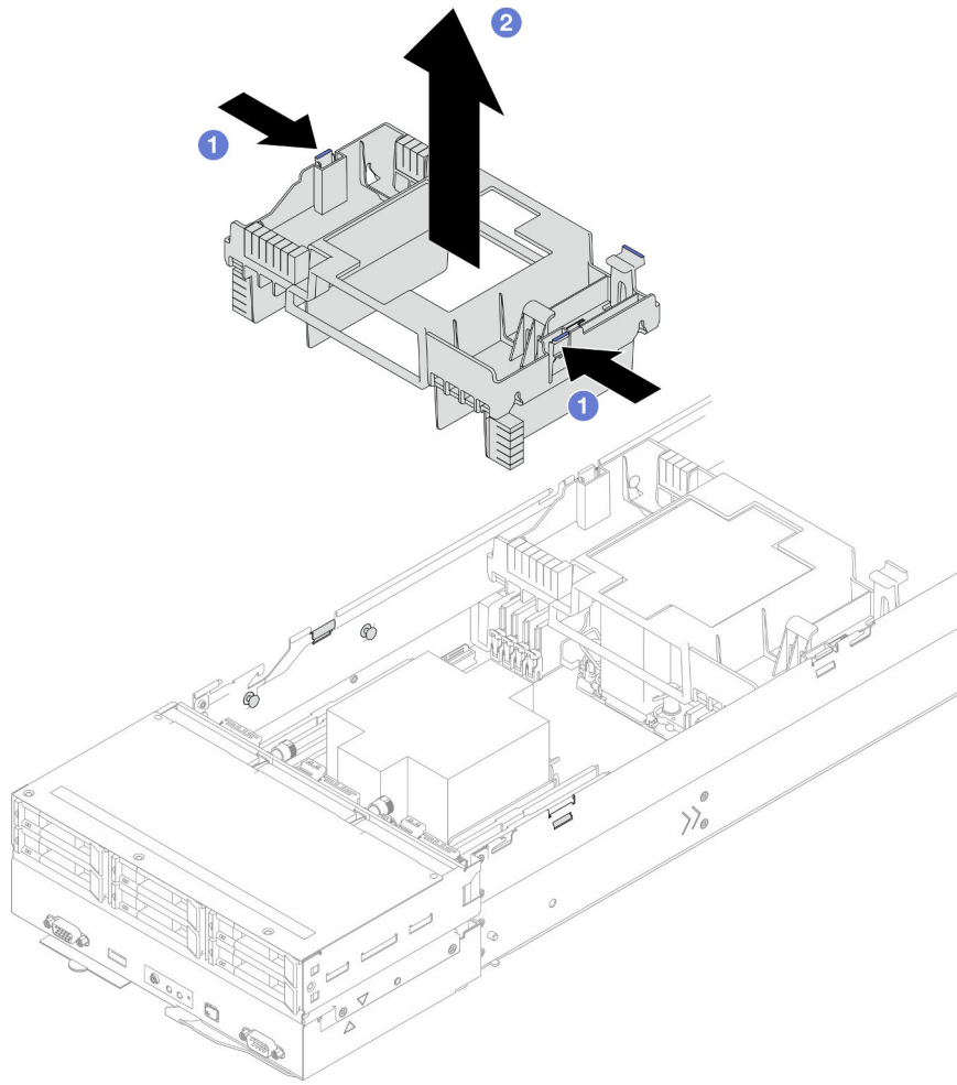
Figura 38. Rimozione del deflettore d'aria anteriore
