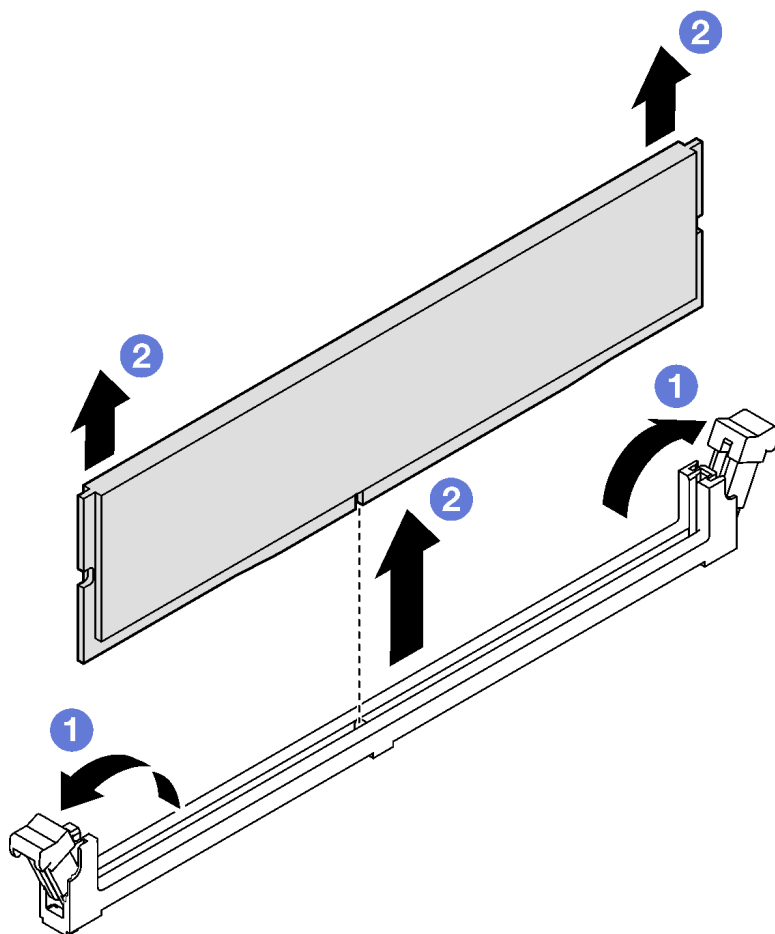
Figura 77. Rimozione di un modulo di memoria
