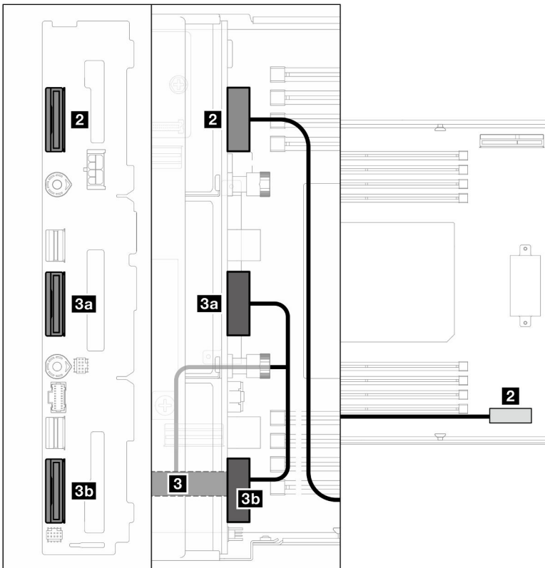
Figura 139. Instradamento dei cavi NVMe
