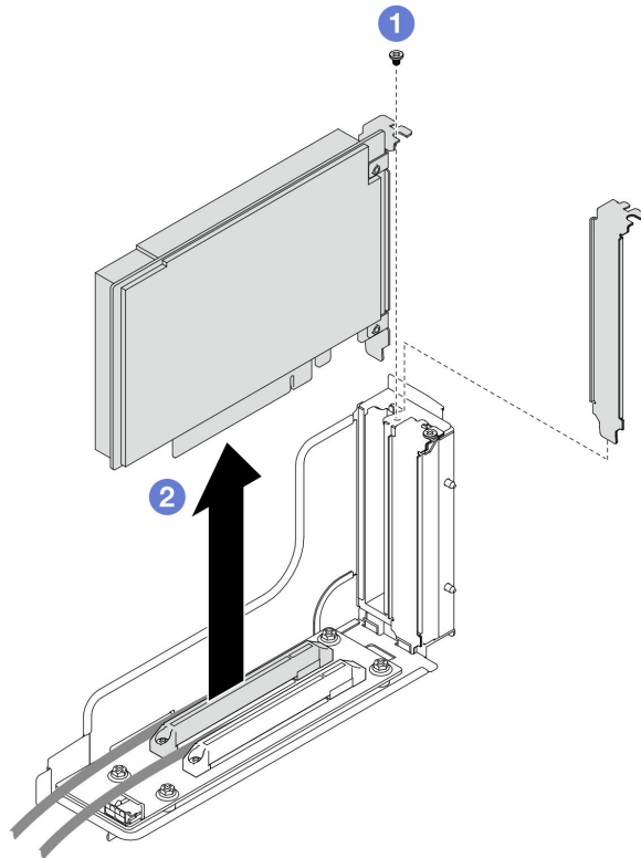
Figura 88. Rimozione di un adattatore PCIe
