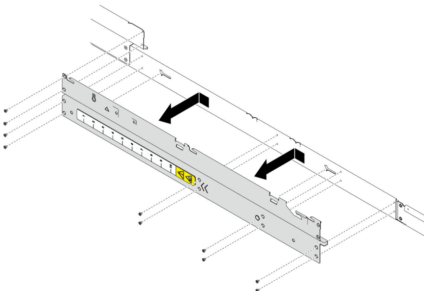
Figura 114. Rimozione della staffa laterale
