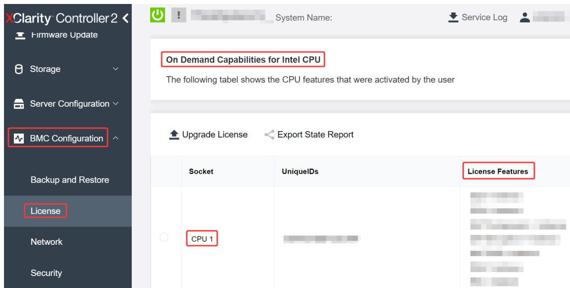
Figura 153. Verifica delle funzioni Intel On Demand installate in un processore nella GUI Web di XCC
