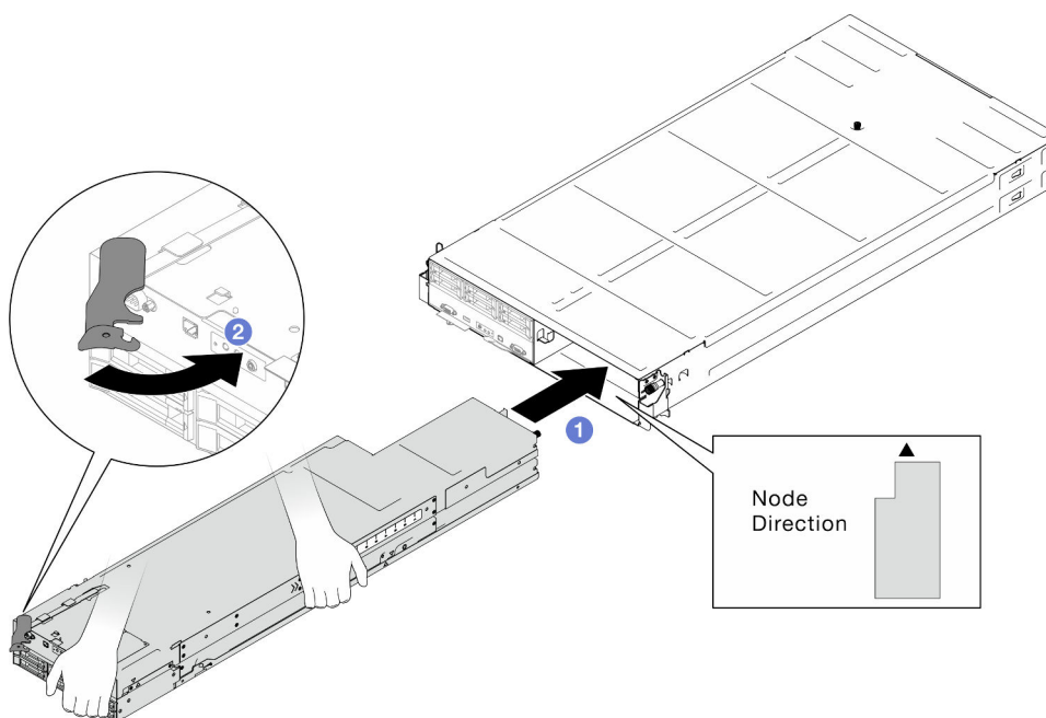
Figura 37. Installazione del nodo nel vassoio destro
