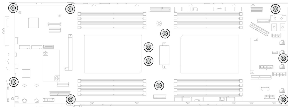
Figura 126. Installazione delle viti sulla scheda di sistema
