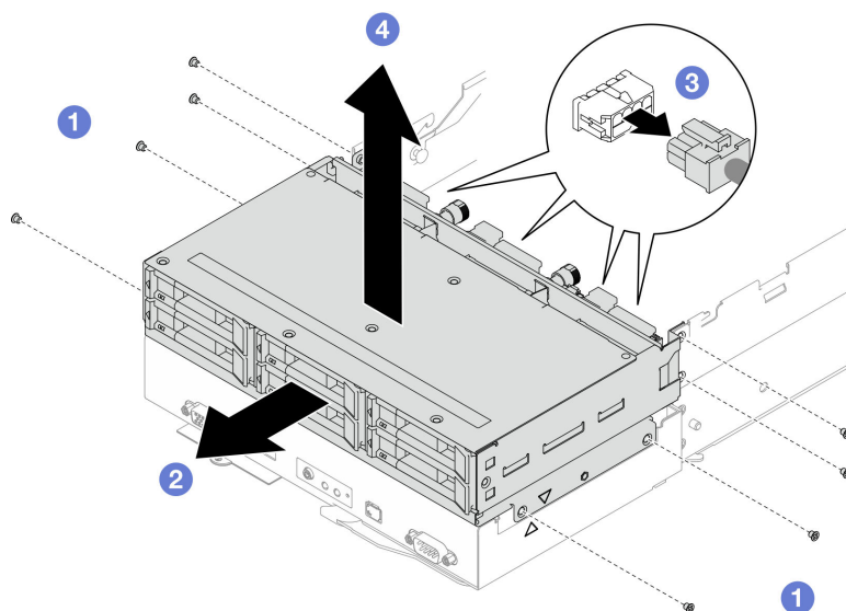
Figura 49. Rimozione dell'assieme del telaio unità
