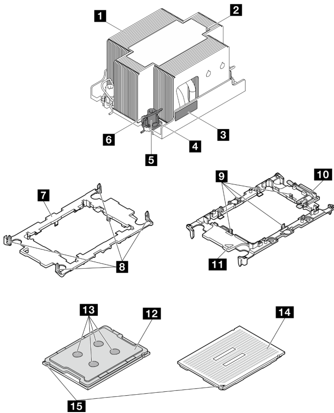
Figura 104. Componenti del PHM
