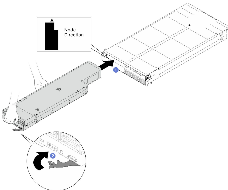
Figura 36. Installazione del nodo nel vassoio sinistro
