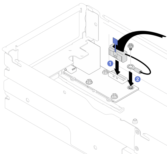
Figura 148. Installazione del cavo I/O posteriore e del cavo di messa a terra
