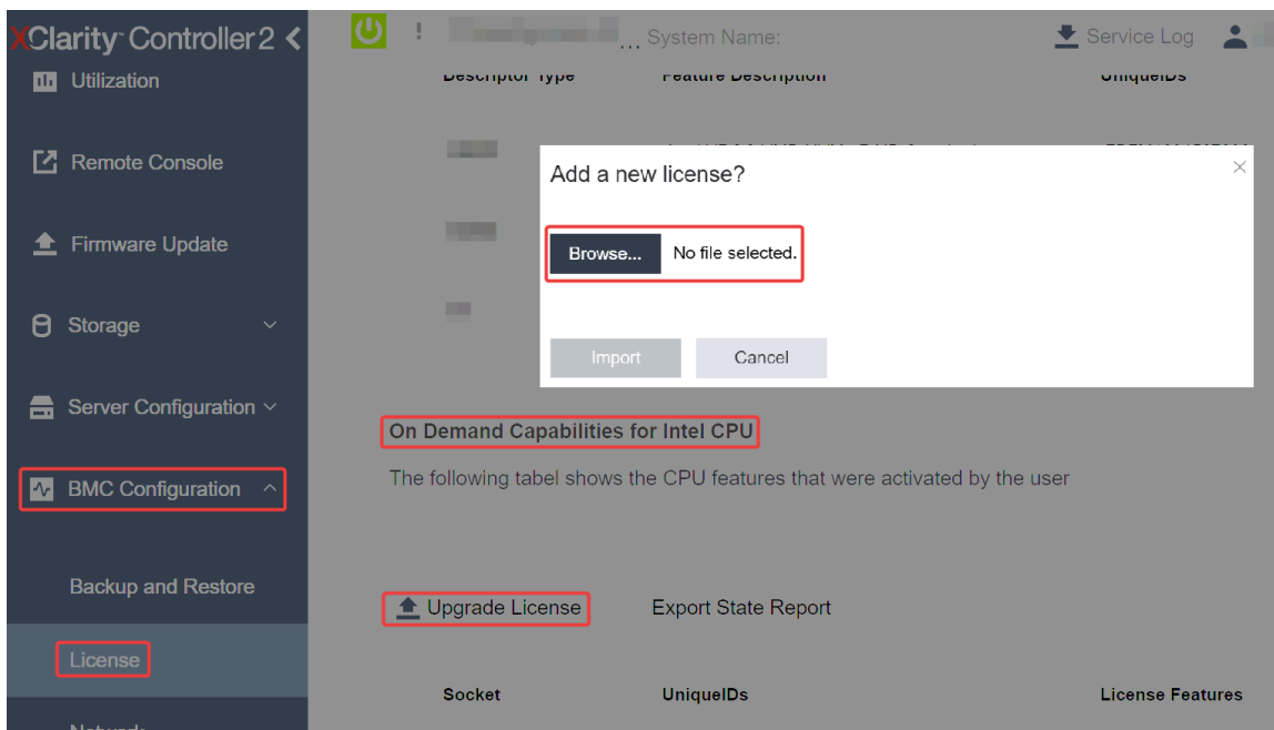
Figura 151. Caricamento della chiave di attivazione tramite la GUI Web di XCC
