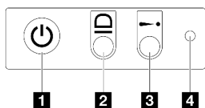
図 11. 前面オペレーター・パネル・ボタンと LED
