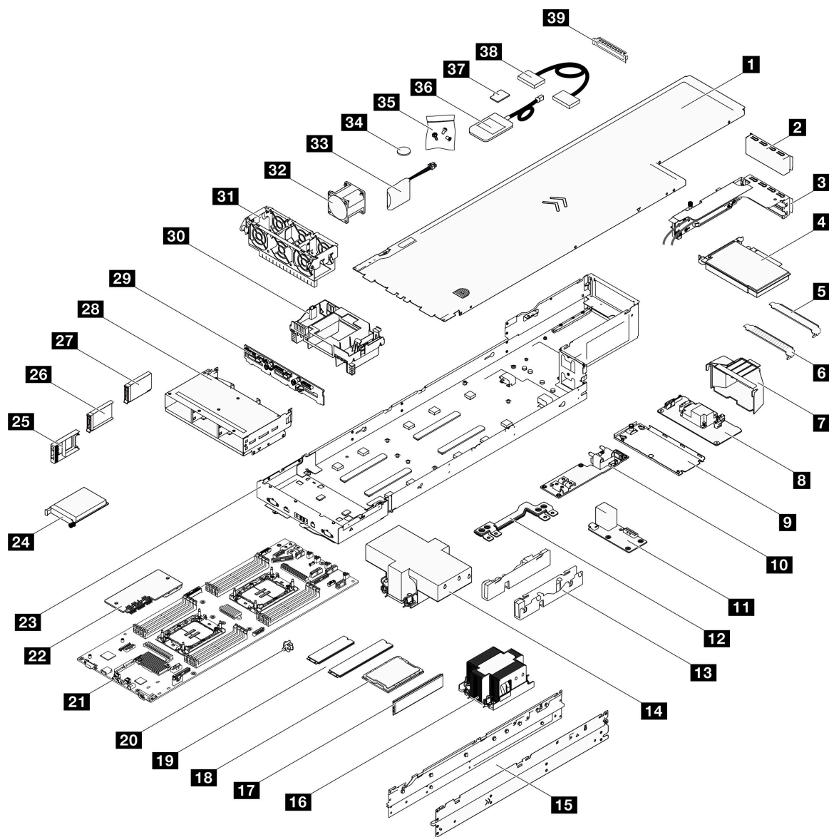
図 16. ノード・コンポーネント
