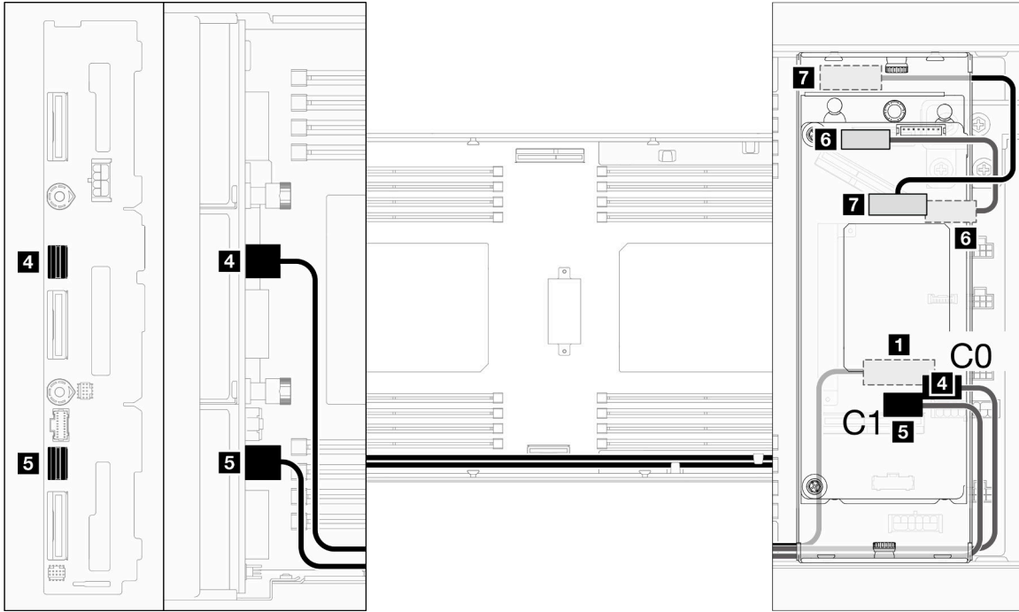
그림 127. SATA 및 CFF RAID 케이블 배선
