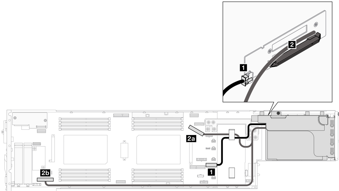
그림 130. PCIe 라이저 케이블 배선 - 프로세서 1개
