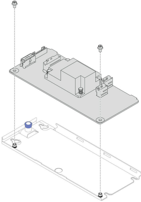
그림 29. 트레이에서 내부 CFF RAID 어댑터 분리
