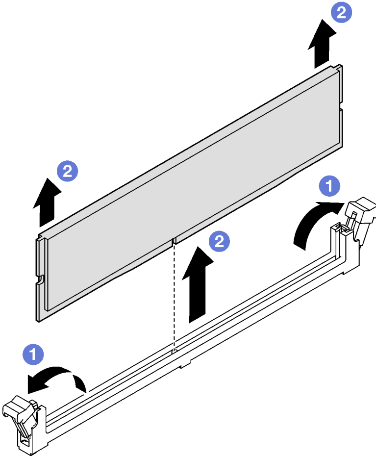
그림 63. 메모리 모듈 제거
