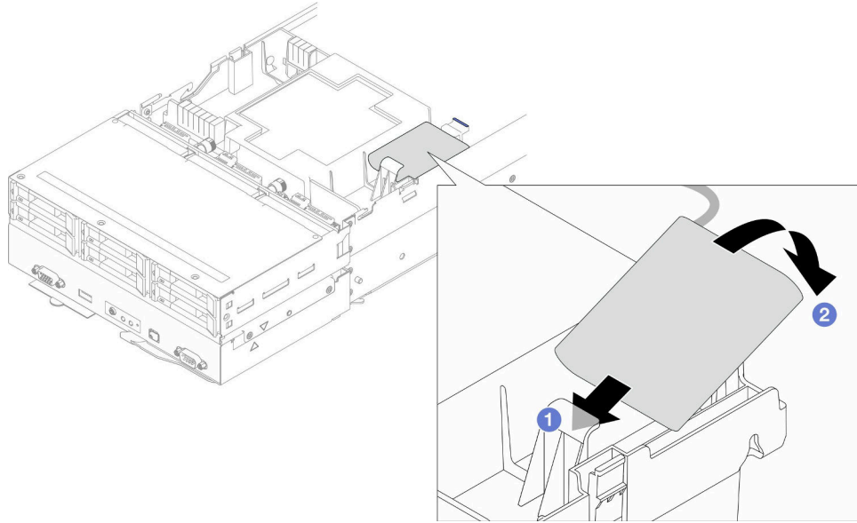
그림 44. 플래시 전원 모듈 설치
