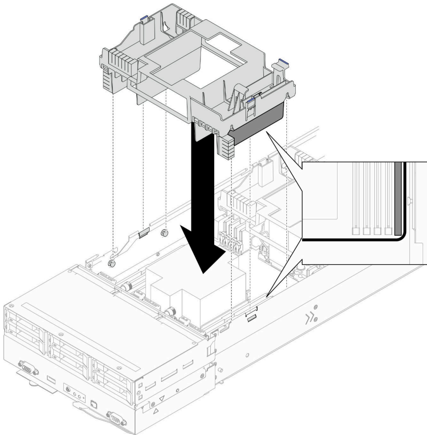
그림 26. 전면 공기 조절 장치 설치
