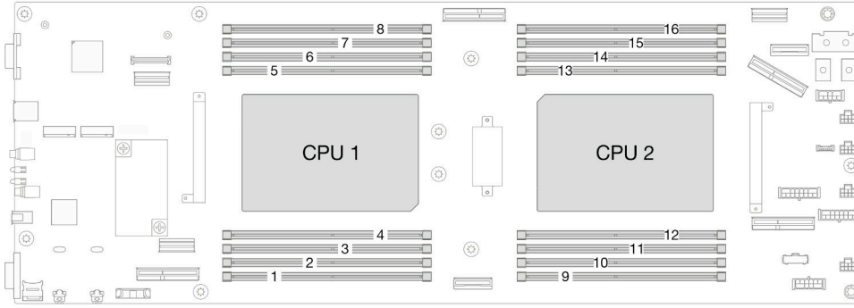
그림 62. 메모리 모듈 및 프로세서 레이아웃
