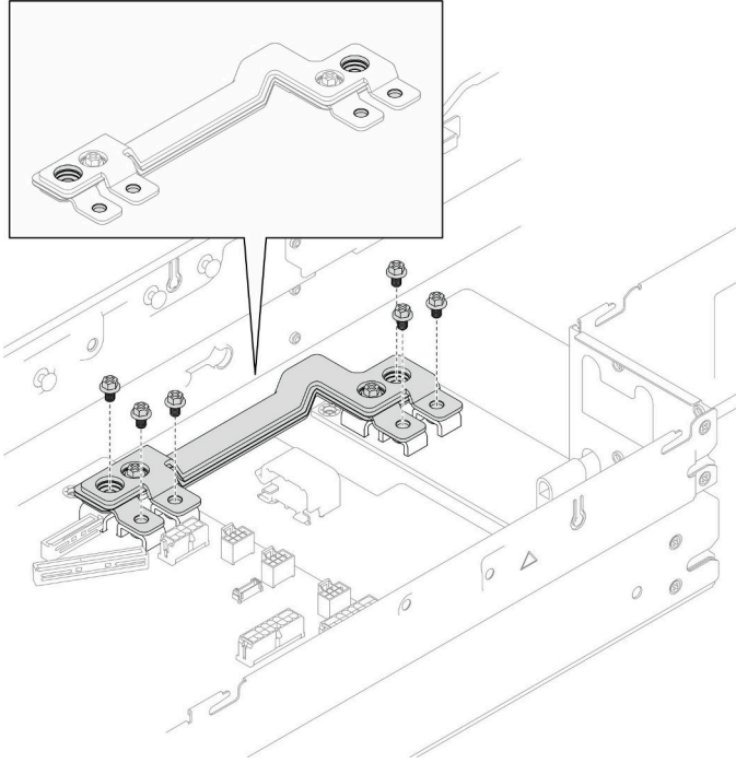
그림 82. 전원 버스 바 외부 나사 설치
