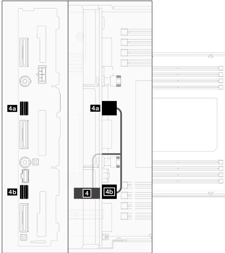
그림 123. SATA 케이블 배선 - CFF RAID가 없는 구성
