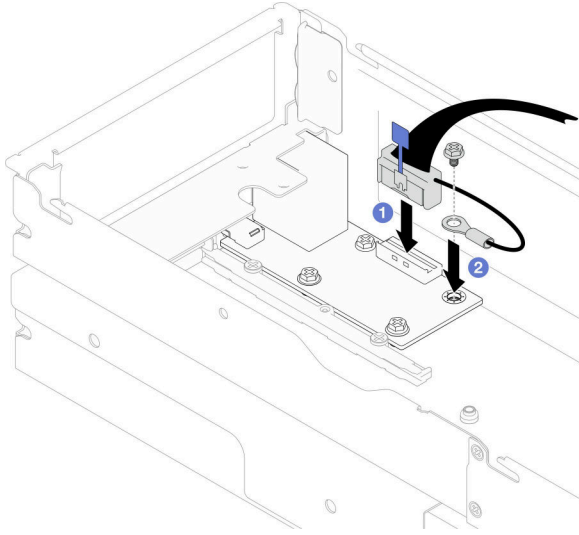
그림 99. 뒷면 I/O 케이블 및 접지 케이블 설치
