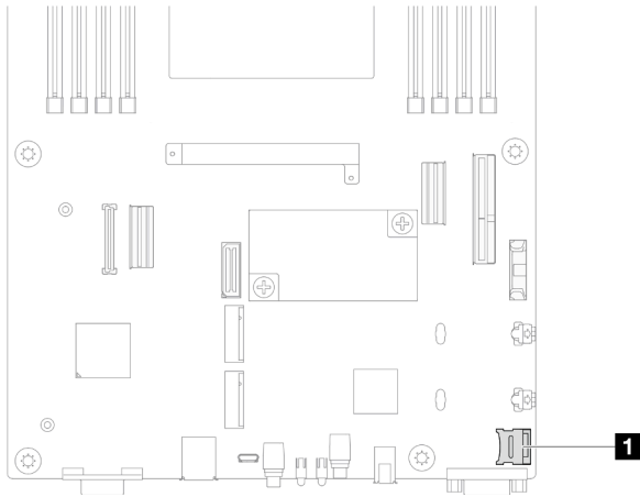
그림 68. MicroSD 소켓의 위치
