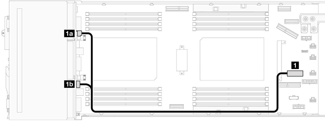
그림 124. 드라이브 백플레인 전원 케이블 배선
