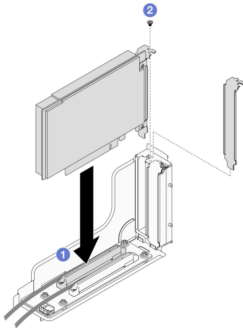
그림 76. PCIe 어댑터 설치
