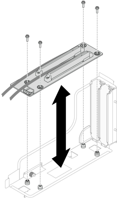
그림 75. PCIe 라이저 카드 교체
