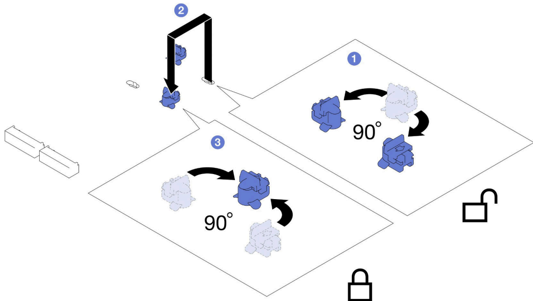
그림 59. M.2 드라이브 고정장치 조정
