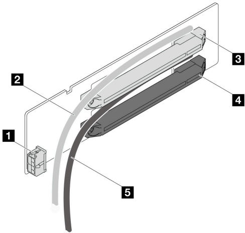
그림 119. 2슬롯 PCIe 라이저 카드 커넥터 및 케이블
