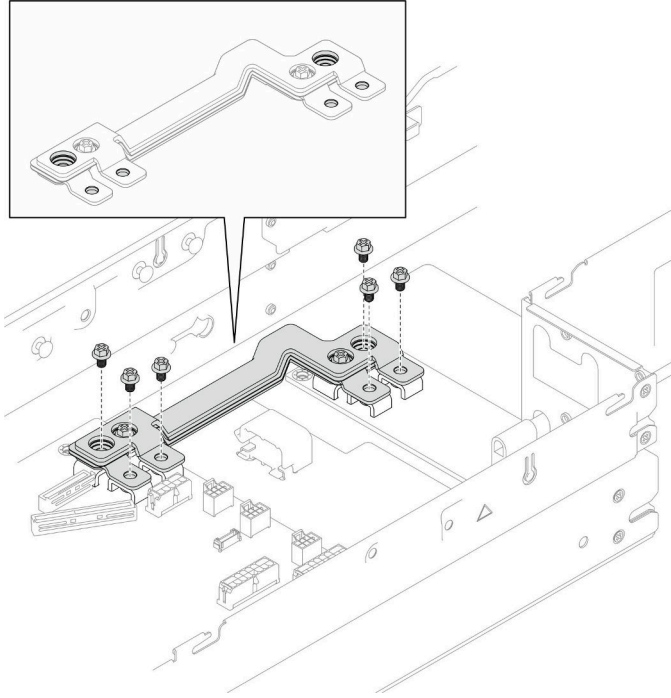
그림 79. 전원 버스 바의 외부 나사 제거
