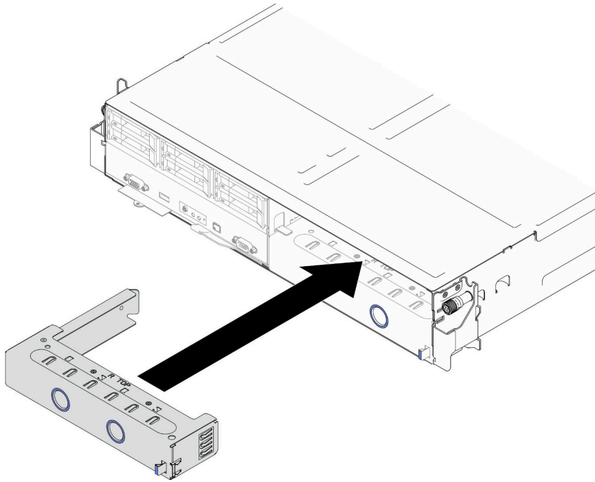
그림 18. 앞면 노드 트레이 필터 설치
