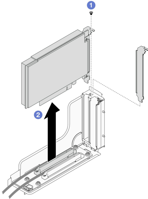
그림 74. PCIe 어댑터 제거
