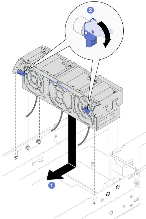
그림 42. 팬 케이스 설치
