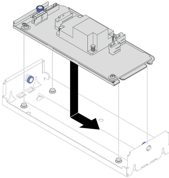
그림 30. 브래킷에 내부 CFF RAID 어댑터 설치
