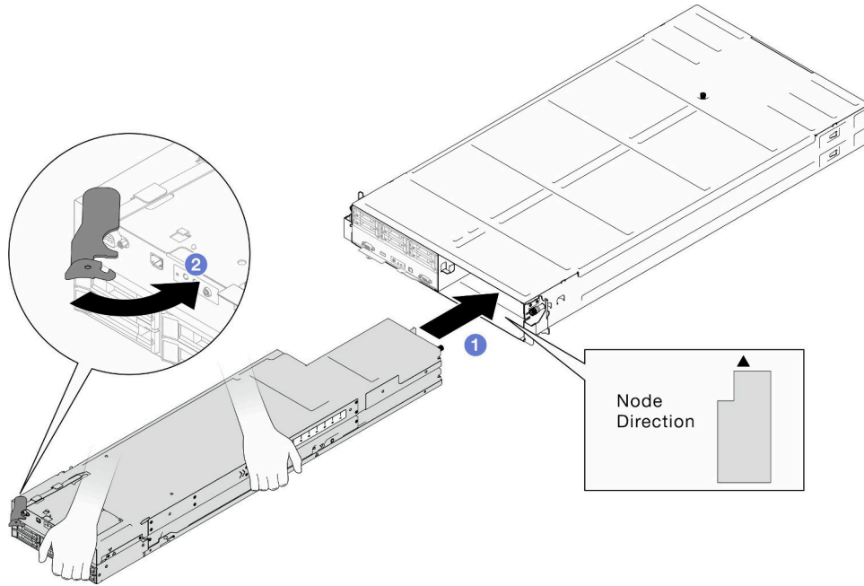
그림 23. 오른쪽 트레이에 노드 설치
