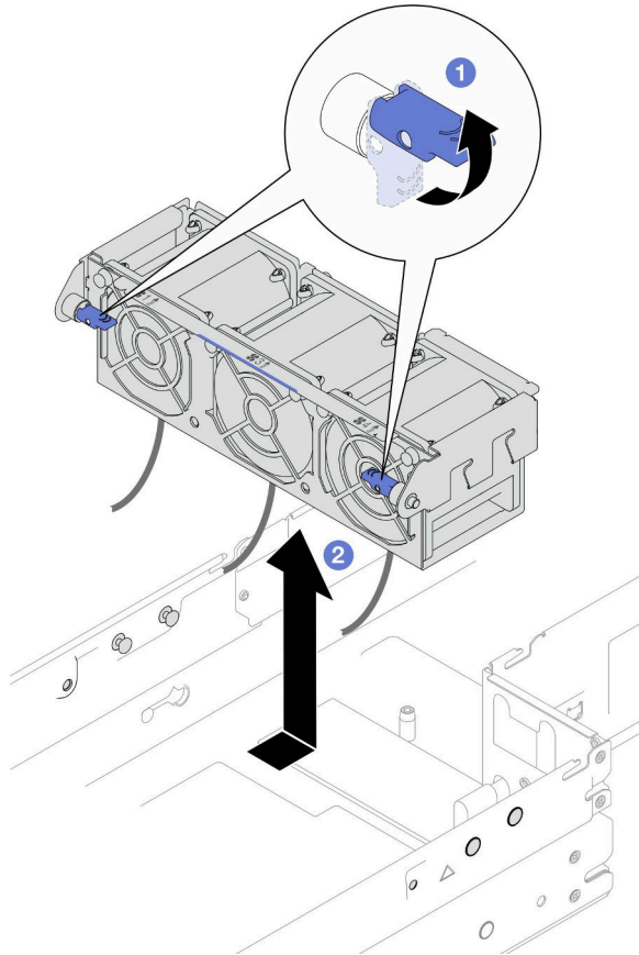
그림 39. 팬 케이지 제거
