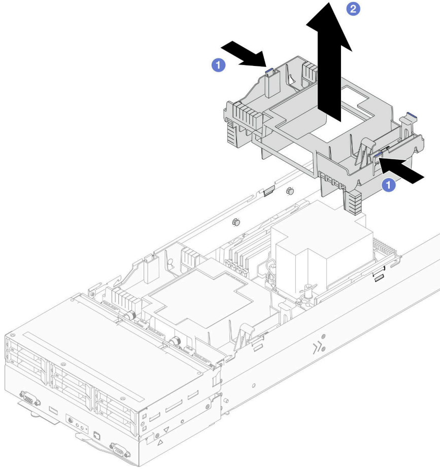
그림 25. 뒷면 공기 조절 장치 제거
