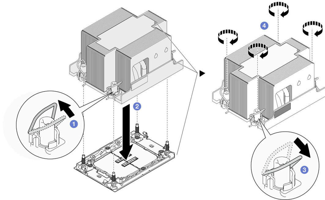
그림 94. 2U 표준 PHM 설치
