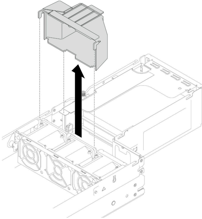
그림 47. GPU 통풍관 제거
