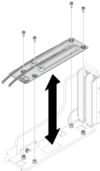
그림 73. PCIe 라이저 카드 교체
