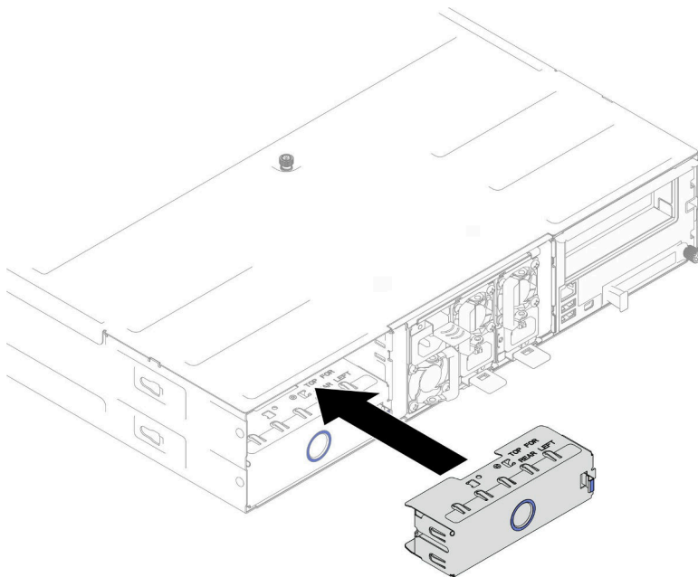
그림 19. 뒷면 노드 트레이 필터 설치
