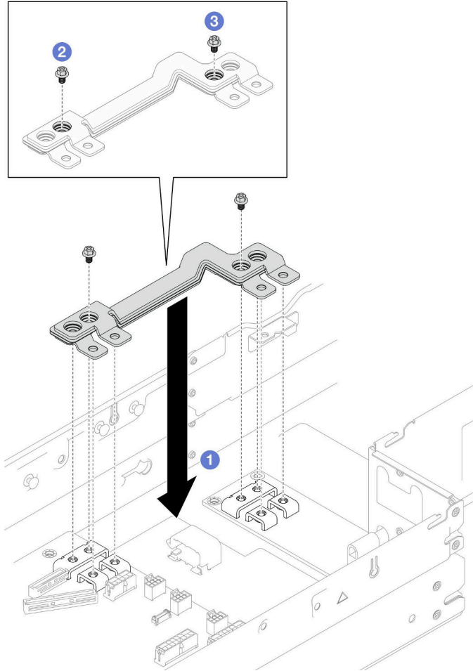
그림 81. 전원 버스 바 설치
