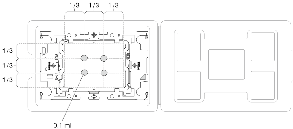
그림 92. 운송 트레이에 프로세서가 있는 열전도 그리스 도포
