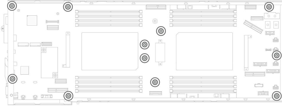
그림 112. 시스템 보드에 나사 설치
