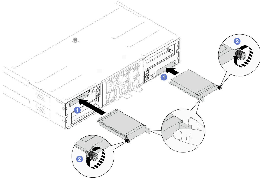
그림 71. 뒷면 OCP 모듈 설치
