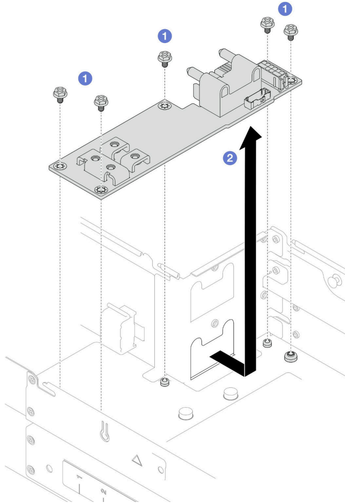
그림 83. 전원 분배 보드 제거
