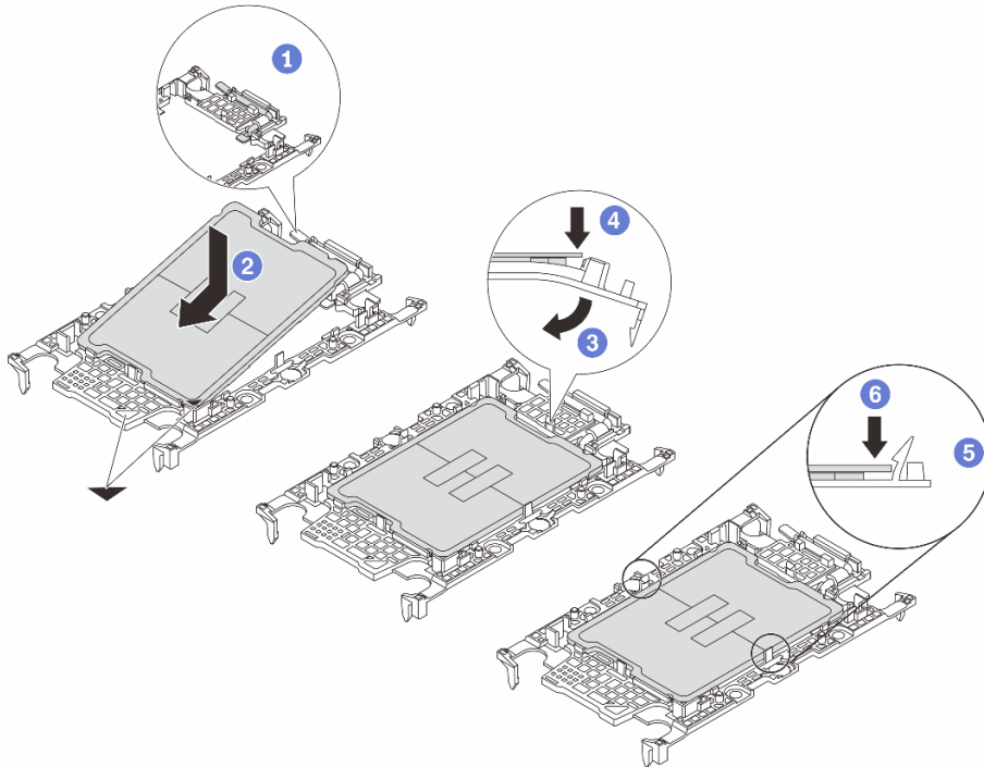
그림 91. 프로세서 캐리어 설치
