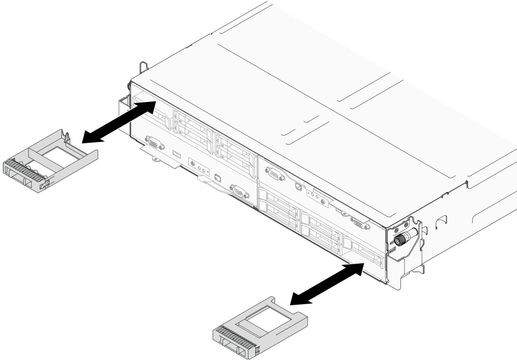
그림 51. 드라이브 필러 교체
