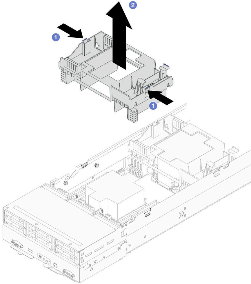
그림 24. 전면 공기 조절 장치 제거
