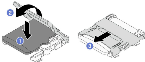
그림 69. MicroSD 카드 설치
