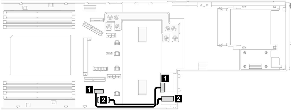
그림 132. 전원 분배 보드의 케이블 배선
