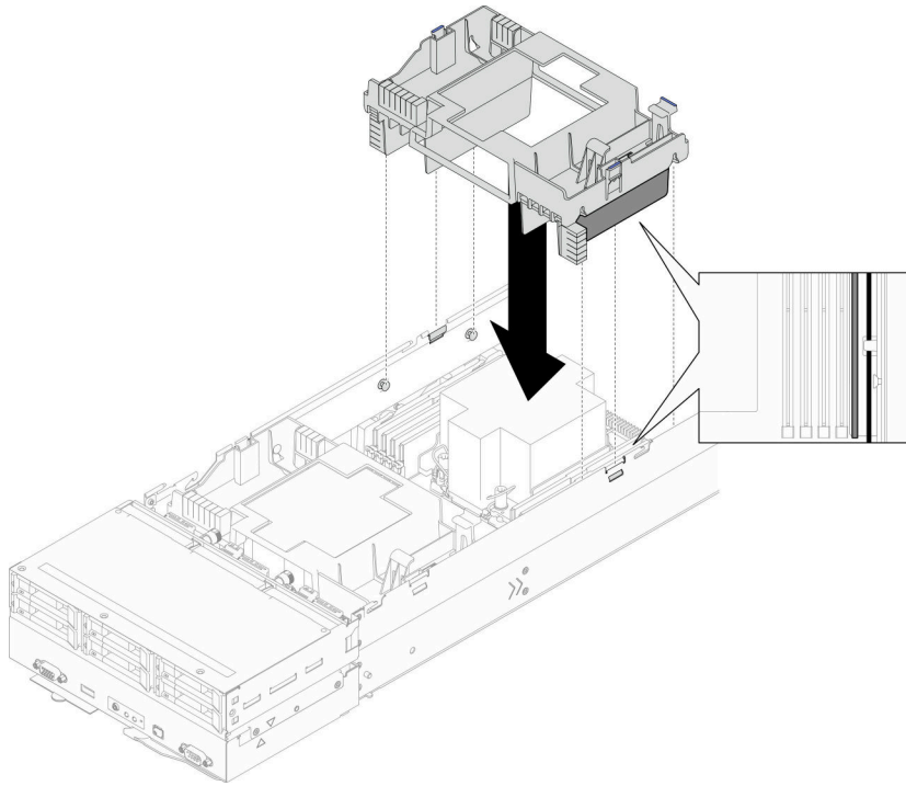
그림 27. 뒷면 공기 조절 장치 설치
