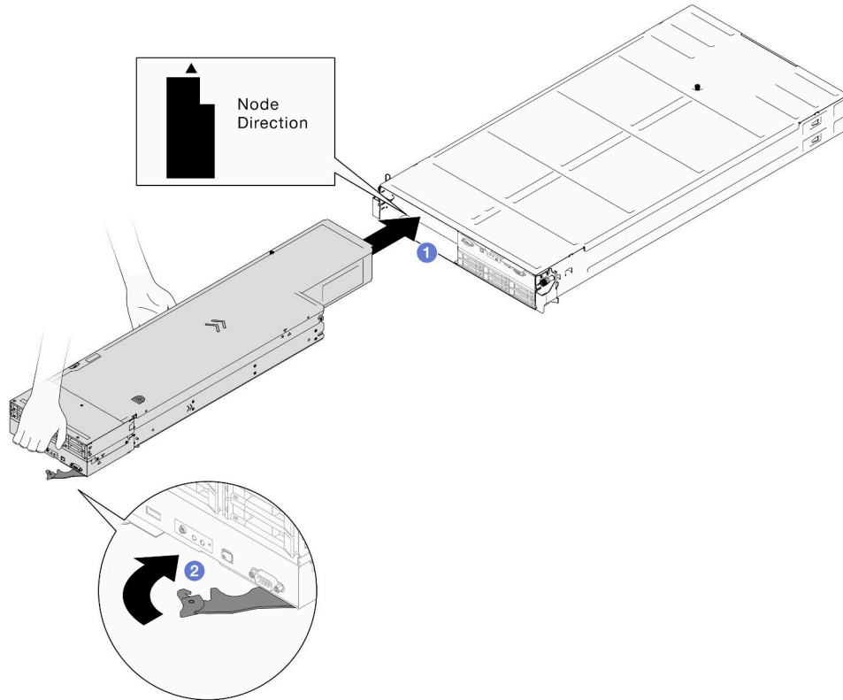
그림 22. 왼쪽 트레이에 노드 설치
