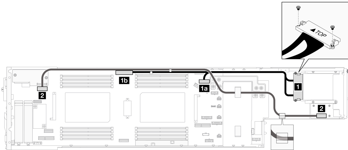
그림 133. 뒷면 I/O 모듈 및 OCP 모듈의 케이블
