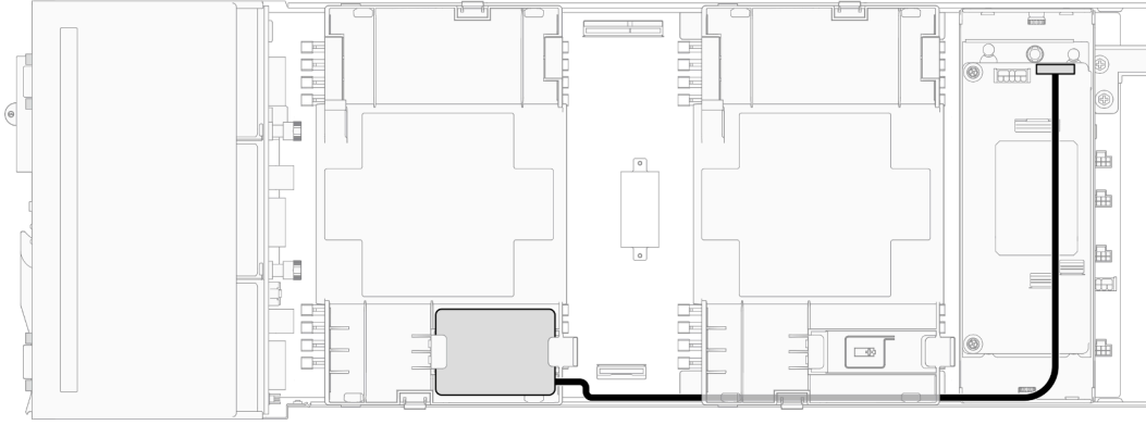
그림 129. CFF RAID 및 플래시 전원 모듈 케이블
