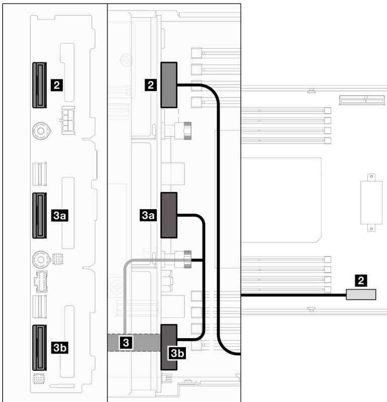
그림 125. NVMe 케이블 배선
