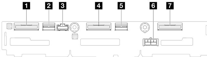
그림 116. 2.5인치 드라이브 백플레인
