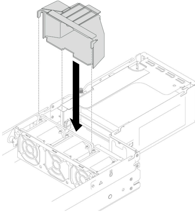
그림 48. GPU 통풍관 설치
