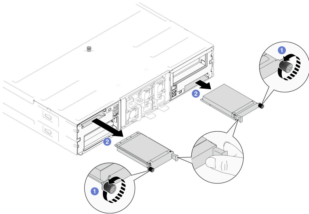
그림 70. 뒷면 OCP 모듈 제거
