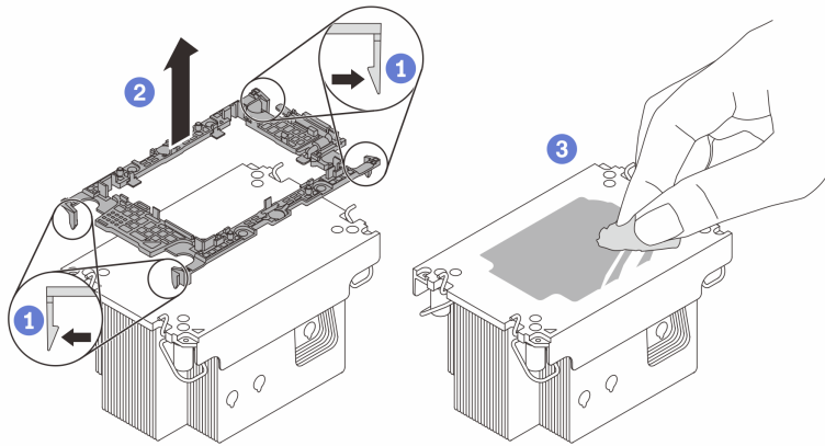
그림 89. 방열판에서 프로세서 캐리어 분리 중
