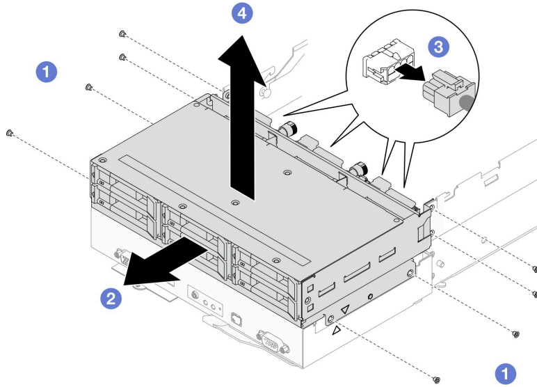
그림 35. 드라이브 케이지 어셈블리 제거
