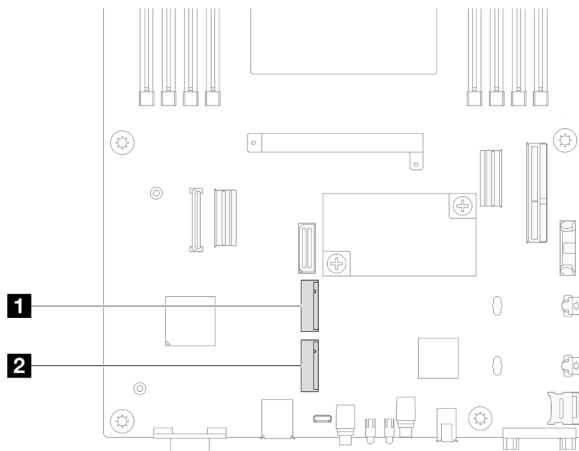
그림 60. 시스템 보드에서 M.2 베이의 위치
