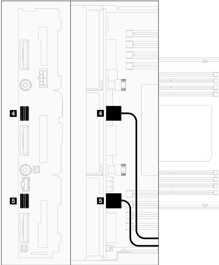
그림 126. 드라이브 백플레인의 SATA 케이블
