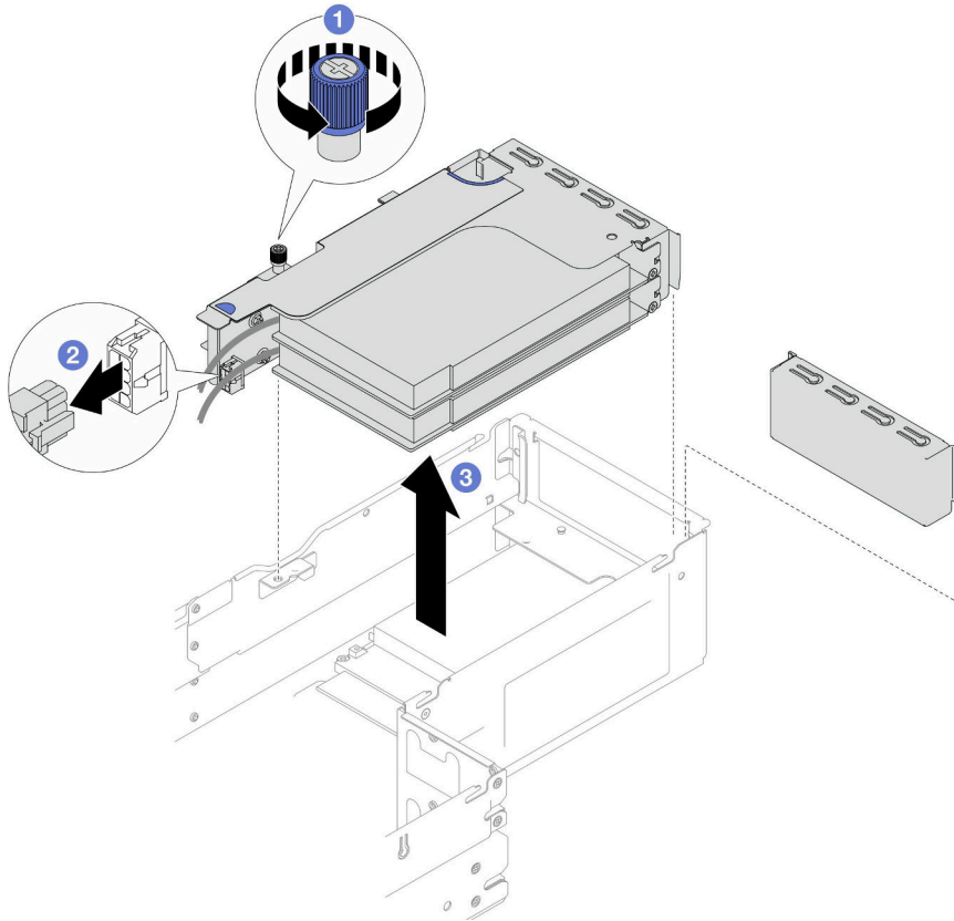
그림 72. PCIe 라이저 어셈블리 제거
