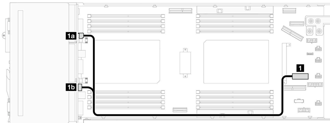
그림 121. 드라이브 백플레인 전원 케이블 배선
