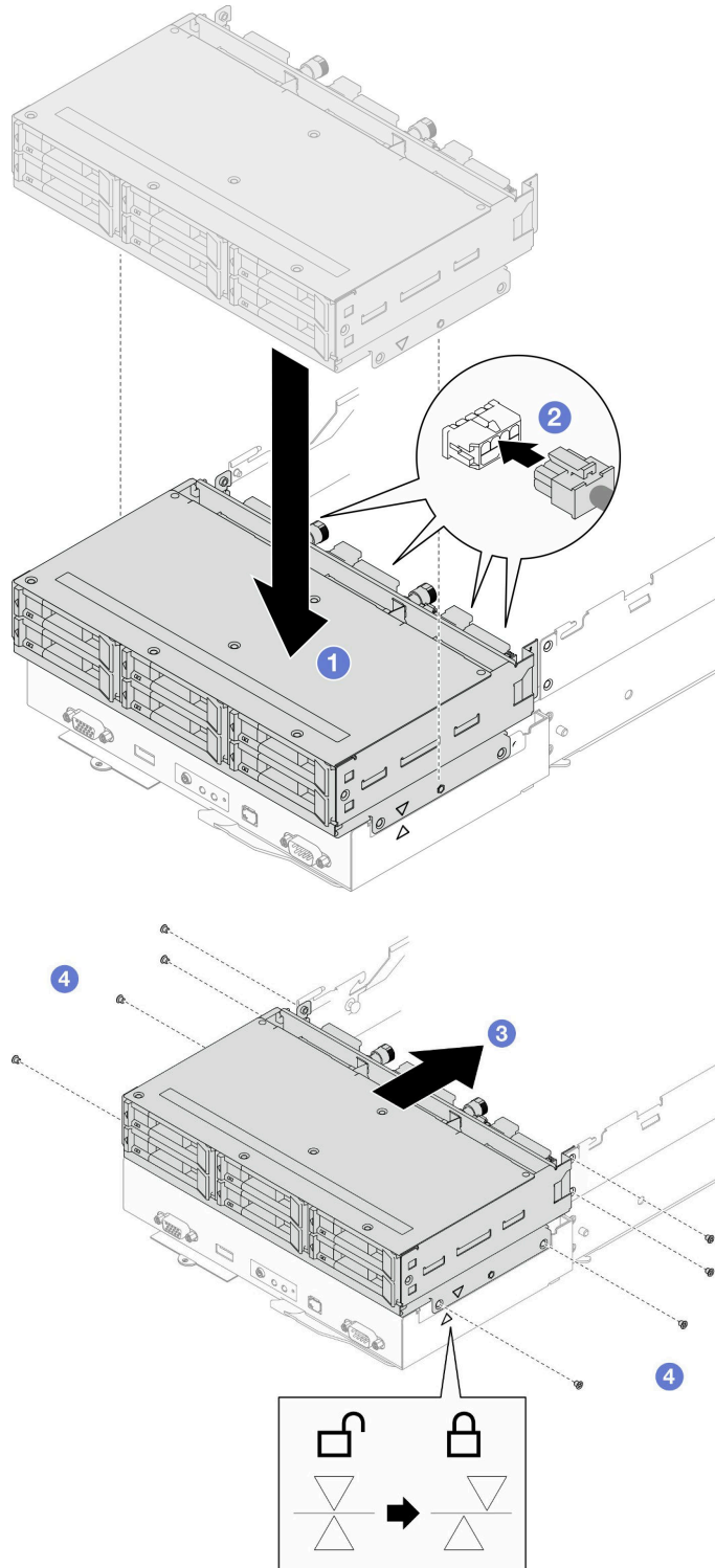
그림 38. 드라이브 케이지 어셈블리 설치
