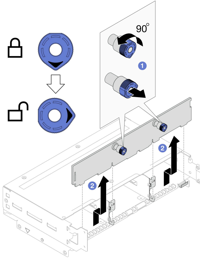
그림 36. 드라이브 백플레인 제거
