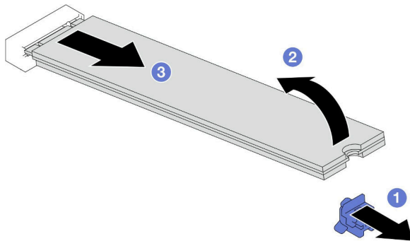
그림 58. M.2 드라이브 제거
