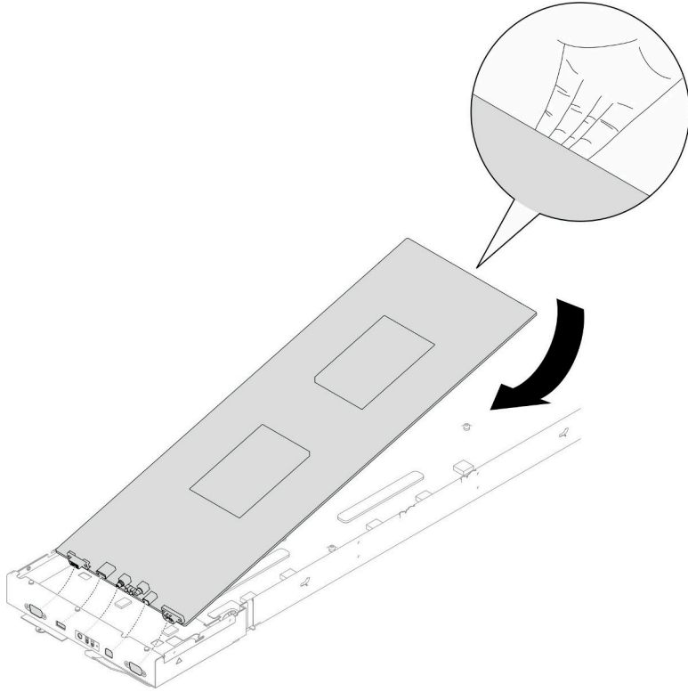
그림 110. 시스템 보드 설치
