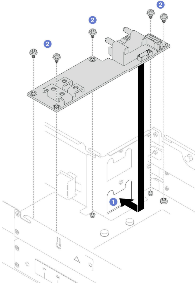
그림 84. 전원 분배 보드 설치
