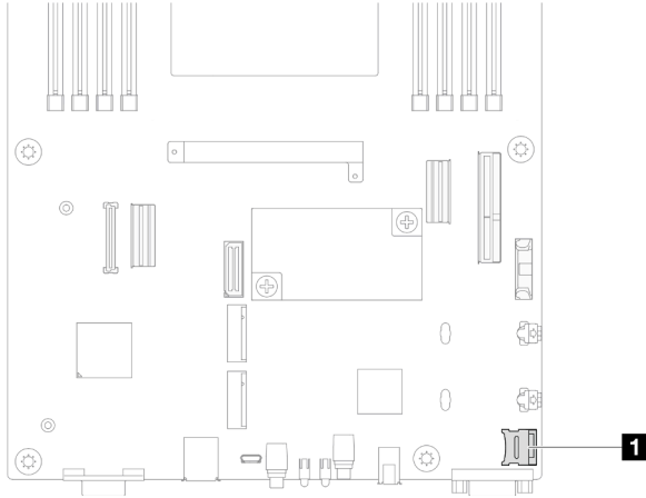
그림 66. MicroSD 소켓의 위치
