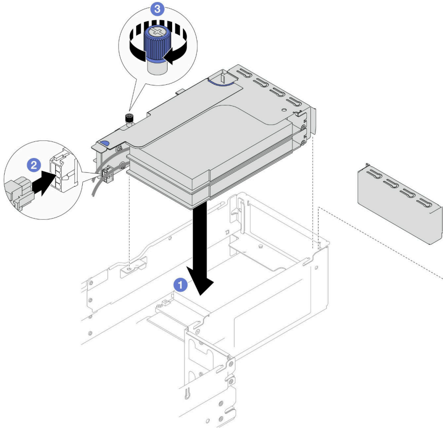
그림 78. PCIe 라이저 어셈블리 설치
