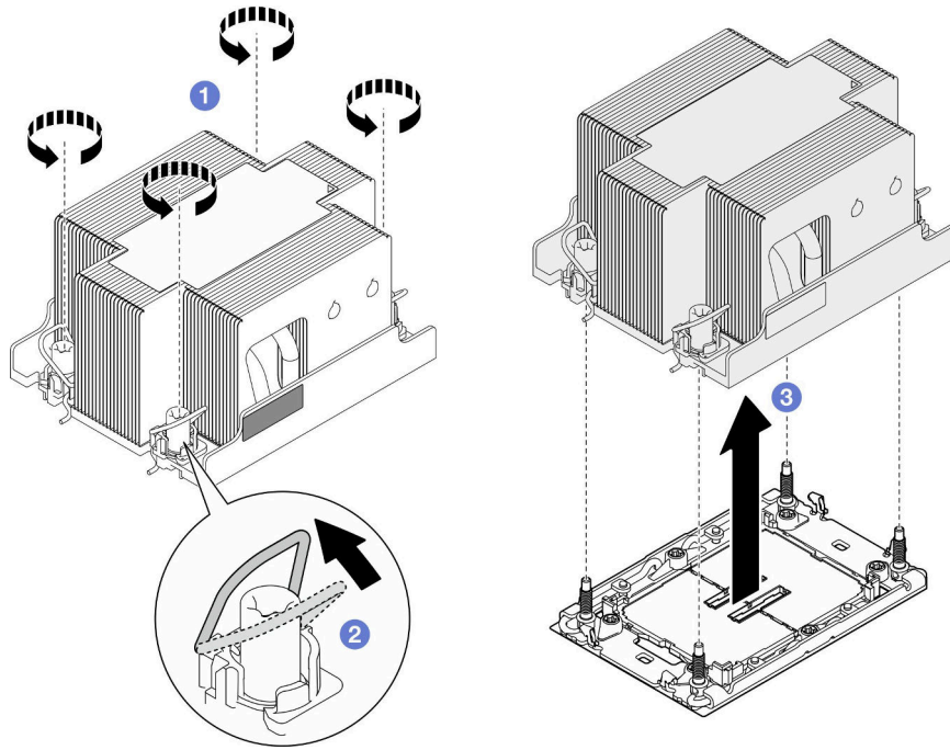
그림 86. 2U 표준 PHM 제거
