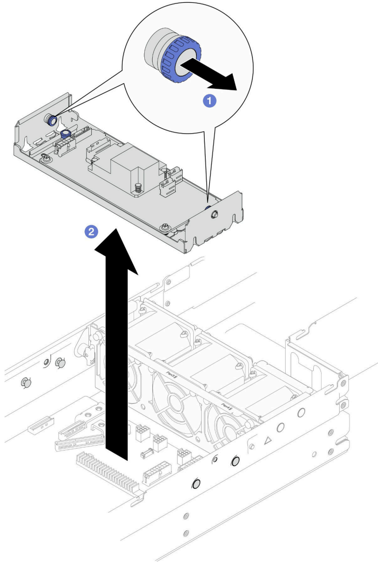
그림 55. 내부 어댑터 브래킷 제거
