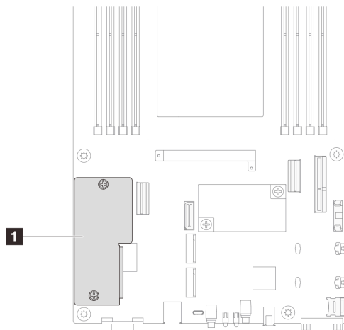
그림 104. 펌웨어 및 RoT 보안 모듈의 위치
