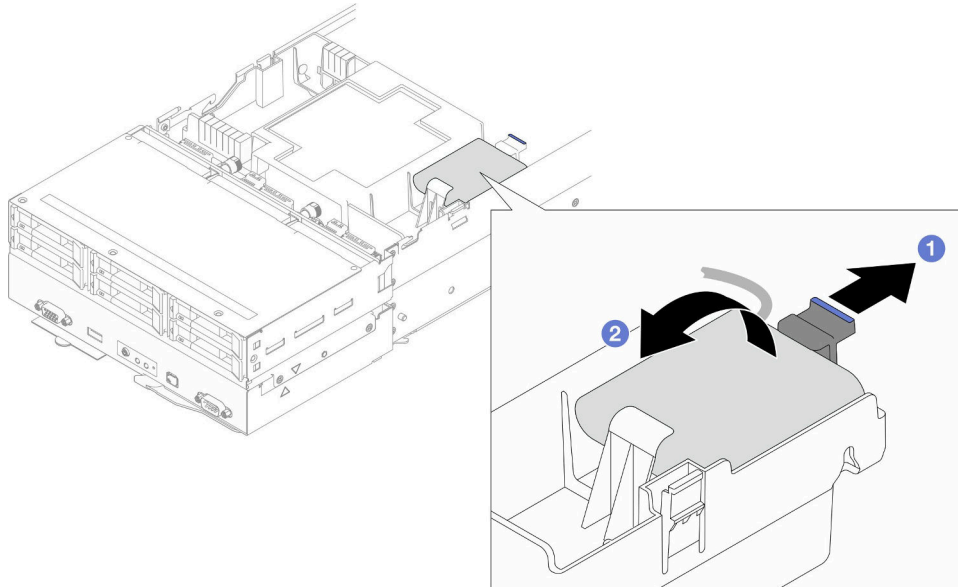
그림 43. 플래시 전원 모듈 제거
