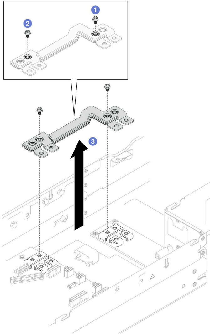
그림 80. 전원 버스 바 제거
