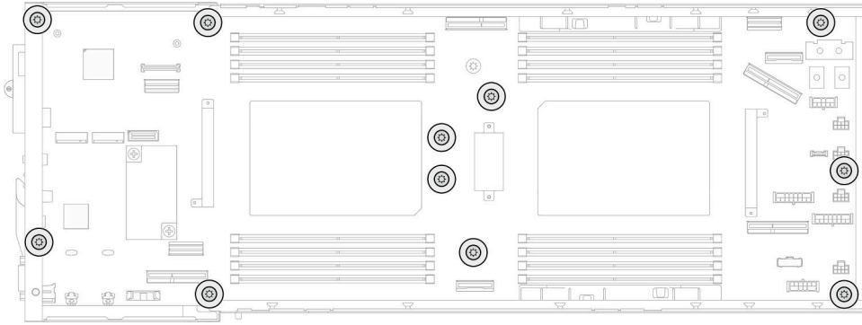
그림 108. 나사 제거
