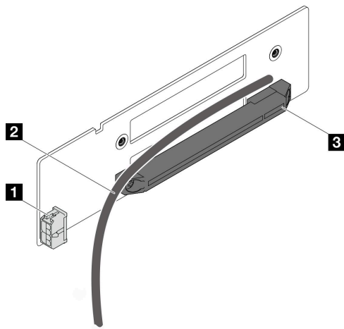
그림 118. 1슬롯 PCIe 라이저 카드 커넥터 및 케이블
