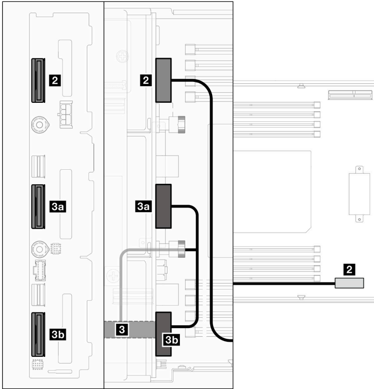
그림 122. NVMe 케이블 배선
