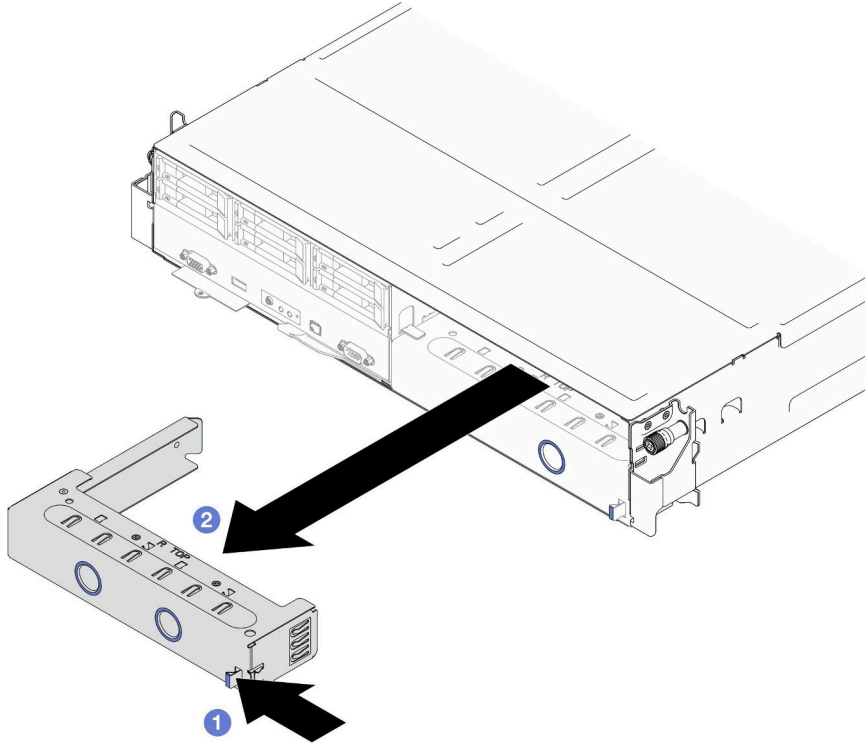
그림 20. 앞면 노드 트레이 필러 제거
