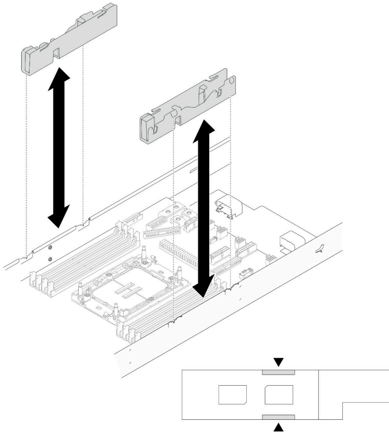
그림 113. 케이블 덕트 교체
