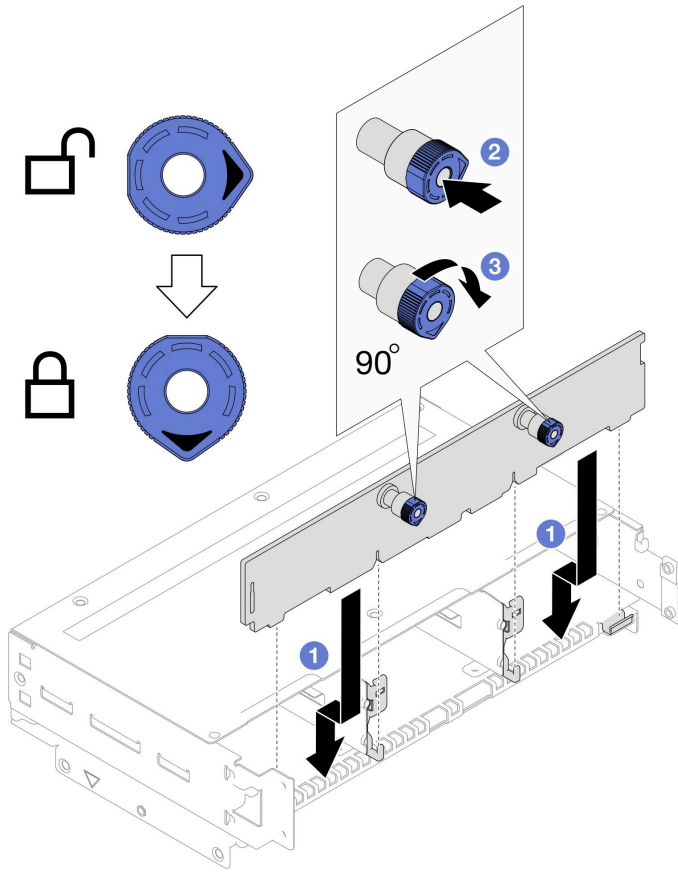
그림 37. 드라이브 백플레인 설치
