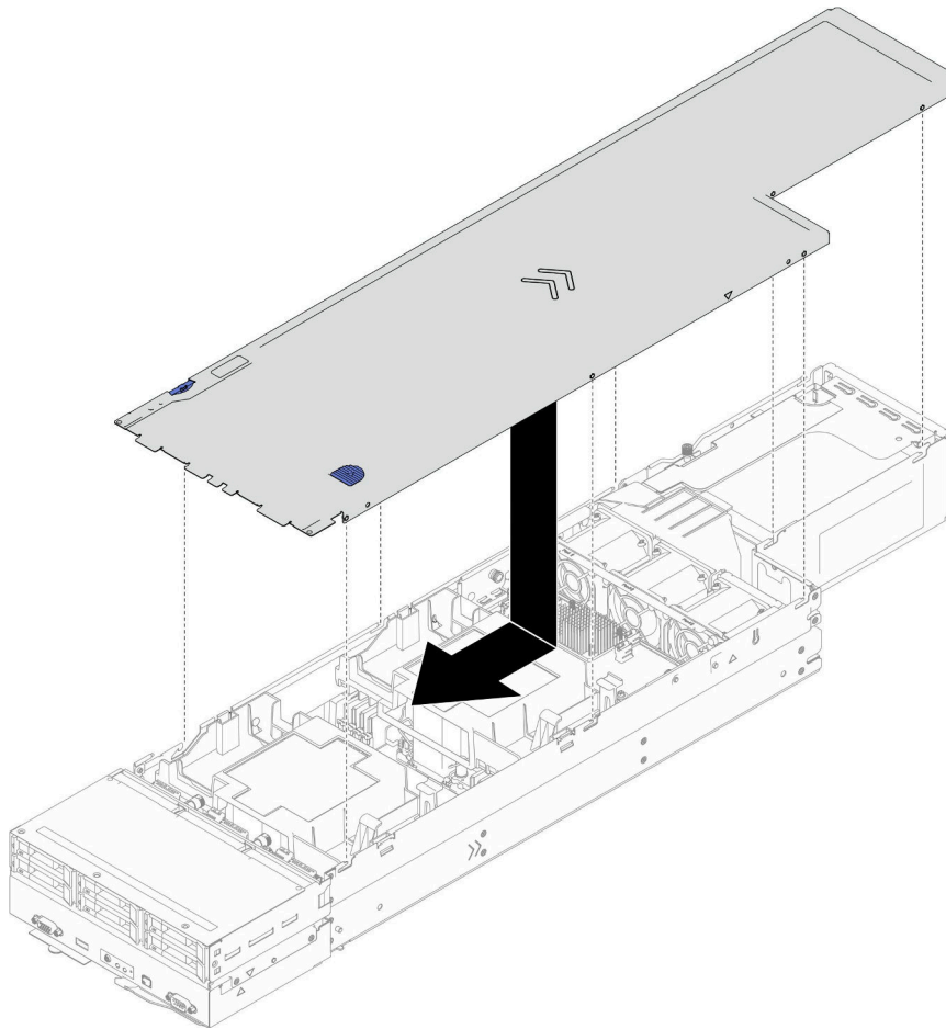
그림 115. 윗면 덮개 설치
