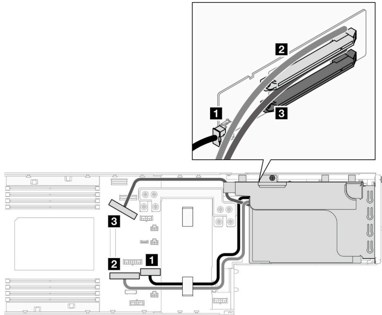
그림 131. PCIe 라이저 케이블 배선 - 프로세서 2개
