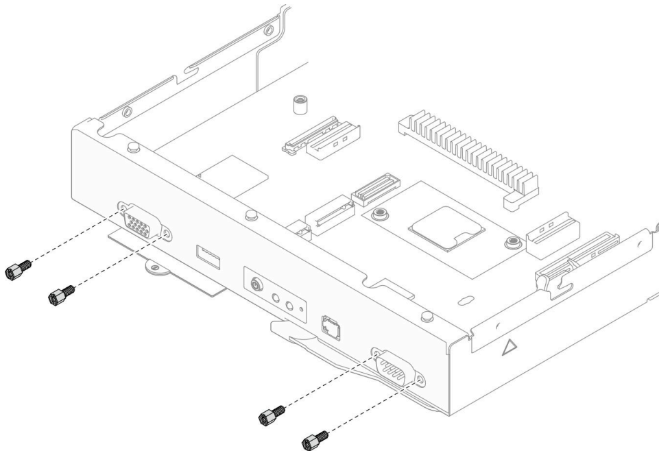
그림 111. 앞면에 시스템 보드 나사 설치
