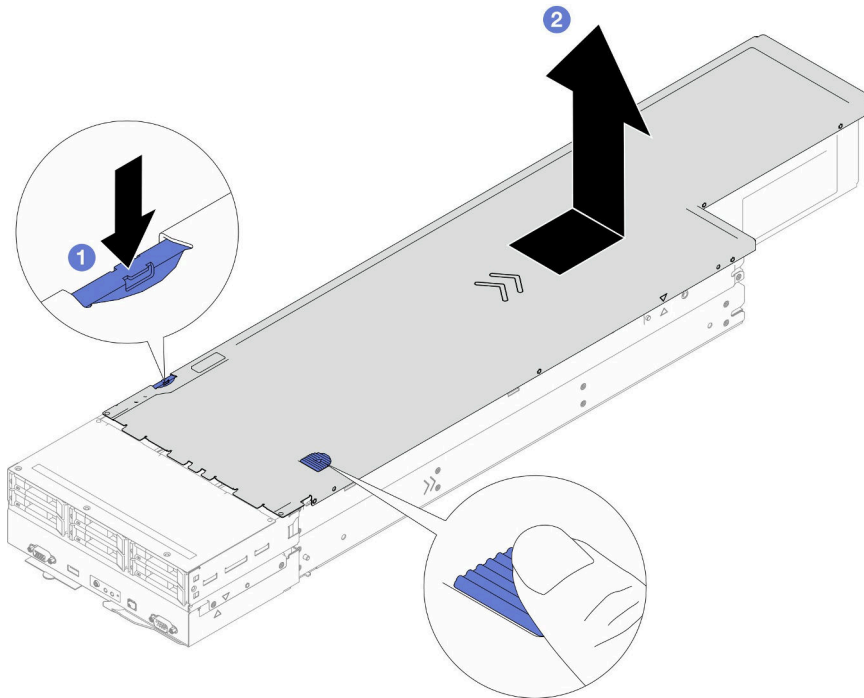
그림 114. 윗면 덮개 제거
