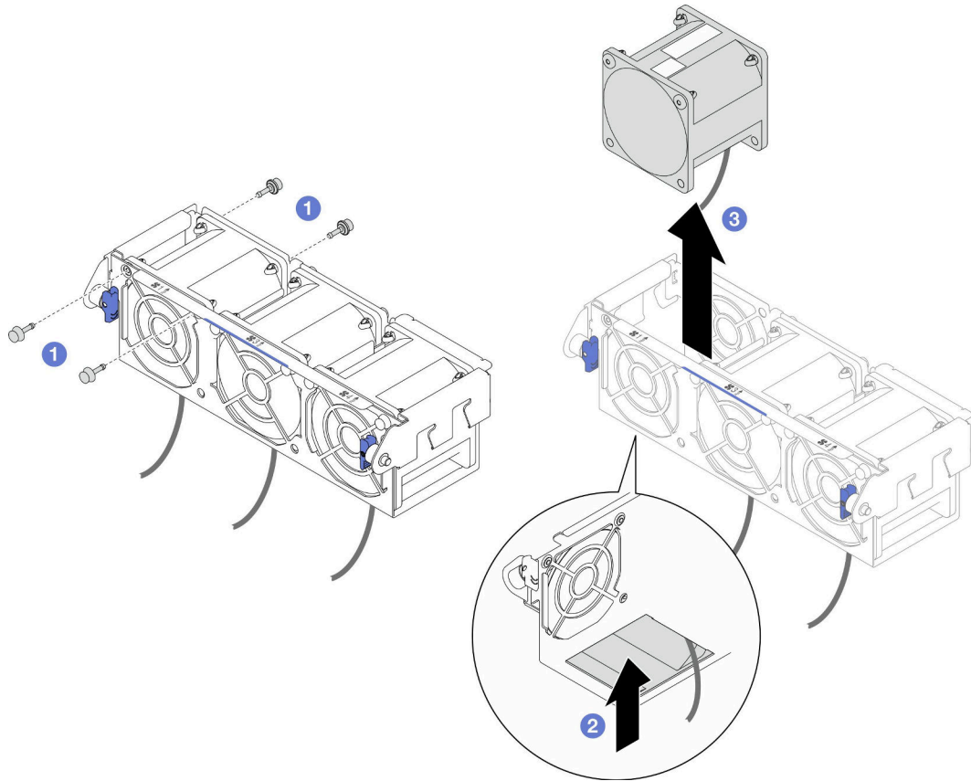
그림 40. 팬 제거
