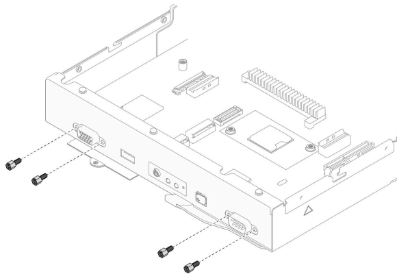
그림 107. 나사 제거
