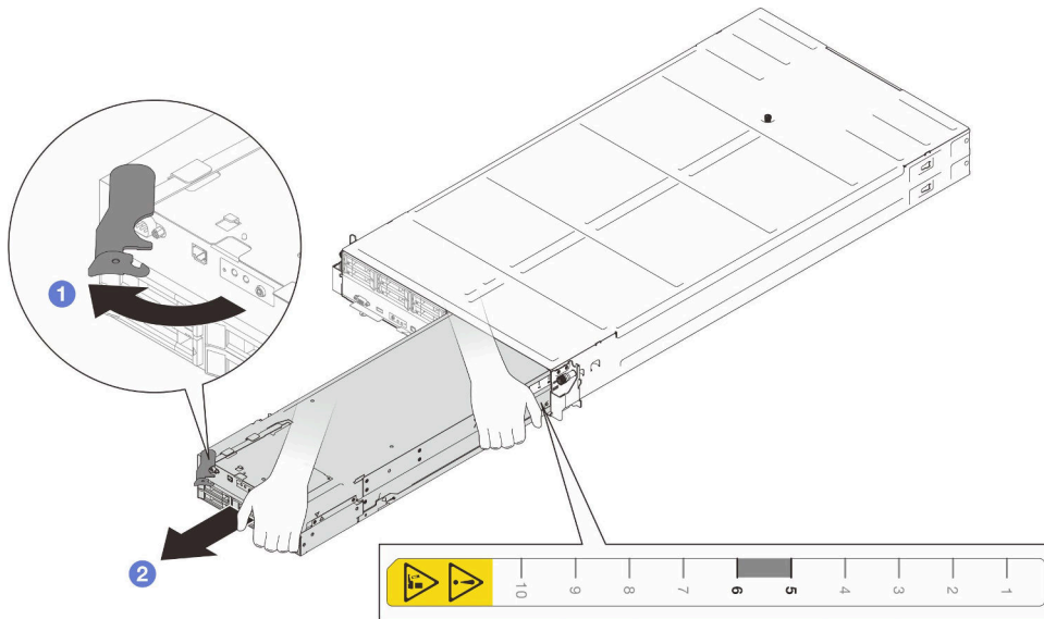
그림 17. 오른쪽 트레이에서 노드 제거
