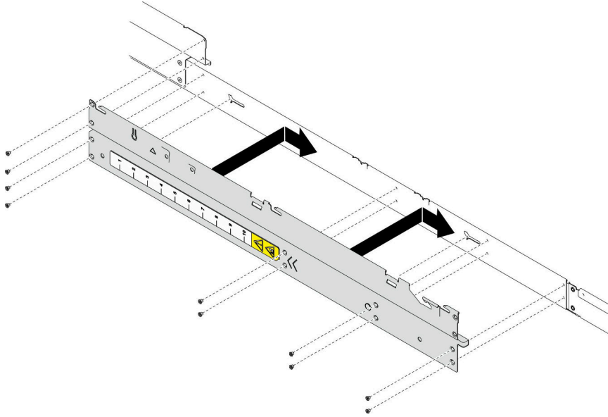
그림 101. 측면 브래킷 설치
