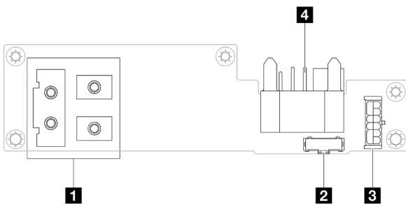
그림 120. 전원 분배 보드 커넥터
