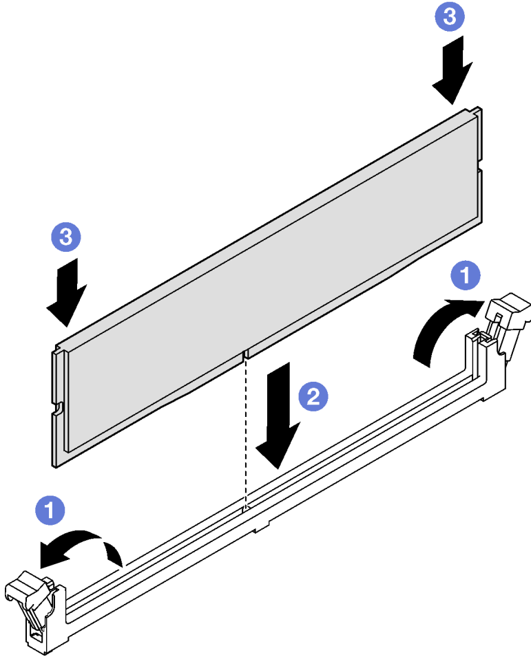
그림 65. 메모리 모듈 설치
