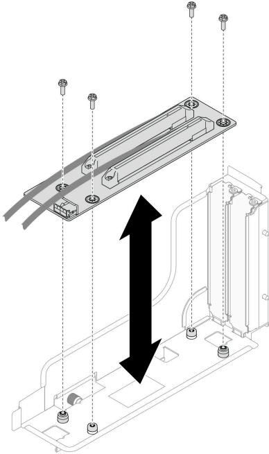
그림 77. PCIe 라이저 카드 교체
