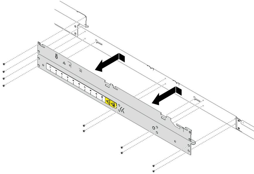
그림 100. 측면 브래킷 제거
