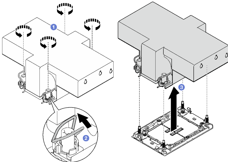
그림 87. 2U 성능 PHM 제거
