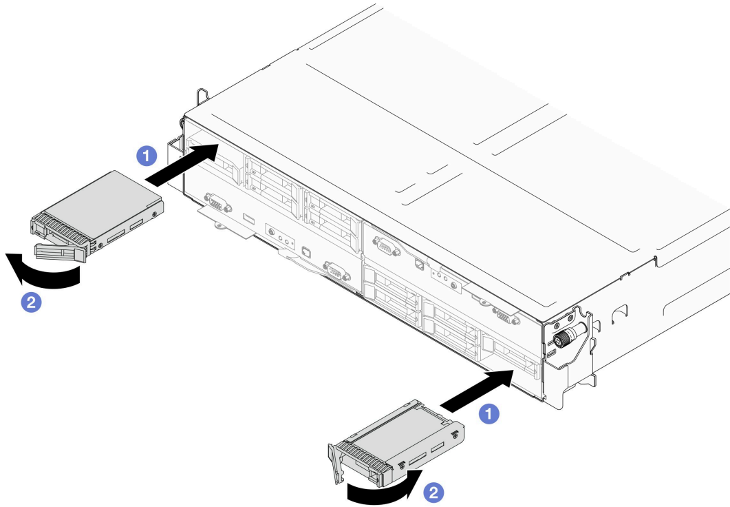
그림 53. 7mm 솔리드 스테이트 드라이브 설치
