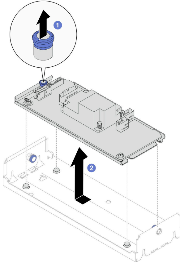
그림 28. 내부 CFF 어댑터 제거
