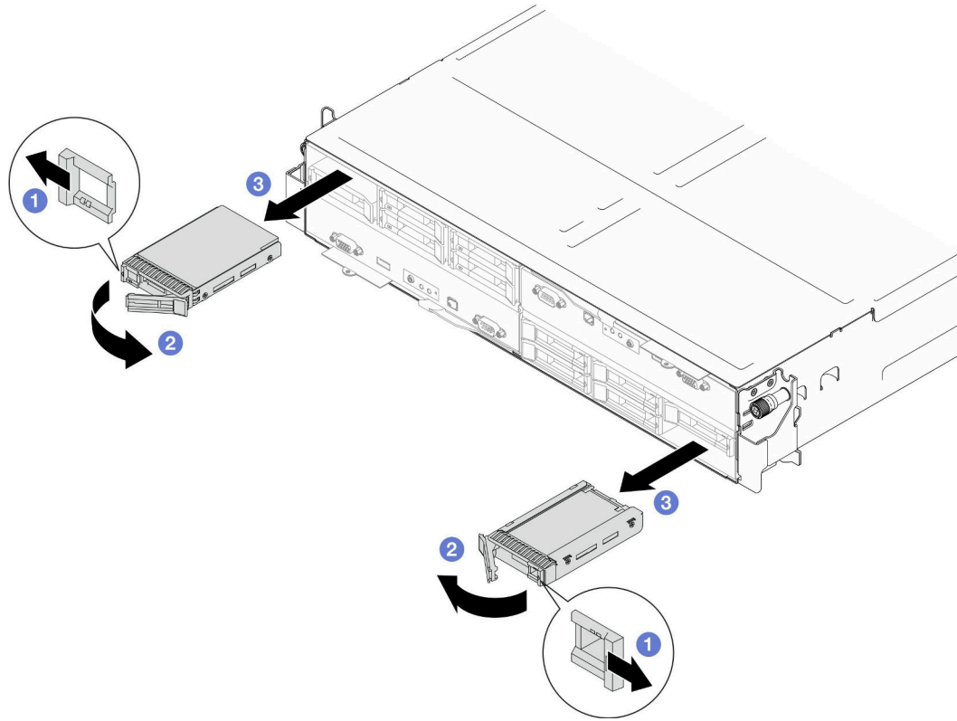
그림 50. 15mm 솔리드 스테이트 드라이브 제거
