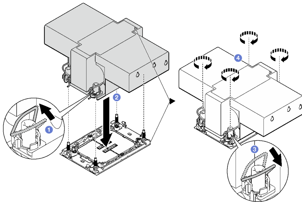
그림 95. 2U 성능 PHM 설치
