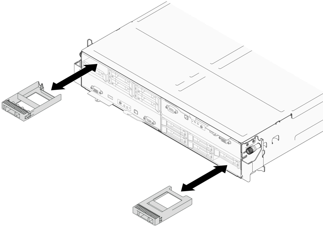
그림 52. 드라이브 필터 교체
