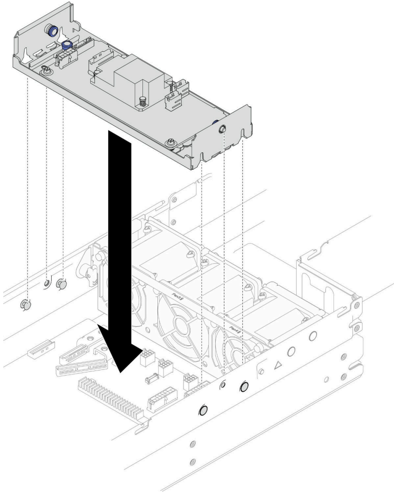
그림 56. 내부 어댑터 브래킷 설치
