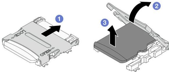
그림 67. MicroSD 카드 제거
