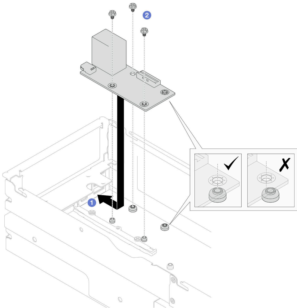
그림 98. 뒷면 I/O 모듈 설치
