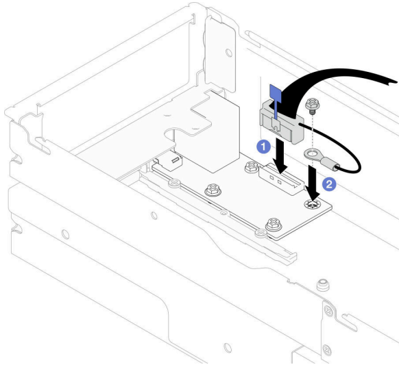
그림 134. 뒷면 I/O 케이블 및 접지 케이블 설치
