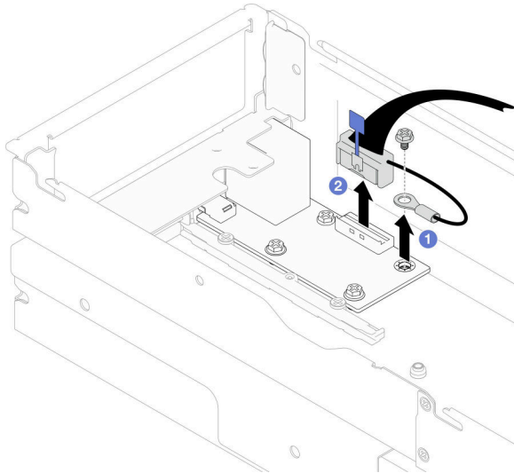
그림 96. 뒷면 I/O 케이블 및 접지 케이블 제거
