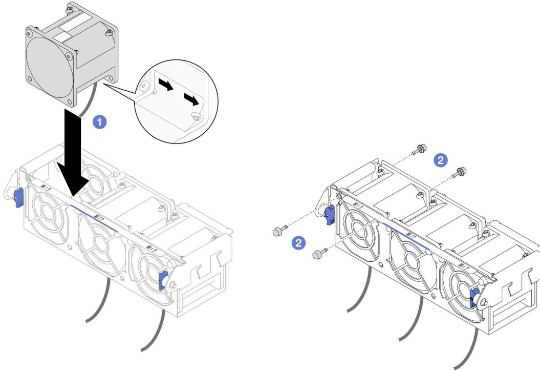
그림 41. 팬 설치
