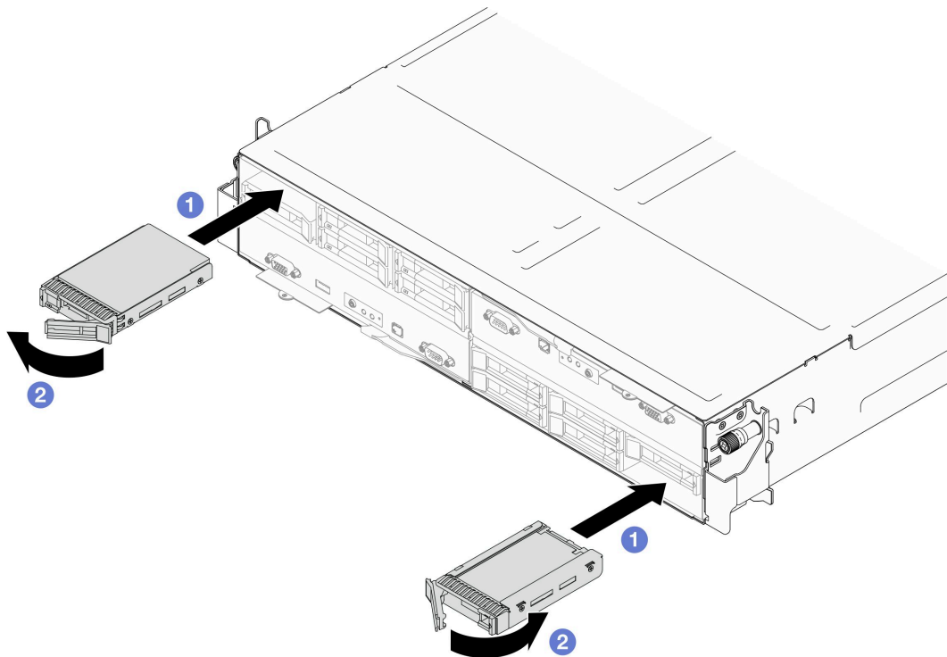
그림 54. 15mm 솔리드 스테이트 드라이브 설치
