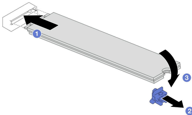
그림 61. M.2 드라이브 설치
