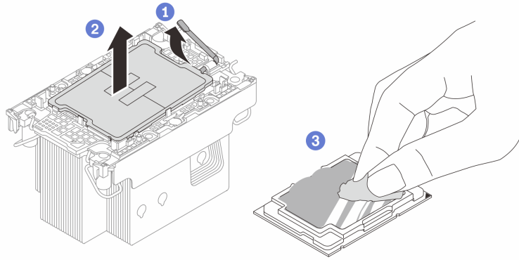
그림 88. 방열판 및 캐리어에서 프로세서 분리 중
