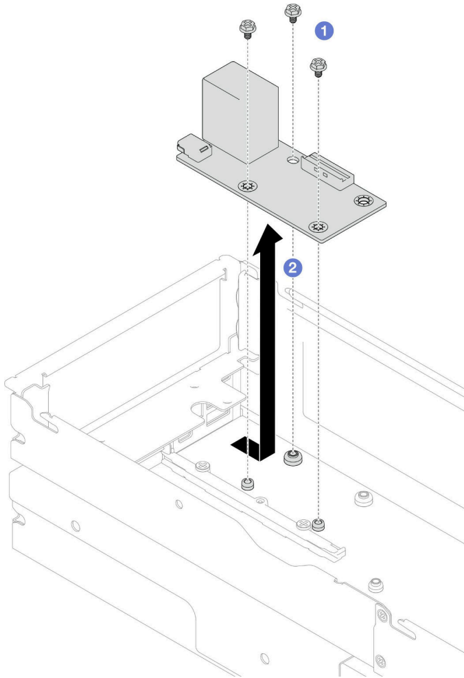
그림 97. 뒷면 I/O 모듈 제거
