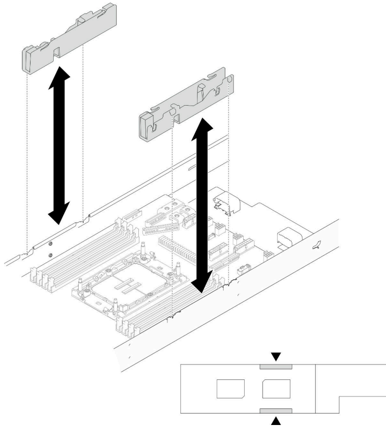
그림 106. 케이블 덕트 교체
