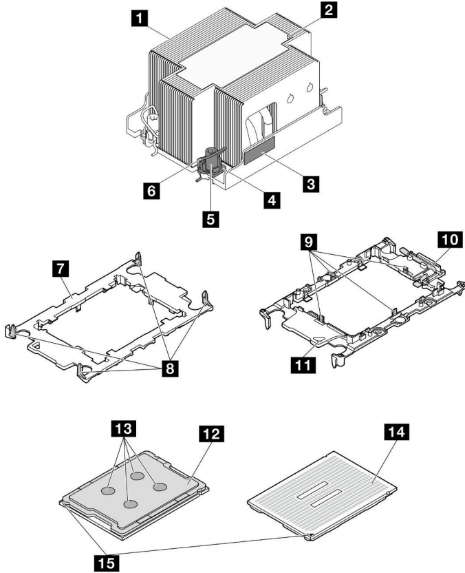
그림 90. PHM 구성 요소
