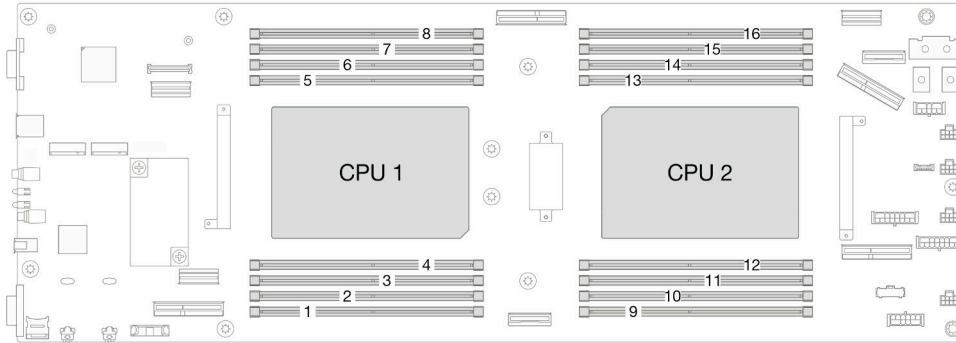
그림 64. 메모리 모듈 및 프로세서 레이아웃
