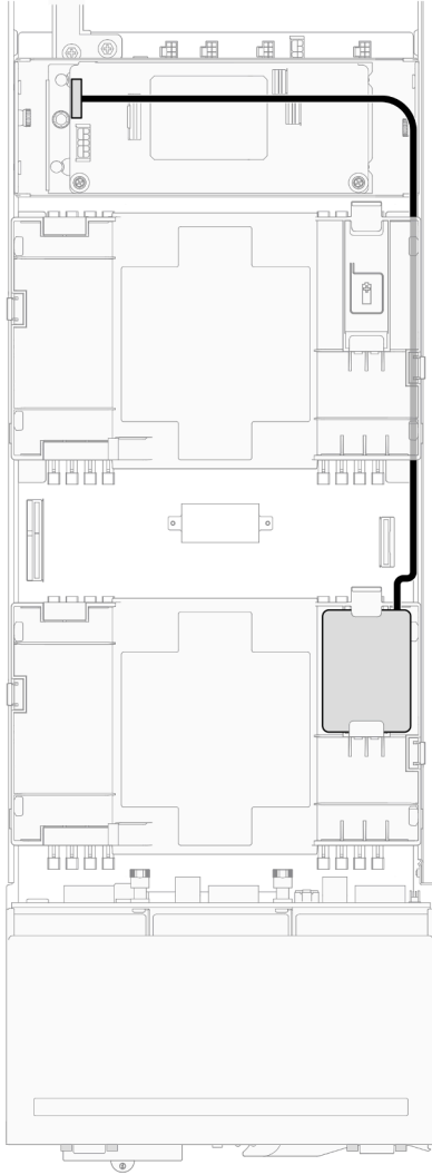
그림 46. CFF RAID 및 플래시 전원 모듈 케이블
