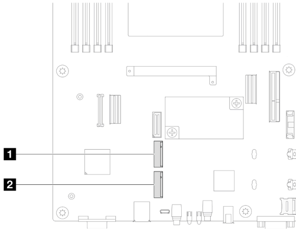
그림 57. 시스템 보드에서 M.2 베이의 위치
