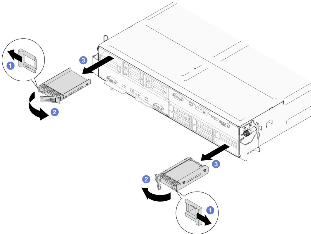
그림 49. 7mm 솔리드 스테이트 드라이브 제거
