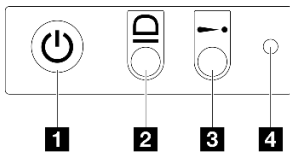
그림 11. 앞면 오퍼레이터 패널 버튼 및 LED
