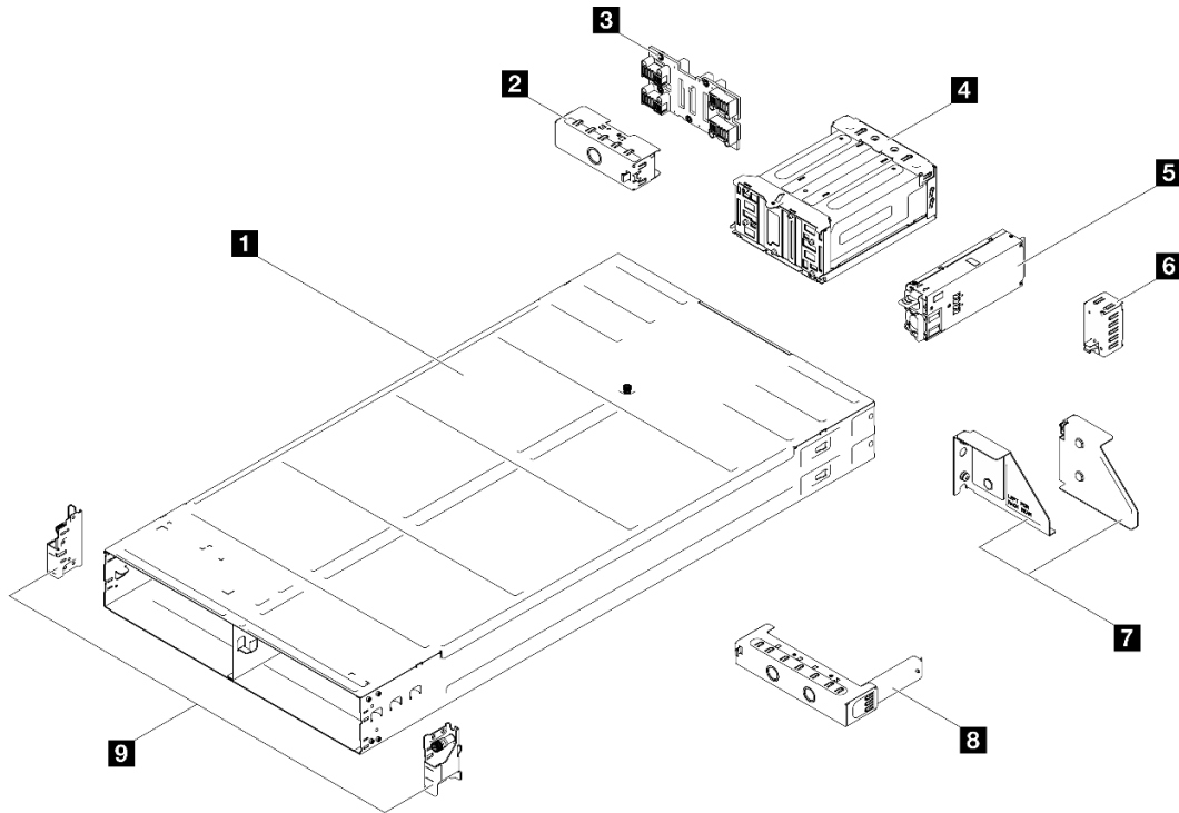
그림 15. 새시 구성 요소
