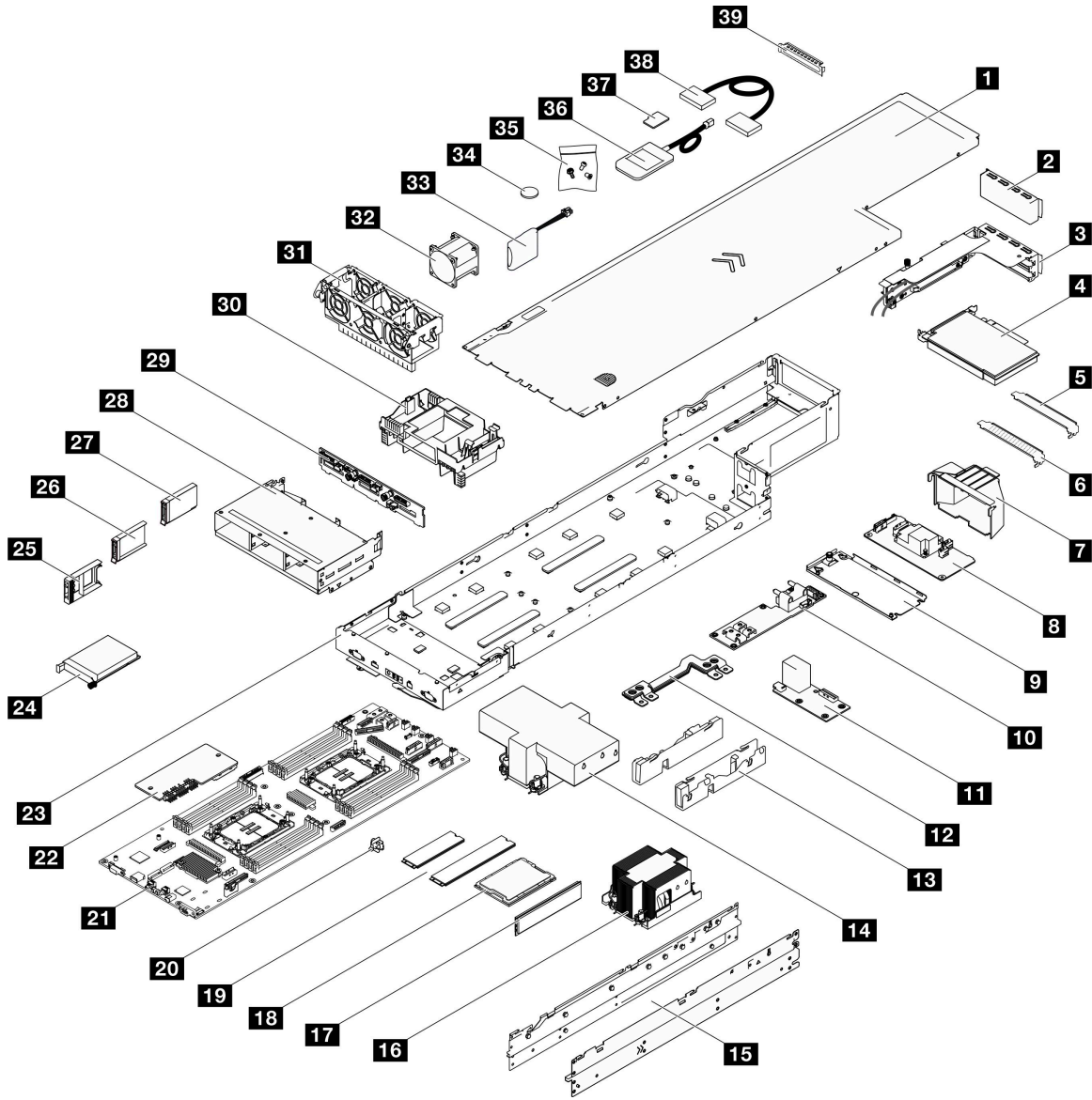
그림 16. 노드 구성 요소
